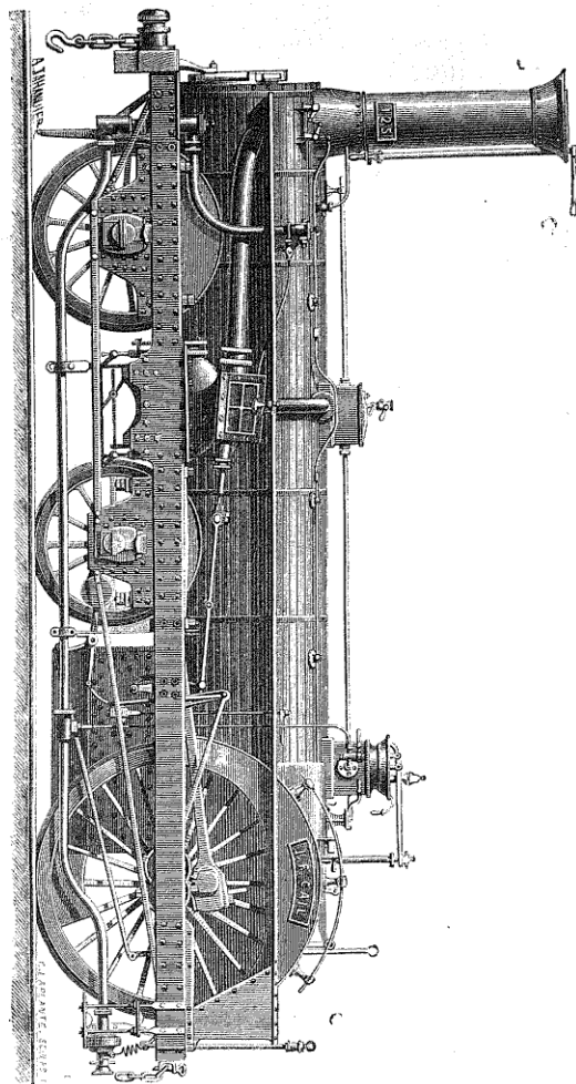
Fig. 82. — Vue extérieure d'une locomotive type Gramphon.
