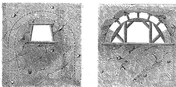
Fig. 25 et 24. — Percement d'un tunnel; galerie provisoire.
