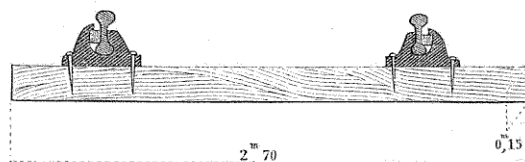
Fig. 57. — Assemblage d'une traverse et des coussinets.
