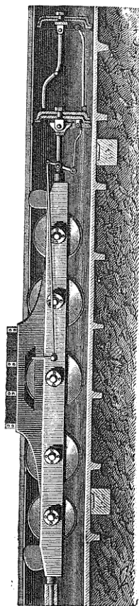
Fig. 417. — Tube pneumatique du chemin de fer atmosphérique de Saint-Germain.
