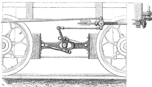
Fig. 101. — Mécanisme d'un frein.
