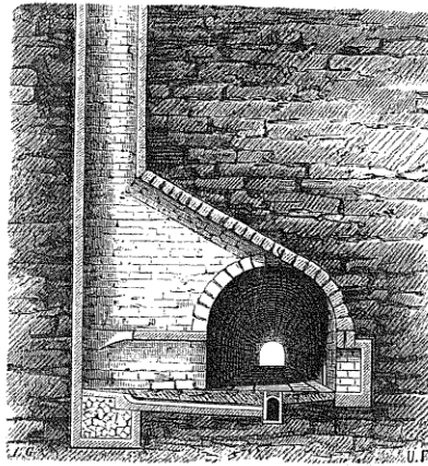
Fig. 50. — Coupe du tunnel dans l'axe d'un puits.
