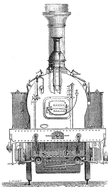
Fig. 85. — Vue d'arrière de la locomotive.
