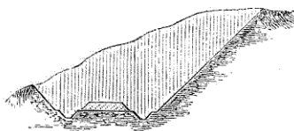
Fig. 15. — Profil en travers du tracé.
