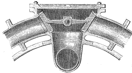
Fig. 80.7.— Régulateur à tiroir ; coupe transversale.
