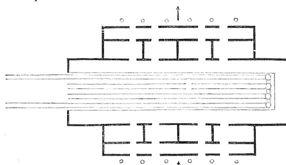
Fig. 105. — Gare tête de ligne; premier système.
