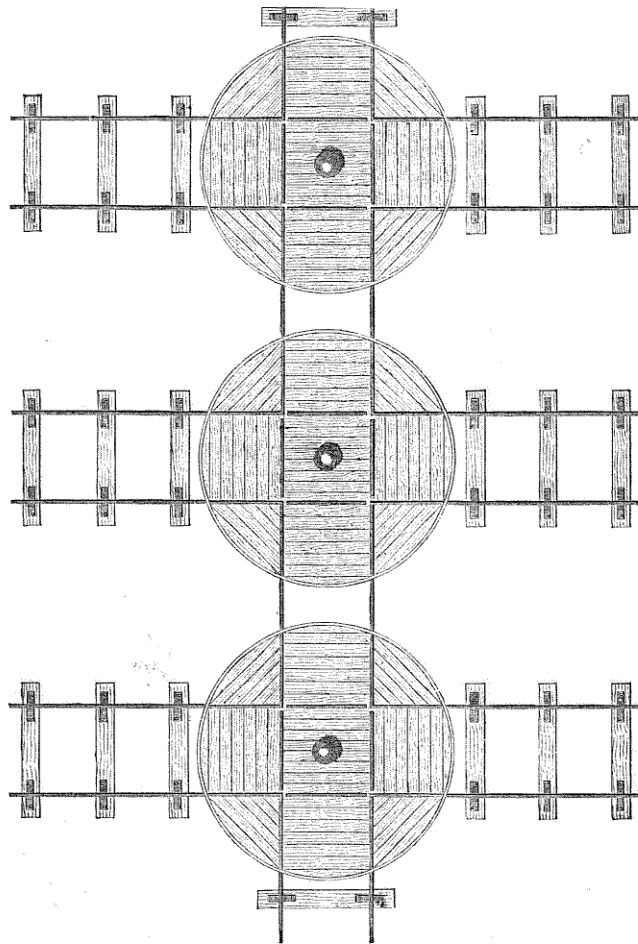
Fig. 72. — Système de plaques rectangulaires pour voies parallèles.
