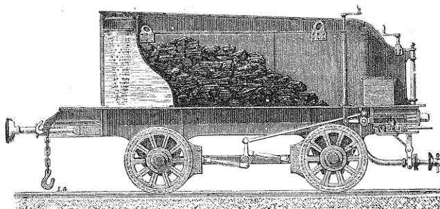
Fig. 86. — Le tender; coupe longitudinale; vue intérieure.
