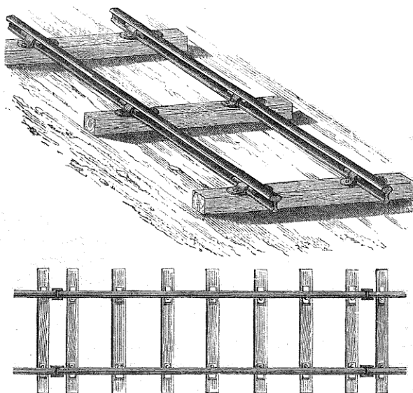
Fig. 59 et 60. — Vue et plan d'une portion de voie.
