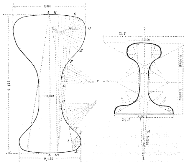
Fig. 53. — Gabarit d'un rail à simple champignon.
