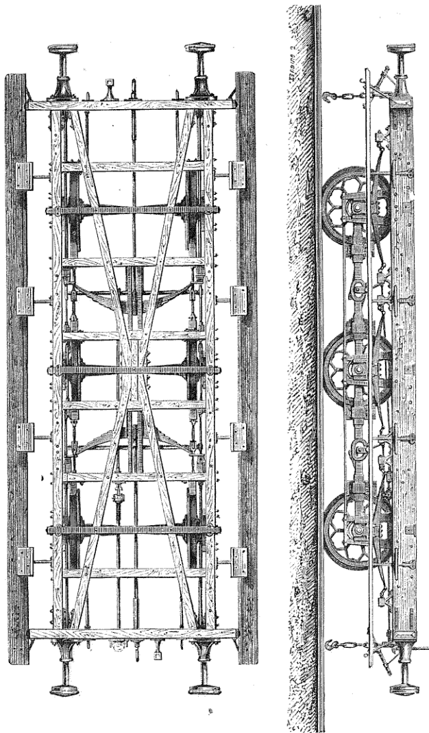
Fig. 55. — Plan et élévation d'un train de voiture de 2 e classe.
