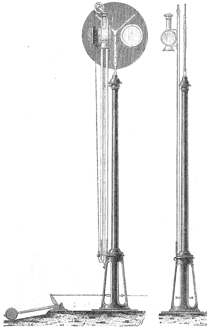
Fig. 128. — Disque signal; vue d'arrière.
