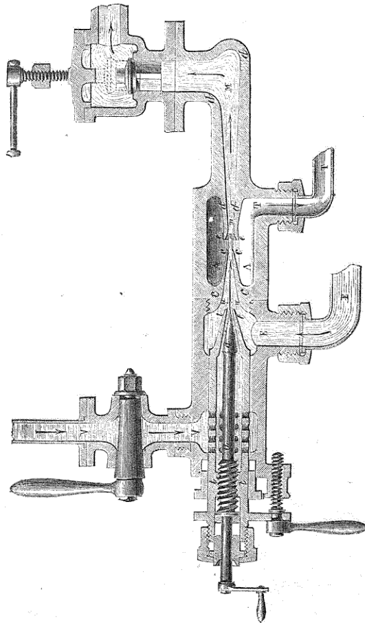
Fig. 85. — Coupe de l'injecteur Giffard.
