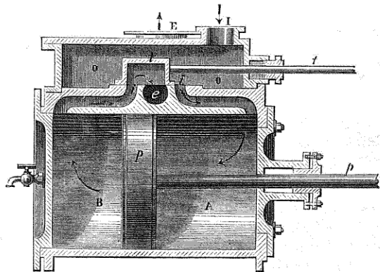
Fig. 76. — Mouvements corrélatifs du piston et du tiroir ; seconde position.
