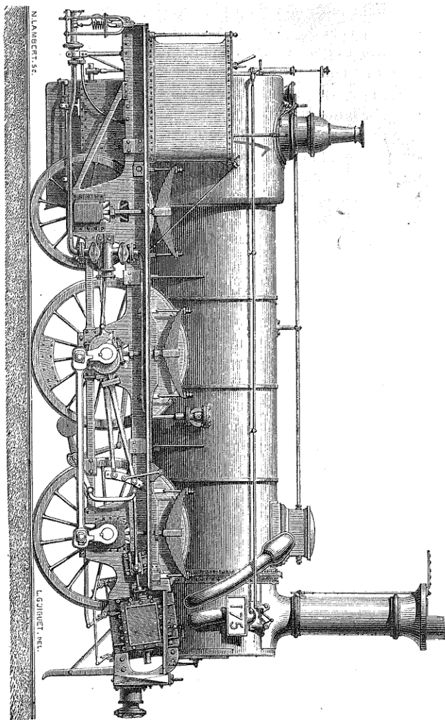
Fig. 81. — Vue extérieure de la locomotive; mécanisme de la distribution; pompes alimentaires, etc.
