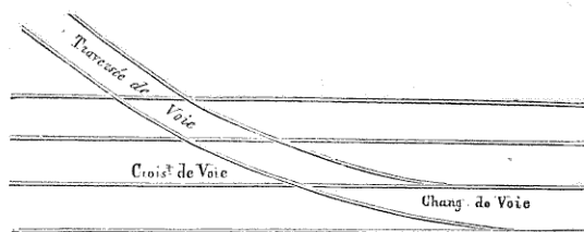
Fig. 65. — Changement, croisement et traversée de voie.
