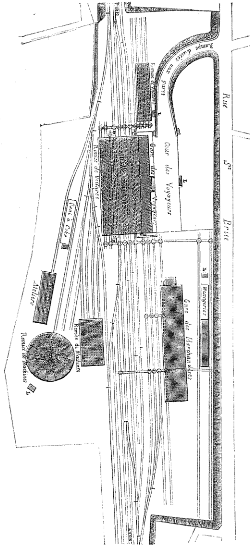
Fig. 110.—Plan de la gare de Mâcon; chemin de fer de Paris à Lyon.
