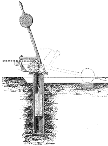
Fig. 150. — Manœuvre du disque signal.
