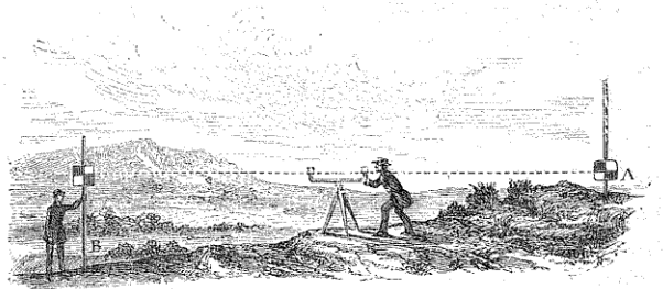
Fig. 8. — Opération du nivellement.
