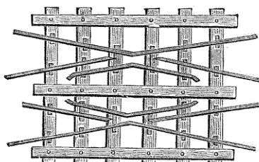
Fig. 65. — Traversée de voie.
