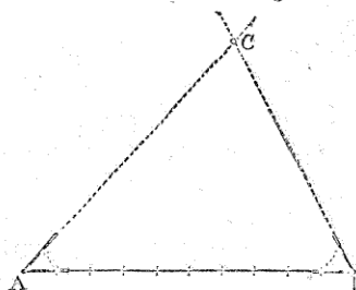
Fig. 4. — Construction d'un triangle.
