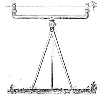
Fig. 6. — Niveau d'eau.
