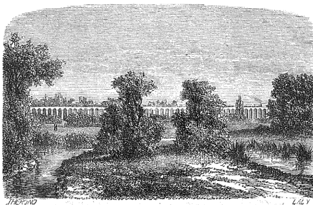
Fig. 40. — Vue générale du viaduc de l'Indre.
