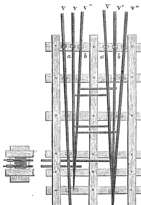
Fig. 67. — Aiguilles pour un changement de voie double.
