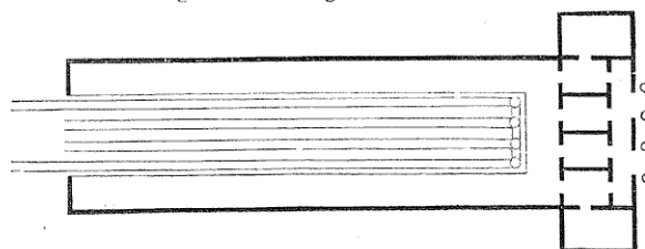
Fig. 104. — Gare tête de ligne; second système.
