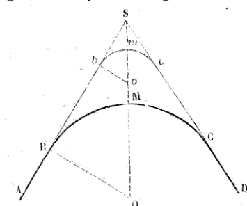
Fig. 17. — Raccordement de deux portions droites du tracé.
