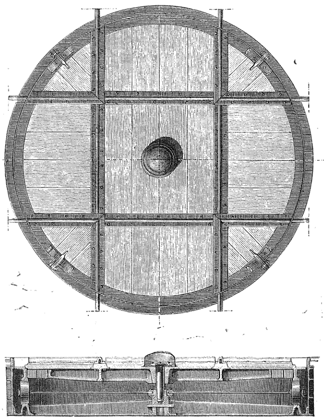
Fig. 69. — Plaque tournante rectangulaire; vue intérieure de la fosse.
