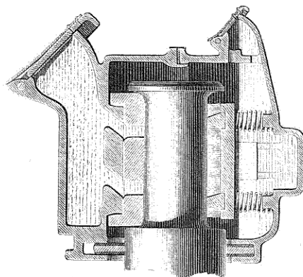
Fig. 94. — Boîte à huile et à graisse; vue intérieure.
