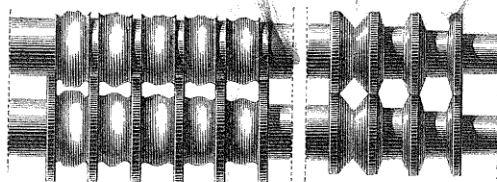
Fig. 53. — Trains lamineurs pour la fabrication des rails.
