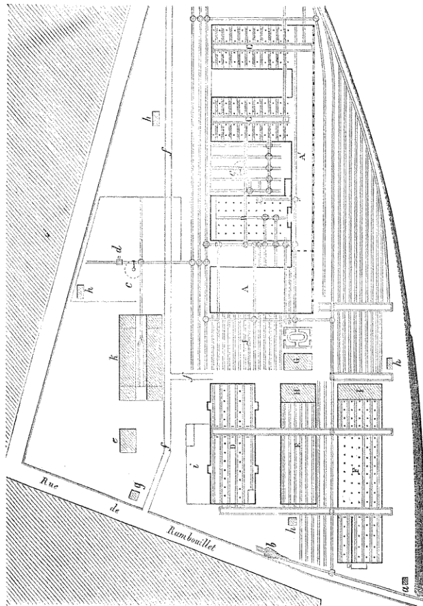
Fig. 108. — Plan des ateliers de la gare de Paris, sur la ligne de Lyon.
