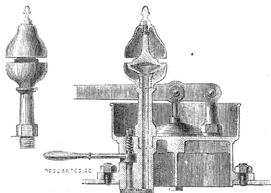
Fig. 84. — Sifflet à vapeur et soupapes de sûreté de la locomotive.
