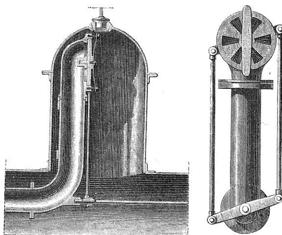
Fig. 78. — Régulateur à papillon; coupe de profil. Fig. 79. — Vue de face.
