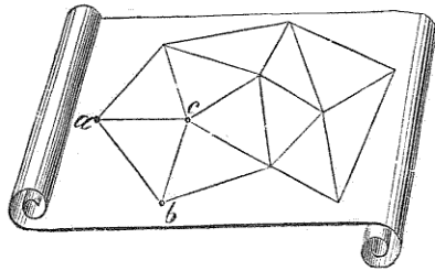
Fig. 5. — Canevas topographique.
