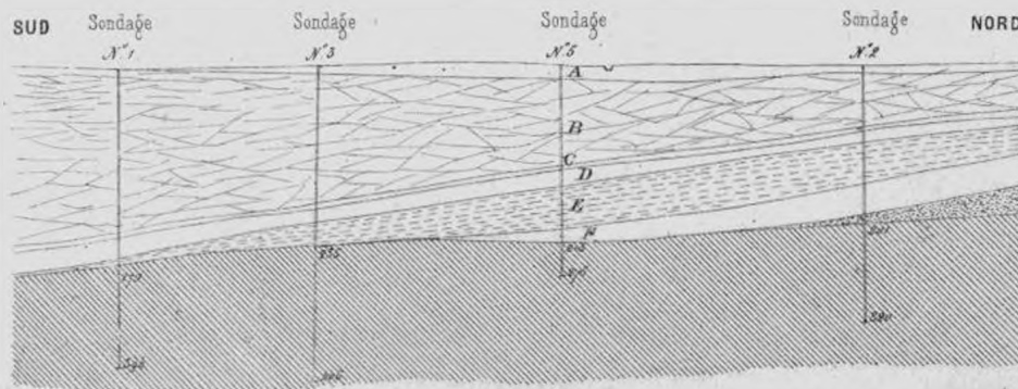
COUPE DES MORTS TERRAINS DU BOIS DU LUC à HAVRE
