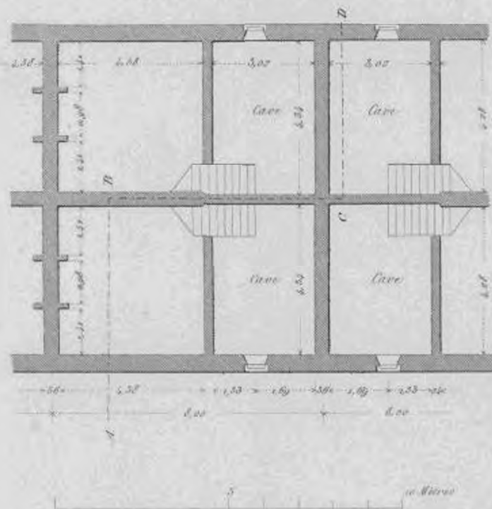
Fondations et caves.
