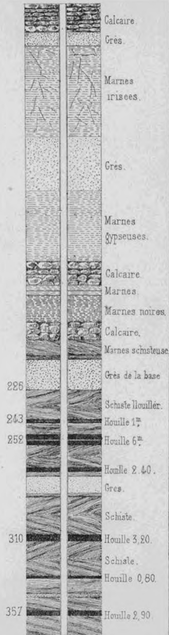
Sondage de Malbosc (Bassin du Gard)
