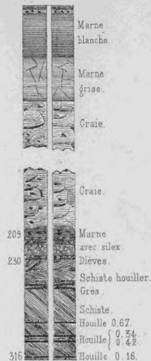
Sondage de Chlin (Mons)
