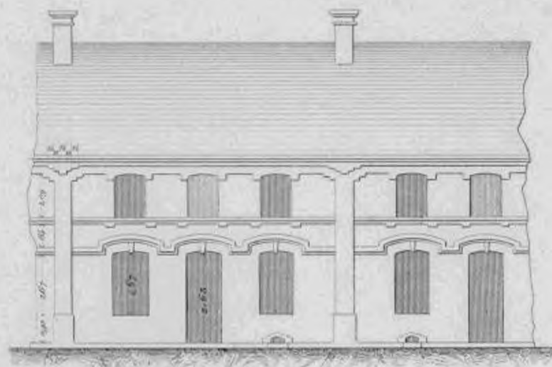
Élévation principale (des deux côtés.)
