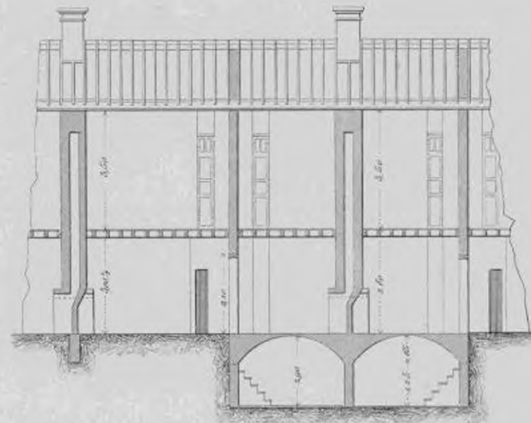
Coupe M.N.
