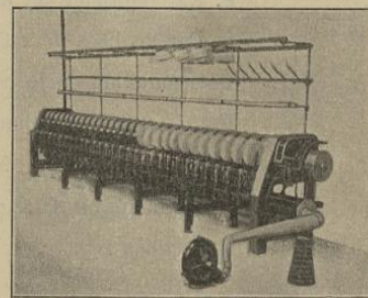
Machine à gazer, Système RYO
