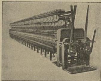
Métier continu à retordre, Système RYO, à broches commandées par engrenages
