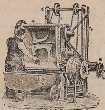
“L'UNIVERSELLE” TYPE VII en position de se décharger.
