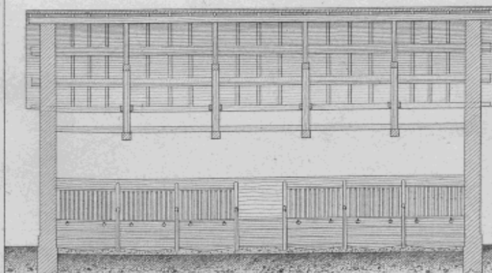
Coupe longitudinale
