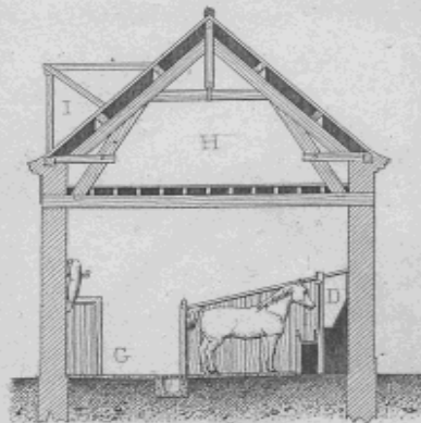
Coupe transversale
