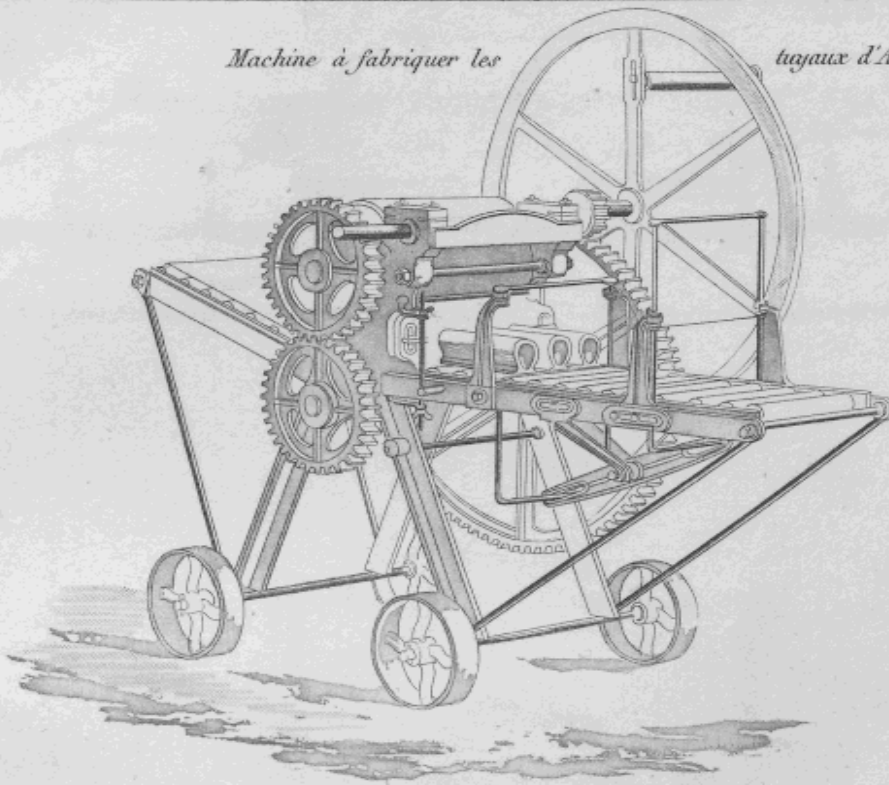
Machine de Clayton
