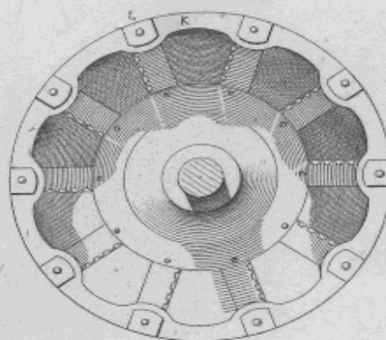
Fig. 4. Coupeur
