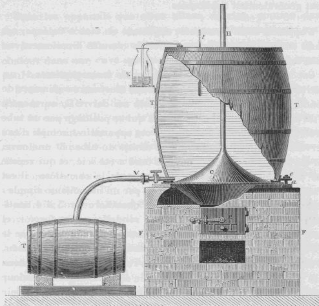
APPAREIL DE M. ROSSIGNOL Chauffant 6 hectolitres à l'heure Fig. 46.
