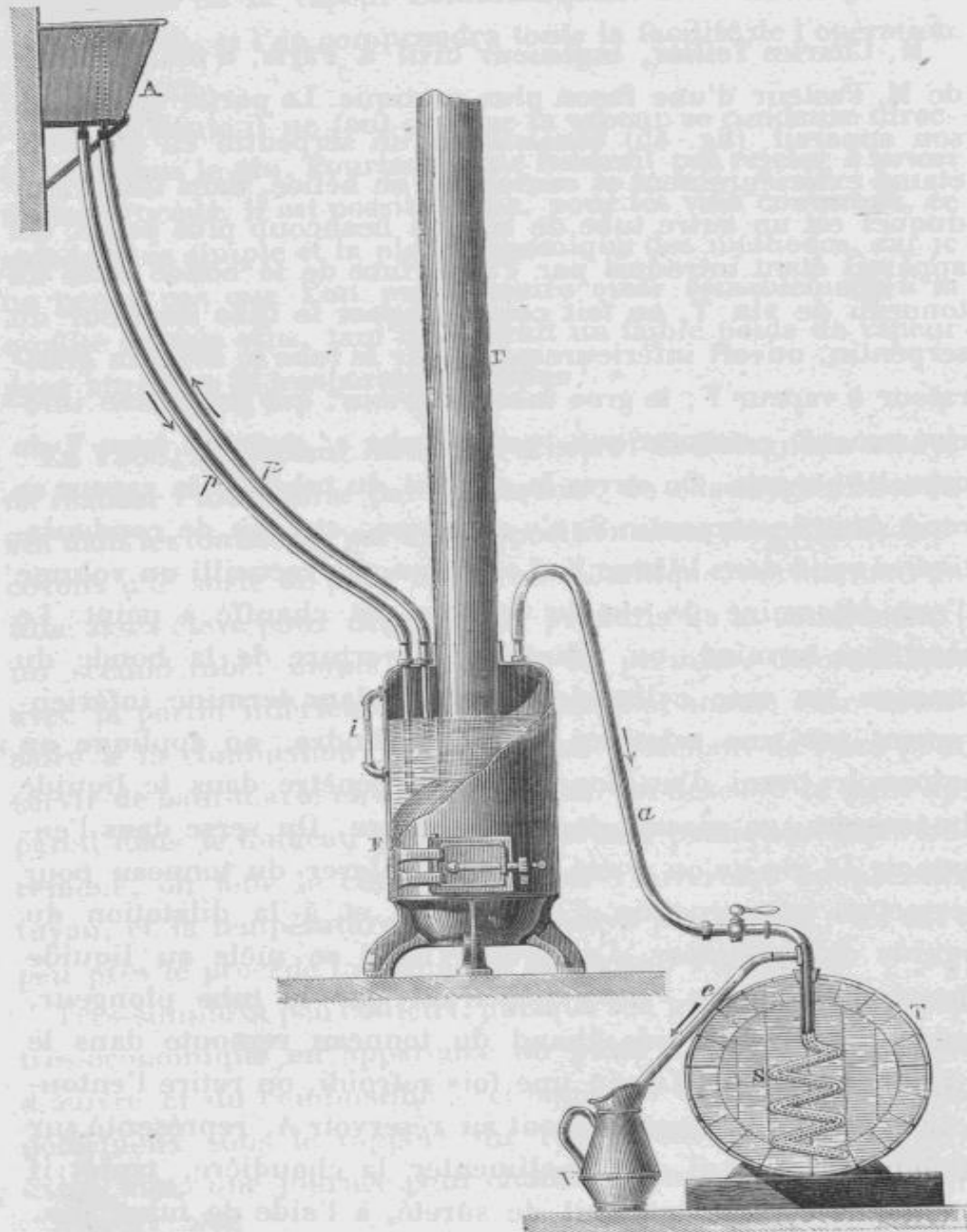
APPAREIL DE M. CH. TELLIER Chauffant 228 litr. à l'heure Fig. 45.
