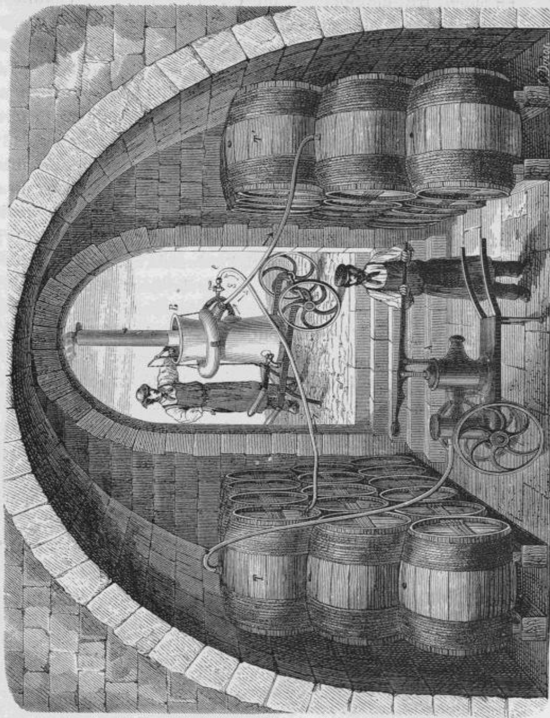
VUE D'ENSEMBLE DE L'APPAREIL TERREIL DES CHÊNES Fig. 54.
