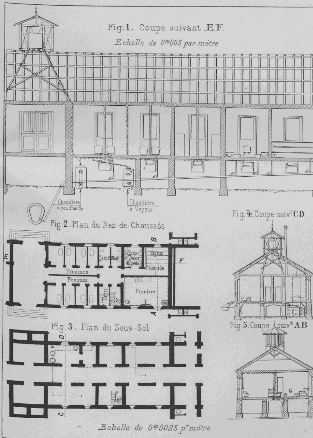
Installation de Bains et de Douches.
