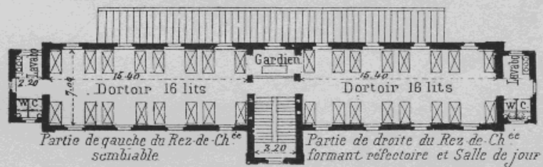
Fig. 3. Pavillon des Epidémies - Plan du Rez-de-Chaussée
