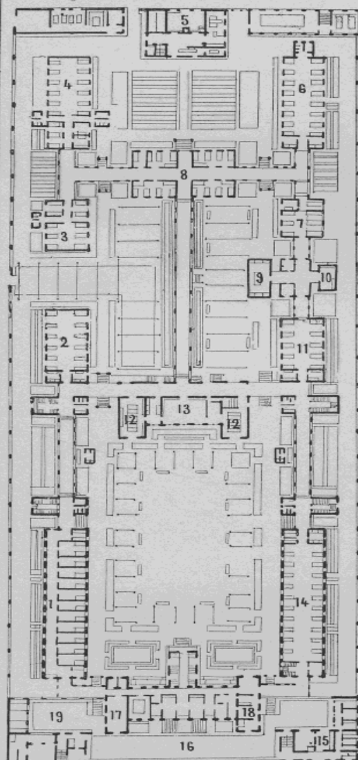
Fig.1. Plan du Rez-de-Chaussée
