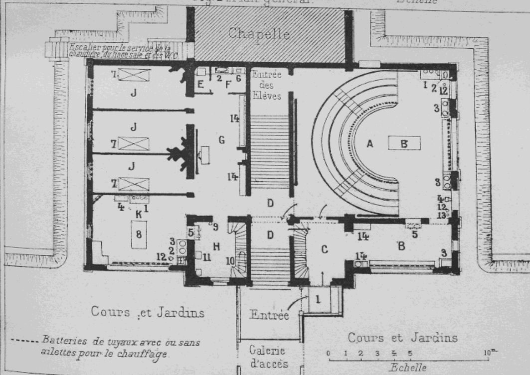
Fig. 2 Plan général.
