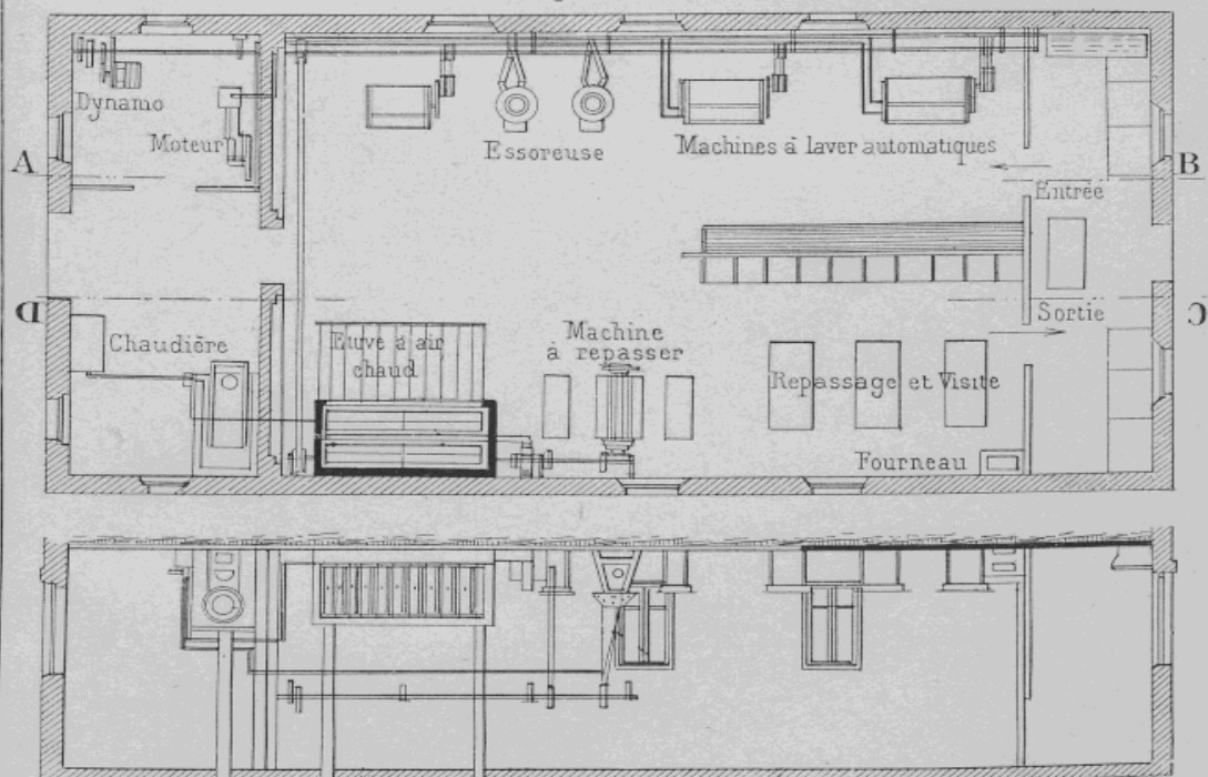
Fig.3. Coupe CD
