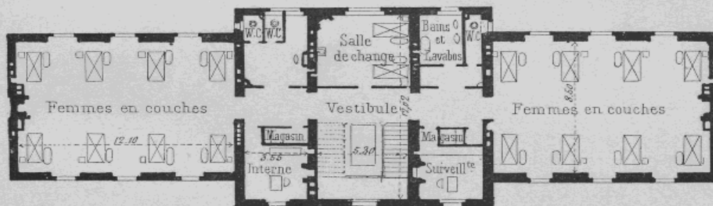
Fig. 2. Plan du 1 er et 2 e Etages.
