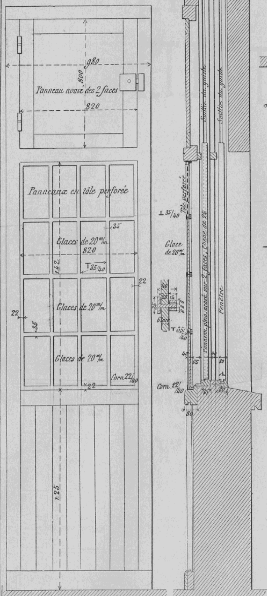
Fig. 6. Détail de la porte
