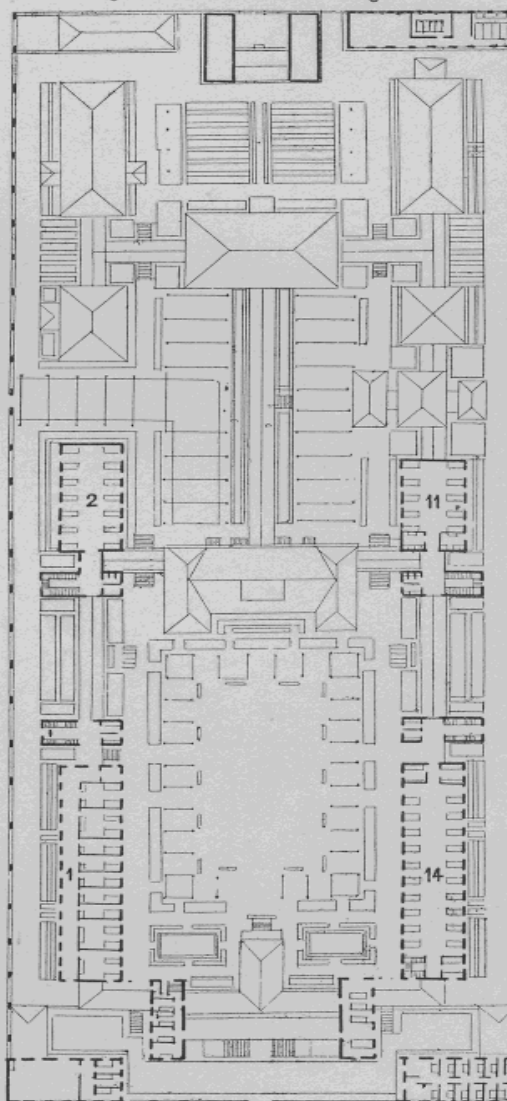
Fig.2. Plan de l'Etage
