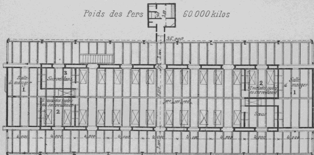
Fig. 3. Plan du 1 er Etage
