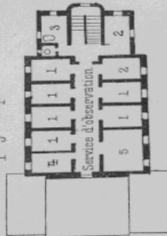
Fig. 3. Plan du 1 er Etage de la polyclinique
