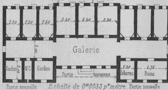
Fig.1. Plan du pavillon.
