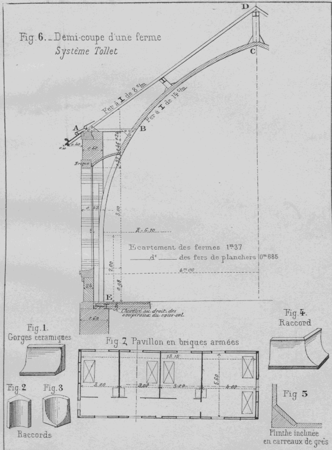
Détails de construction.
