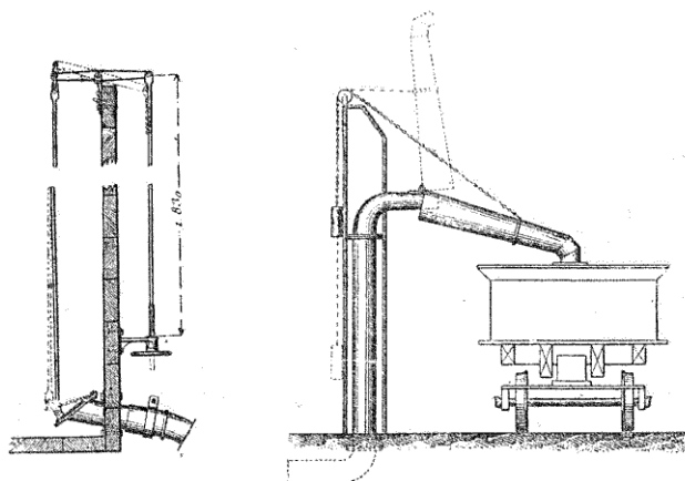
Fig. 306. — Prises d'eau.
