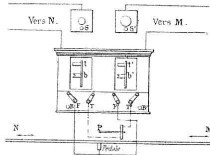
FIG. 261. — Block Flamache et Schubart.
