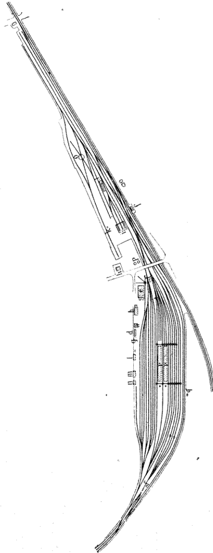
Fig. 31. — Triage par la gravité (dos d'âne). Gare d'Argentueil.
