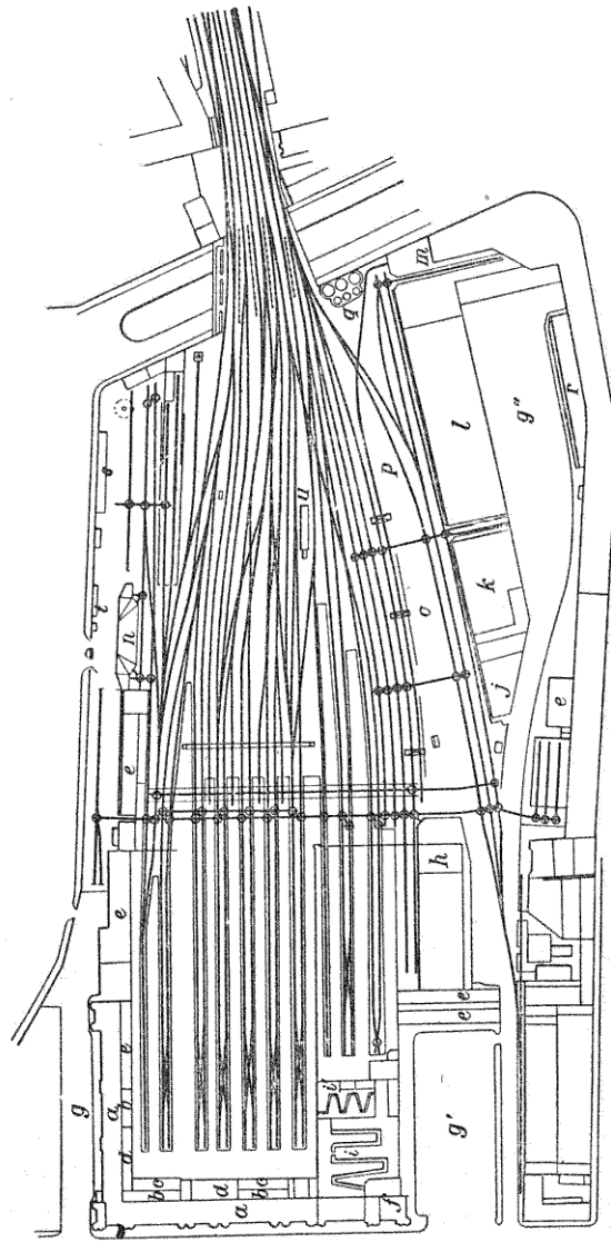
Fig. 13. — Gare du Nord.
