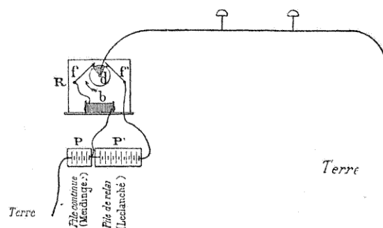
FIG. 267. — Relai.
