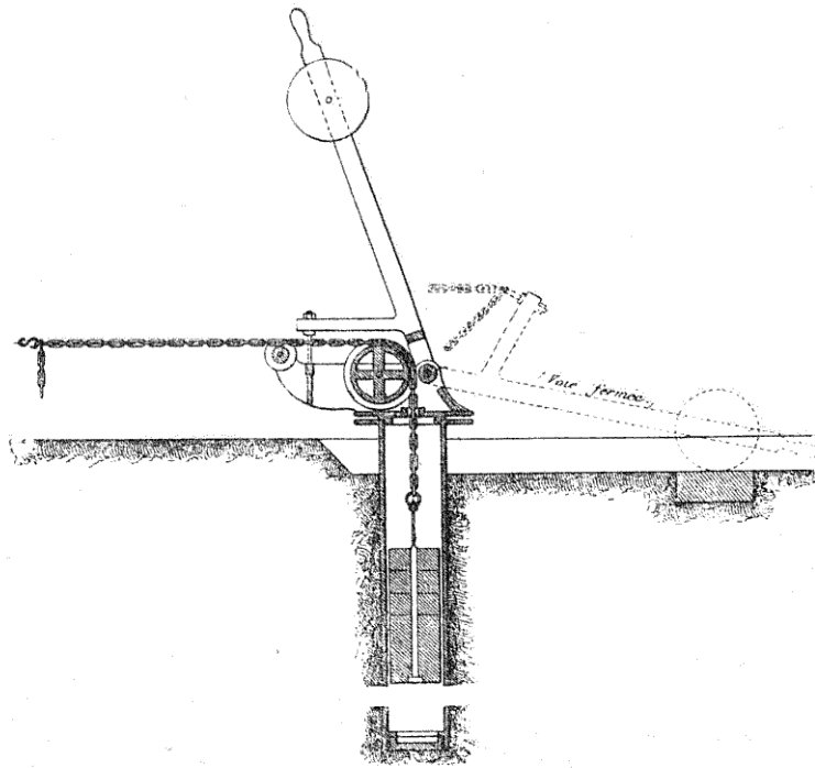
FIG. 66. — Levier de manœuvre du Lyon.
