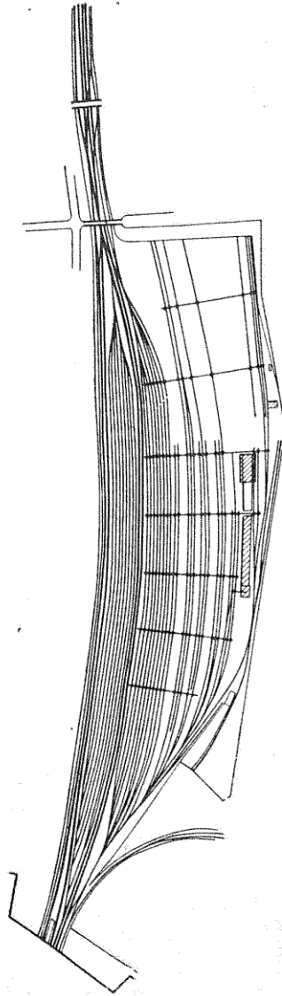
Fig. 27. — Triage par plaques (Conlaus).
