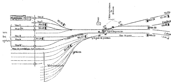
FIG. 6. — Gare de bifurcation à tronç commun.
