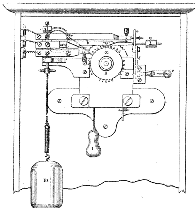
FIG. 270. — Transmetteur intermédiaire.
