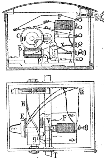
FIG. 241. — Serrure n° 3.
