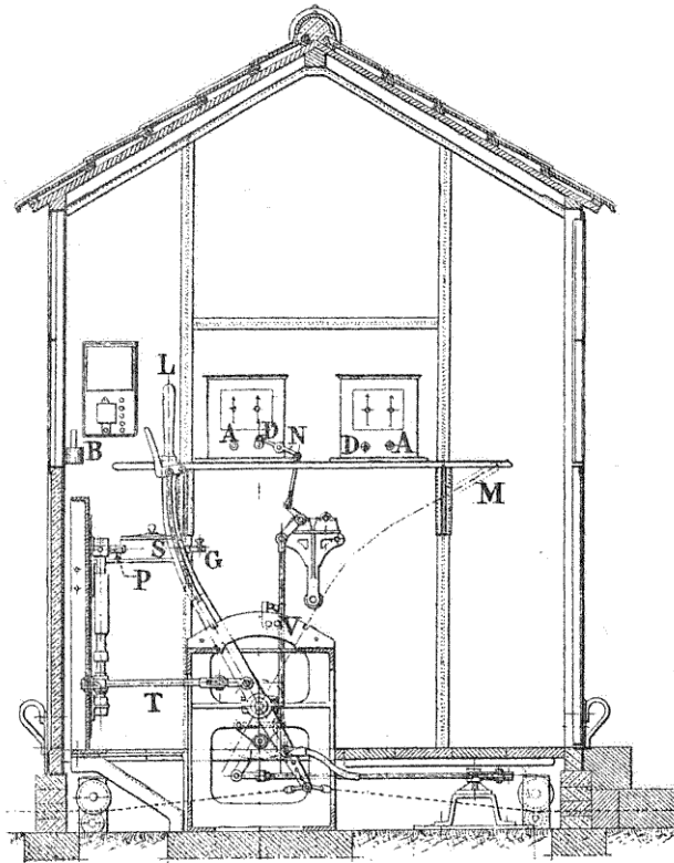
FIG. 232. — Montage des différentes pièces.
