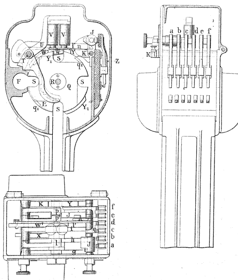
FIG. 258. — Détails des organes d'enclenchement.
