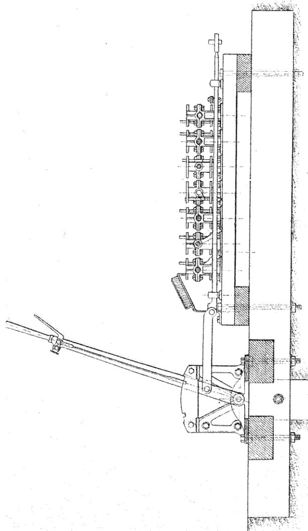
FIG. 148. — Endechement Vignier (Manœuvre d'aiguille).
