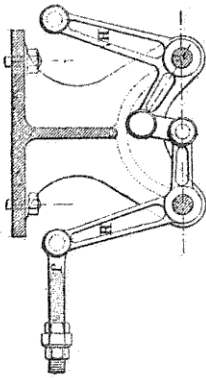
Compensateur vertical
