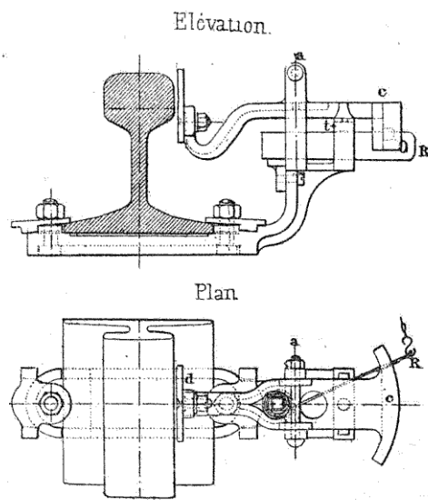
FIG. 282. — Pédale.
