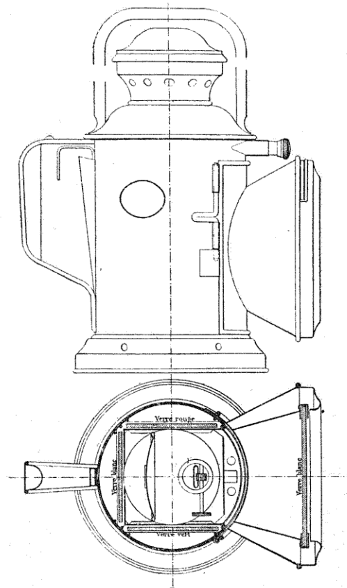
FIG. 56. — Lanterne à un seul feu variable.
