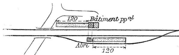
FIG. 2. — Gare à quais croisés.
