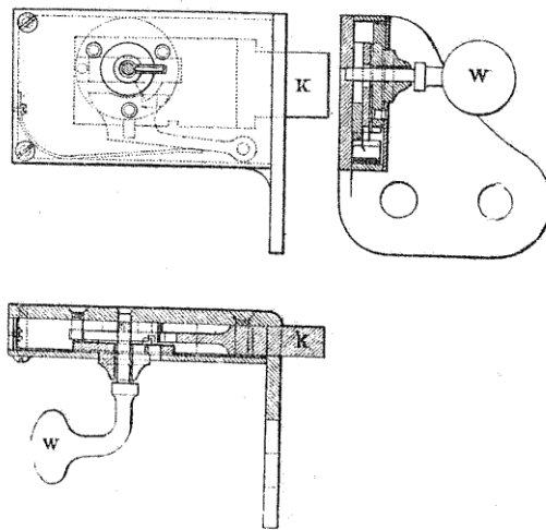
FIG. 234. — Verron d'arrêt.
