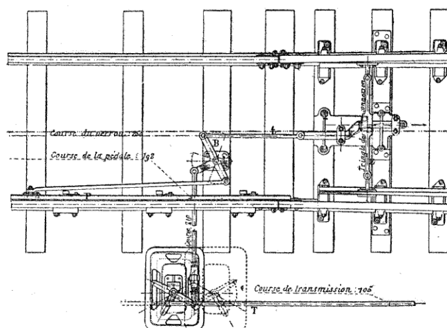
FIG. 114. — Verrou-aiguille Poulet.
