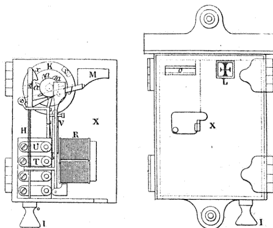
FIG. 243. — Appareil Memento.
