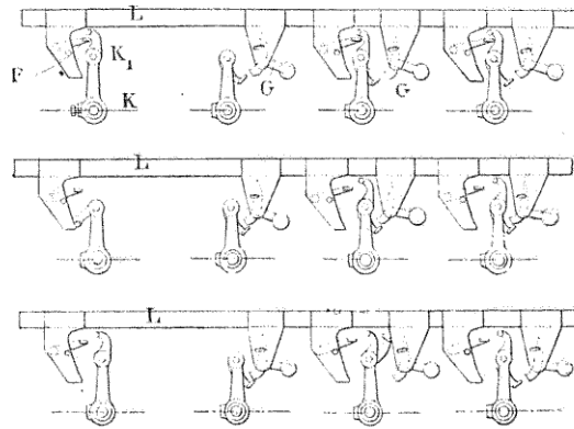
FIG. 189. — Règles d'enclenchement.
