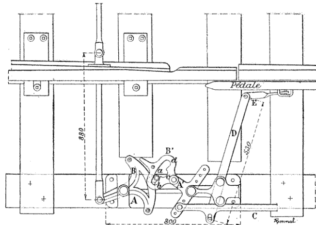
Fig. 112. — Verrou-aiguille Marcelet.
