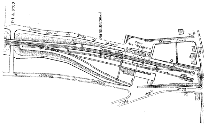
Fig. 9. — Gare terminus.
