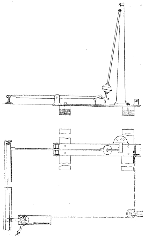
FIG. 278. — Dromopétard Le Boulengé.
