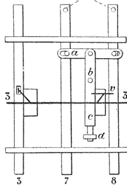
FIG. 151. — Enclenchements ternaires.
