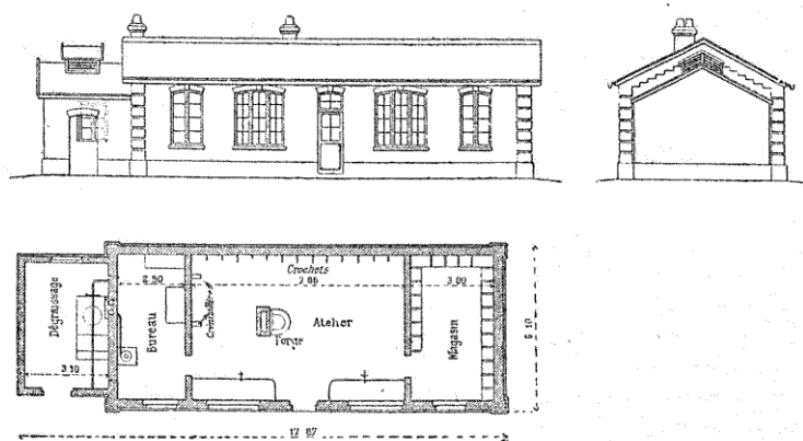
FIG. 299. — Poste de visiteurs.
