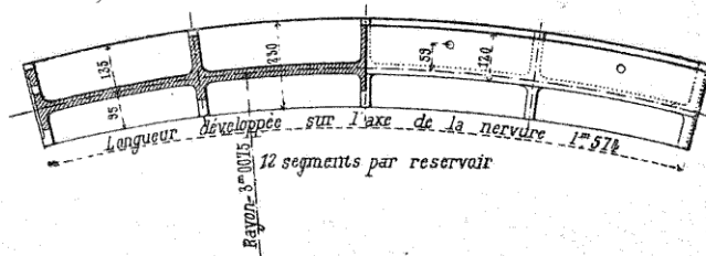
FIG. 305. — Réservoir de 100 à 150 mètres cubes.
