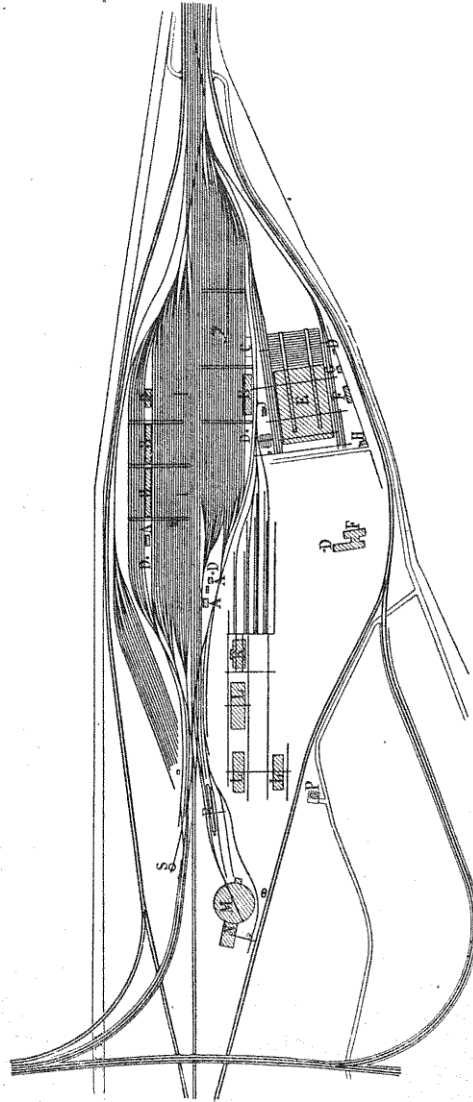
Fig. 38. — Triage par chariots à vapeur (Gare de Villeneuve-Saint-Georges).
