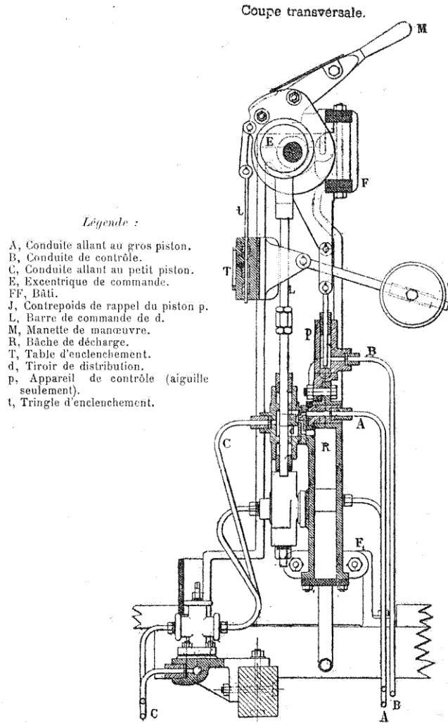
FIG. 130. — Appareil de commande.
