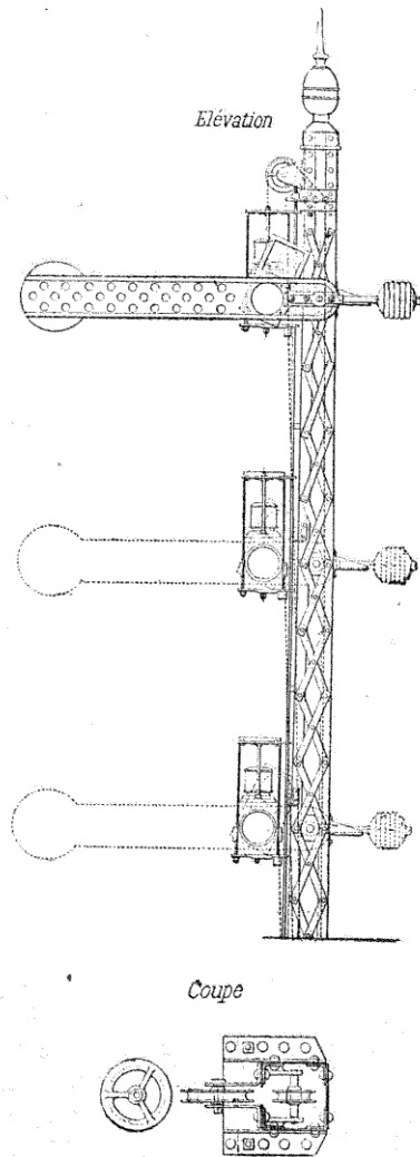
FIG. 79. — Sémaphore à trois ailes.
