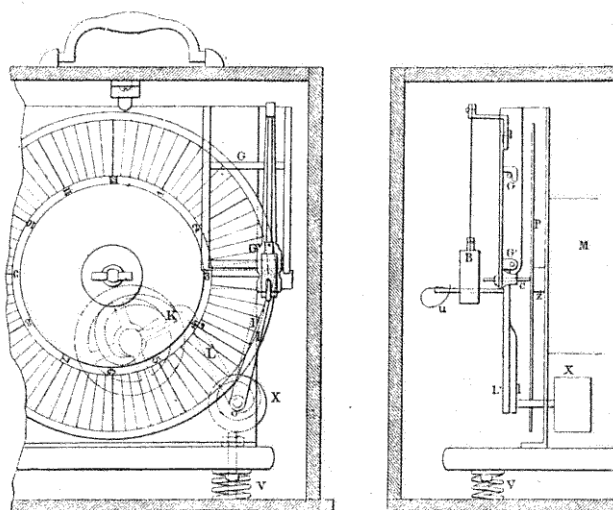
FIG. 273. — Contrôleur Brunot.
