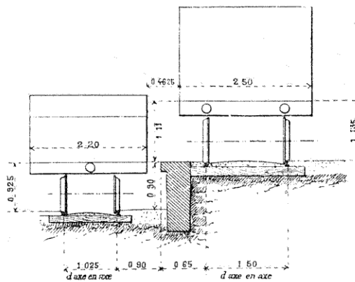
FIG. 41. — Transbordement en fosse.
