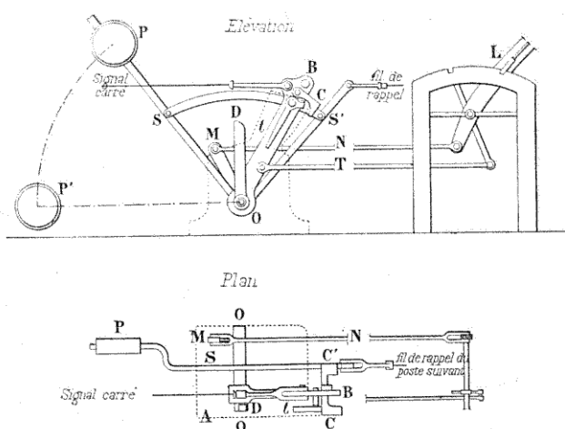
Fig. 235. — Cantonnement mécanique de l'Ouest.
