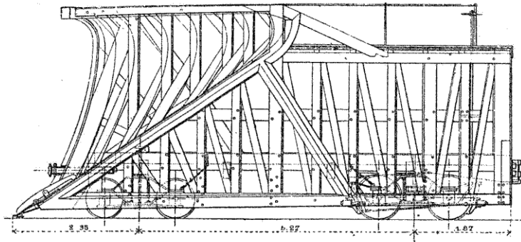
FIG. 303. — Chasse-neige sur véhicule.
