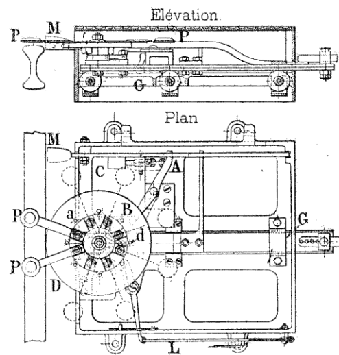
Fig. 71. — Porte-pétards Lirand.
