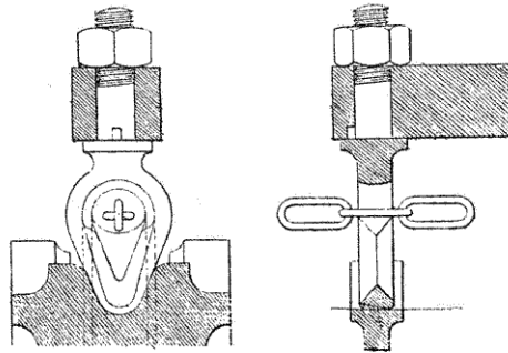
FIG. 67. — Détails de l'agrafe.
