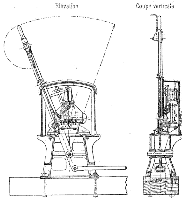
FIG. 201. — Enclenchements de l'État français.
