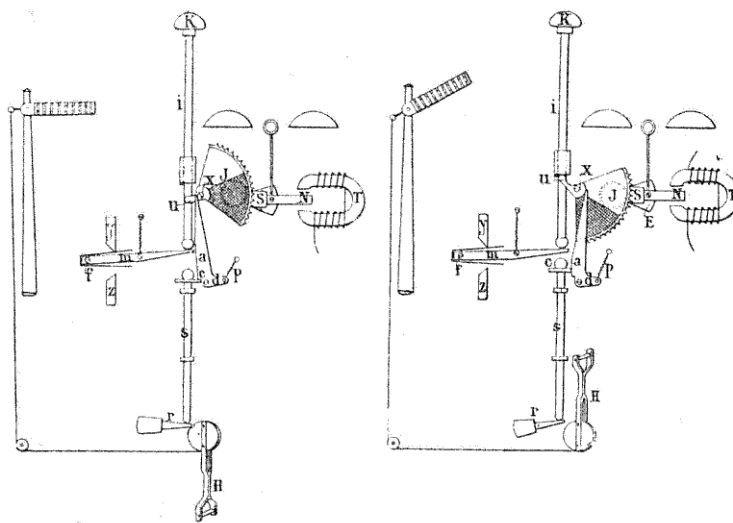
FIG. 236. — Block Siemens.
