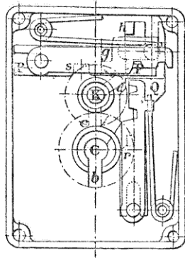
FIG. 211. — Vue intérieure.
