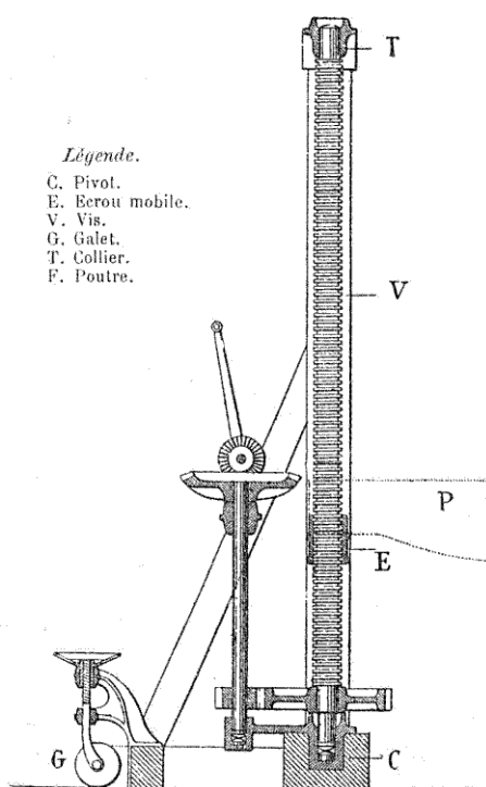
FIG. 295. — Vérin spécial pour le levage des locomotives.
