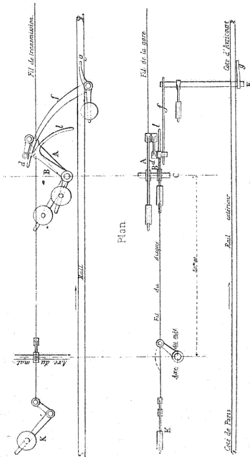
FIG. 87. — Système Guillaume.
