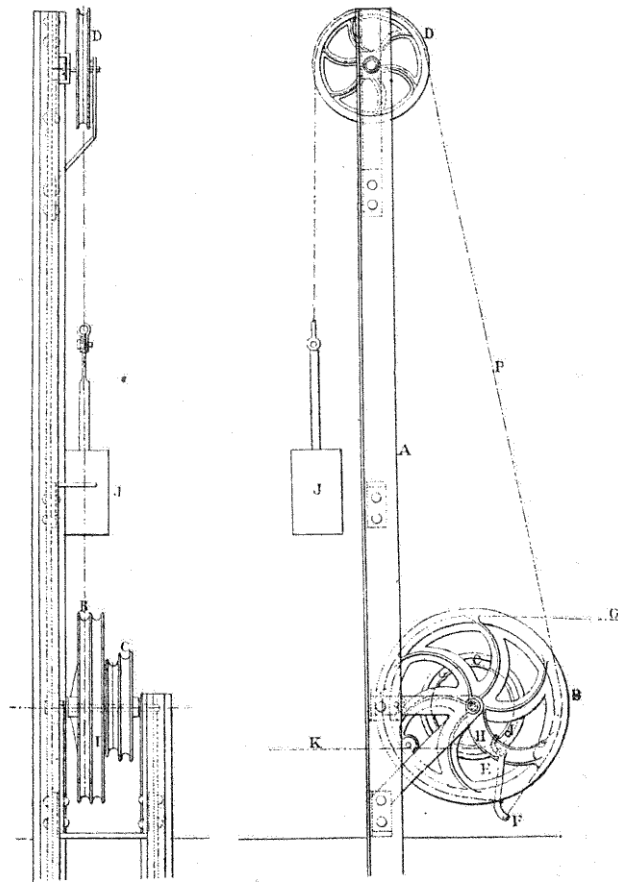
FIG. 96. — Compensateur Dujour.
