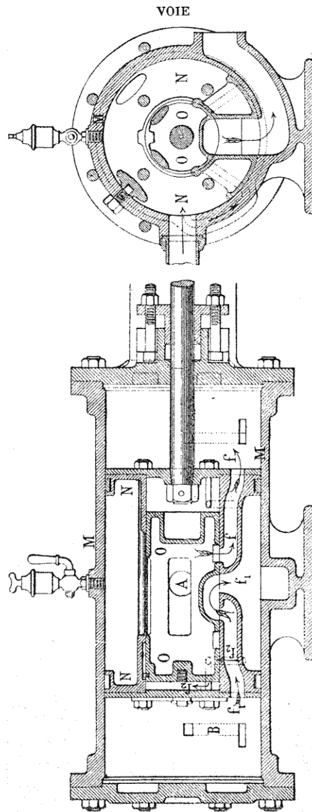
Fig. 307. — Pompe à basse pression.
