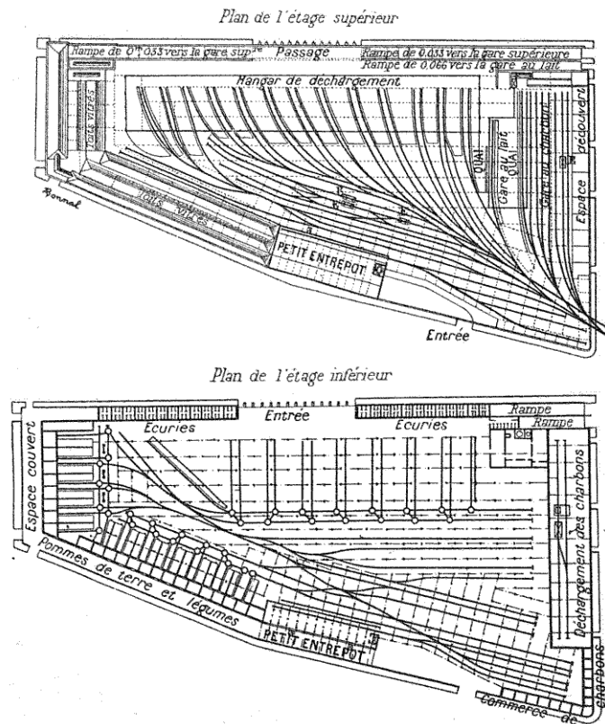
FIG. 36. — Gare de Simer-Town.
