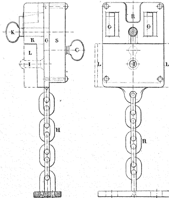
FIG. 210. — Serrure agencée.
