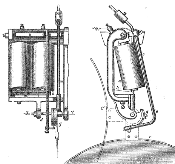
FIG. 249. — Manœuvre du signal de Hall.
