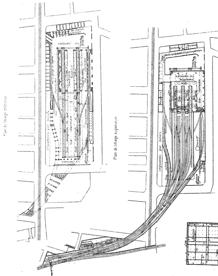
Fig. 37. — Gare de Manchester.
