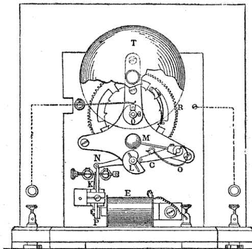
Fig. 253. — Récepteur Jouselin.
