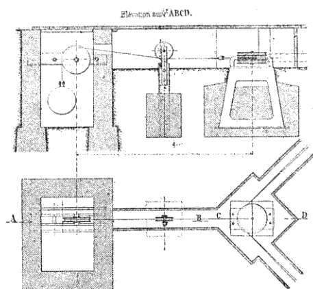
FIG. 119. — Contrepoids compensateur.
