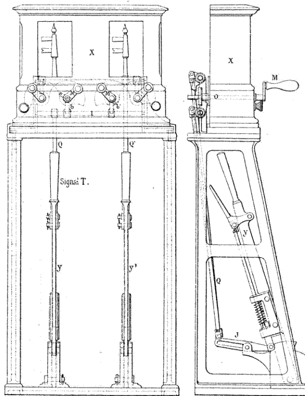
FIG. 262. — Enclenchement mécanique.
