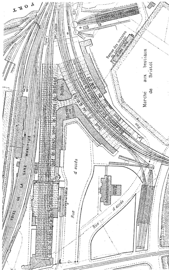
Fig. 106. — Gare de Bristol.
