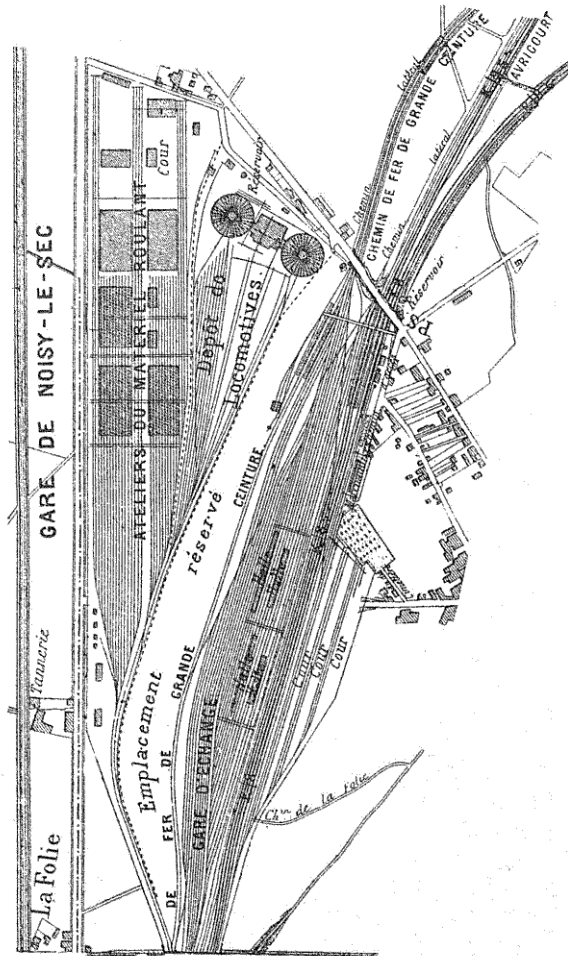
Fig. 38. — Gare d'échange (Noisy-le-Sec).
