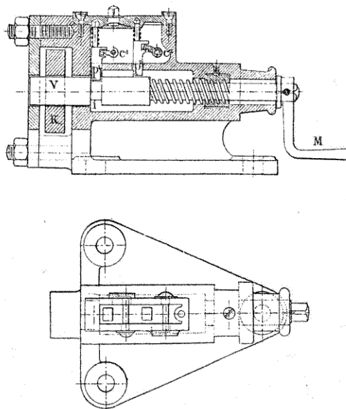
FIG. 207. — Serrure Klaus.
