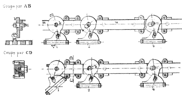
FIG. 165. — Solution générale des enclenchements (Dujour).
