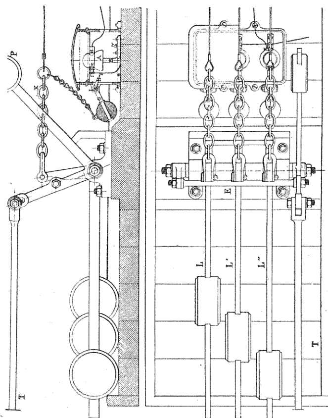
FIG. 63. — Signal commandé de plusieurs points (Ouest).
