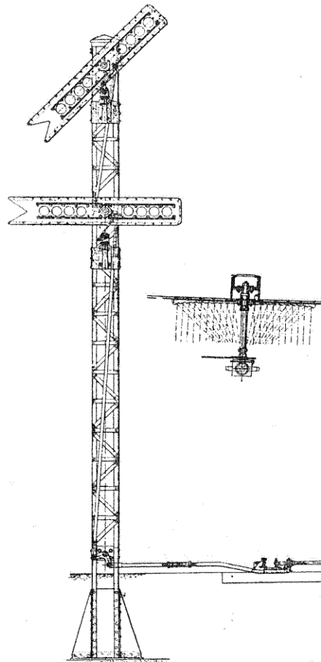
FIG. 83. — Indicateur de direction de l'Est.
