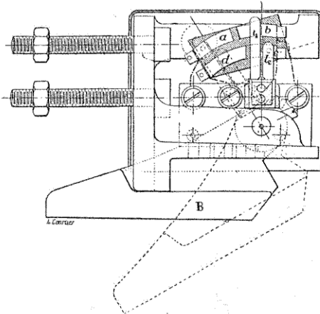
FIG. 242. — Commutateur.
