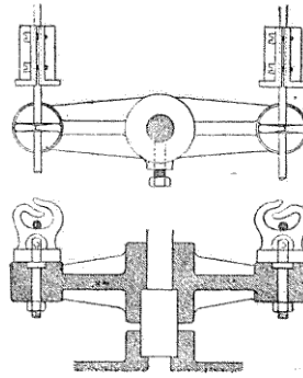
FIG. 142. — Manœuvre d'un mât de rappel.
