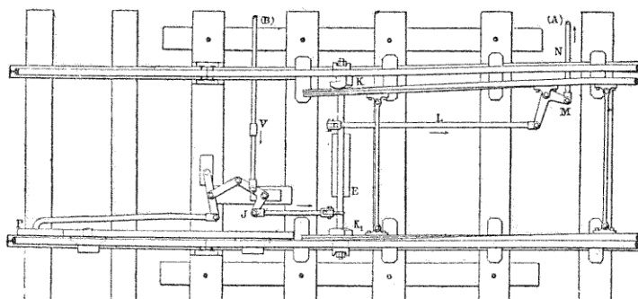
FIG. 116. — Calage Servetaz.
