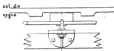
Aiguille verrouillée.
