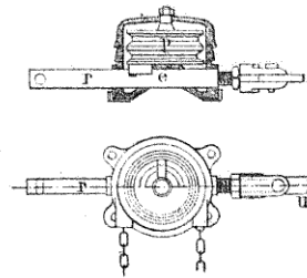
FIG. 171. Enclenchement d'une aiguille par le signal.
