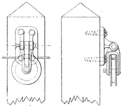
Fig. 93. — Poulie universelle.
