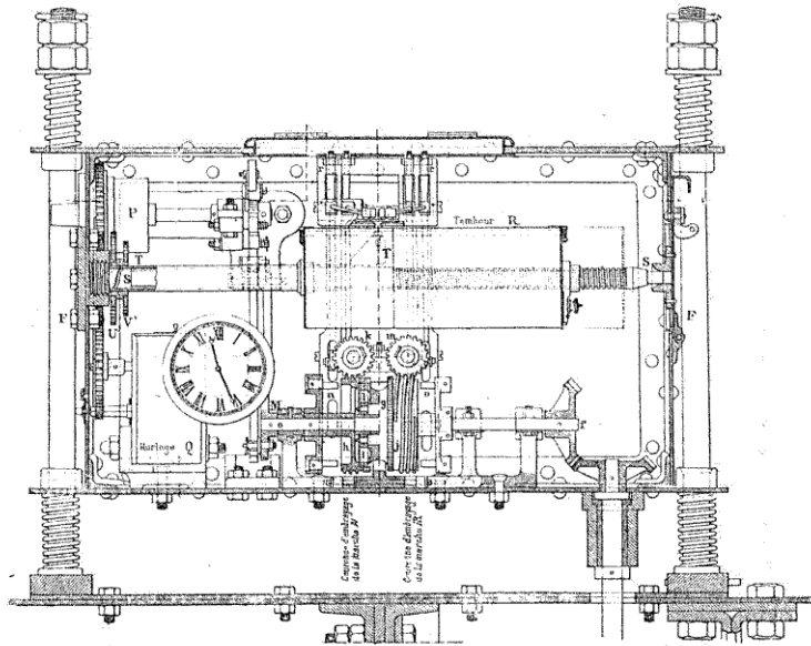
FIG. 275. — Chronotachymètre du P.-L.-M.
