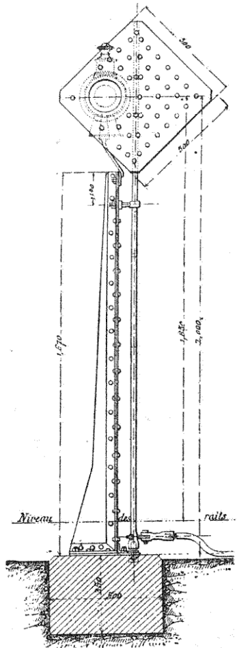
FIG. 86. — Indicateur de position d'aiguille (Midi).
