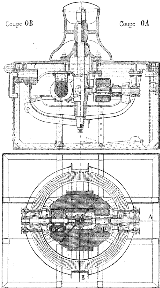
FIG. 54. — Cabestan électrique.
