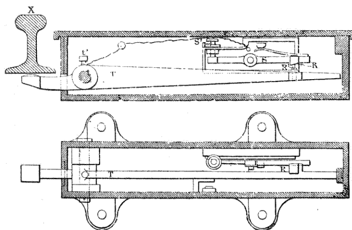
FIG. 245. — Pédales de Hodgson.
