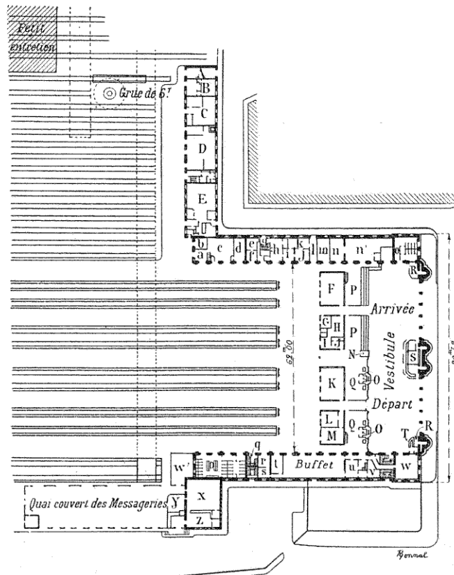
FIG. 46. — Gare Terminus (Tours).
