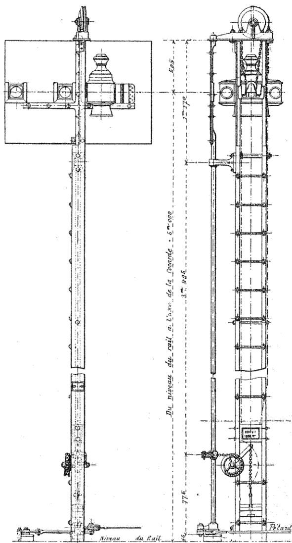
FIG. 77. — Signal carré de l'Ouest.
