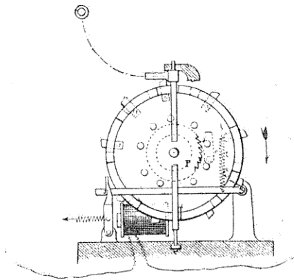
FIG. 265. — Détails du mécanisme.
