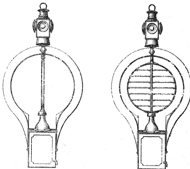
FIG. 247. — Signal de block automatique.
