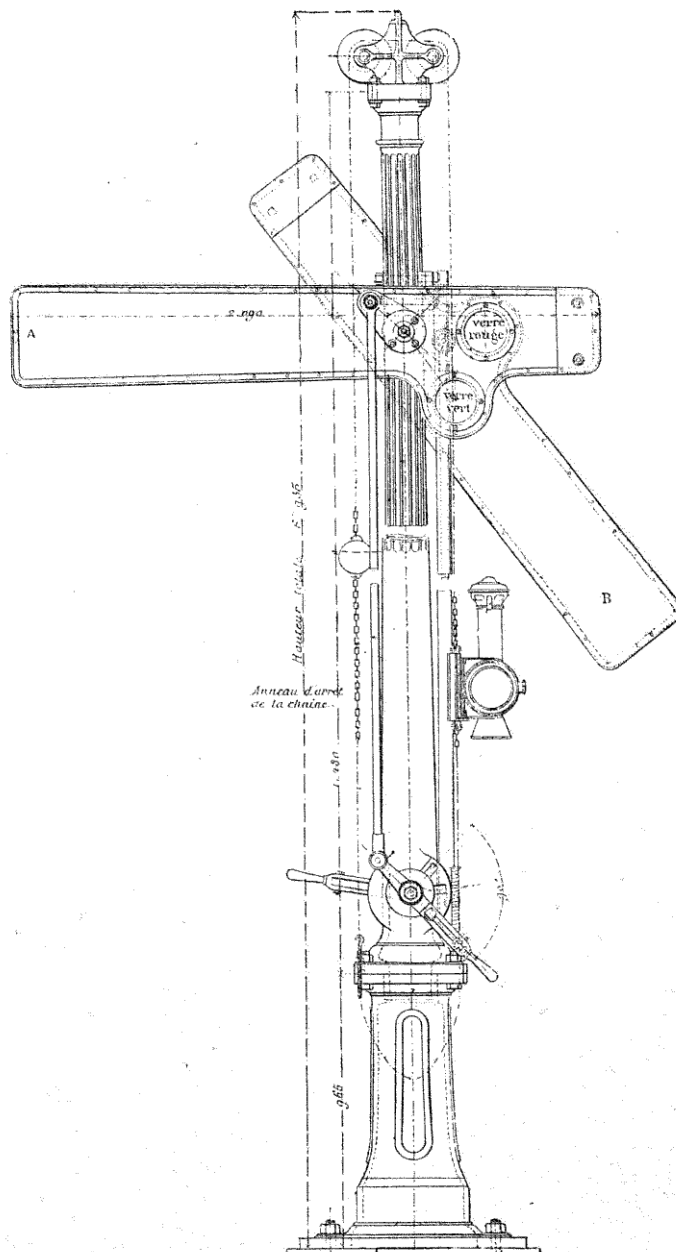
Fig. 81. — Sémaphore de block du Lyon.
