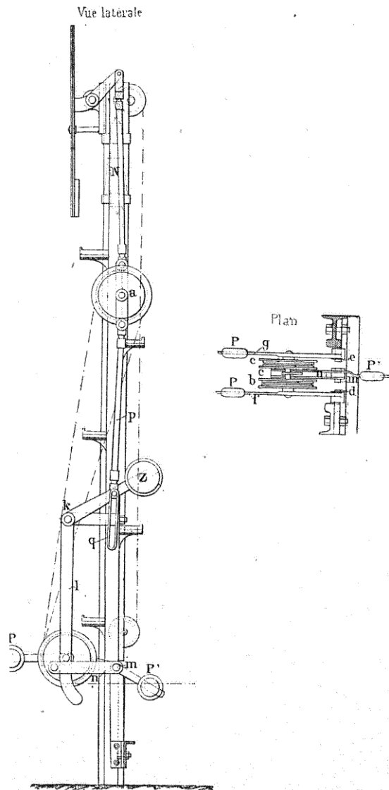
FIG. 76. — Système Gast.
