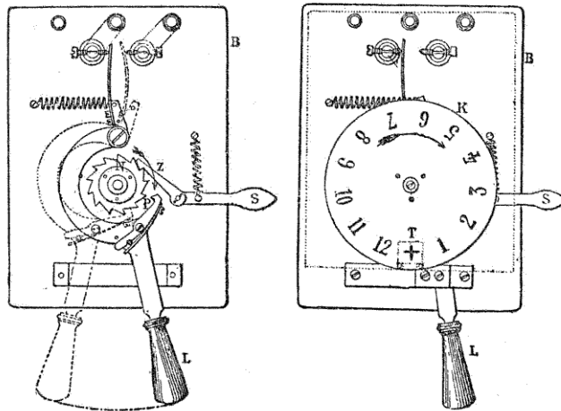
Fig. 252. — Transmetteur Jouselin.
