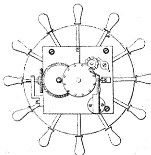
FIG. 251. — Avertisseur Walker.
