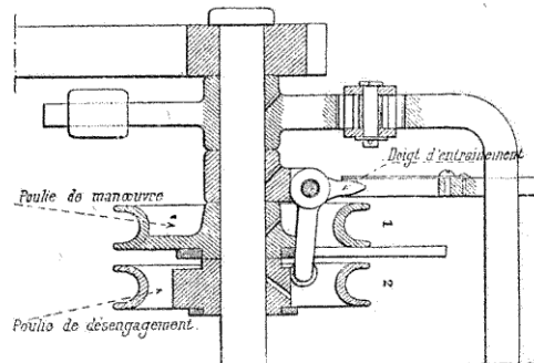
Fig. 179. — Désengageur circulaire.
