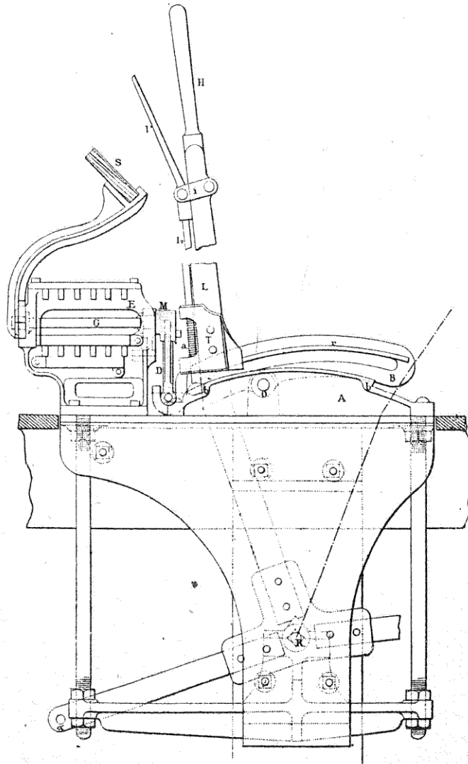
FIG. 155. — Enclenchement Saxby (type anglais).
