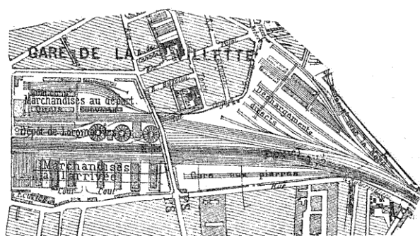
FIG. 48. — Halles perpendiculaires.
