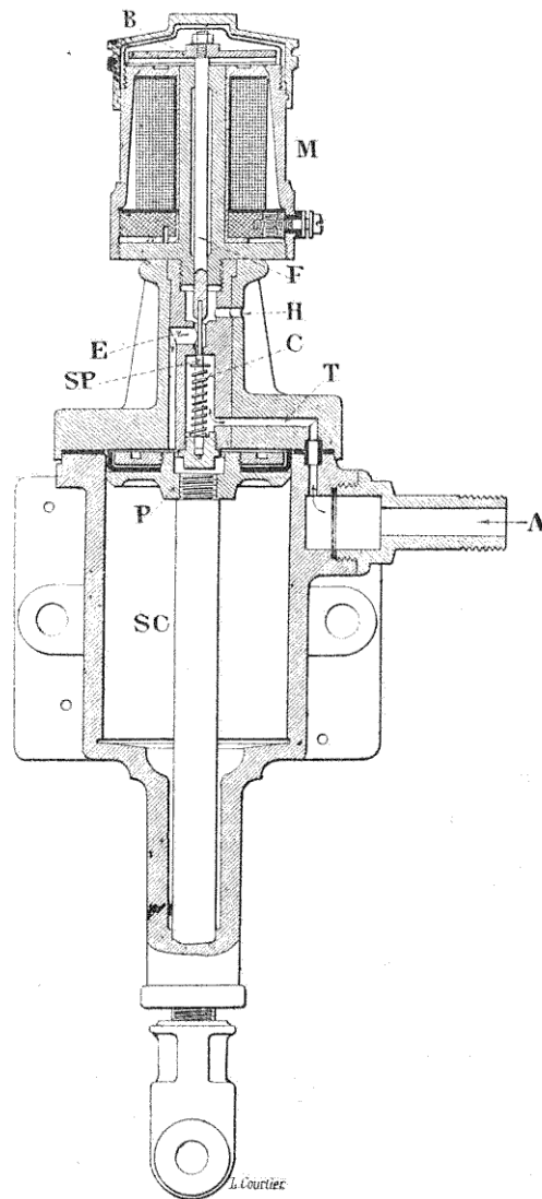
FIG. 132. — Manœuvre électro-pneumatique d'un signal.
