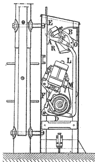
FIG. 135. — Manœuvre électrique des signaux.
