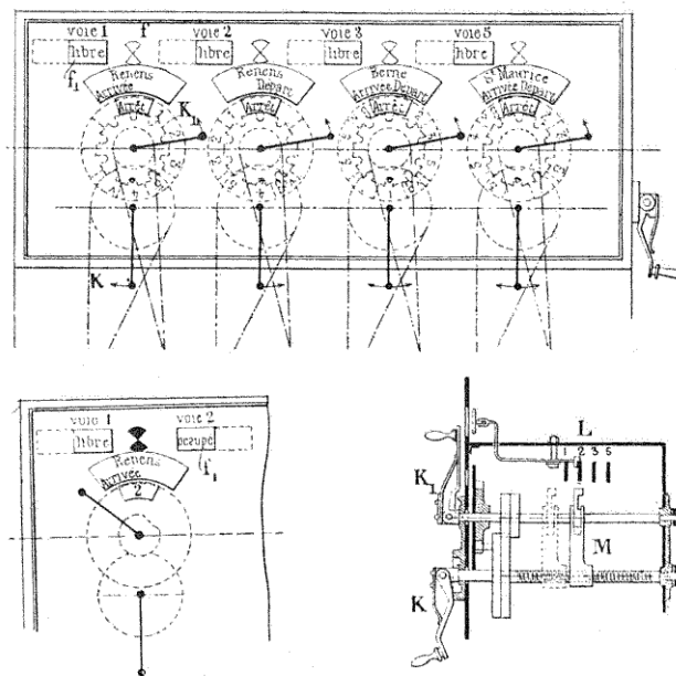
FIG. 188. — Bloc central.
