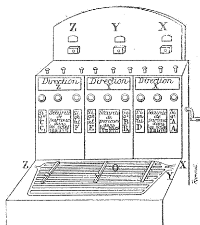
FIG. 195. — Bloc central.
