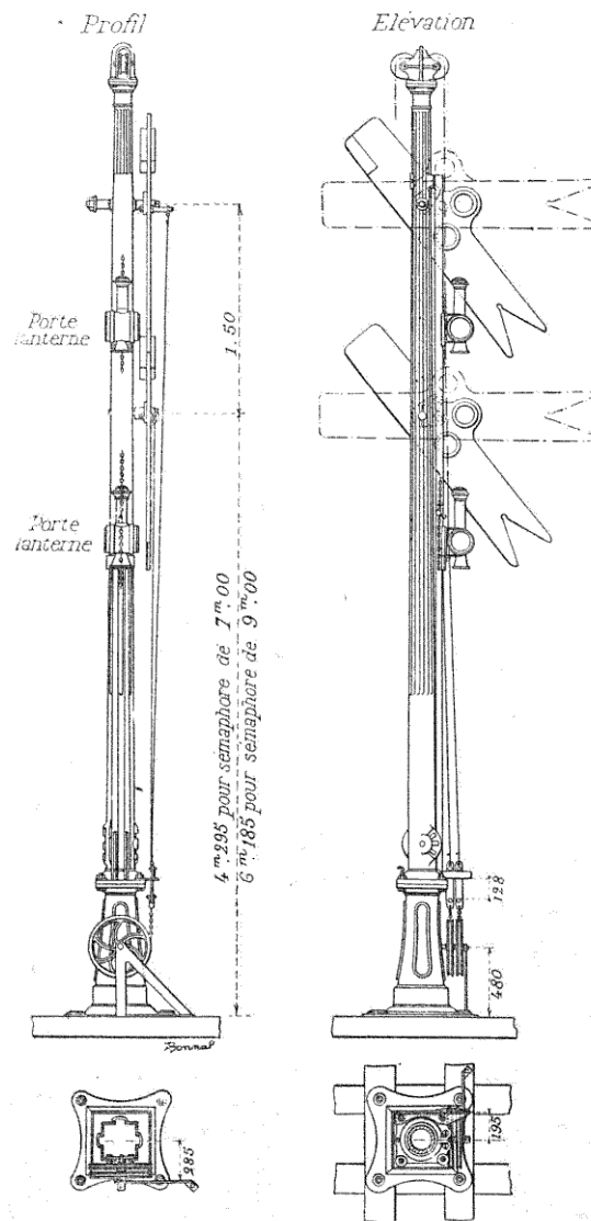
FIG. 82. — Sémaphore de bifurcation du Lyon.
