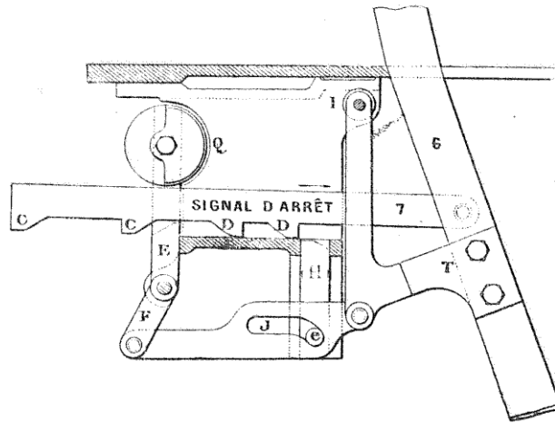
Fig. 107. — Commande du signal d'arrivée par celui de la pédale.
