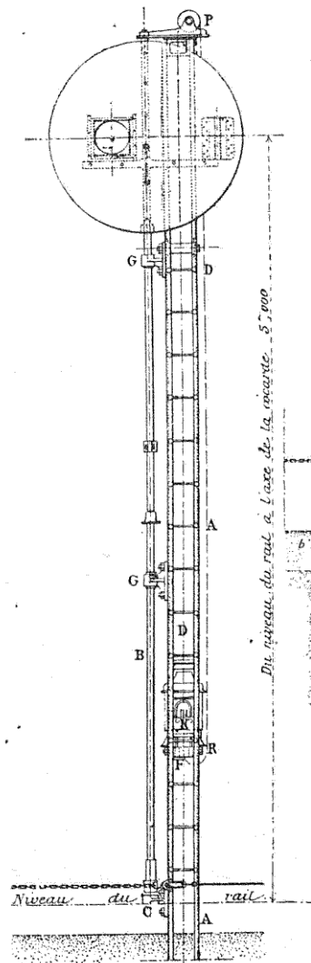
FIG. 60. — Disque avancé de l'Ouest.
