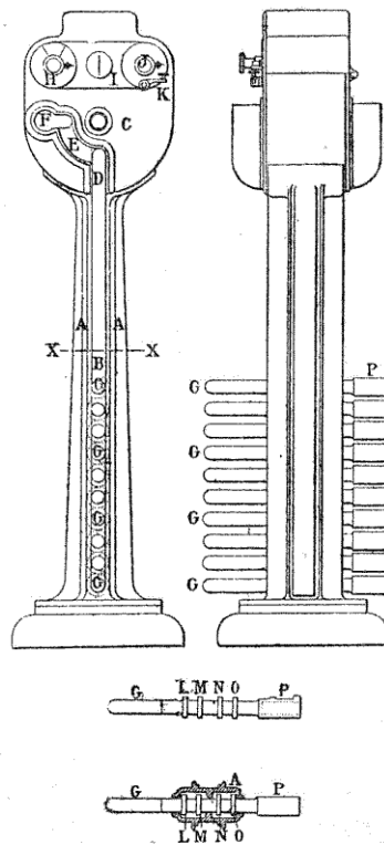
FIG. 257. Bâton-pilote électrique.
