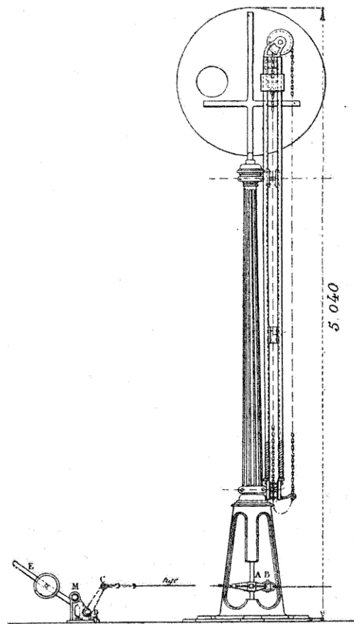
FIG. 61. — Disque de l'Est.
