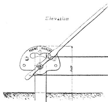
FIG. 70. — Levier de manœuvre à deux fils.
