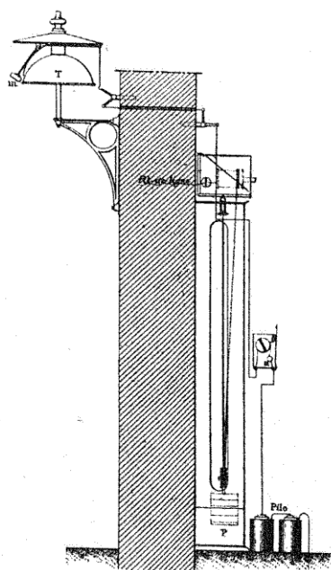
FIG. 271. — Cloche Léopolder.
