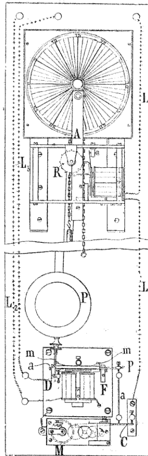
FIG. 279. — Enregistreur Rabier et Leroy.
