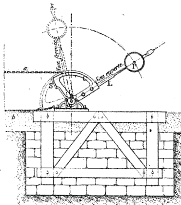
FIG. 61. — Levier de manœuvre (Ouest).
