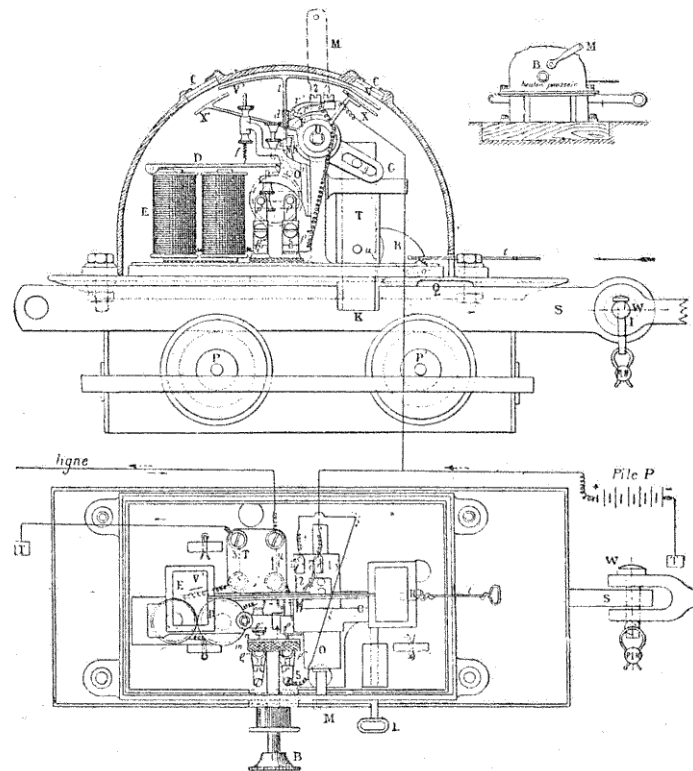
FIG. 204. — Verrouillage d'un levier isolé.
