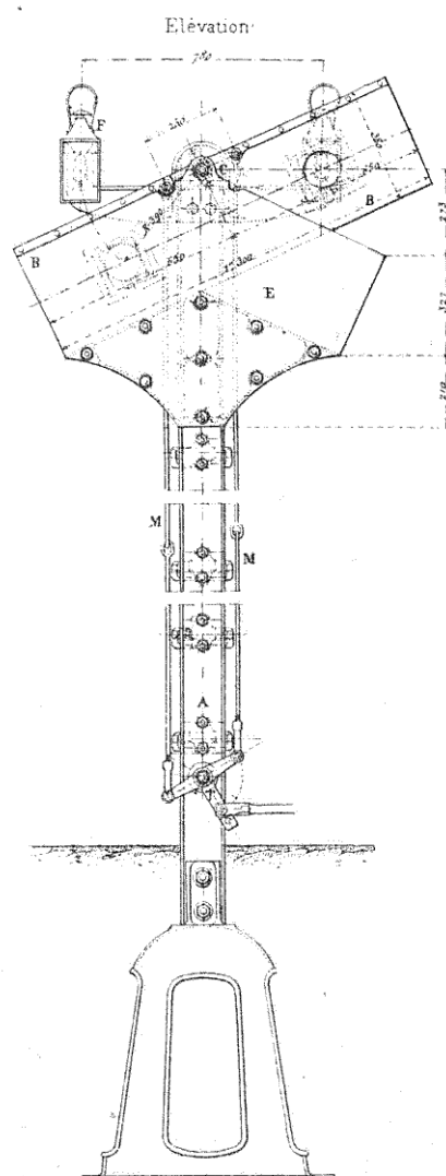
FIG. 84. — Indicateur de direction (Ouest).
