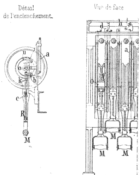
FIG. 170. — Système Froitzheim (transmissions par fils).
