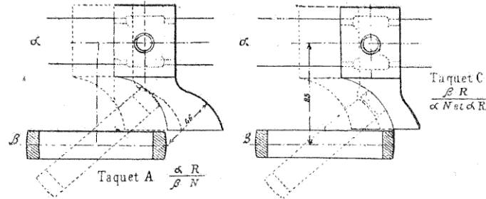
Fig. 158. — Grils et taquets.
