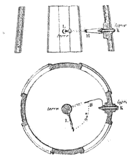
Fig. 141. — Contrôleur du Lyon.
