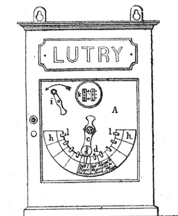
FIG. 268. — Ensemble du transmetteur.
