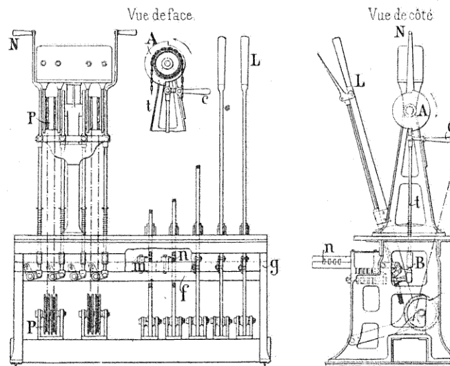
FIG. 169. — Système Froitzheim (Transmissions rigides).
