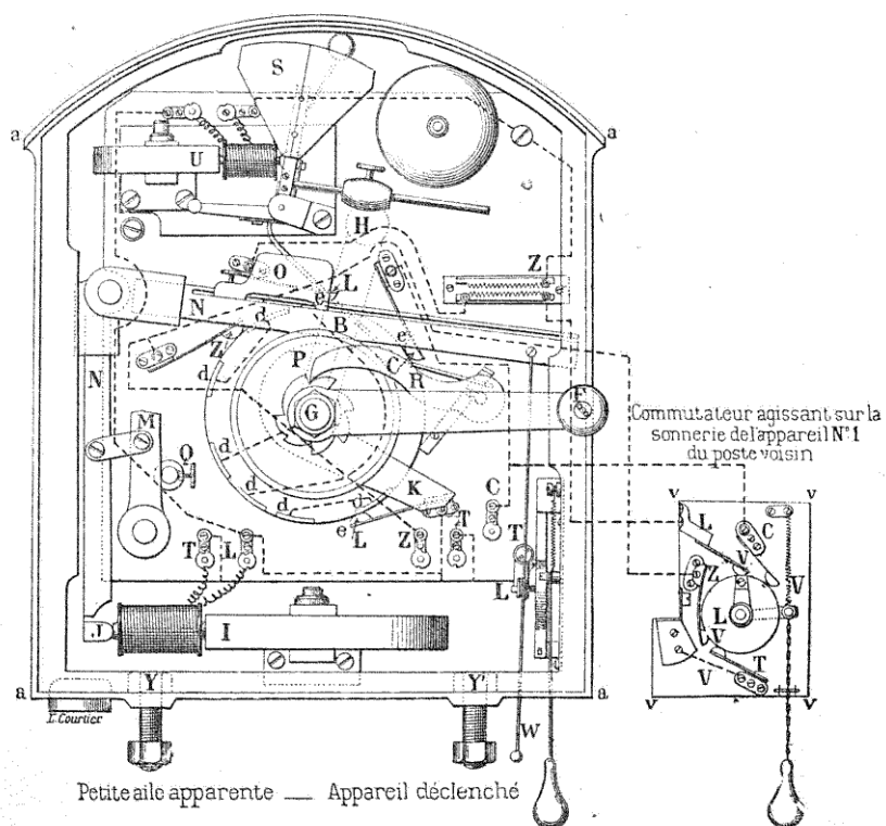
FIG. 239. — Boîte n° 2.
