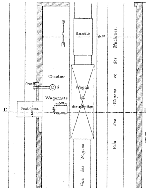
FIG. 288. — Chargement direct par wagonnets.
