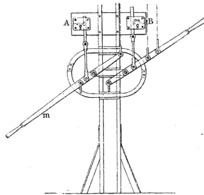
FIG. 208. — Levier verrouillé.
