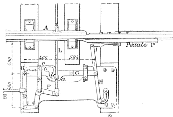
Fig. 111. — Verron-aiguille Dujour.
