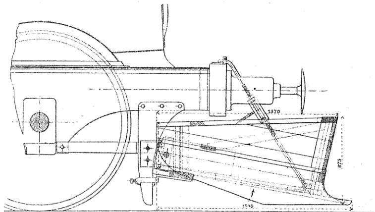
FIG. 302. — Chasse-neige à l'avant de la machine.
