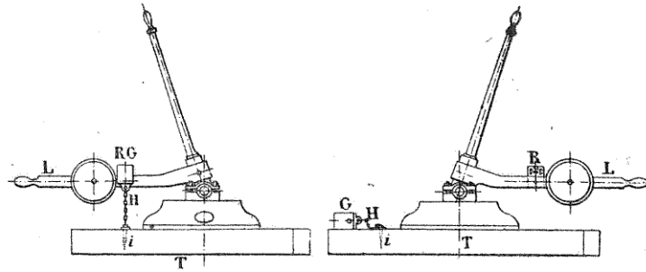
FIG. 209. — Montage d'une serrure.
