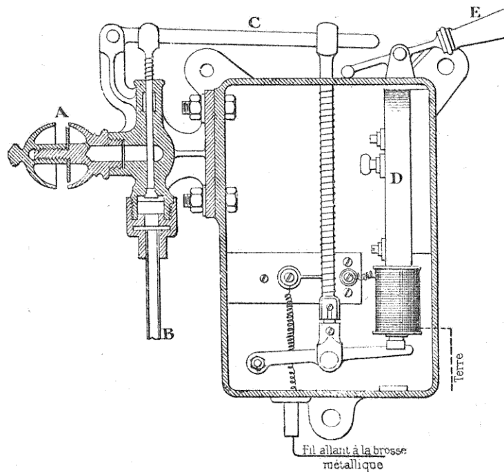
FIG. 90. — Sifflet électromoteur
