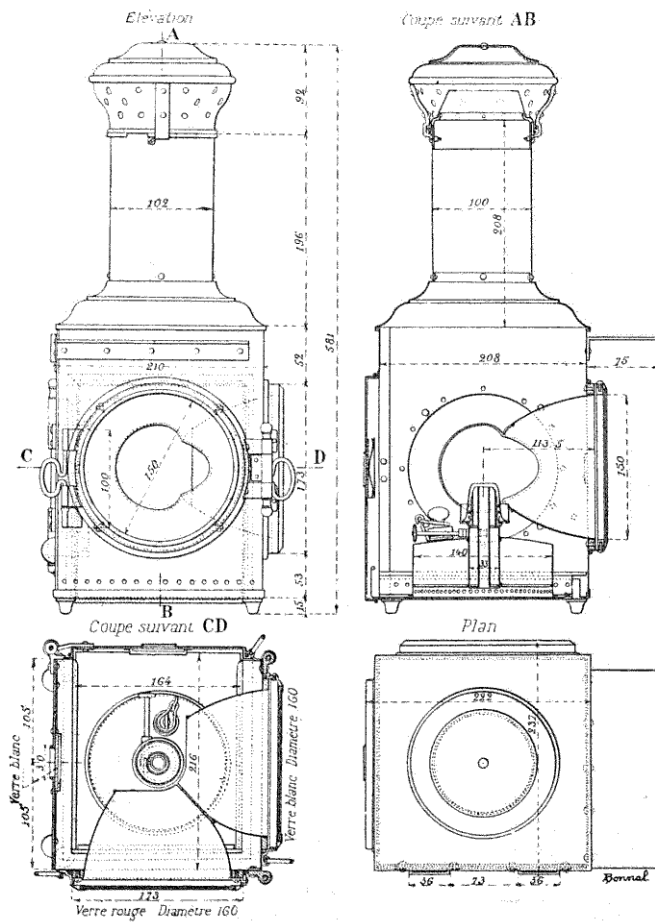
FIG. 9.— Lanterne fixe au pétrole, bec rond (Lyon).
