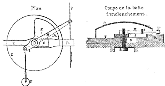
FIG. 175. — Enclenchement Rothmuller.
