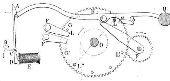
FIG. 266. — Mécanisme de la cloche de l'Etat belge.
