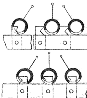
FIG. 168. — Enclenchement Heidrich.
