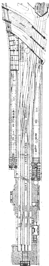
Fig. 20. — Gare de Postdam.
