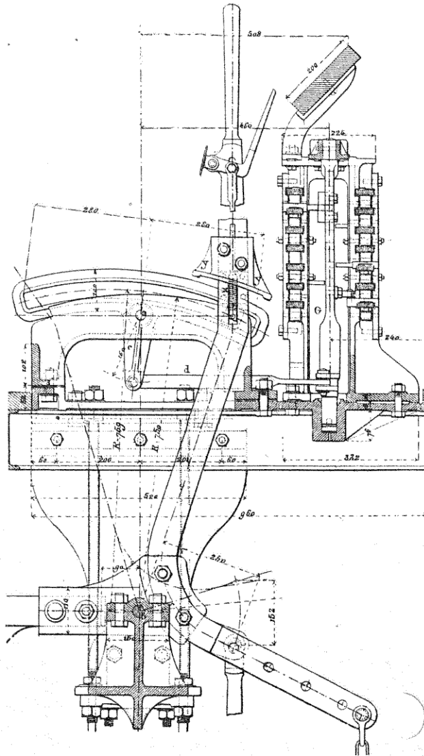
FIG. 156. — Enclenchement Saxby (type P.-L.-M.).
