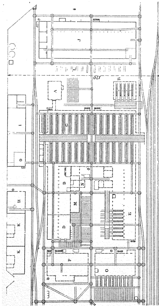
Fig. 297. — Ateliers d'Heilennes (Traction).
