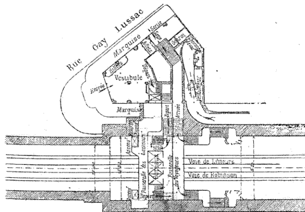
FIG. 3. — Bâtiment surélevé (gare du Luxembourg).
