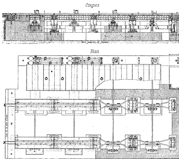
FIG. 293. — Appareil de pesage.
