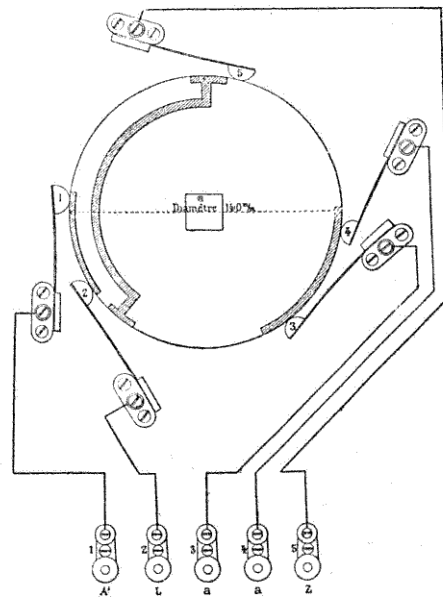
FIG. 260. — Commutateur répéteur-interrupteur.
