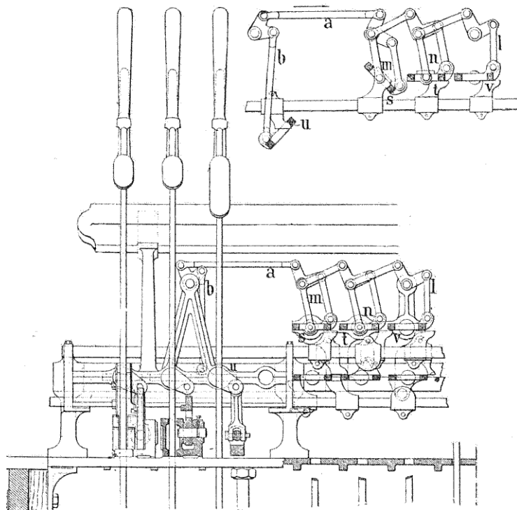
FIG. 166. — Solution générale des enclenchements (Saxby).
