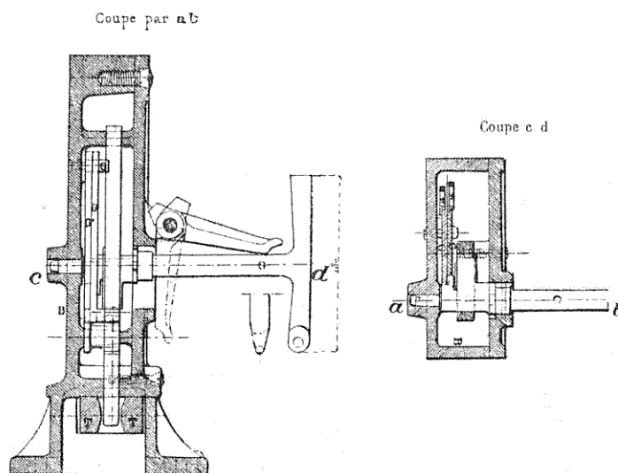
FIG. 206. — Serrure Annett.
