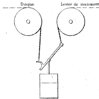
FIG. 94. — Compensateur Robert.
