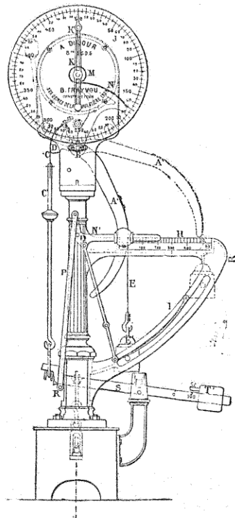
FIG. 51. — Balance Dujour.
