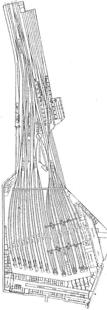
Fig. 11. -- Gare Saint-Lazare.
