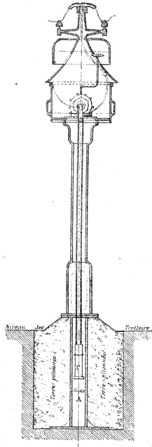
FIG. 264. — Cloche Siemens.
