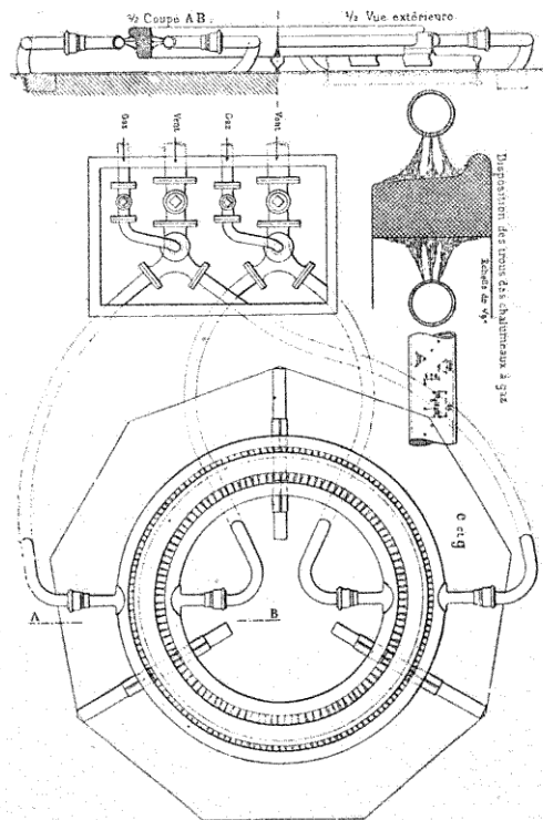
Fig. 296. — Emballage au gaz.
