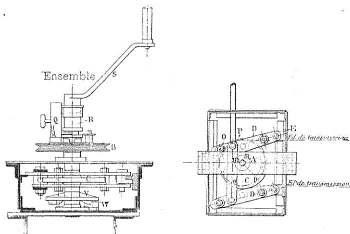
FIG. 124. — Manœuvre par came (État néerlandais).
