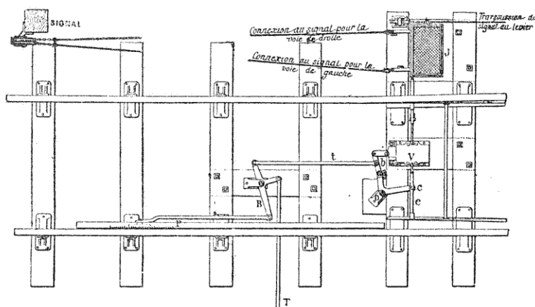
Fig. 113. — Verrou-aiguille Saxby et Farmer.
