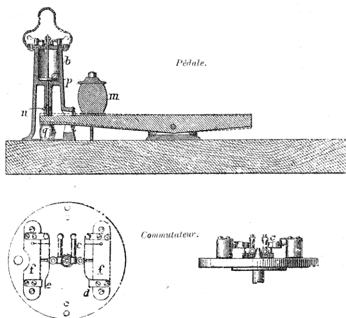
Fig. 248. — Block de Hall.
