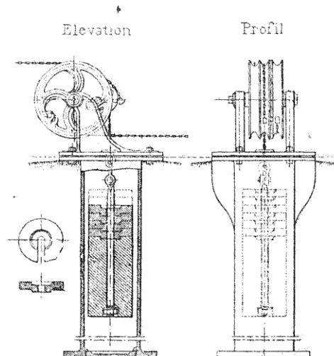
FIG. 97. — Compensateur pour faible entrevoie.
