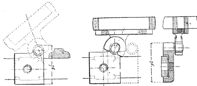
Fig. 157. — Manœuvre des tringles.
