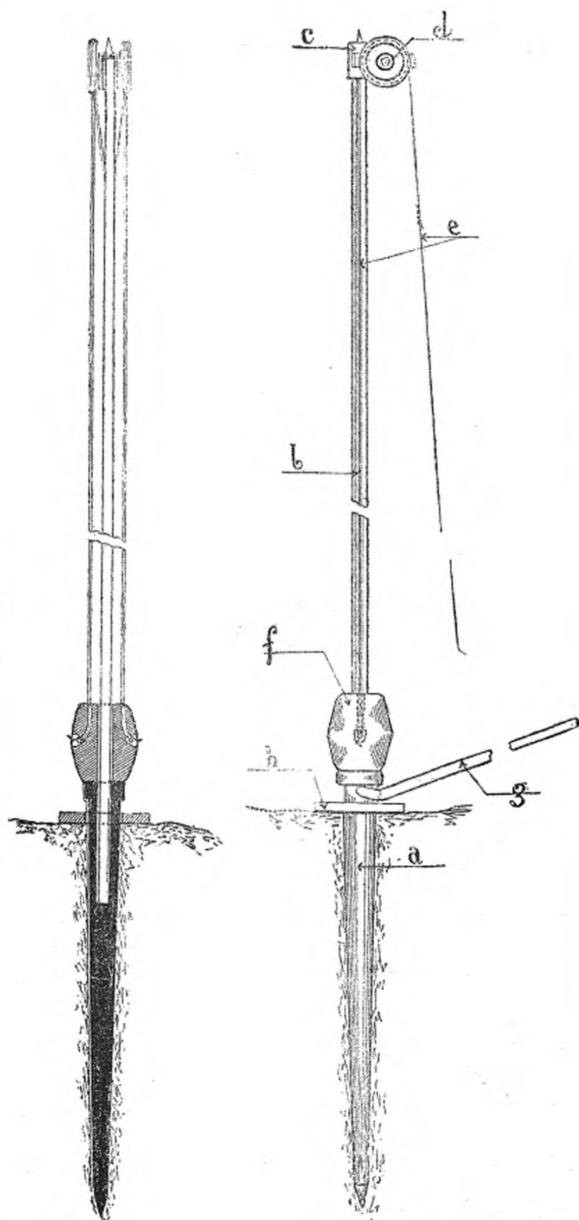
(Fig. 1). Appareil de placement des poteaux.
