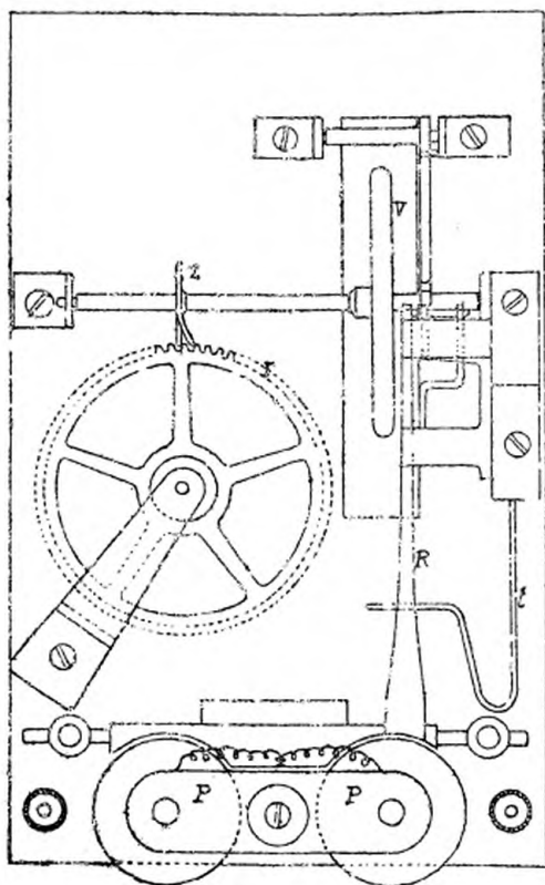
Fig. 3. Cadran récepteur système Vaudeplancke.
