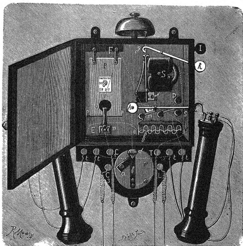
Pantéléphone De Loch-Labye (vue intérieure).
