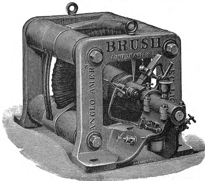
Machine dynamo Brush-Victoria, exposée à Anvers par la Compagnie l'Électrique, de Bruxelles. Type D2 autoregulatrice alimentant 160 lampes à incandescence de 20 candles de 65 volts.
