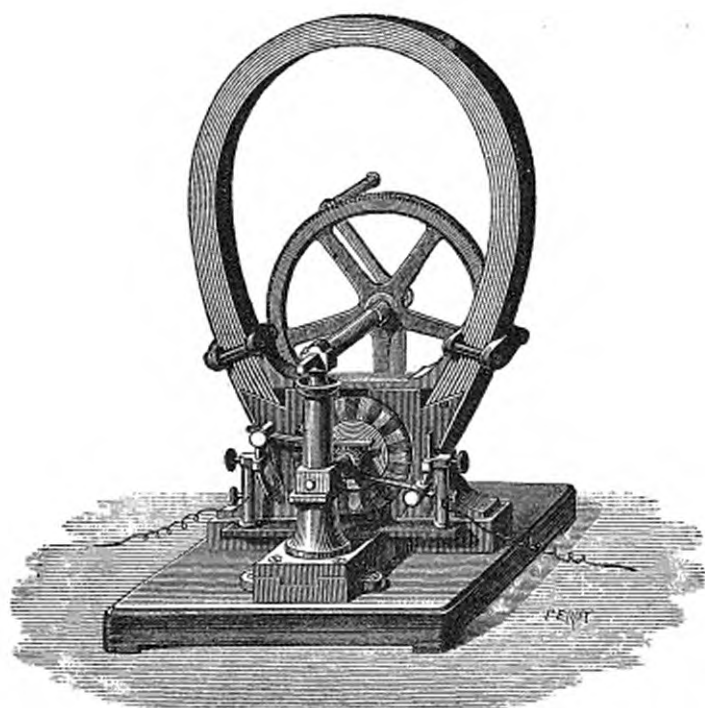
Petite machine de Gramme (modèle de laboratoire .
