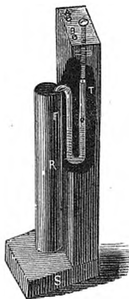
Avertisseur Raikem.
