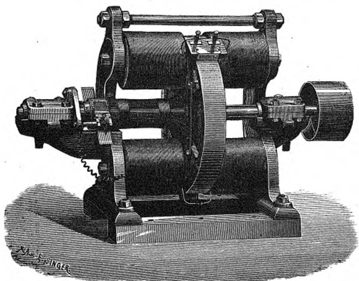
Machine dynamo-électrique de M. S. Schuckert, de Nuremberg, pouvant allumer depuis 2 jusque 14 foyers de 1,000 bougies normales, et depuis 5 lampes à incandescence Edison jusque 72 de 16 bougies; " 15 " " Swan " 100 de 16 "
