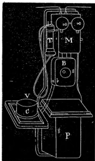
Modification apportée par M. Van Rysselberghe au poste Blake Bell B T avec magneto M pour la téléphonie à longue distance (adoptée par l'administration des télégraphes du Wurtemberg).
