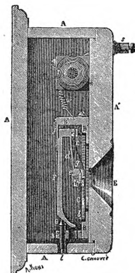
Transmetteur Blake.
