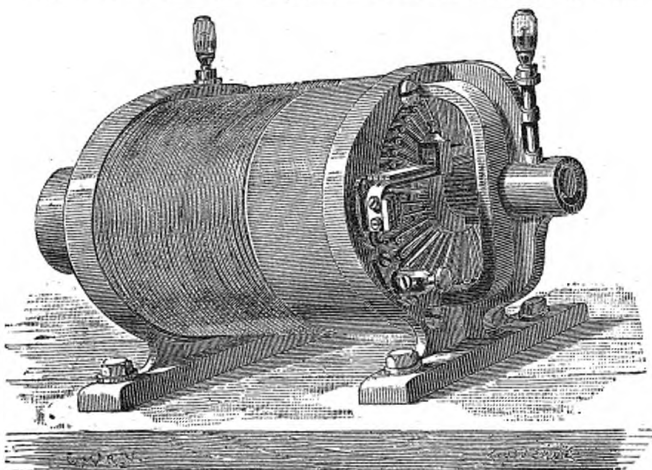
Machine Gramme. Petit modèle-type de 8 ampères, construit dans les ateliers de la Compagnie générale d'Electricité.
