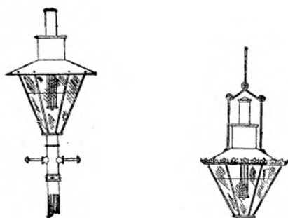
Lampe Brush à arc, avec lanterne et commutateur, installée à l'Exposition d'Anvers par la Compagnie « l'Electrique, » de Bruxelles. (Chaque lampe brûle pendant 16 heures.)
