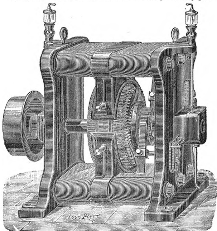
Machine de Gramme.
