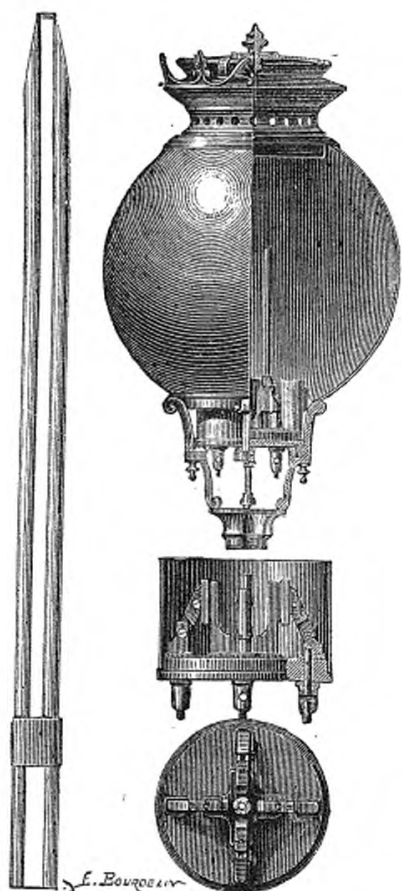
Foyer Jablochkoff (bougie de 4 m/m, donnant une lumière de 45 carcel, force absorbée 1 cheval-vapeur), monté sur candélabre.
