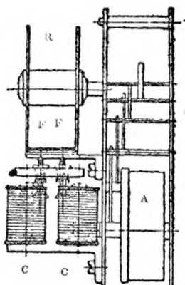
(Fig. 2). Appareil enregistreur Ritzerfeld. Coupe transversale.
