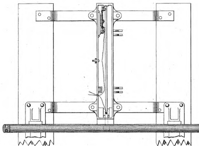
PLAN DE LA PÉDALE-CONTACT AGISSANT PAR LA FLEXION DU RAIL.
