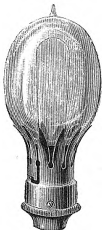
Lampe à incandescence Victoria Brush de 65 volts et de 20 candles, avec support à batonnette.
