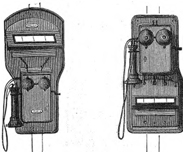
Transmetteurs Ader, modifiés par M. F. Van Rysselberghe, avec sonneries magneto et récepteurs Bell. Modèles employés par l'administration des télégraphes de l'Etat (1).
