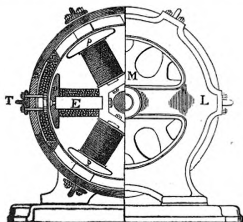
(Fig. I.) Machine dynamo de Zypernowsky.
