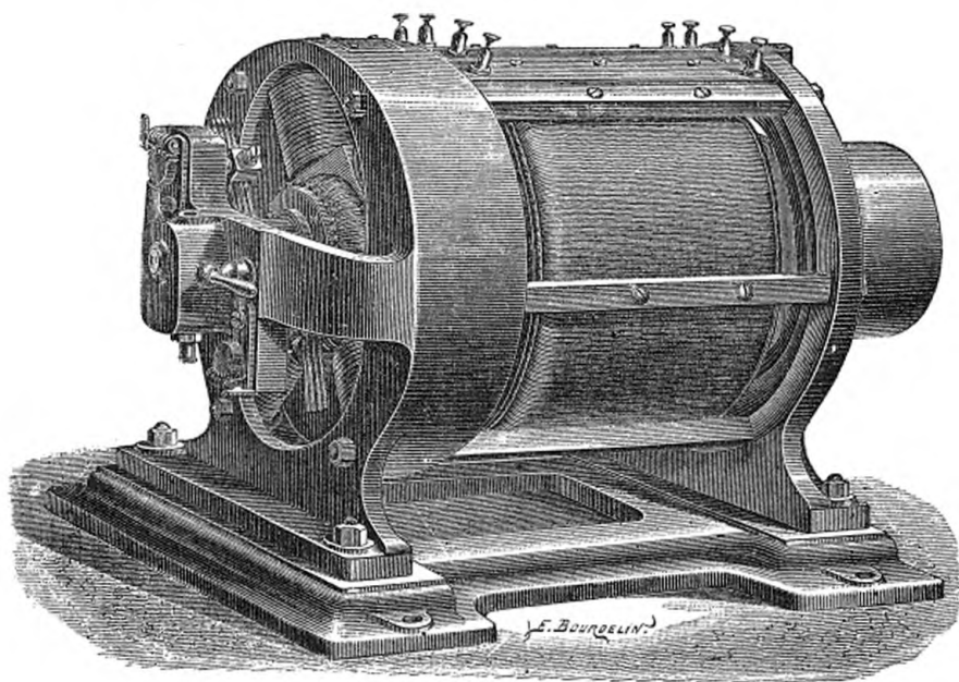
Machine Gramme auto-excitatrice à courants alternatifs, pour l'éclairage par les bougies Jablockhoff (modèle de 20 foyers).
