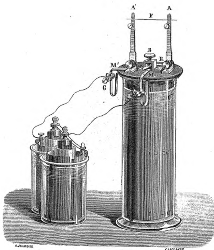
Pile secondaire de M. Gaston Planté.
