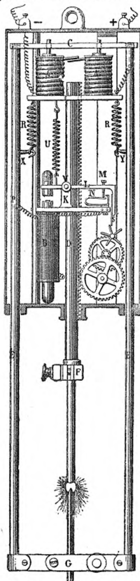
Régulateur de Gramme. — Type de 125 becs-carcel.
