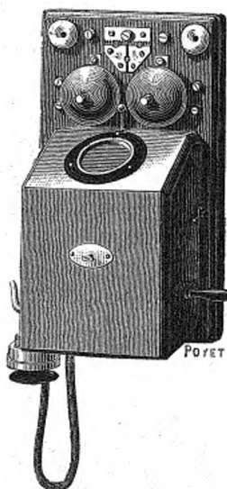
Nouveau transmetteur de M. l'ingénieur Berthon, construit dans les ateliers de la Société Générale des Téléphones de Paris. (Poste complet avec récepteur et sonnerie Magneto.)
