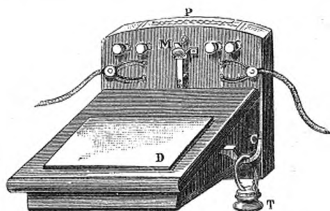
Transmetteur et récepteur d'Ader (1).
