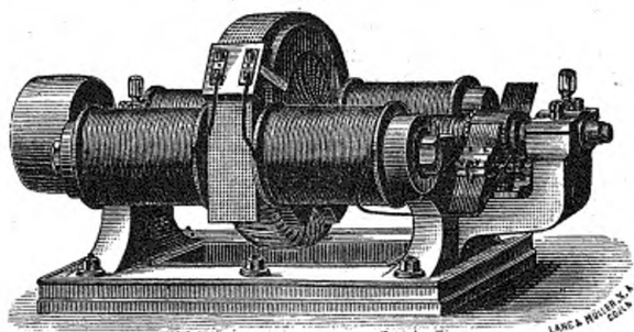
Machine dynamoélectrique à anneaux plats, système C. Dornfeld et E. Cramer, construite dans les ateliers de MM. Spiecker et Cie, de Cologne (type n° IV pour 4 lampes à arc, 23 ampères, 100 volts; type n° IV pour 25 lampes à incandescence de 16/20 bougies, 110 volts).
