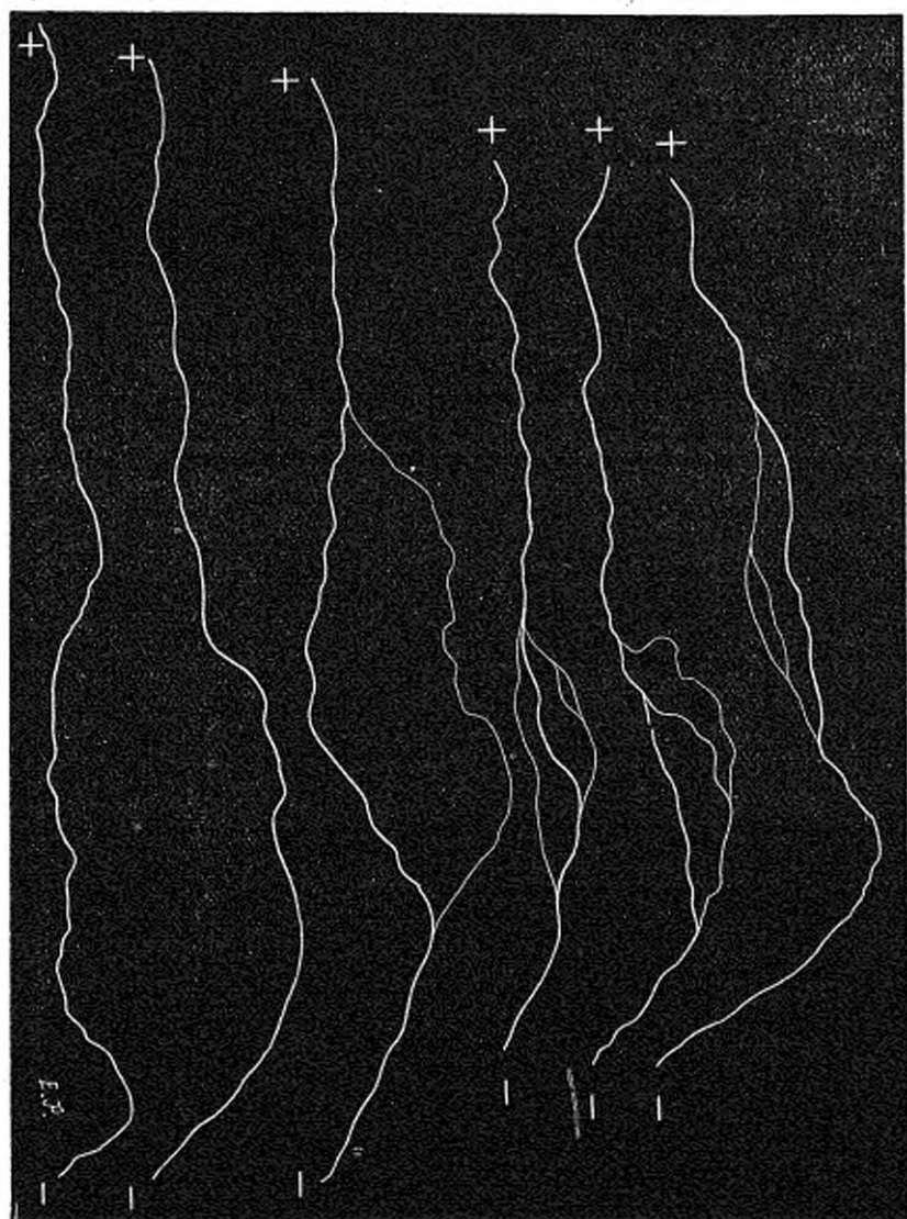
(Fig. 1). Étincelles produites au moyen de la machine rhéostatique de M. Gaston Planté.
