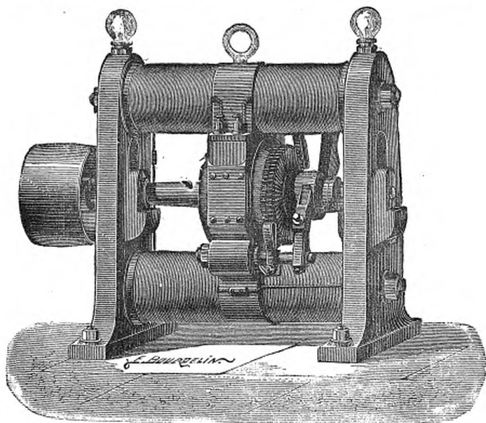
Machine de Gramme.
