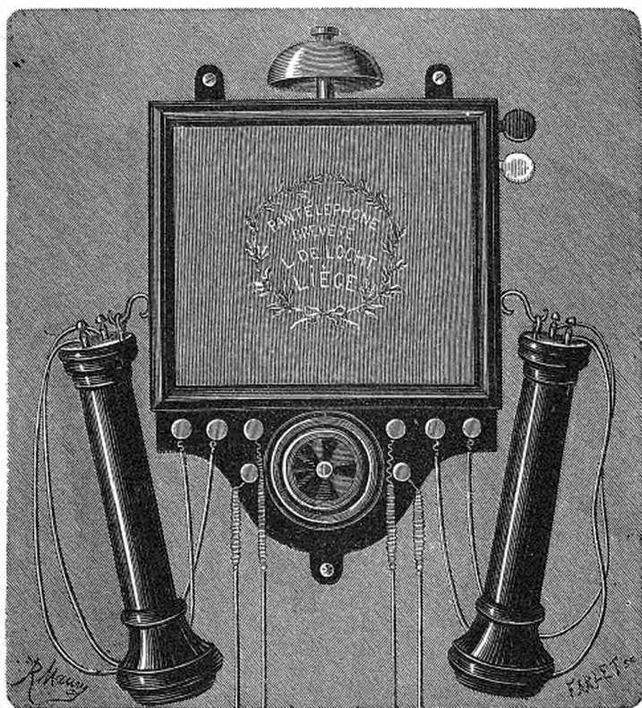
Pantéléphone De Loch-Labye (vue extérieure), exposé dans le compartiment de l'administration des télégraphes de l'Etat.
