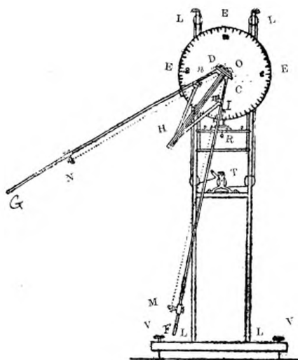
Photomètre de M. E. Rousseau.
