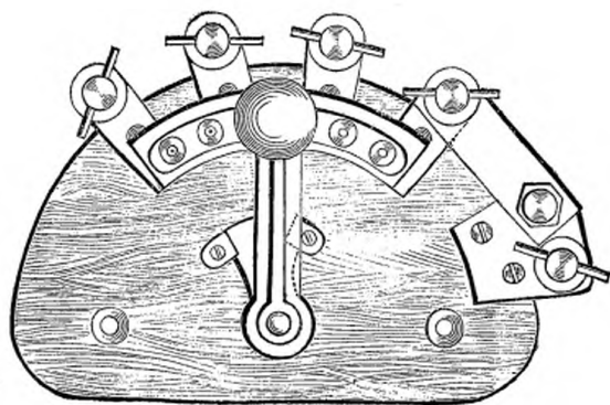
Commutateur de Gulcher.
