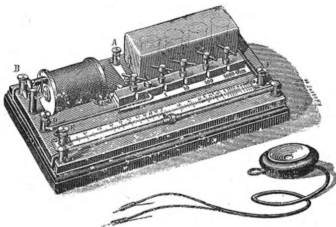
Rhéomètre universel du professeur Kohlrausch.
