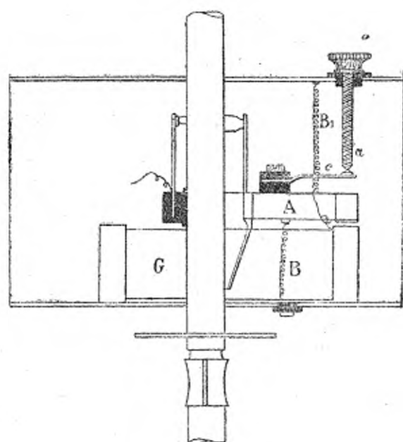
Schema de la lampe.
