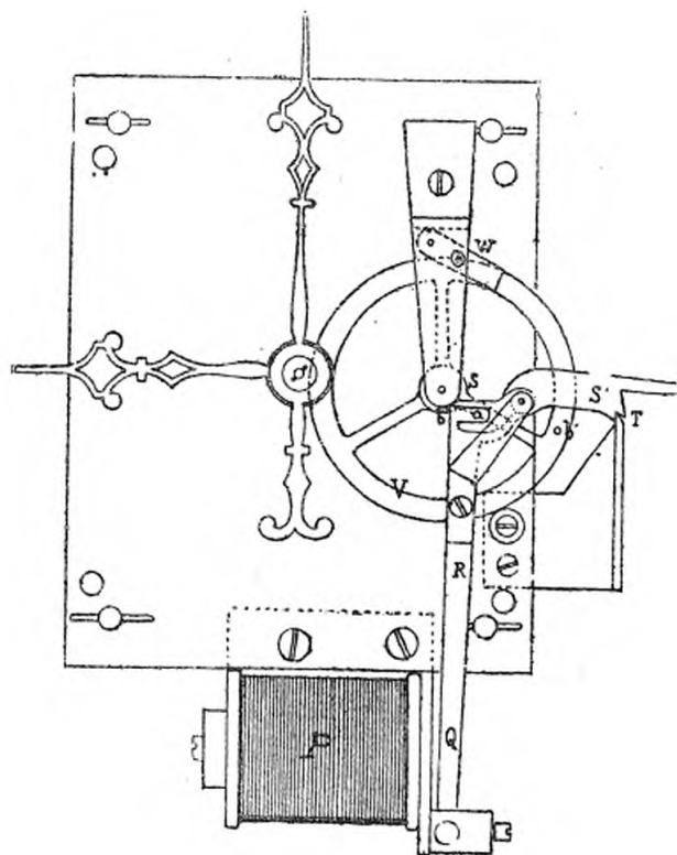
Fig. 1. Régulateur système Vaudeplancke.
