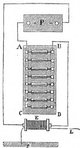
Schema du transmetteur Van Rysselberghe.
