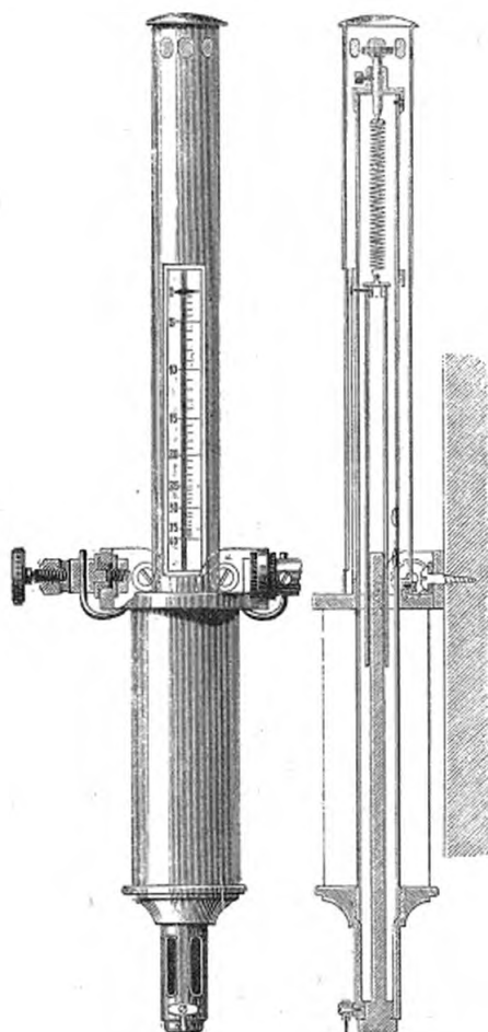
Galvanomètres à spirale, ammètres et voltmètres.
