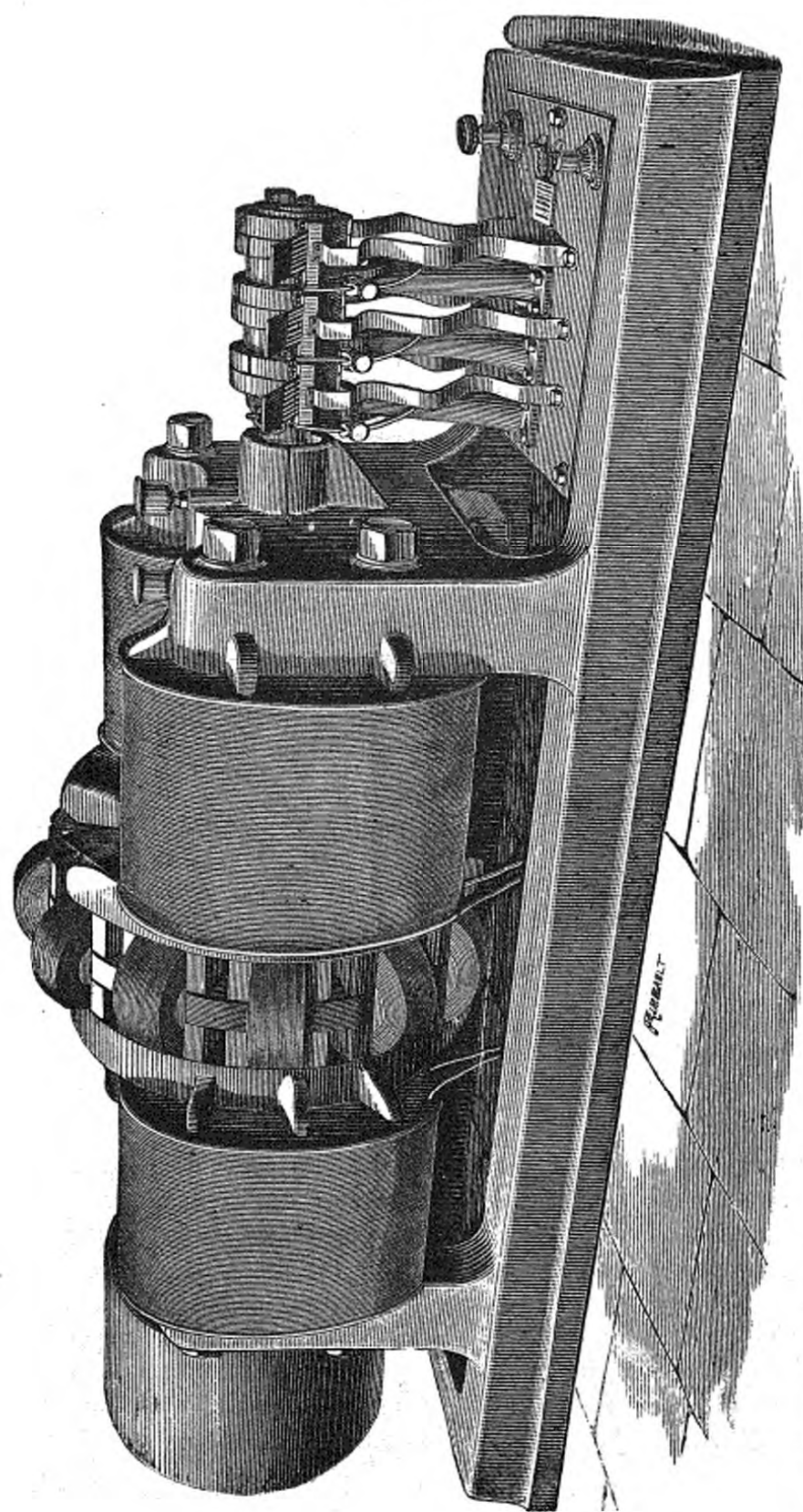
Machine dynamo, système Brush, à nouvel anneau, alimentant 31 lampes de 4,000 candelles, absorbant 20 ampères ou 62 lampes de 10 ampères, exposée par la Compagnie « l'Éclairique » dans la galerie des machines à l'Exposition d'Anvers.
