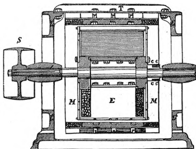
(Fig. II.) Coupe de la machine dynamo de Zypernowsky.
