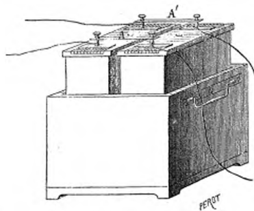
Modèle des premiers accumulateurs créés par M. Gaston Planté (1).
