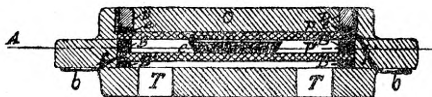
Coupe CD
