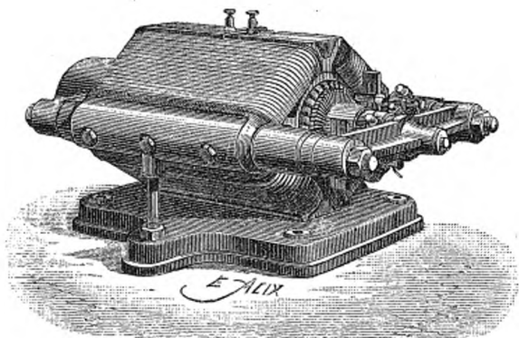
Machine dynamo électrique de de Méritens.
