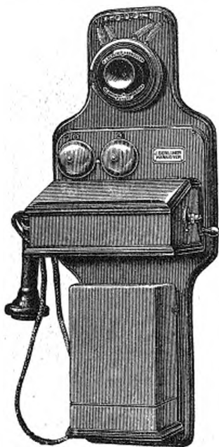
Microphone Berliner, avec sonnerie magneto et récepteur téléphonique de Bell, boîte à piles, etc.
