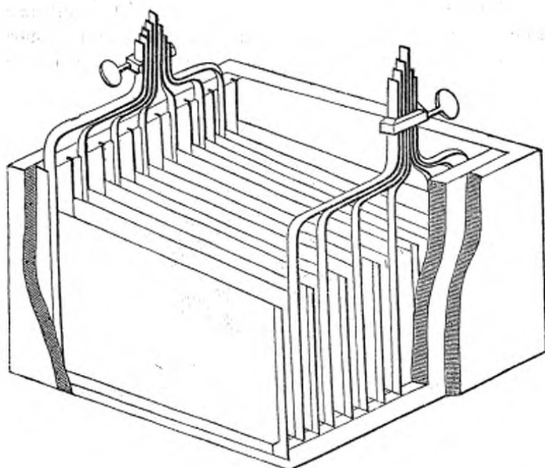
Accumulateur René Tamme (1), exposé à Anvers par la maison H. Tamme et C ie , de Bruxelles.
