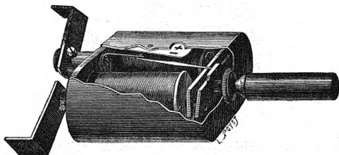
Sonnerie d'essai pour piles et accumulateurs, de MM. Barbier et Pierret, de Paris.
