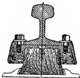
Isolateur de rail central pour le tramway électrique du système Daft.
