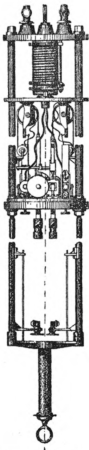
Lampe de Gulcher, installée par la Compagnie générale d'électricité pour l'éclairage d'une partie de la galerie des machines de l'Exposition à Anvers. (Type de 2500 bougies.)
