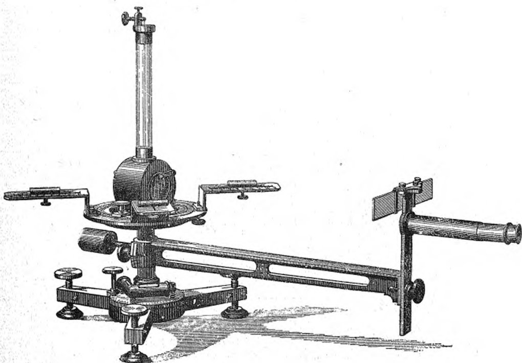
Variomètre portatif d'intensité locale du magnétisme terrestre.
