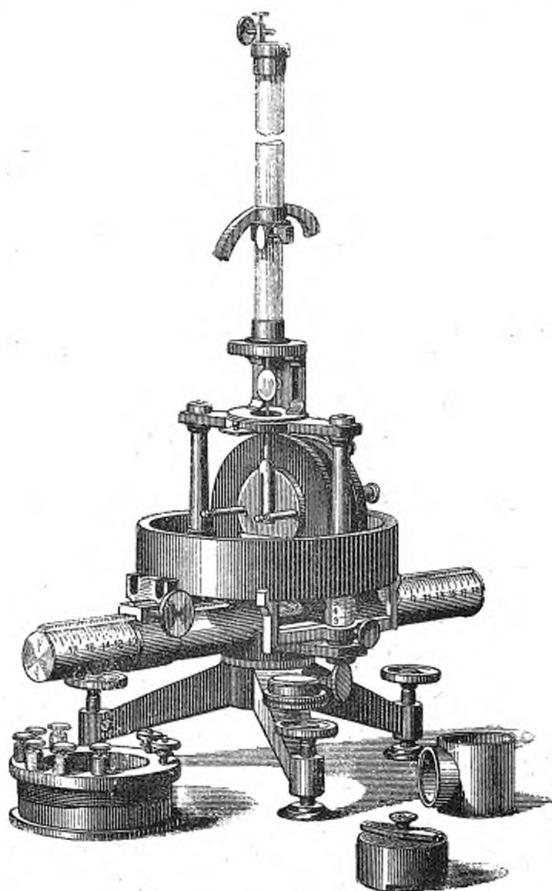
Grand galvanomètre à miroir aperiodique.
