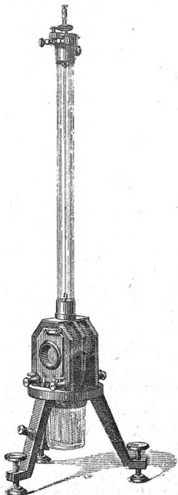
Electro-dynamomètre à un fil pour de faibles courants.
