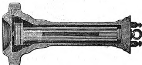
Téléphone de Bell (coupe transversale). Nouveau modèle, avec gaine en ébonite, employé actuellement par l'administration des télégraphes et par les compagnies de téléphones en Belgique.
