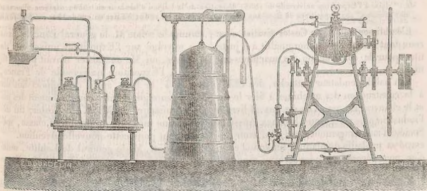
Machines à eau de Seltz, de 800 à 3,000 francs.
