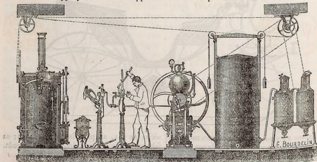
Appareil saturateur à deux corps de pompe et producteur fonctionnant par une petite machine à vapeur et produisant dix mille bouteilles par jour.
