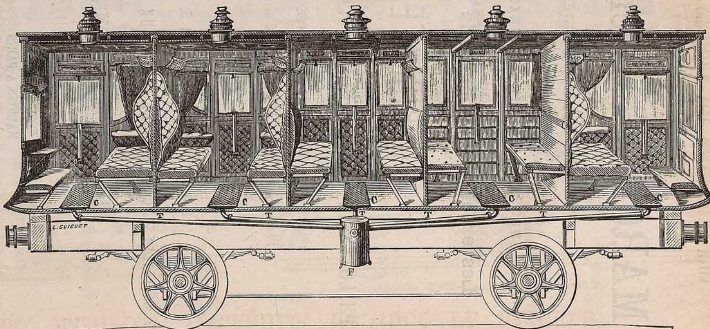
F. Foyer chauffant 5 compartiments. C. Chauffetteries de 2 mètres longueur et 30 cent. largeur. O. Tuyau du chargement du combustible.
