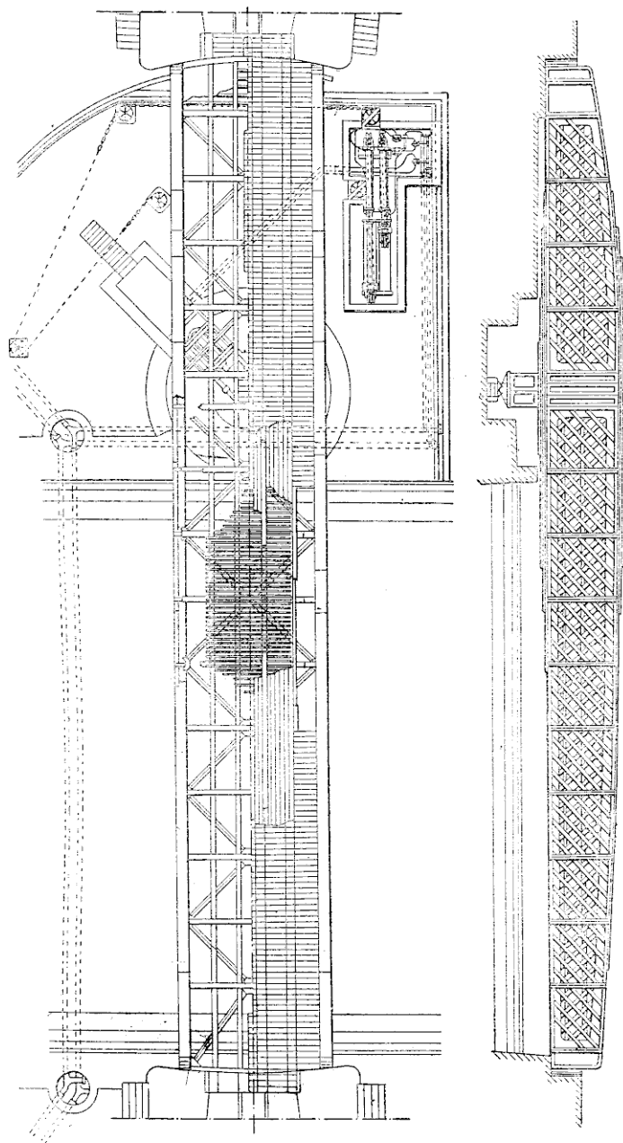
Élévation et plan du pont tournant de l'écluse Belloc.
