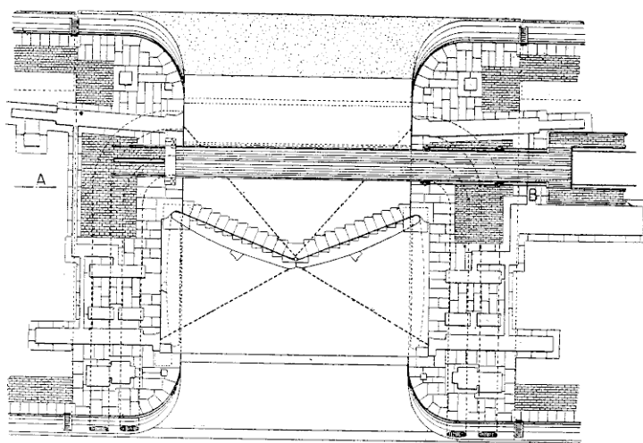
Plan de l'écluse.
