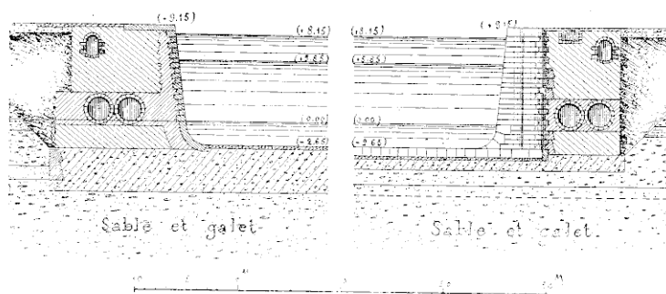
Coupe transversale de l'écluse Bellot.
