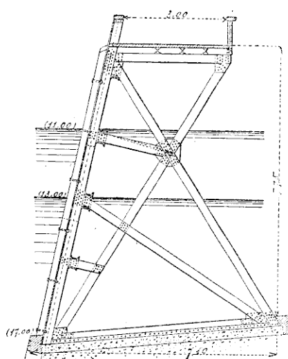
Estacade métallique du brise-lames sud.
