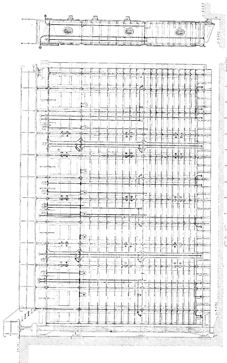
Élévation et coupe d'un vantail des portes de l'écluse Belloc.
