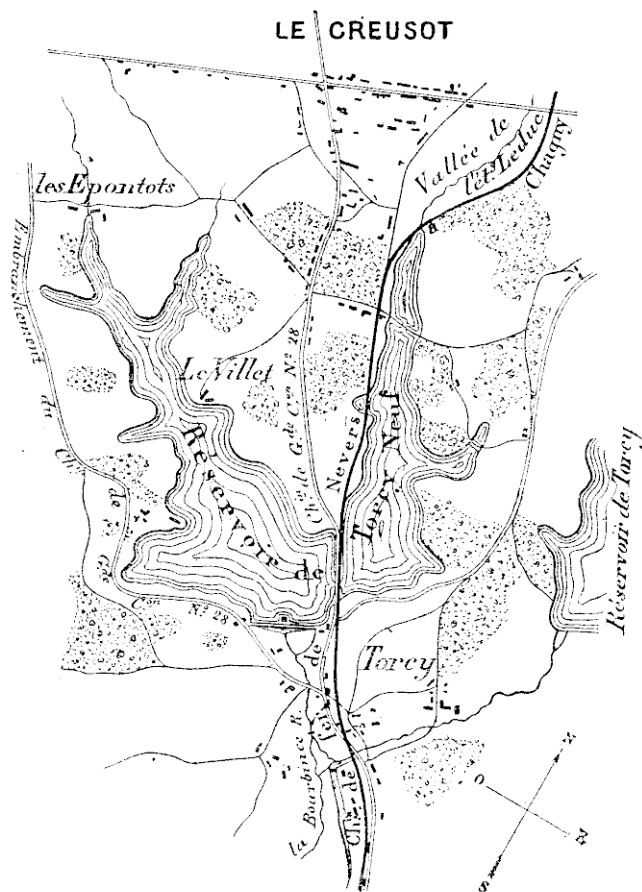
Plan général du Réservoir.
