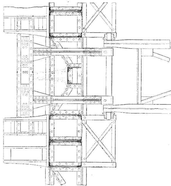
Suspension des cadres du barrage de Port-Mort.
