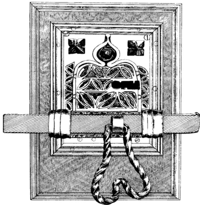
SERRURE A VERTEVELLE DU XVI e SIÈCLE MONTÉE SUR UN PLATEAU EN BOIS
