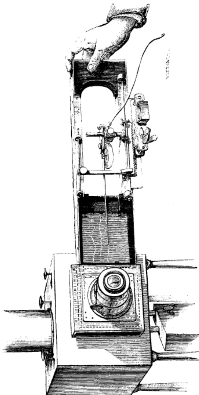
Fig. 55. — Polygraphe à projection. — L'appareil est représenté au moment où on le retire du mégascope à lumière électrique dans lequel il a tracé des graphiques de mouvements qui lui étaient transmis d'une distance de 45 mètres au moyen d'un tube de caoutchouc. On voyait les graphiques se former en traits lumineux sur l'écran. Ces figures étaient amplifiées environ à 30 diamètres.
