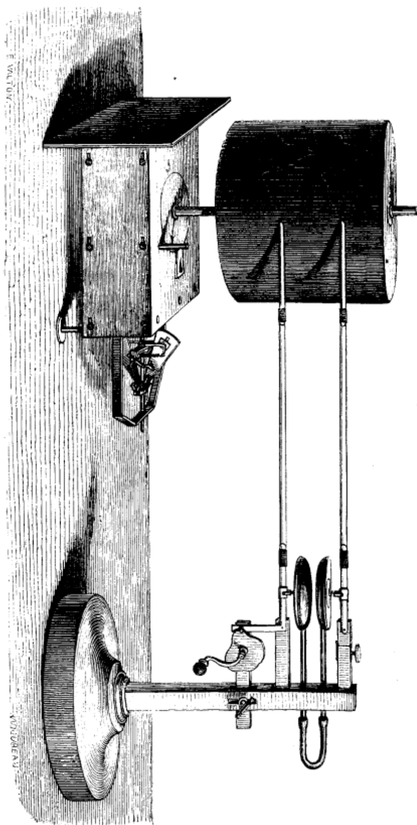
Fig. 57. — Appareil servant à vérifier les appareils enregistreurs d'après la méthode de Doulers.
