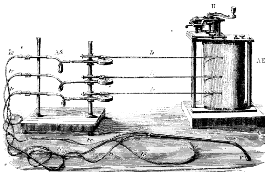
FIG. 36. — Cardiographe de Chauveau et Marey.
