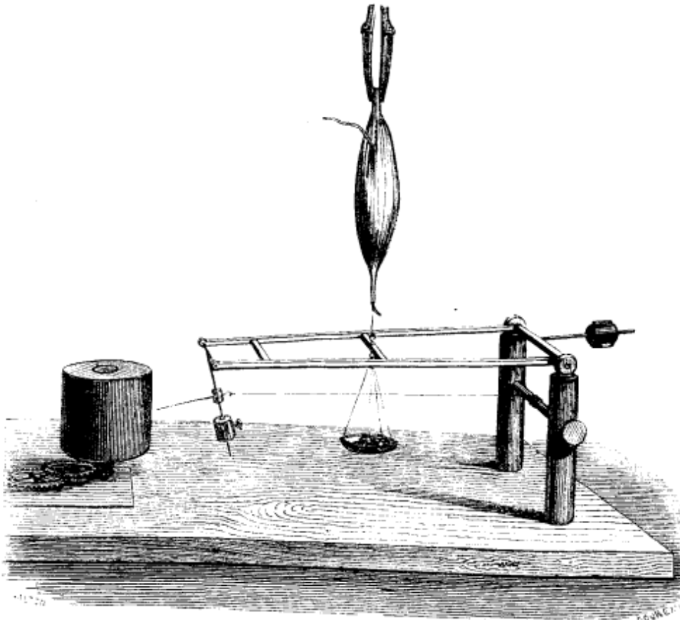
FIG. 28. — Myographe de Helmholtz.
