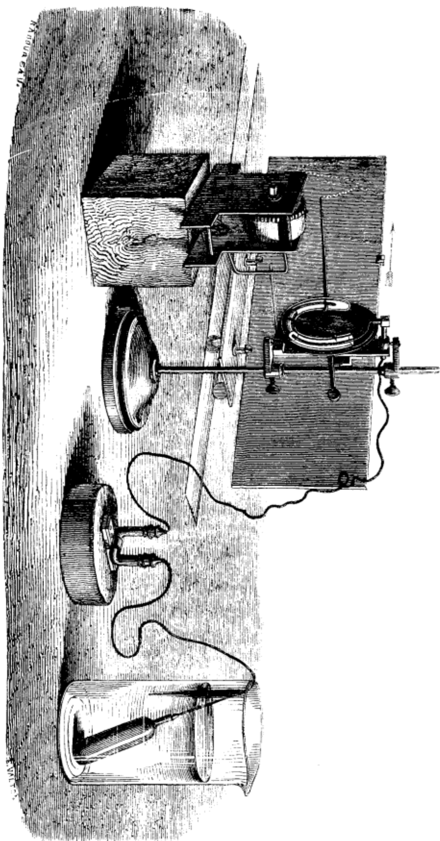
Fig. 58. — Thermographe ou appareil enregistreur des variations de la température.
