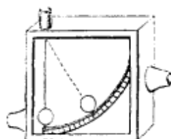
FIG. 45. — Hémotachomètre de Vierordt.
