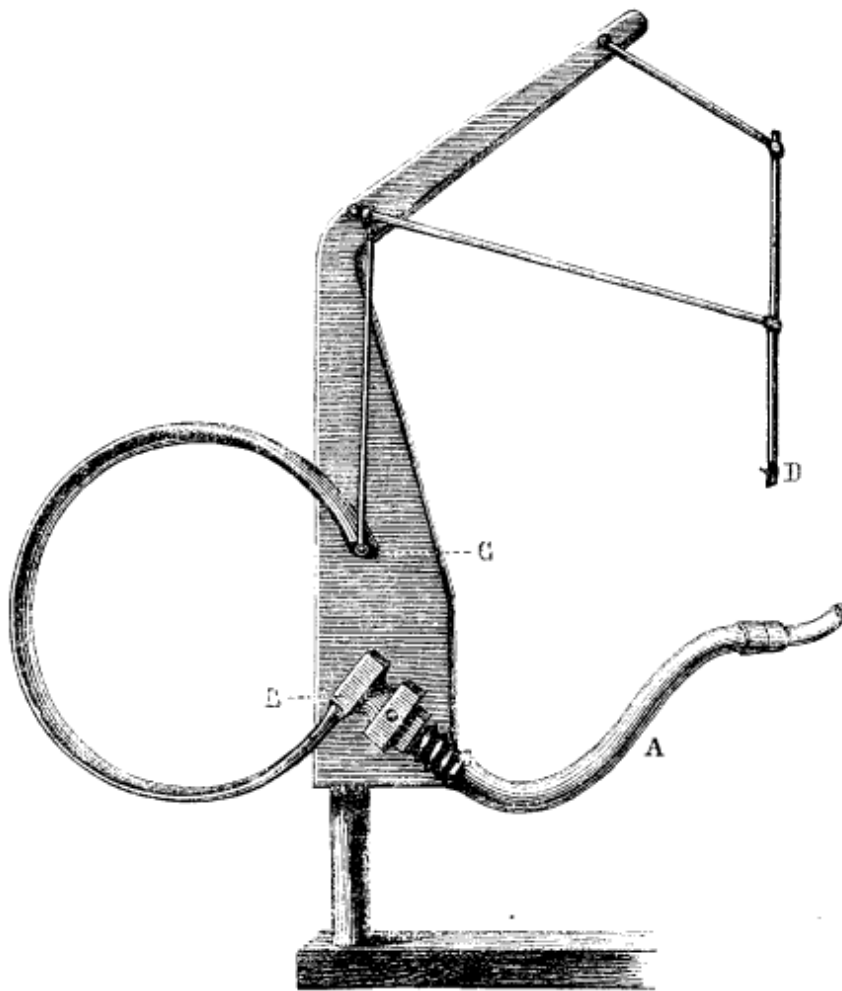
FIG. 44. — Kymographion à ressort de Fick.
