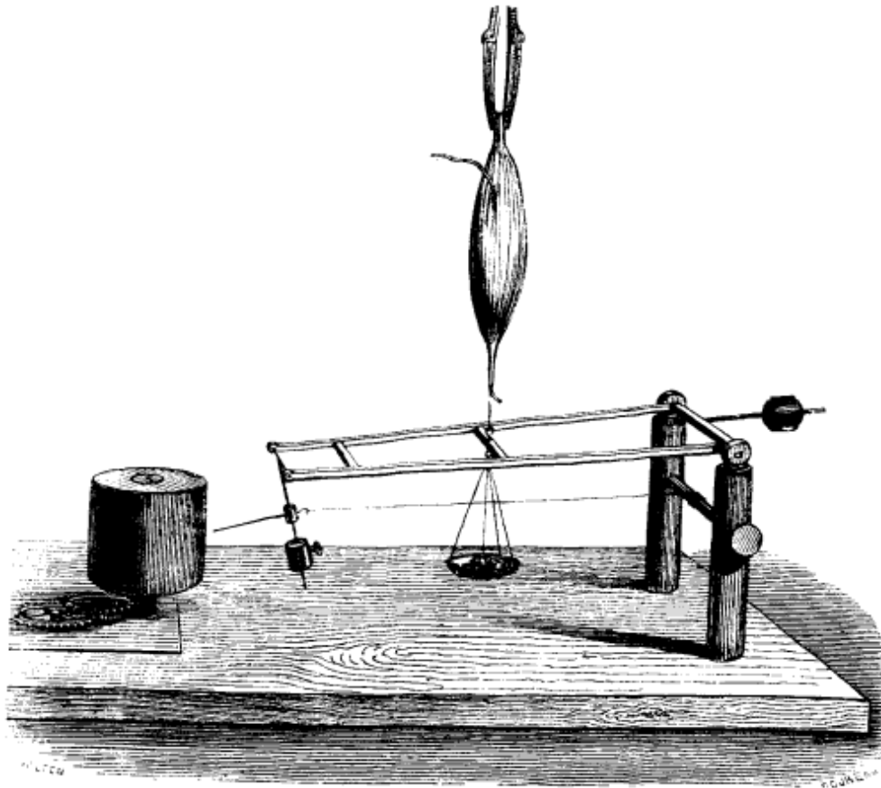
FIG. 59. — Myographe de Helmholtz.
