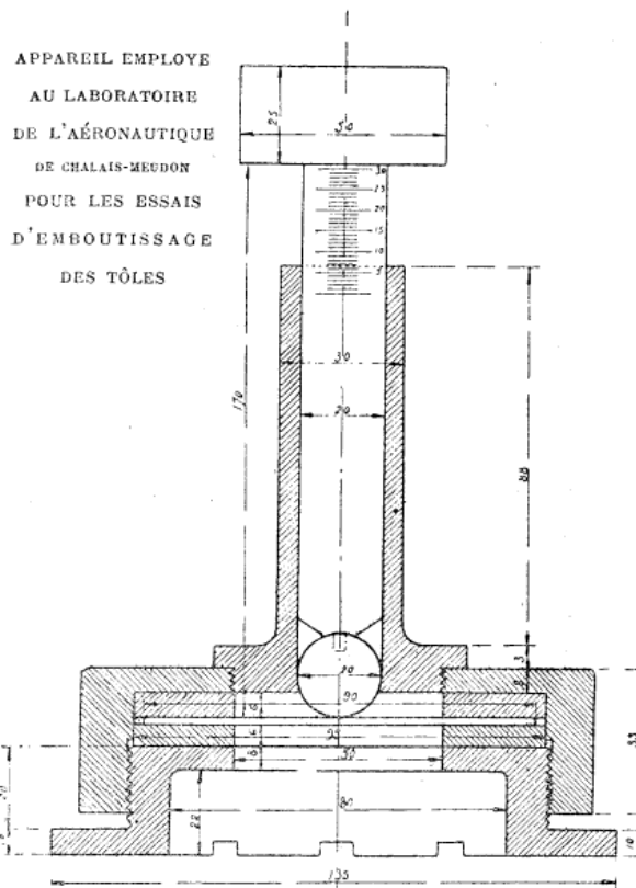
Fig. 3. — Essai des tôles d'acier à l'emboutissage.
