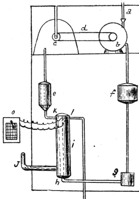
Fig. 80. — Calorimètre Junkers enregistreur.
