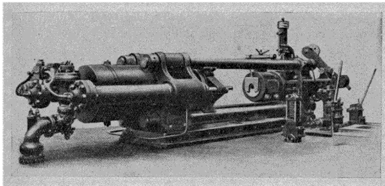
Fig. 1. — Presse de 600 tonnes à filer les métaux (S. O. M. U. A.) (Aluminium et alliages).
