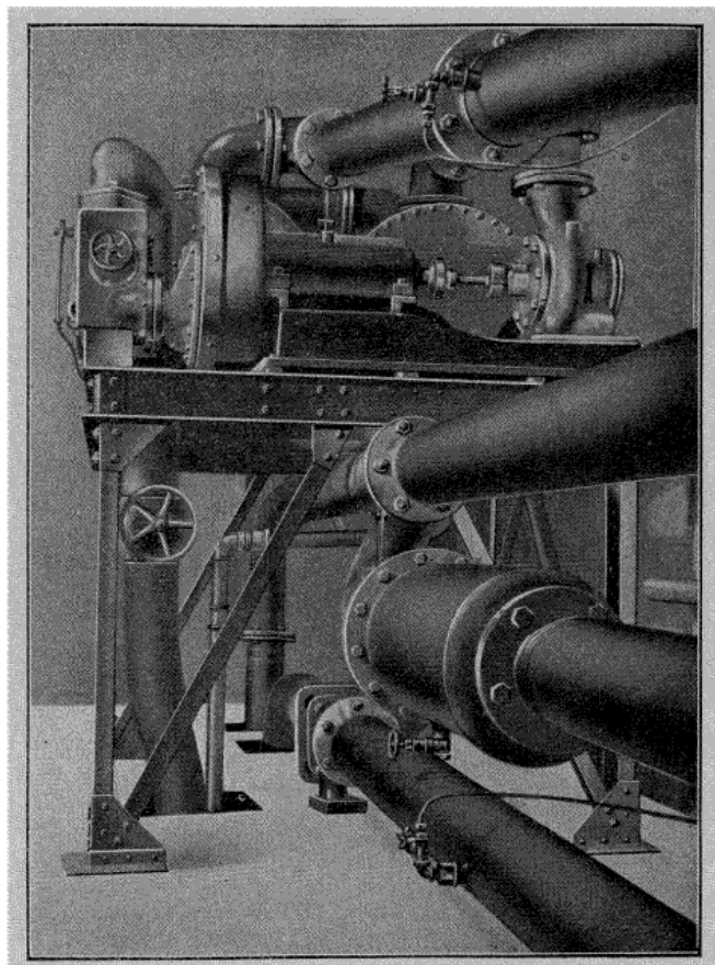
Fig. 16. — Groupe de circulation système dynamo-circuit pour un groupe de 17 immeubles.
