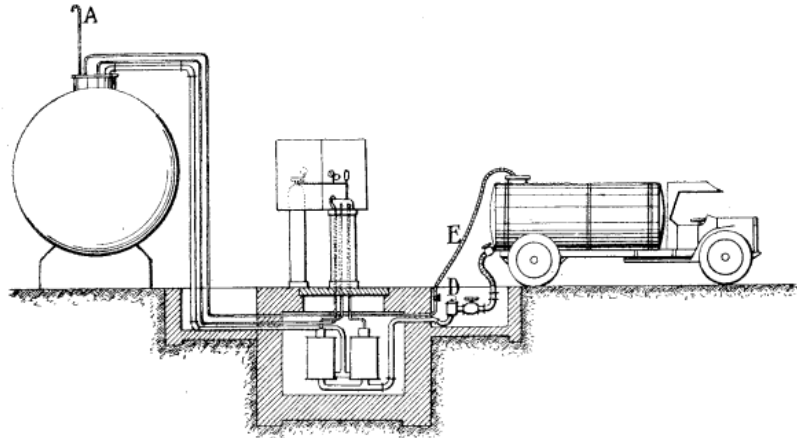
Fig. 12. — Installation de sécurité. Système Mauclère, à semi-récupération de vapeurs. Ravitaillement par camion-citerne d'un réservoir en surface.
