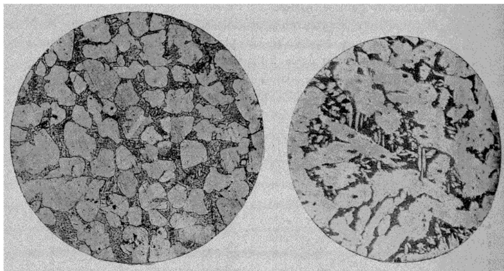
Fig. 27. — Bronze d'aluminium (Al = 9,5 p. 100). Recuit. Grossissement : 50 d. Fig. 28. — Bronze d'aluminium (Al = 9,5 p. 100). Trempe à 550°. Grossissement : 50 d.
