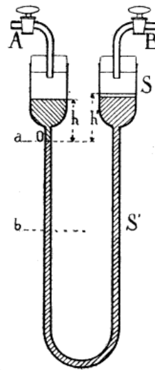
Fig. 43. — Manomètre à deux liquides non miscibles.
