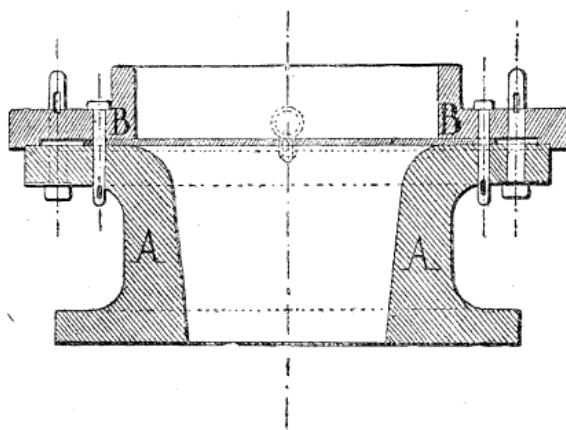
Fig. 1. — Dispositif du montage des tôles essayées à l'emboutissage par le Jern Kontor suédois.
