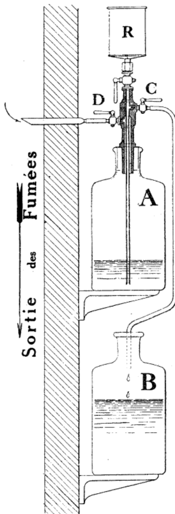
Fig. 8. — Dispositif échantillonneur.
