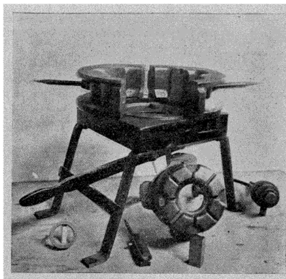
Fig. 3. — Dynamo-démarreur, palier côté commande (moule démonté).
