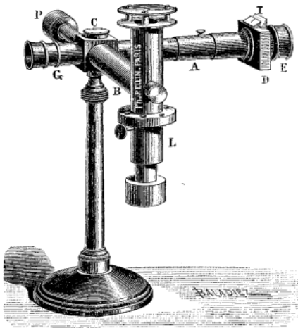
Fig. 36. — Pyromètre optique Le Chatelier (vue d'ensemble).
