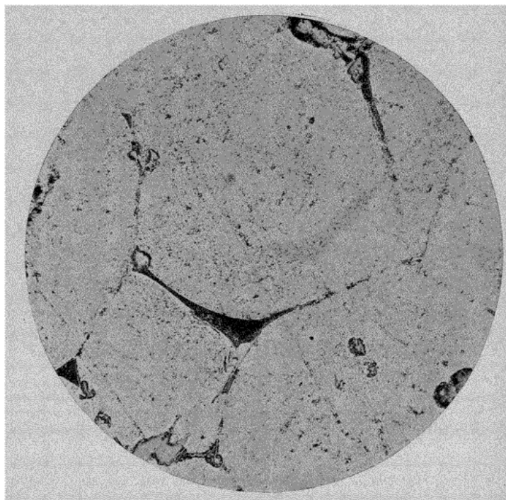
Fig. 42. — Duralumin. Attaque par NaOH pendant 30 secondes. Trempé à 475^\circ Grossissement : 200 d.
