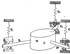
Fig. 5. — Schéma d'un appareil triple.
