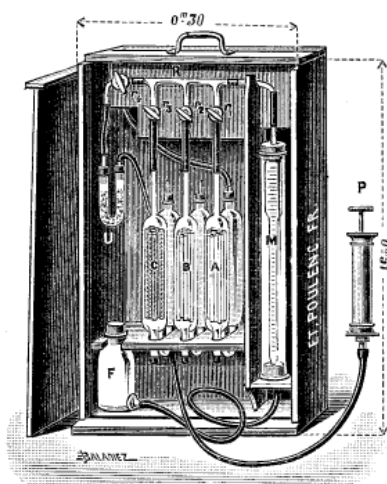
Fig. 3. — Appareil Orsat-Lunge, modèle Poulenc.
