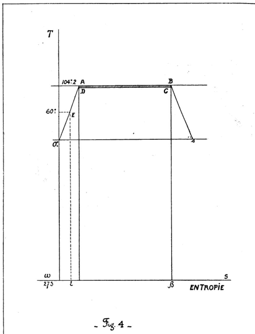
Fig. 4. — Diagramme entropique.
