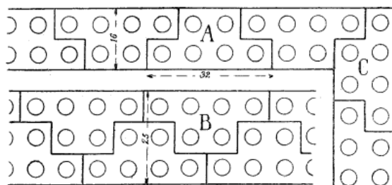
Fig. 1 et 2. — Assemblage des moellons agglomérés « Entur ».
