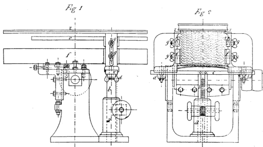
Planche B. — Fac-similé de la planche de dessins annexée à la demande d'addition, en date du 4 juillet 1918, au brevet d'invention pris le 7 juillet précédent par M. H. Vollet.
