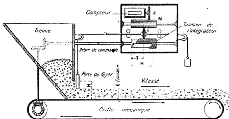
Fig. 76. — Compteur de charbon volumétrique « Lea coal meter ».
