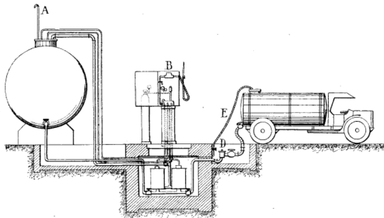
Fig. 13. — Installation de sécurité. Système Mauclère, à semi récupération de vapeurs, avec poste pouvant être utilisé indifféremment pour l'emmagasinage et le soutirage.
