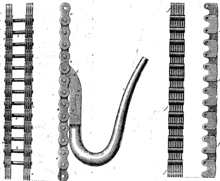
Fig. 58-59. — Chaine sans fin dite chaine Galle.
