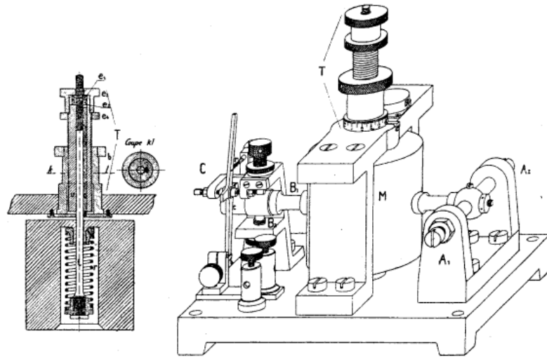
Fig. 3. — Modèle étudié par le Laboratoire d'Essais des Arts et Métiers permettant de faire agir le ressort à la traction ou à la compression de mesurer \pm \gamma .
