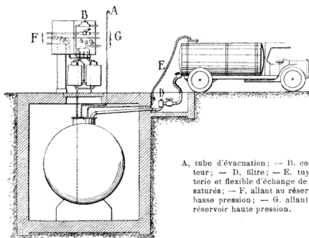
Fig. 10. — Installation de sécurité. Système Maclère, à récupération intégrale des vapeurs.
