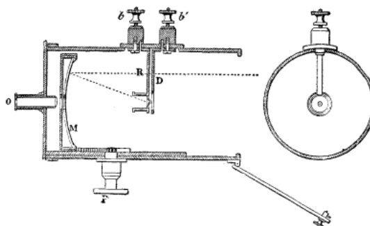
Fig. 34. — Pyromètre à radiation totale Féry (coupe).
