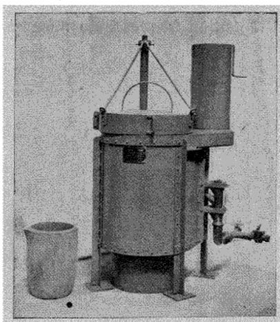
Fig. 3. — Four Méker.
