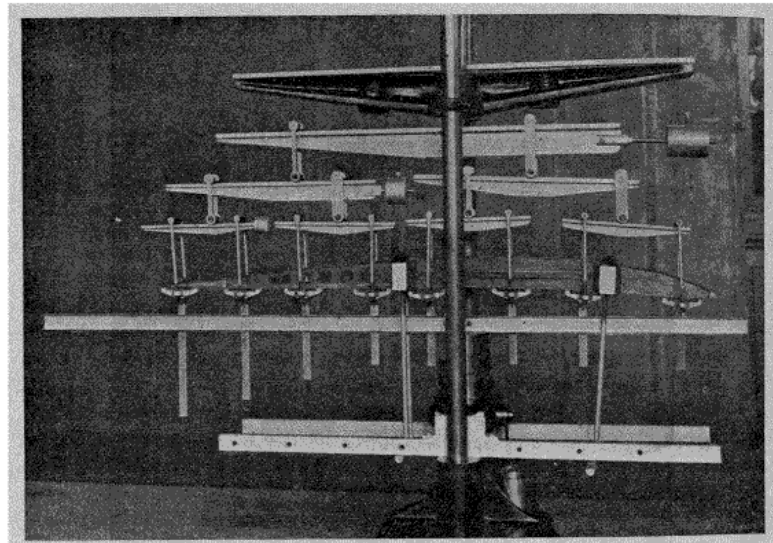
Fig. 5. — Appareil pour l'essai des nervures d'avions.
