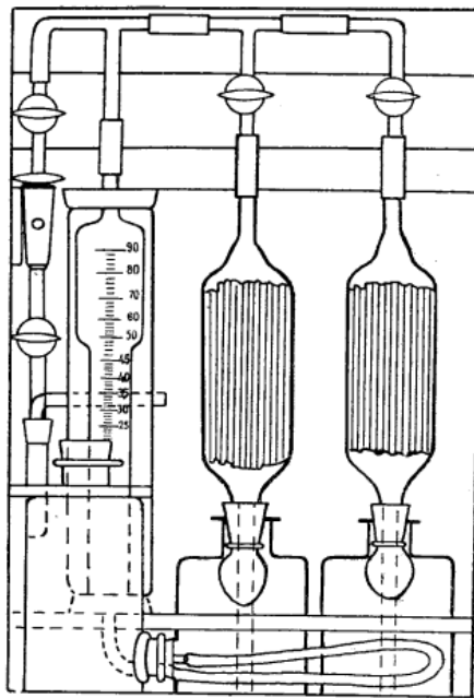
Fig. 1. — Appareil Orsat-Salleron à deux cloches.
