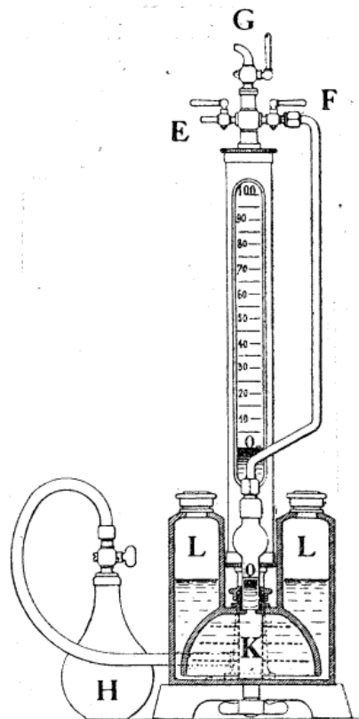
Fig. 6. — Coupe de l'analyseur Van Houtte.
