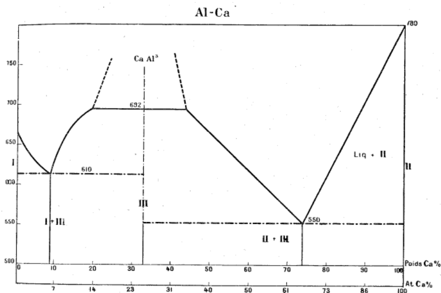
Fig. 41. — Diagramme des alliages Aluminium-Calcium.
