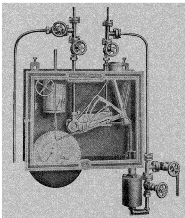
Fig. 64. — Compteur Gehre à compensateur.
