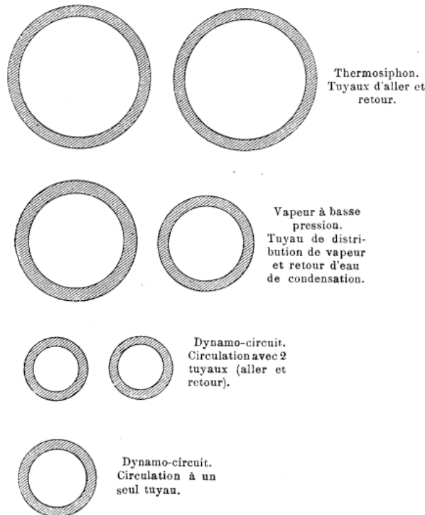
Fig. 13. — Comparaison entre les diamètres moyens des tuyauteries suivant les différents systèmes.
