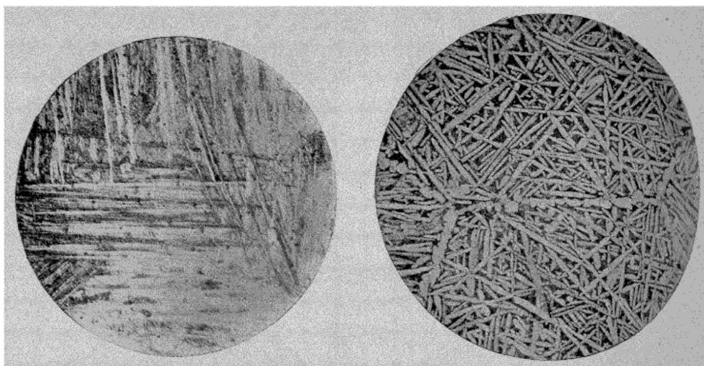
Fig. 33. — Bronze d'aluminium (Al = 11,9 p. 100). Trempé à 900°. Grossissement : 50 d. Fig. 34. — Bronze d'aluminium (Al = 9,95 p. 100). Trempé et revenu. Grossissement : 200 d (Portevin).
