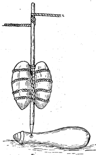
Fig. 74. — Tarière néo-zélandaise (d'après Chapman).
