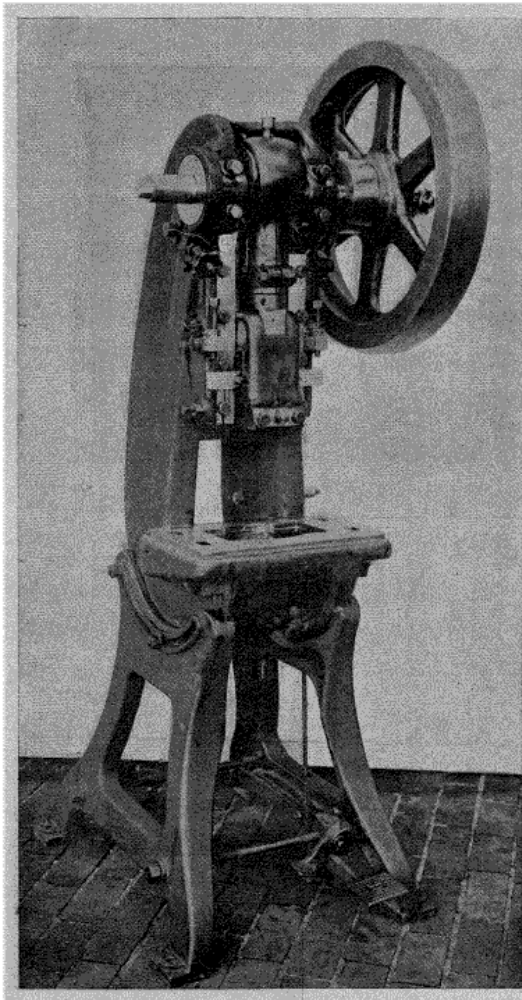
Fig. 8. — Presse Bliss.
