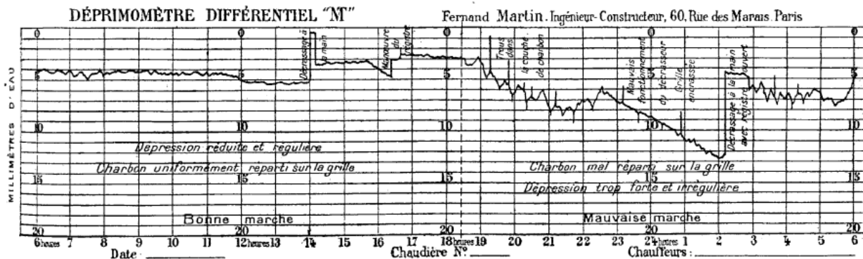
Fig. 48. — Diagramme de déprimomètre différentiel.
