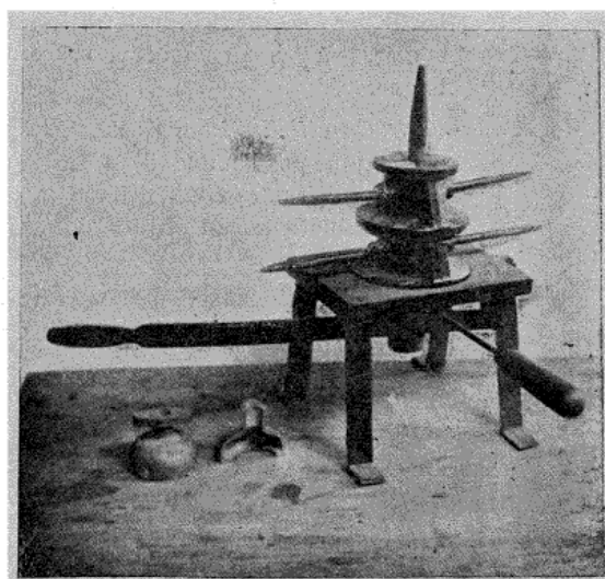
Fig. 5. — Boîte de remplissage d'huile (moule démonté, pièces coulées, dont l'une coupée par l'axe).
