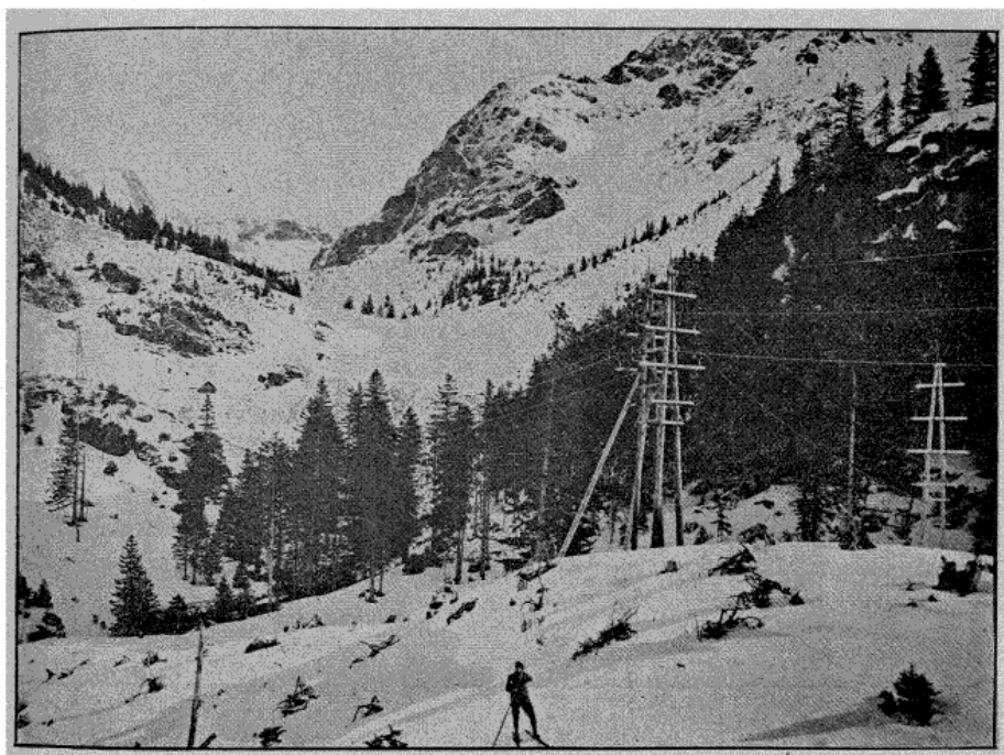
Fig. 11. — Une portée de 400 m à 1 600 m d'altitude.
