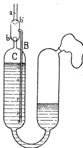
Fig. 4. — Élément barboteur à soupape automatique.
