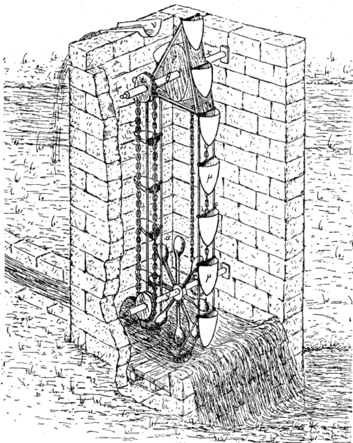
Fig. 52. — Roue hydraulique actionnant une noria à l'aide de poulies et de chaînes de transmission (Philon de Byzance, 2 siècles av. J.-C.).
