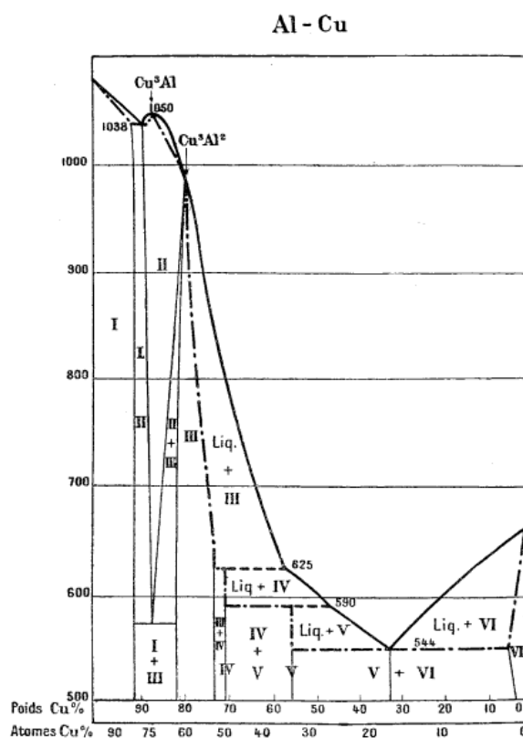
Fig. 6. — Diagramme des alliages Aluminium-Cuivre.
