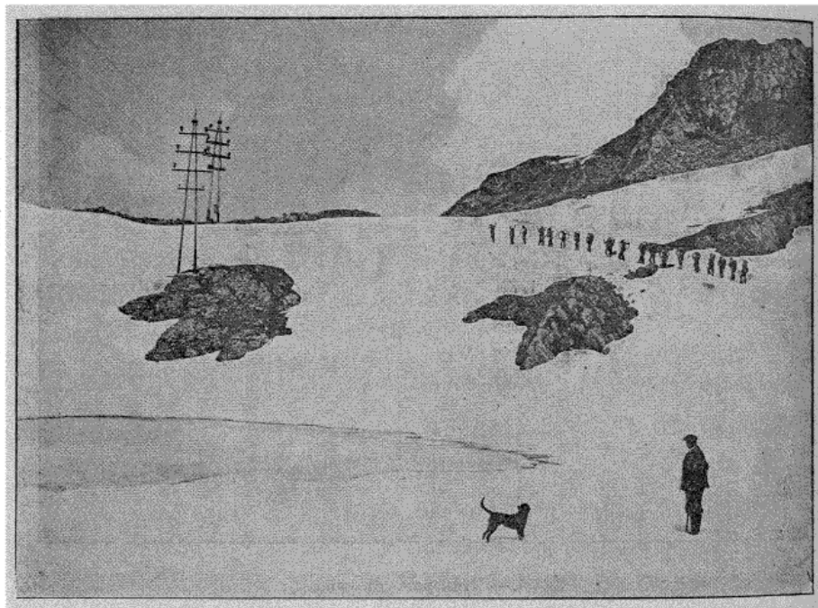
Fig. 8. — La ligne à 2.000 m d'altitude.
