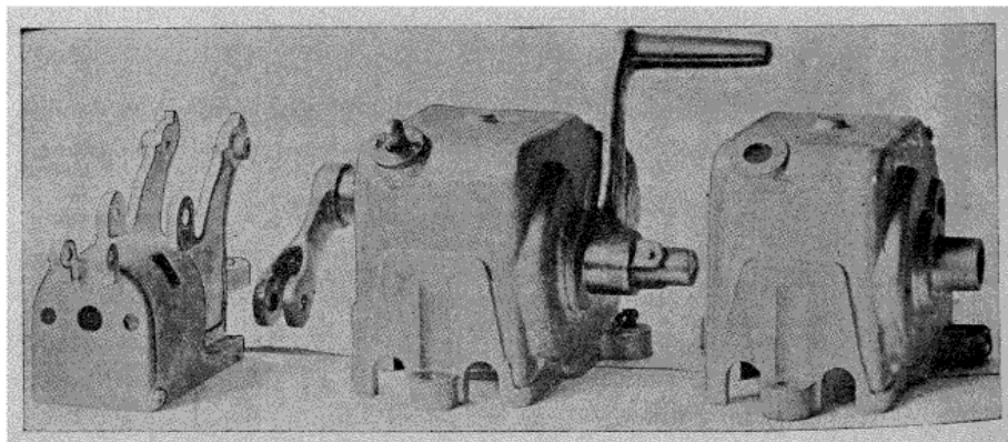
Fig. 21. — De gauche à droite : Bâti de disjoncteur unipolaire, type Neostyle; Mécanisme complet de disjoncteur type Carter; — Boîte de mécanisme de disjoncteur type Carter.
