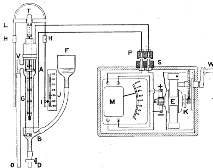
Fig. 84. — Analyseur « Dionic ».
