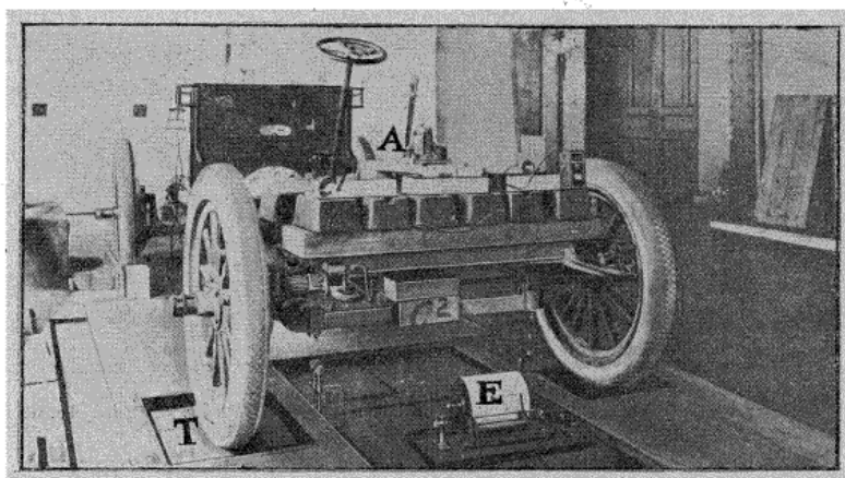
Fig. 11. — Essai d'une suspension d'automobile sur le chemin de roulement du Laboratoire des Arts et Métiers.
