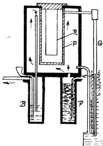
Fig. 26. — Schéma de l'analyseur Stérose.
