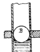
Fig. 60. — Détail du flotteur.
