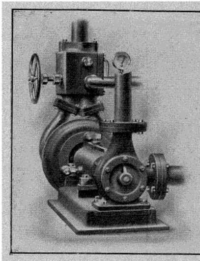
Fig. 2. — Groupe moteur-pompe.
