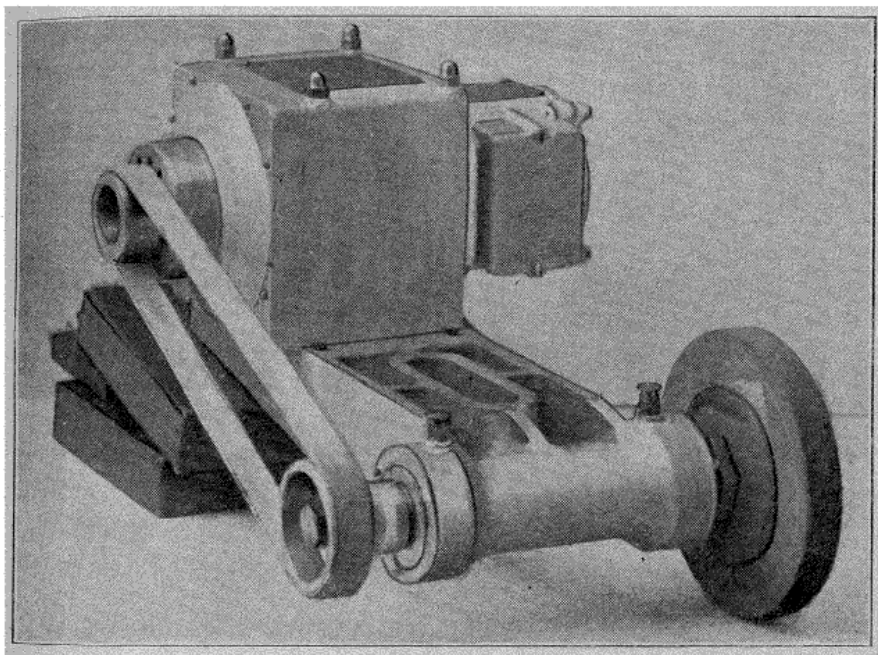
Fig. 1. — Rectifieuse portable électrique Volet (en aluminium).
