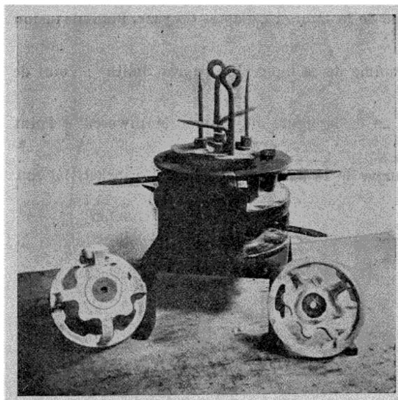
Fig. 1. — Dynamo-démarrreur, palier côté collecteur. (Moule monté, deux pièces coulées montrant les deux faces principales.)
