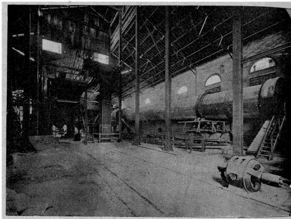
Fig. 4. — Four-séchoir à alumine (Usines de Salindres).
