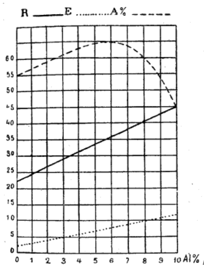
Fig. 23. — Caractéristiques mécaniques des alliages aluminium-cuivre.
