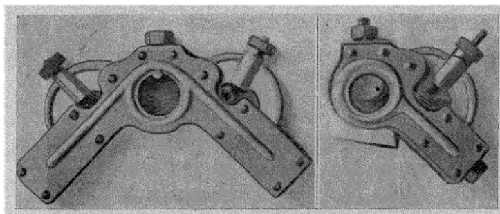
Fig. 36. — Porte-balais en aluminium.
