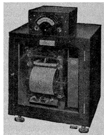
Fig. 11. — Galvanomètre enregistreur Cambridge.
