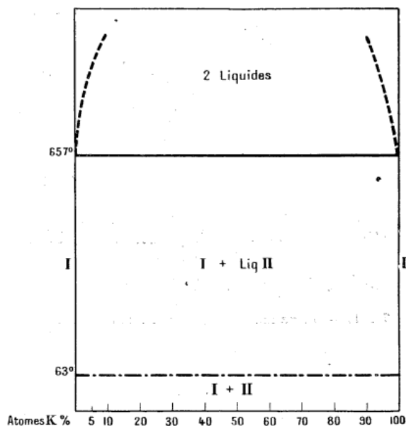
Fig. 43. — Diagramme des alliages Aluminium-Potassium.
