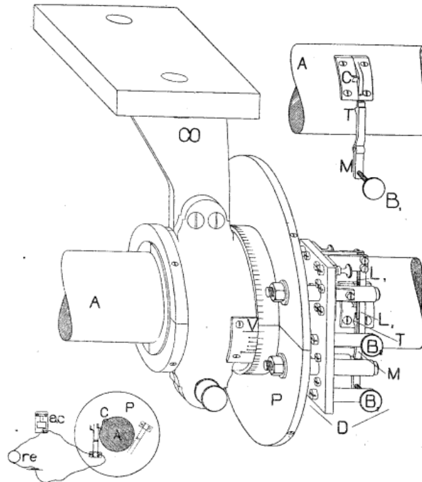
Fig. 14. — Sélecteur pour accéléromètre de rotation.
