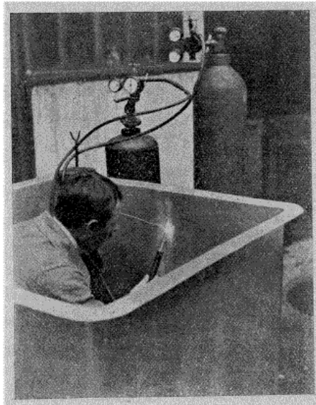
Fig. 8. — Soudure montante de l'aluminium.
