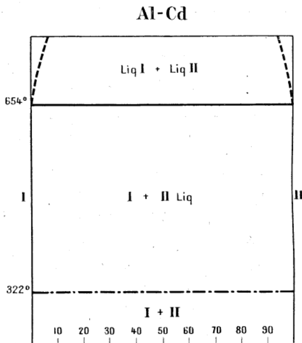
Fig. 13. — Diagramme des alliages Aluminium-Cadmium.
