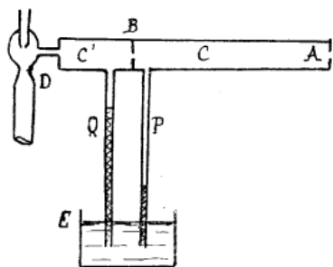
Fig. 25. — Principe de l'analyseur Uehling.
