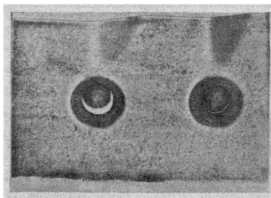
Fig. 9. — Plissements latéraux de la bande emboutie, le métal a godé par suite de la compression à la flexion.
