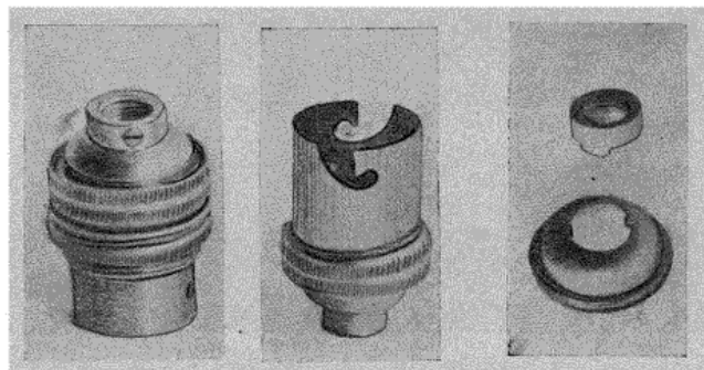
Fig. 13. — Supports de lampes montés. Support embouti. Support avec culot à raccord décolleté.
