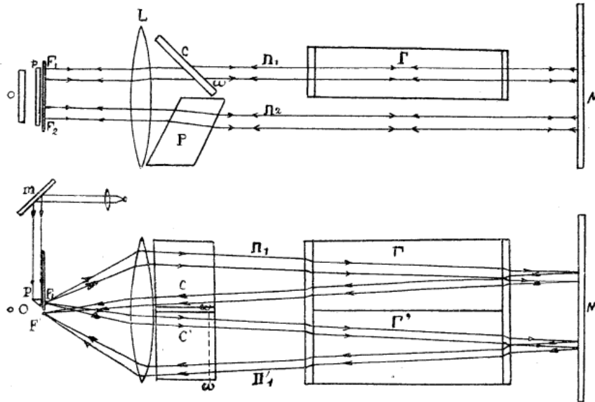
Fig. 12. — Schéma du réfractomètre de lord Rayleigh.
