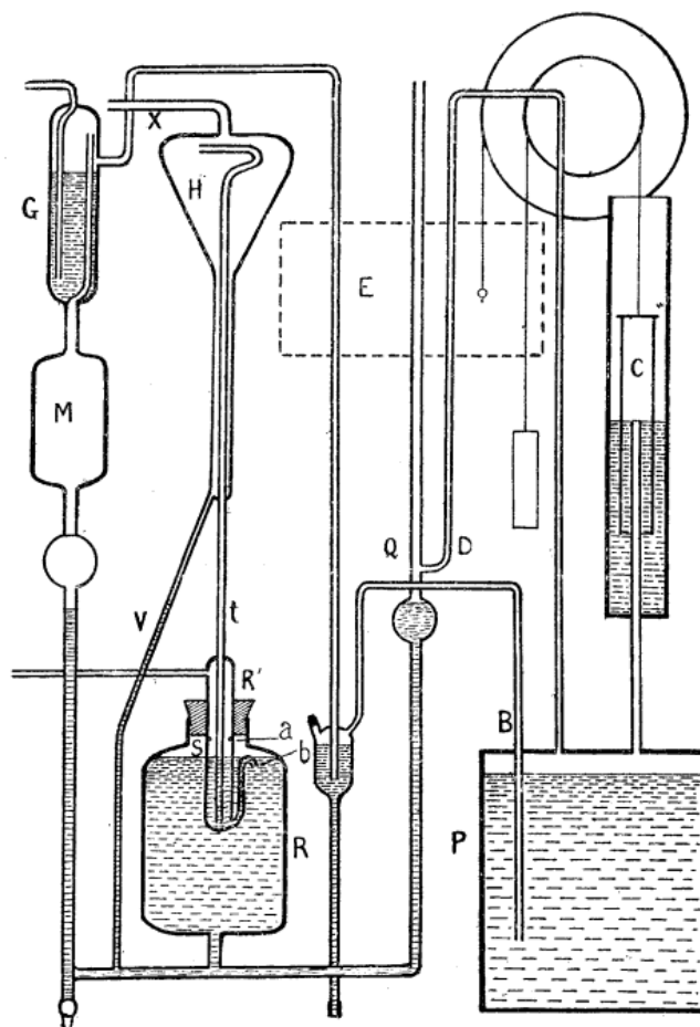
Fig. 21. — Analyseur automatique Mono.
