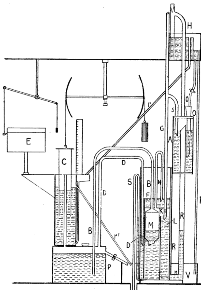
Fig. 20. — Analyseur automatique Simmance et Abady.
