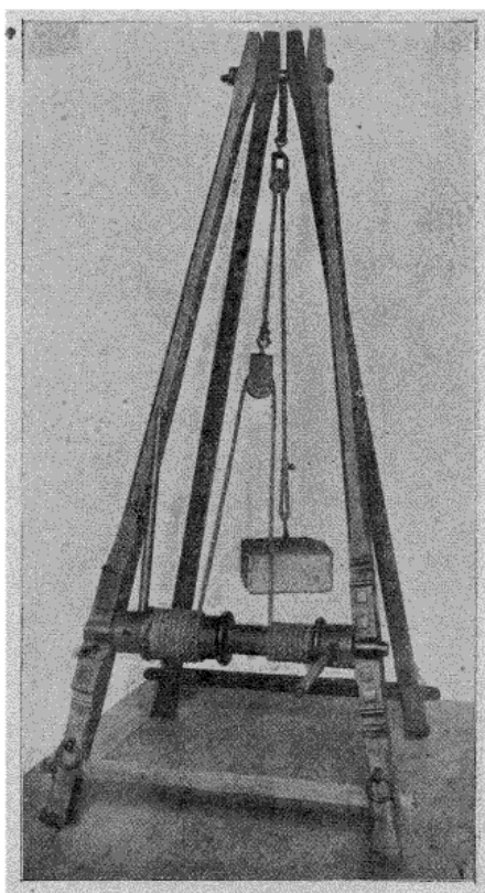
Fig. 88. — Chèvre chinoise avec treuil différentiel (Conservatoire des Arts et Métiers, n° 1122).
