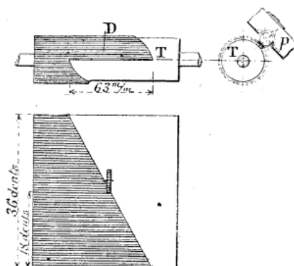
Fig. 73. — Dispositif d'intégration automatique.
