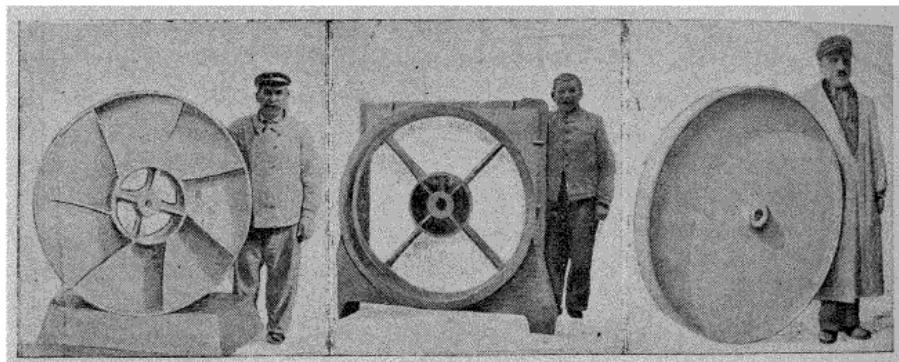
Fig. 2. — Rotor de ventilateur en aluminium, poids : 50 kg.
