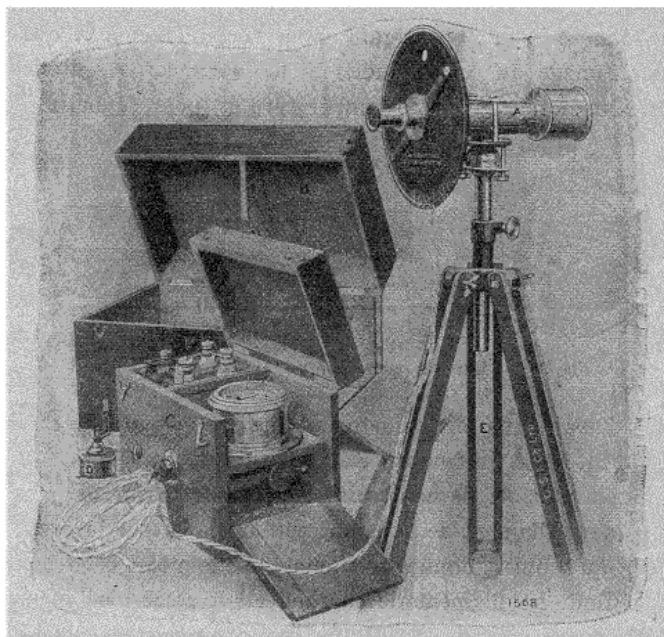
Fig. 38. — Pyromètre optique Cambridge.
