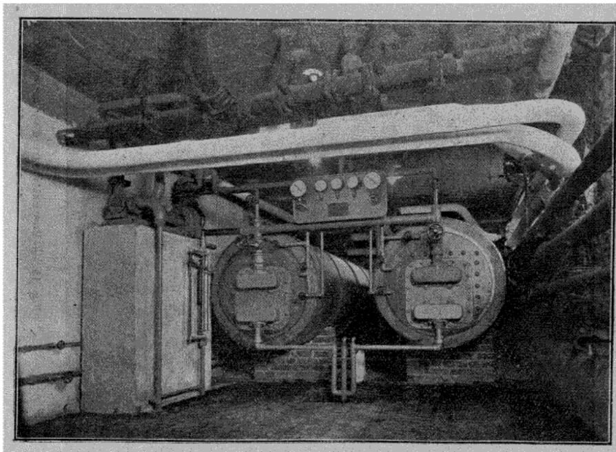
Fig. 14. — Appareils de production et de distribution d'eau chaude dans un hôpital.
