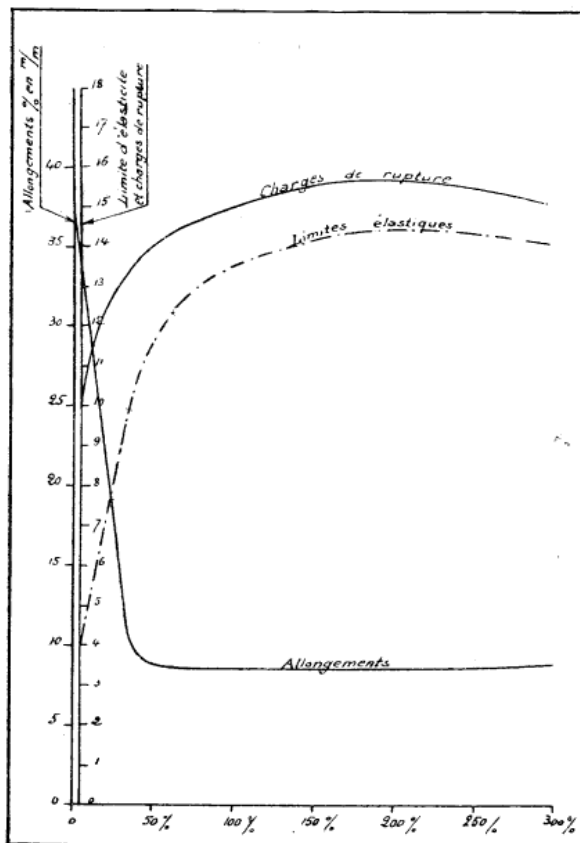
Fig. 18. — Variation des caractéristiques mécaniques (R, E, A) de l'aluminium en fonction du degré d'écroutissage (Grad).
