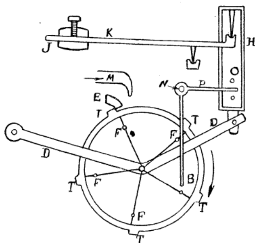
Fig. 75. — Schéma du compteur de charbon Martin.
