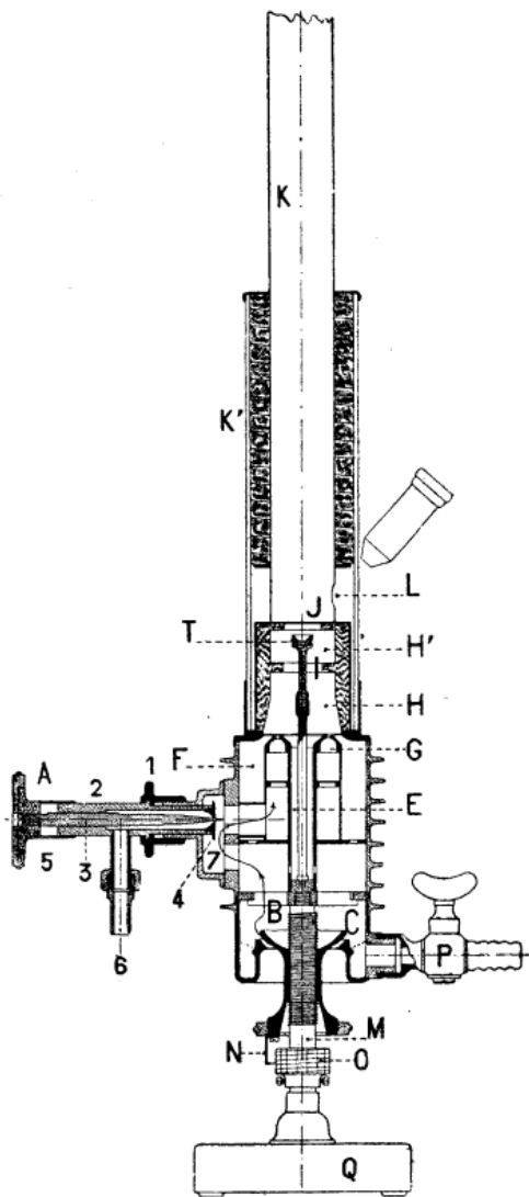
Fig. 83. — Comburimètre Grebel (coupe verticale).
