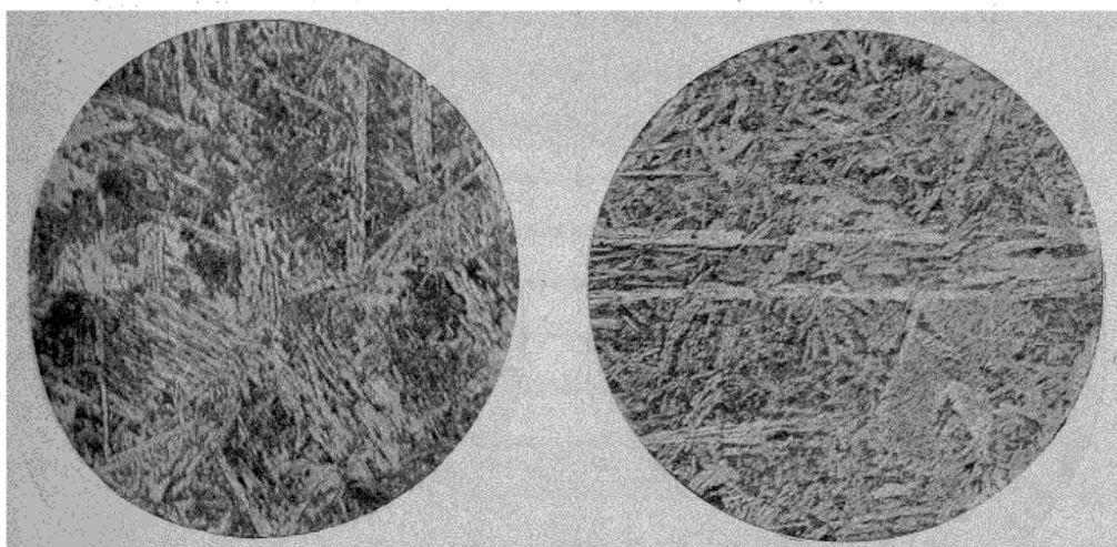
Fig. 31. — Bronze d'aluminium (Al = 9,5 p. 100). Fig. 32. — Bronze d'aluminium Al = 11,9 p. 100). Trempe à 950°. Trempe à 800°. Grossissement : 200 d. Grossissement : 200 d.
