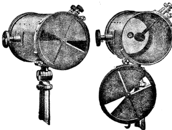
Fig. 33. — Pyromètre télescopique Féry à diaphragme basculant.
