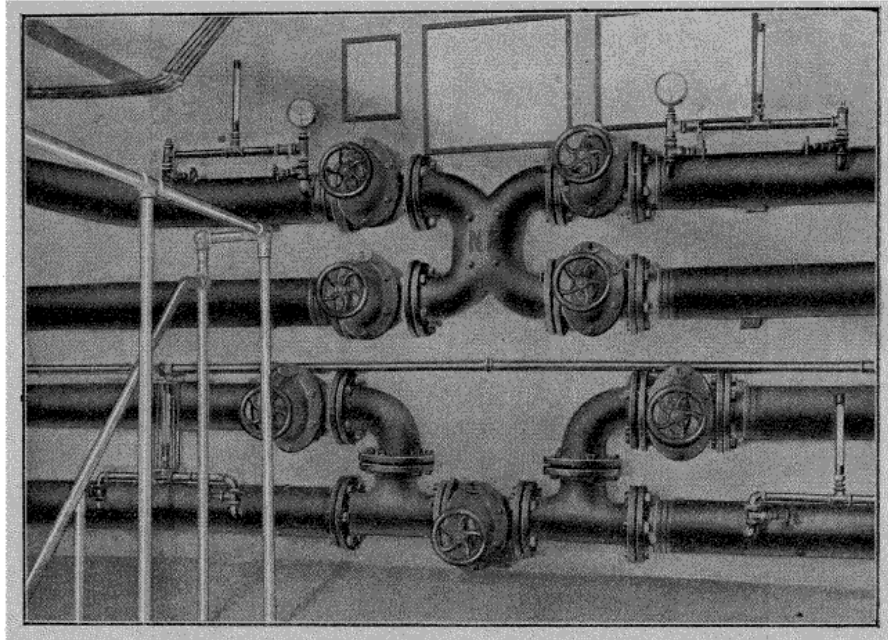
Fig. 17. — Tuyauteries et vannes d'intercommunication entre deux groupes de circulation.
