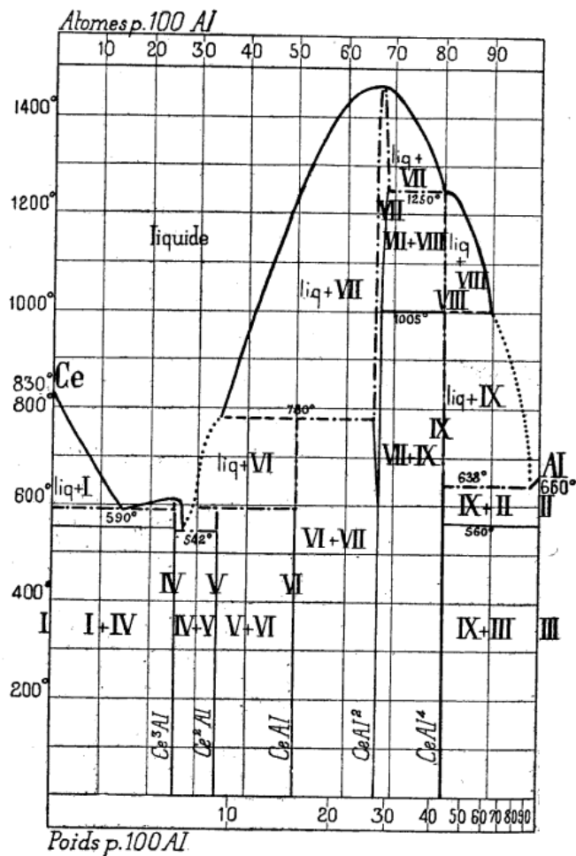
Fig. 10 ter. — Diagramme des alliages Aluminium-Cérium.
