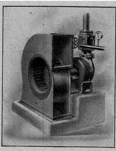
Fig. 3. — Ventilateur centrifuge actionné par turbine à vapeur.
