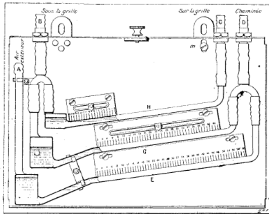
Fig. 42. — Déprimomètre différentiel Alba.
