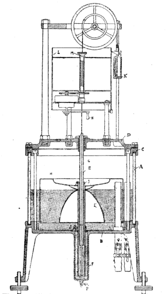
Fig. 57. — Débitmètre Intégra.
