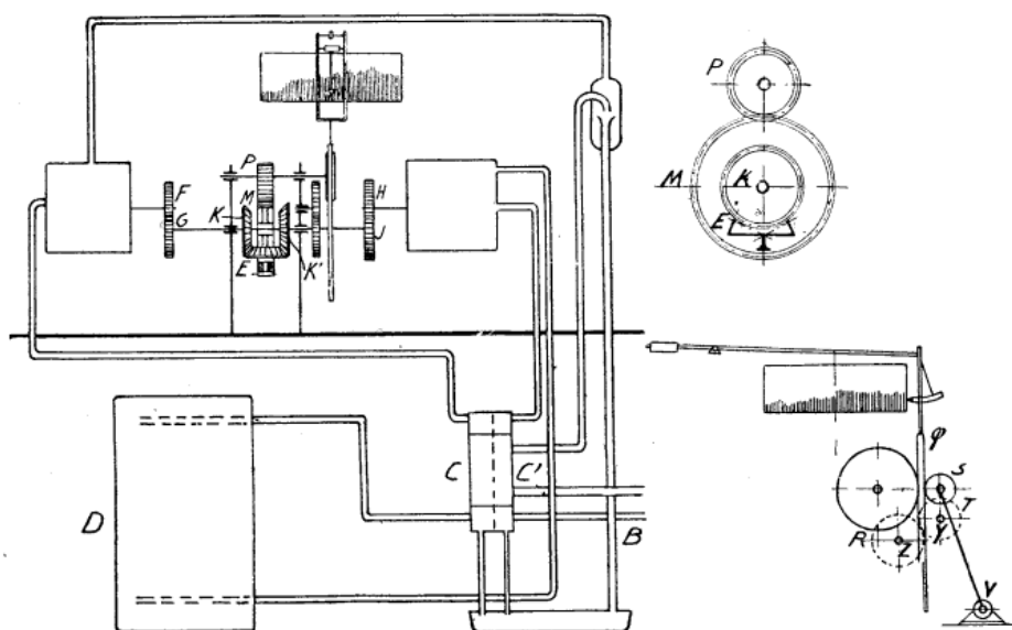
Fig. 24. — Analyseur automatique Pintsch Bayer.
