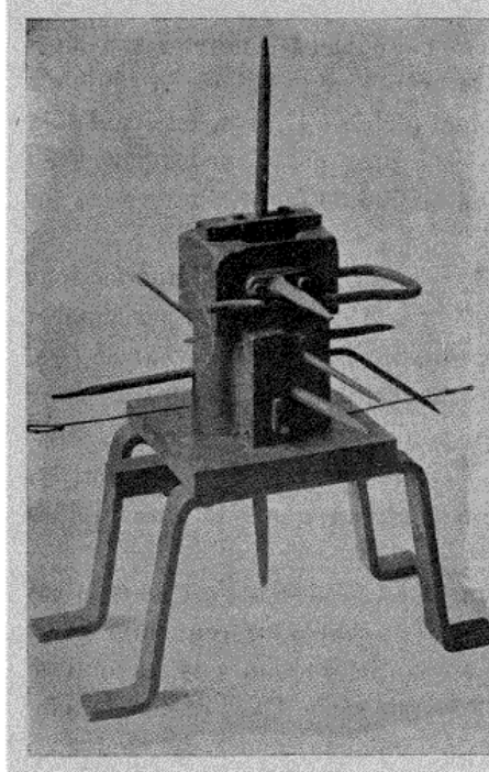
Fig. 1. — Coquille à mouler l'aluminium, fermée.
