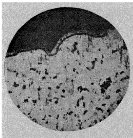
Fig. 10. — Coupe d'un tube de fer calorisé.
