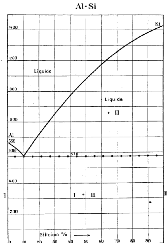
Fig. 1. — Diagramme des alliages Aluminium-Silicium.
