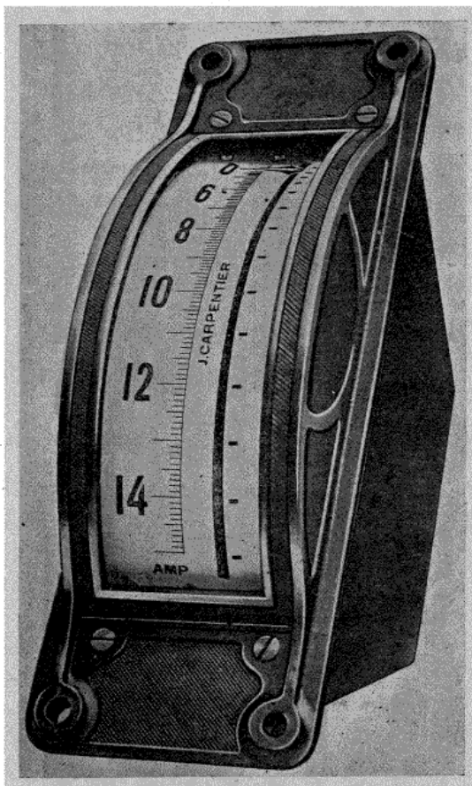
Fig. 52. — Ampermètre de profil Carpentier à bâti d'aluminium.
