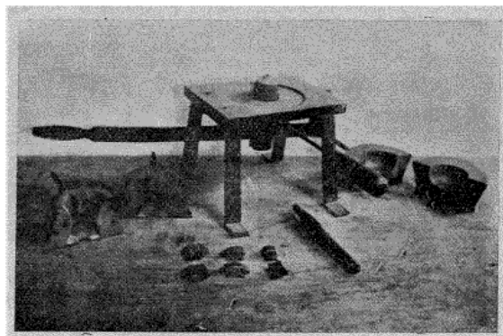
Fig. 6. — Boîte de remplissage d'huile (moule démonté avec parties démontables).
