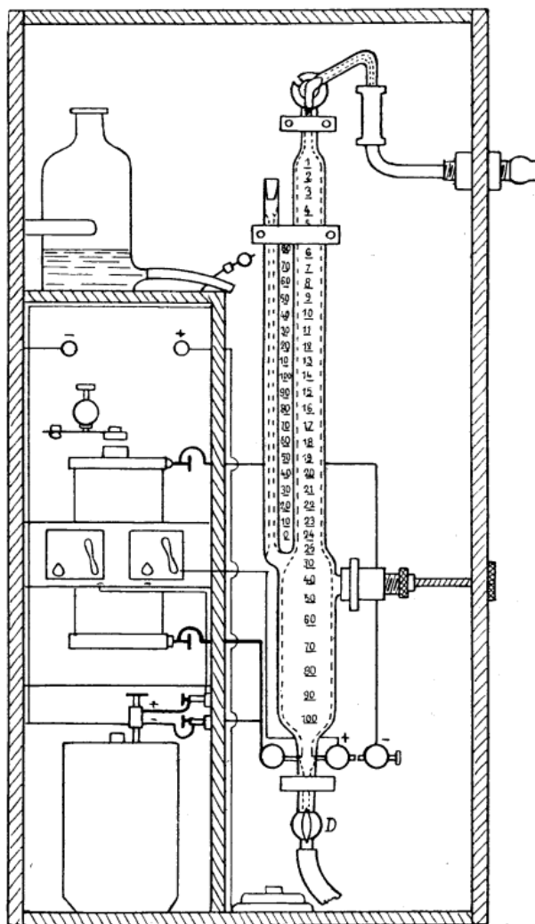
Fig. 81. — Calorimètre Union.
