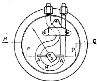
Fig. 59. — Coupe schématique du manomètre Piette.
