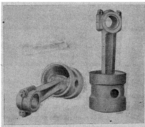
Fig. 7. — Assemblage de pistons et bielles d'aluminium.
