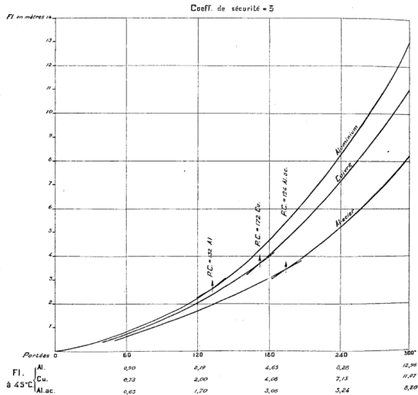
Fig. 2. — Flèches maxima à 45^{\circ} de câbles équivalents en cuivre, en aluminium et en aluminium-acier.
