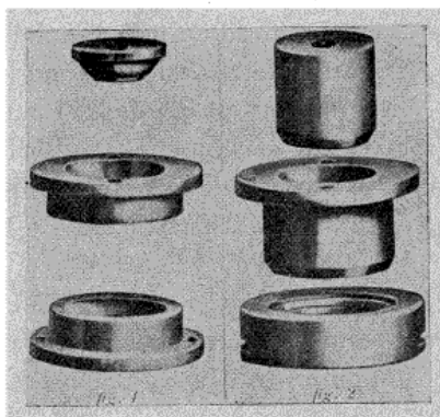
Fig. 3. — Accessoires d'emboutissage.
