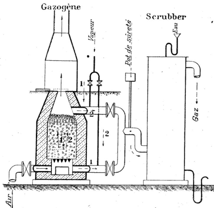
Fig. 9. — Schéma de l'appareil Dellwick-Fleischer. Gaz non carburé.
