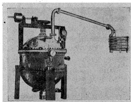
Fig. 13. — Autoclave avec agitateur mécanique et serpentin condenseur.
