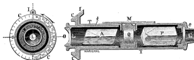
Fig. 39. — Lunette pyroscopique de Mesuré et Nouel.
