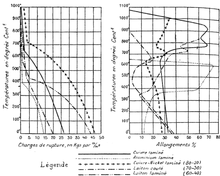
Fig. 16 et 17. — Variation de la charge de rupture et de l'allongement de l'aluminium et de différents métaux en fonction de la température.
