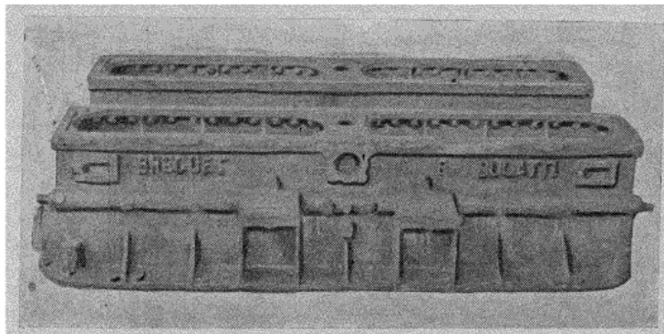
Fig. 9. — Carter en magnésium pour moteur d'avion Bugatti-Breuet de 500 ch.
