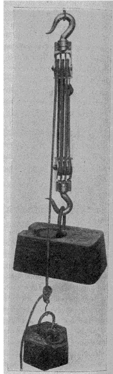
Fig. 89-90. — Mesure de l'effort de traction sur un palan, pour monter une charge de poids connu.
