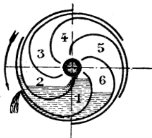
Fig. 70. — Schéma du tambour du compteur Reiser. : position B.
