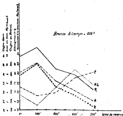
Fig. 25. — Influence du revenu sur un bronze d'aluminium trempé à 800°.
