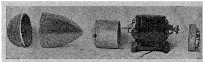
Fig. 33. — Moteur universel et pièces détachées.
