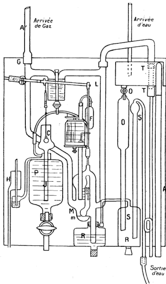
Fig. 14. — Appareil Ados simple.
