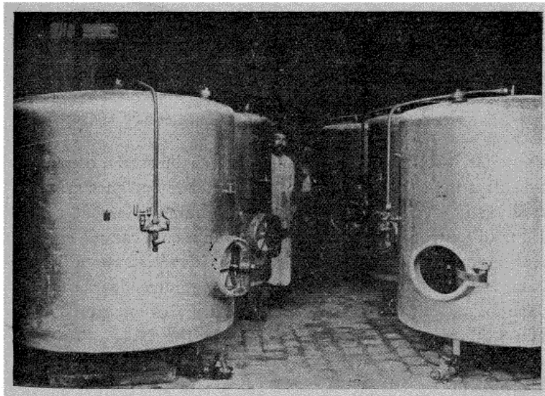
Fig. 12. — Cave avec tanks de brasserie en aluminium (Établissements Odam).
