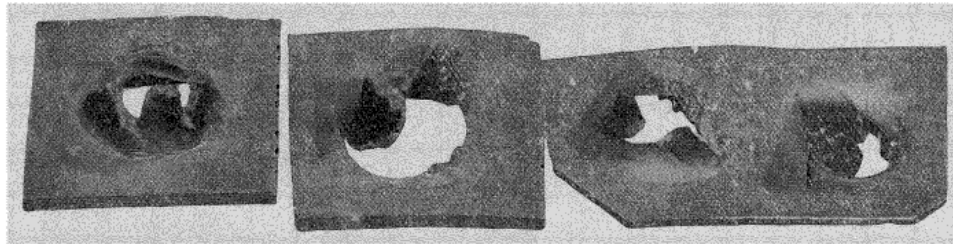
Fig. 14 à 17. — Essais d'emboutissage dynamiques de bronzes durs.
