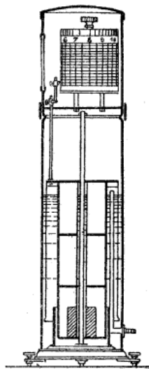
Fig. 44. — Coupe d'un déprimomètre à cloche.
