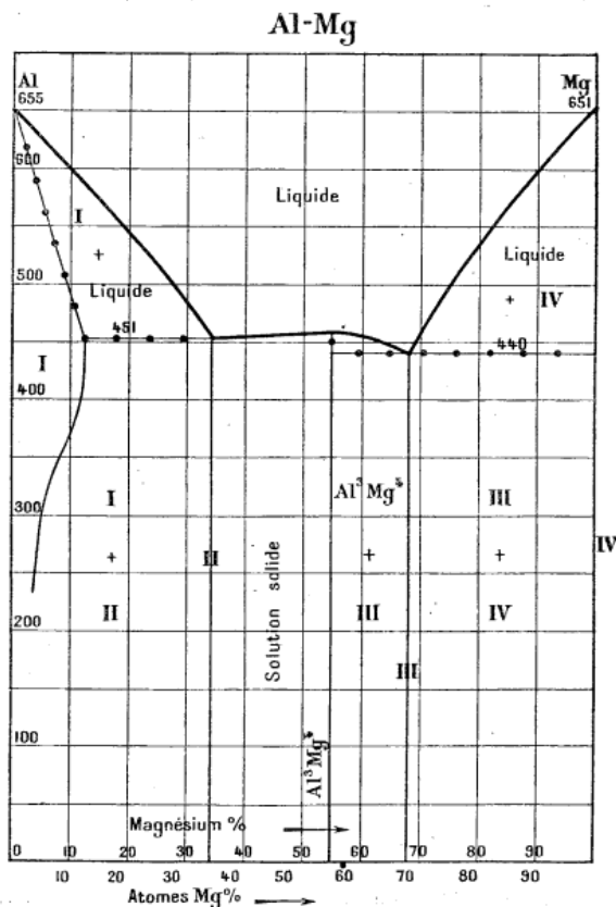
Fig. 3. — Diagramme des alliages Aluminium-Magnésium.
