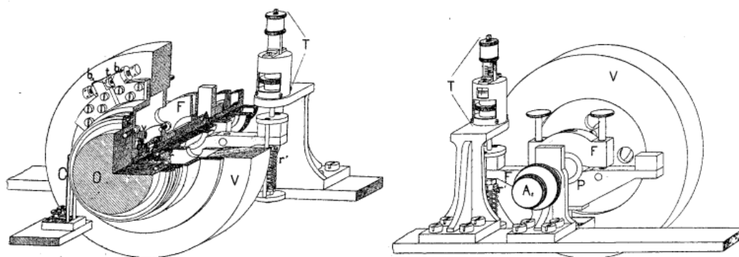
Fig. 12 et 13. — Accéléromètre de rotation. — Modèle construit au Laboratoire de M. Königs.
