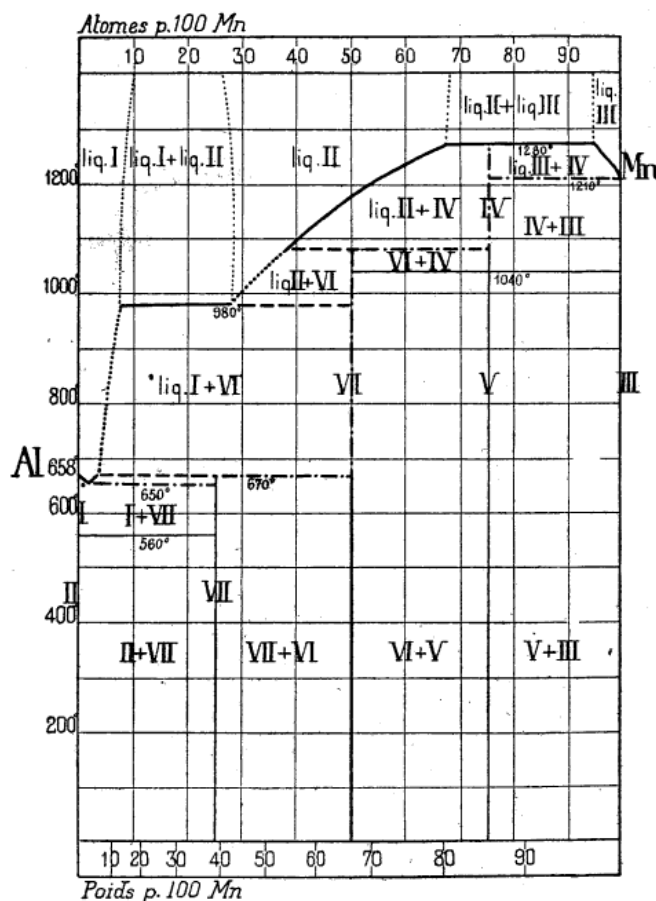
Fig. 12 bis. — Diagramme des alliages Aluminium-Manganèse.
