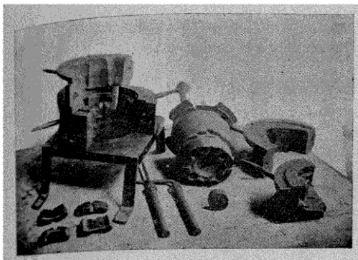
Fig. 2. — Dynamo-démarreur, côté collecteur (moule partiellement démonté).
