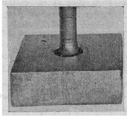
Fig. 4. — Poinçon et matrice pour essai d'emboutissage.
