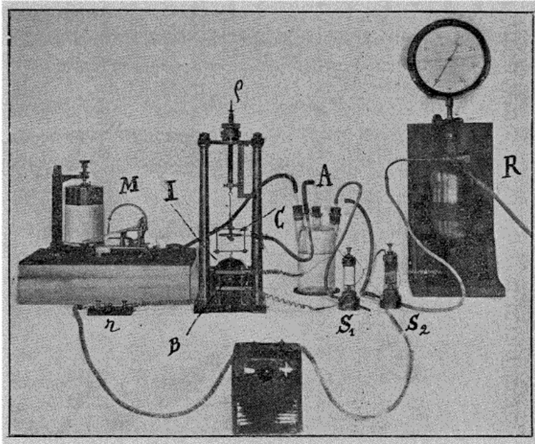
Fig. 15. — Accéléromètre enregistreur (appareil d'étude exécuté au Laboratoire des Arts et Métiers et au Laboratoire de M. Kœnigs).
