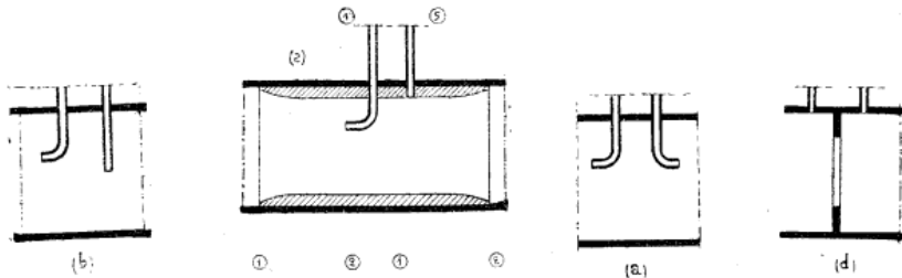
Fig. 50. — Tube de Pitot.
