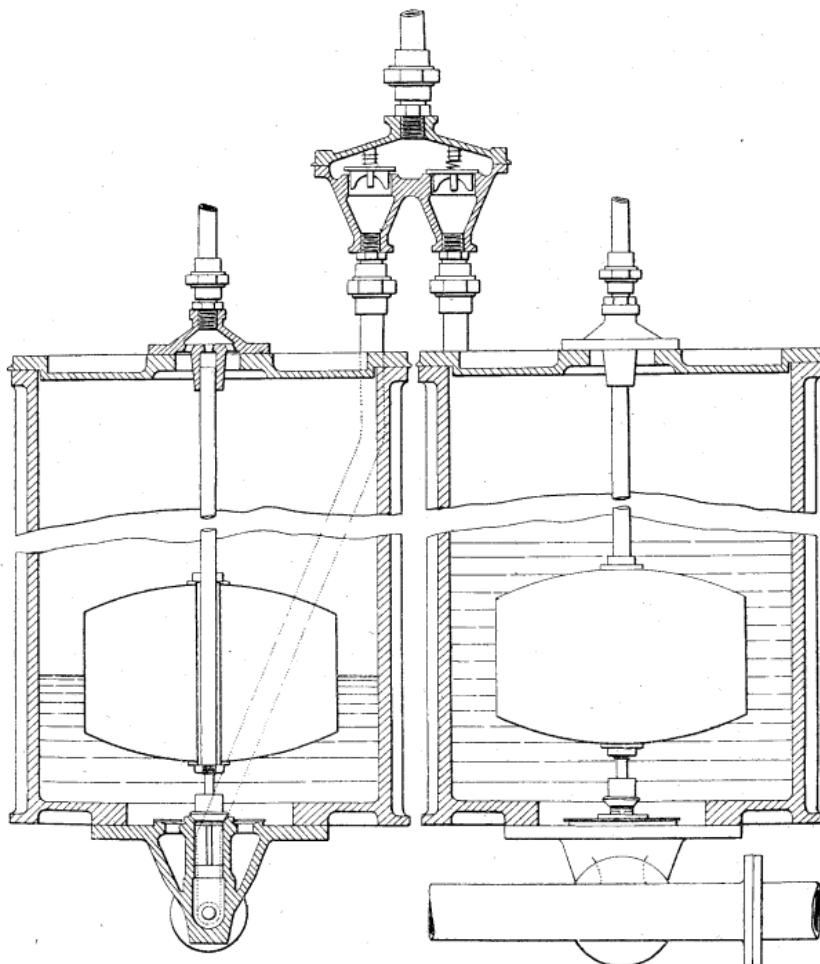
Fig. 2. — Ensemble du groupe des deux réservoirs conjugués.
