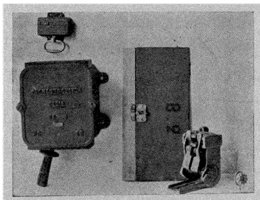
Fig. 56. — Signal d'alarme. Interrupteur, verrou et porte-balai.
