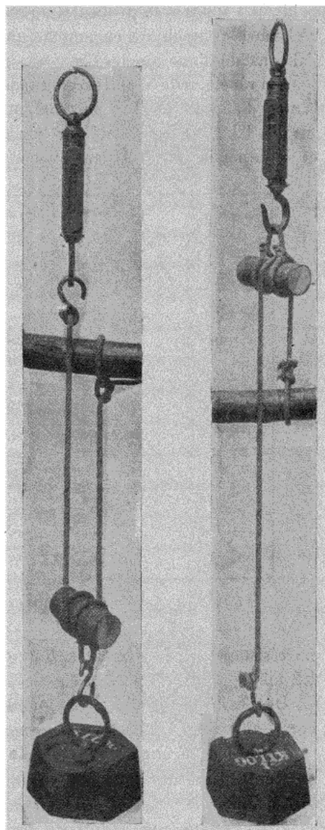
Fig. 27. — Levier funiculaire du deuxième genre.
