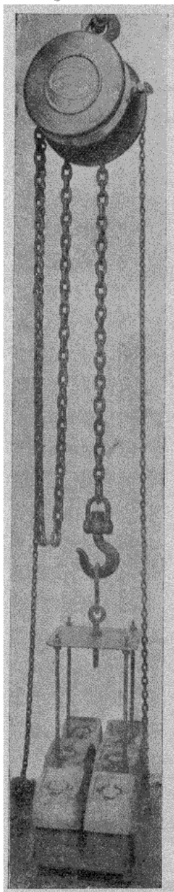
Fig. 94. Palan à engrenages.
