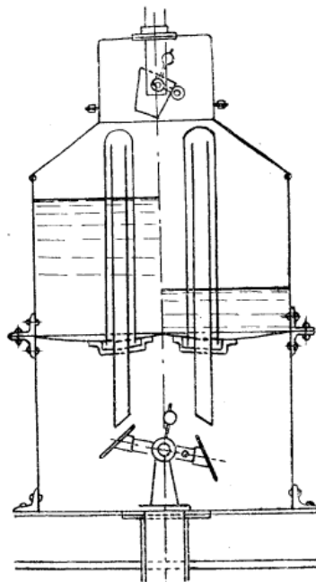
Fig. 71. — Compteur d'eau à siphon intermittent Martin.
