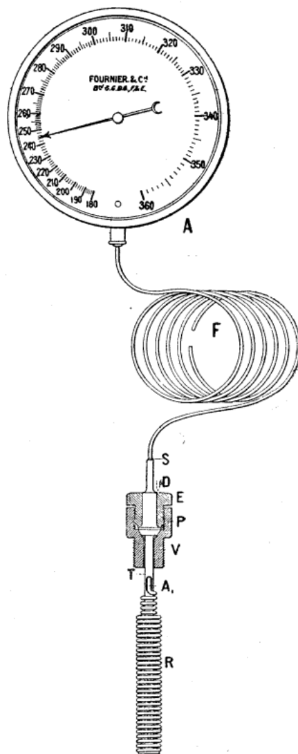
Fig. 32. — Pyromètre Fournier pour vapeur surchauffée.
