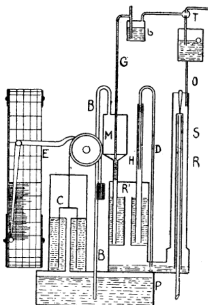
Fig. 18. — Schéma de l'appareil Eckardt.
