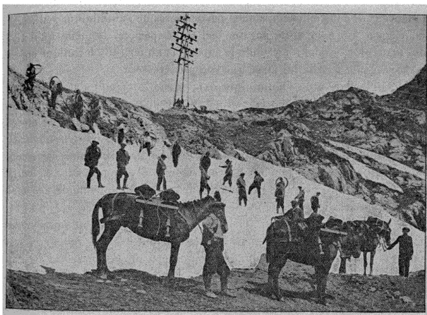
Fig. 6. — Transport du câble et des isolateurs.
