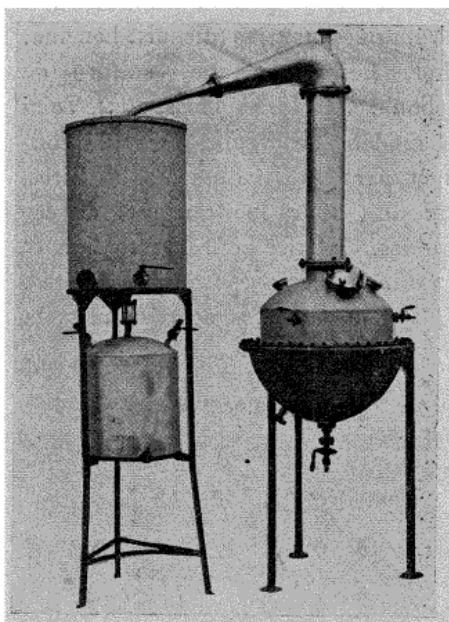
Fig. 14. — Appareil pour la distillation des essences (Odam et C ie ).
