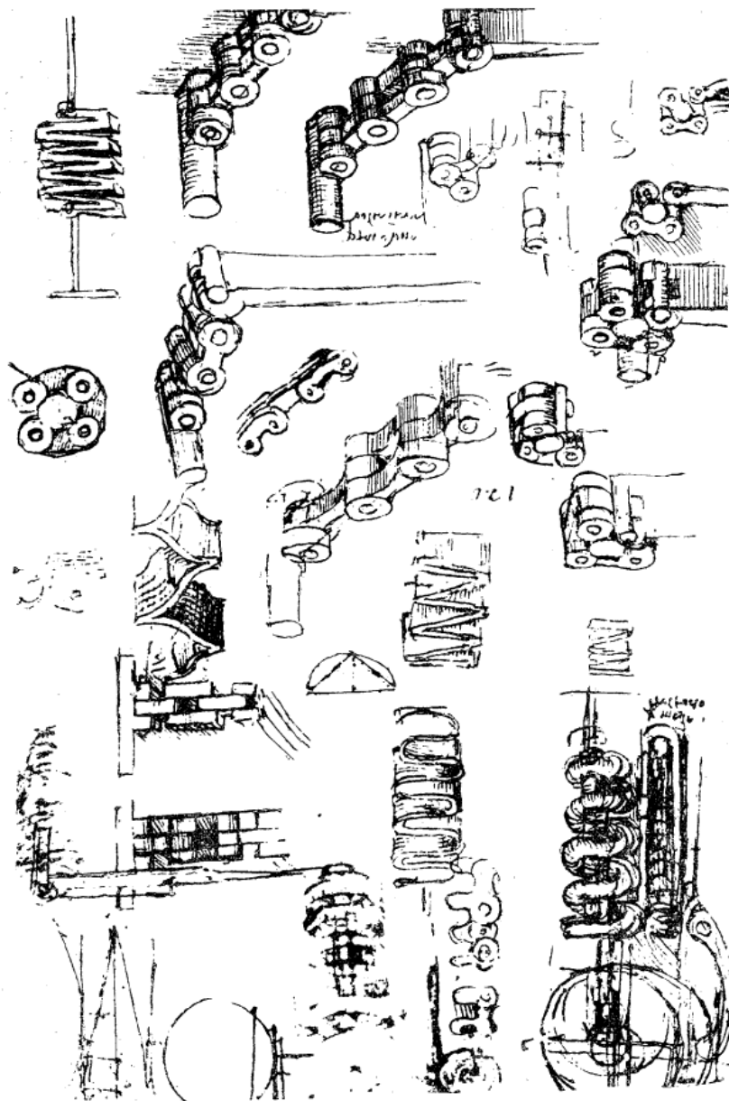
Fig. 57. — Chaines à maillons superposés de Léonard de Vinci.
