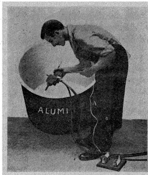
Fig. 9. — Métallisation d'une cuve en aluminium.
