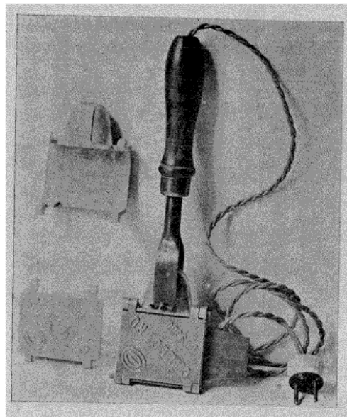
Fig. 30. — Fer à souder électrique à monture d'aluminium.
