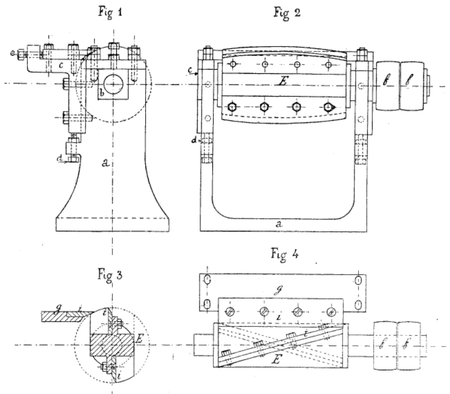
Planche A. — Fac-similé de la planche de dessins annexée à la demande de brevet d'invention de M. H. Vollet, en date du 7 juillet 1917.
