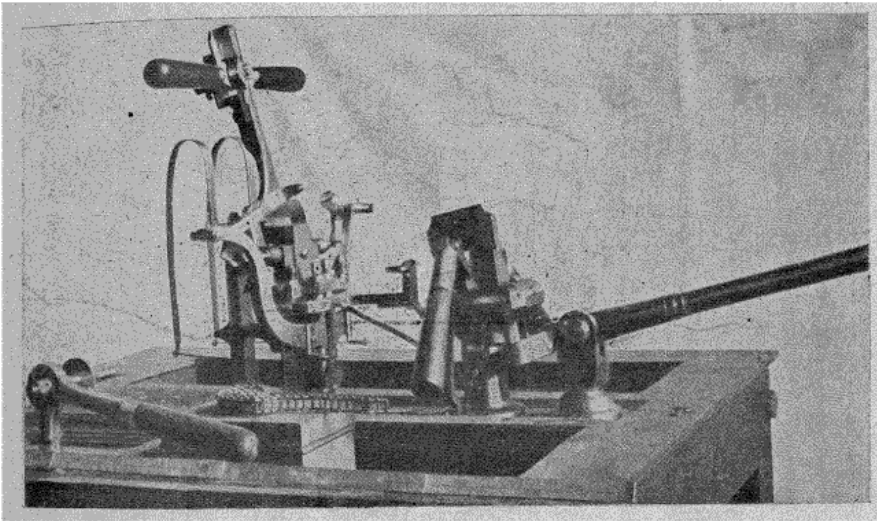
Fig. 56. — Machine imaginée par Vaucanson pour fabriquer la chaîne à maillons articulés et de forme rectangulaire (Conservatoire des Arts et Métiers, n° 6).
