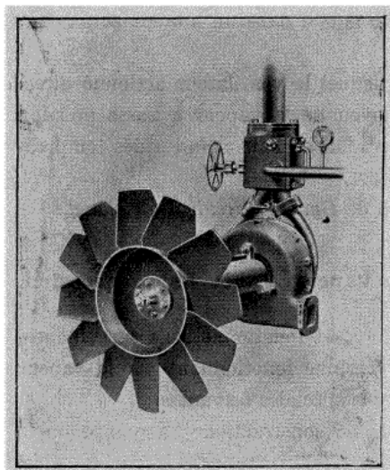
Fig. 1. — Groupe moteur-ventilateur.
