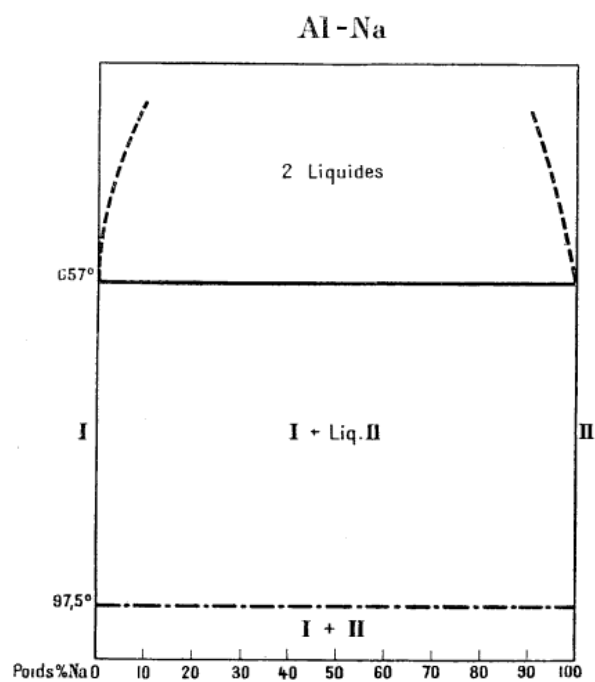
Fig. 16. — Diagramme des alliages Aluminium-Sodium.
