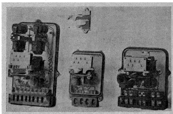
Fig. 45. — Compteurs électriques.
