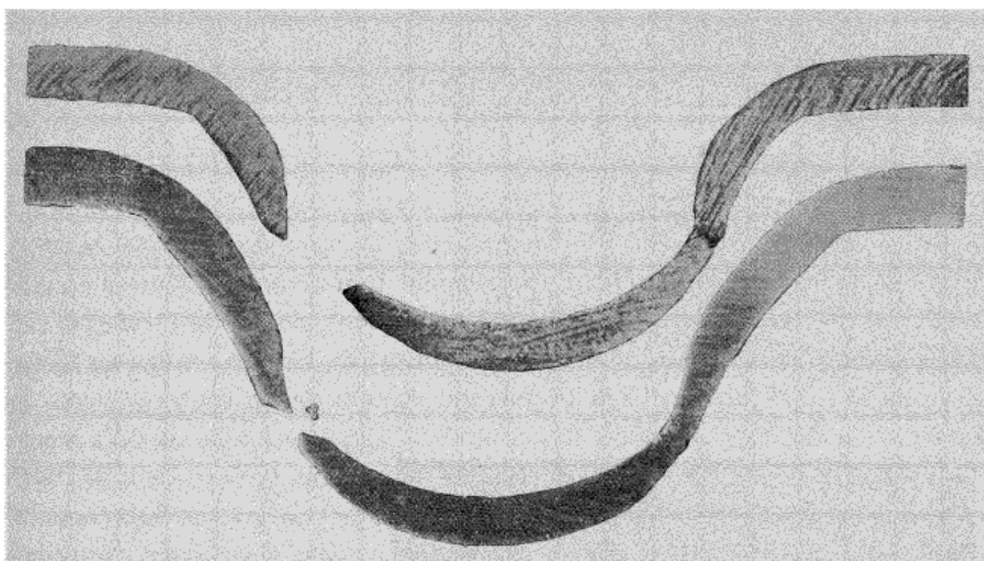
Coupes d'emboutissage montrant les déformations du métal.
