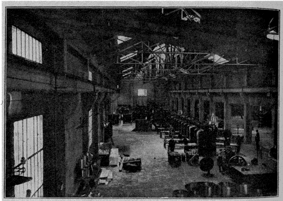
Fig. 21. — Série de petits laminoirs à aluminium de l'usine de Chambéry (Société de l'Aluminium français).
