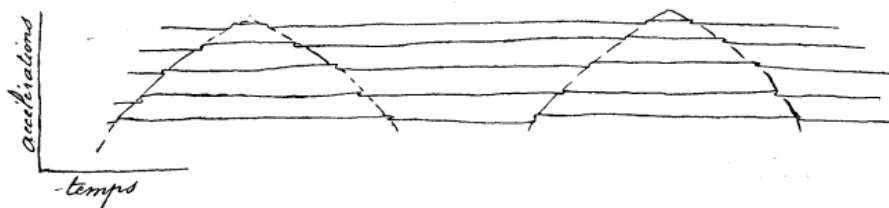
Fig. 9. — Enregistrement d'un mouvement sinusoïdal simple.
