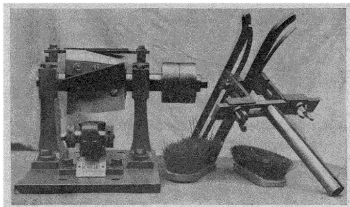
Fig. D. — Vue perspective des dispositions de la machine de M. H. Vollet. La machine sans ses protecteurs : dispositif montrant séparément le montage des couteaux et le système de guidage des brosses à travailler.
