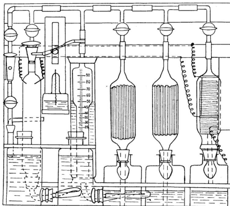
Fig. 2. — Appareil Orsat complet, modèle de l'O. C. C. R.
