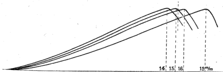
Fig. 5. — Dix grammes superposés de 4 emboutissages successifs effectués avec le même poinçon et avec des matrices de 14, 15, 16, 19 mm de diamètres.
