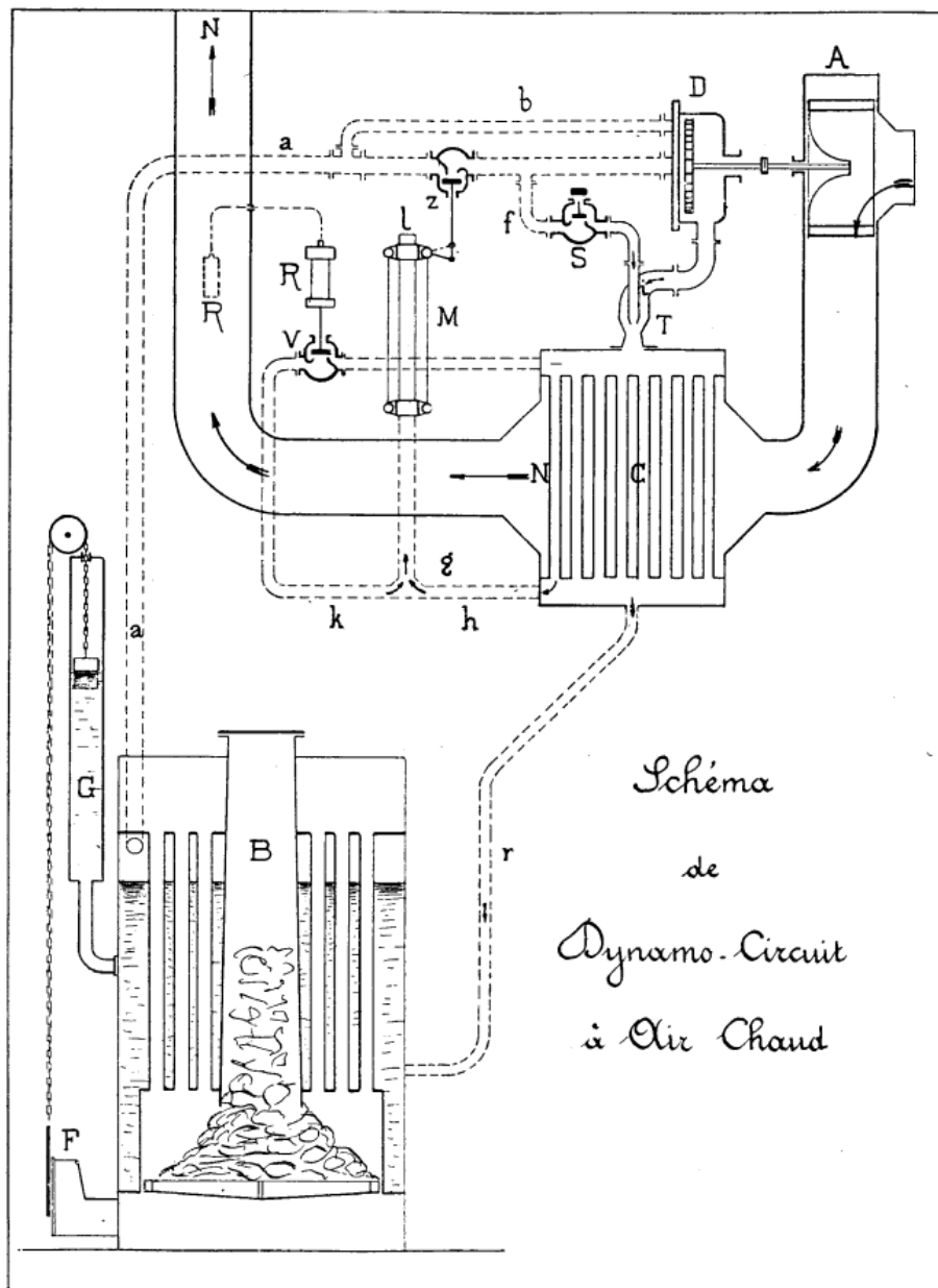
Fig. 20. — Schéma de dynamo-circuit à air chaud.
