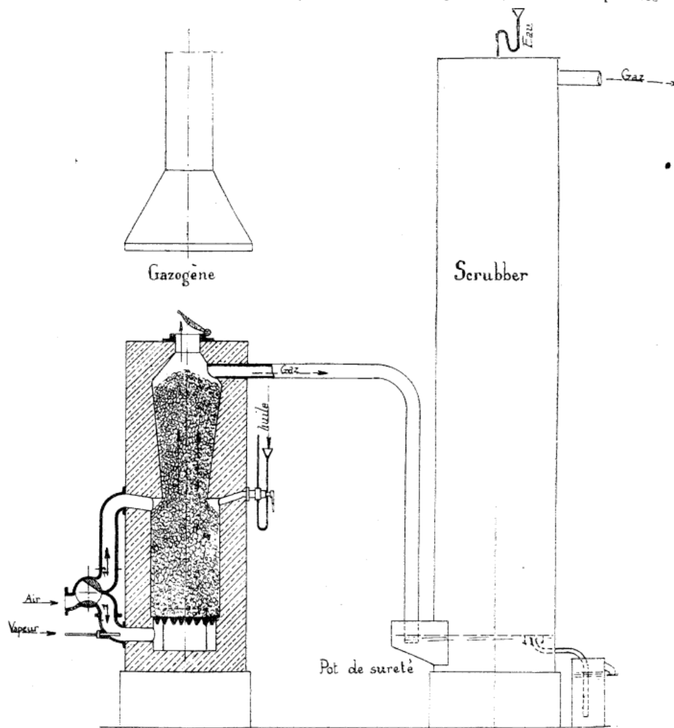
Fig. 8. — Schéma de l'appareil de la Société de Construction d'Appareils pour Gaz à l'eau. Gaz carburé.
