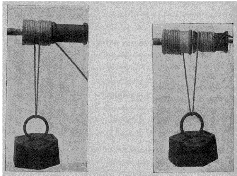
Fig. 87. — Treuil différentiel produisant un effet utile.
