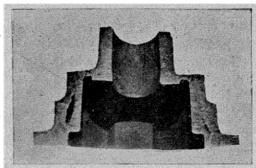
Fig. 35. — Pièce en bronze d'aluminium avec soufflure.
