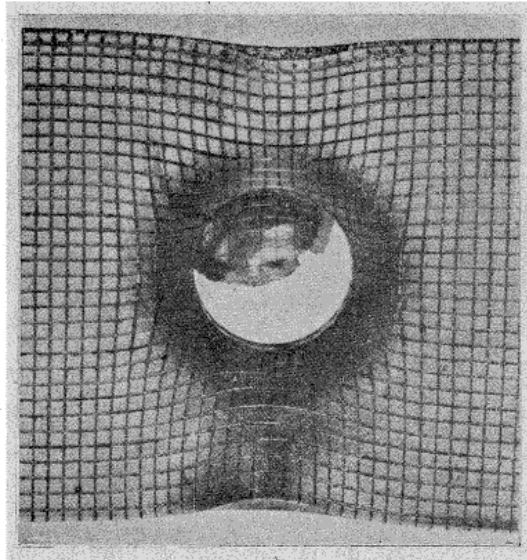
Fig. 10. — Déformation latérale dans l'emboutissage.
