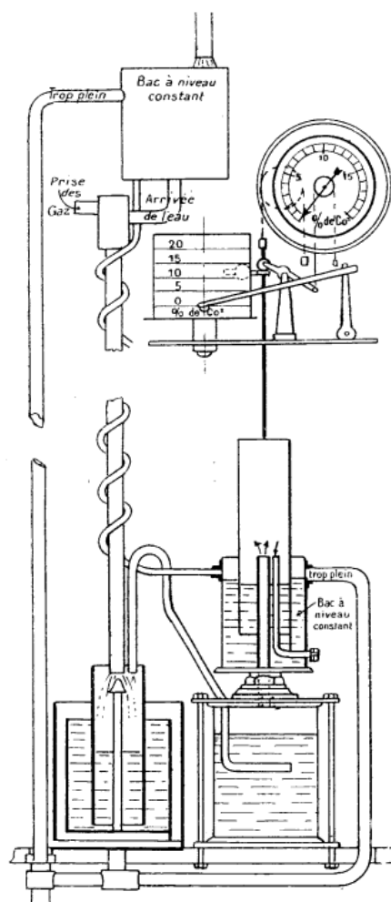
Fig. 27. — Analyseur automatique Maxant-Berger.
