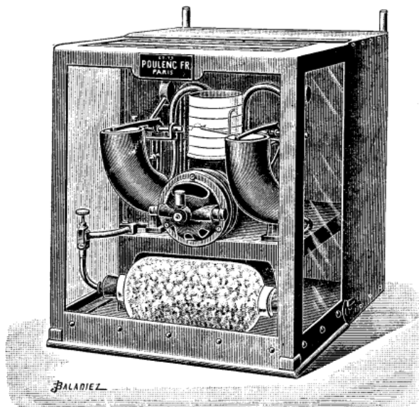
Fig. 22. — Analyseur automatique Brenot-Poulenc.
