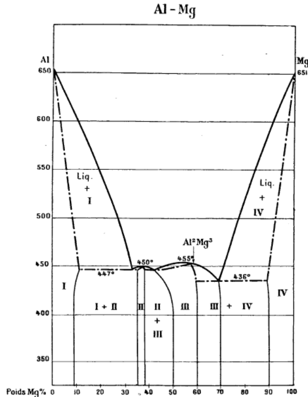
Fig. 4. — Diagramme des alliages Aluminium-Magnésium (dernières déterminations).
