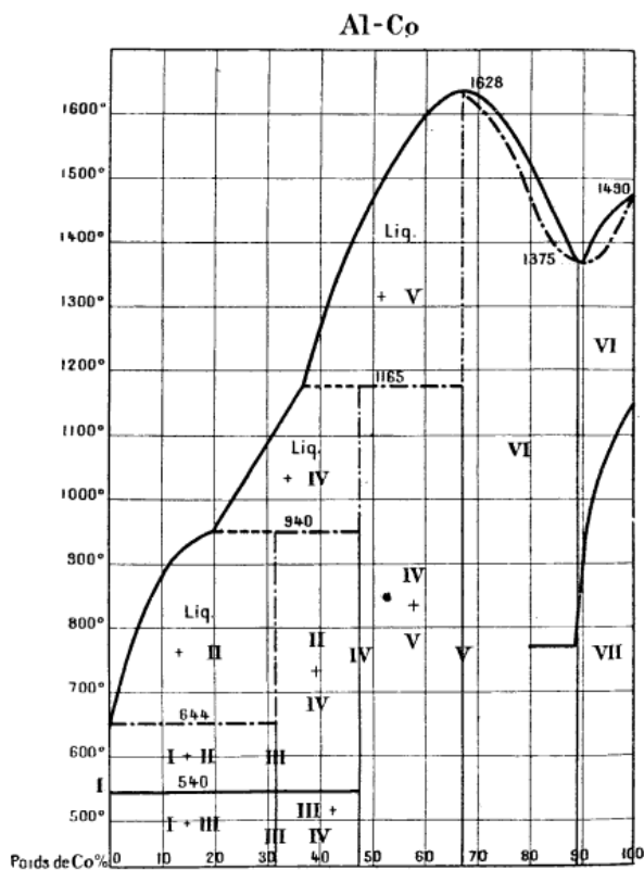
Fig. 8. — Diagramme des alliages Aluminium-Cobalt.
