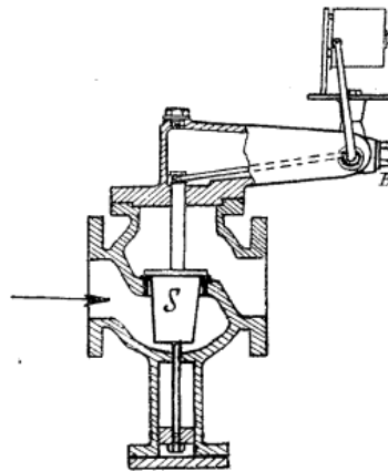
Fig. 62. — Compteur de vapeur Claassen.
