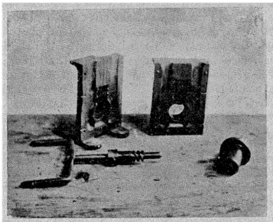
Fig. 11. — Collier de la vis de commande d'accélérateur (Moule démonté, montrant la vis formant noyau).
