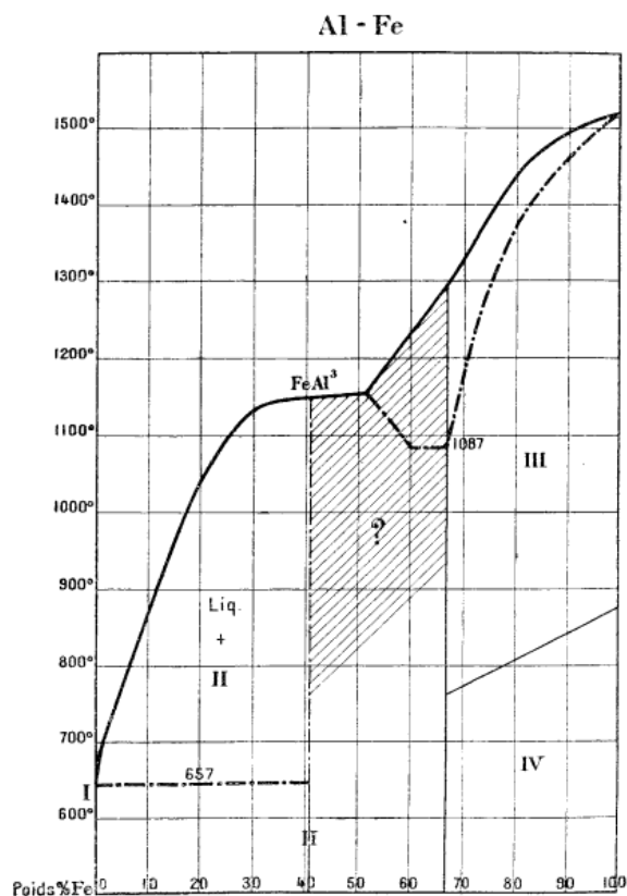
Fig. 10. — Diagramme des alliages Aluminium-Fer.
