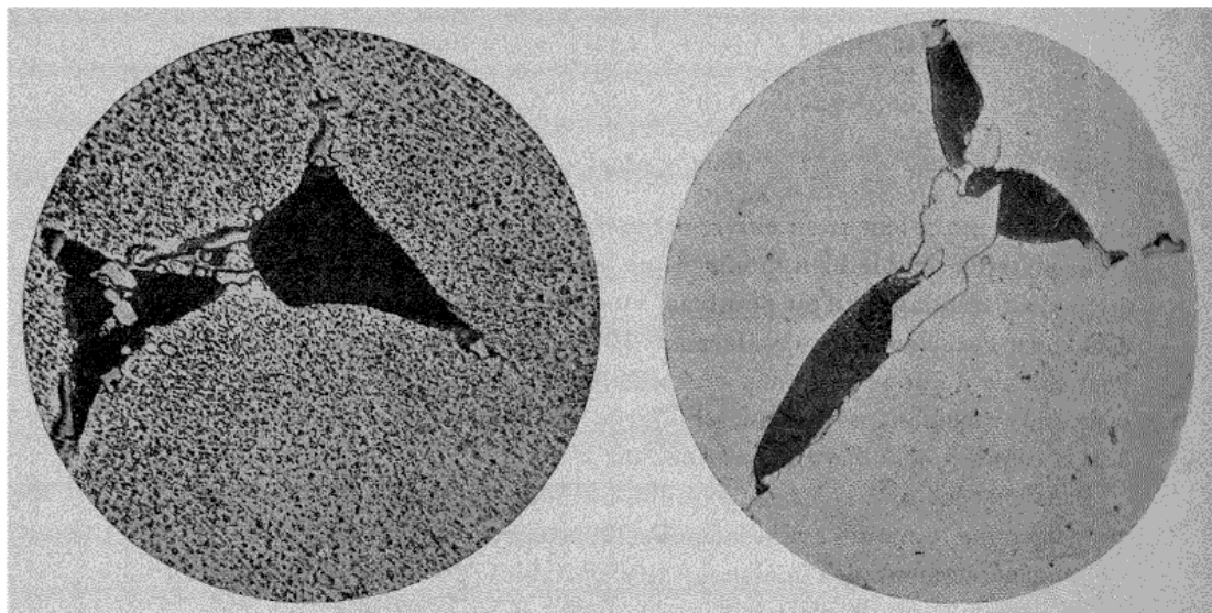
Fig. 39. — Duralumin. Attaque par NaOH pendant 30 secondes. Trempe à 475°, revenu à 425°. Grossissement : 430 d.
