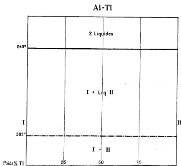
Fig. 17. — Diagramme des alliages Aluminium-Thallium.
