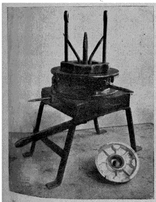
Fig. 4. — Dynamo-démarreur, palier côté commande (moule monté, pièce obtenue).
