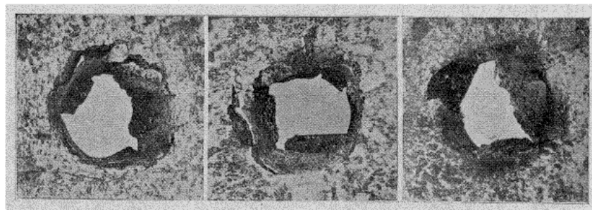
Fig. 18 à 20. — Essais d'emboutissage dynamiques de tôles d'acier peu ductiles.
