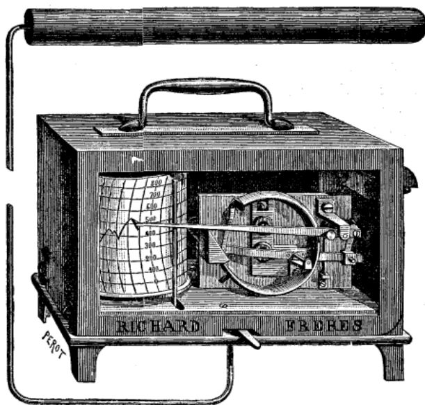
Fig. 31. — Thermomètre enregistreur à gaz Richard.
