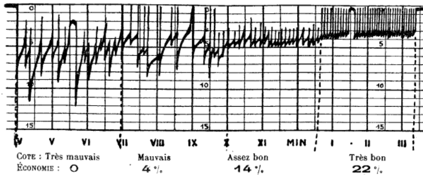
Fig. 47. — Diagramme d'un autre type de déprimomètre simple.
