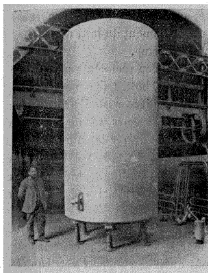
Fig. 14. — Tank de brasserie en aluminium de 150 hl. Hauteur : 9 m. Diamètre : 2,25 m. Poids : 930 kg. Tôle de 1 mm. Pression d'épreuve : 1,6 kg : cm 2 (Etablissement Girel).
