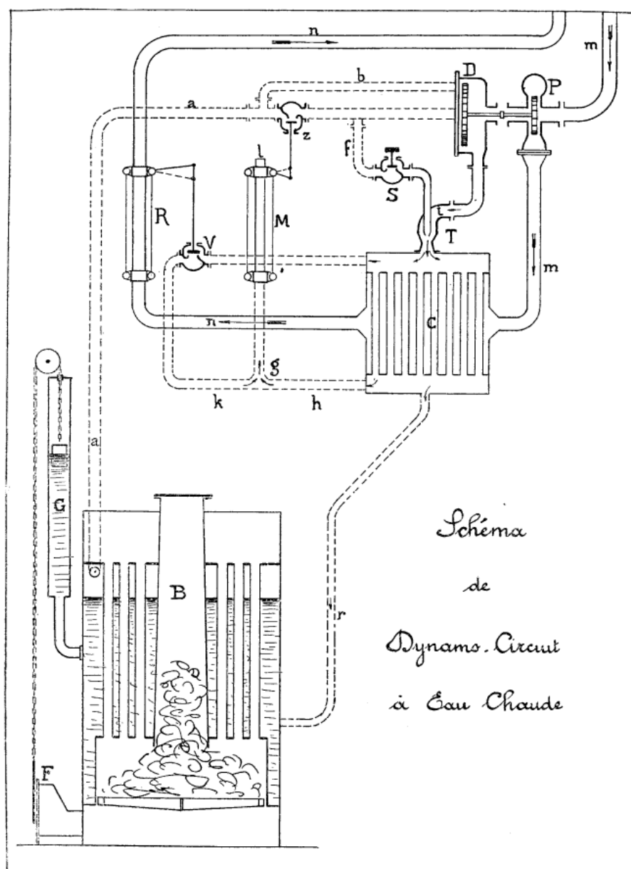
Fig. 7. — Schéma de dynamo-circuit à eau chaude.
