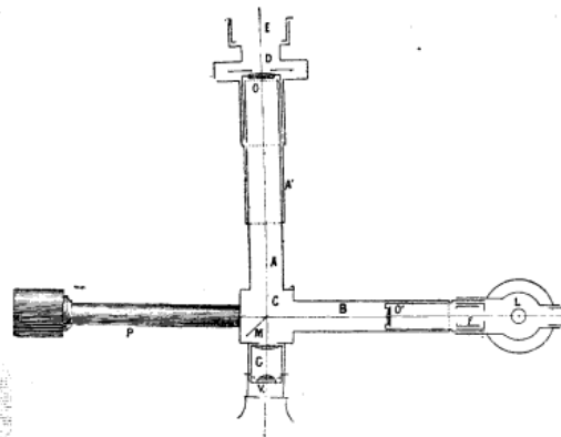
Fig. 36 bis. — Pyromètre optique Le Chatelier (coupe longitudinale).
