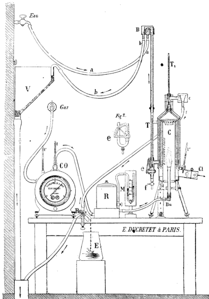
Fig. 79. — Calorimètre Junkers.
