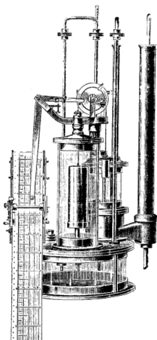
Fig. 17. — Analyseur automatique Eckardt.
