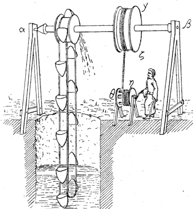
Fig. 30. — Poulie de commande à mouvement discontinu actionnant une noria (Philon de Byzance, 2 siècles av. J.-C.).
