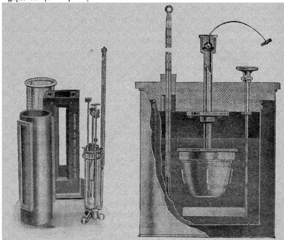
Fig. 77. — Calorimètre Rosenhain.
