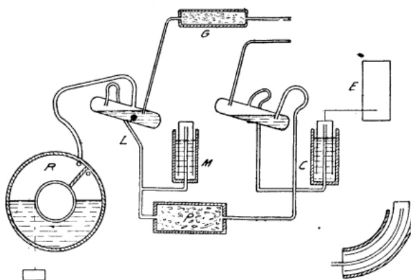
Fig. 23. — Schéma du fonctionnement de l'appareil Brenot-Poulenc.
