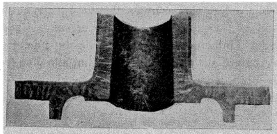
Fig. 38. — La même pièce que figure 37 sans défaut, après attaque.
