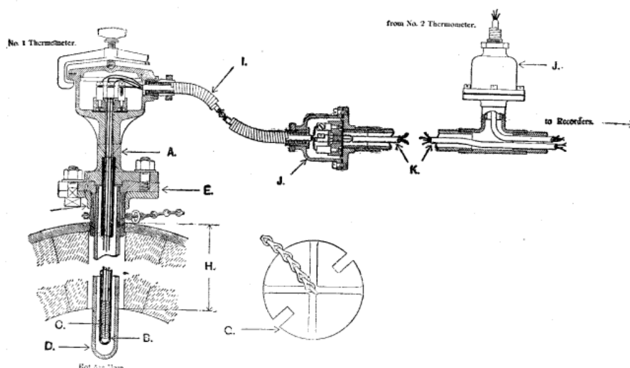
Fig. 40. — Pyromètre à résistance Cambridge.
