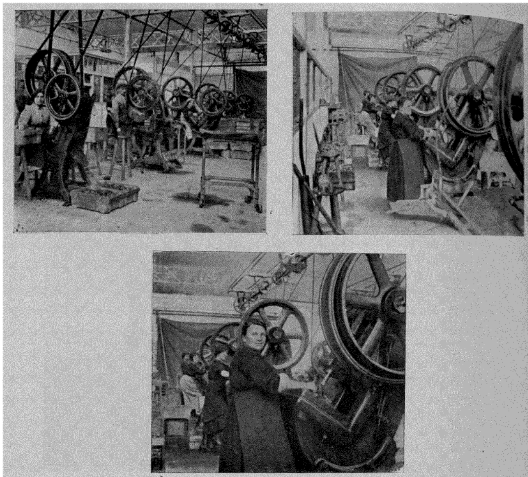
Fig. 9, 10 et 11. — Fabrication des supports de lampes dans les ateliers de l'Appareillage électrique Grivolos.
