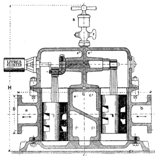
Fig. 65. — Compteur d'eau Schmid.
