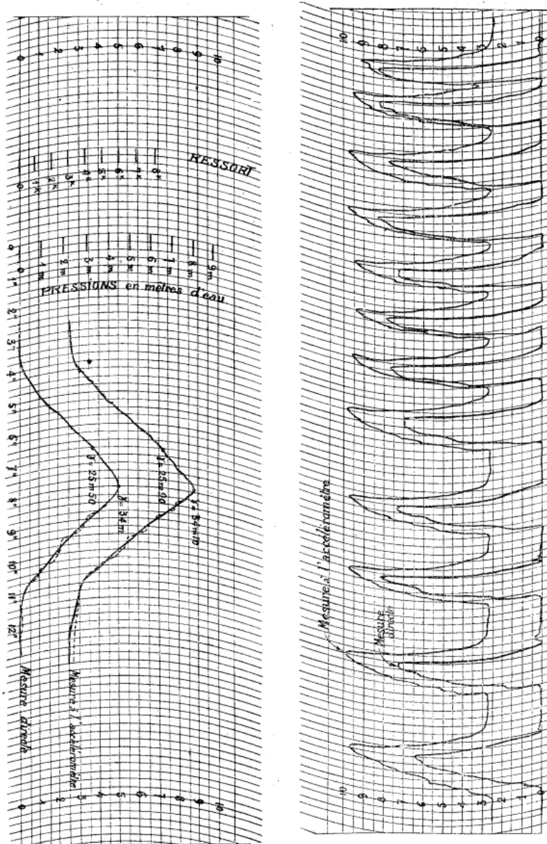
Fig. 18 et 19. — Courbe enregistrée par l'accéléromètre enregistreur comparée aux mêmes instants à une courbe d'accélérations rapidement variables « dans le temps ».
