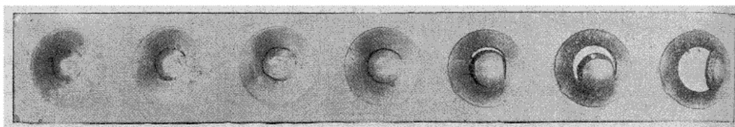
Fig. 22. — Vue des proues de sept emboutissages successifs à flèche croissante.
