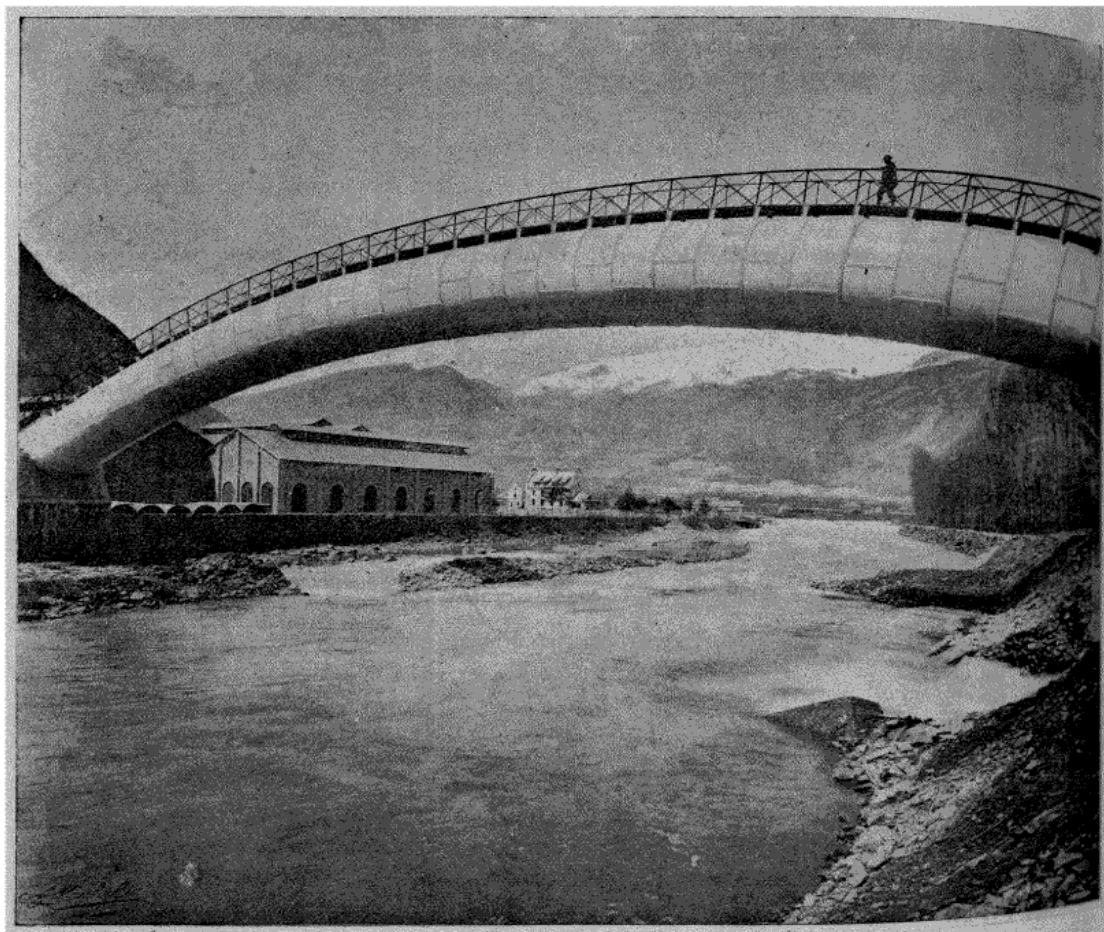
Fig. 7. — Usine de Saint-Jean-de-Maurienne : conduite forcée de 3,30 m de diamètre à la traversée de l'Arc.
