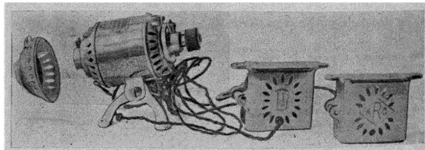
Fig. 58. — Moteur de machine à coudre avec son rhéostat.
