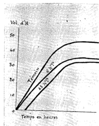
Fig. 2. — Dégagement d'hydrogène (mesuré en centimètres cubes) provoqué par l'attaque de l'aluminium par un liquide en fonction du temps.
