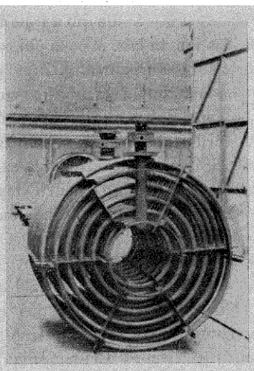
Fig. 15. — Emploi de l'aluminium en brasserie : Serpentin en aluminium à 6 enroulements de 8 spires. Longueur totale 360 m. (Etablissement Girel.)
