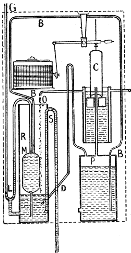
Fig. 19. — Analyseur automatique Van Houtte.
