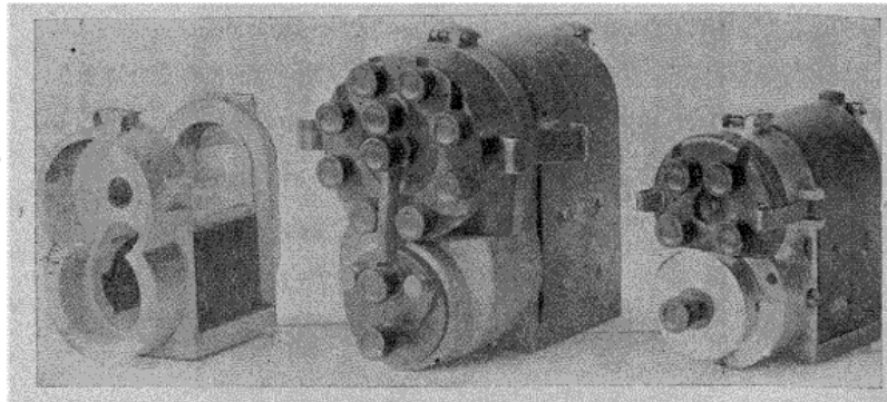
Fig. 32. — Bâtis de magnétos Monobloc.
