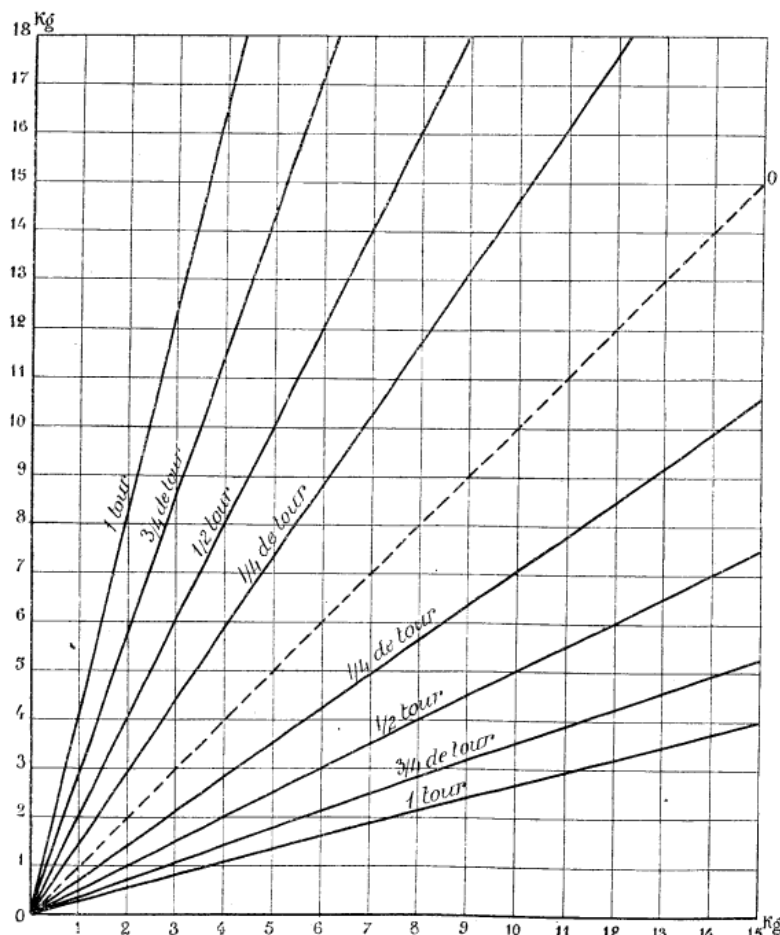
Fig. 31. — Graphique de la résistance au frottement d'une corde de 10 mm de diamètre.
