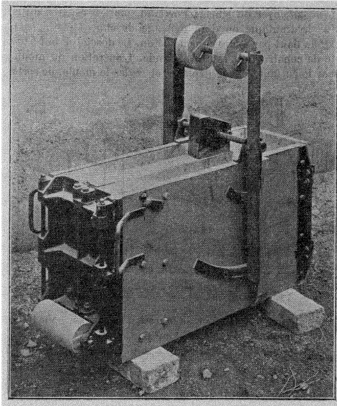
Fig. 2. — Moule de la Société du Béton monolithe.
