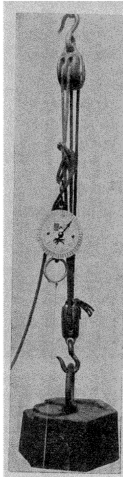
Fig. 89-90. — Mesure de l'effort de traction sur un palan, pour monter une charge de poids connu.
