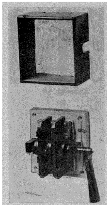
Fig. 24. — Interrupteur avec extrémité de poignée de manœuvre en aluminium.
