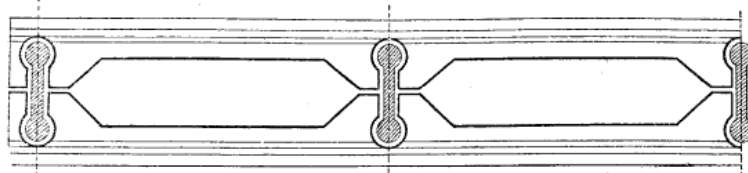
Fig. 1. — Vue de la brique Stéphane assemblée.
