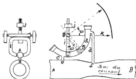
Fig. 58. — Compteur d'air comprimé Piette.
