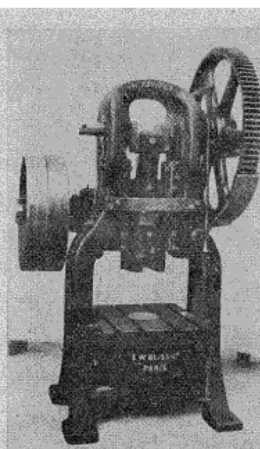
Fig. 3. — Presse à emboutir l'aluminium. Presse pour objets de grand diamètre.
