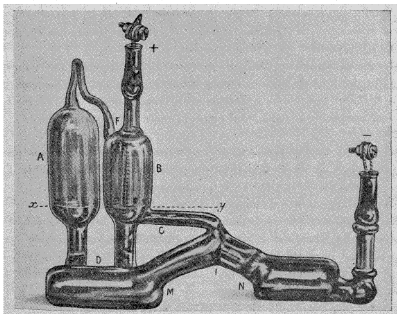
Fig. 2. — Vue de la lampe à mercure, système Henri George.
