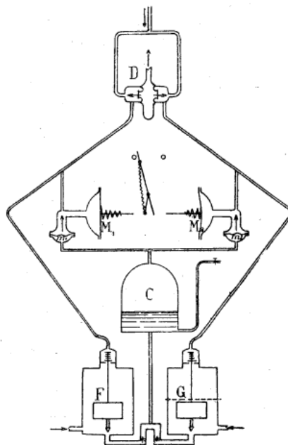
Fig. 11. — Schéma d'agencement d'un appareillage inverseur de marche à fonctionnement automatique.
