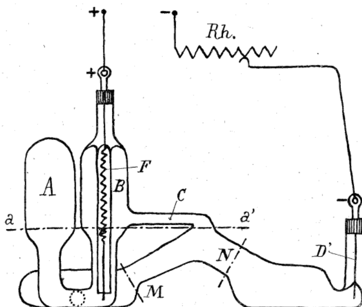
Fig. 1. — Coupe schématique de la lampe à mercure, système Henri George.
