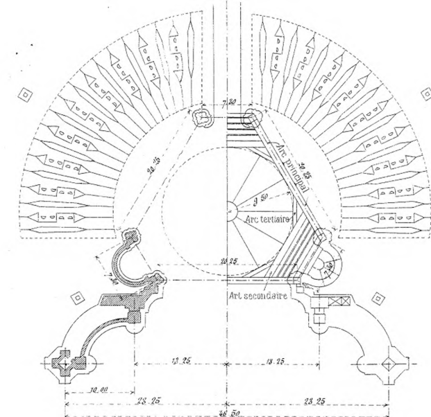
Plan de la porte et des guichets
