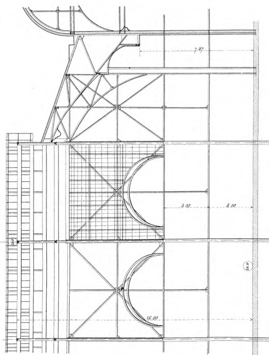
Coupe suivant MN
