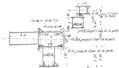
Plan des pieds des piliers
