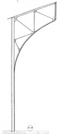
Coupe suivant EF
