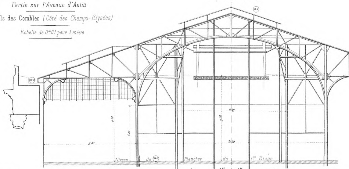
Coupe suivant ABCD
