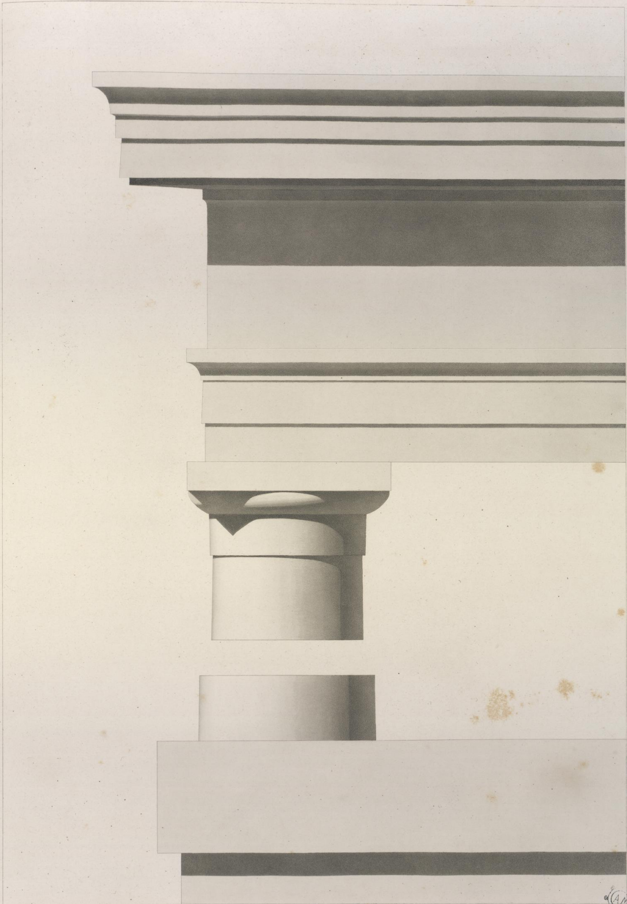
SOUBASSEMENT, CHAPITEAU ET ENTABLEMENT DU TEMPLE DE LA PIÉTÉ À ROME au huitième de l'exécution
