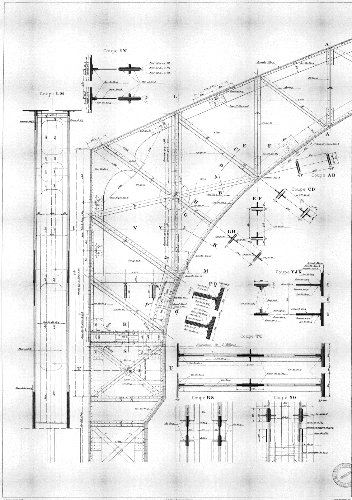
FERMES DE 50 m — DÉTAILS DE LA FERME (TYMPAN)
