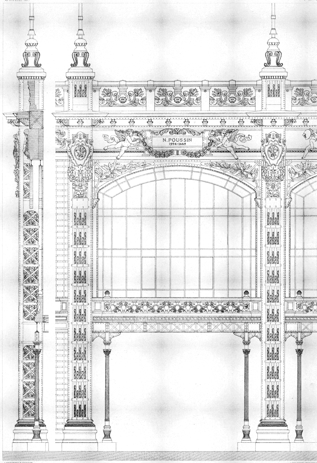
DÉTAIL D'UNE TRAVÉE
