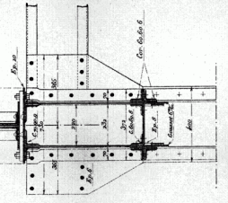
Coupe EF HI GO
