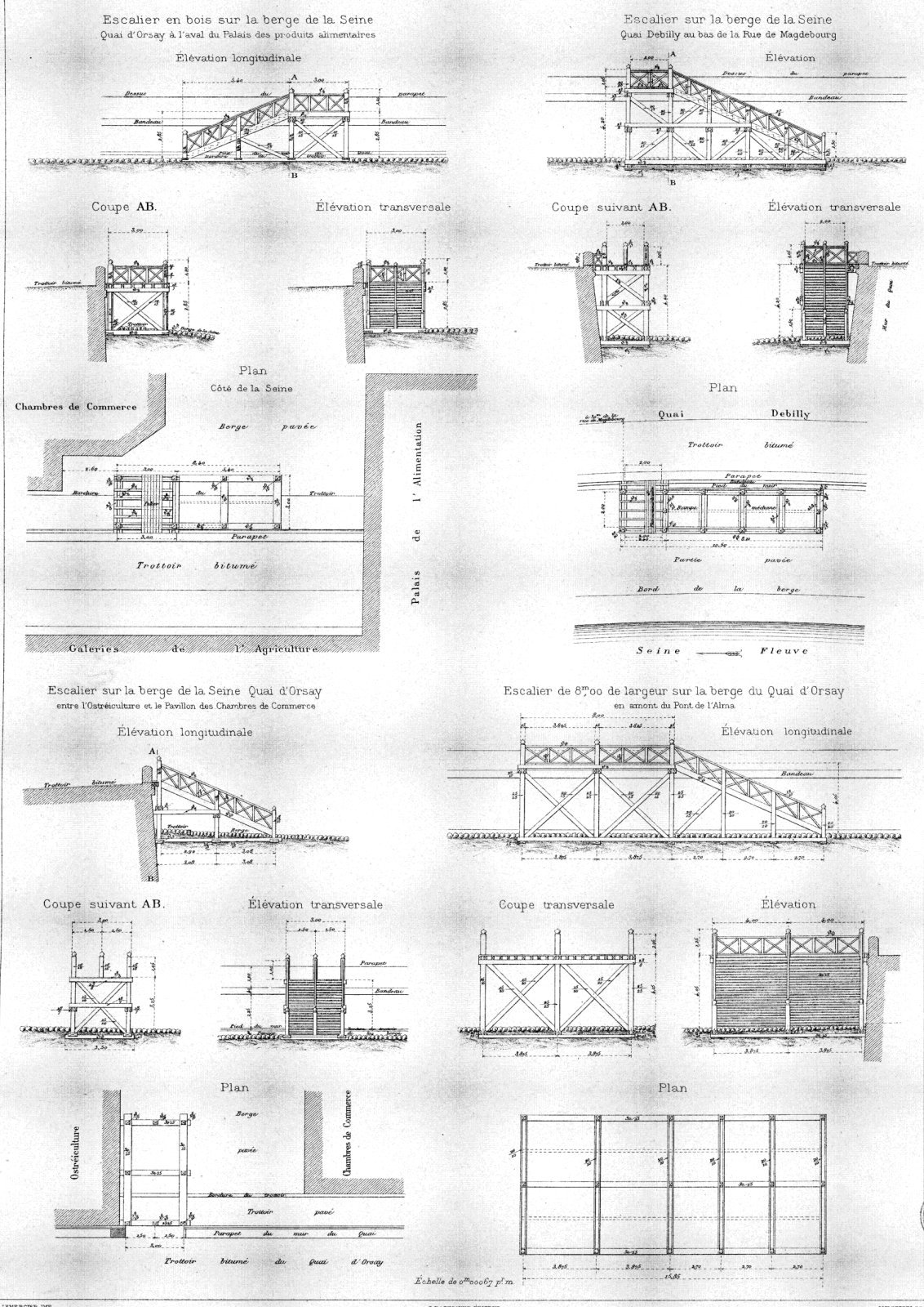
ESCALIERS METTANT EN COMMUNICATION LES BERGES ET LES QUAIS
