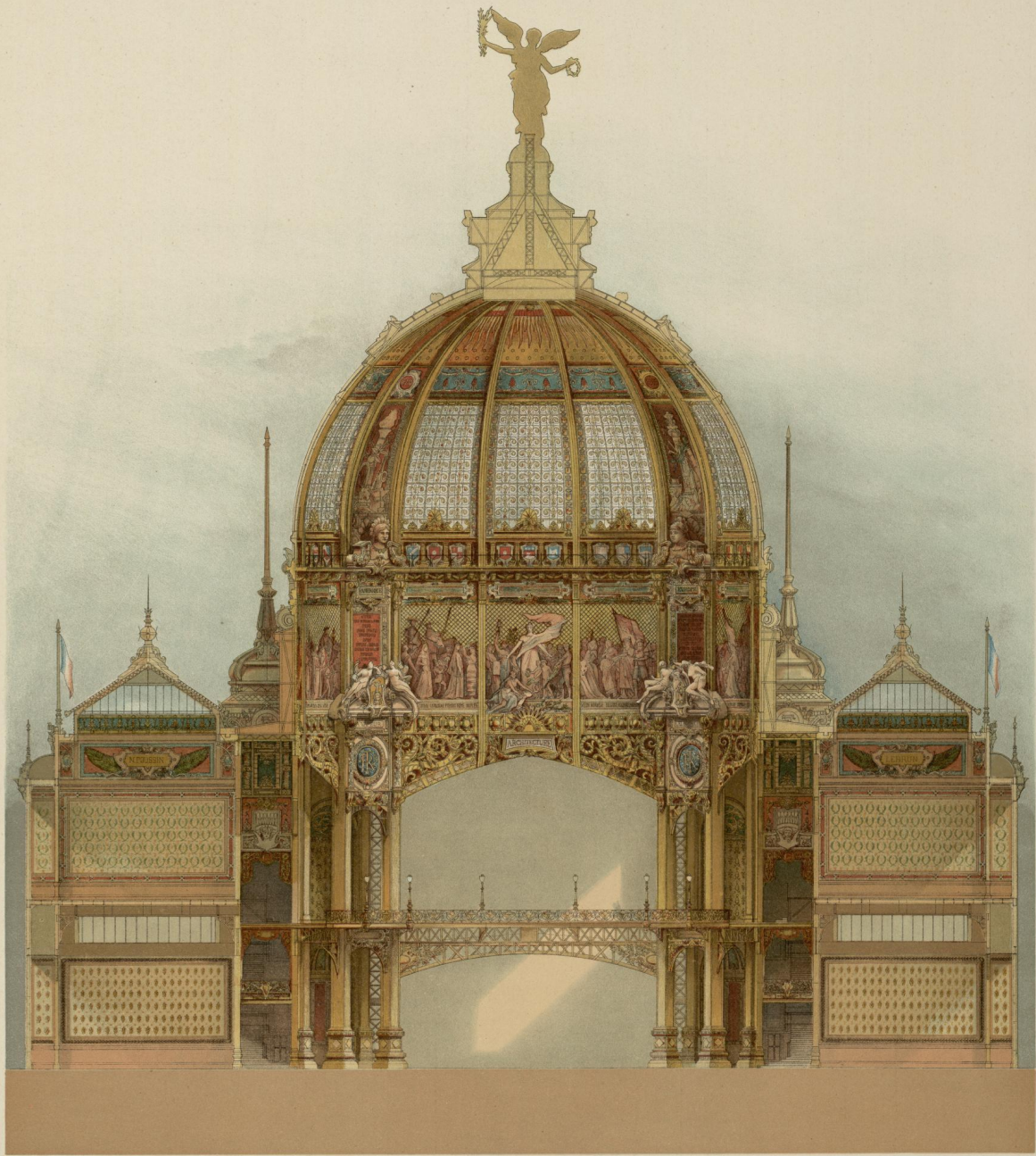
DÔME CENTRAL — COUPE PARALLÈLE À LA SEINE
