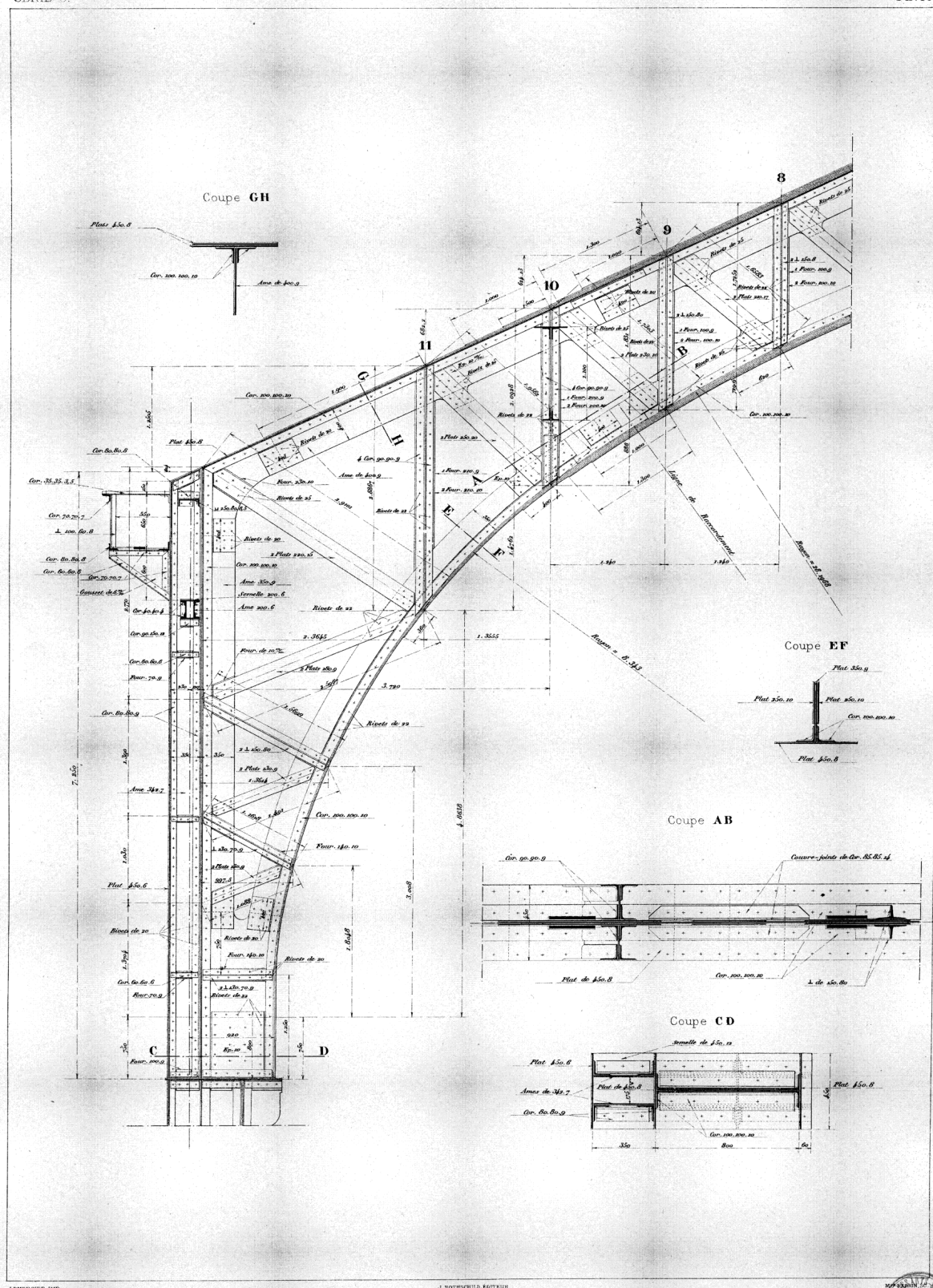
FERMES DE 30 M —ÉLEVATION DE LA PARTIE INFÉRIEURE.
