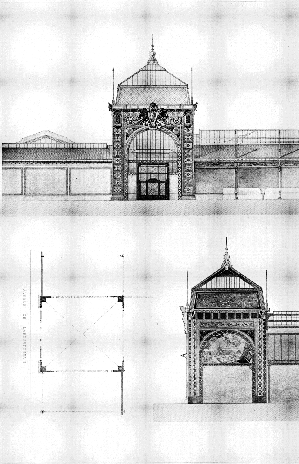
PAVILLON DE RACCORDEMENT — PLAN — FAÇADE — COUPE
