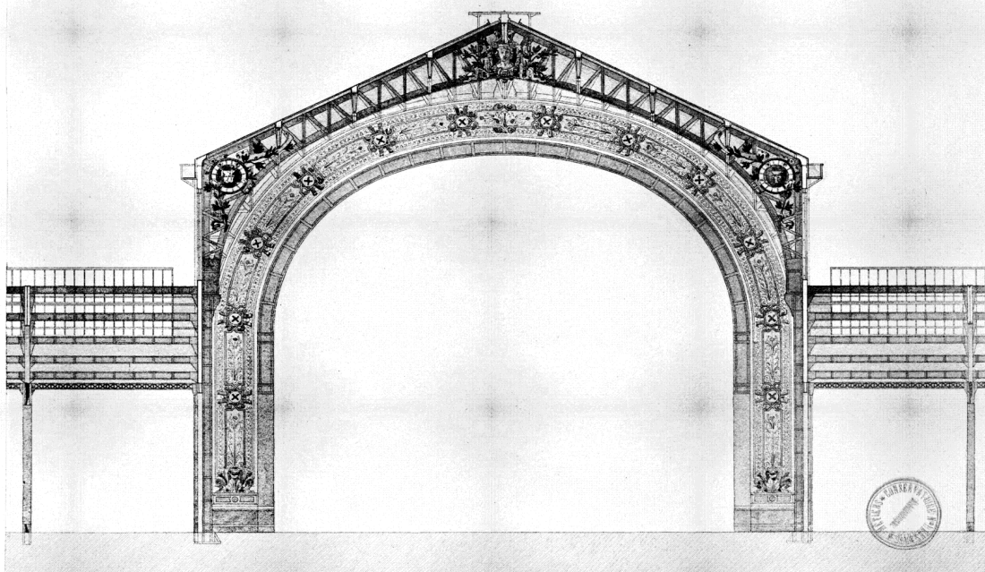
GALERIE DE 30 MÈTRES — COUPES TRANSVERSALES
