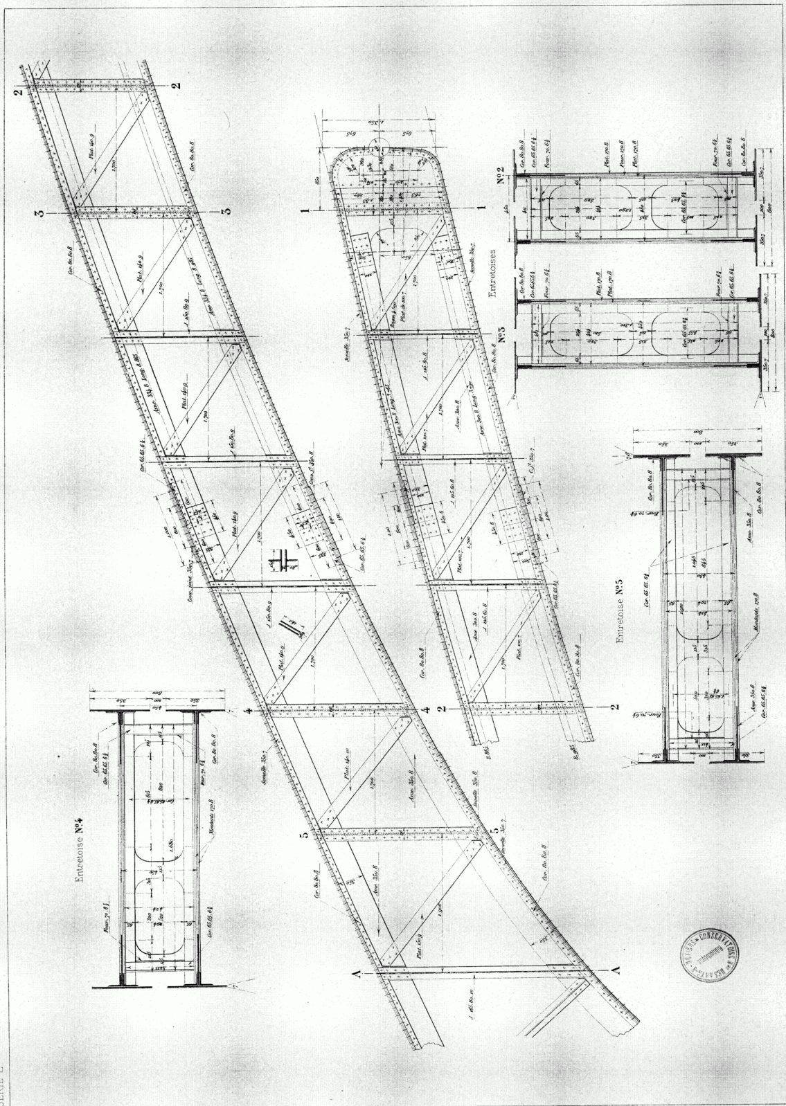
FERMES DE 50 m — DÉTAILS D'UNE FERME (DU SOMMET AU TYMPAN)
