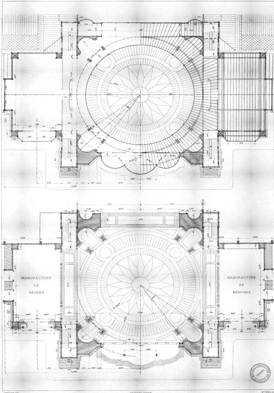
DÔME CENTRAL — PLANS DU REZ-DE-CHAUSSÉE ET DE L'ÉTAGE
