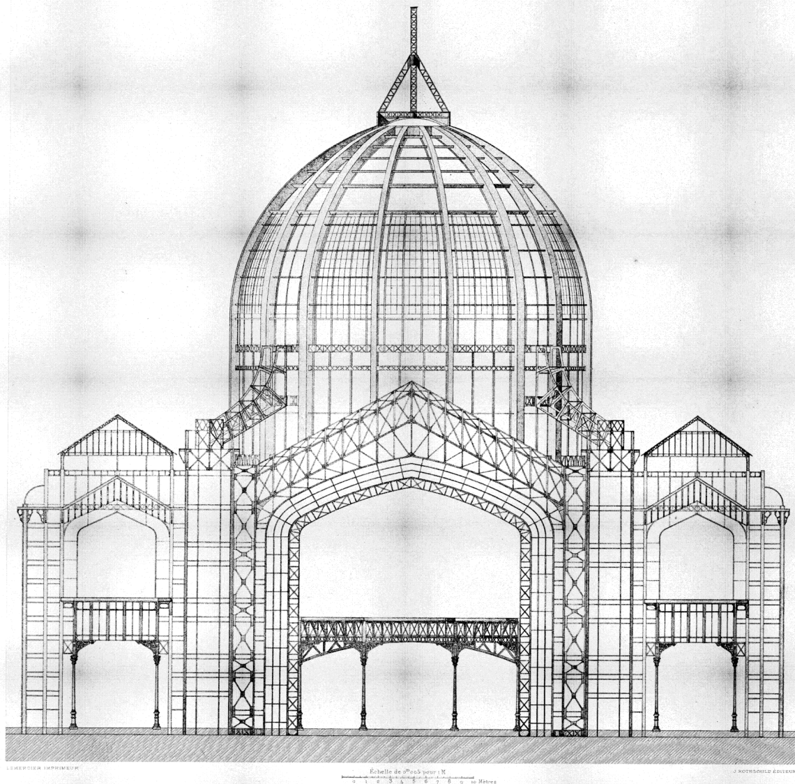
DÔME CENTRAL, FAÇADE — OSSATURE MÉTALLIQUE
