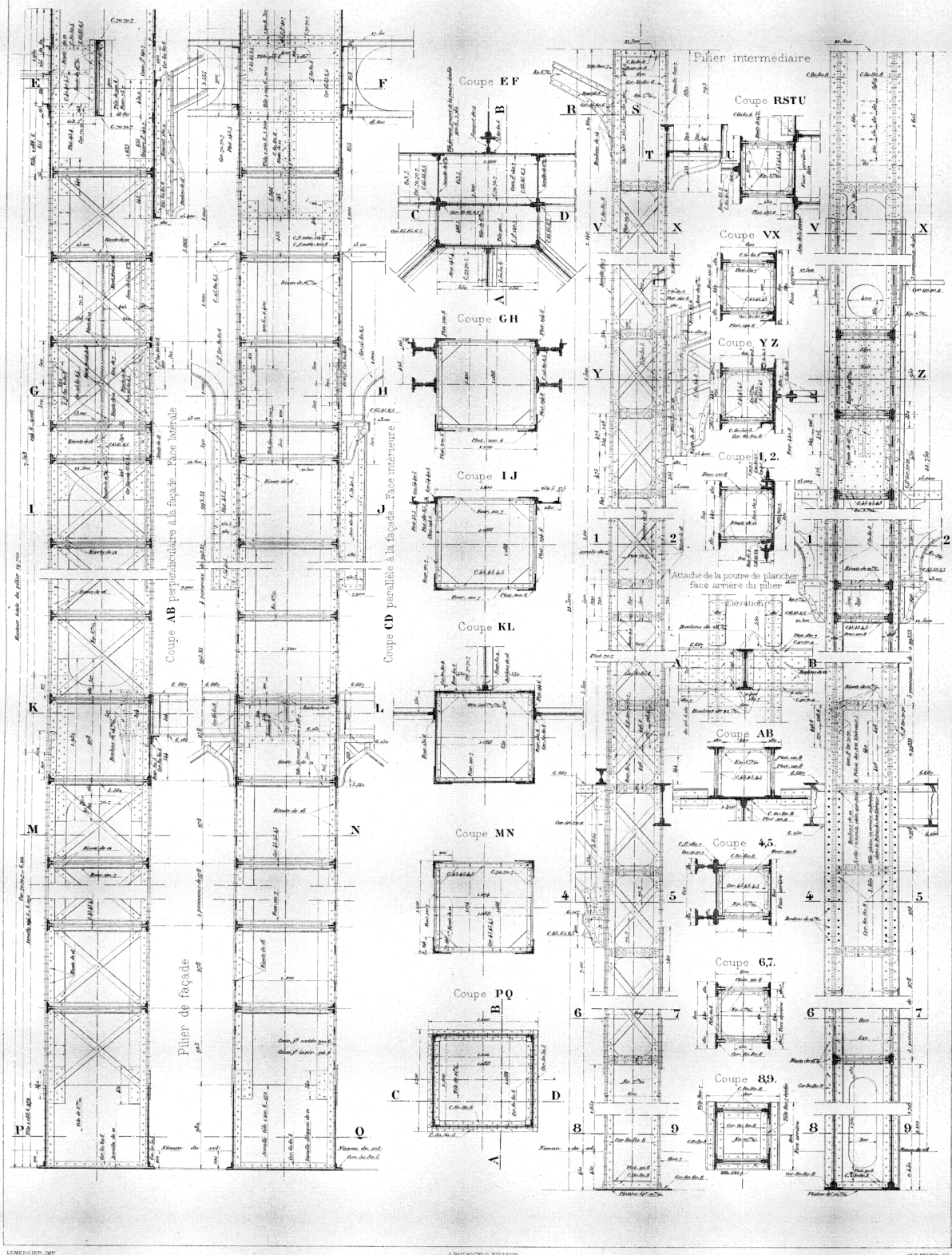
FERMES DE 50 m — PILIERS
