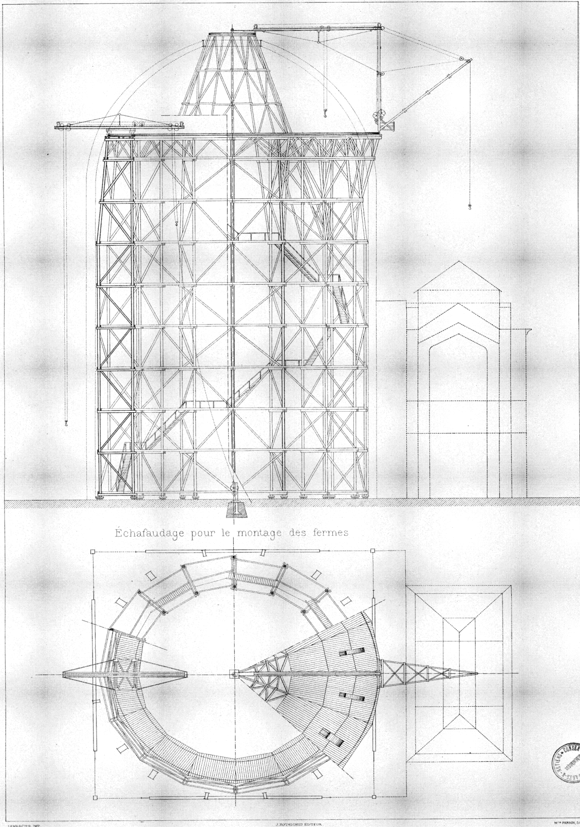
DÔME CENTRAL — CONSTRUCTION MÉTALLIQUE
