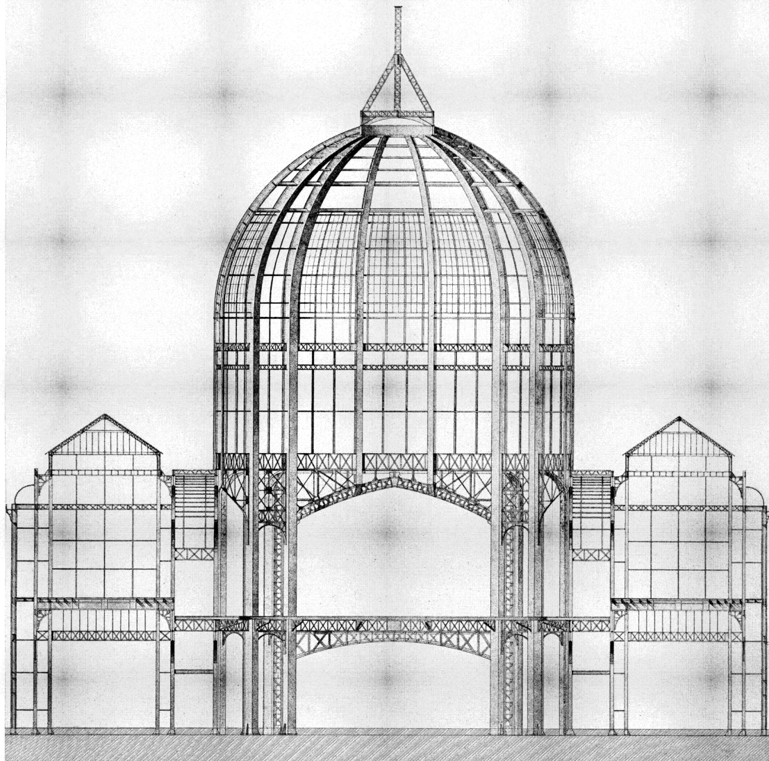
DÔME CENTRAL. COUPE — OSSATURE MÉTALLIQUE
