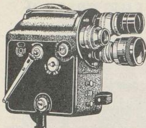
Dimensions, sans objectif : 14 x 21 x 9 cm Poids, sans objectif 2 kg. 900
