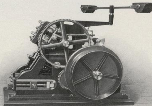
Machine automatique à faire à chaud les plaques à souder les métaux Brevetée S. G. D. G.
