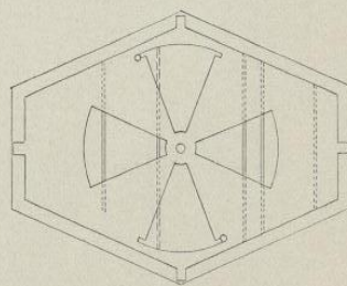
VENTILATEUR A CLAPETS construction en zinc pour application dans les parois en Briques NEUTRAL N° 9.
