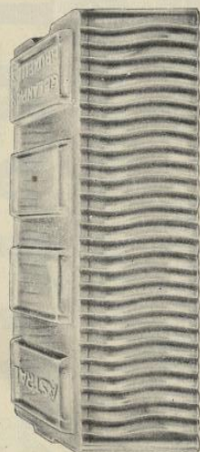
Dim.: 240 x 80 x 70 mm. - Poids approx.: 1300 gr. Environ 60 pièces au mètre carré.
