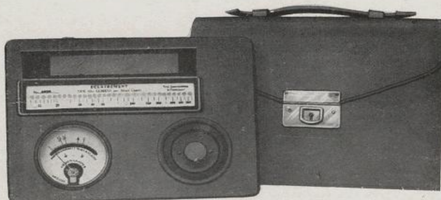
Luxmètre MAZDA avec son étui Dimensions : 210 m/m \times 160 m/m \times 45 m/m
