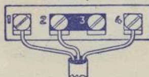
Montage triphasé
