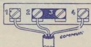
Montage continu 3 fils
