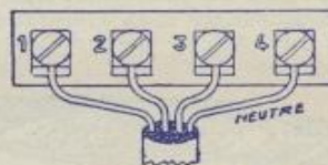
Montage triphase avec neutre
