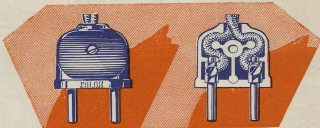
Fiche prise 6 ampères P.C. 6
