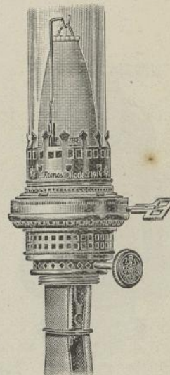
N° 111 bis. Bec à incandescence au pétrole "Kronos"; qualité supérieure, éclairage intensif (employer la cheminée n° 11). la pièce...
