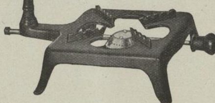
N° 23. Réchaud "Le Trèfle" à gaz d'alcool, socle carré fonte émaillée gris-bleu céramique, largeur 24 \frac{1}{16} , hauteur du socle 7 \frac{1}{16} , gazéificateur et réservoir en cuivre poli, fonctionnement très simple, la pièce. . . . .
