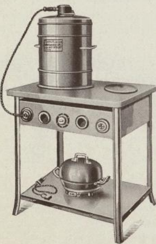
Cuisinière Electro-Econome avec plaque chauffante
