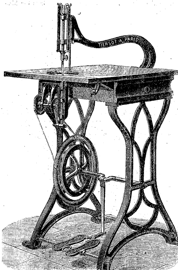
MACHINE PARISIENNE RECTILIGNE. — N° 48
