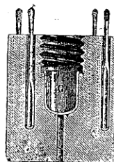
Vue en coupe de la boîte à forets
