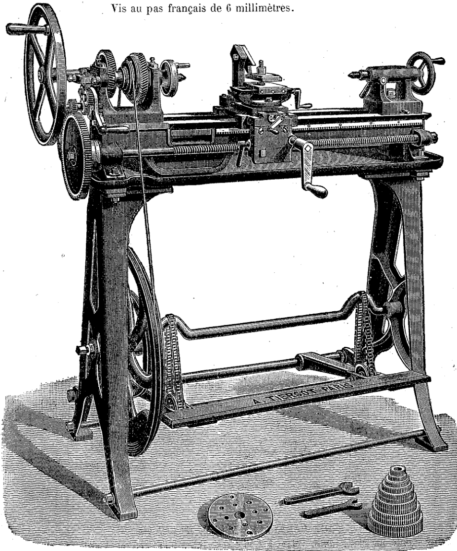
TOUR PARALLÈLE RENFORCÉ, N° 400
