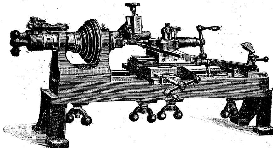
La gravure ci-dessus montre l'appareil à fileter en fonction
