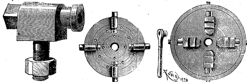
Plateaux universels à trous garnis de 4 poupées à pompes.
