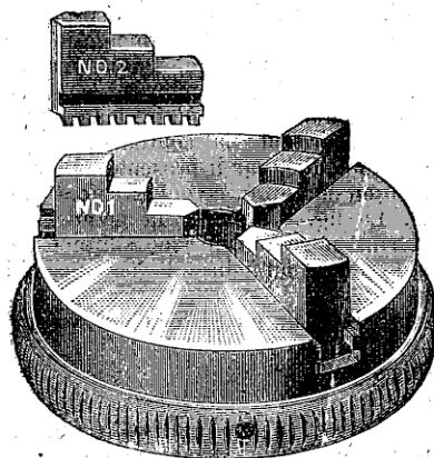
Plateau universel de Whiton, à levier
