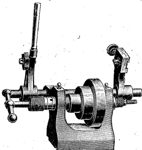
La gravure ci-dessus montre l'appareil à fileter en fonction
