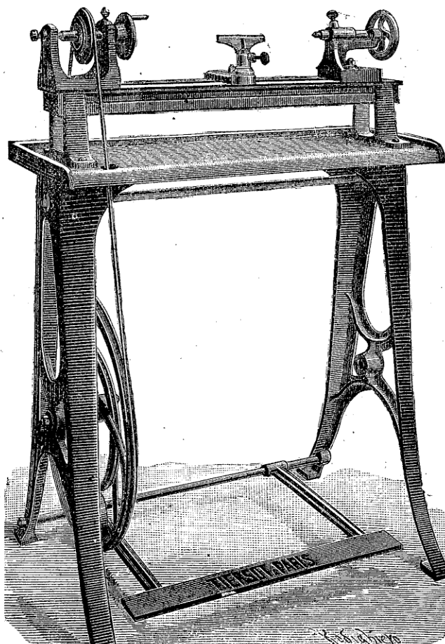
TOURS AMATEURS, PIEDS RENFORCÉS N os 364 bis et 365 bis
