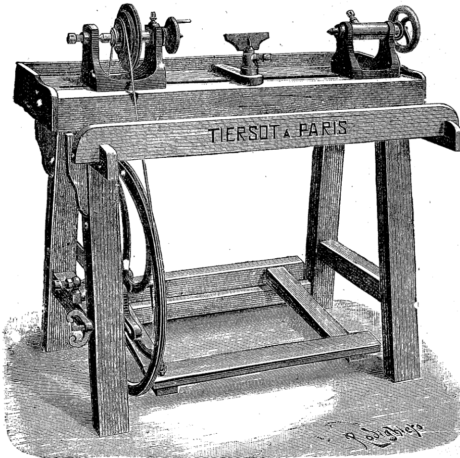
TOUR A BIDET, N° 344
