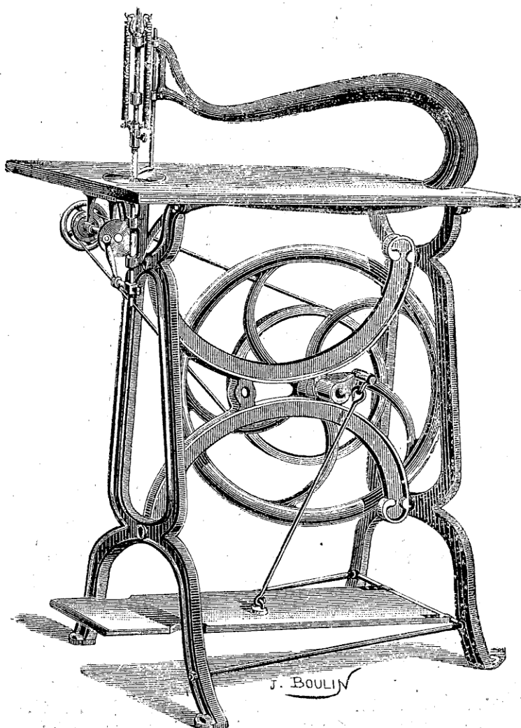
MACHINE RECTILIGNE. — N° 16 bis.
