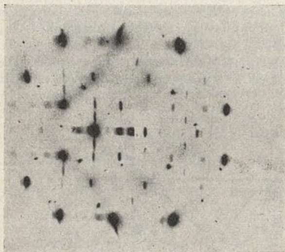
Alliage Al-Cu après un revenu de 30 h. à 150°.
