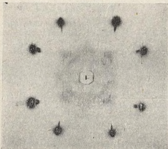
Alliage Al-Ag après un revenu de 100 h. à 150°.
