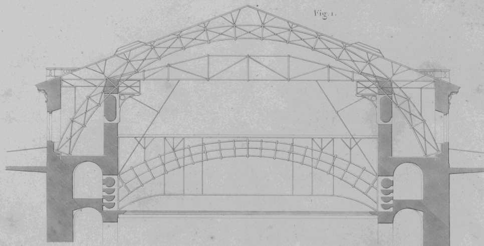
CHARPENTE EN FER SUR LA SALLE DU THÉÂTRE ALEXANDRA A S T PETERSBOURG.
