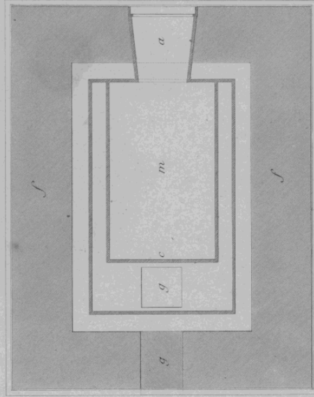
Plan du Calorifère.
