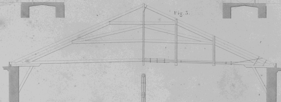
CHARPENTE DU THÉÂTRE MICHEL A S T PETERSBOURG.
