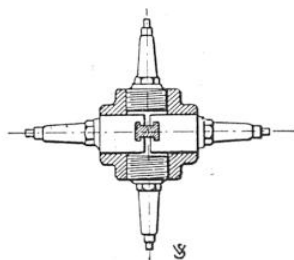
Tête d'étoile mobile armée de ses pointes, vue de face.
