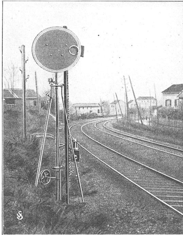
SIGNAL AVANCÉ D'UNE GARE
