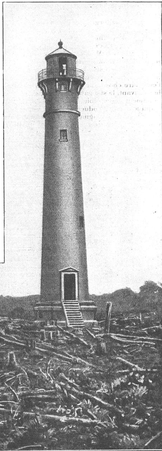
UN DES PHARES ÉRIGÉS EN PLEINE BROUSSE AUX BORDS DU CANAL (SECTION DU PACIFIQUE)
