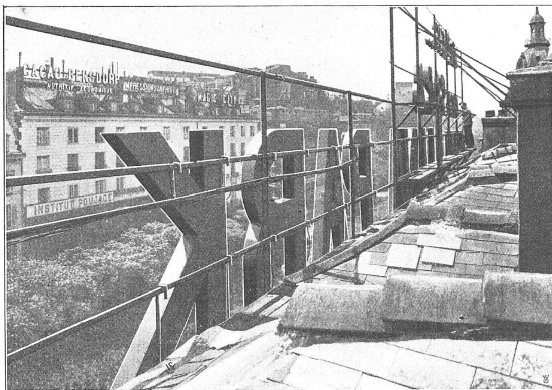
CETTE VUE D'ARRIÈRE DE L'ENSEIGNE CI-CONTRE REPRÉSENTE L'ARMATURE MÉTALLIQUE
