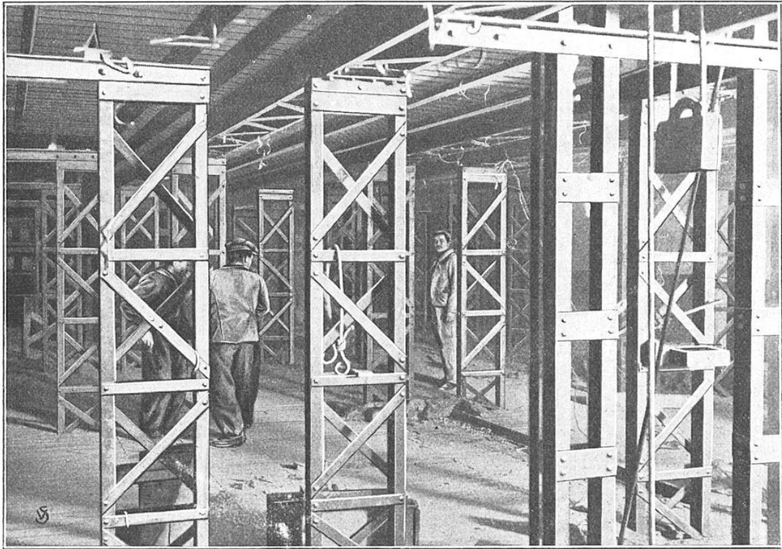
PENDANT LES REPRÉSENTATIONS, LA SCÈNE SERA LOURDEMENT CHARGÉE Malgré la forêt des piliers nécessaires, presque tout le plancher (que l'on voit au haut de la photographie) peut s'abaisser et remonter par sections, suivant les besoins de la mise en scène.
