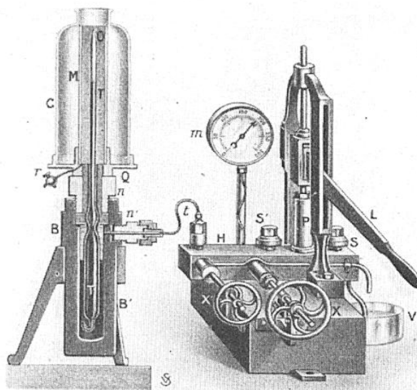
PREMIER APPAREIL DE CAILLETET POUR LA LIQUÉFACTION DES GAZ
