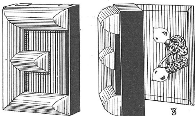
LETTRES EN VERRE MOULÉ, DÉPOLI, DITES « LUCIOLES » Au lieu d'employer un nombre de lampes suffisant pour dessiner le contour de la lettre, on utilise seulement une ou deux ampoules dont la lumière se diffuse sur un fond réflecteur.
