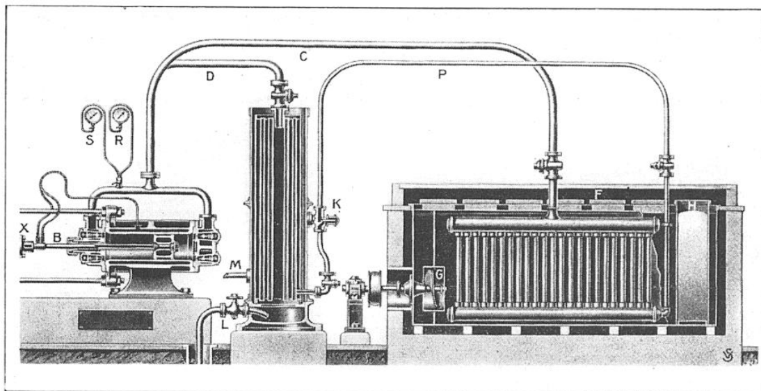
COUPES SCHEMATIQUES EN ÉLEVATION ET EN PLAN D'UNE INSTALLATION POUR LA FABRICATION DE LA GLACE ARTIFICIELLE (PROCÉDÉ RAOUL PICTET A L'ANHYDRIDE SULFUREUX)
