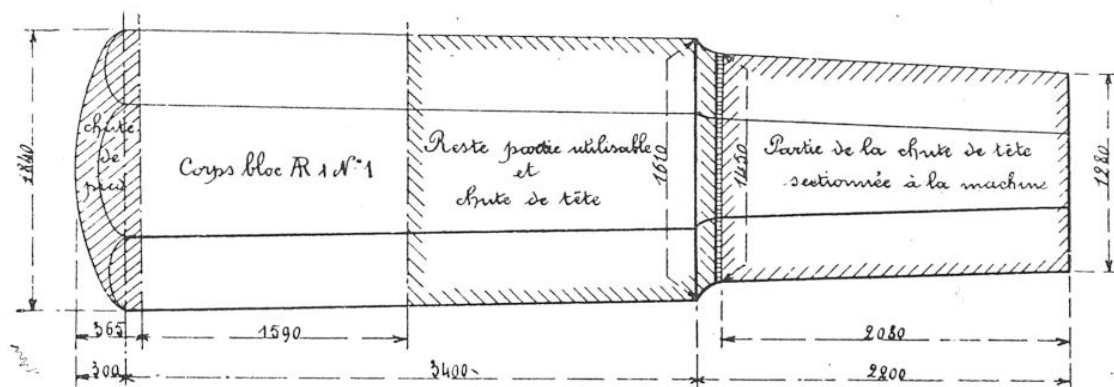
COTES DU LINGOT DESTINÉ A LA FABRICATION DU CORPS-ARRIÈRE
