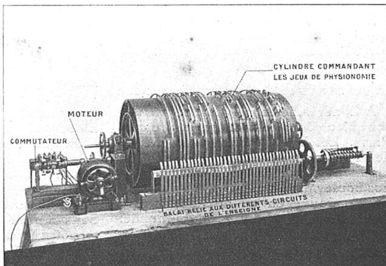
Le commutateur qui réalise les effets de l'enseigne ci-dessus.
