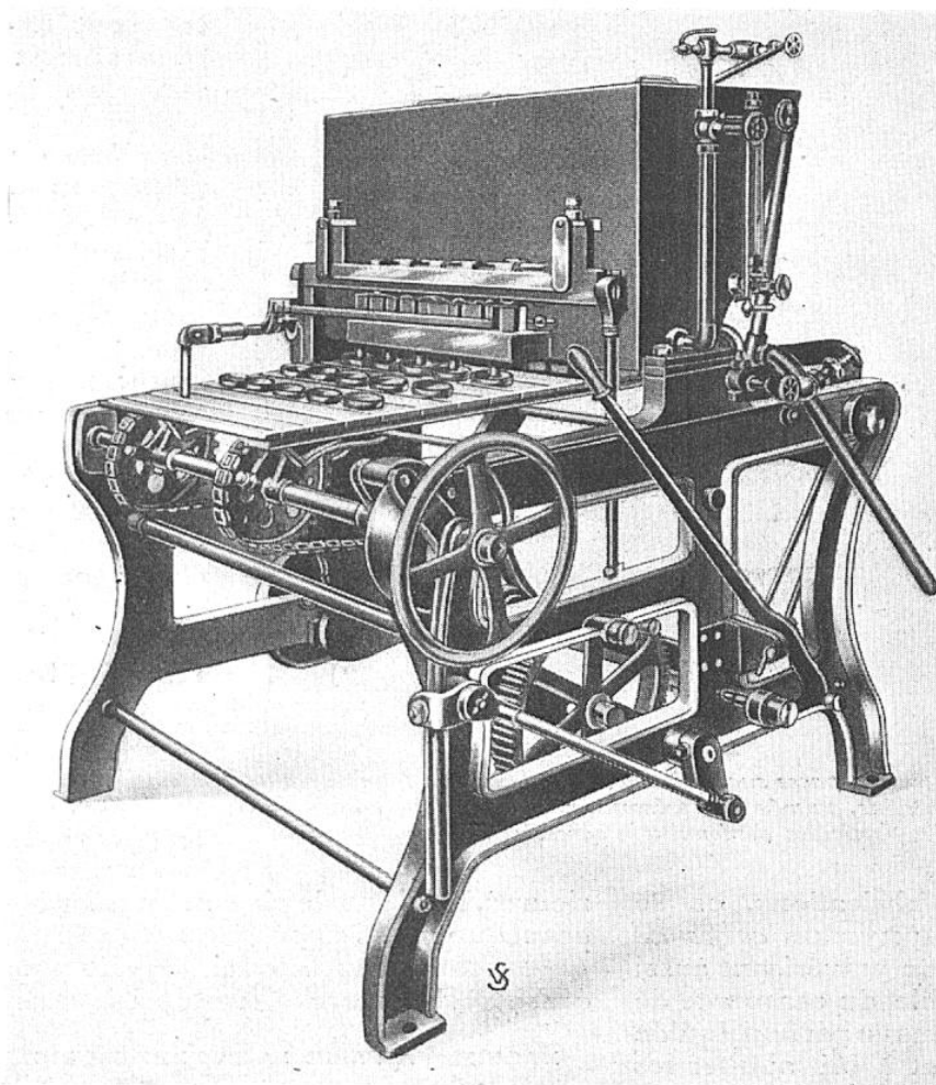
MACHINE A REMPLIR LES BOITES
