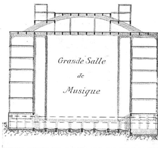
COUPE TRANSVERSALE DE L'OSSATURE
