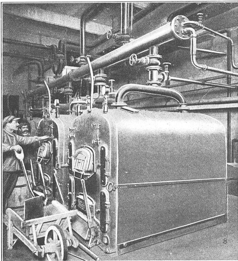
CINQ CHAUDIÈRES DE VOLUME CONSIDÉRABLE ASSURENT LE CHAUFFAGE PARFAIT DE TOUT L'ÉDIFICE
