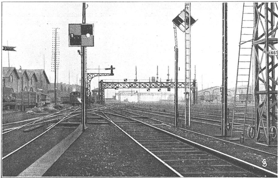
SIGNAUX DE PROTECTION D'UNE BIFURCATION
