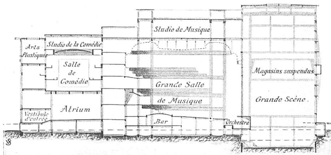
COUPE LONGITUDINALE DE L'OSSATURE EN CIMENT ARMÉ
