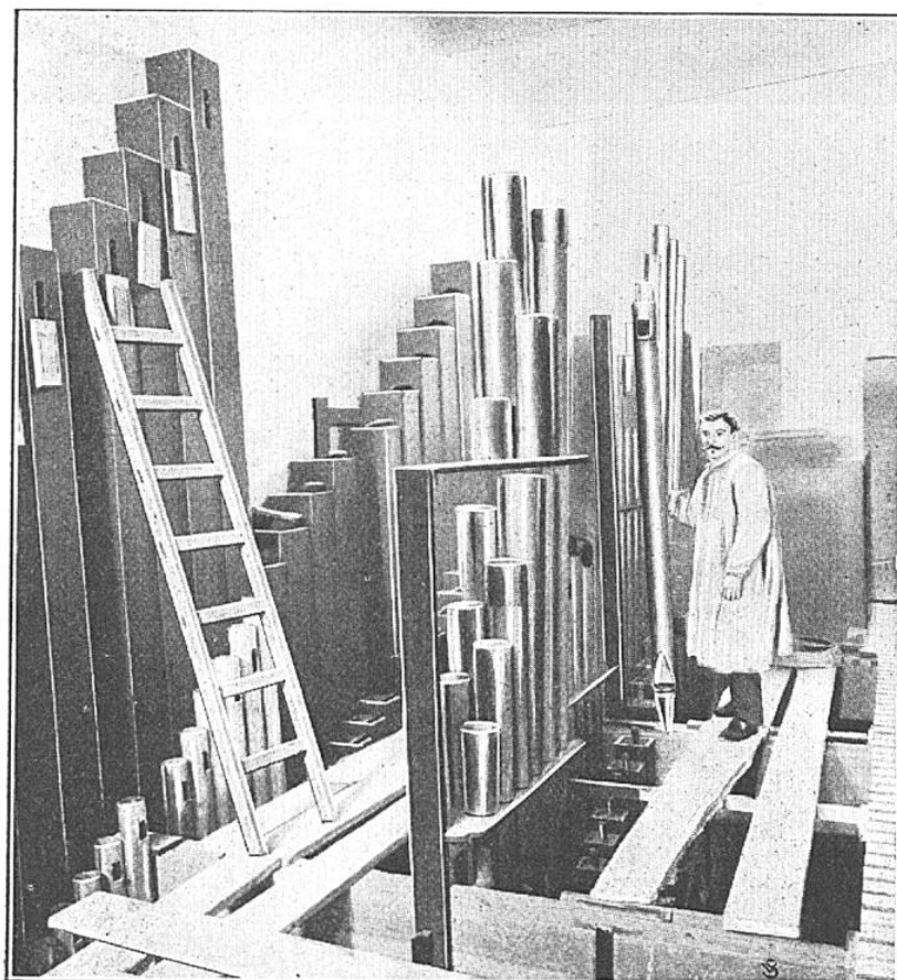
MONTAGE DES TUYAUX DU GRAND ORGUE DANS LES COMBLES DE LA SALLE D'AUDITIONS MUSICALES
