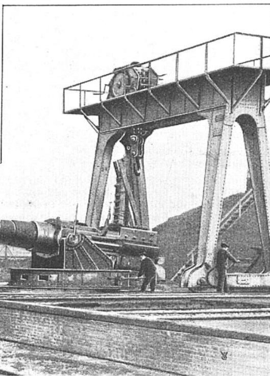
PIÈCE DE 30 CM MONTÉE SUR AFFÛT PROVISOIRE POUR LES PREMIERS TIRS D'ÉPREUVE
