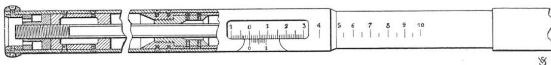
Mécanisme du vernier pour la lecture des indications de l'étoile mobile.
