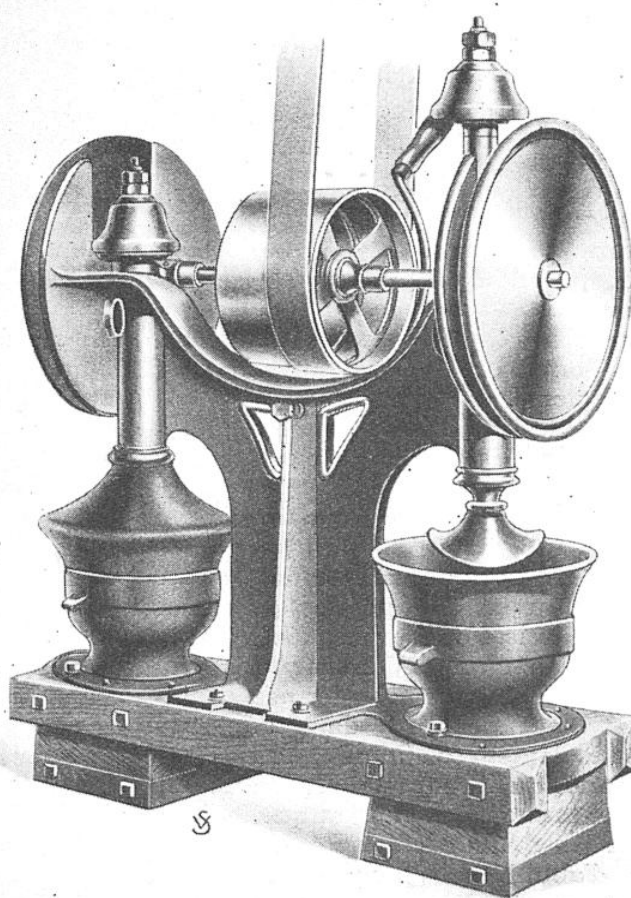
CONCASSEUR A PILONS
