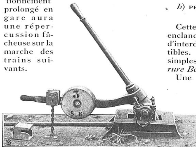
SERRURE BOURÉ IMMOBILISANT UNE AIGUILLE Au bout de sa chaîne on voit la serrure fermée et empêchant toute manœuvre intempestive du levier.
