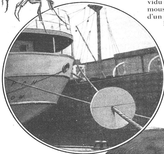
Les disques, placés sur les câbles, ne peuvent être franchis par les rats et les empêchent de quitter le navire. Ils sont obligatoires dans les ports de certains pays.
