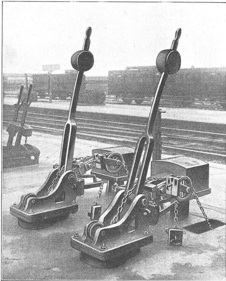
DEUX SERRURES BOURÉ OUVERTES
