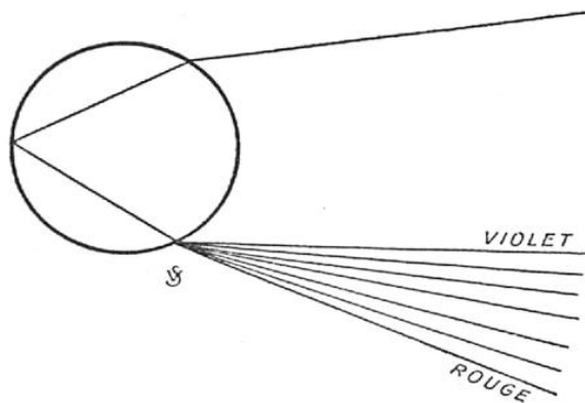
FIG. 6. — LUMIÈRE SOLAIRE TOMBANT SUR UNE BOULE DE VERRE (UNE SEULE RÉFLEXION)
