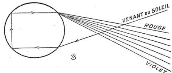
FIG. 7. — LUMIÈRE TOMBANT SUR UNE BOULE DE VERRE (DEUX RÉFLEXIONS)
