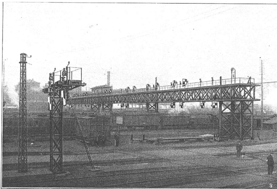
PASSERELLE DES SIGNAUX DE LA GARE DU NORD A PARIS
