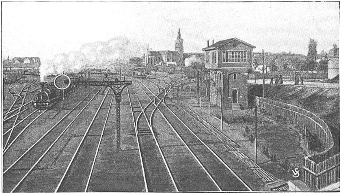
LES APPROCHES DE LA GARE DE CHALON-SUR-SAONE SUR LE P.-L.-M. Photographie typique montrant la complication des aiguillages commandés par un seul poste surélevé Saxby dans une gare d'importance ordinaire. On voit le poste à droite.
