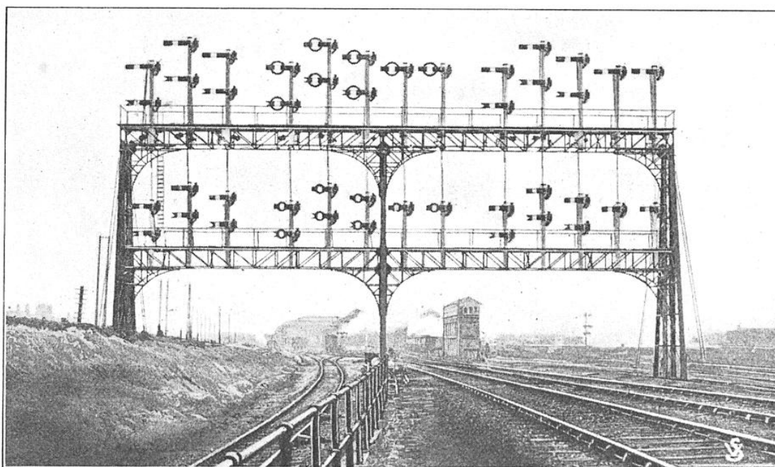
PASSERELLE PROTÉGÉANT LES ABORDS D'UNE GARE ANGLAISE On peut voir ici que les signaux anglais sont beaucoup plus surélevés que les nôtres. Les mécaniciens peuvent, à très grande distance, les apercevoir et distinguer leurs indications.
