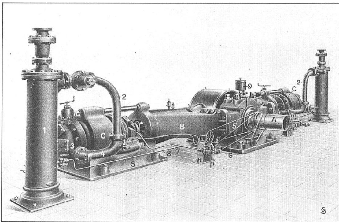
TYPE INDUSTRIEL D'UN COMPRESSEUR DOUBLE SULZER A AMMONIAQUE, CAPABLE DE PRODUIRE 6 000 KILOGRAMMES DE GLACE A L'HEURE OU 144 TONNES EN 24 HEURES
