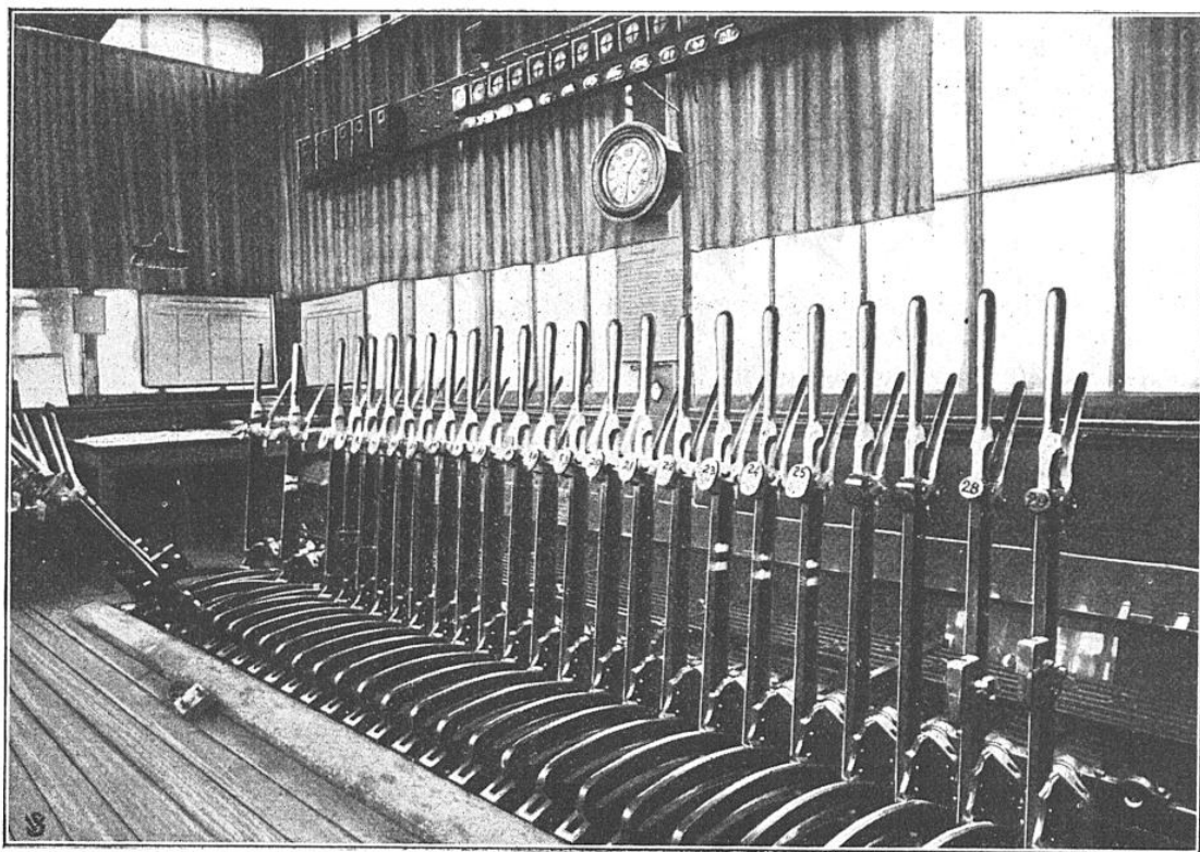
INTÉRIEUR D'UN POSTE D'AIGUILLAGE SAXBY
