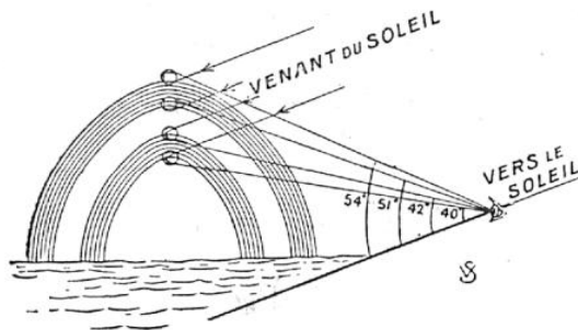
FIG. 5. — LES DEUX ARCS-EN-CIEL
