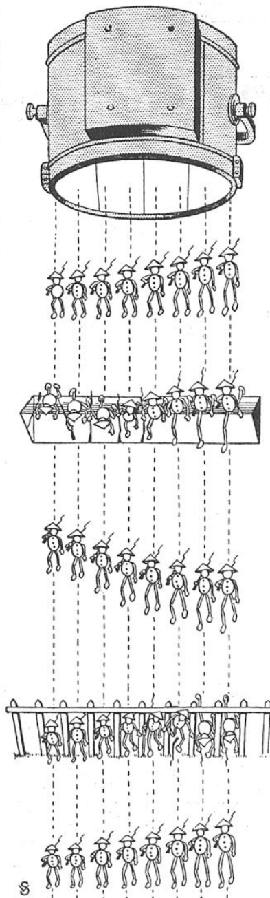
FIG. 1. — COMMENT LES ONDES LUMINEUSES PASSENT A TRAVERS LE PRISME
