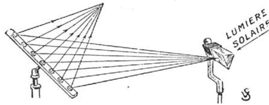
FIG. 7. DÉCOMPOSITION ET RECOMPOSITION DE LA LUMIÈRE BLANCHE
