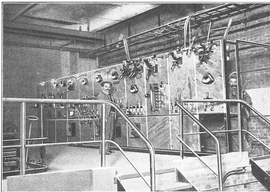
LE TABLEAU PRINCIPAL DE DISTRIBUTION DE L'ÉLECTRICITÉ DANS LE THÉÂTRE
