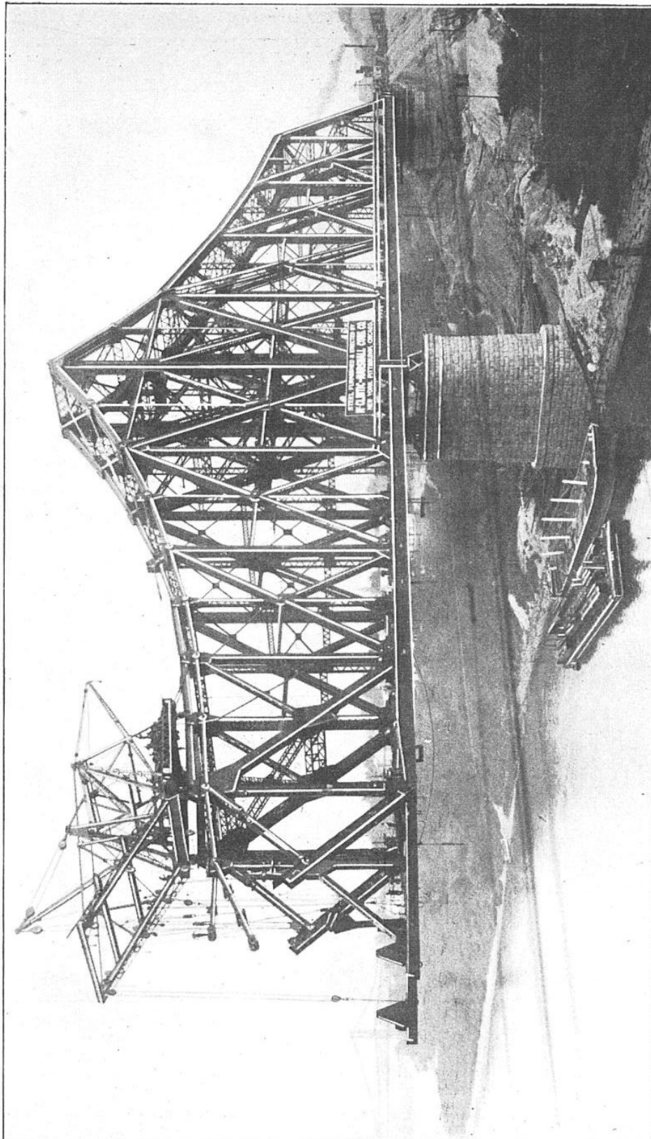
Le pont étant parvenu à un état d'avancement plus complet, on voit le système formé par une ferme de rive et par une moitié de la ferme centrale, en équilibre sur la pile nord avec un ensemble analogue reposant sur la pile sud au moment où l'on commence la construction du tablier de raccordement. La grue de montage, maintenue en équilibre par un contrepois composé de gueuses de fonte, permet de travailler en porte à faux dans le vide; elle circule au moyen de galets de roulement sur un chemin courbe constitué par des larges plats rivés à la partie supérieure des deux poutres de rive.
