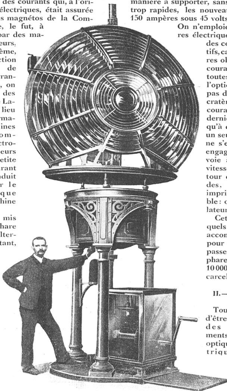
APPAREIL D'ÉCLAIRAGE DU PHARE DE GRAYS HARBOUR Ce feu-éclair de troisième ordre construit par les établissements Lepaute présente des éclats alternatifs blancs et rouges. La face représentée correspond à la lumière rouge.
