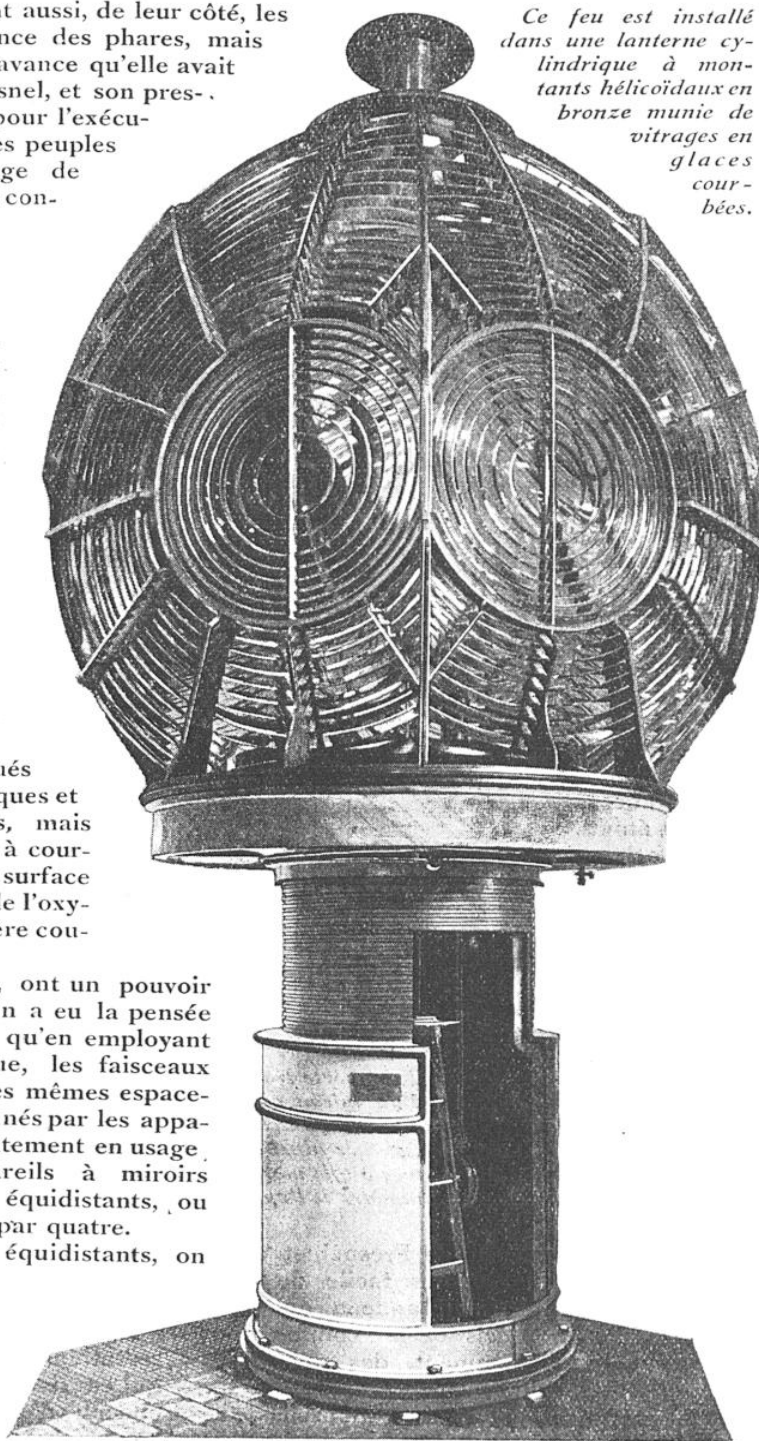
APPAREIL POUR PHARE DE PREMIER ORDRE.
