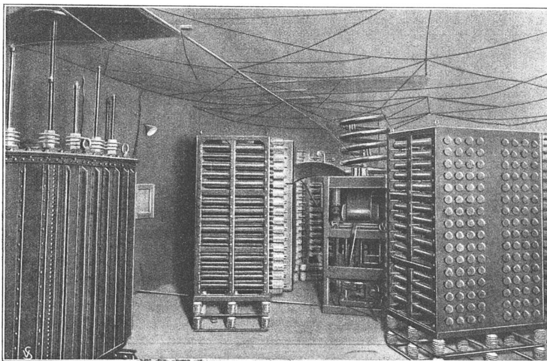
FIG. 7.- SALLE DE LA HAUTE TENSION ET DE L'ÉCLATEUR DU POSTE SOUTERRAIN DE LA TOUR EIFFEL. Lorsque le poste fonctionne, les étincelles éclatent dans cette salle avec un bruit formidable et il y est expressément interdit d'y pénétrer à cause du danger de mort qu'on y court.
