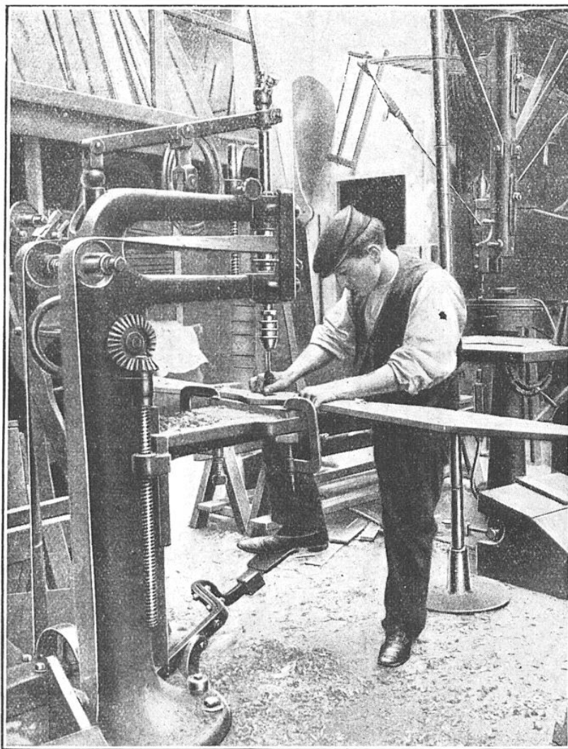
PERÇAGE DES PLANCHES QUI DOIVENT CONSTITUER L'HÉLICE
