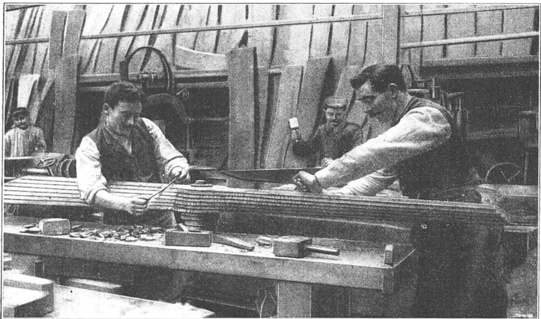
PREMIER ÉBAUCHAGE DE LA SURFACE DES PALES
