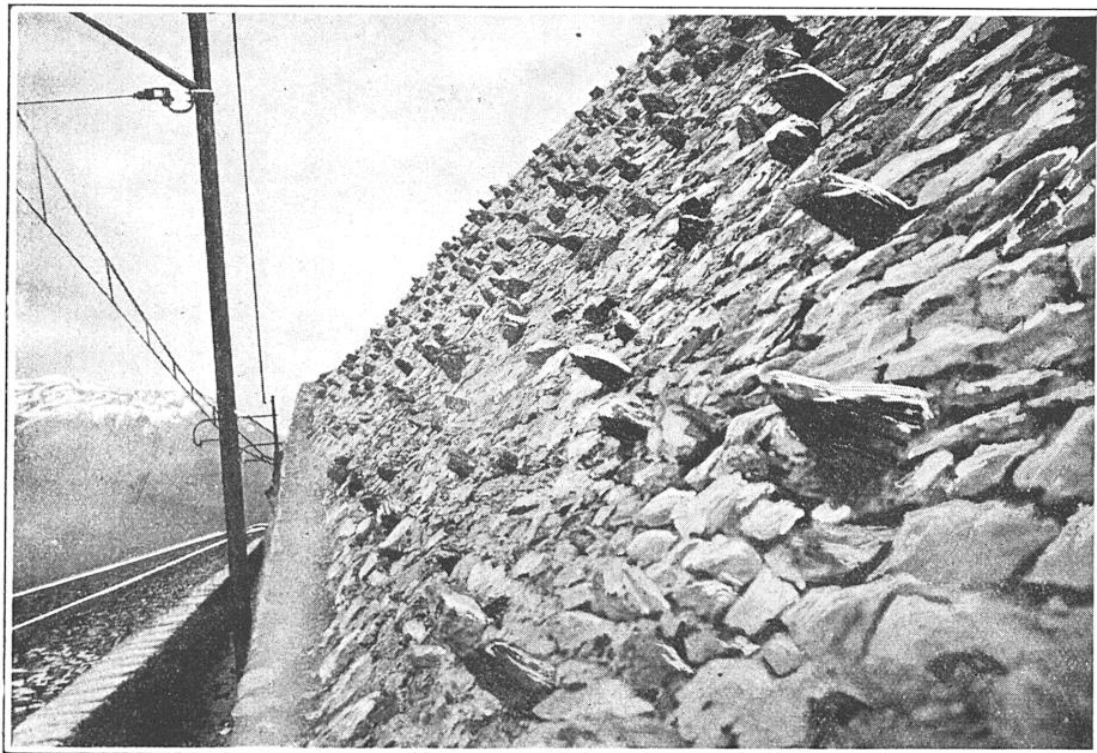
TRAVAUX DE PROTECTION CONTRE LES AVALANCHES ET LES ÉBOULIS AU SUD DU TUNNEL
