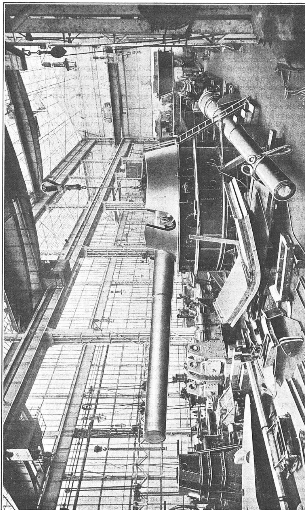
Atelier de montage de la maison Armstrong Whitworth, à Elswick (Angleterre), desservie par quatre ponts transbordeurs aériens, mus électriquement, à chemins de roulement superposés. Dans cet atelier, les tourelles cuirassées sont complètement assemblées comme elles le seront sur le navire, leurs mouvements sont essayés; les tourelles sont ensuite démontées et transportées à bord.
