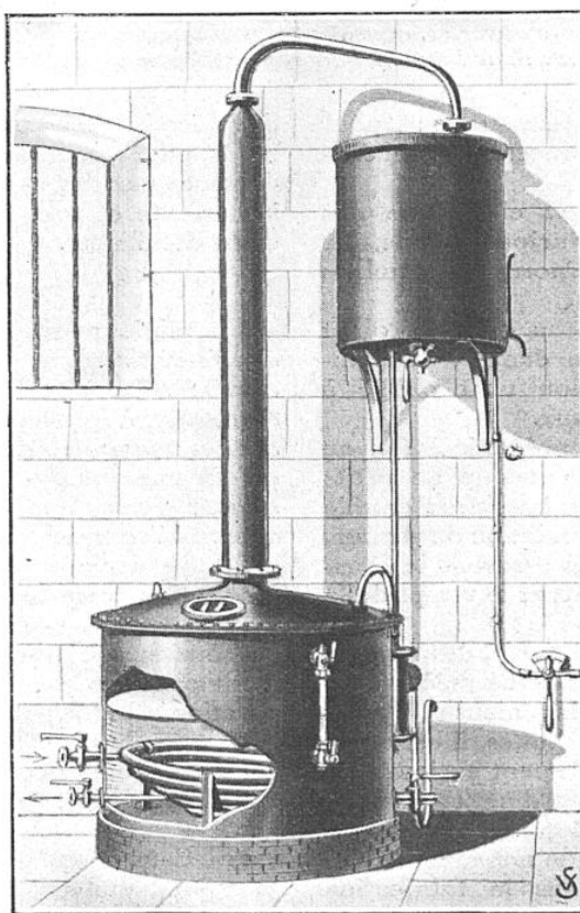
APPAREIL A FONCTIONNEMENT CONTINU POUR LA PRÉPARATION DE L'EAU DISTILLÉE
