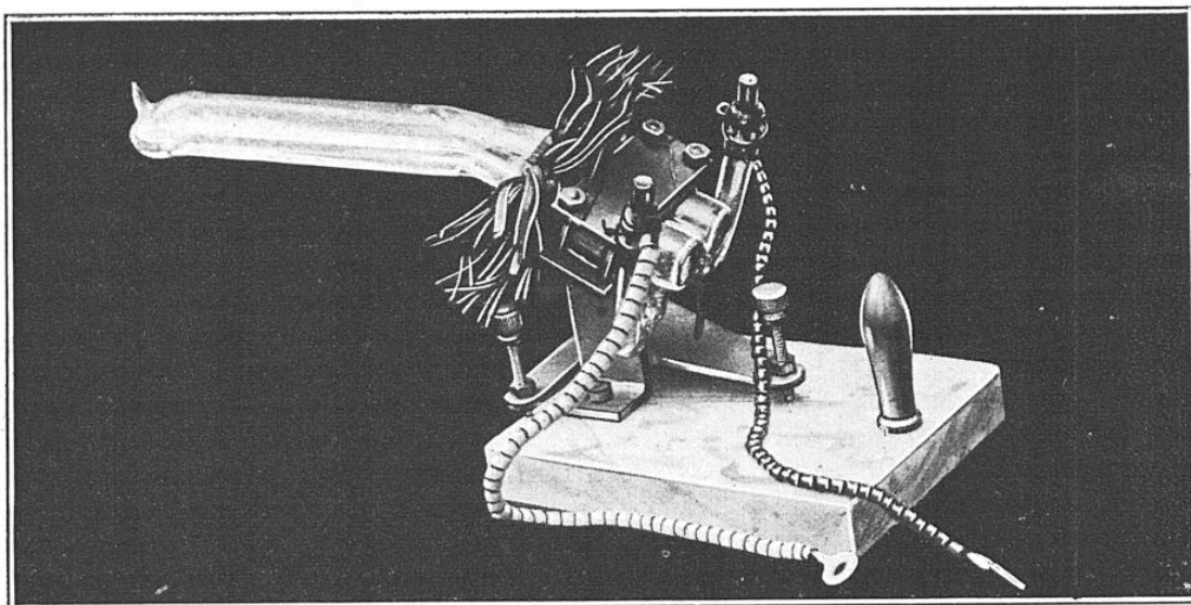
FIG. 4. — LAMPE A VAPEUR DE MERCURE, EN QUARTZ, D'UNE PUISSANCE EXTRÊME Cette lampe est construite pour un courant de 500 volts. Des microbes, placés jusqu'à une distance de 40 cm de cette lampe, sont tués par les rayons U. V. en moins d'une seconde.
