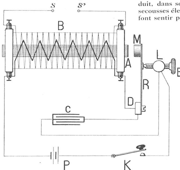
FIG. 2. — CONNEXIONS DE LA BOBINE DE RUHKORFF
