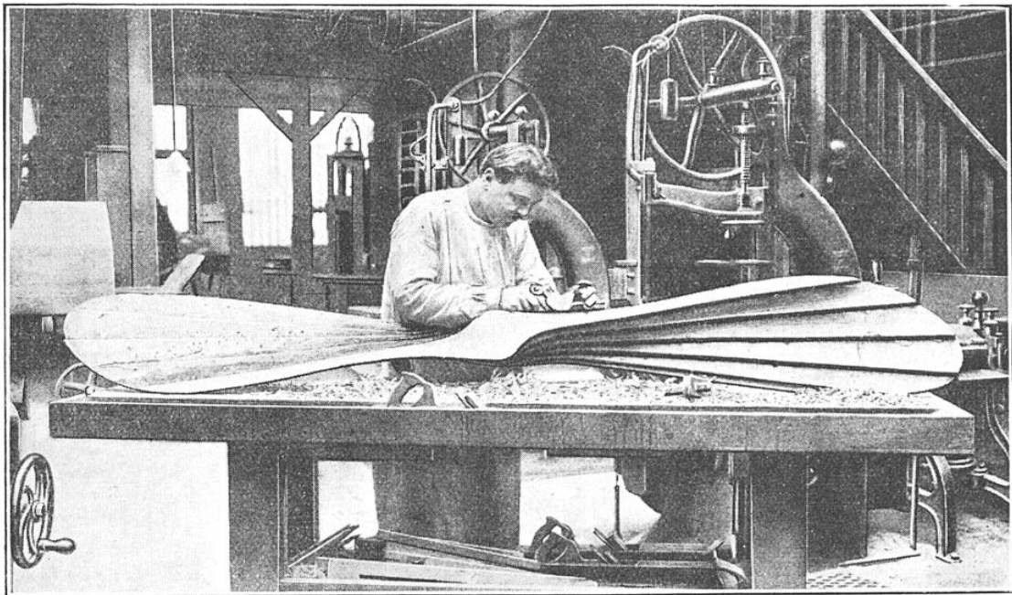
TAILLAGE SUIVANT GABARIT D'UNE HÉLICE D'AÉROPLANE
