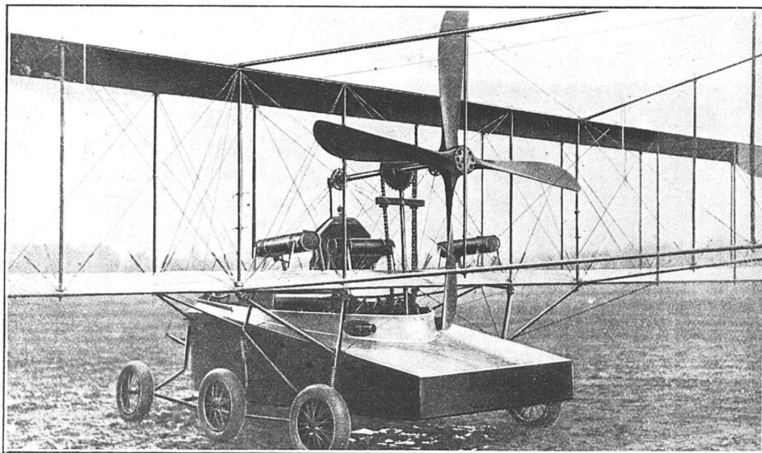
HÉLICE A QUATRE PALES MONTÉES SUR UN HYDROAVION
