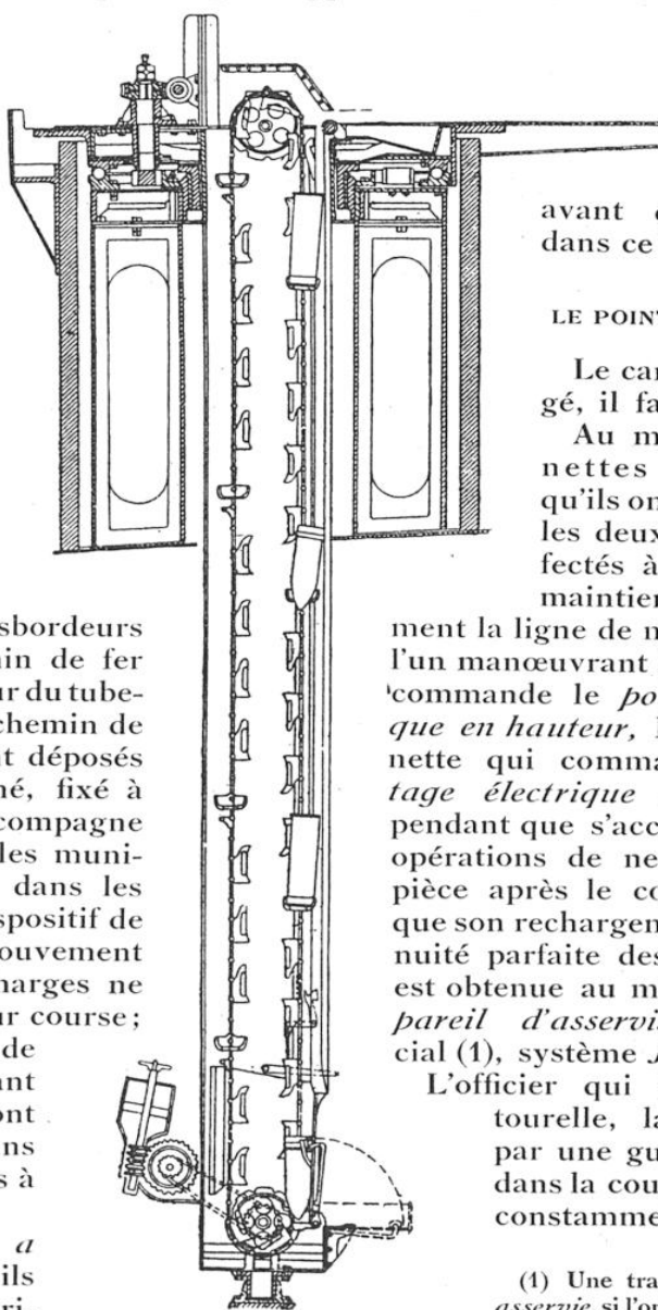
NORIA POUR CANONS DE 15 CM
