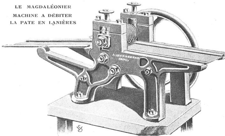
La masse pilulaire est fractionnée en lanières étroites ou magdaléons à l'aide d'une série de couteaux circulaires disposés verticalement.
