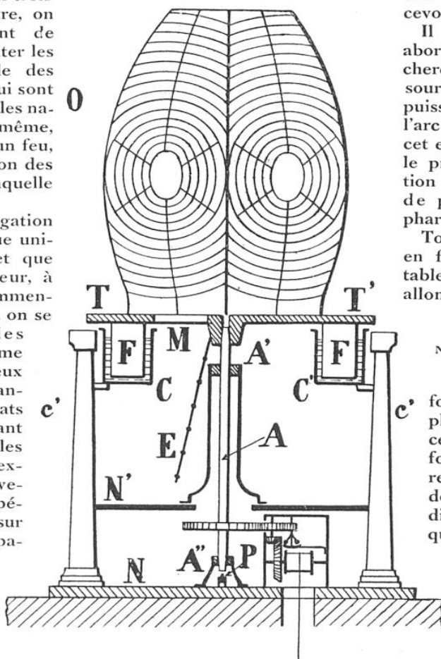
SCHEMA D'UN APPAREIL A ÉCLATS TOURNANT SUR FLOTTEUR A MERCURE
