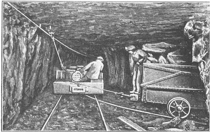
MANŒUVRE A LA MACHINE AU FOND DE LA MINE
