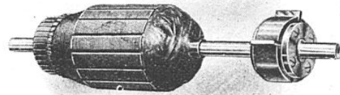
Vue de la poulie et du moteur débarrassés de leurs carters.
