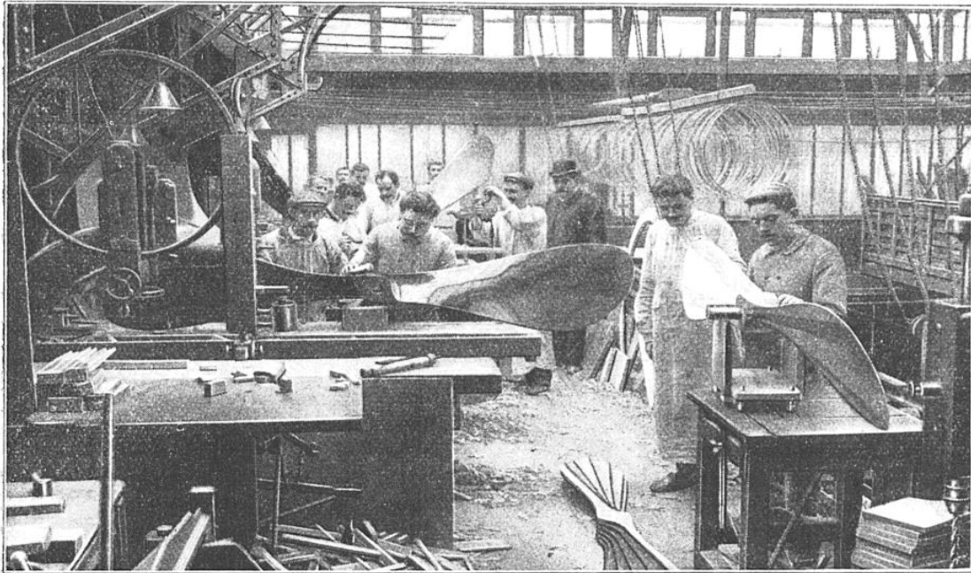
ATELIER DE CONSTRUCTION DES HÉLICES « P. A. »
