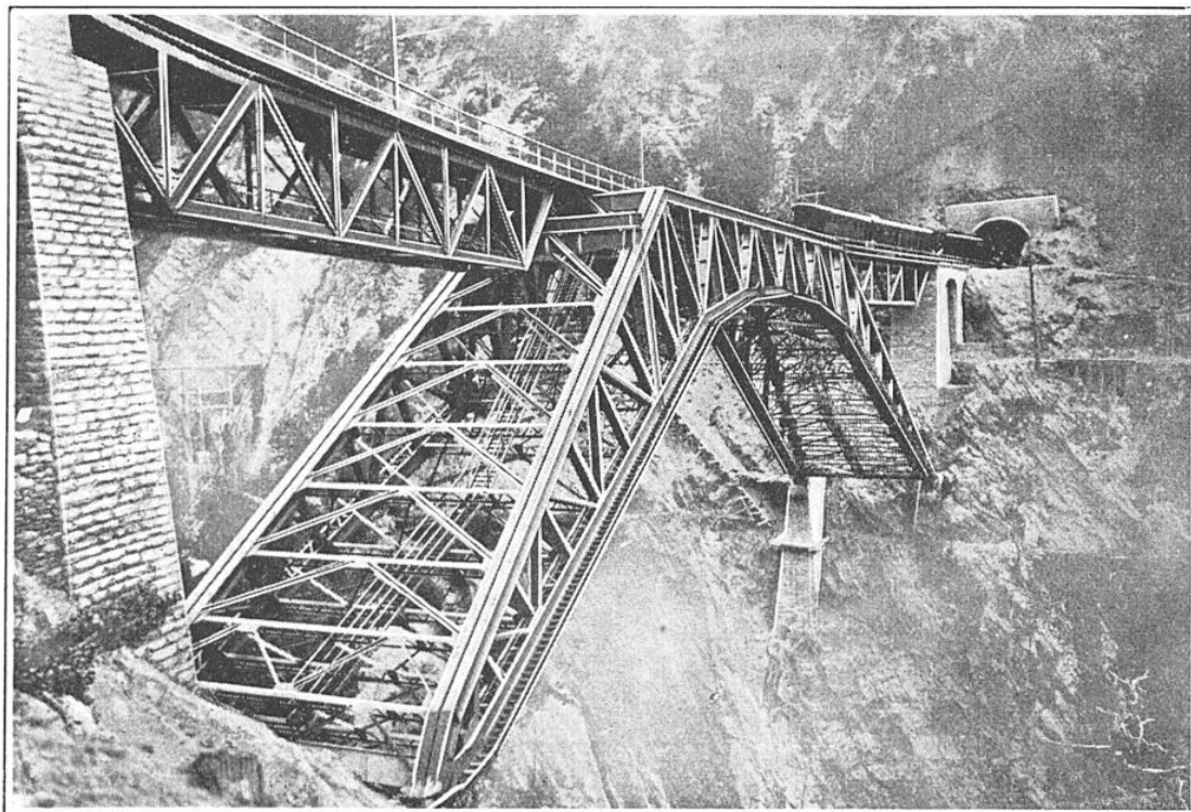
DEUX VUES DU VIADUC MÉTALLIQUE DU BIESCHTAL SUR LE VERSANT SUD
