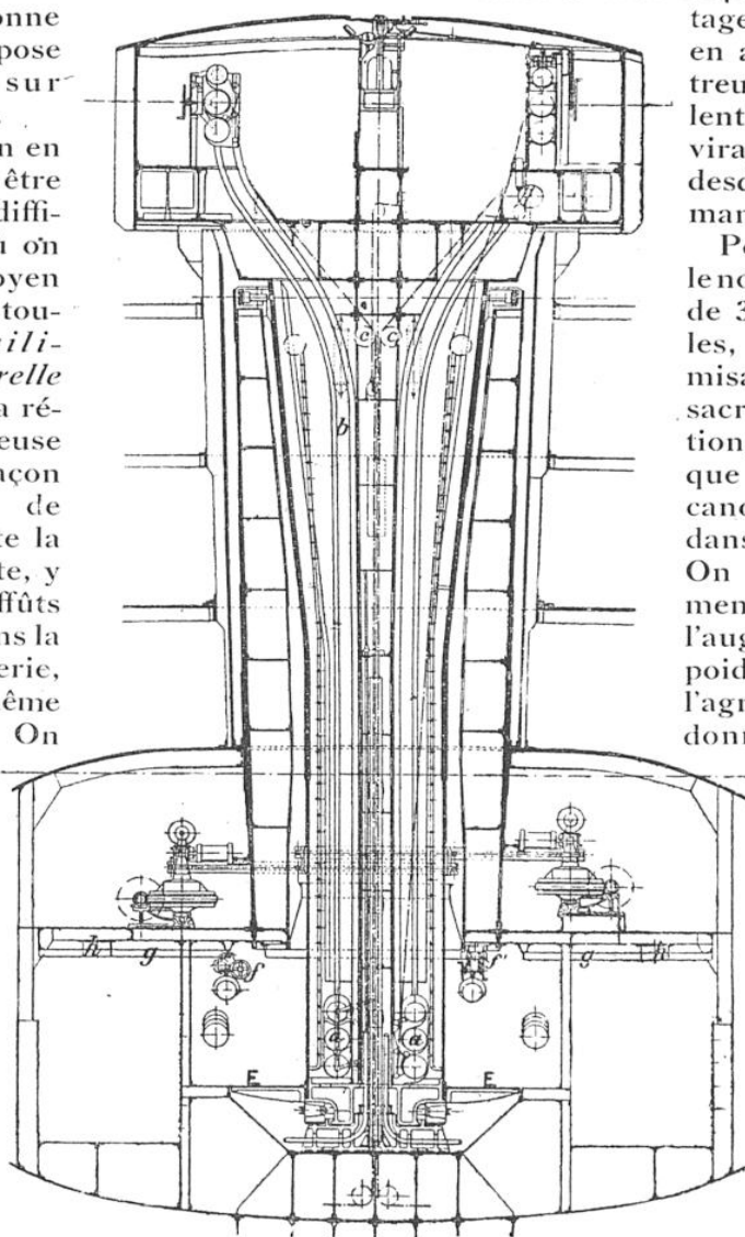
COUPE D'UNE TOURELLE FERMÉE A DEUX CANONS
