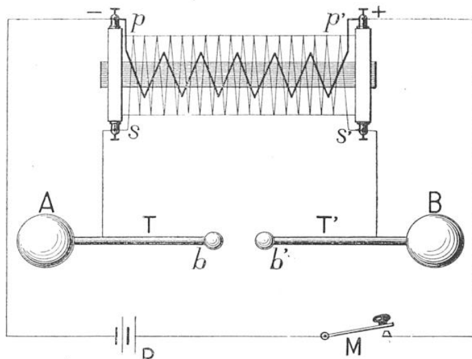
FIG. 1. — OSCILLATEUR DE HERTZ
