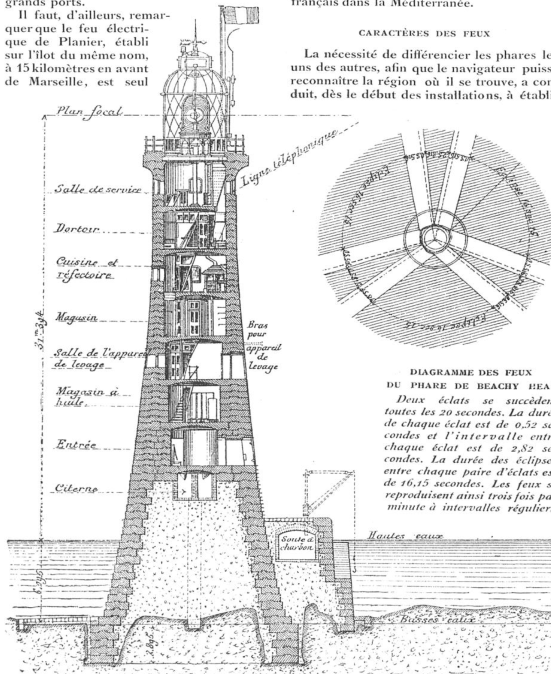
COUPE VERTICALE DU PHARE DE BEACHY HEAD (ANGLETERRE)
