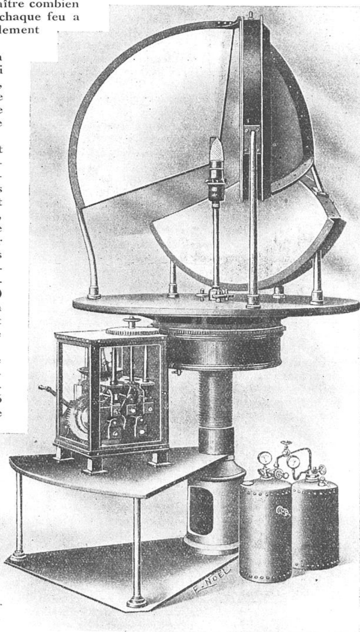
APPAREIL A RÉFLECTEURS MÉTALLIQUES. GROUPE DE 3 ÉCLATS
