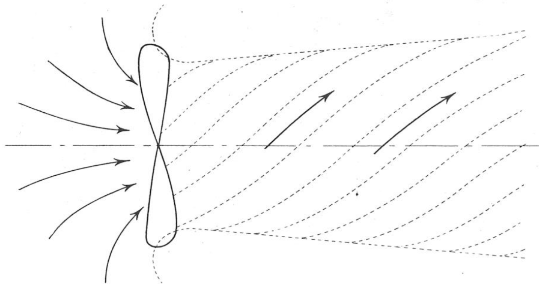
MARCHE DES FILETS D'AIR ASPIRÉS ET REFOULÉS PAR L'HÉLICE
