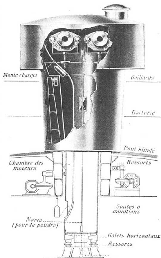
TOURELLE LOUGHER A DEUX CANONS
