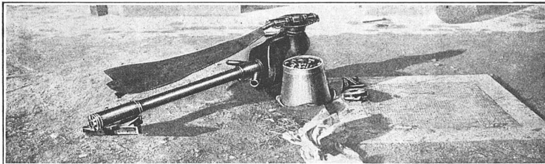
L'hélice mécanique qui a causé l'accident du dirigeable « République ». La pale qui manque s'est détachée du moyeu et a crevé l'enveloppe.
