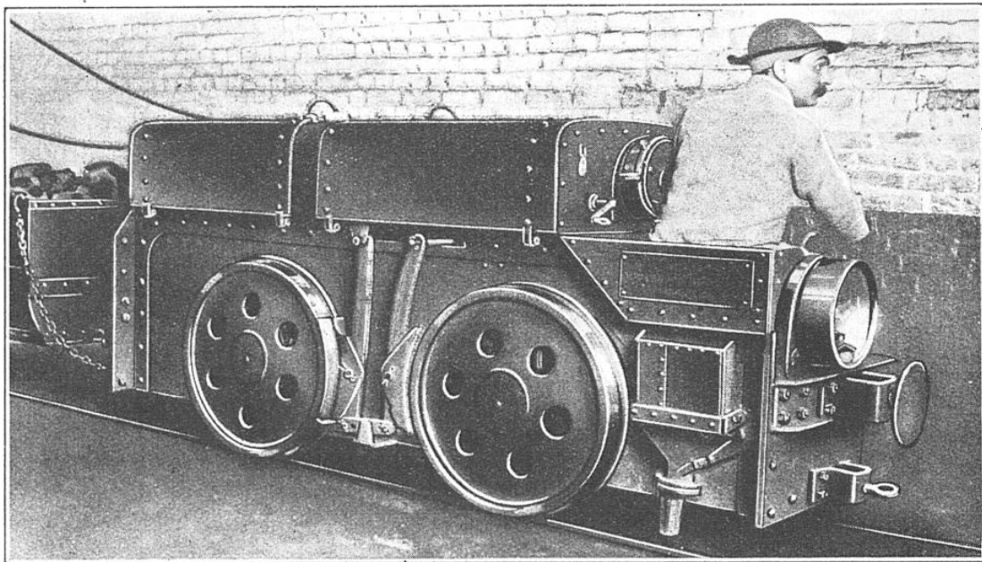
LOCOMOTIVE ÉLECTRIQUE SYSTÈME SIEMENS
