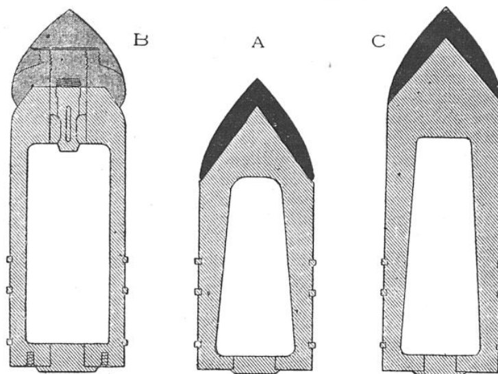
PROJECTILES DE LA GROSSE ARTILLERIE DE BORD FRANÇAISE
