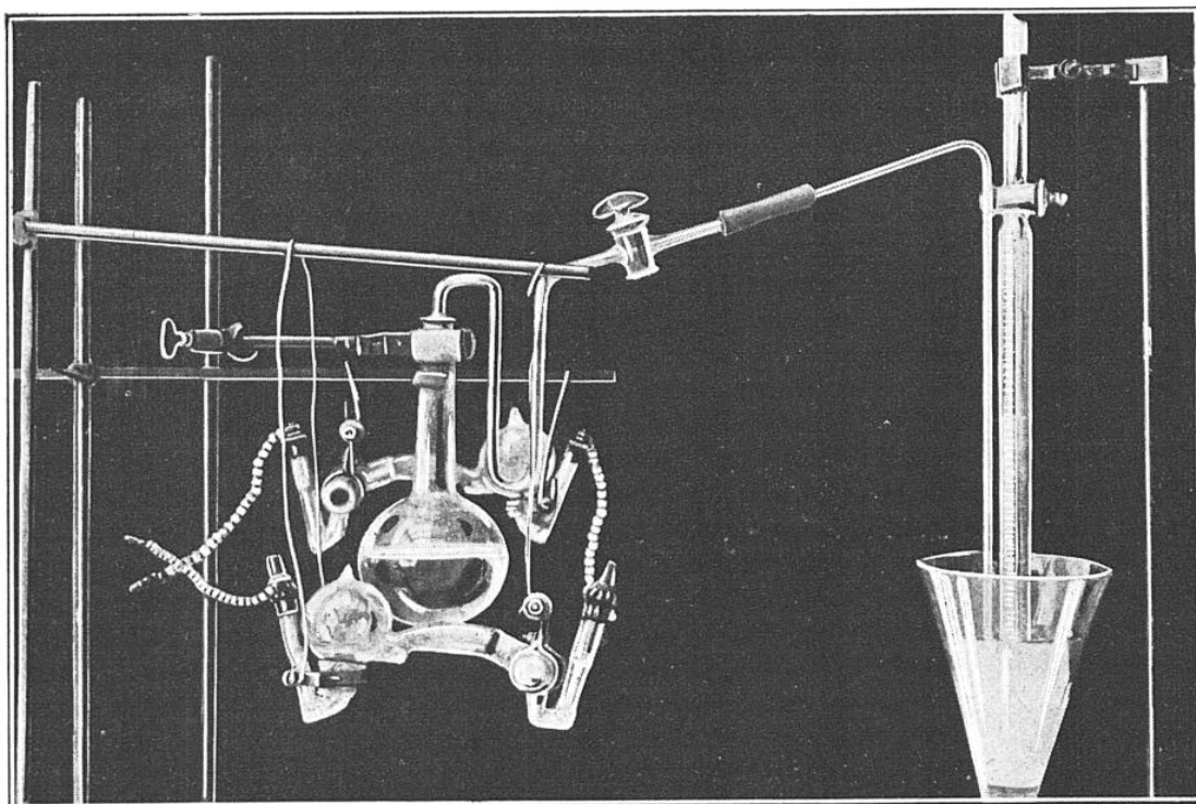
FIG. 5. — DISPOSITIF PERMETTANT D'ÉTUDIER LA FERMENTATION PRODUITE PAR LES RAYONS U. V. Une solution de sucre de fruits — la lévulose — est placée dans un ballon en quartz qui se trouve entre deux lampes à mercure. Il se produit de l'aldéhyde formique, de l'alcool et de l'oxyde de carbone. Les rayons U. V. réalisent donc une transformation du sucre qui n'avait pu être produite jusqu'alors que par des cellules vivantes ou par des ferments.
