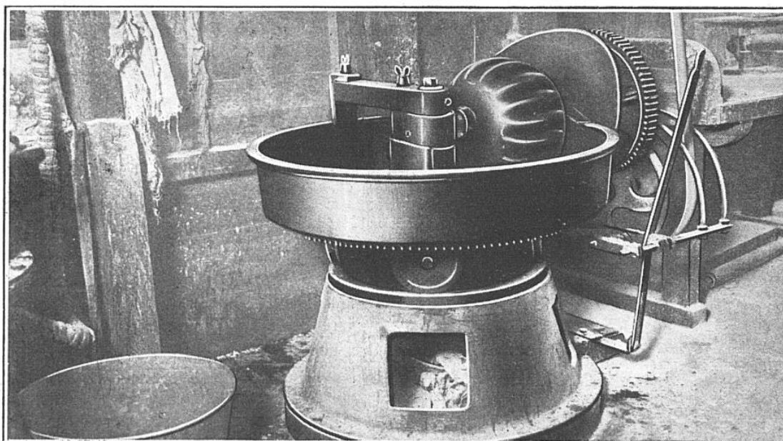
MACHINE A MALAXER LES PÂTES A PILULES
