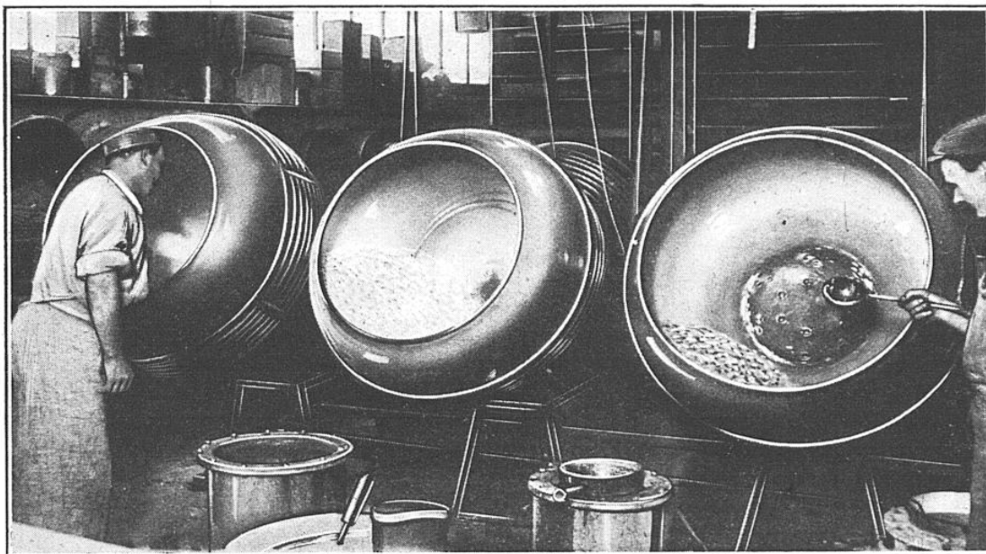
APPAREILS POUR L'ENROBAGE DES DRAGÉES ET LES PILULES A REVÊTEMENT DE SUCRE
