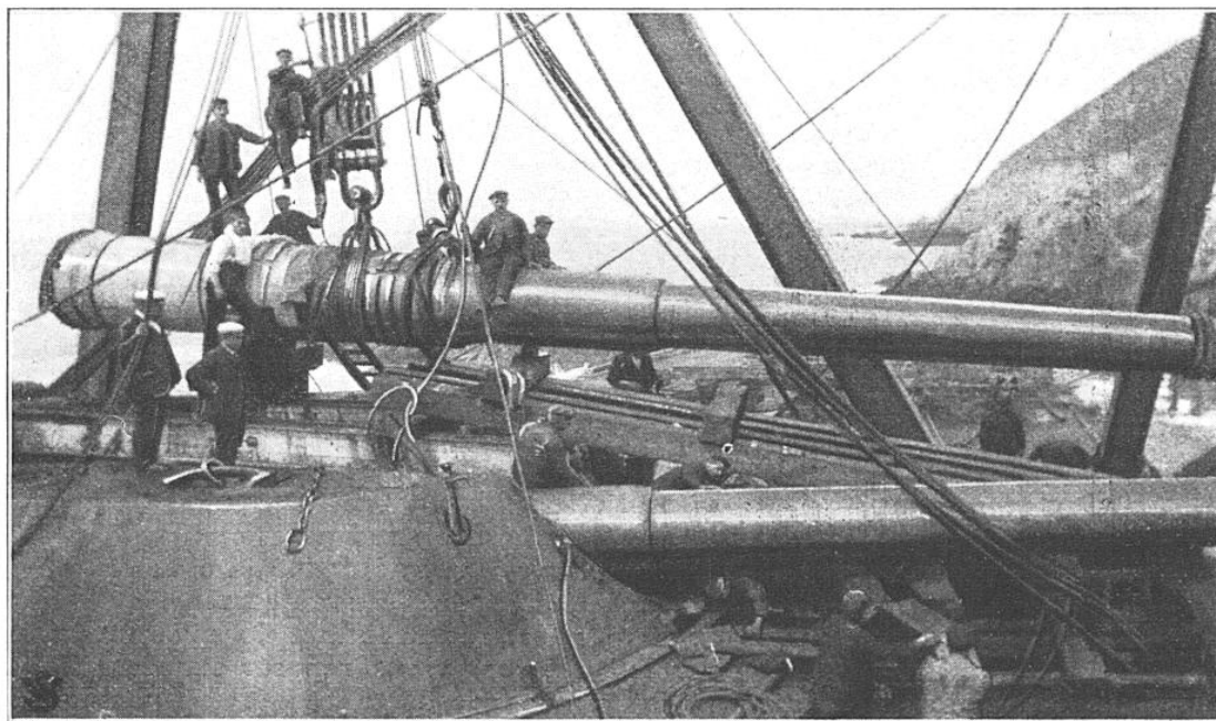
MISE A BORD D'UN CANON DE TRENTE CENTIMÈTRES
