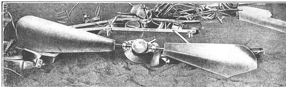
Le dirigeable « République » comportait deux hélices. Voici la deuxième encore presque intacte après et malgré l'accident.
