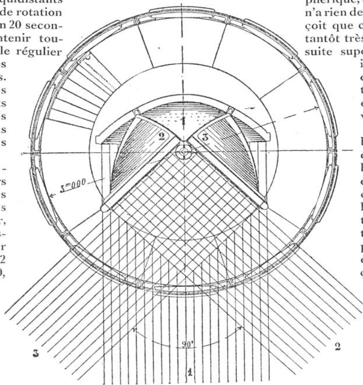
FEU-ÉCLAIR A GROUPE DE 3 ÉCLATS
