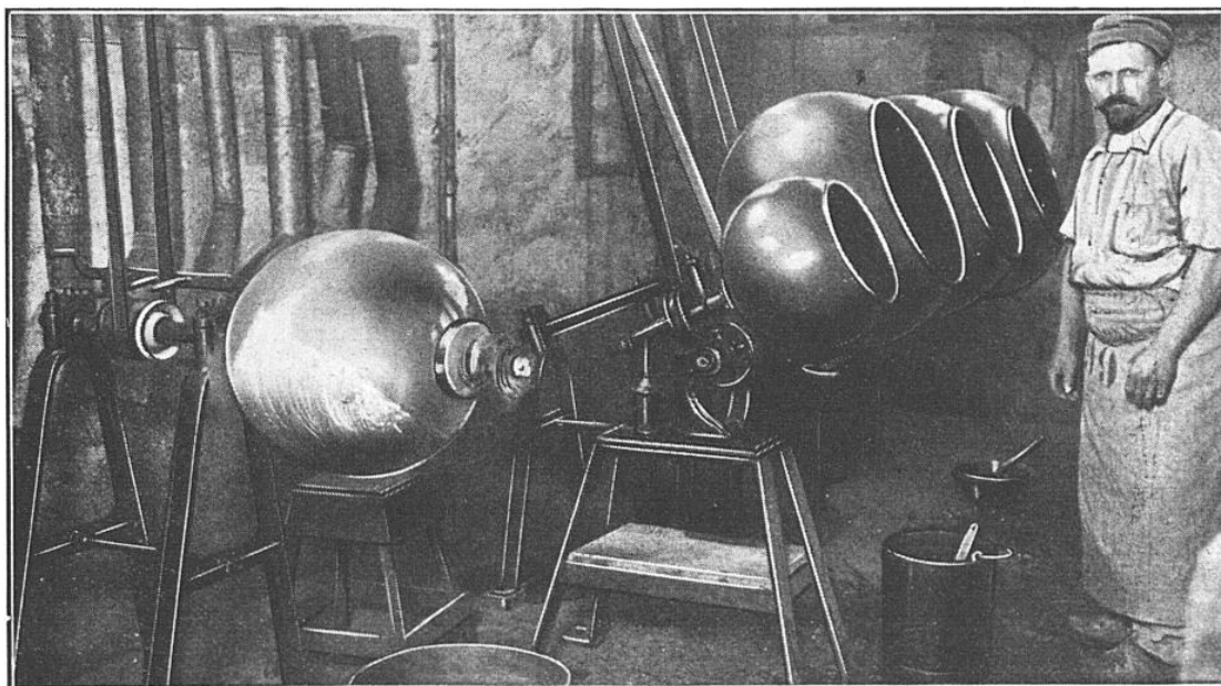
AUTRE VUE DU MÊME ATELIER AVEC, A GAUCHE, LA SPHÈRE D'ARGENTURE
