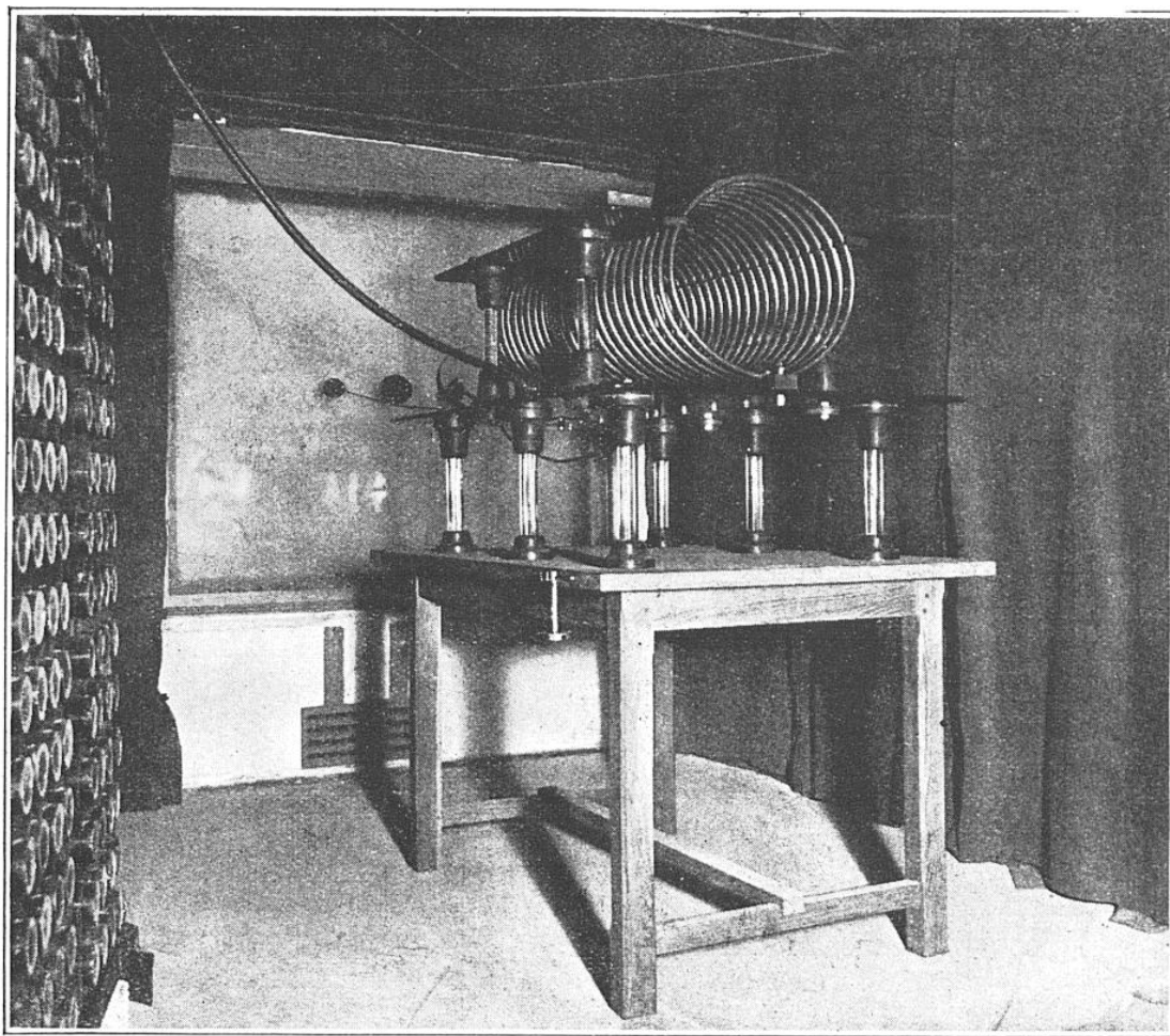
FIG. 5. — ARRIVÉE DE L'ANTENNE DANS LE POSTE SOUTERRAIN DE LA TOUR EIFFEL On la voit entrer au centre du mur et elle est reliée à une bobine de self-induction, dite bobine d'accord, au moyen d'un curseur qui permet d'intercaler un nombre variable de spires.
