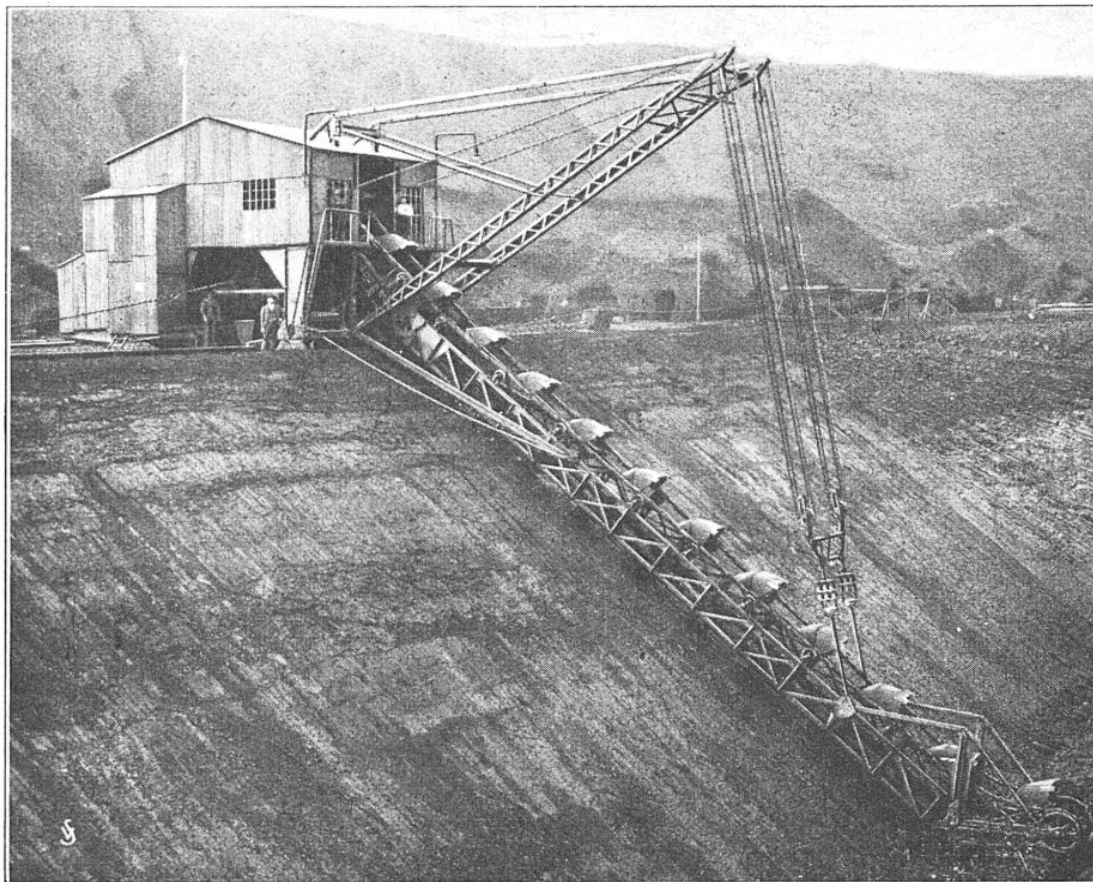
EXCAVATEUR A GODETS TRAVAILLANT A SEC DANS UNE TRANCHEE.
