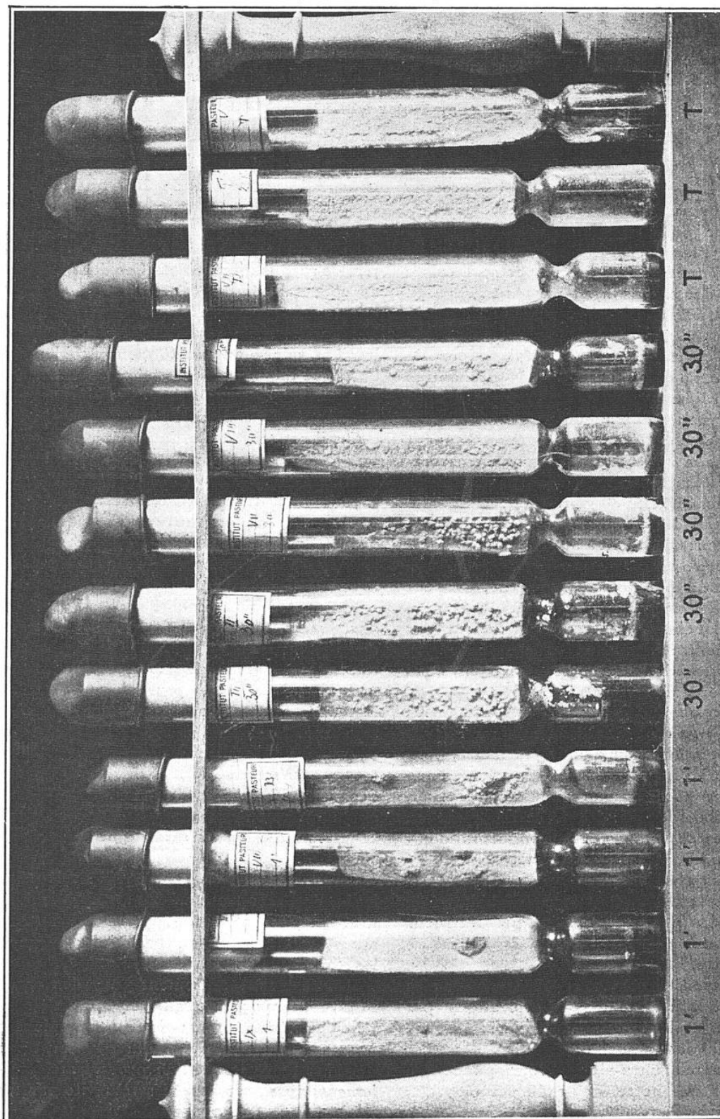
FIG. 1. — SÉRIE DE TUBES A ESSAIS MONTRANT L'INFLUENCE MICROBICIDE DES RAYONS ULTRA-VIOLETS (voir page 179) Les tubes de gauche, qui ont été exposés aux rayons U. V. pendant une minute, ne contiennent plus de bacilles vivants.
