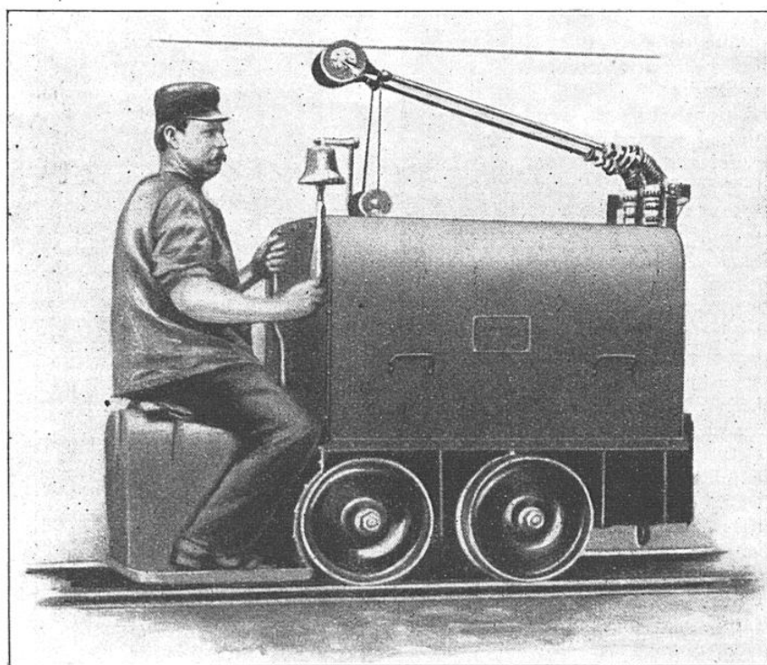
LOCOMOTIVE ÉLECTRIQUE SYSTÈME SCHUCKERT
