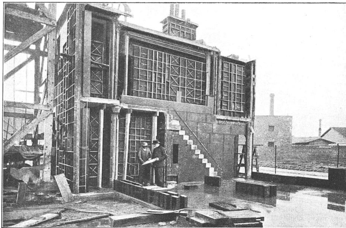
VUE D'UNE DES FACES INTERNES PENDANT L'ASSEMBLAGE DES PLAQUES DU MOULE
