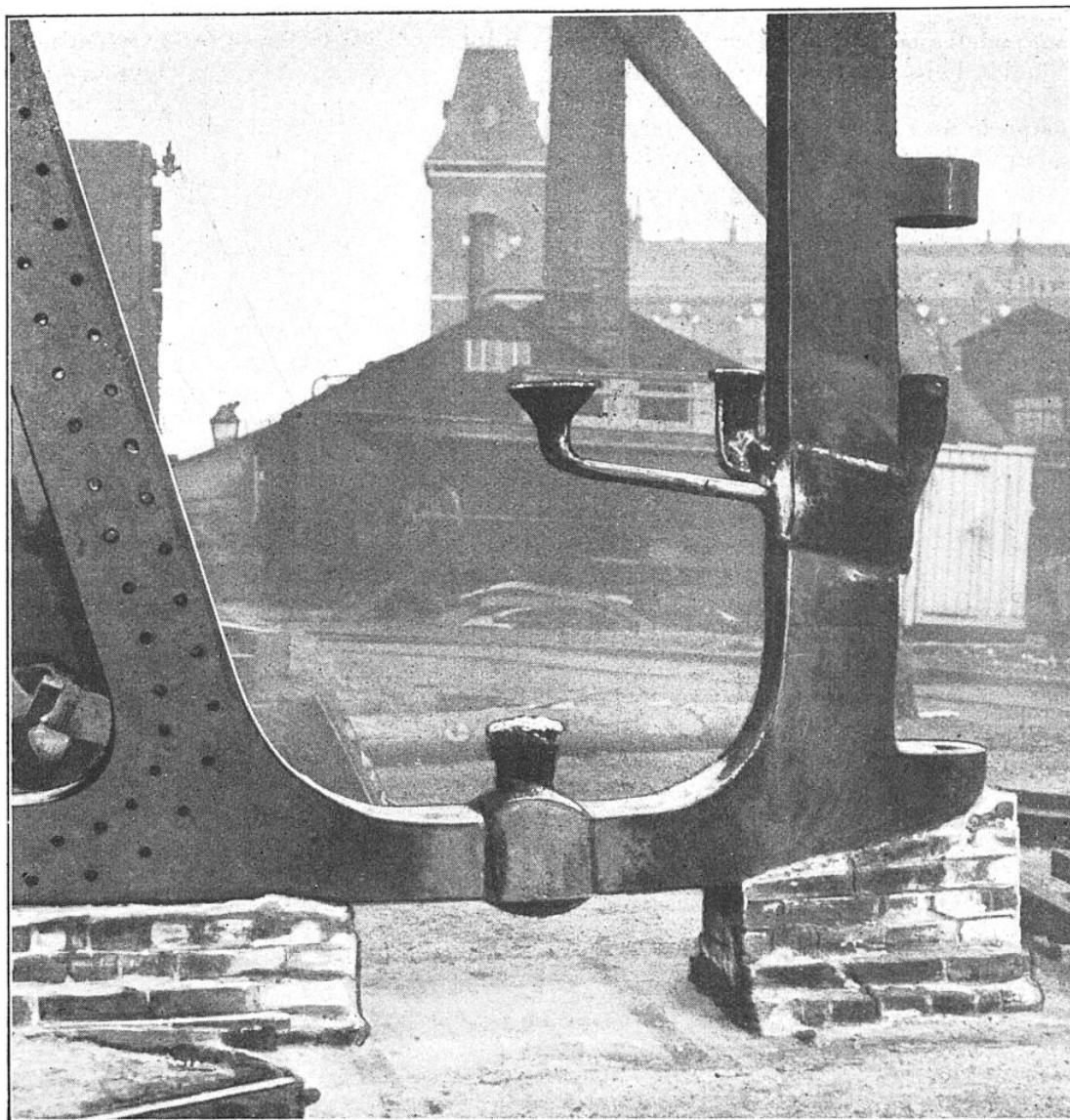
VUE D'UN ÉTAMBOT DE NAVIRE APRÈS RÉPARATION PAR SOUDURE
