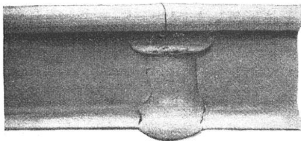
JOINT GOLDSCHMIDT SOUDÉ POUR RAILS
