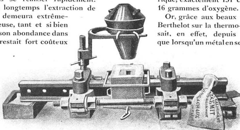
DISPOSITIF POUR LE SOUDAGE DE DEUX RAILS BOUT A BOUT DANS TOUTE LEUR SECTION
