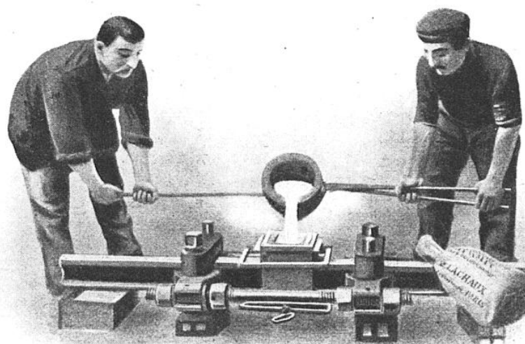
DISPOSITIF POUR SOUDURE SANS BOURRELETS
