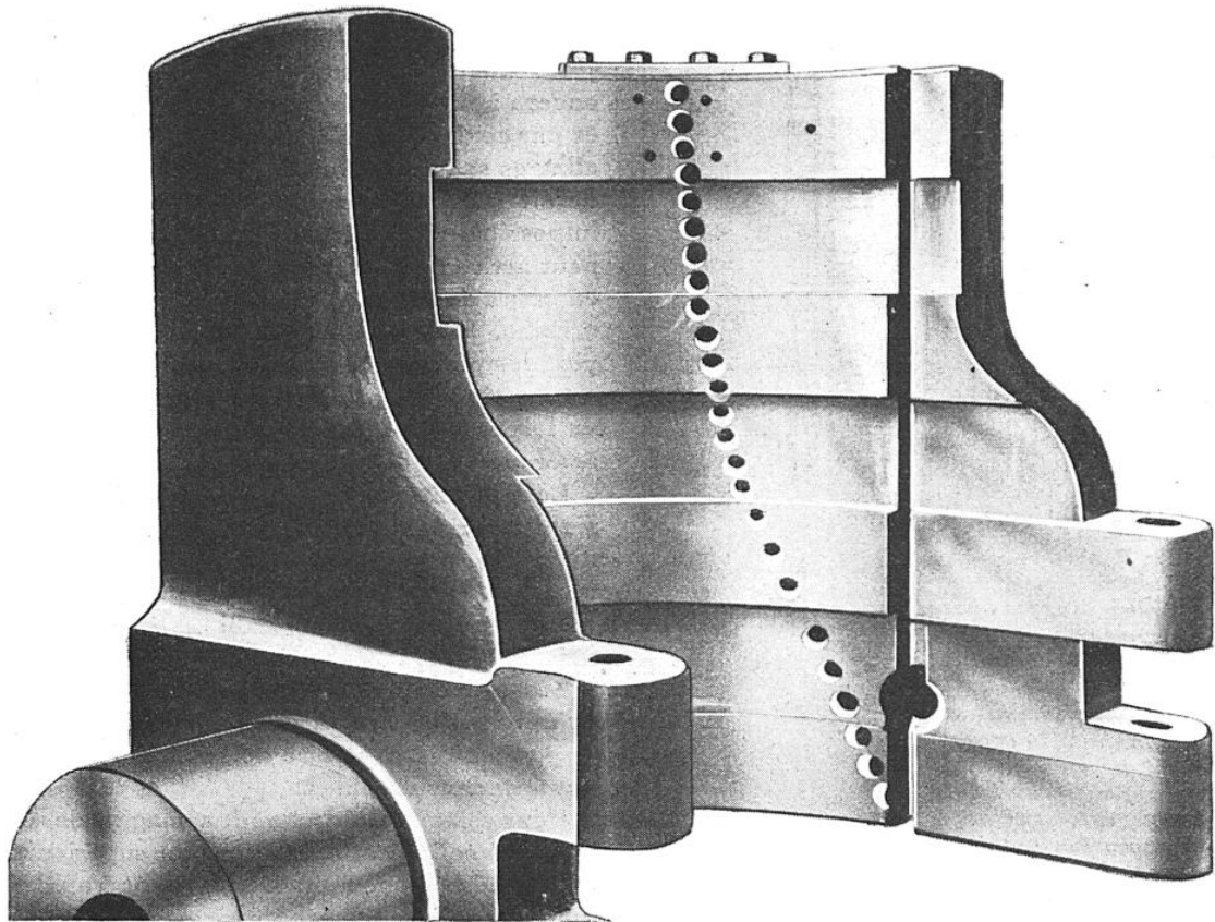
MANCHON A TOURILLONS D'UN CANON DE 305 MILLIMÈTRES ROMPU, PRÉPARÉ POUR ÊTRE SOUDÉ Des trous ont été percés tout le long de la fissure afin de permettre au fer thermit de pénétrer dans la pièce brisée sous une épaisseur suffisante pour constituer une soudure homogène et solide.
