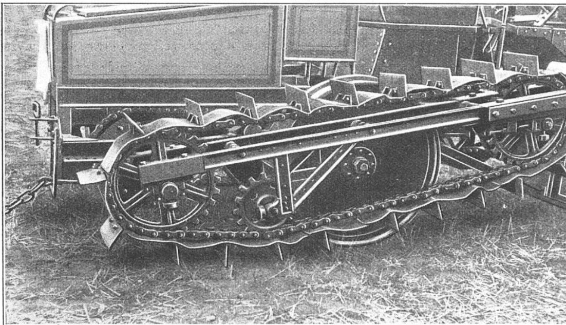
DÉTAILS DE LA CHAÎNE MOTRICE DU TRACTEUR LEFEBVRE
