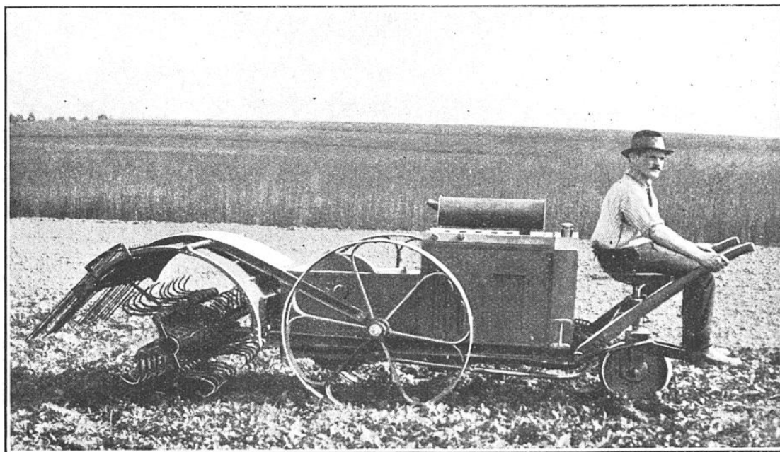
LE MOTOCULTEUR TYPE « VIGNERON » OU « MARAICHER »
