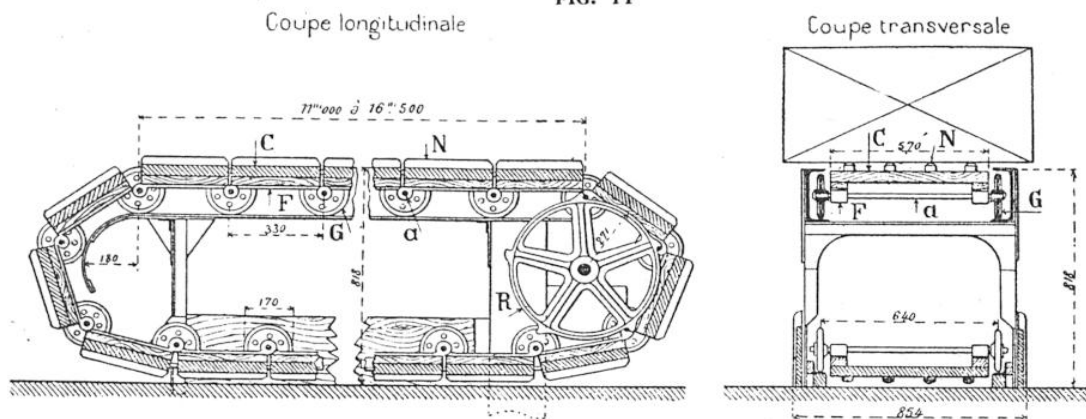
Coupe longitudinale et transversale d'un banc mobile. L'appareil est constitué par une chaîne de chariots C roulant sur des galets G. Chaque chariot est articulé au suivant par l'essieu a des galets communs. R roue motrice ; F longeron ; a essieu ; G galet ; N demi-fer rond.
