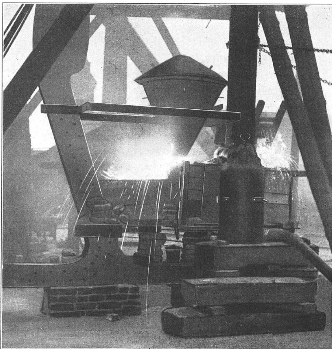
CHANTIER DE COULÉE INSTALLÉ POUR L'OPÉRATION REPRÉSENTÉE PAGES 168 ET 173
