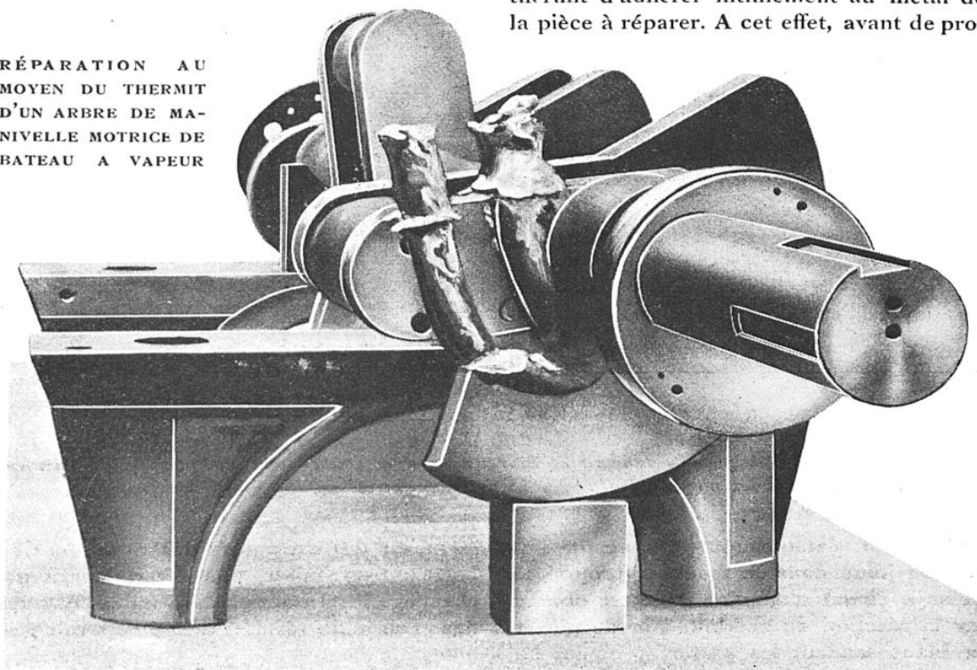
L'emploi du thermit a permis de sauver l'arbre et de le remettre en service au bout de quelques jours, dans d'excellentes conditions de sécurité.
