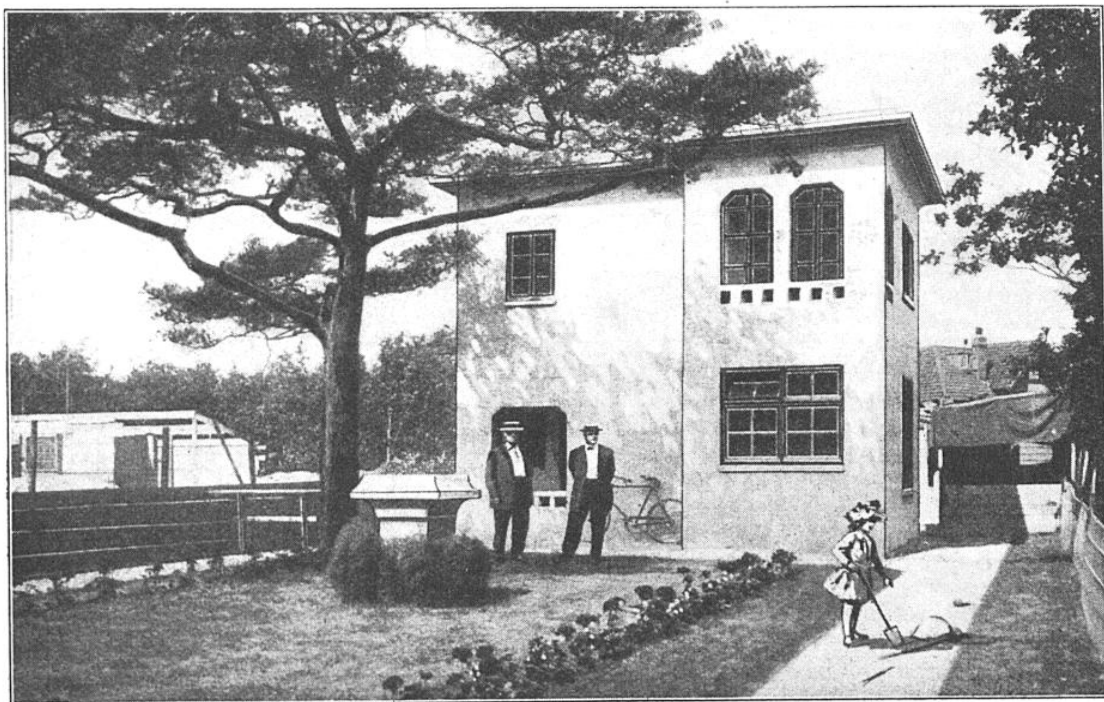
VUE DE LA MAISON MOULÉE DE SANTPOORT, COMPLÈTEMENT TERMINÉE
