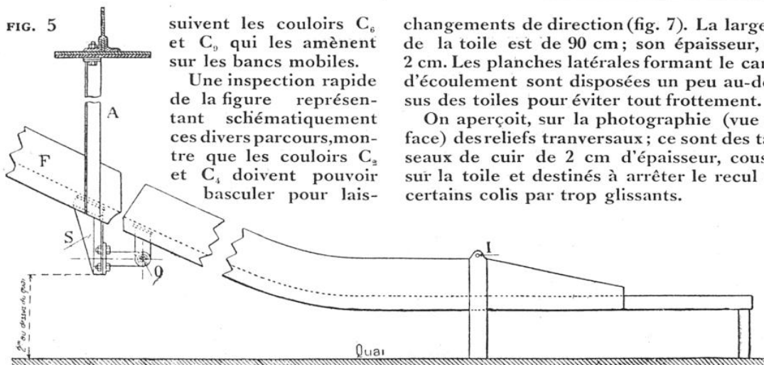
Schéma montrant l'articulation des grands couloirs mobiles, qui permet, lorsque ces couloirs restent inutilisés, de les relever afin de laisser plus d'espace libre sur le quai.
