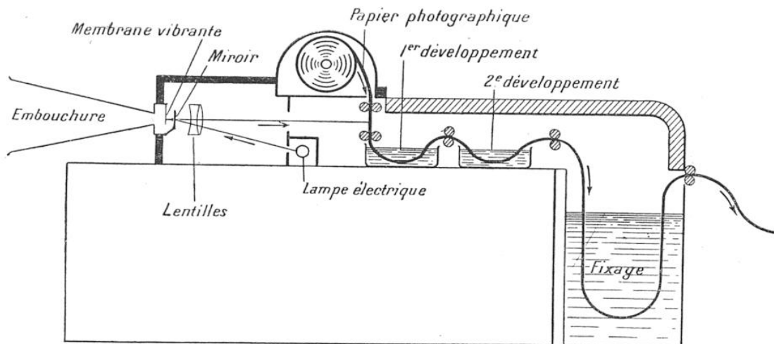
COUPE SCHÉMATIQUE DE L'APPAREIL QU'EMPLOIE M MARAGE POUR PHOTOGRAPHIER LA VOIX
