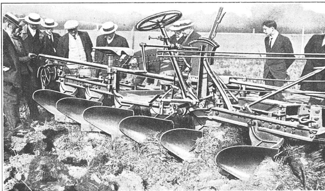
VUE DES SOCS ET DES COMMANDES D'UNE MOTOCHARRUE
