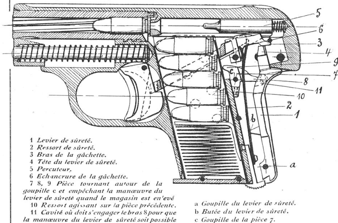
FIG. 6. — LE MÉCANISME DE SÛRETÉ DANS LA POSITION DU TIR ET LE PERCUTEUR A L'ABATTU
