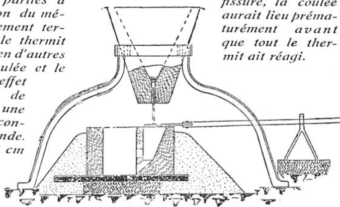
CREUSET AUTOMATIQUE. DÉBOUCHAGE DU TROU DE COULÉE
