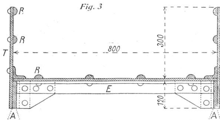
COUPE TRANSVERSALE D'UN COULOIR DE DESCENTE
