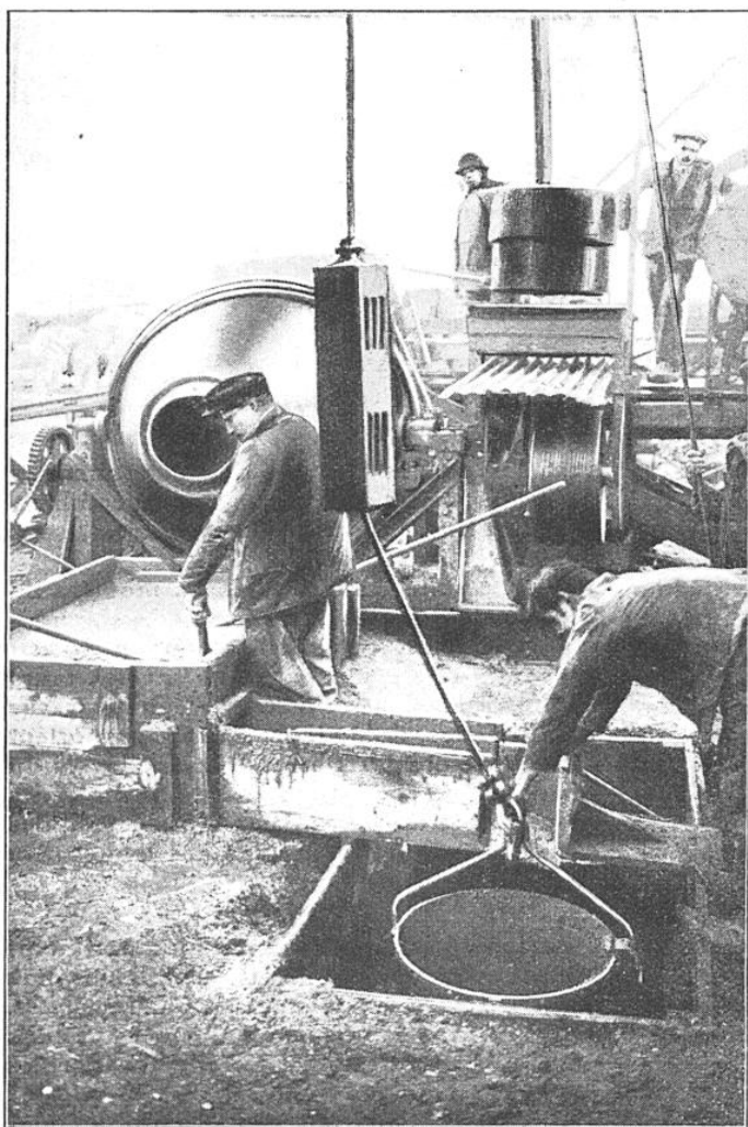
CHANTIER DE PRÉPARATION DU BÉTON FLUIDE
