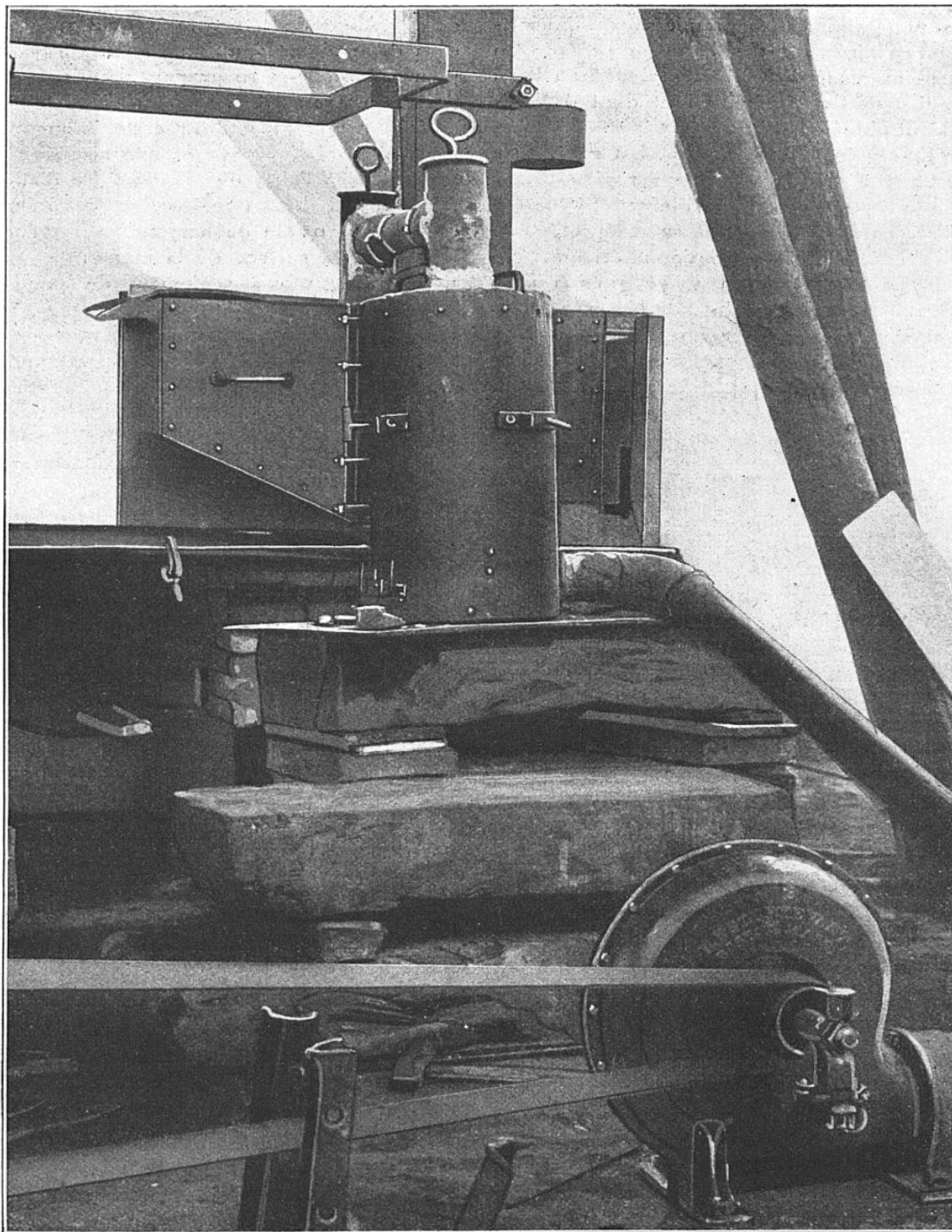
SÉCHAGE DU MOULE SERVANT A LA PRÉPARATION D'UN ÉTAMBOT DE NAVIRE
