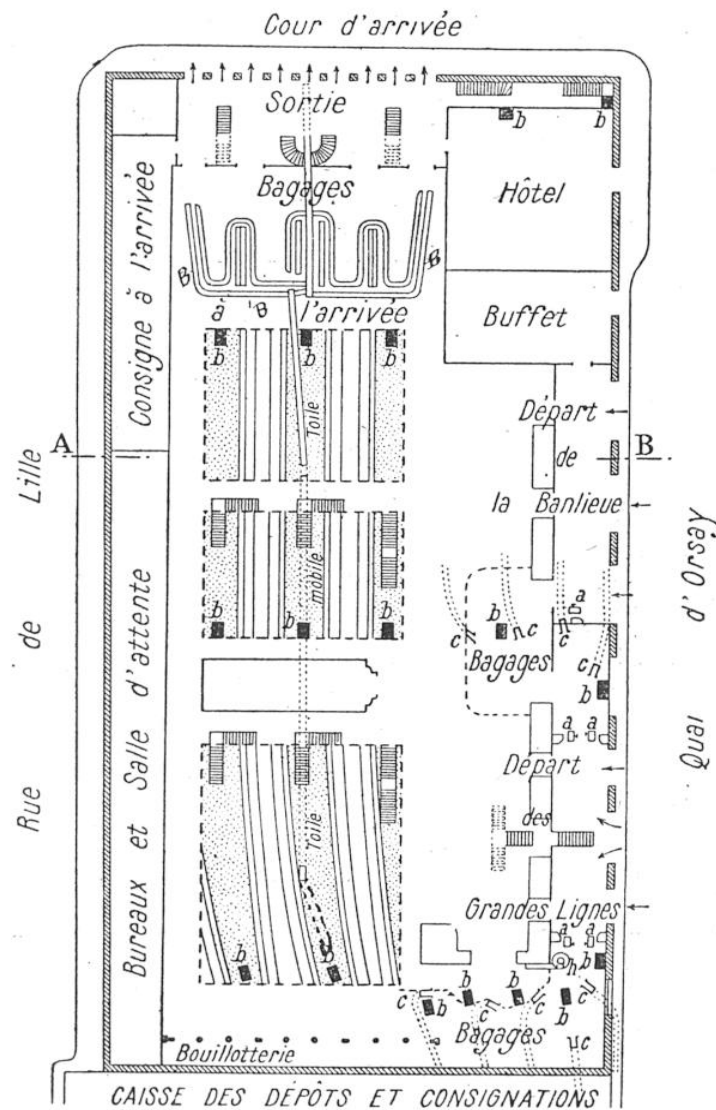
Plan du Rez-de-Chaussée (Fig. 2)
