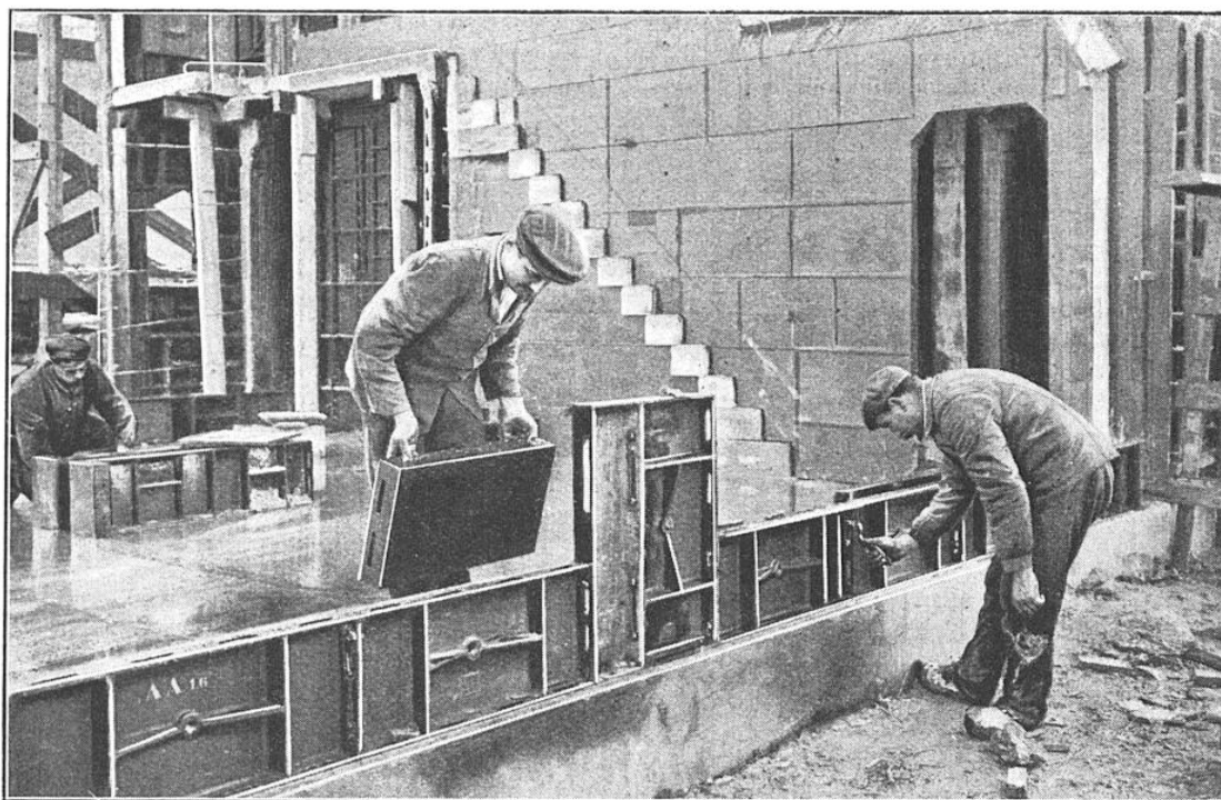
ASSEMBLAGE DES PREMIÈRES PLAQUES DEVANT CONSTITUER L'UNE DES FACES DE LA MAISON
