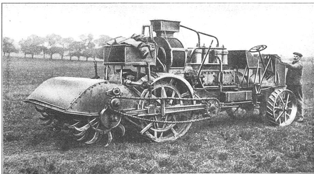
LABOUREUSE-PIOCHEUSE ARRÊTÉE ET AU TRAVAIL
