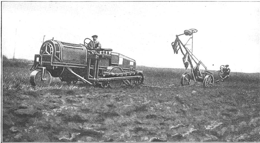
TRACTEUR AUTOMOBILE LEFEBVRE REMORQUANT UNE CHARRUE A BASCULE
