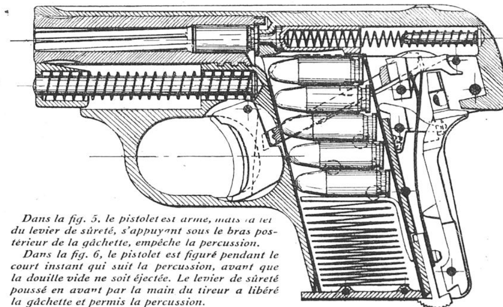
FIG. 6. — LE MÉCANISME DE SÛRETÉ DANS LA POSITION DU TIR ET LE PERCUTEUR A L'ABATTU
