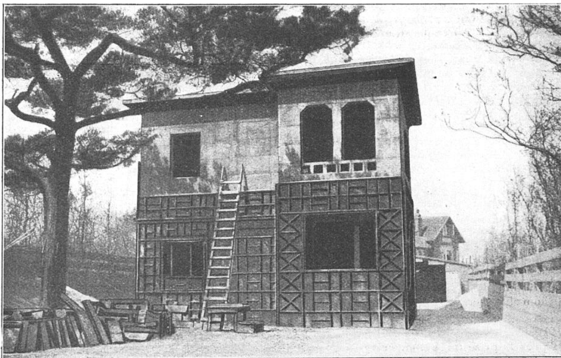
LE DÉMOULAGE DE LA MAISON COULÉE EN BÉTON, ÉDIFIÉE A SANTPOORT (HOULANDE)
