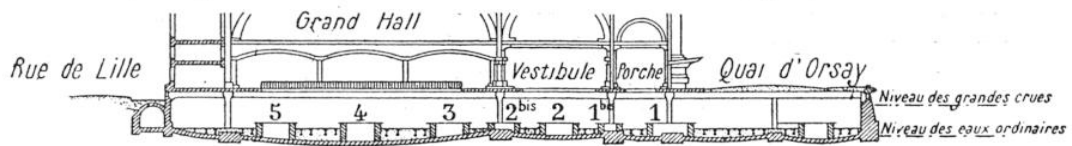
Coupe transversale suivant AB (Fig. 1)
