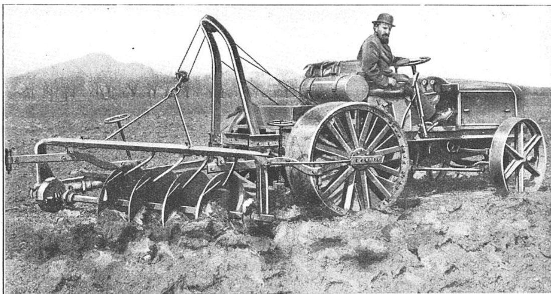
CHARRUE AUTOMOBILE A DISQUES SYSTÈME GILBERT
