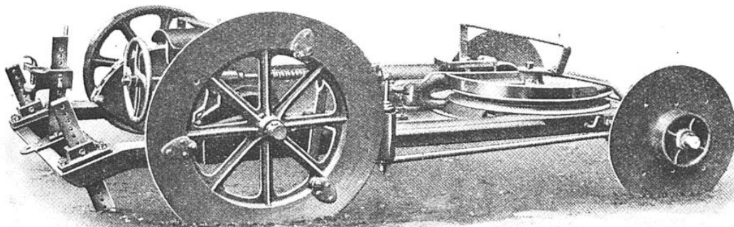
ANCRE AUTOMATIQUE POUR LE LABOURAGE A CABLE AVEC LOCOMOBILE UNIQUE
