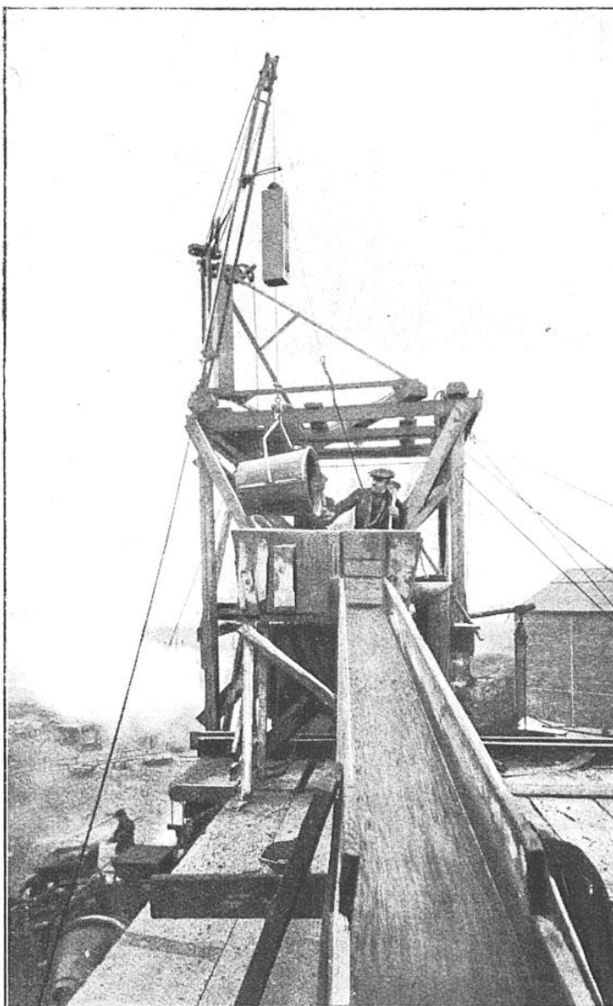
LA COULÉE DU BÉTON ENTRE DEUX PAROIS DE FONTE
