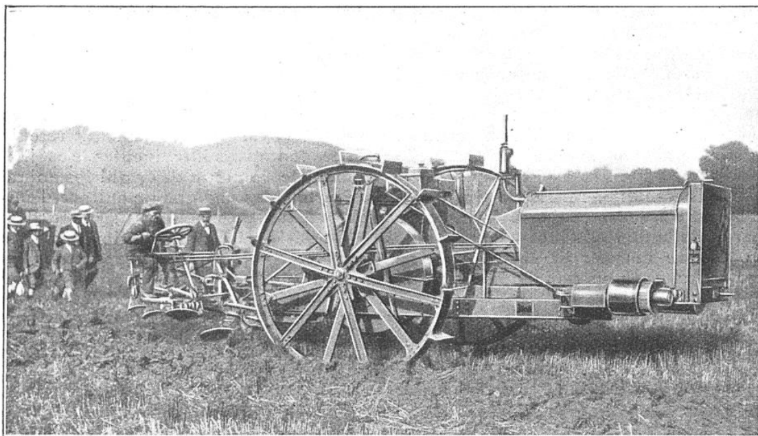
ASPECT LATÉRAL D'UNE LABOUREUSE STOCK
