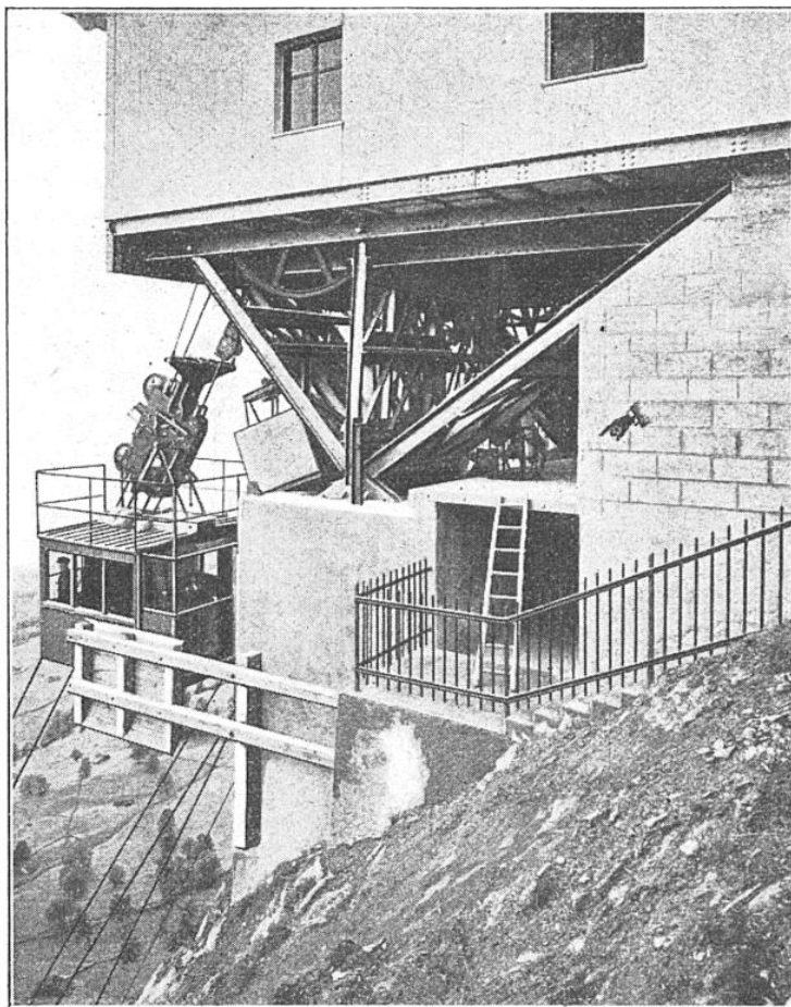
STATION SUPÉRIEURE D'UN FUNICULAIRE (WETTERHORN)
