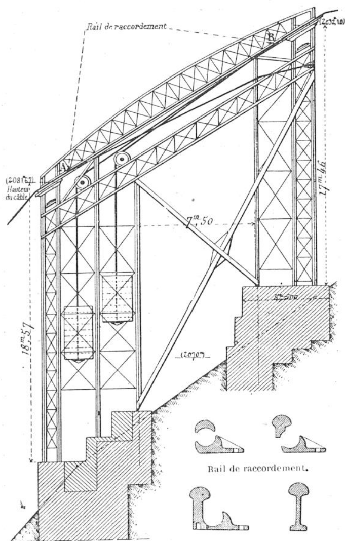
POSTE INTERMÉDIAIRE D'ANCRAGE ET DE TENSION DES CÂBLES
