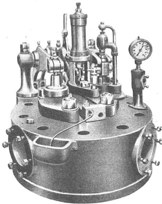
CULASSE D'UN MOTEUR DIESEL
