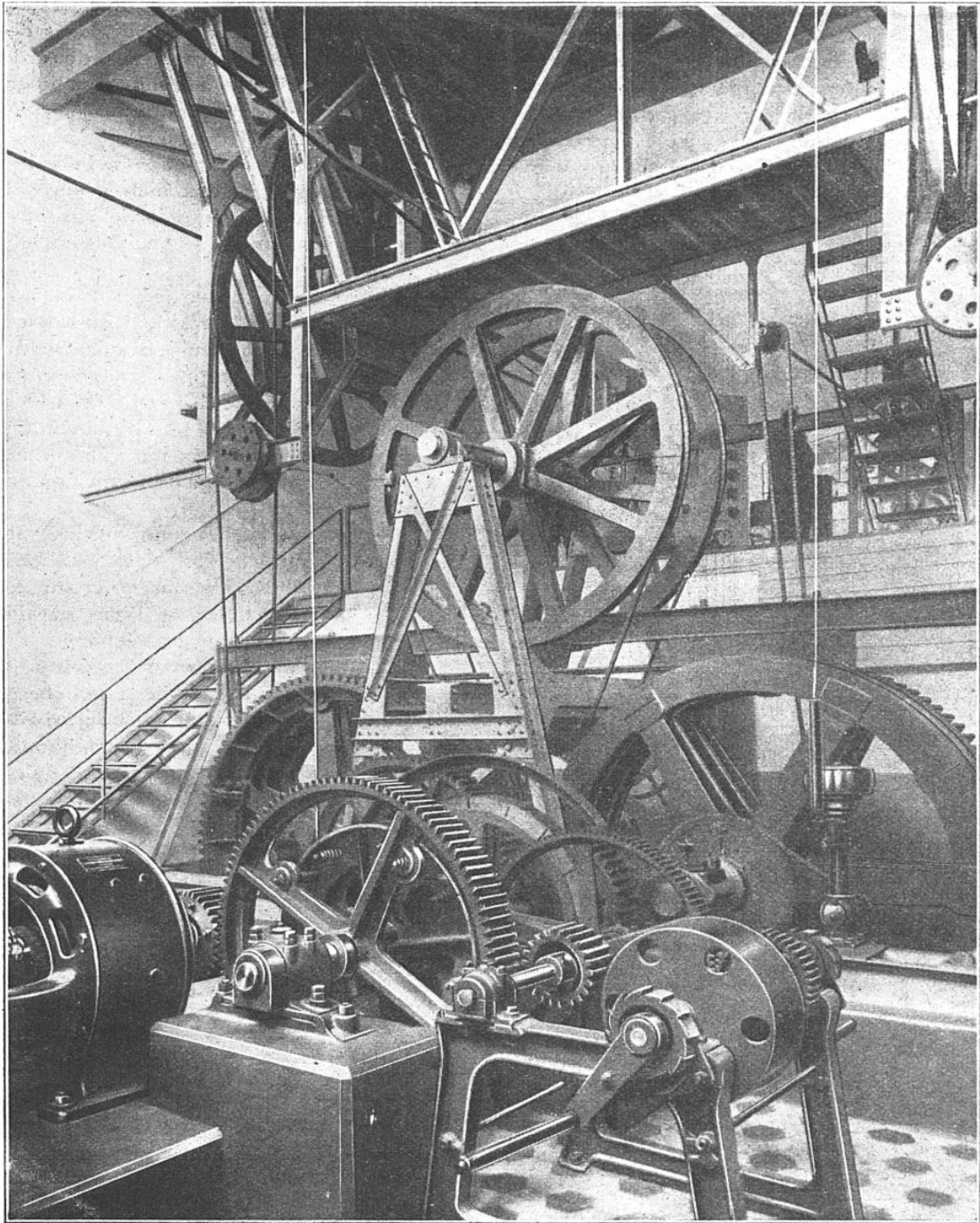
MÉCANISME MOTEUR DE LA LIGNE DU MONT KOHLERER
