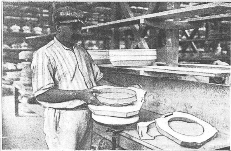
DÉMOULAGE D'UNE PIÈCE COULÉE DANS UN MOULE EN PLÂTRE
