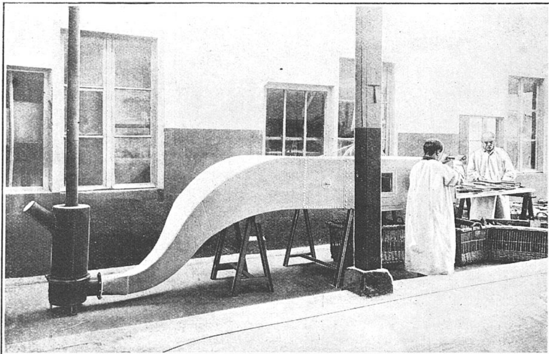
L'APPEL D'AIR PRODUIT PAR LE TIRAGE D'UN POËLE SUFFIT A ASPIRER LES POUSSIÈRES
