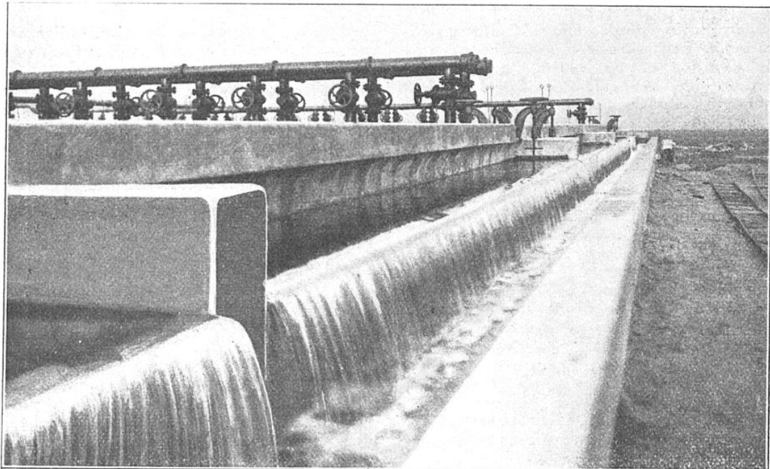
A la sortie des dégrossisseurs, l'eau se déverse en cascade dans le bassin de préfiltration où elle subira une épuration et une clarification plus complètes, avant de passer dans les filtres à sable.
