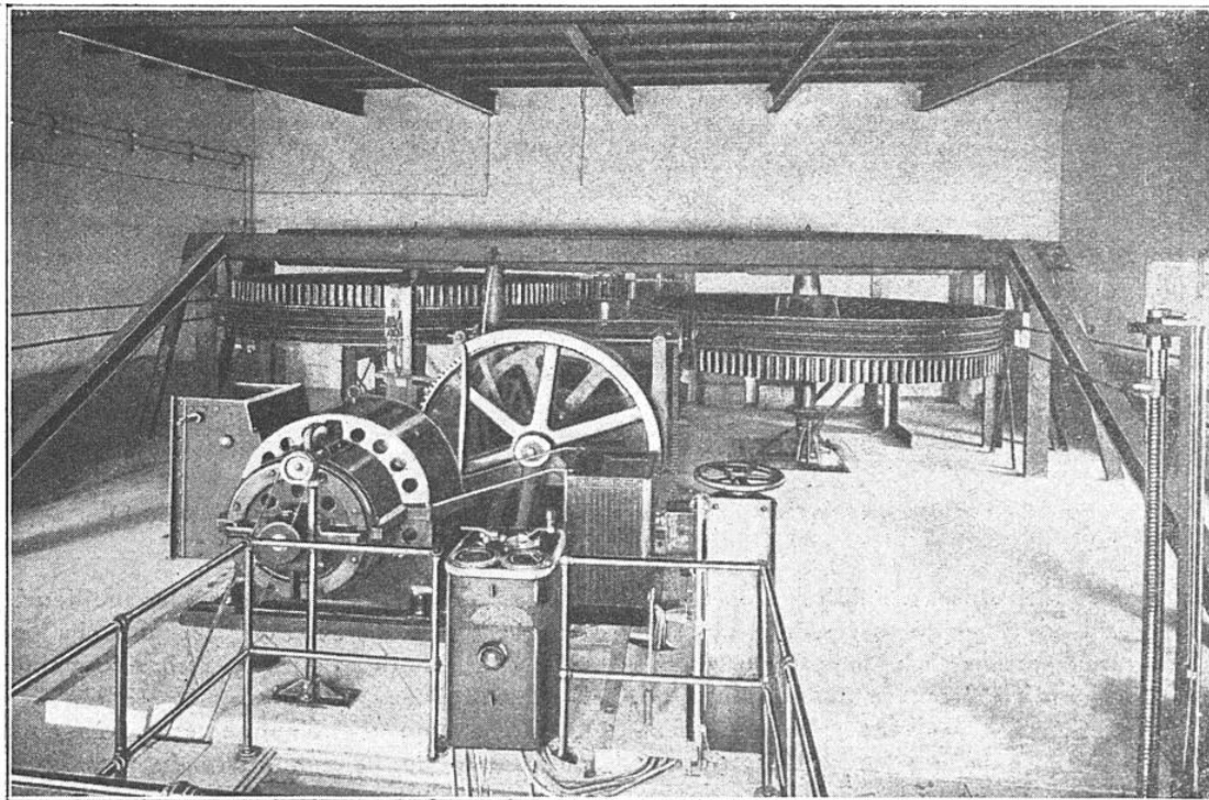
TREUILS MOTEURS DES CÂBLES DE REMORQUE (FUNICULAIRE DU WETTERHORN)
