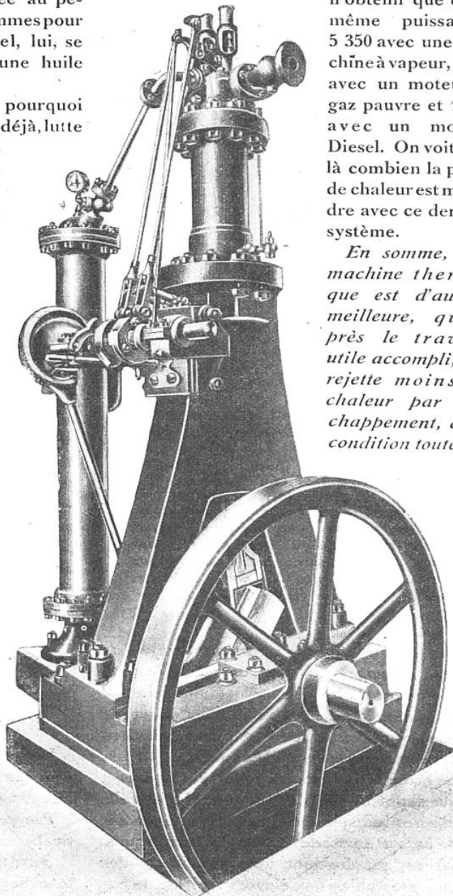
LE PREMIER MOTEUR DIESEL CONSTRUIT A AUGSBURG (1893)
