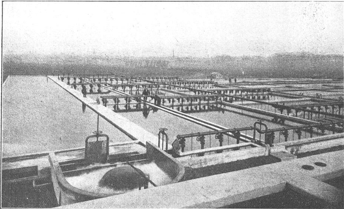
Dans l'installation de Roubaix-Tourcoing, l'eau, avant de passer dans les dégrossisseurs, laisse déposer une partie de ses impuretés dans le bassin de décantation visible à gauche de la figure.
