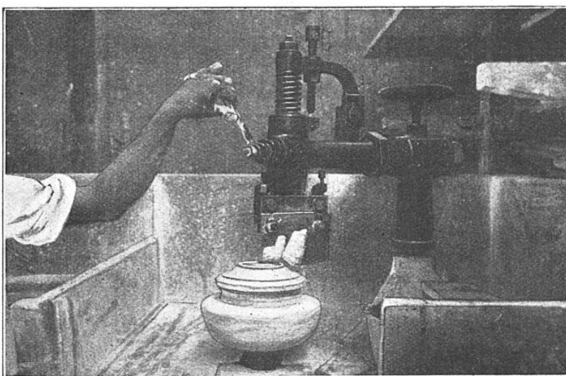
MACHINE A DÉCOUPER LE PIED ET LE PROFIL EXTÉRIEUR DES ASSIETTES
