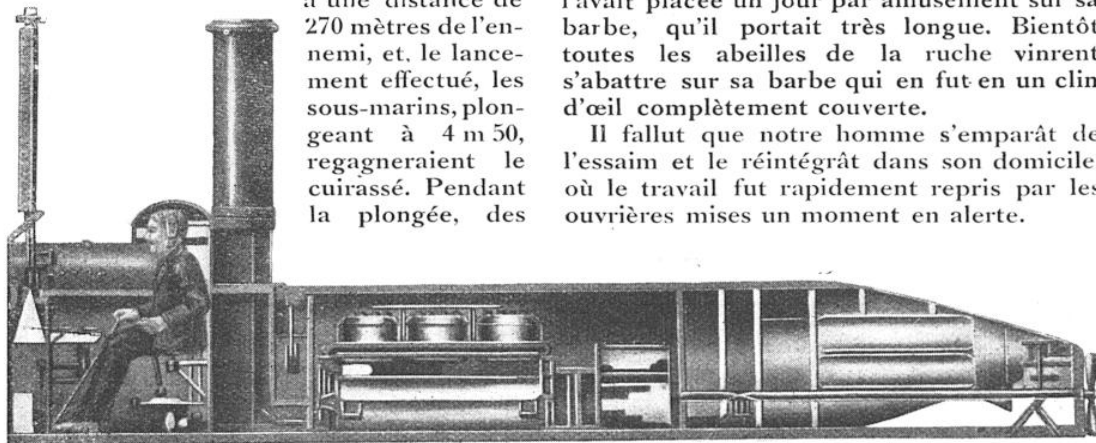
INTÉRIEUR DU TORPILLEUR SOUS-MARIN
