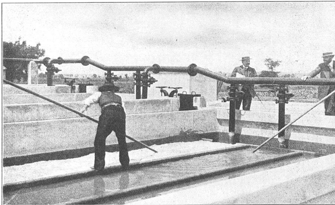
NETTOYAGE D'UN DÉGROSSISSEUR DE L'INSTALLATION FILTRANTE DE SAINT-GILLES-DU-GARD
