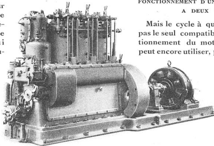
MOTEUR SULZER-DIESEL DU TYPE FIXE
