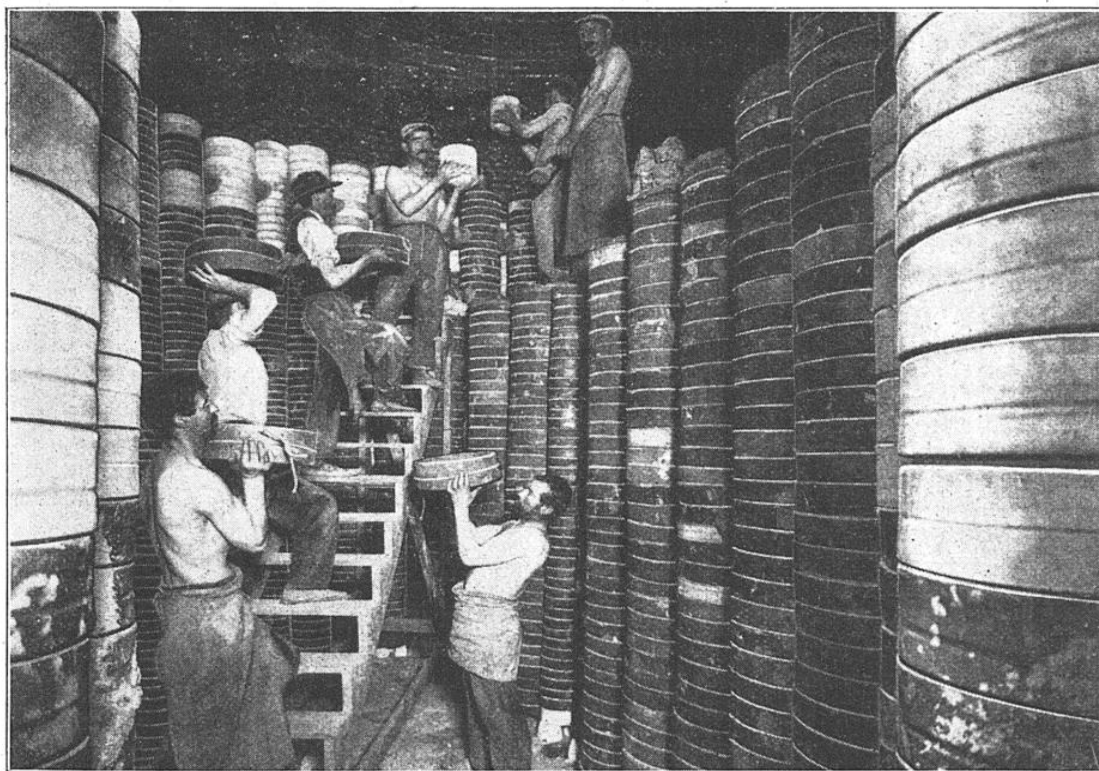
EMPILAGE DES CASSETTES DANS UN FOUR A PORCELAINE
