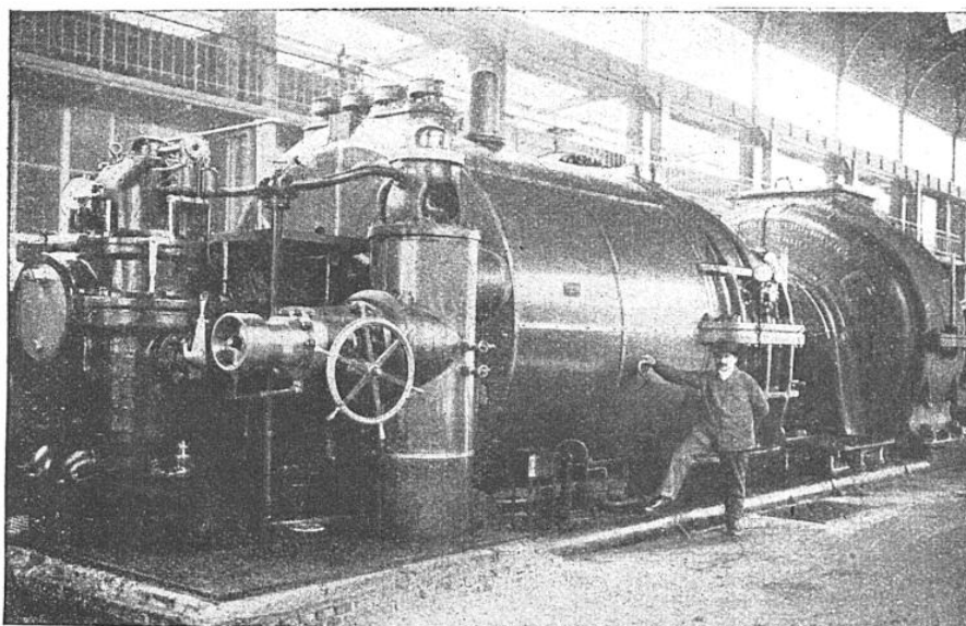
Société d'Electricité de Paris, Usine de Saint-Denis. Turbine à vapeur de 25.000 HP, 750 tours
