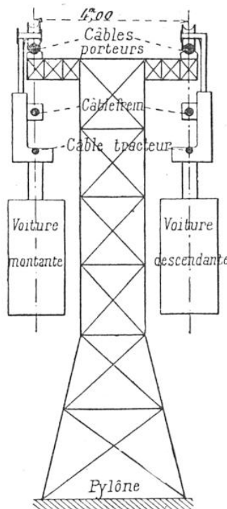
DISPOSITION DES ÉLÉMENTS D'UN FUNICULAIRE AÉRIEN
