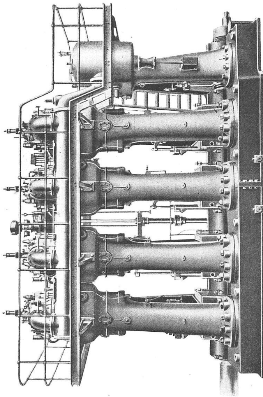
MOTEUR CARELS-DIESEL A DEUX TEMPS ; PUISSANCE 1000 CHEVAUX
