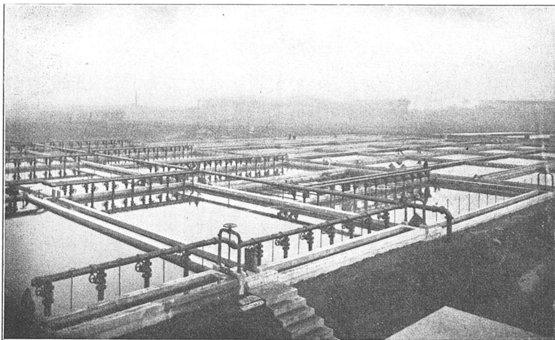
VUE D'ENSEMBLE DES BASSINS FILTRANTS DES VILLES DE ROUBAIX-TOURCOING
