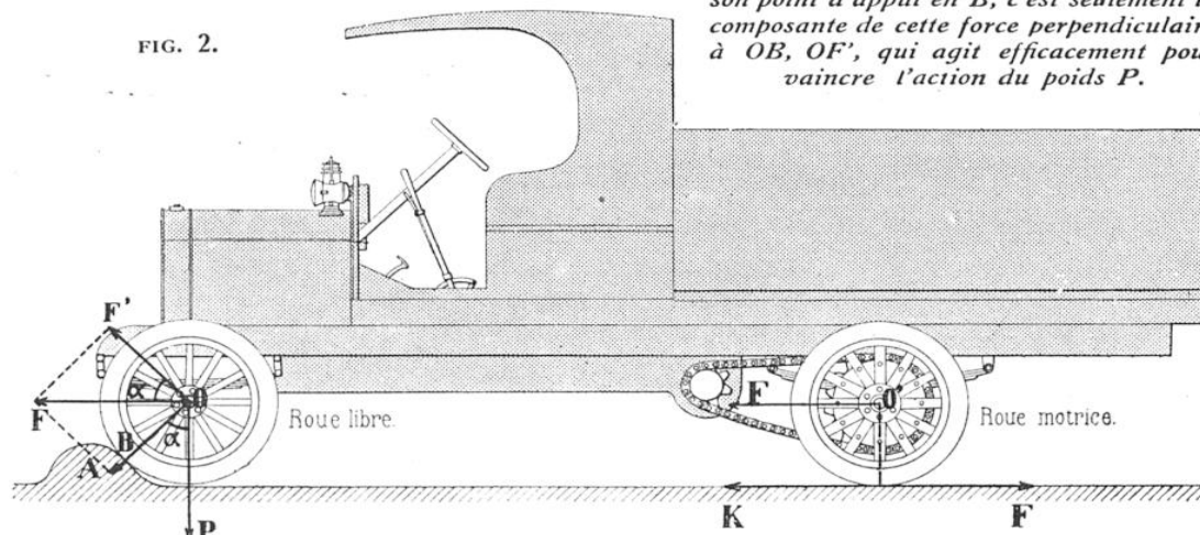
CAMILION ABORDANT UN OBSTACLE PAR UNE ROUE NON MOTRICE
