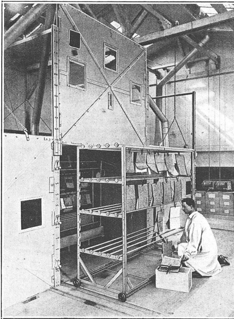
LA DÉSINFECTION DES LIVRES PAR L'ALDÉHYDE FORMIQUE
