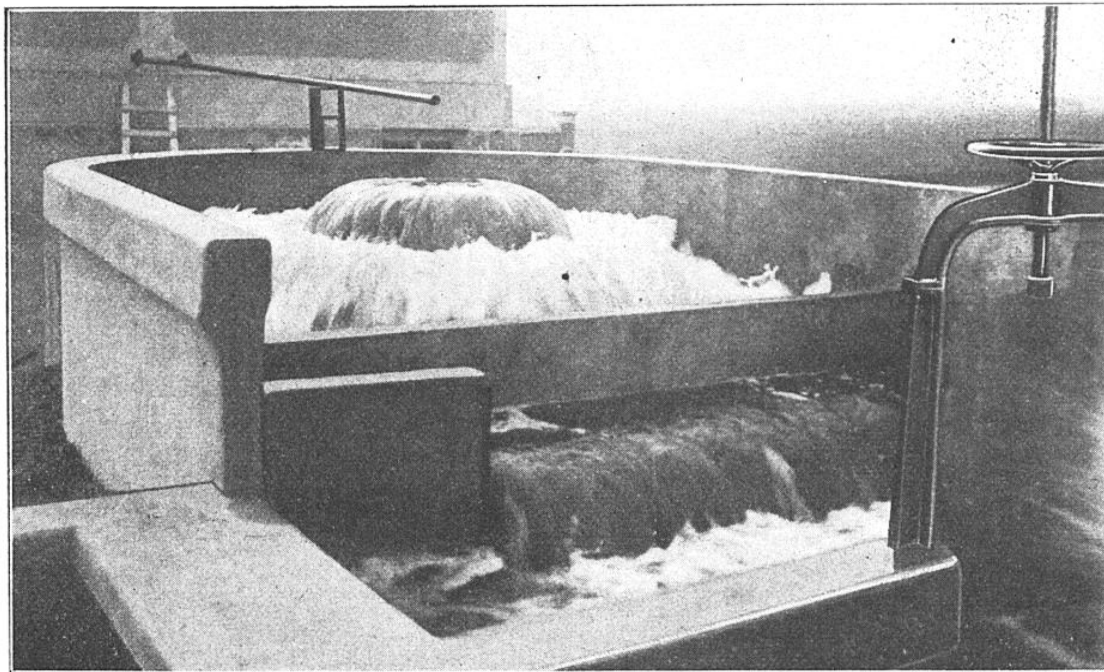
VANNE D'ADMISSION DE L'EAU BRUTE DANS LE BASSIN DE DÉCANTATION
