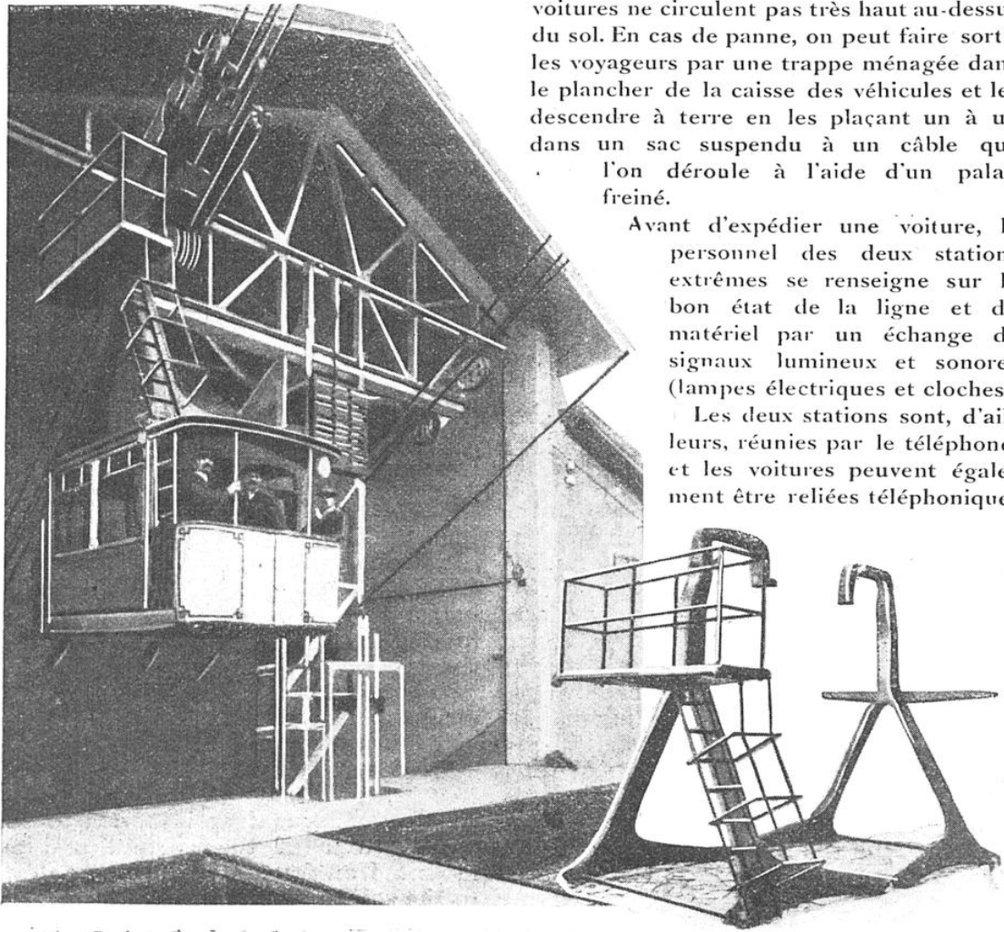
STATION INFÉRIEURE DU FUNICULAIRE A VOYAGEURS DU MONT KOHLERER
