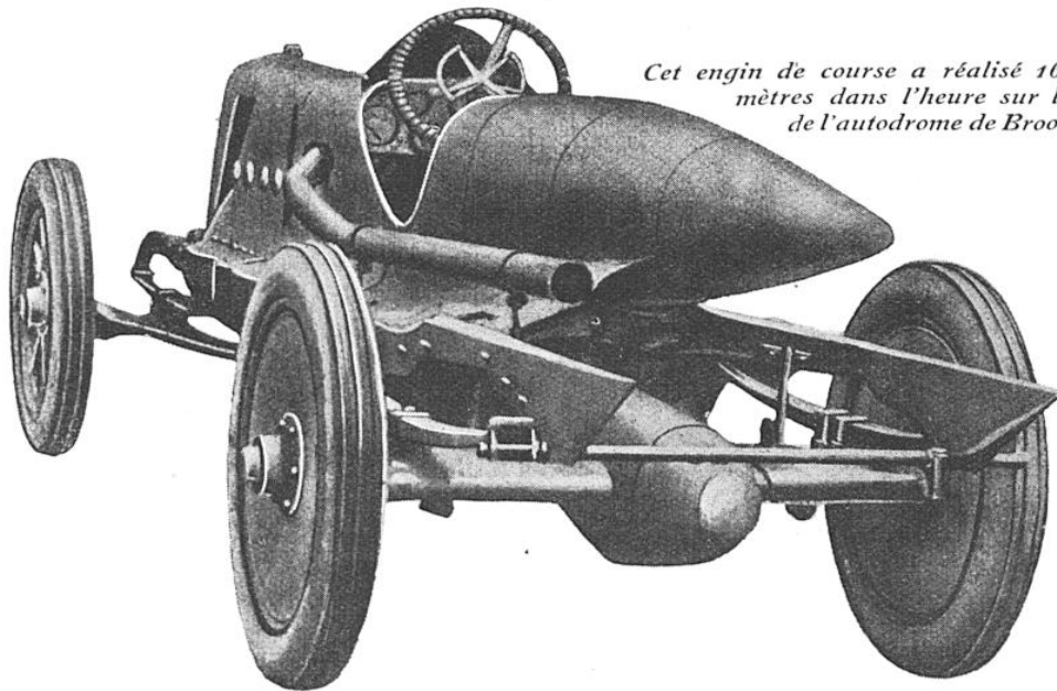
L'AUTOMOBILE DE COURSE TALBOT QUI VIENT DE RÉALISER CETTE PROUESSE
