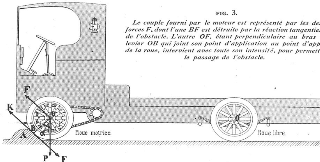
CAMION ABORDANT UN OBSTACLE PAR UNE ROUE MOTRICE
