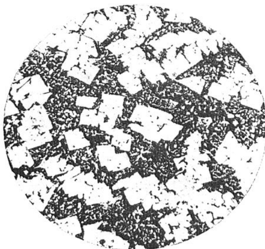
TYPE D'ALLIAGE POUR COUSSINETS
