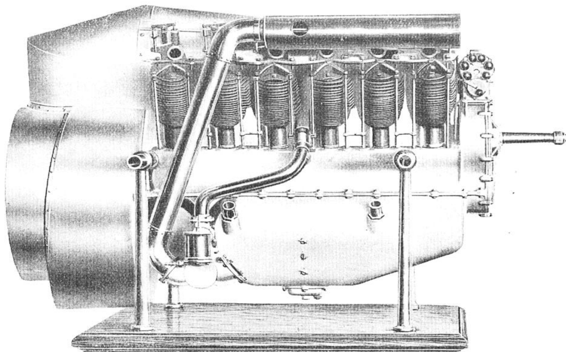
UN DES MODÈLES DE MOTEURS D'AVIATION RENAULT
