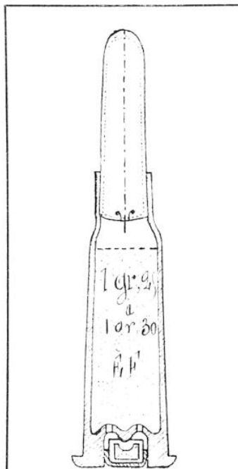
CARTOUCHE A BLANC (Grandeur naturelle)
