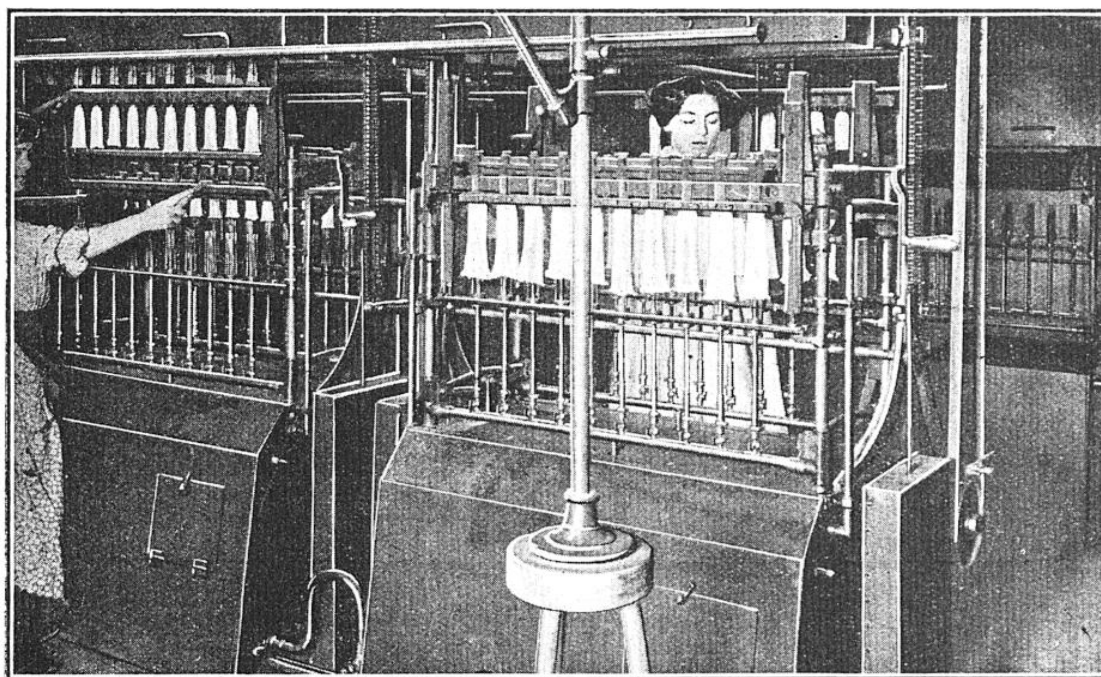
LES MANCHONS, DISPOSÉS SUR LES SUPPORTS DU FOUR A MOUFLE, VONT ÊTRE BRULÉS
