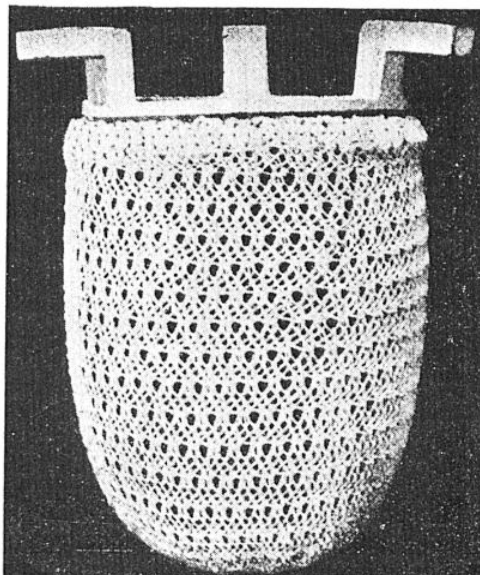
MANCHON A FLAMME RENVERSÉE TYPE COURANT
