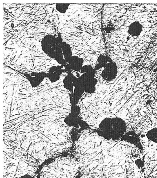
ACIER TREMPÉ A BASSE TEMPÉRATURE
