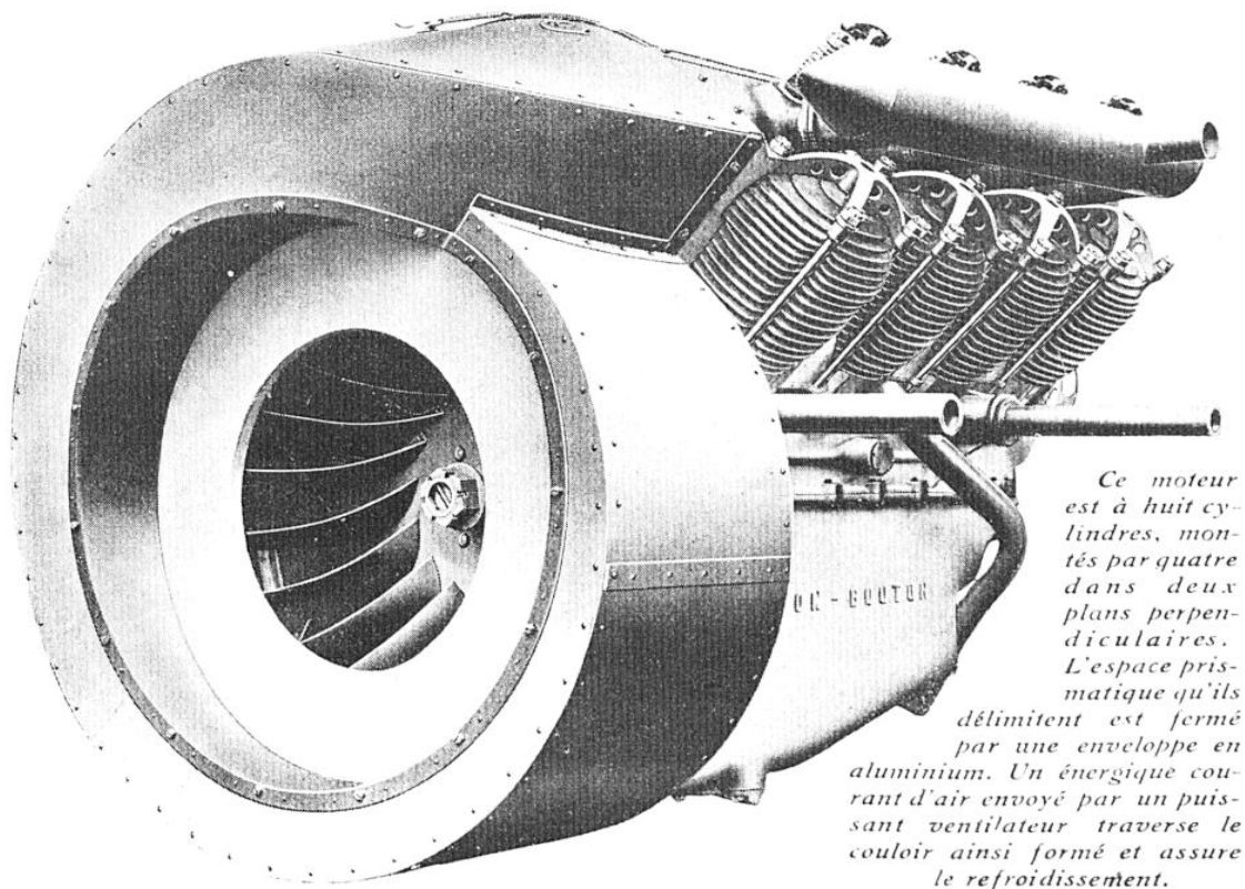
LE MOTEUR 80 CHEVAUX DE DION-BOUTON
