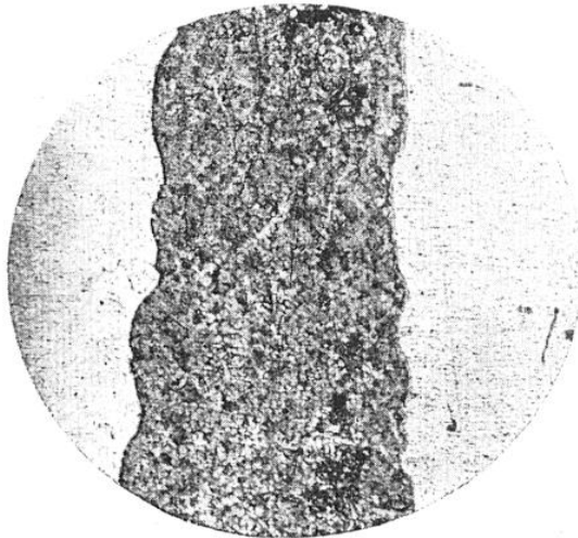
COUPE AGRANDIE D'UNE MAUVAISE SOUDURE
