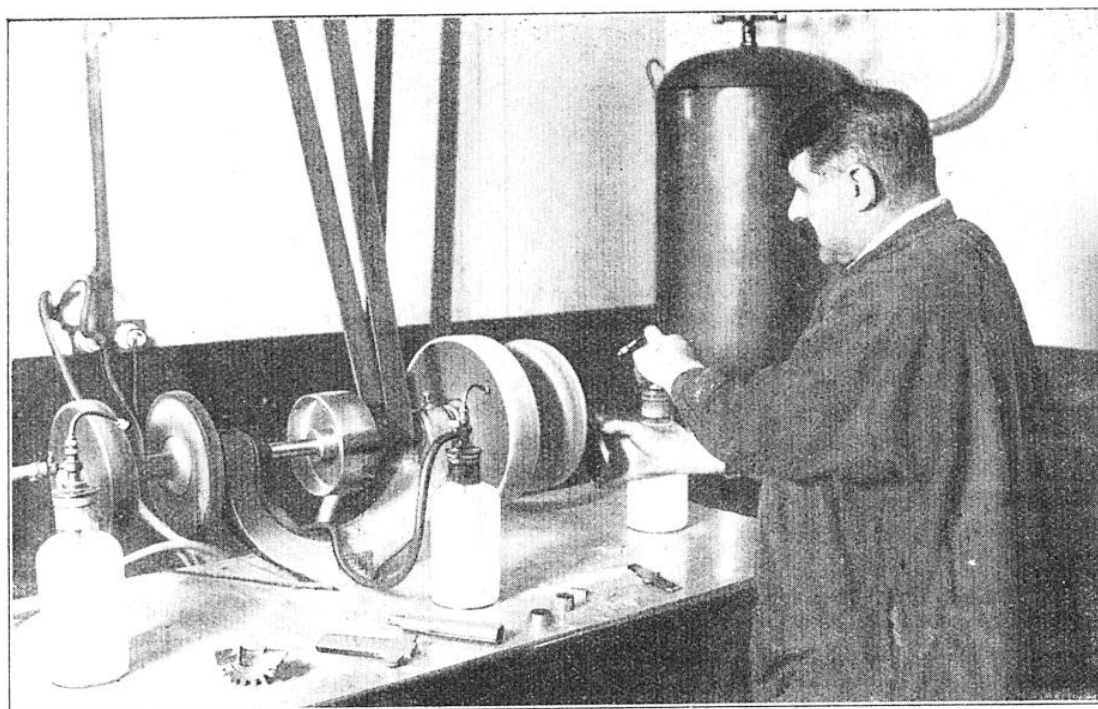
LE FINISSAGE DES COUPES SE FAIT SUR UN BANC DE POLISSAGE A DEUX PAIRES DE MEULES Le polissage est une opération extrêmement délicate qui doit se terminer dans une salle complètement isolée; l'alumine, en grains de grosseur déterminée, est projetée sur le drap des meules par un vaporisateur qui reçoit l'air comprimé du réservoir placé à droite de l'opérateur.
