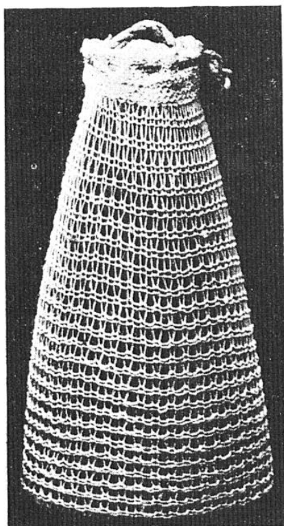
Manchon confectionné spécialement pour l'éclairage au benzol. Les mailles sont larges et la forme est celle d'un cône assez ouvert.
