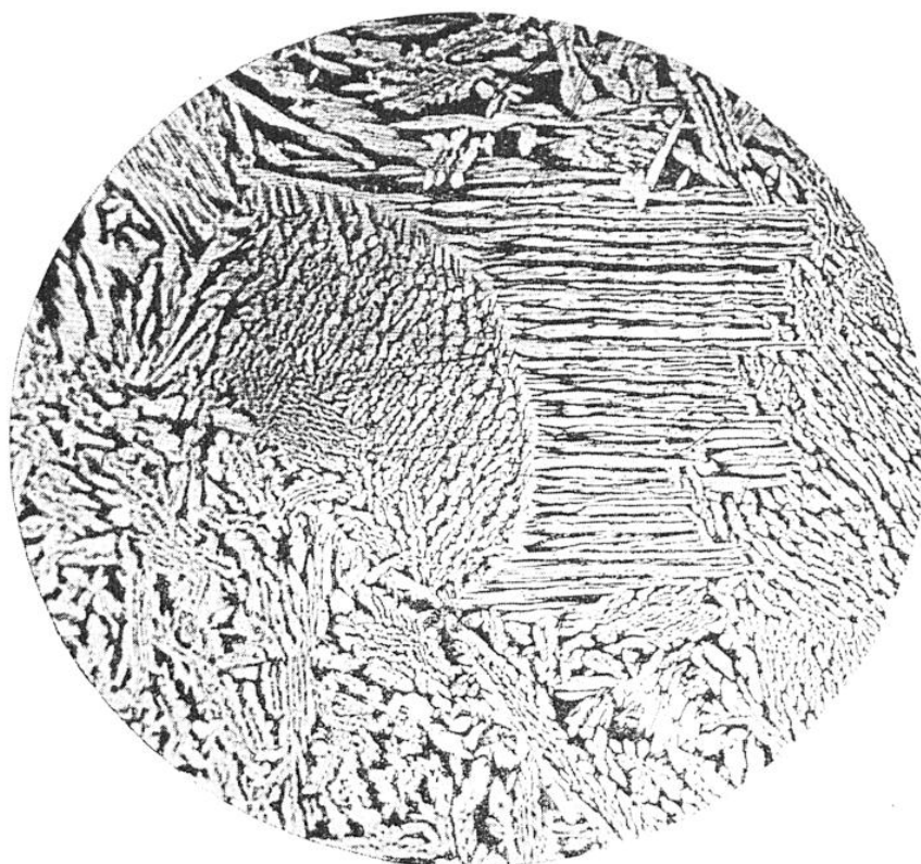
BRONZE D'ALUMINIUM COMPOSÉ SELON UNE FORMULE DE SAINTE-CLAIRE DEVILLE
