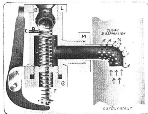
COUPE DE L'ÉCONOMISEUR « FRANCE »
