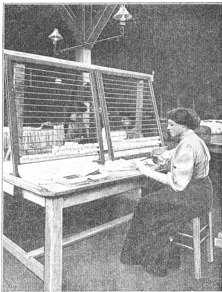
APPLICATION DU LIQUIDE DE DURCISSAGE
