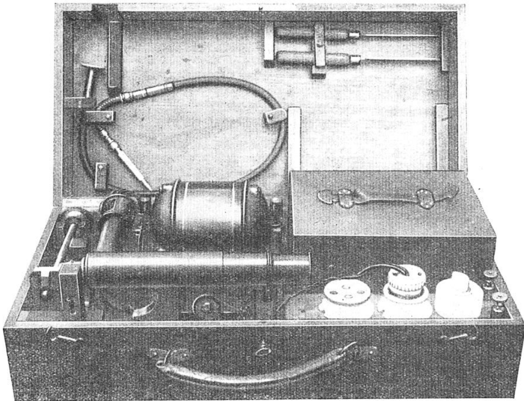
TROUSSE PORTATIVE DE MÉTALLOGRAPHIE MICROSCOPIQUE
