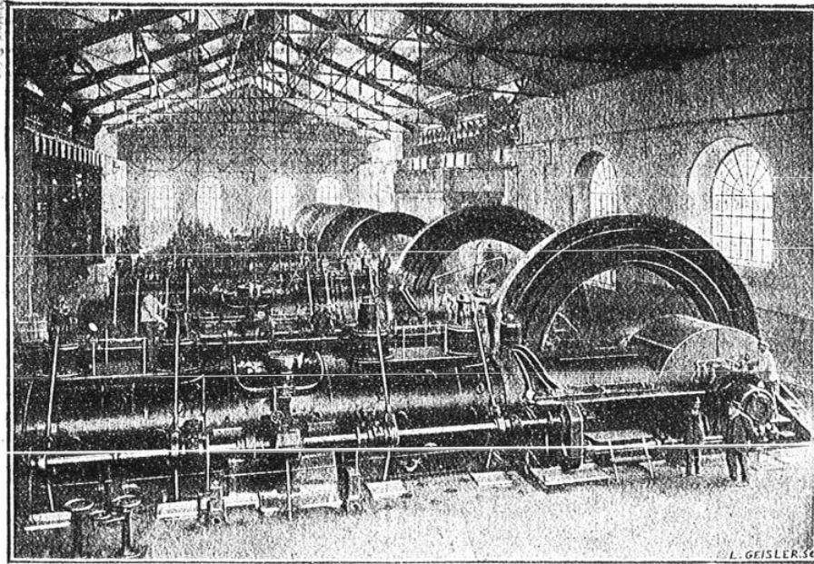
Station Centrale de la C ie des Forges et Aciéries de la Marine et d'Homécourt à Homécourt. Puissance des Alternateurs 18.000 chev.
