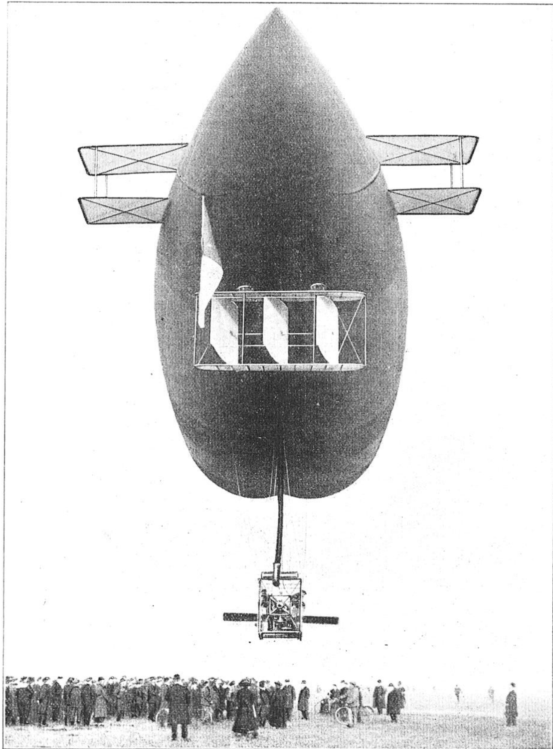
LES PLANS STABILISATEURS ET LES GOUVERNAILS DU DIRIGEABLE "ASTÉA-TORRÈS"
