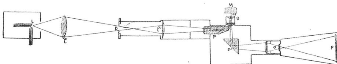
SCHÉMA DE LA MARCHÉ DES RAYONS DANS L'APPAREIL DE M. H. LE CHATELIER
