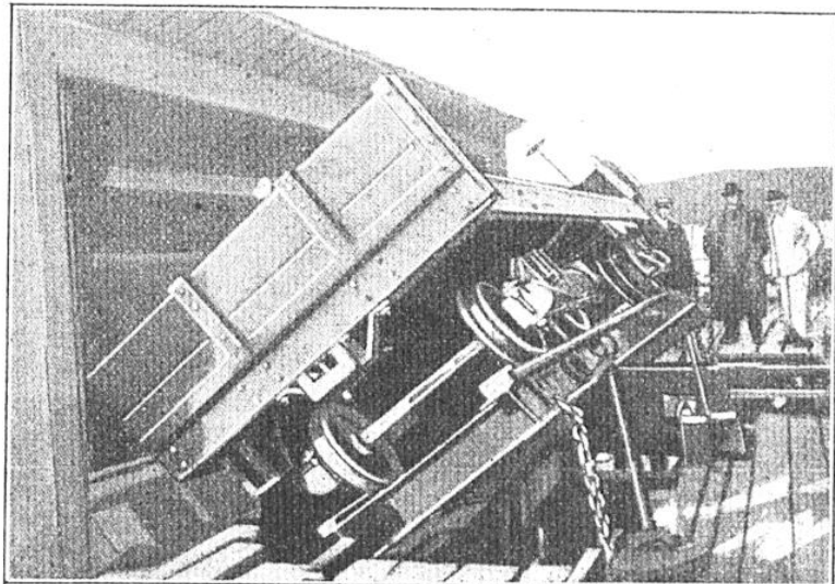
La plateforme se soulevant sur ses charnières prend un angle de 45° et permet au chargement de tomber dans le concasseur.
