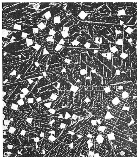
MÉTAL DOUX POUR ORGANES DE FROTTEMENT
