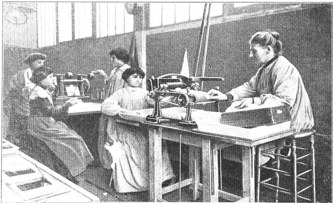
DANS CERTAINES USINES L'ESSORAGE SE FAIT AU MOYEN DE MACHINES APPELÉES CALANDRES Si l'on n'enlève pas l'excédent de liquide au moyen d'uneessoreuse centrifuge, comme dans la gravure du haut, on emploie une calandre munie de cylindres en caoutchouc.
