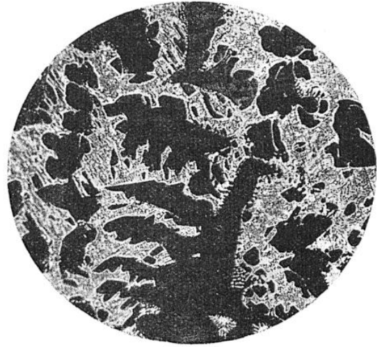
BRONZE CONTENANT 20 % D'ÉTAIN
