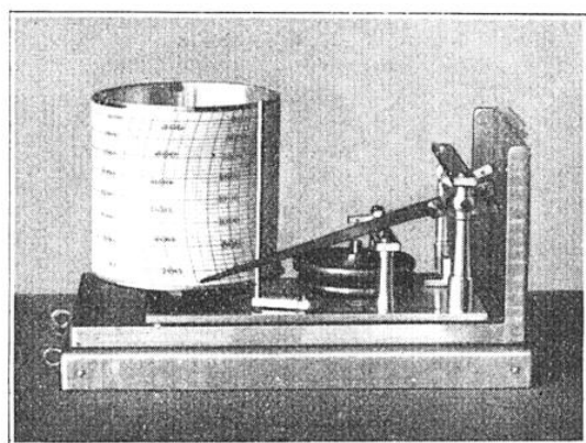
BAROMÈTRE ENREGISTREUR RICHARD POUR LA MESURE DES ALTITUDES
