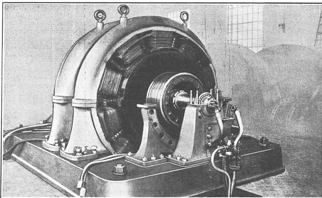
LA MASSE FORMIDABLE DU ROTOR DE CETTE DYNAMO TOURNE SUR BILLES
