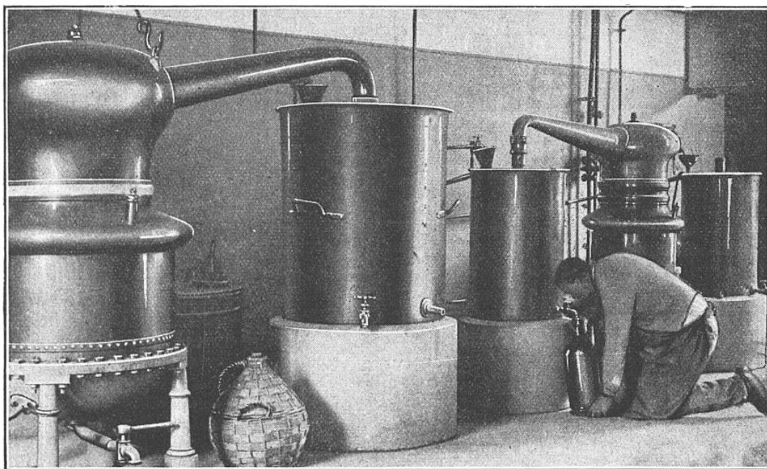
APRÈS SA DISTILLATION, LE CHLOROFORME PURIFIÉ EST SOUTIRÉ DES ALAMBICS
