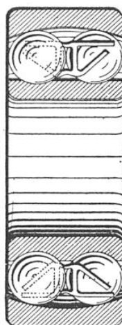
ROULEMENT DOUBLE AVEC ROTULE SUR BILLES
