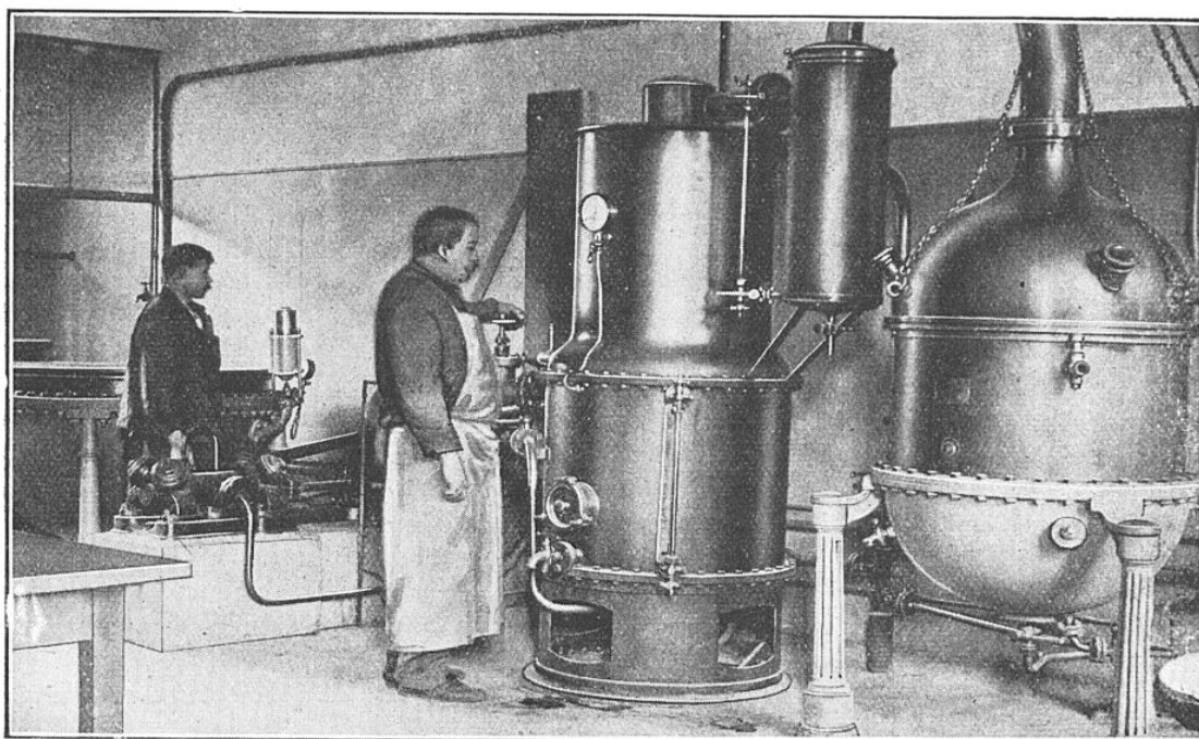
LES EXTRAITS MÉDICAMENTEUX SONT PRÉPARÉS DANS UN ALAMBIC DE CINQ CENTS LITRES
