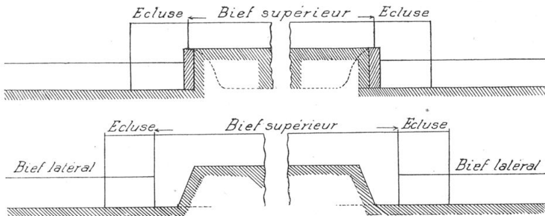
COUPES D'UNE ÉCLUSE ORDINAIRE ET D'UNE ÉCLUSE DU TYPE BUNAU-VARILLA
