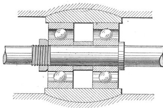
TÊTE D'ARBRE MONTÉE SUR ROULEMENT A DOUBLE RANGÉE DE BILLES ET ROTULE EXTÉRIEURE
