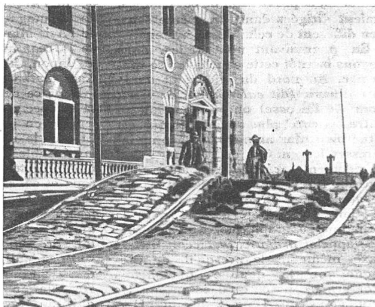
CE QU'UN SÉISME FAIT D'UNE LIGNE DE TRAMWAYS
