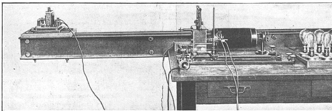
FIG. 1. — L'ACCÉLÉROMÈTRE DE MM. BOYER-GUILLON ET AUCLAIR ET SON ENREGISTREUR
