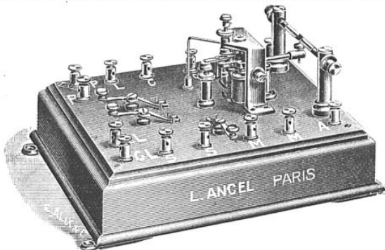
Récepteur de TSP à cohéreur pour enregistrement. N° 4024 du catalogue
