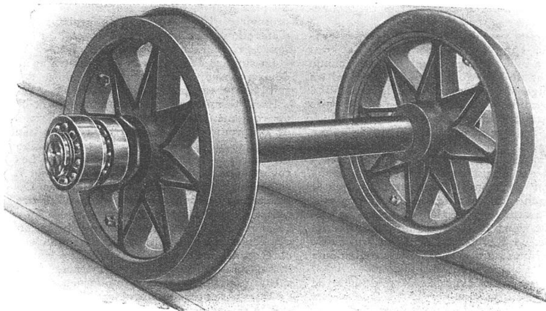
CHACUNE DE CES ROUES EST MONTÉE SUR DEUX ROULEMENTS A DOUBLE RANGÉE DE BILLES
