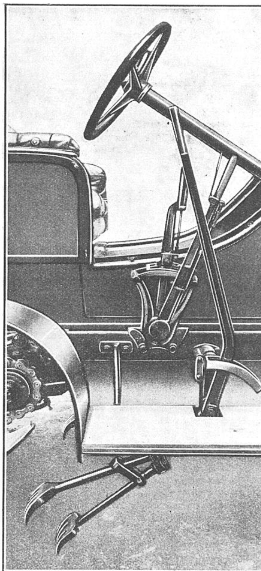
LE FREINAGE EST OBTENU A L'AIDE DE PUISSANTES GRIFFES QUI MORDENT LE SOL
