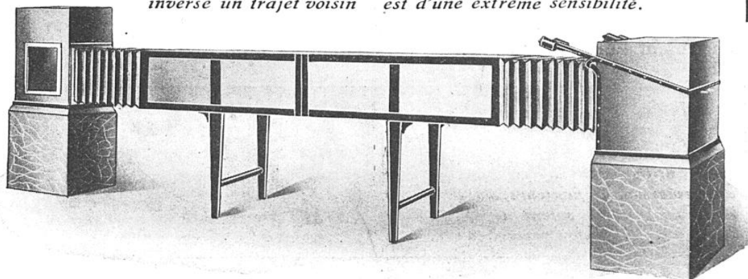
LES BOÎTES PROTECTRICES ET LE COULOIR QUI RELIE LES PENDULES AU CYLINDRE ENREGISTREUR
