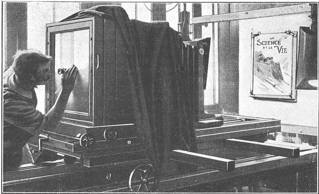
L'EMPLACEMENT DE LA TRAME DANS L'APPAREIL PHOTOGRAPHIQUE EST DÉTERMINÉ AVEC SOIN. Avant l'exposition de la pellicule, on déplace la trame jusqu'à ce que son image, formée sur une lame de verre et regardée avec un microscope de mise au point, présente un aspect bien défini.
