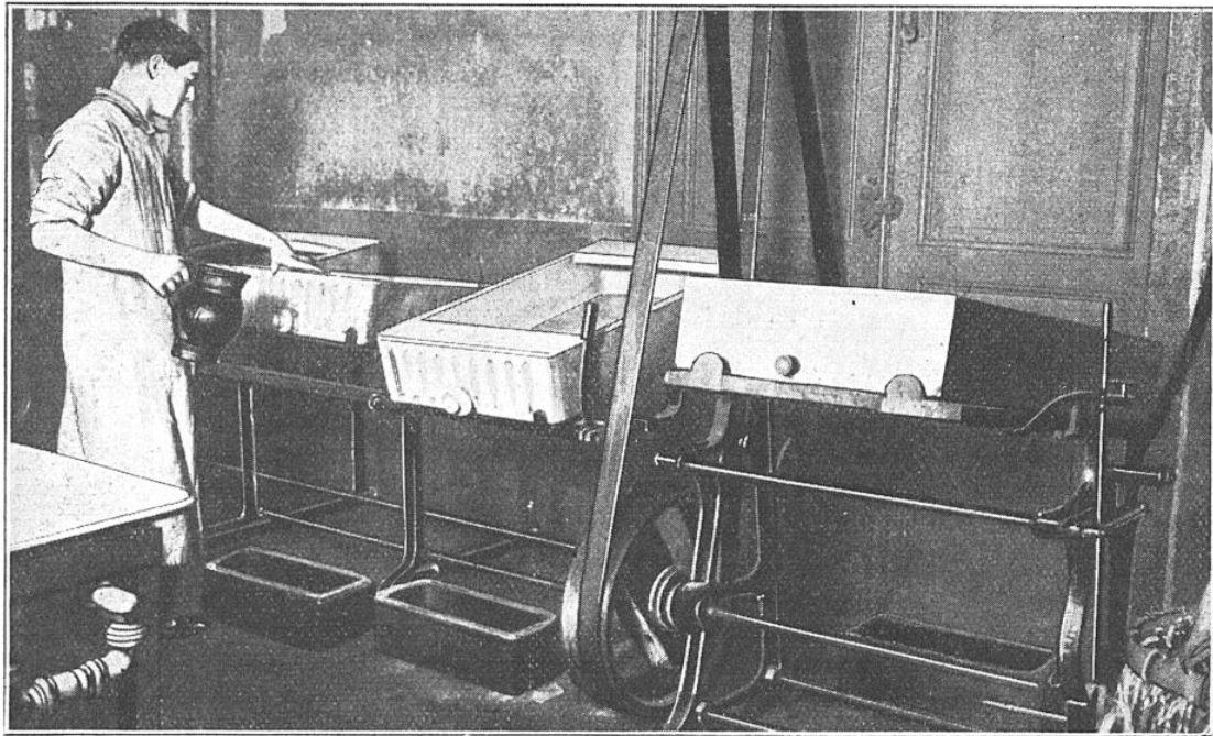
LA « MORSURE » DES CLICHÉS SE FAIT DANS DES CUVES BASCULANTES
