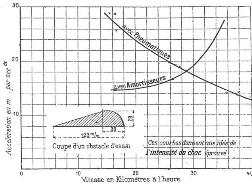
FIG. 4. — DIAGRAMMES COMPARATIFS FOURNIS PAR L'ACCÉLÉROMÈTRE
