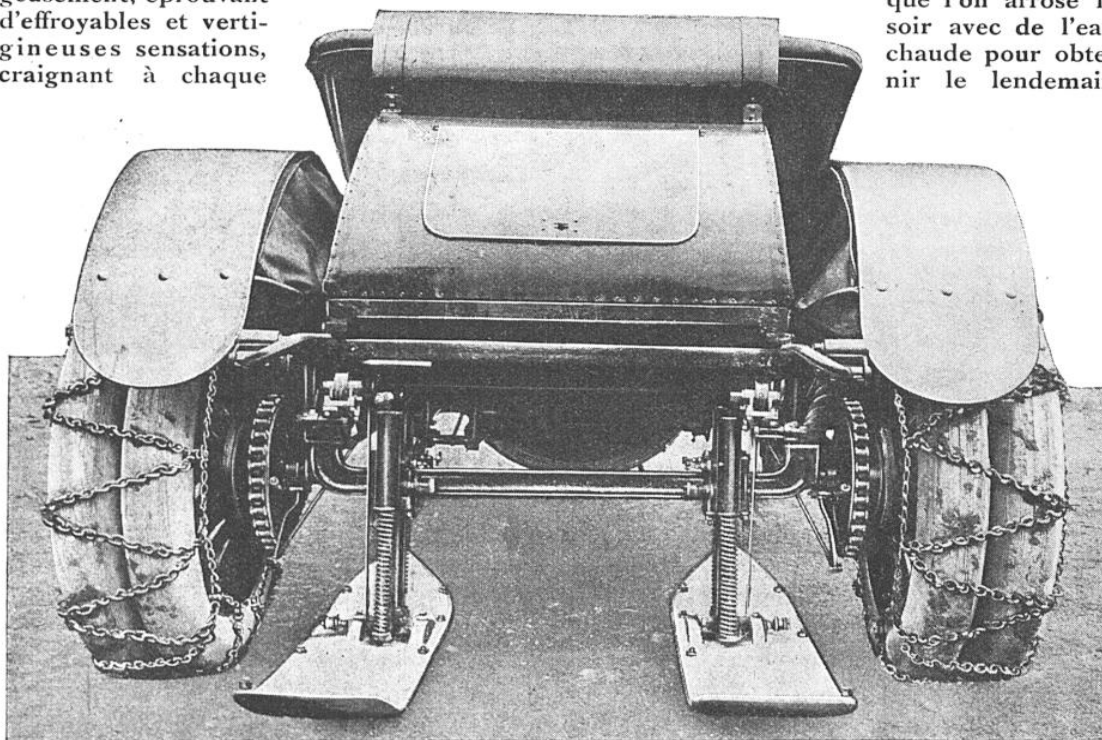
LES PATINS ET LES ROUES MOTRICES D'UNE AUTOMOBILE TRANSFORMÉE EN TRAÎNEAU
