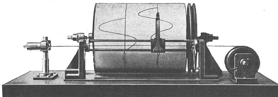
FIG. 5. — CET APPAREIL ENREGISTRE LES FLEXIONS DES RESSORTS AU PASSAGE D'UN OBSTACLE. Le crayon inscripteur est commandé par un fil d'acier horizontal dont une extrémité se fixe à l'organe de la voiture dont on veut mesurer les déplacements verticaux. A l'autre bout, le fil s'enroule sur un treuil muni d'un ressort intérieur qui assure la tension nécessaire.
