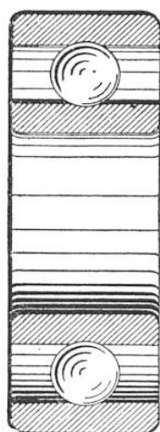
Coupe d'un roulement à rangée de billes unique.
