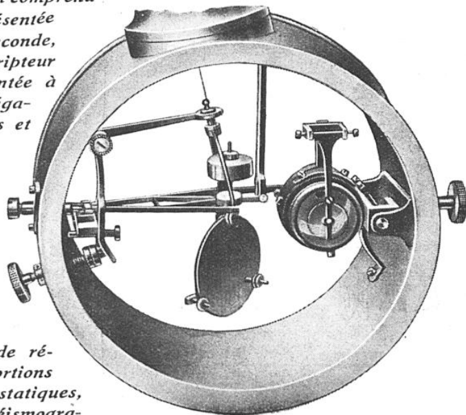
DÉTAIL DU DISPOSITIF DE SUSPENSION
