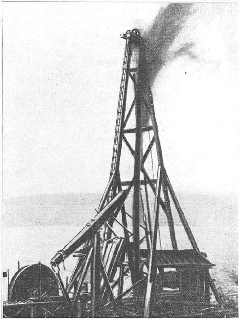
PUITS DE PÉTROLE A COLONNE JAILLISSANTE
