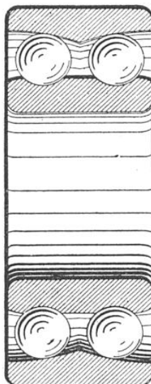
Type ordinaire de roulement à double rangée de billes.
