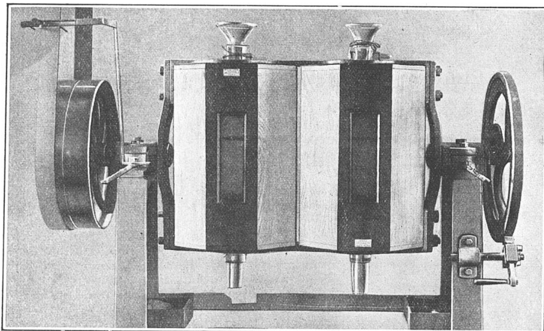
AGITATEUR ROTATIF EMPLOYÉ POUR LA RECTIFICATION DU CHLOROFORME
