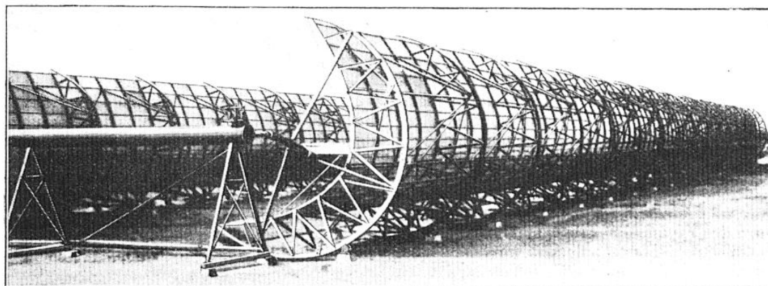
A L'APPROCHE DU COUCHER DU SOLEIL LES APPAREILS SONT TRÈS FORTEMENT INCLINÉS Les châssis supportant l'ensemble des miroirs et des générateurs demeurent constamment face au soleil grâce au mouvement progressif d'inclinaison que leur communique l'astre lui-même, par l'intermédiaire d'un thermostat également exposé aux rayons solaires.
