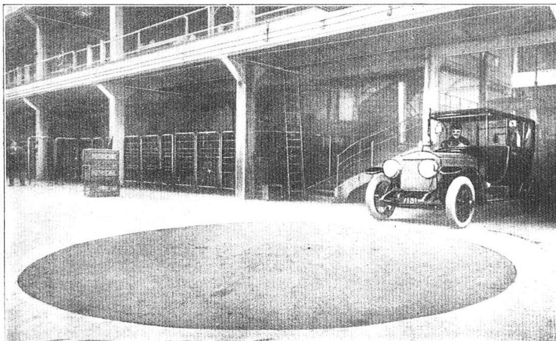
DANS CE GARAGE, LES AUTOS TOURNENT SUR DES PLAQUES ET PRENNENT L'ASCENSEUR Cette voiture conduite par son chauffeur manœuvre pour se placer sur la plaque tournante, au sortir de l'ascenseur électrique qui l'a descendue de son boxe situé à un étage supérieur.
