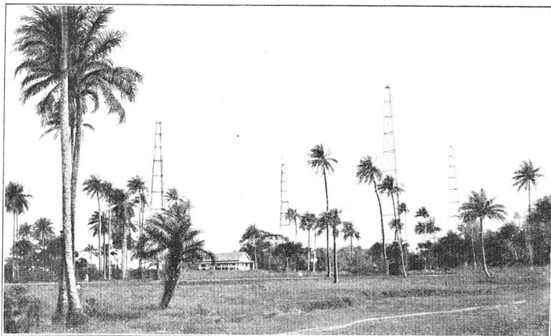
POSTE DE TÉLÉGRAPHIE SANS FIL DE CONAKRY (GUINÉE FRANÇAISE)
