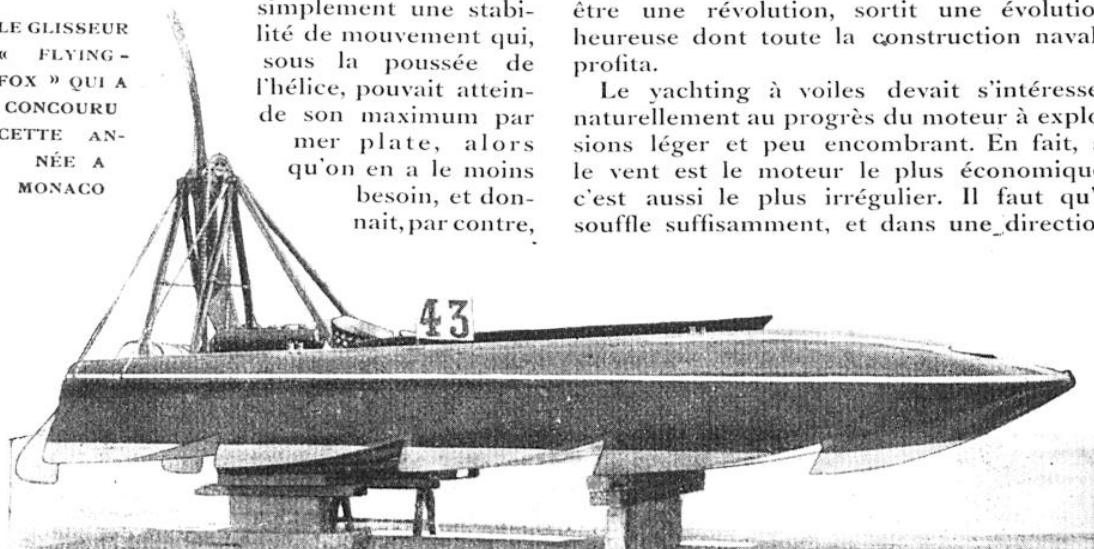
Les premiers bateaux à hélice aérienne étaient à fond plat. On a reconnu depuis qu'on obtenait un déjaugage plus complet en disposant sous la coque plusieurs plans inclinés ou redans.
