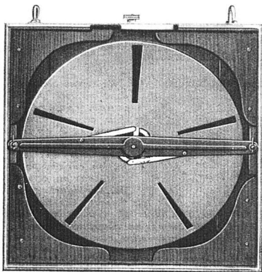
DISQUE OBTURATEUR DU CHRONOPHOTOGRAPHE
