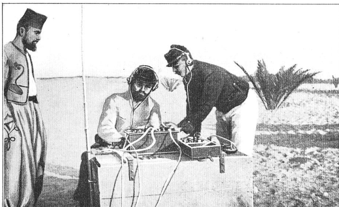
POSTE EMPORTÉ PAR LE GÉNÉRAL BAILLOUD LORS DE SA TRAVERSÉE DU SAHARA A chacune des étapes de la caravane, un mât démontable était dressé et on écoutait les radiotélégrammes envoyés par les postes de Sainte-Marie-de-la-mer, d'Alger ou de Taourirt (Maroc).
