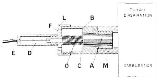
COUPE DE LA PRISE D'AIR « CELER »
