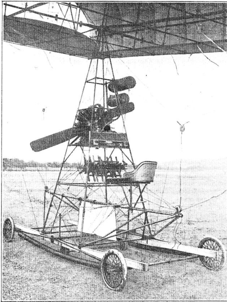
LE TRAIN D'ATERRISSAGE ET LE MOTEUR DE L'AÉROPLANE
