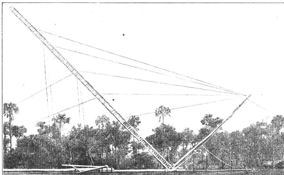
DRESSAGE D'UNE ÉCHELLE-OBSERVATOIRE SUPPORTANT L'ANTENNE D'UN POSTE MOBILE Cette opération s'effectue comme pour le mât démontable avec une bique. Le chef de poste peut du sommet de cette échelle, surveiller les alentours et faire des levés topographiques.
