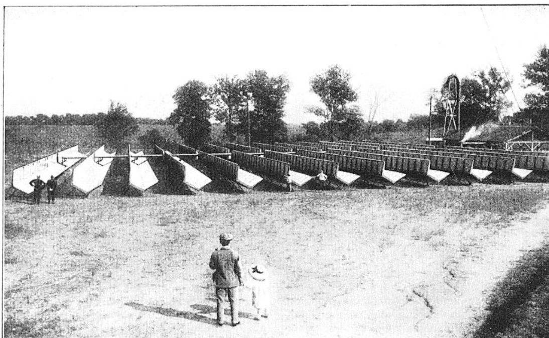
VUE D'ENSEMBLE DE L'INSTALLATION D'ESSAI ÉTABLIE PAR M. SHUMAN, PRÈS DE PHILADELPHIE
