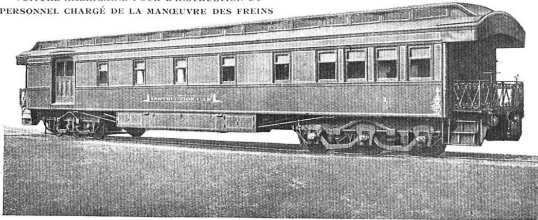
Ce véhicule à douze roues renferme tout le matériel de freinage correspondant aux plus longs trains de voyageurs. On s'en sert aux États-Unis pour entraîner les agents en vue de l'emploi judicieux, en toute circonstance, des freins continus automatiques.
