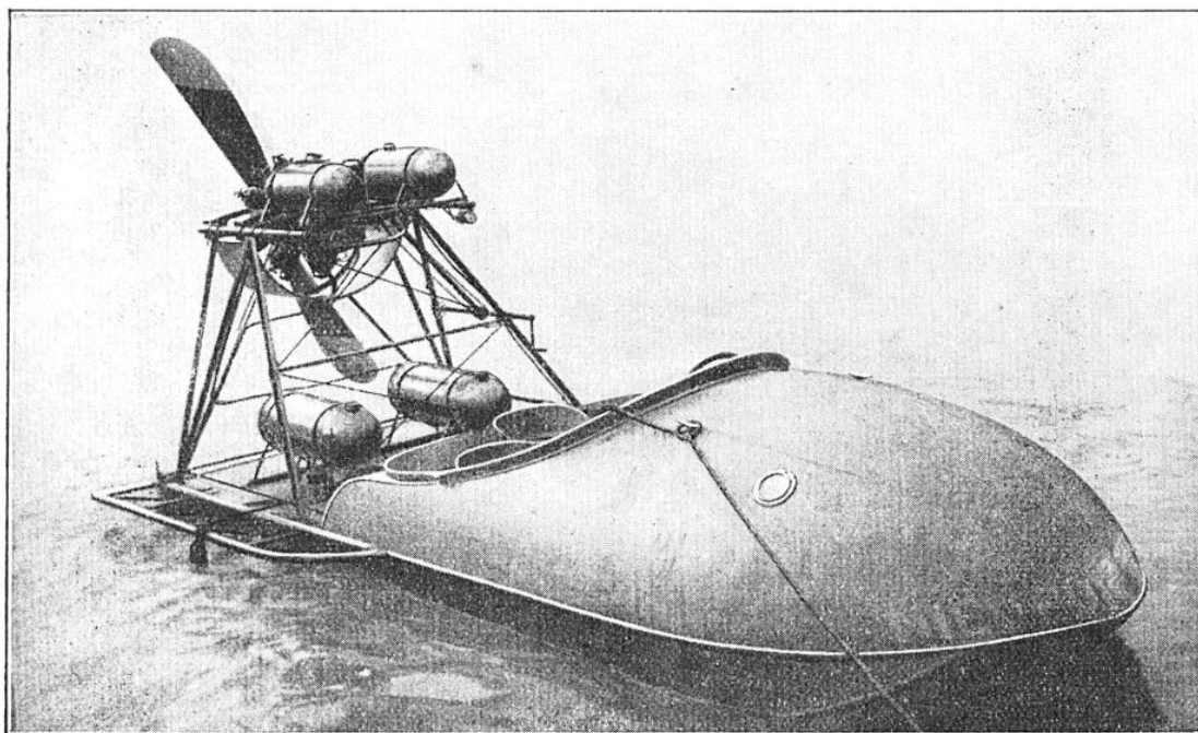
L'EMPLOI DE L'HÉLICE AÉRIENNE A CRÉÉ UNE NOUVELLE FORME DE YACHTING Voici un type d'hydroplane établi récemment par la maison Nieuport. Avec son hélice de trois mètres de diamètre actionnée par un moteur de 160 HP, il peut faire jusqu'à 60 kilomètres à l'heure.
