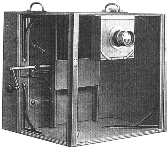
UN CHRONOPHOTOGRAPHE VU DE FACE
