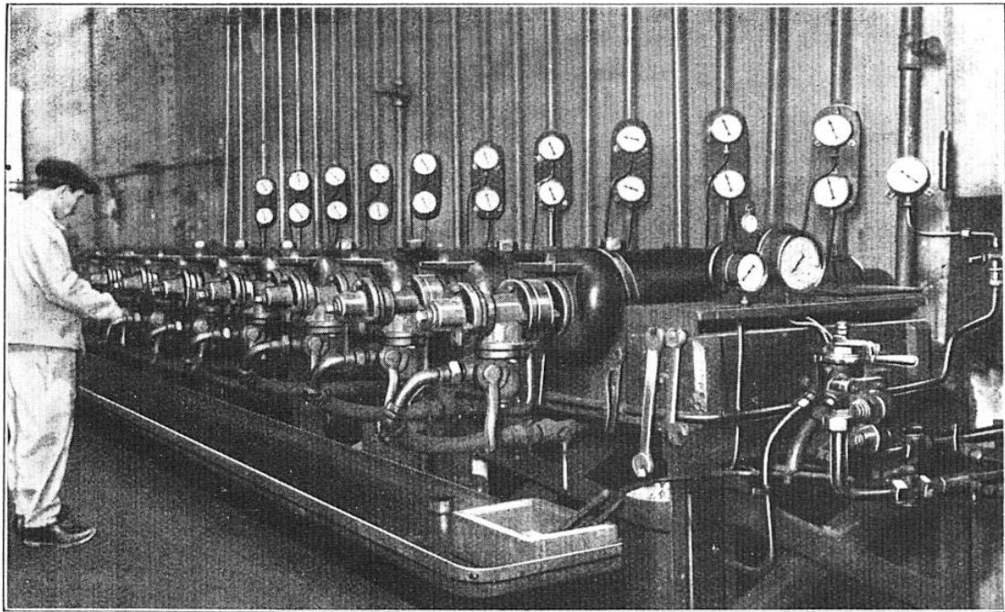
BANC POUR L'ESSAI DES TRIPLES VALVES A L'ATELIER
