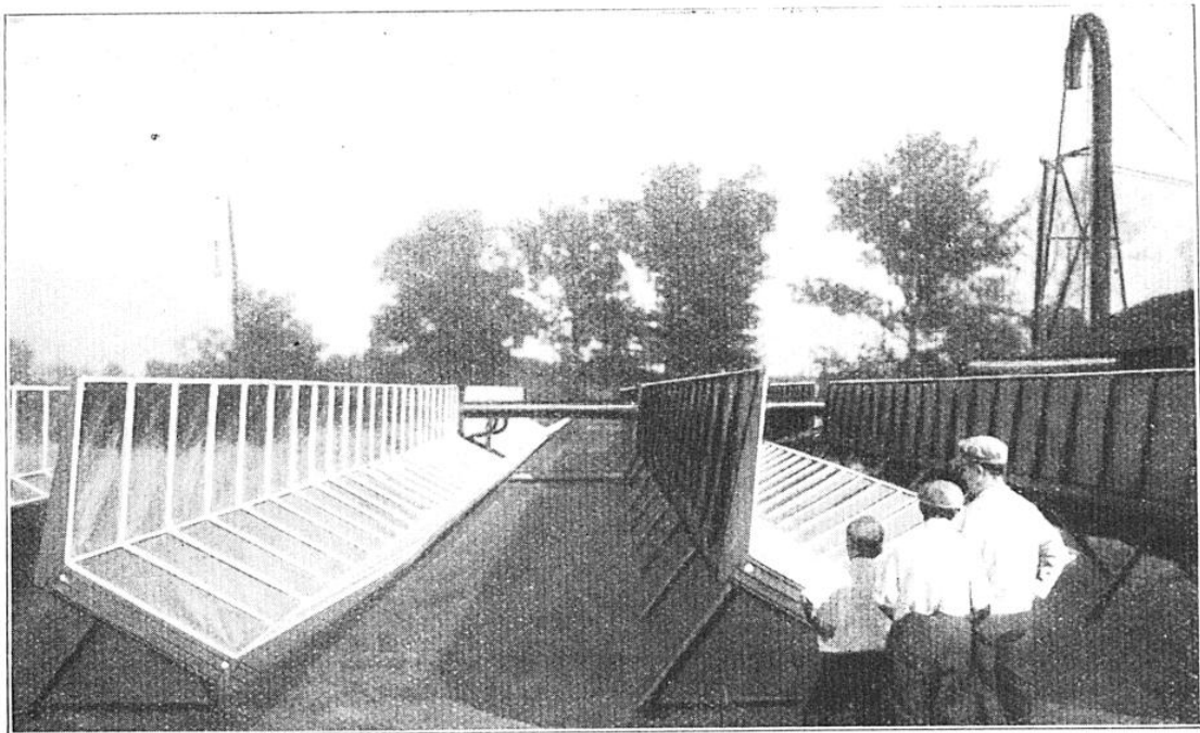
COLLECTEURS DE CHALEUR SOLAIRE AVEC, AU SECOND PLAN, LA CONDUITE GÉNÉRALE DE VAPEUR Toutes les trois semaines on inclinait un peu plus les collecteurs de façon que les miroirs puissent concentrer toujours la plus grande quantité possible de rayons sur les générateurs de vapeur. Il suffisait, pour cela, de soulever d'un côté les collecteurs sur leurs supports.
