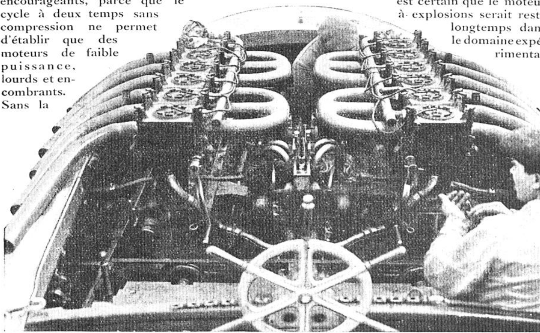
LA MACHINERIE MONSTRUEUSE D'UN CANOT AUTOMOBILE DE COURSE
