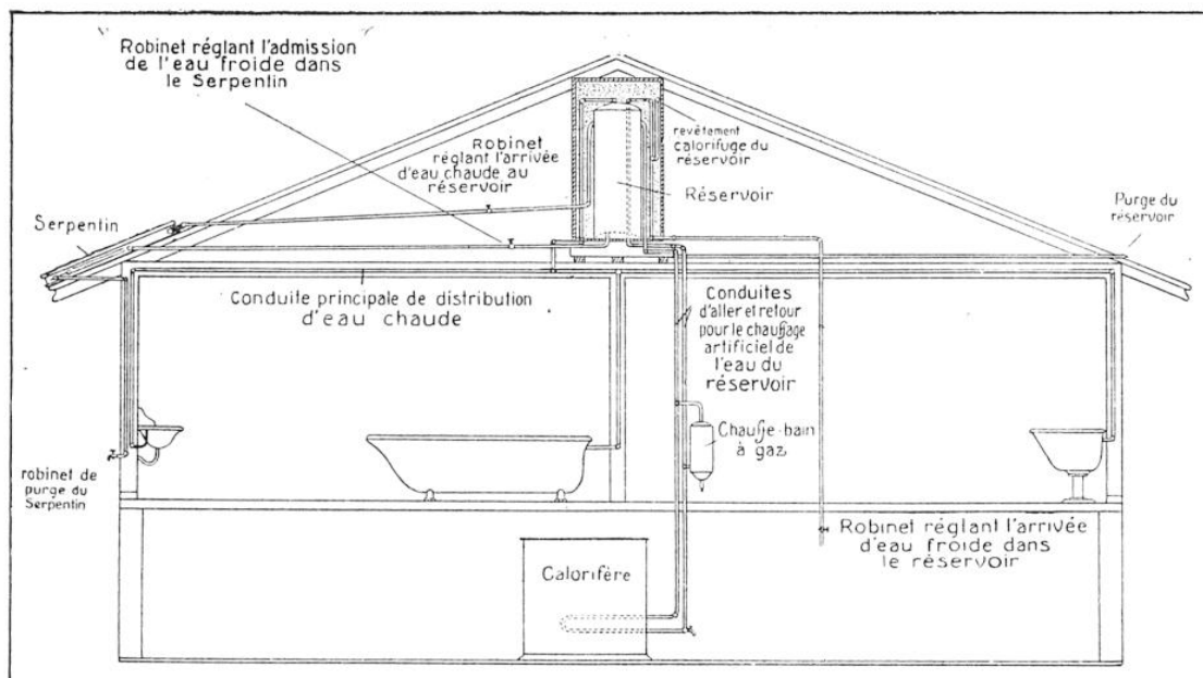
COUPE D'UNE MAISON DONT LES LOCATAIRES CHAUFFENT LEUR EAU ÉCONOMIQUEMENT
