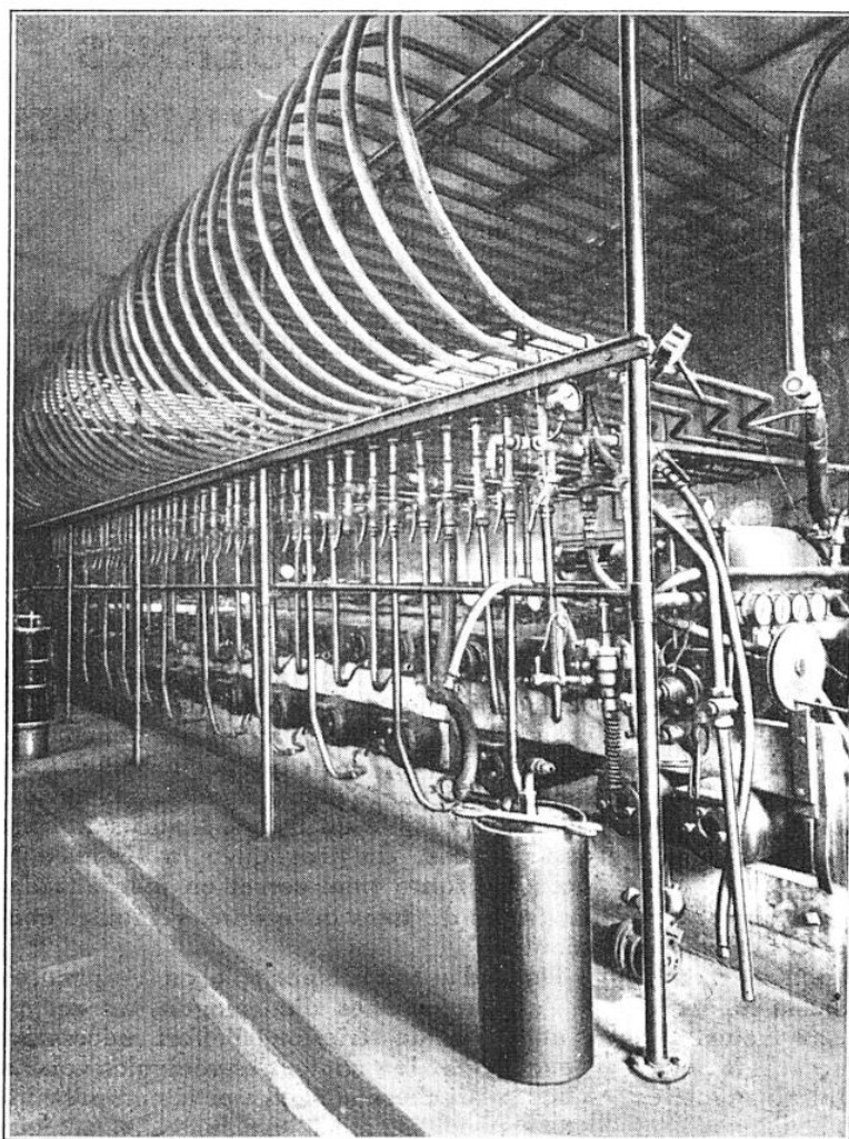
ESSAI AUX ATELIERS DES APPAREILS DE FREINAGE D'UN TRAIN
