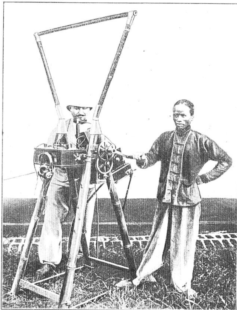
POSTE MOBILE DES TROUPES D'OCCUPATION AU TONKIN
