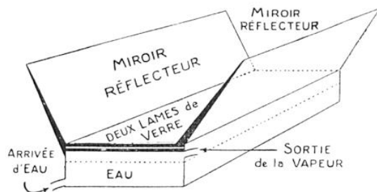
Schéma explicatif de la construction des premiers récepteurs solaires conçus et essayés par M. Shuman, à Philadelphie.
