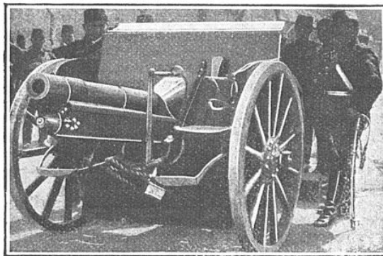
LA NOUVELLE PIÈCE DE CAMPAGNE TURQUE
