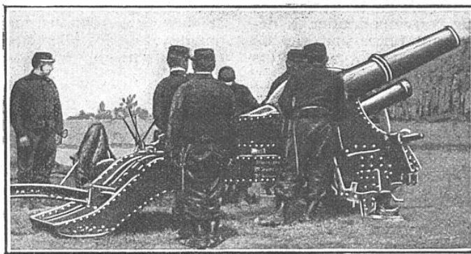
CANON COURT DE 155 MILLIMÈTRES, MODÈLE 1881
