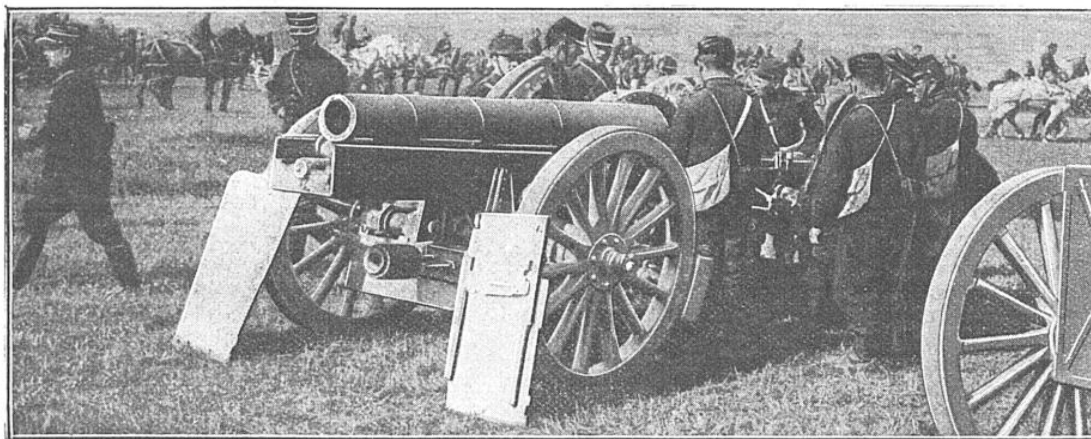
CANON RAIMBAULT DE 155 MILLIMÈTRES A TIR RAPIDE
