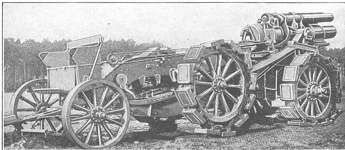
OBUSIER DE SIÈGE DE 21 CENTIMÈTRES ET SON AVANT-TRAIN
