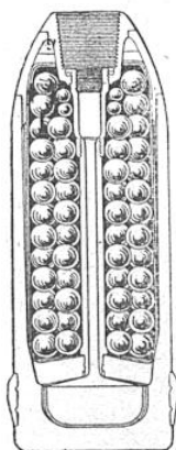
OBUS CHARGÉ DE BALLES, DIT SHRAP- NELL.
