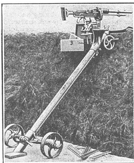
MITRAILLEUSE BELGE MUNIE D'UN SUPPORT A CRÉMAILLÈRE POUR LA HISSER A LA CRÊTE D'UN TALUS
