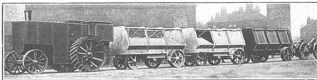
TRAIN BLINDÉ MARCHANT SUR ROUTE POUR LE TRANSPORT DU PETIT MATÉRIEL D'ARTILLERIE DE CAMPAGNE ET DES MUNITIONS
