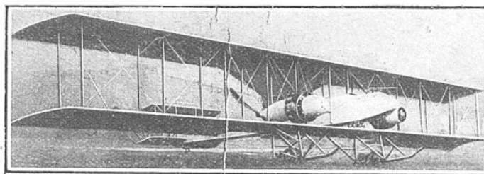
BIPLAN CONSTRUIT A CHALAIS-MEUDON
