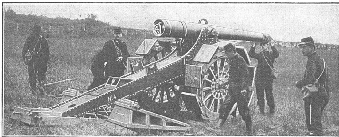
PIÈCE DE 120 MILLIMÈTRES MONTÉE AVEC CEINTURES DE ROUES
