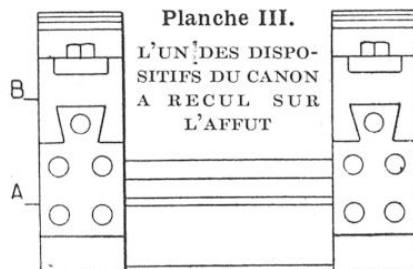
Planche III. L'UN DES DISPOSITIFS DU CANON A REcul SUR L'AFFUT A, glissières; B, patins porte-tourillons à queue d'aronde glissant sur les glissières et venant, à l'aide d'un piston, comprimer un ressort puissant disposé dans un cylindre relié à l'affût qui reste fixe.
