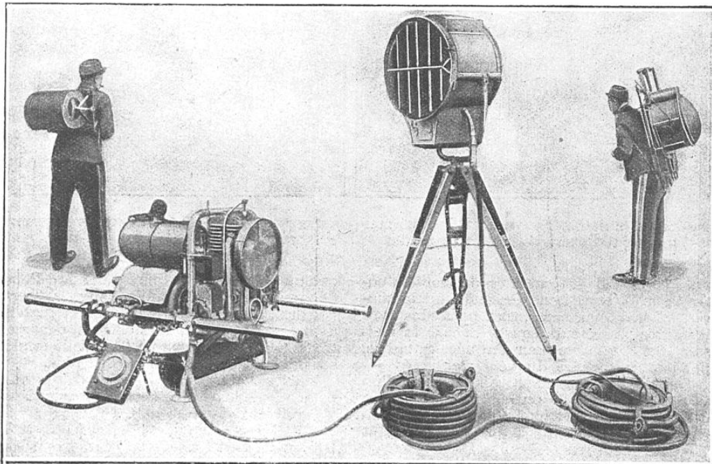
PROJECTEUR DE 1,20 m EN BATTERIE, AVEC SON GROUPE ÉLECTROGÈNE
