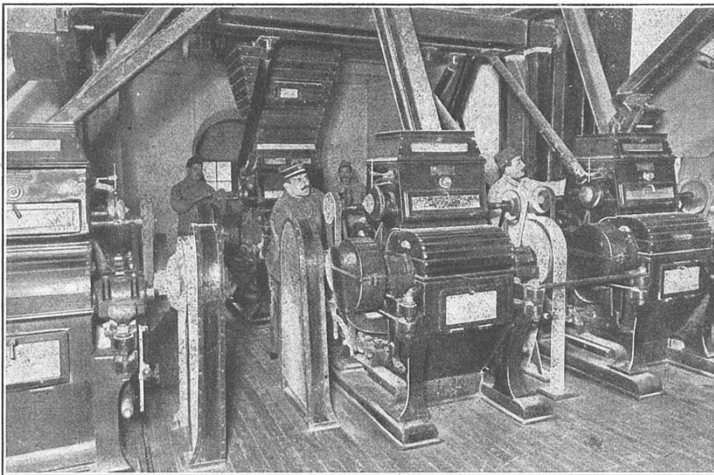
GROUPE DE CYLINDRES SERVANT A LA MOUTURE DU BLÉ
