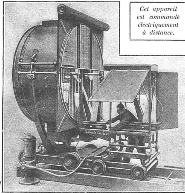
PROJECTEUR DE DEUX MÈTRES DE DIAMÈTRE POUR LA DÉFENSE DES CÔTES ET DES FORTERESSES
