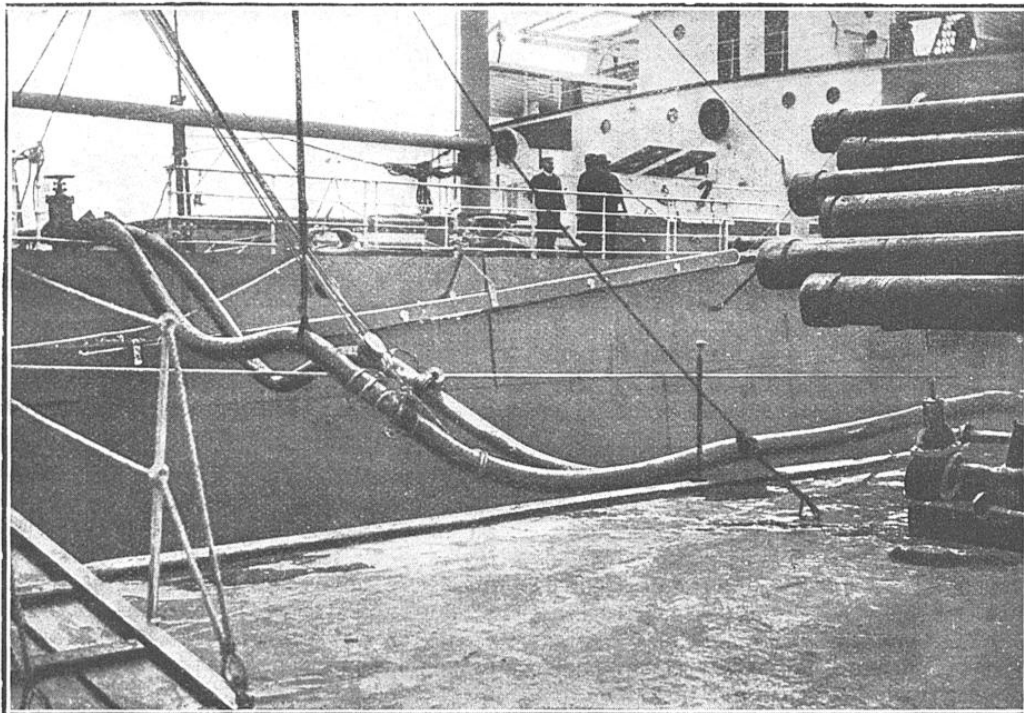
REMPLISSAGE DES SOUTES A PÉTROLE D'UN NAVIRE A QUAI L'opération est infiniment plus simple, et quelques hommes suffisent pour la mener à bonne fin.
