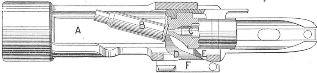
FIGURE MONTRANT COMMENT S'OPÈRE L'ÉJECTION DE L'ÉTUI D'UNE CARTOUCHE TIRÉE A, Boîte de culasse ; B, étui vide ; C, percuteur après le départ du coup ; D, éjecteur ; E, talon d'arrêt ; F, arrêt de culasse.
