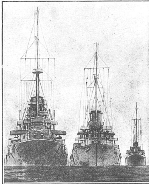
ERSATZ-WÖRTH, cuirassé de 28.000 t s (23 nœuds): Longueur 175 m , largeur 28 m , tirant d'eau 8 m 50. Artillerie: 8 canons de 38 cm, en 4 tourelles. Épaisseur minimum du cuirassement: 28 cm. Turbines de 60.000 chevaux; 4 hélices. Chaudières chauffées à la houille et au pétrole. SEYDLITZ, croiseur de bataille 25.000 t s (27 nœuds): Artillerie: 10 canons de 28 cm., 12 de 15 cm. Turbines Parsons de 63.000 chevaux; 3 hélices. Chaudières chauffées à la houille et au pétrole. S. 36-31, contre-torpilleur de 820 t s (32 nœuds): Turbines de 63.000 chevaux; chaudières mixtes.
