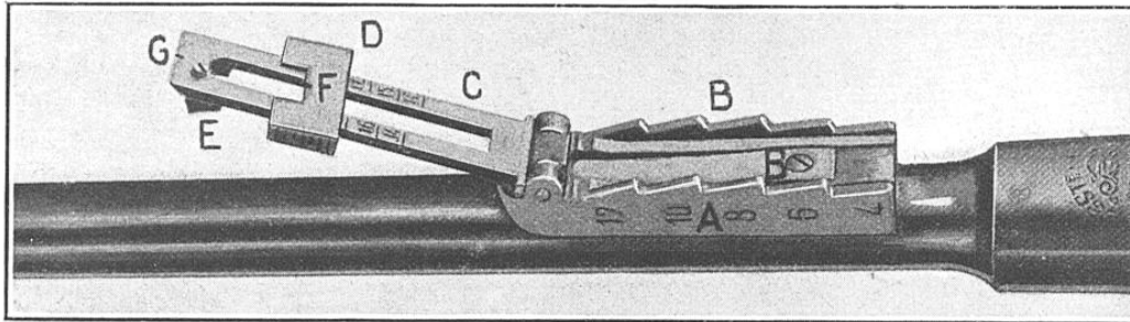
LA HAUSSE DU FUSIL MOSSINE
