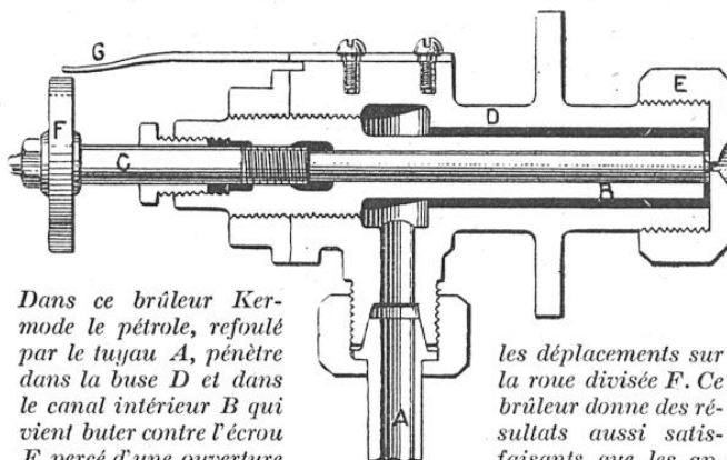
BRÛLEUR-PULVÉRISATEUR A PRESSION, TYPE MARINE
