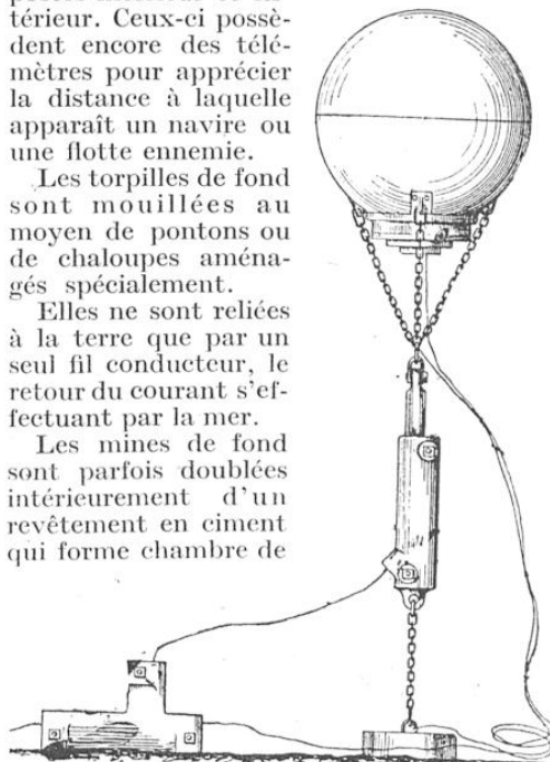
ON VOIT ICI LA MINE RETENUE PRÈS DE SON CRAPAUD PAR UN DISPOSITIF RENFERMANT UNE PETITE CHARGE EXPLOSIVE
