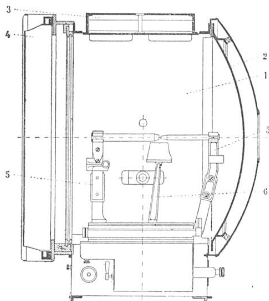
PROJECTEUR DE 60 CENTIMÈTRES, POUR VOITURE AUTOMOBILE OU HIPPOMOBILE 1, corps cylindrique ou tambour de l'appareil ; 2, miroir parabolique ; 3, ventilations ; 4, appareil d'occlusion ; 5, 5, porte-charbons ; 6, cendrier.
