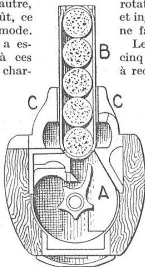
LE TRANSPORTEUR ROTATIF A PRÊT À RECEVOIR LES CARTOUCHES DU CHARGEUR B, CELUI-CI ÉTANT INTRODUIT DANS LA BOÎTE DE CULASSE C, C
