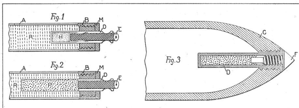
Planche IV. — CARTOUCHES-AMORCES POUVANT SERVIR DE DÉTONATEURS POUR LES OBUS ET OBUS-TORPILLES A PANCLASTITE
