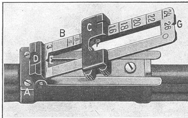
LA HAUSSE DU MANNLICHER MODÈLE 1895
