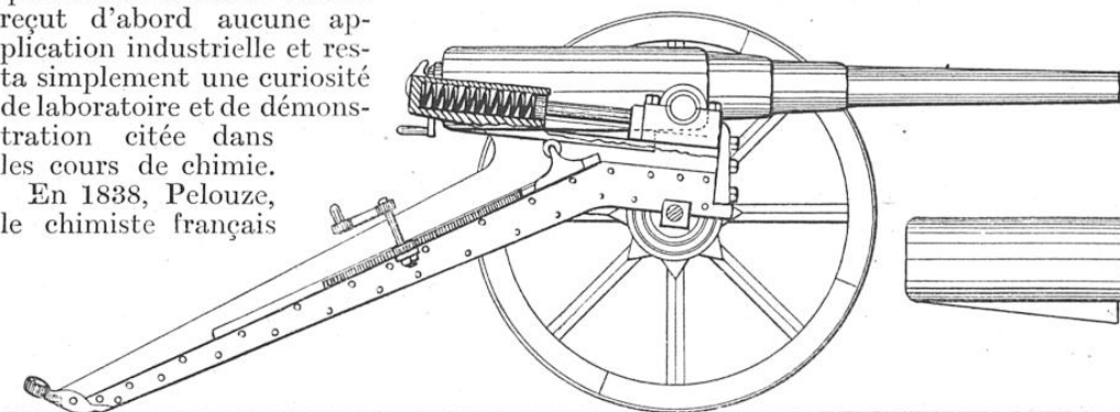
Planche II. — CANON A REcul SUR L'AFFUT INVENTÉ PAR M. TURPIN, EN 1881
