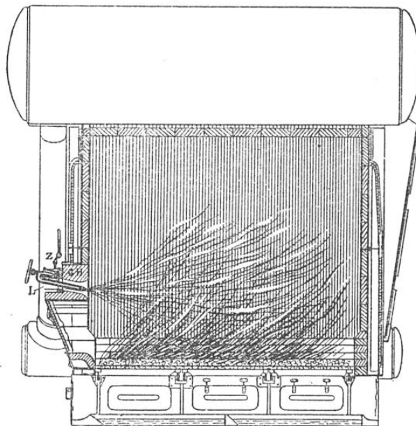
COUPE DU FOYER A PÉTROLE SYSTÈME KOERTING
