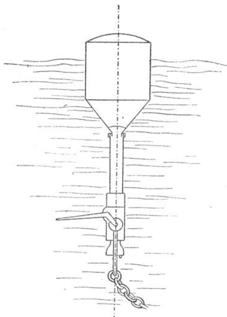
CLOCHE SUSPENDUE DANS UNE BOUÉE ET FONCTIONNANT AUTOMATIQUEMENT SOUS L'ACTION DES VAGUES
