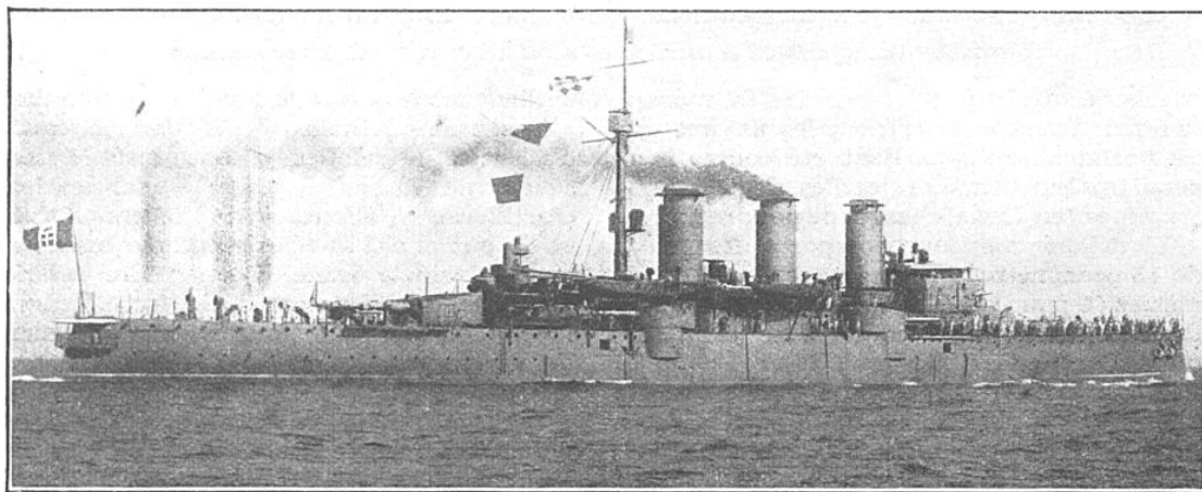
LE CROISEUR-CUIRASSÉ "AMALFI", DE 10.000 TONNES, 20.000 CH.; VITESSE : 22,5 NŒUDS L'armement se compose de 4 canons de 25 centimètres répartis par paires en deux tourelles axiales doubles et de 8 canons de 19 centimètres, dans quatre tourelles centrales.
