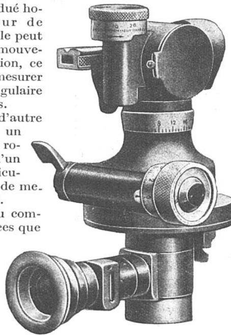
HAUSSE PANORAMIQUE POUR LE POINTAGE DES CANONS DE PETIT CALIBRE
