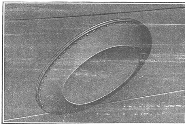
Le diaphragme de l'oscillateur Fessenden encastré extérieurement dans la coque d'un navire.
