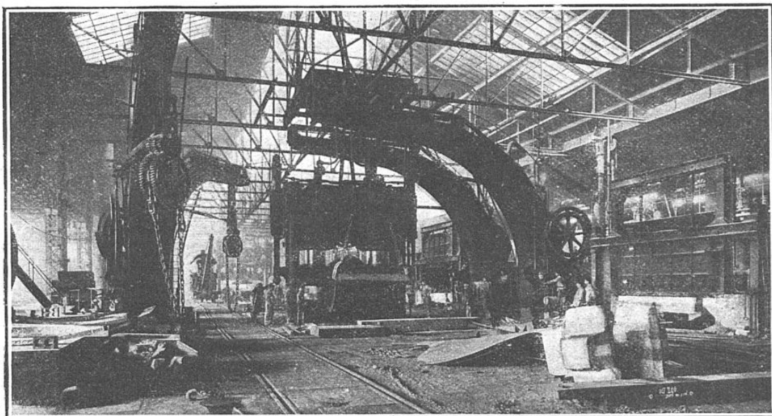
L'UNE DES GRANDES PRESSES HYDRAULIQUES A FORGER ET A GABARIER, DE 6.000 TONNES Ces presses puissantes, par leur travail silencieux, ont détrôné les marteaux-pilons.
