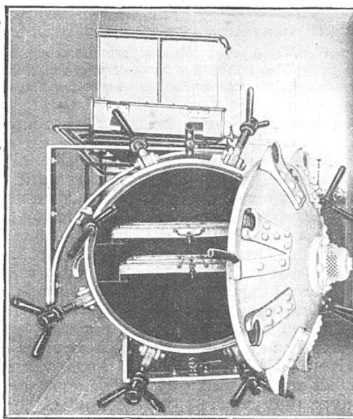
LE MÊME APPAREIL OUVERT
