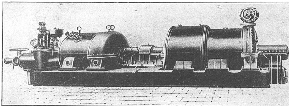
TURBO-COMPRESSEUR D'AIR SYSTÈME ZOELLY
