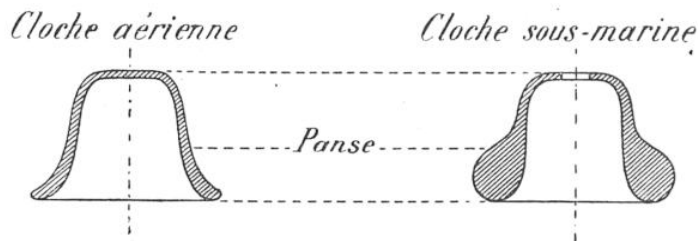
PROFILS ET TRACÉS COMPARÉS D'UNE CLOCHE TERRESTRE ET D'UNE CLOCHE SOUS-MARINE
