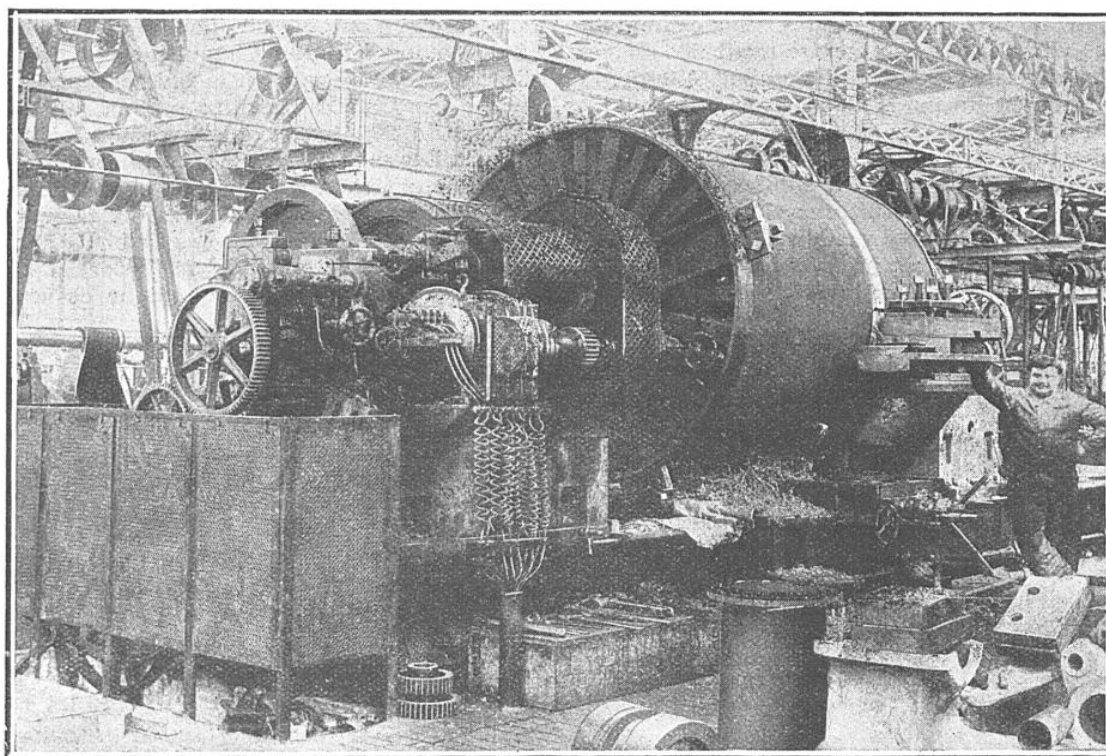
TOURNAGE DE LA PARTIE MOBILE D'UNE TURBINE MARINE
