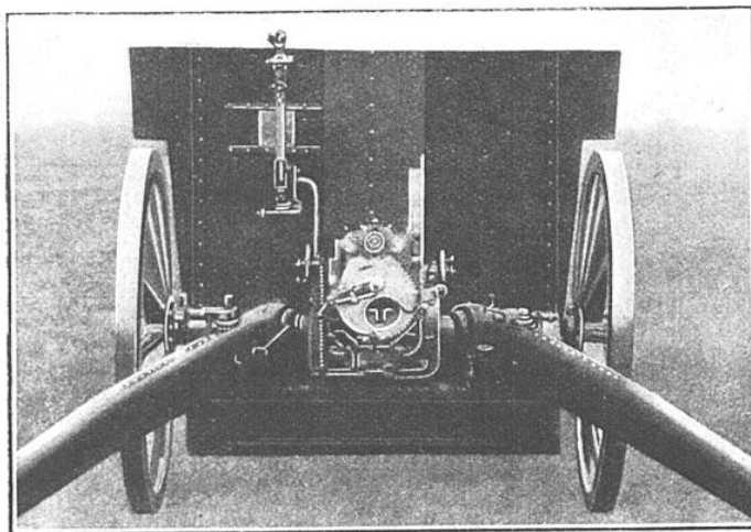
LA NOUVELLE PIÈCE DE CAMPAGNE ITALIENNE, A TIR RAPIDE, AVEC SES DEUX DEMI-FLÈCHES D'AFFUT
