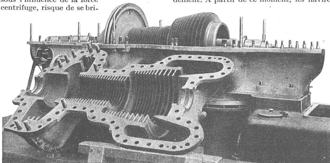
PARTIE MOBILE OU ROTOR ET ENVELOPPE D'UNE TURBINE MARINE A HAUTE PRESSION
