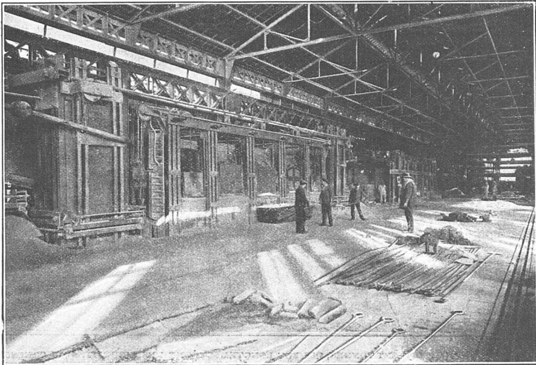
BATTERIES DE FOURS A ACIER, DU TYPE CRÉÉ PAR L'INGÉNIEUR MARTIN, MORT RÉCEMMENT. Une chargeuse électrique, que l'on aperçoit à l'extrémité droite de la photographie, permet de charger très rapidement cette longue suite de fours de 35 et 50 tonnes.
