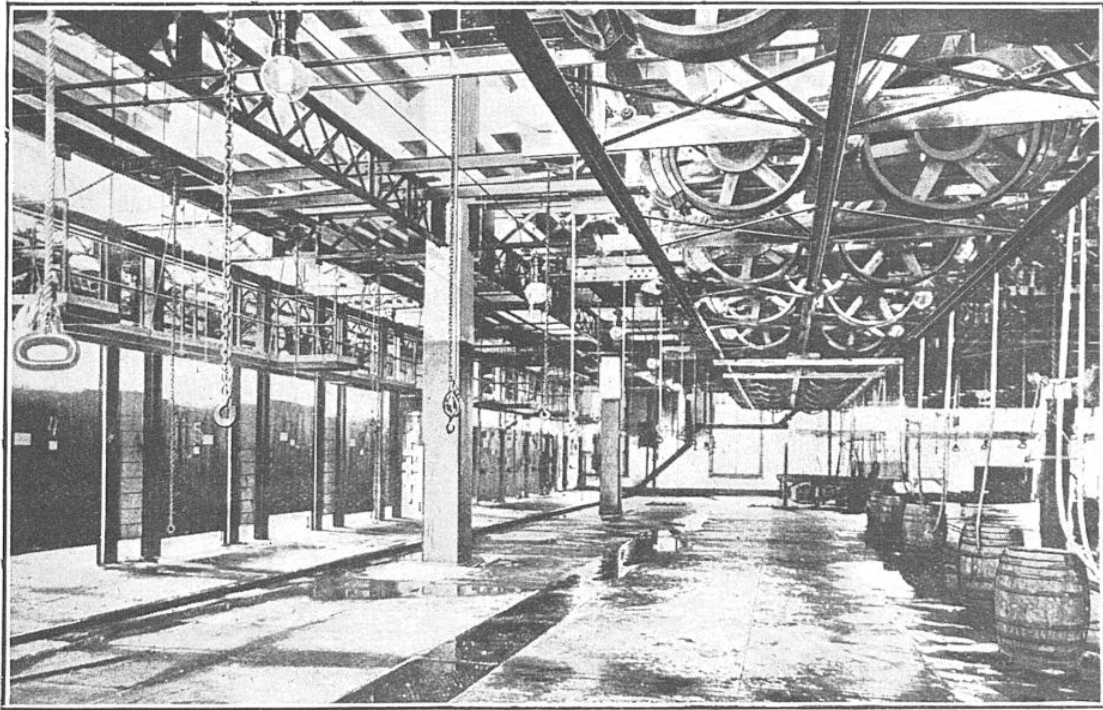
LES AGENCEMENTS MÉCANIQUES D'UNE SALLE D'ABATAGE DE BŒUFS
