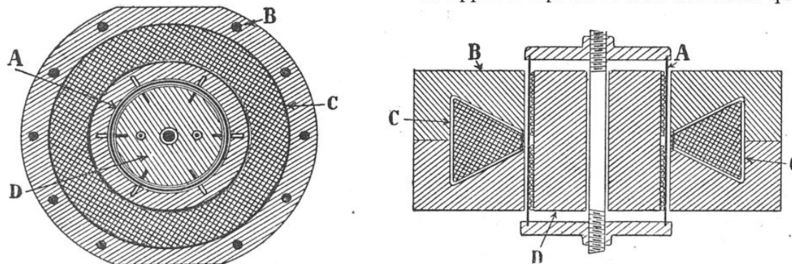
COUTES SCHÉMATIQUES DE L'OSCILLATEUR DU PROFESSEUR FESSENDEN
