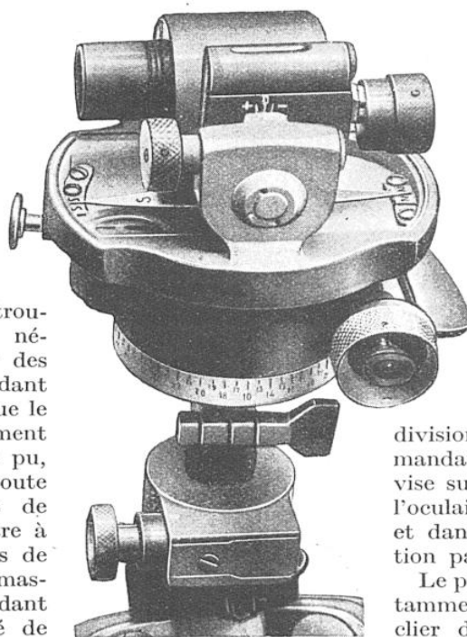
CERCLE DE POINTAGE A BOUSSOLE EMPLOYÉ DANS L'ARTILLERIE DE CAMPAGNE ET L'ARTILLERIE DE MONTAGNE ALLEMANDES
