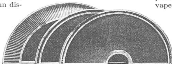
ROUES FIXES DE LA MÊME TURBINE
