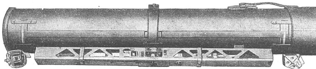
ÉTUI, ARMATURE INTÉRIEURE ET PRISMES D'EXTRÉMITÉS DU TÉLÉMÈTRE BARR AND STROUD
