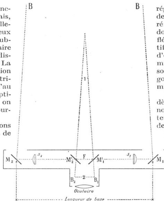
COUPE SCHÉMATIQUE D'UN TÉLÉMÈTRE MONOSTATIQUE A COÏNCIDENCE
