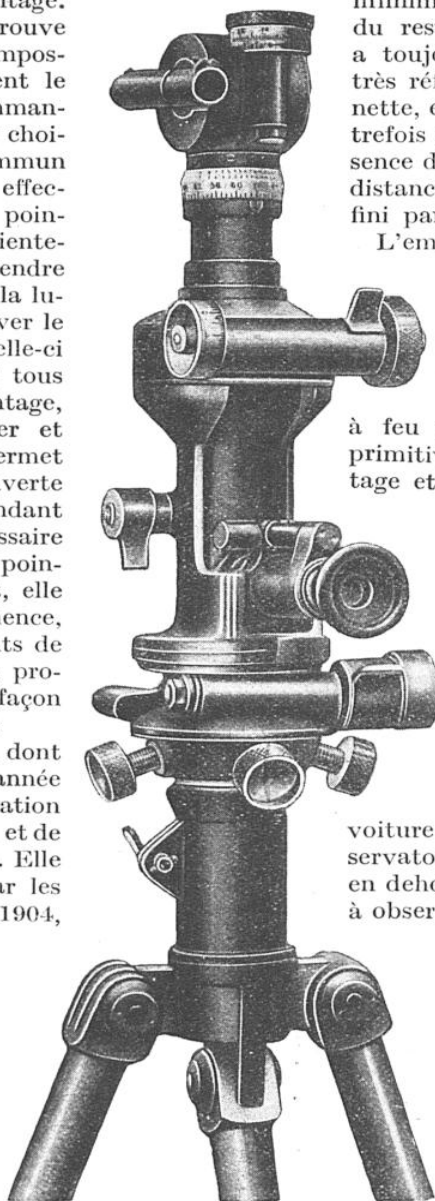
LUNETTE PANORAMIQUE DE BATTERIE MONTÉE EN TRÉPIED
