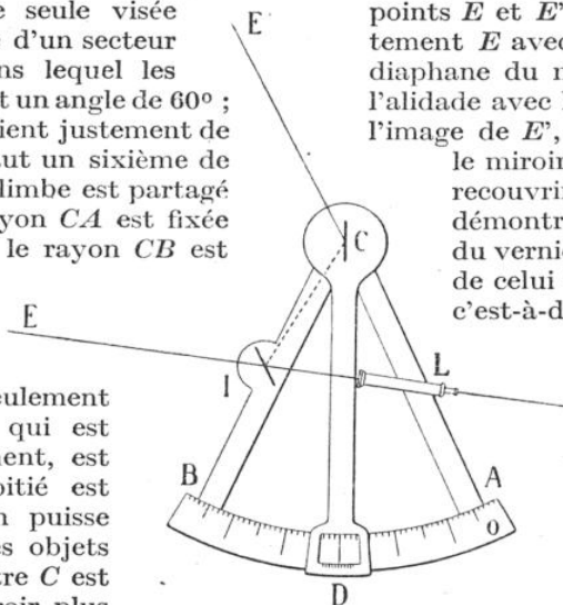
LE SEXTANT DE NEWTON
