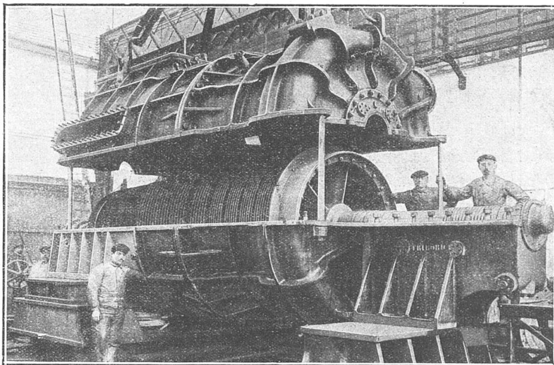
TURBINE A BASSE PRESSION SUR FOSSE D'ESSAIS, EN COURS DE MONTAGE
