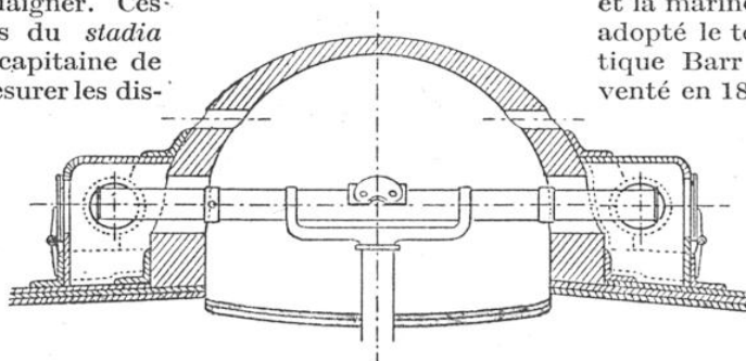
CAPOT BLINDÉ ABRITANT UN TÉLÉMÈTRE SUR LE TOIT D'UNE TOURELLE, A BORD D'UN CUIRASSÉ
