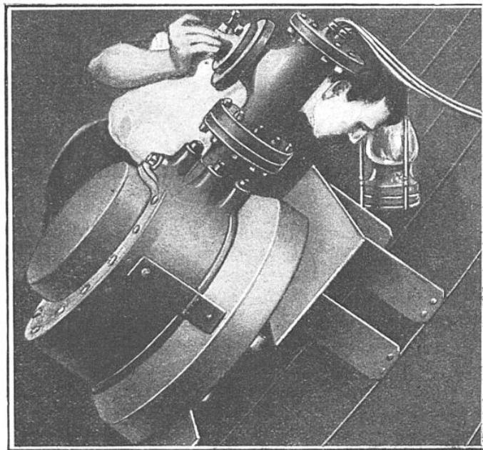
Montage d'un oscillateur Fessenden contre la coque d'un navire. Un deuxième appareil est fixé de l'autre bord.
