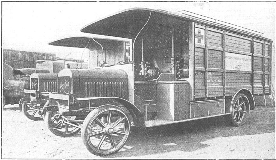
LES TROIS CAMIONS CONSTITUANT L'AMBULANCE CHIRURGICALE AUTOMOBILE MARCILLE Le camion figurant au premier plan de la photographie renferme les groupes électrogènes, pour l'éclairage de l'ambulance, et tout le matériel chirurgical nécessaire aux opérations.
