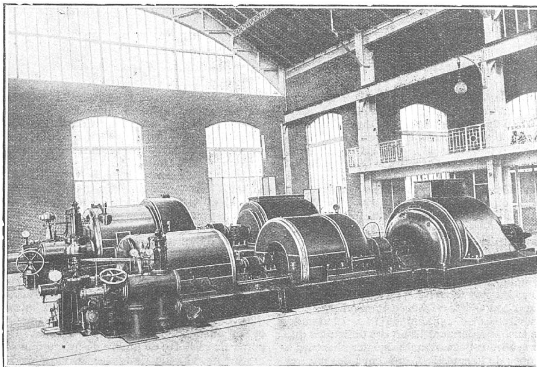
TURBINE COMPOUND ZOELLY EN SERVICE AUX HOUILLÈRES DE BÉTHUNE
