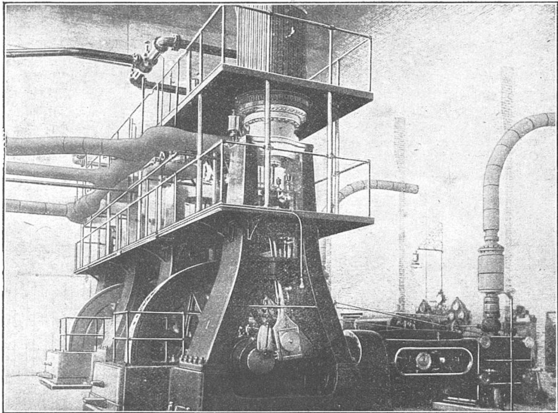
MACHINES FRIGORIFIQUES DU TYPE VERTICAL, SYSTÈME YORK
