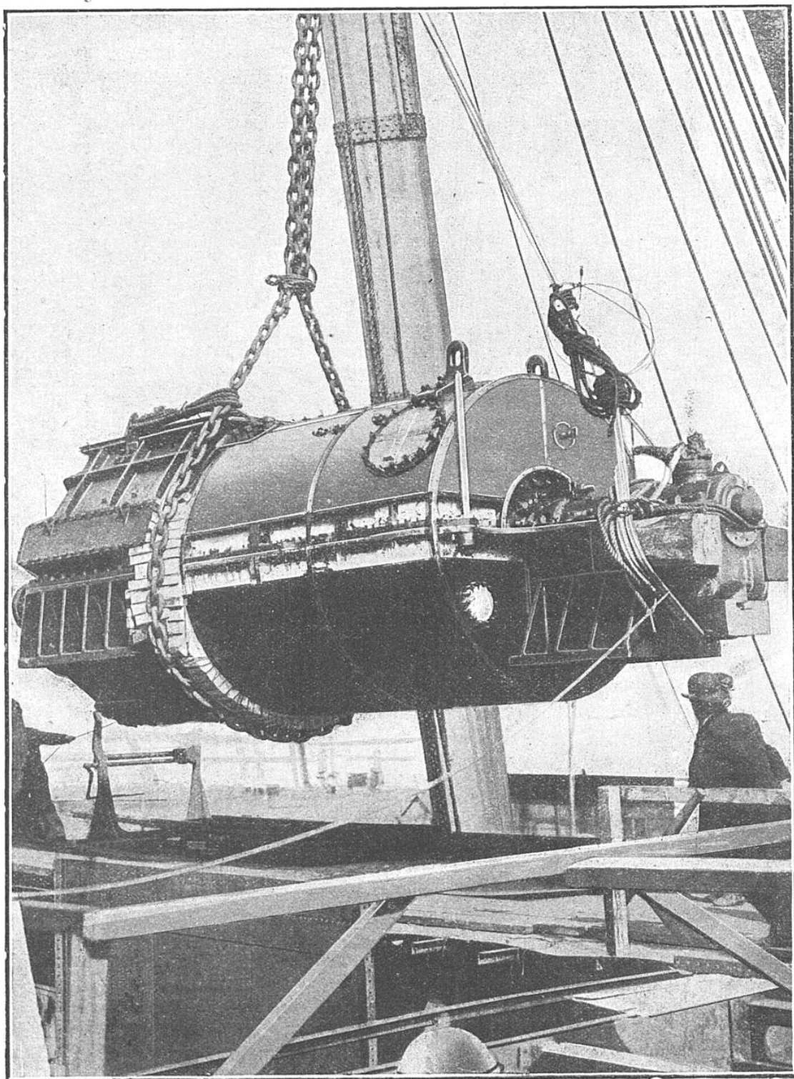
EMBARQUEMENT D'UNE TURBINE A HAUTE PRESSION A BORD D'UN NAVIRE Cette opération, assez délicate, exige l'emploi d'une bigue ou mâtire de grande puissance.
