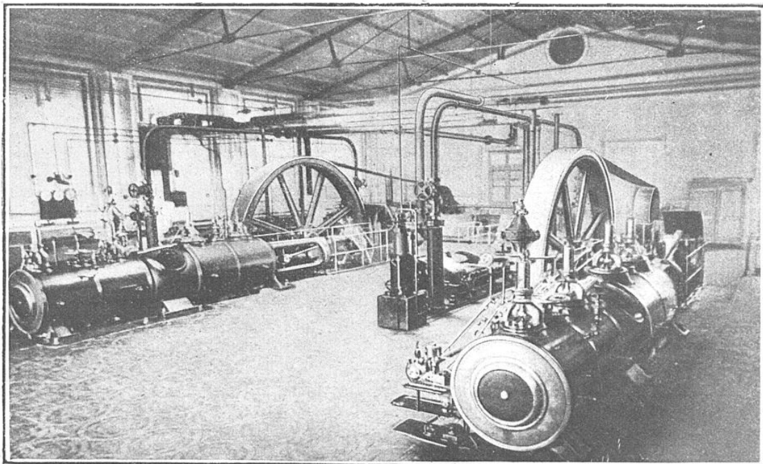
SALLE DES MACHINES SERVANT A PRODUIRE LE FROID DANS L'ENTREPOT FRIGORIFIQUE
