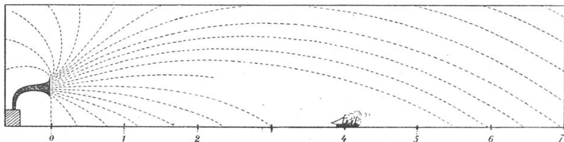
ZONE D'OPACITÉ ACOUSTIQUE DANS UNE ATMOSPHÈRE OPTIQUEMENT LIMPIDE
