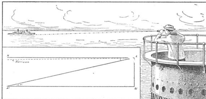
DÉTERMINATION DES DISTANCES DE TIR PAR LA MÉTHODE DITE DE DÉPRESSION
