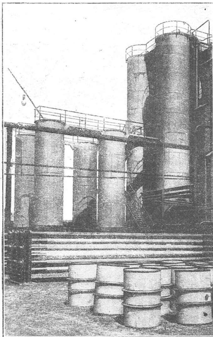
COLONNES A CLAIRES POUR LE LAVAGE DES GAZ ET RÉFRIGÉRANT MULTITUBULAIRE OU PASSENT LES HUILES DE GOUDRON APRÈS LEUR DÉBENZOLAGE
