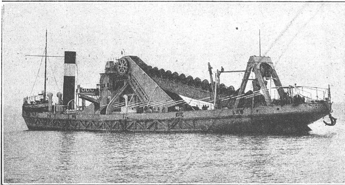
DRAGUE MARINE PORTEUSE, A GODETS, CONSTRUITE A RENFREW (ÉCOSSE) POUR L'ENTRETIEN ET L'APPROFONDISSEMENT DU CHENAL D'ACCÈS DE PORT-SAÏD
