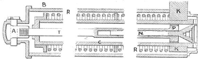
SCHÉMA DU BERCEAU ET DU FREIN DU 77 ALLEMAND
