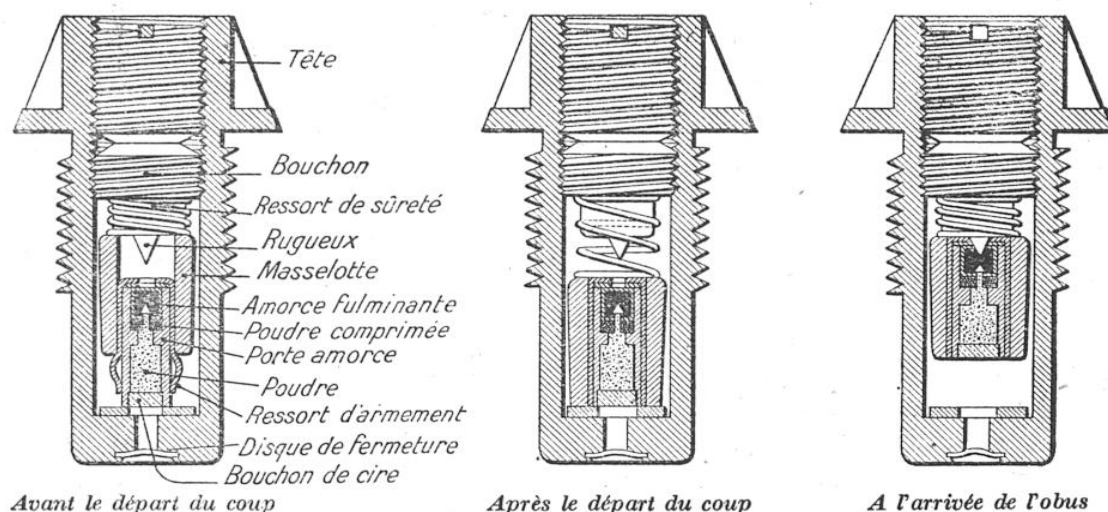
LES TROIS POSITIONS DU MÉCANISME INTÉRIEUR DE LA FUSÉE PERCUTANTE
