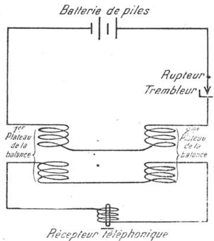
FIG. 5. — REPRÉSENTATION SCHÉMATIQUE DE LA BALANCE D'INDUCTION DE HUGHES
