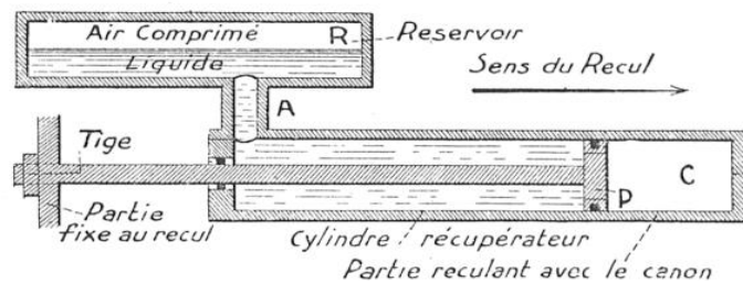
RÉCUPÉRATEUR DU FREIN HYDRAULIQUE ALLEMAND
