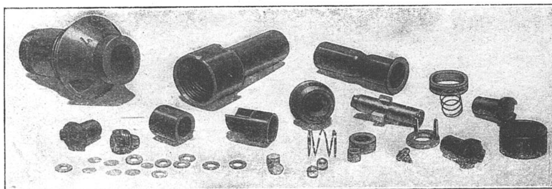
L'ASSEMBLAGE DE CES DIFFÉRENTES PIÈCES CONSTITUE LA FUSÉE PERCUTANTE
