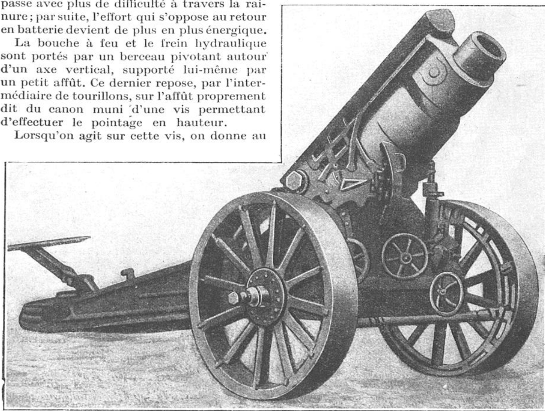
MORTIER DE CAMPAGNE KRUPP, DE 21 CENT., AVEC SON FREIN SURMONTANT LA PIÈCE
