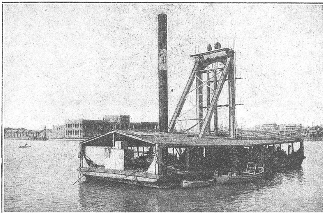
PILON DÉROCHEUR CONSTRUIT PAR LOBNITZ ET C O POUR L'APPROFONDISSEMENT DU CANAL ET EMPLOYÉ DANS LA SECTION DE SUEZ AUX LACS AMERS
