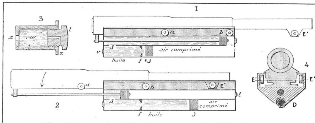
SCHEMA DU FONCTIONNEMENT DU FREIN DE TIR DANS LE CANON DE 75
