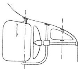
FIG. 4. — GOUVERNAIL AUXILIAIRE COMPENSÉ
