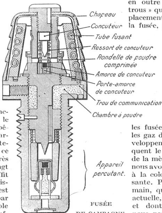
FUSÉE DE CAMPAGNE DITE FUSÉE A DOUBLE EFFET
