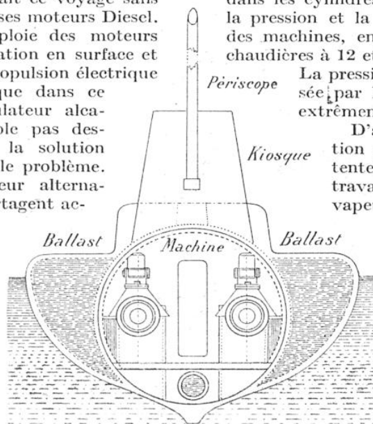
COUPE D'UN SOUS-MARIN ALLEMAND
