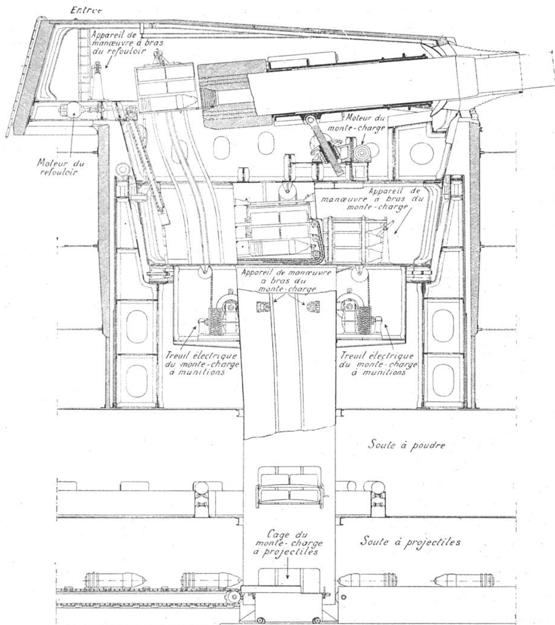
COUPE VERTICALE D'UNE TOURELLE ITALIENNE A DEUX CANONS
