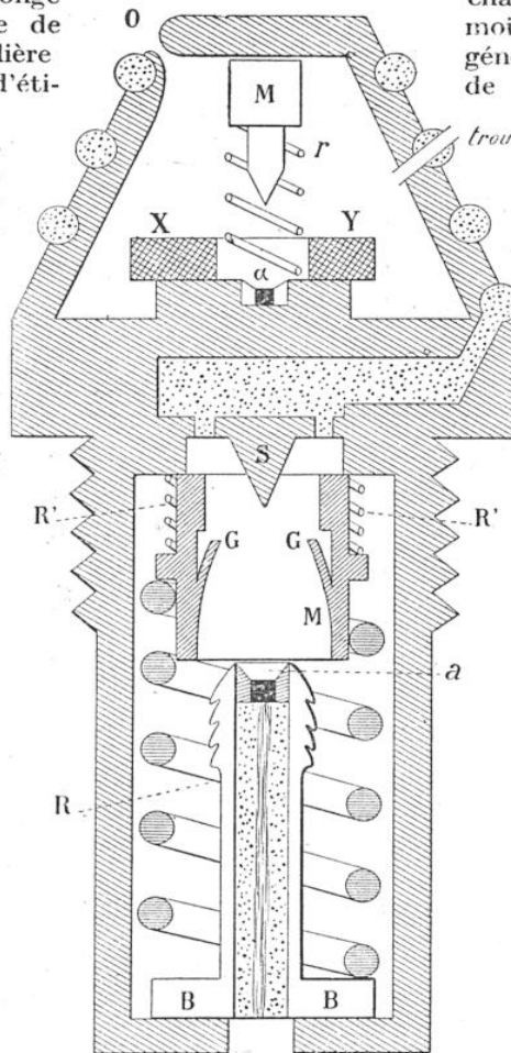
FUSÉE A DOUBLE EFFET DU 75
