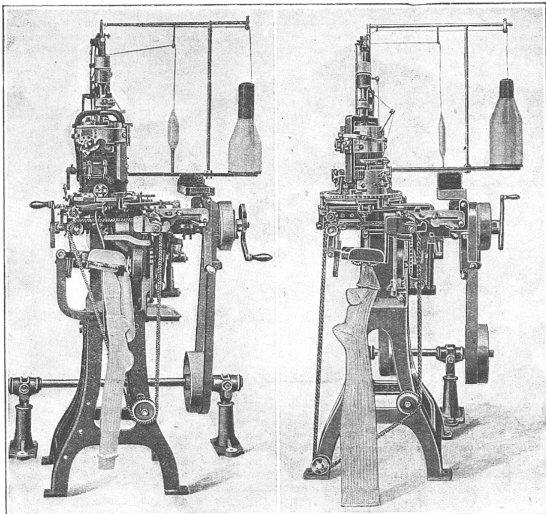
DEUX TYPES DE TRICOTEUSES CIRCULAIRES POUR LA FABRICATION DES BAS
