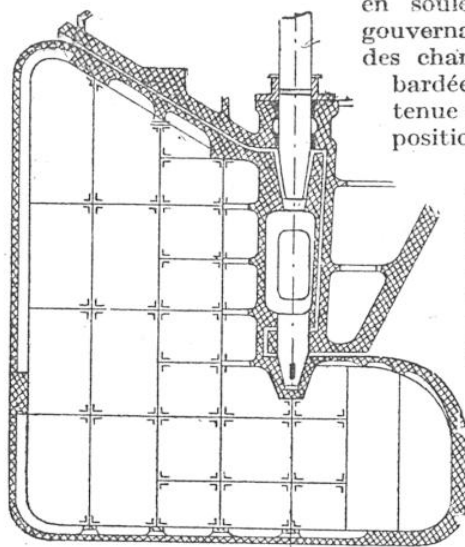
FIG. 3. GOUVERNAIL COMPENSÉ À AILERON
