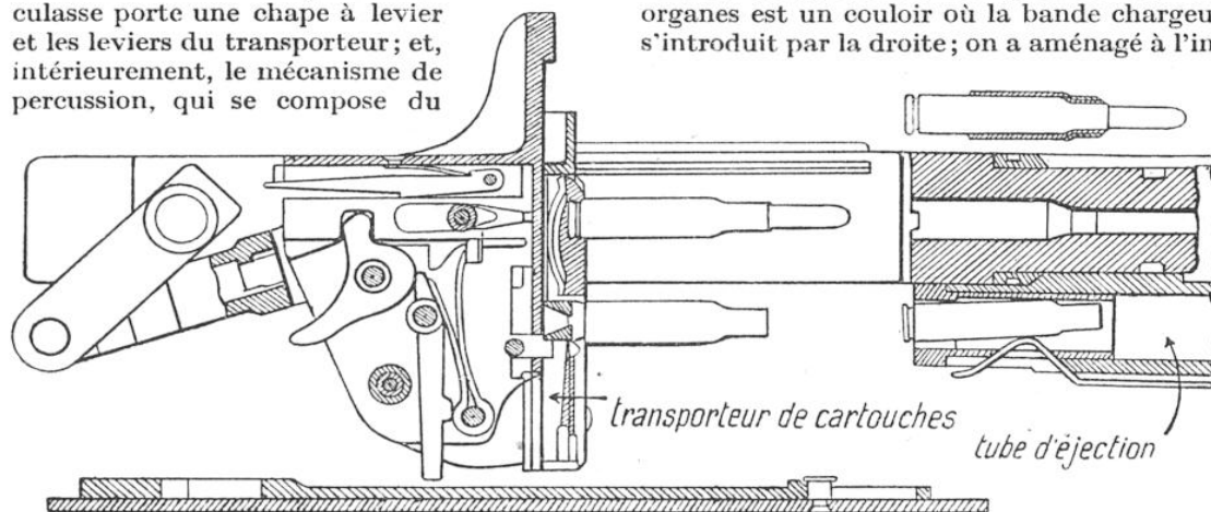
COUPE LONGITUDINALE DE LA CULASSE D'UNE MITRAILLEUSE MAXIM
