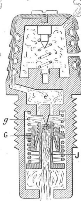
LA MÊME FUSÉE QUAND LE PROJECTILE RENCONTRE LE BUT
