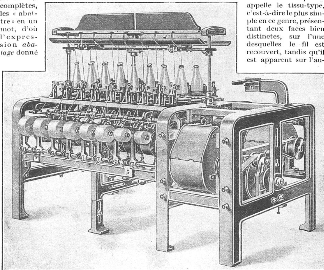
MACHINE A GAZER LE FIL DE COTON POUR LA FABRICATION DE LA BONNETERIE DE FIL
