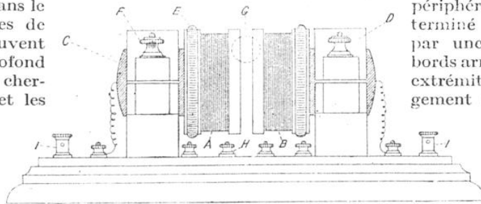
FIG. 9. — GROUPE FIXE DU CHERCHEUR-LOCALISEUR DE M. FRANÇOIS
