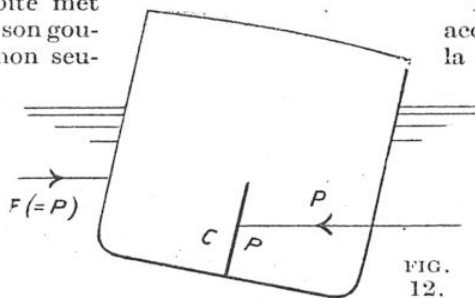
FIG. 12. LORSQU'IL COMMENCE A TOURNER, LE NAVIRE S'INCLINE D'ABORD EN DEDANS DE LA COURBE DE GIRATION
