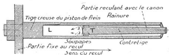
LE MODÉRATEUR DU MÊME APPAREIL
