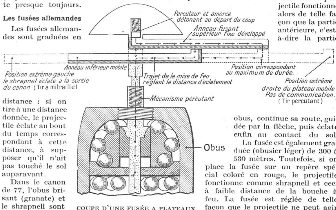
COUPE D'UNE FUSÉE A PLATEAUX
