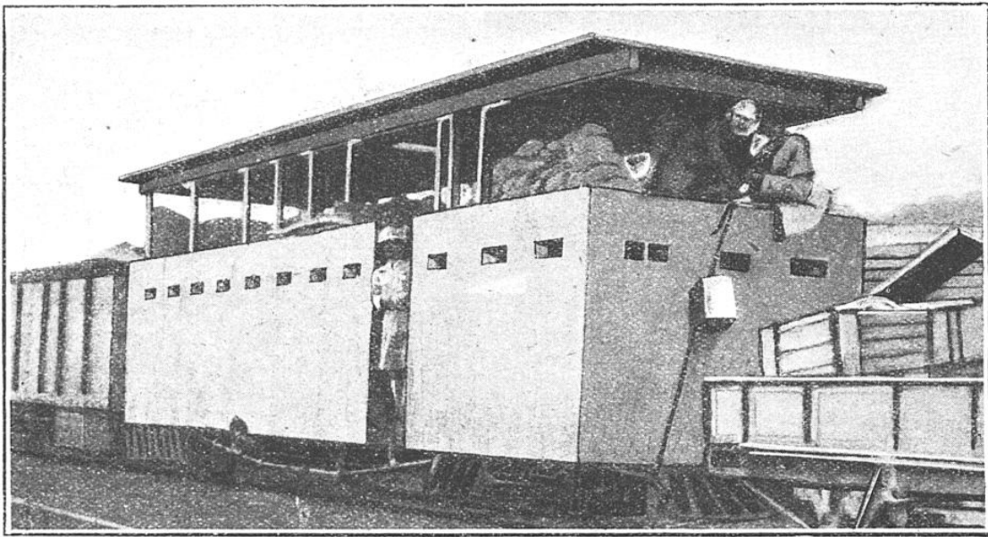
TYPE DE WAGON PROTÉGÉ EMPLOYÉ PAR LES ANGLAIS DANS LE SUD-OUEST AFRICAIN
