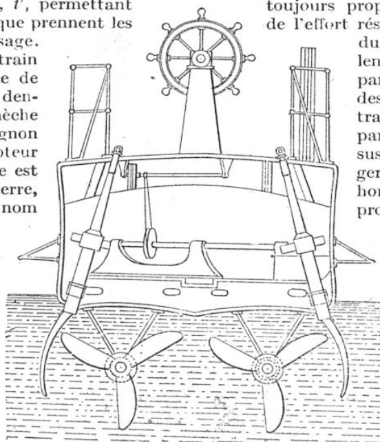
FIG. 6. — GOUVERNAILS ARQUÉS DES TORPILLEURS DU SYSTÈME THORNYCROFT
