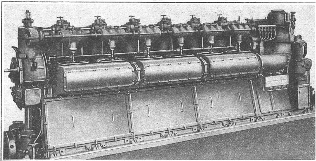
MOTEUR DE SOUS-MARIN CONSTRUIT EN SUISSE PAR LES USINES SULZER, A WINTERTHUR Ces usines ont fourni aux marines américaine et japonaise un certain nombre de moteurs à six cylindres, à deux temps, du type Diesel, qui dérivent des modèles fixes établis par les mêmes constructeurs.
