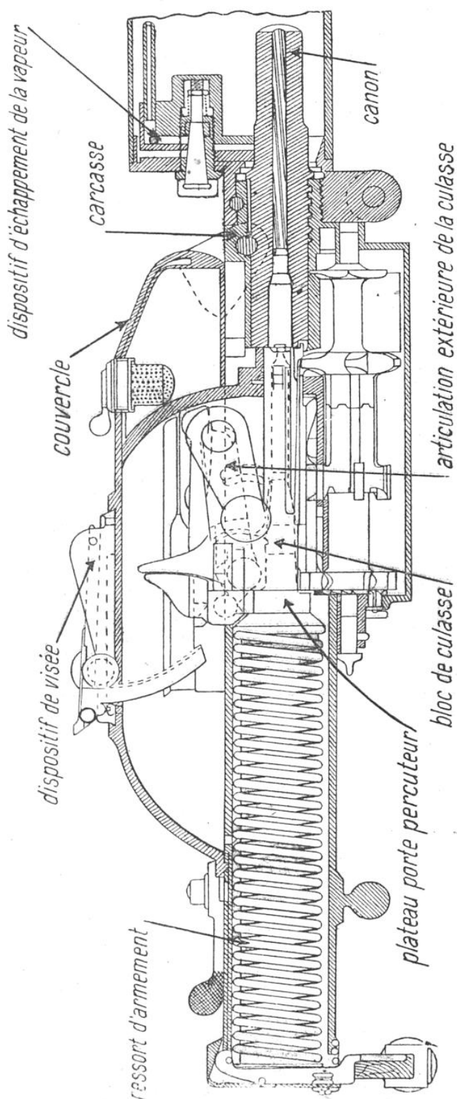
POSITION INITIALE DU PERCUTEUR ET DÉTAIL DU MÉCANISME DE LA MITRAILLEUSE AUTRICHIENNE SCHWARZLOSE
