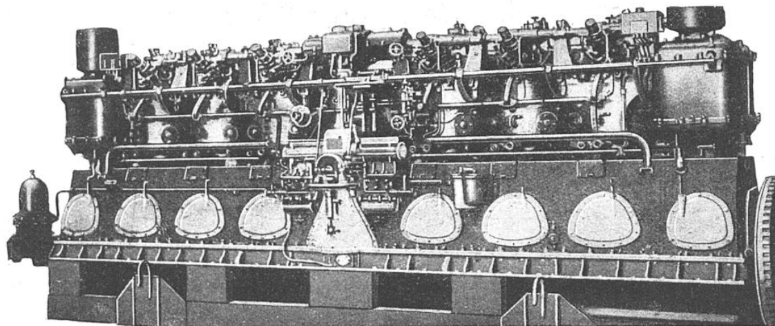
GRUPE-MOTEUR D'UN SOUS-MARIN ALLEMAND, CONSTRUIT AUX CHANTIERS "GERMANIA"
