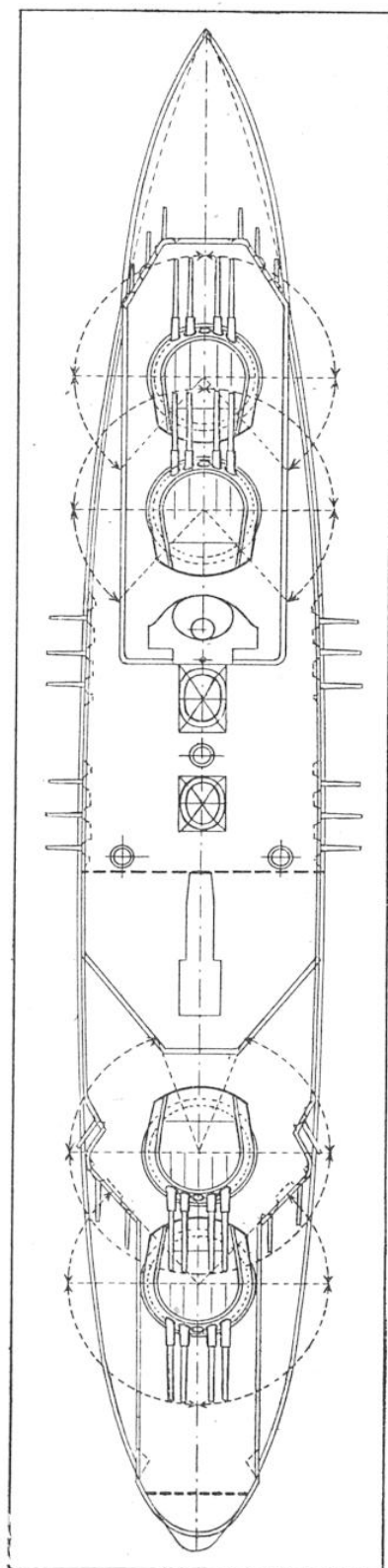
SCHEMA MONTRANT LA POSITION DES TOURELLES A BORD DES CUIRASSES FRANCAIS DU TYPE « DUQUESNE »
