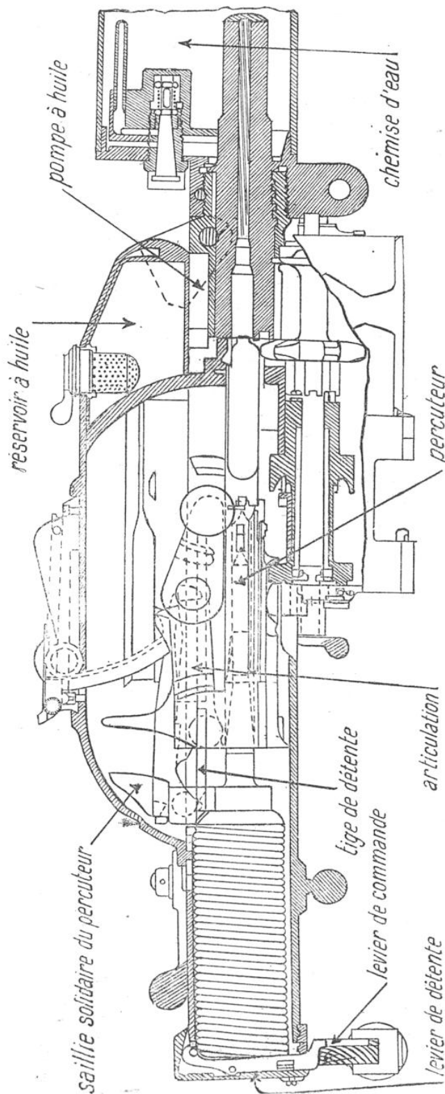
ASPECT DU MÉCANISME PENDANT LA DEUXIÈME POSITION DU PERCUTEUR DE LA MITRAILLEUSE SCHWARZLOSE
