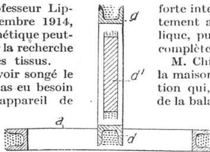
FIG. 7. — COUPE DE L'APPAREIL CHILOWSKY
