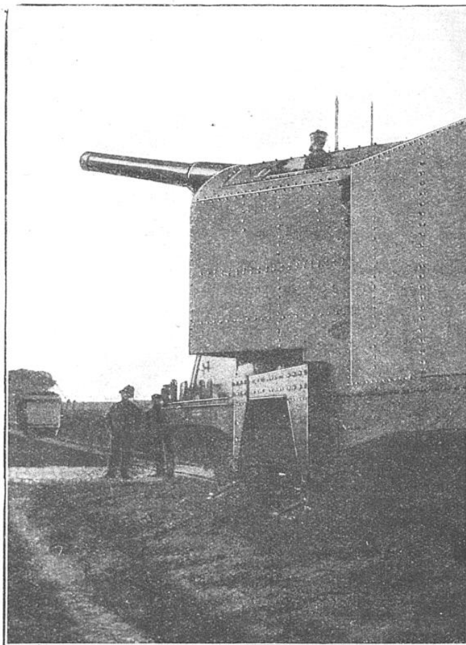
PIÈCE DE MARINE DE MOYEN CALIBRE INSTALLÉE SUR UN TRAIN BLINDÉ FRANÇAIS
