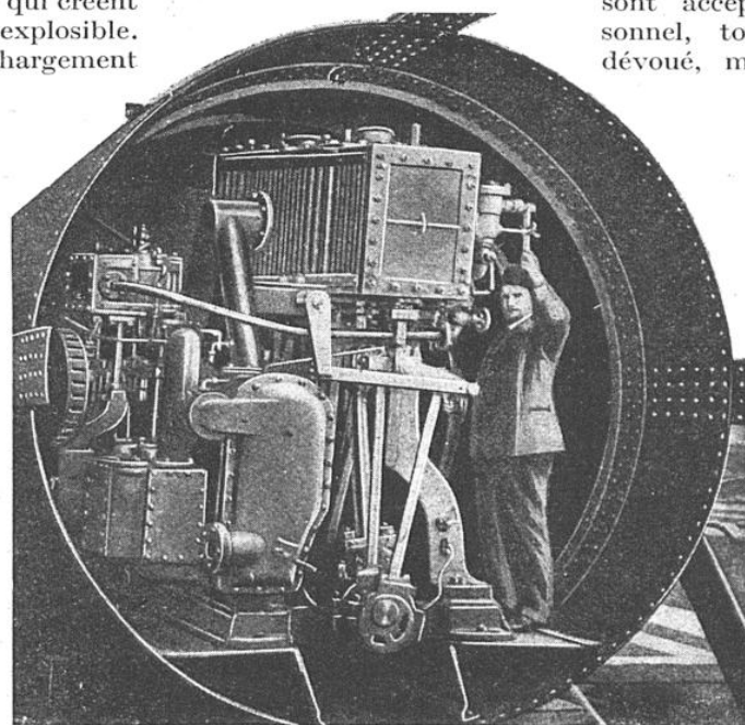
MOTEUR VERTICAL. TYPE PILON, ALIMENTÉ PAR LA CHAUDIÈRE A VAPEUR CI-DESSUS
