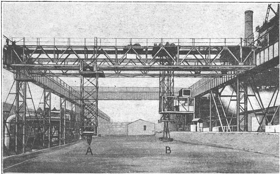
PONT DE COULÉE ÉLECTRIQUE DES ACIÉRIES THYSEN, A HAGONDANGE (LORRAINE ALLEMANDE). — A. MARTEAU CASSE-FONTE ; B, AIMANT DE LEVAGE
