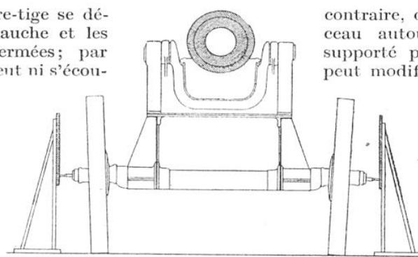
DISPOSITIF DE PANNEAUX INSTALLÉS POUR PERMETTRE D'ENREGISTRER LE REcul D'UN CANON AU MOMENT DU TIR D'ESSAI
