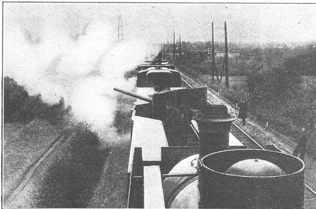
TRAIN BLINDÉ BELGE ARRÊTÉ EN PLEINE VOIE ET FAISANT FEU DE TOUTES SES PIÈCES SUR UN CONVOI DE RAVITAILLEMENT ENNEMI ÉCHELONNÉ LE LONG D'UNE ROUTE
