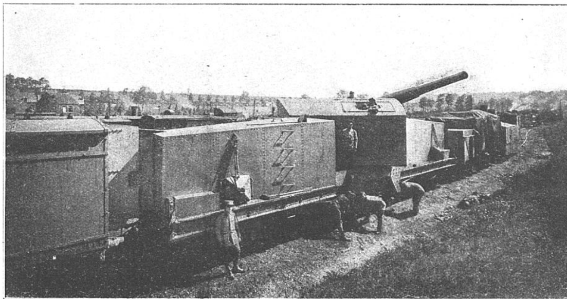
TRAIN BLINDÉ FRANÇAIS PARTANT POUR EFFECTUER UN BOMBARDEMENT
