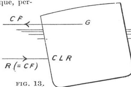
FIG. 13. SI LA BARRE EST MAINTENUE TOUT D'UN BORD, LE NAVIRE SE REDRESSE PUIS S'INCLINE EN SENS INVERSE
