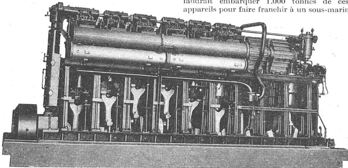
PETIT MOTEUR A COMBUSTION INTERNE, DE 150 CHEVAUX, POUR SUBMERSIBLE
