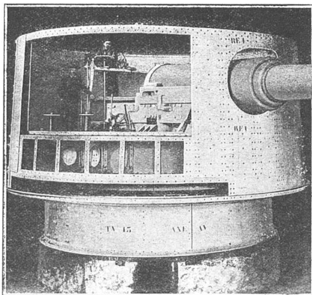
TOURELLE RENFERMANT UN CANON DE 274 mm
