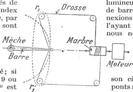
FIG. 8. — ENTRAÎNEMENT DE LA BARRE
