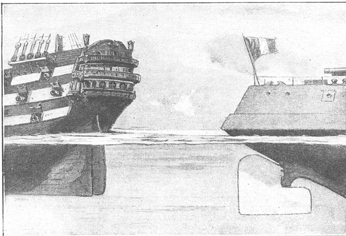
LE GOUVERNAIL D'UN ANCIEN TROIS-PONTS ET CELUI D'UN CUIRASSÉ MODERNE
