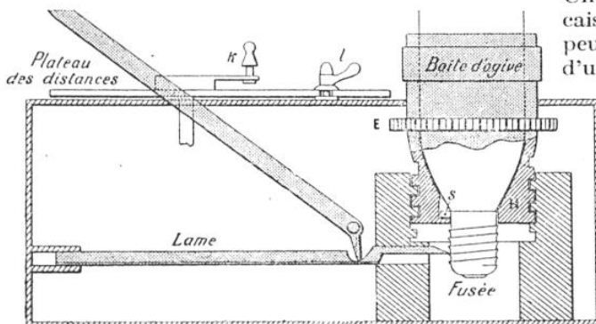
MÉCANISME DE LA PERCÉE D'UNE FUSÉE DANS LE DÉBOUCHOIR DU CANON DE 75
