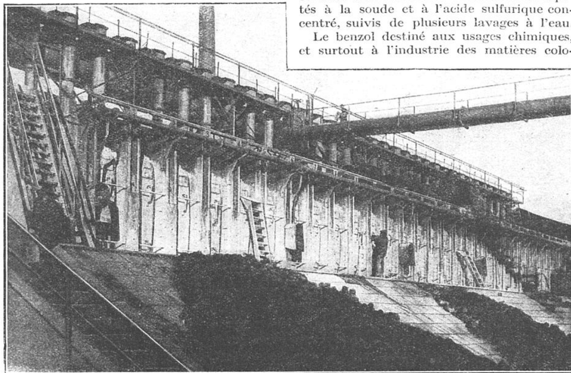
FAÇADE ET AIRE DE DÉFOURNEMENT DE FOURS À COKE, A FIRMINY (LOIRE)
