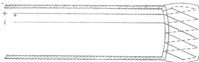
FIG. 4. - SONDE EXPLORATRICE ÉLECTRIQUE DE MM. MAUCLAIRE ET GARIN
