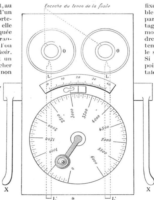
VUE, EN PLAN, DU DÉBOUCHOIR DU 75
