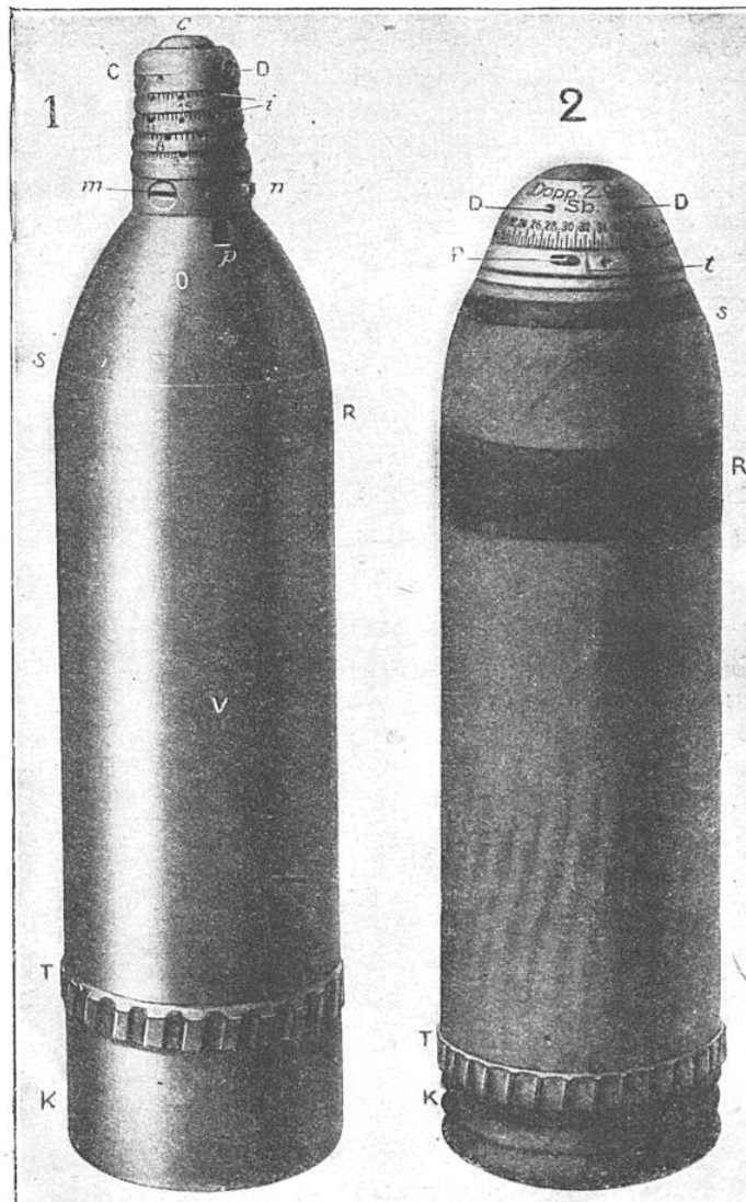
FIG. 1. — SHRAPNELL FRANÇAIS DE 75 FIG. 2. — SHRAPNELL ALLEMAND DE 77 (Ces deux projectiles ont été tirés).
