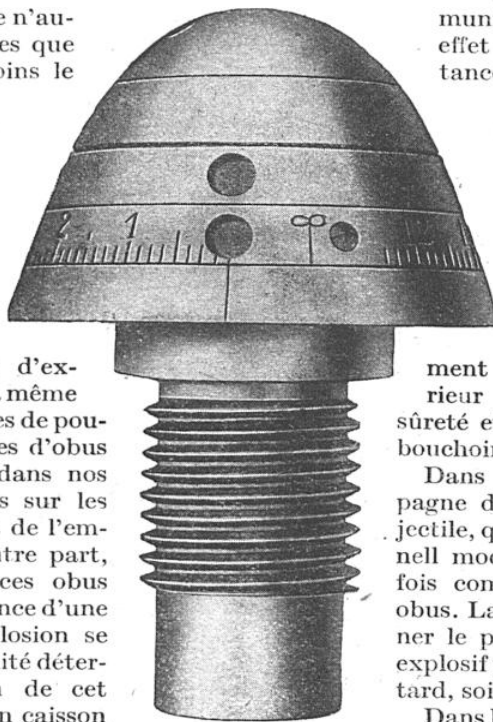
FUSÉE A PLATEAUX
