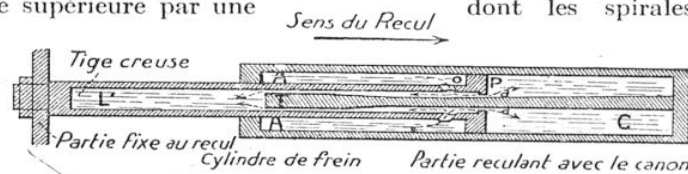
FREIN HYDRAULIQUE D'UN CANON LOURD ALLEMAND
