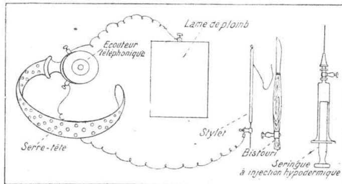
FIG. 3. — MÉTHODE DU DOCTEUR HEURARD POUR LA RECHERCHE DES CORPS MÉTALLIQUES DANS LES TISSUS
