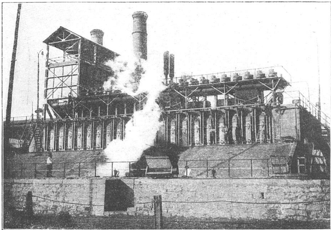
BATTERIE DE FOURS A COKE A DOUBLE BARILLET, VUE DU COTÉ DU DÉFOURNEMENT (MINES DE ROCHE-LA-MOILLÈRE ET FIRMINY)
