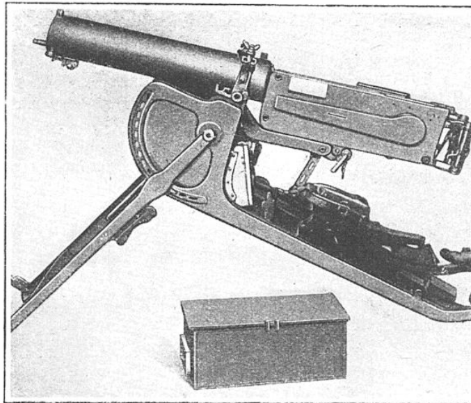
AUTRE SYSTÈME D'AFFUT DE LA MITRAILLEUSE MAXIM
