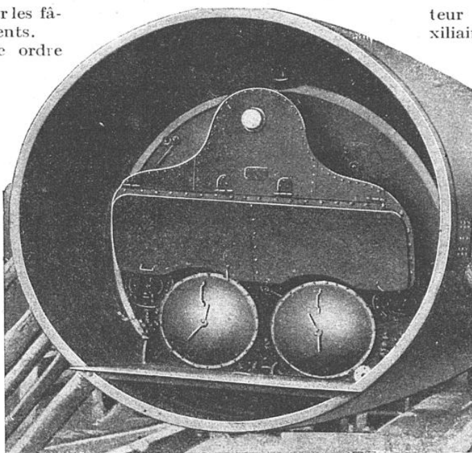
TYPE DE CHAUDIÈRE A VAPEUR INSTALLÉE A BORD D'UN SOUS-MARIN POUR LA MARCHÉ EN SURFACE
