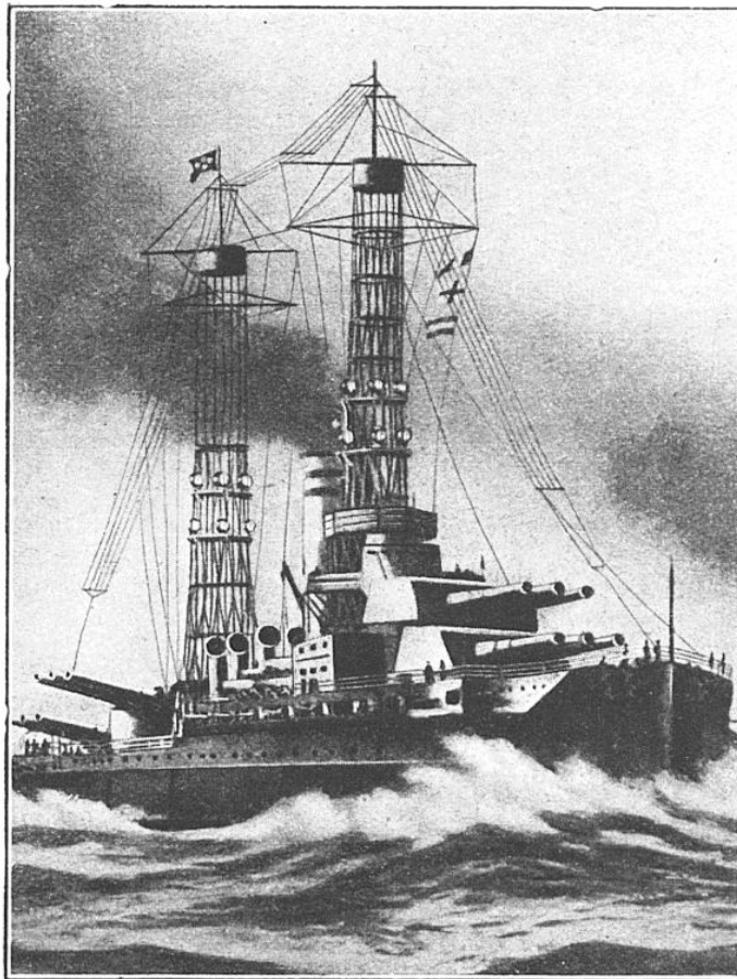
TOURELLES SUPERPOSÉES A TROIS CANONS CHACUNE, DU CUIRASSÉ AMÉRICAIN "PENNSYLVANIA"
