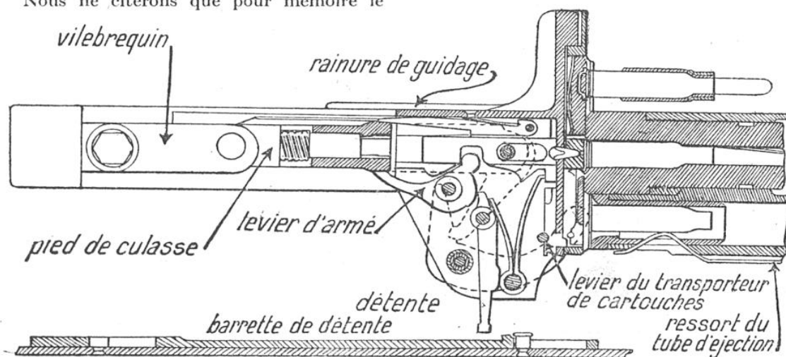
COUPE DU MÊME MÉCANISME, LA CULASSE ÉTANT RAPPROCHÉE DU CANON
