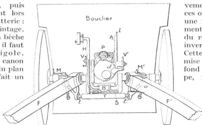
L'AFFÛT ET LE SYSTÈME DE POINTAGE DU CANON DEPORT. T, traverse d'essieu reliée par ses extrémités (t et t') aux deux demi-flèches F F' d'une part, et à l'essieu d'autre part, par deux secteurs à vis de pointage actionnés par les manivelles M et M'. En actionnant ces manivelles, on fait monter ou descendre la traverse d'essieu. — V V', manivelles de pointage; H, bras portant cette manivelle; A, secteur denté de hausse; P, frein de pièce; B', secteur de pointage avec vis sans fin S.
