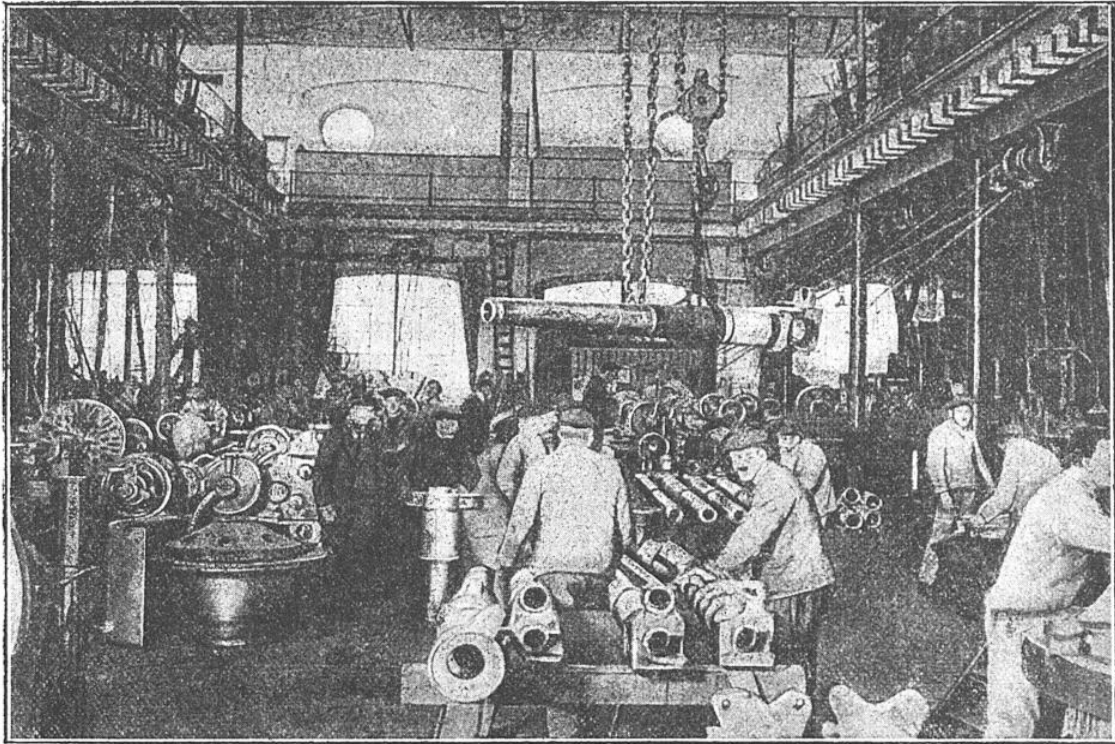
USINAGE DES CANONS DE CAMPAGNE DANS LES ATELIERS DE LA « RHEINISCHE METALLWA- REN UND MASCHINENFABRIK », A DUSSELDORF
