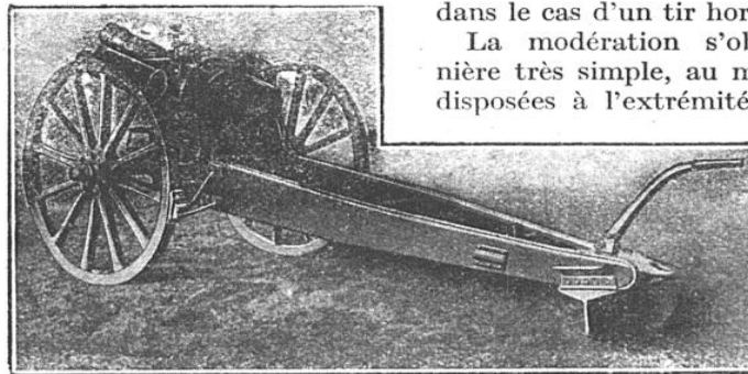
AFFÛT DE L'OBUSIER ANGLAIS VICKERS, DE 120 MM.
