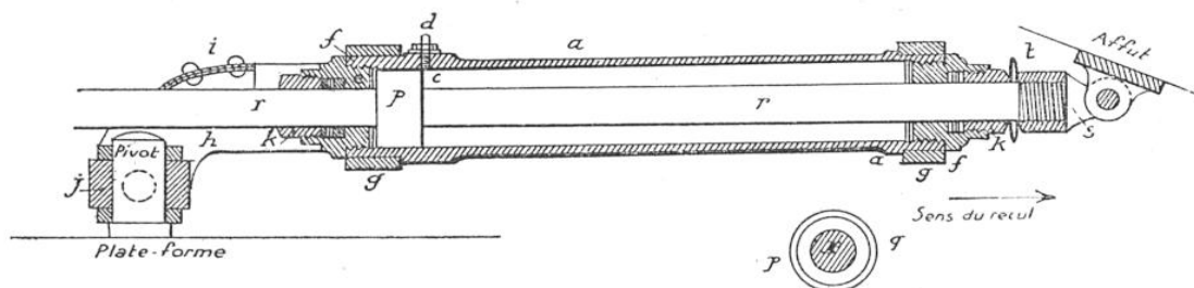
COUPE LONGITUDINALE DU FREIN HYDRAULIQUE DU CANON DE 155 MILLIMÈTRES
