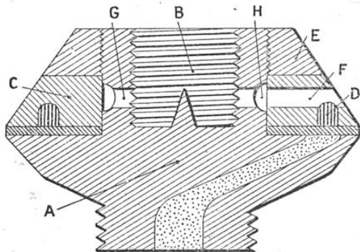
FUSÉE A CADRAN A UN ÉTAGE
