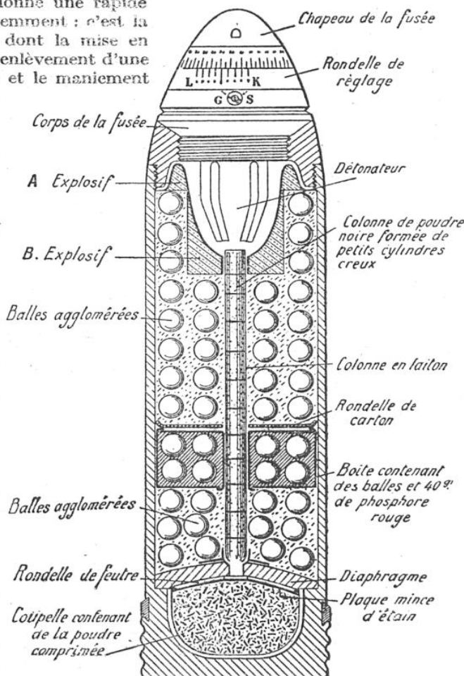
COUPE MONTRANT LE DISPOSITIF DE LA FUSÉE ET LES AGENCEMENTS INTÉRIEURS D'UN SHRAPNELL ALLEMAND
