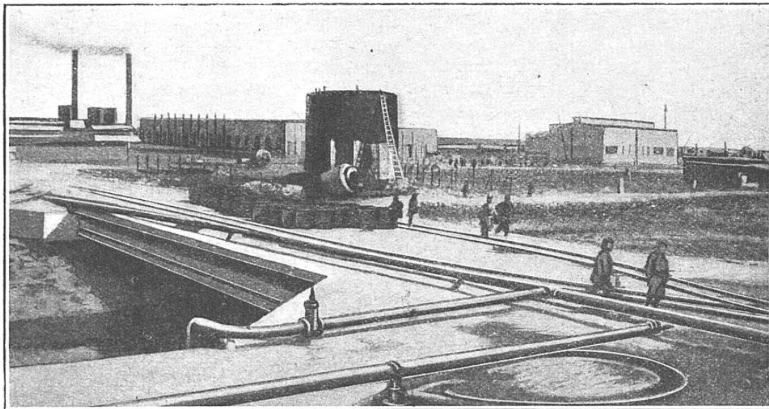
LA RAFFINERIE D'ABADAN. OU SONT TRAITÉS LES PÉTROLES DE L' "ANGLO-PERSIAN CO"
