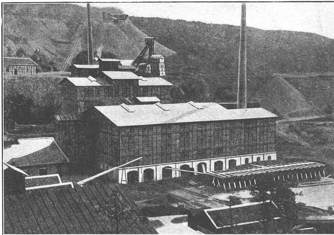
USINE DE TRAITEMENT DES MINERAIS DE PLOMB ET DE ZINC DE LA MINE BERZELIUS (PUISSANCE : 200 TONNES EN DIX HEURES), A BENSBERG (PRUSSE RHÉNANE)
