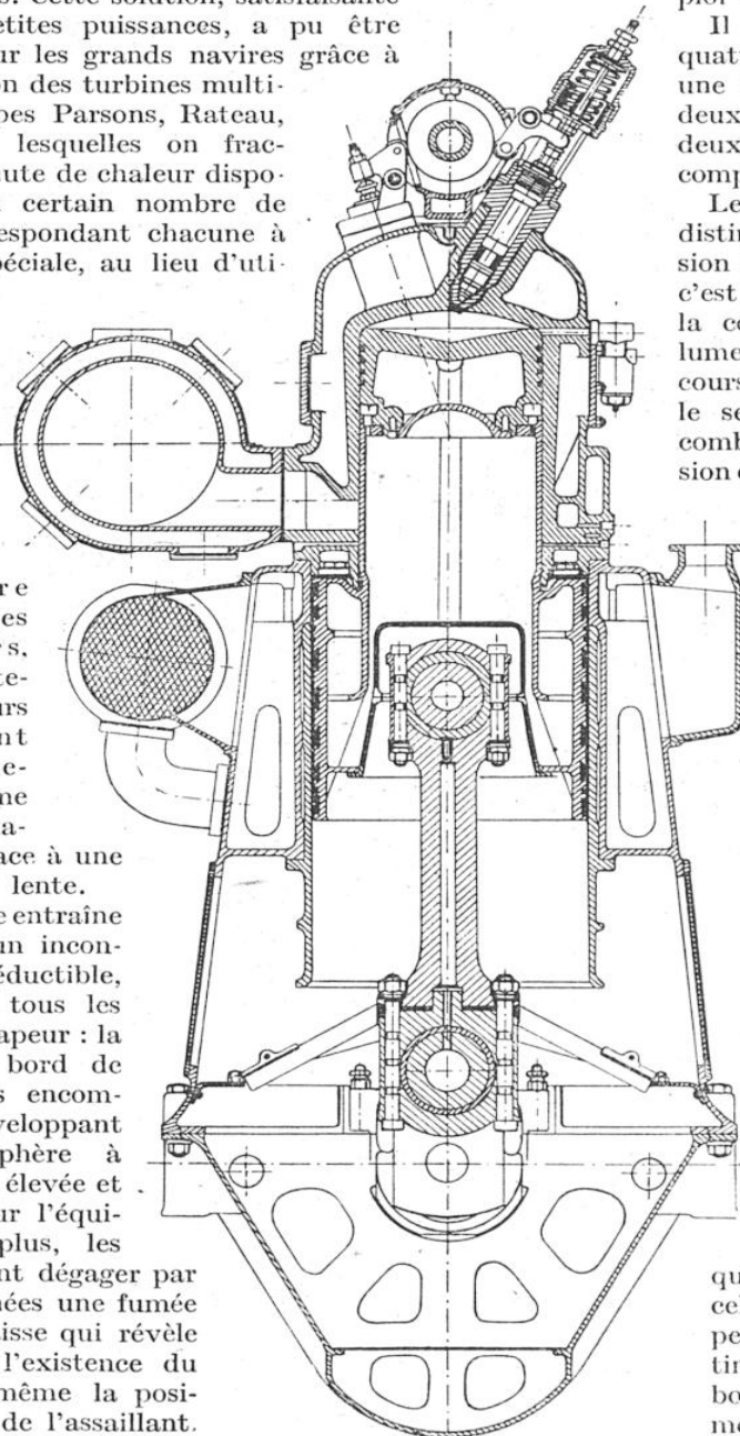
COUPE TRANSVERSALE D'UN CYLINDRE DE MOTEUR DIESEL
