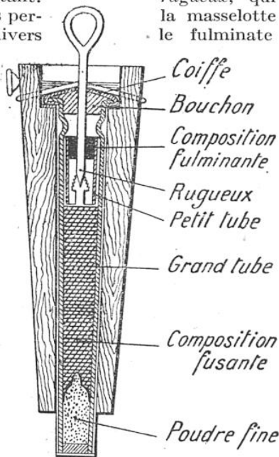
FUSÉE D'UNE GRENADE A MAIN
