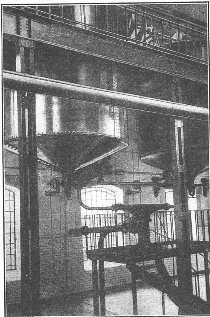
AGITATEUR CENTRIFUGE DANS LEQUEL ON LAVE LE BENZOL A L'ACIDE ET A LA SOUDE
