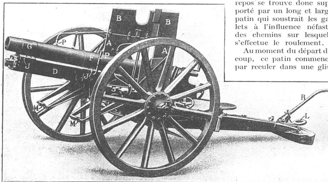
LE CANON DE CAMPAGNE ALLEMAND DE 77 MILLIMÈTRES, A TIR RAPIDE
