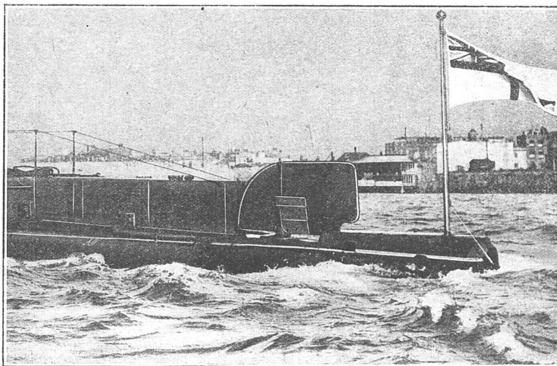
POUR SE DIRIGER SOUS L'EAU, LES SOUS-MARINS POSSÈDENT UN GOUVERNAIL SPÉCIAL, DU TYPE COMPENSÉ, MONTÉ À L'ARRIÈRE DU PONT; ON LE MANŒUVRE À BRAS
