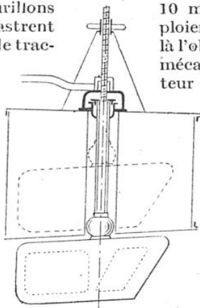
FIG. 5. — GOUVERNAIL AVANT DE TORPILLEUR
