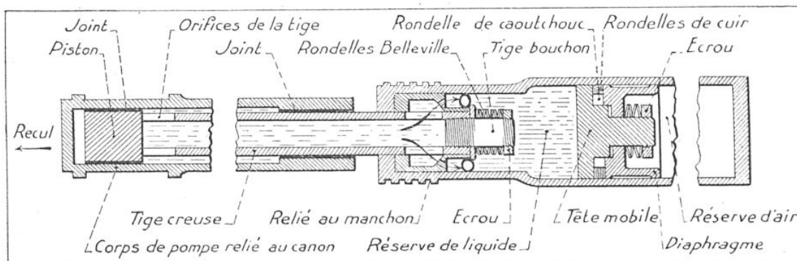
SCHÉMA DU FREIN HYDROPNEUMATIQUE EN USAGE DANS L'ARTILLERIE FRANÇAISE
