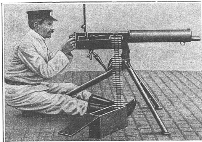
MITRAILLEUSE MAXIM MONTÉE SUR TRÉPIED À SELLETTE, EN POSITION POUR LE TIR HORIZONTAL
