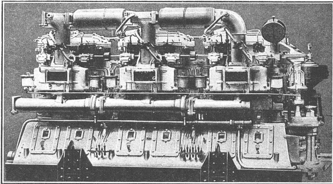
MOTEUR DE SOUS-MARIN ALLEMAND, A SIX CYLINDRES, SYSTÈME KERTING
