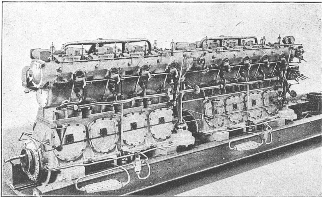
MOTEUR THORNYCROFT CONSTRUIT EN ANGLETERRE POUR LA MARINE ITALIENNE Ce groupe de 350 chevaux, composé de deux moteurs à quatre cylindres, a été fourni en 1908 pour les sous-marins "Otaria" et "Tricheco", de la flotte royale d'Italie
