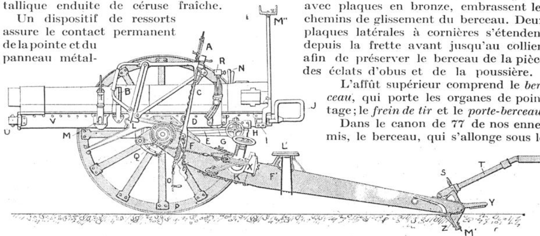
PROFIL ET DÉTAIL DES PIÈCES DU CANON DE CAMPAGNE ALLEMAND DE 77 MILLIMÈTRES
