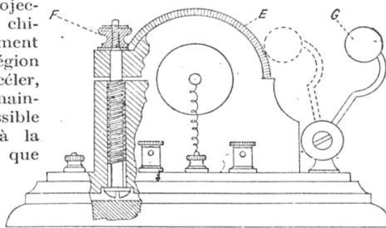
FIG. 10. — VUE EN BOUT DU GROUPE FIXE f, écrou de blocage; e, couronne molletée pour régler la bobine mobile; g, sphère métallique articulée.
