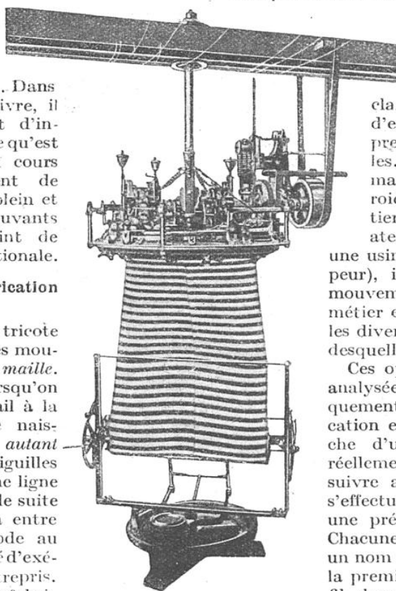
TYPE CLASSIQUE DU MÉTIER A BONNETERIE CIRCULAIRE FRANÇAIS
