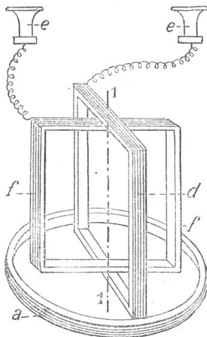
FIG. 8. — APPAREIL DE CHILOWSKY MODIFIÉ
