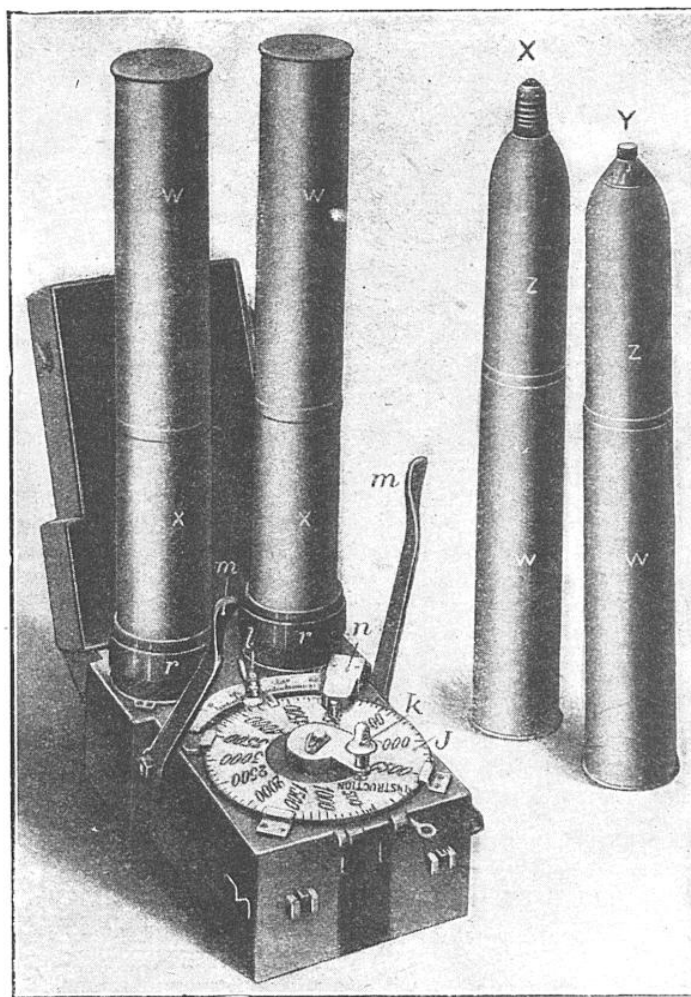
DÉBOUCHOIR DU CANON DE 75 EN POSITION DE DÉBOUCHAGE DE DEUX OBUS À BALLES
