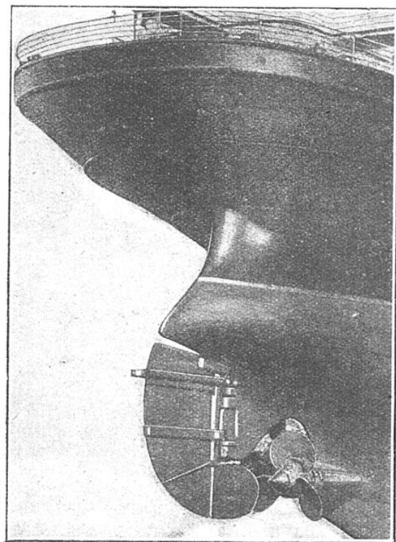
GOUVERNAIL DU PAQUEBOT "CARMANIA"
