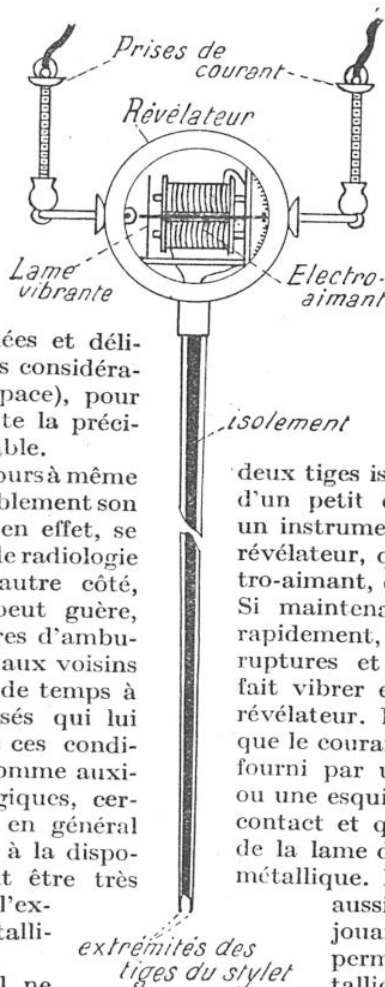
FIG. 1. - EXPLORATEUR ÉLECTRIQUE DE TROUVÉ
