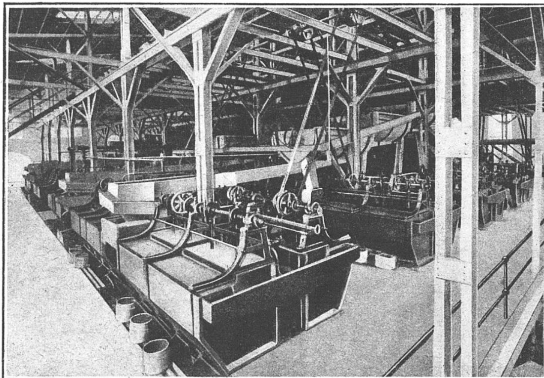
BACS A SECOUSSES SERVANT A LA CLASSIFICATION DES MINERAIS DE PLOMB ET DE ZINC, A LA MINE DIEPENLINCHEN, PRÈS STOLBERG (PRUSSE RHÉNANE)
