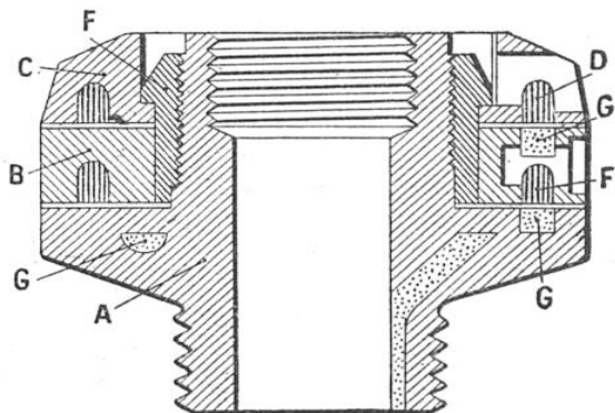
FUSÉE A CADRAN A DEUX ÉTAGES
