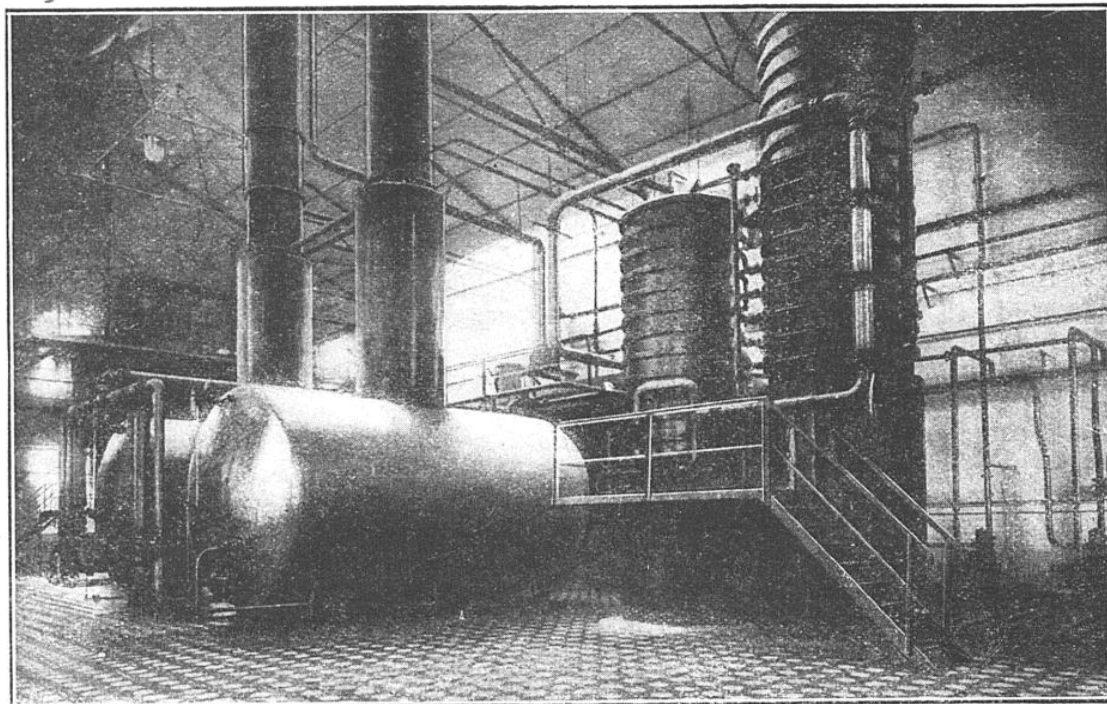
A DROITE : COLONNE DE DISTILLATION DES HUILES BENZOLÉES ; A GAUCHE : CHAUDIÈRES ET COLONNES DE RECTIFICATION DES BENZOLS BRUTS A 50 0/0
