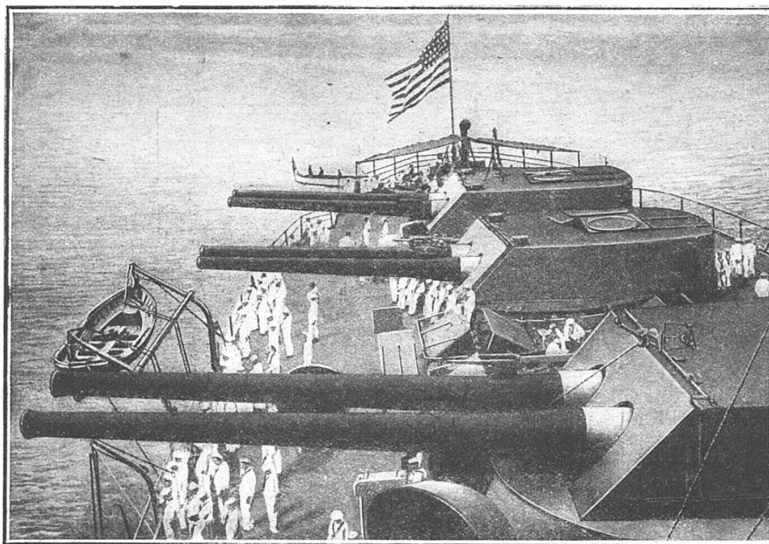
TROIS DES QUATRE TOURELLES ARRIÈRE DU CUIRASSÉ AMÉRICAIN " WYOMING "
