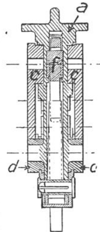
COUPE DU TRANSPORTEUR
