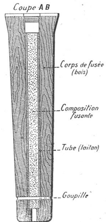
COUPE VERTICALE DE LA FUSÉE EN BOIS A TUBE EXTÉRIEUR EN MÉTAL
