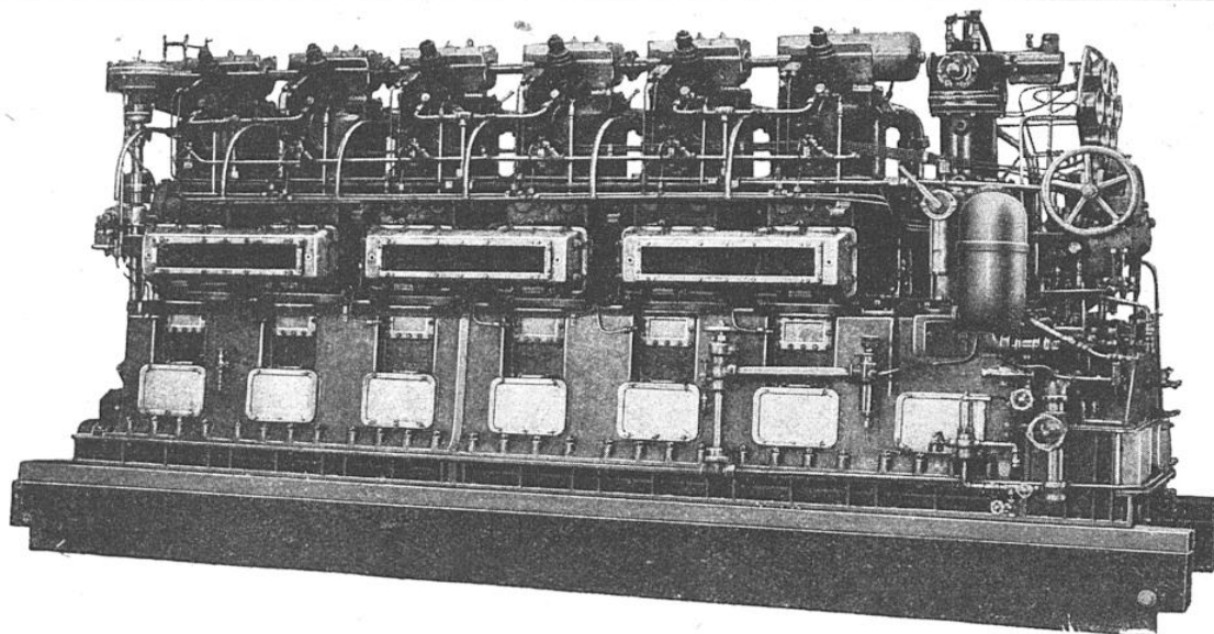
GRUPE MOTEUR DE LA SOCIÉTÉ "ELECTRIC BOAT CO"
