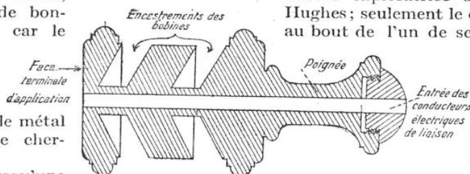
FIG. 11. - COUPE DU CHERCHEUR PROPREMENT DIT
