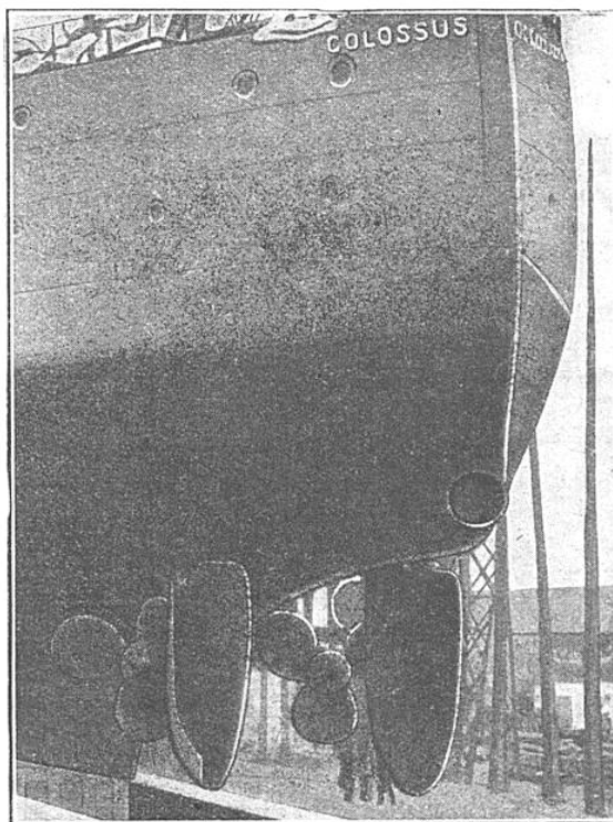
GOUVERNAILS JUMEAUX DISPOSÉS DERRIÈRE UNE HÉLICE POUR RENFORCER LA GIRATION
