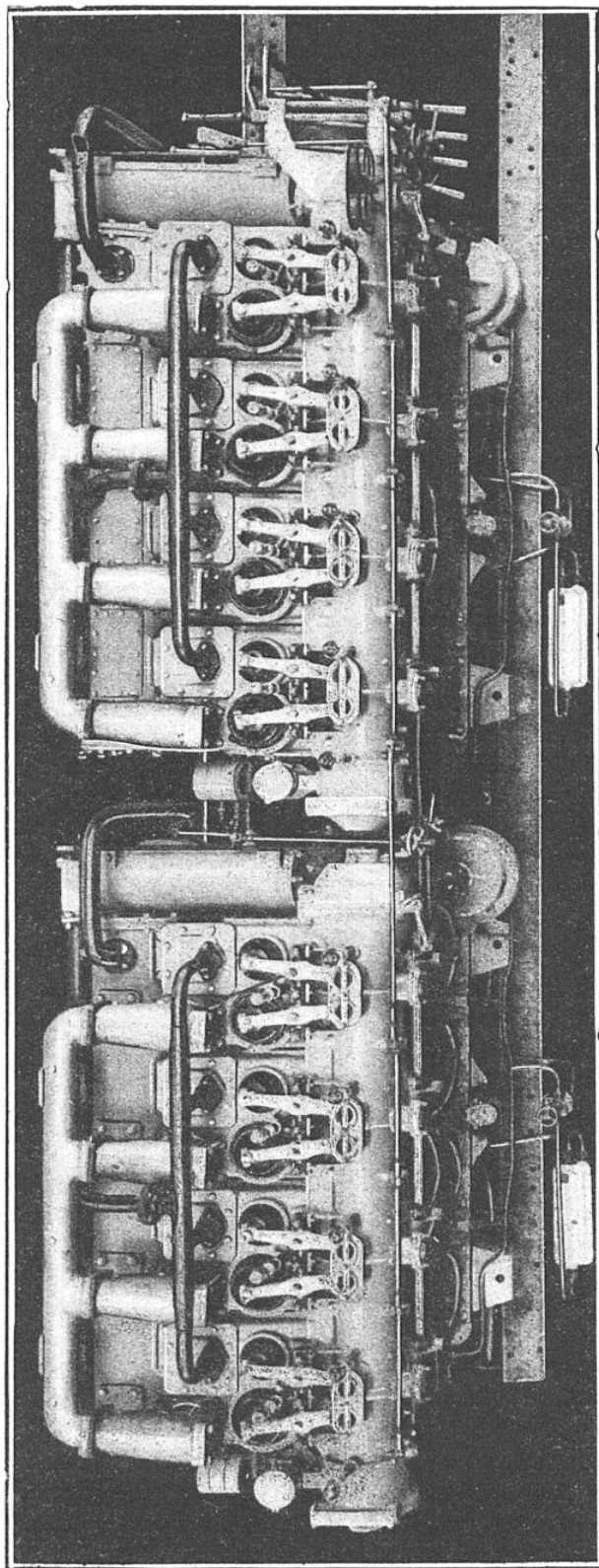
PARTIE SUPÉRIEURE, VUE EN PLAN, D'UN GROUPE MOTEUR THORNYCROFT, MONTRANT LA DISPOSITION DES SOUPAPES
