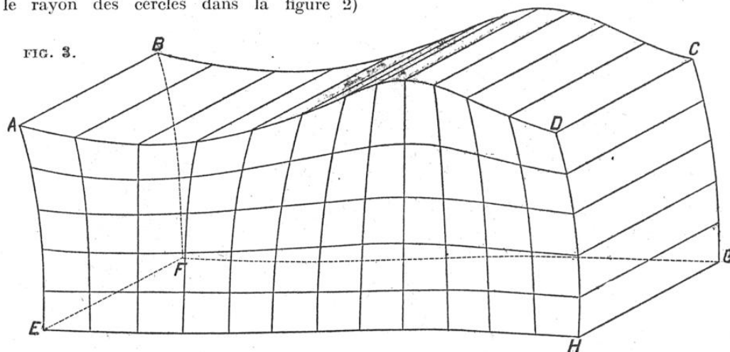
FORMES PRISES DURANT LA HOULE PAR LES SOIXANTE MASSES D'EAU ET LEURS SURFACES LIMITES
