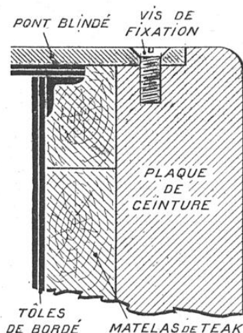
MODE DE POSE DU PONT BLINDÉ
