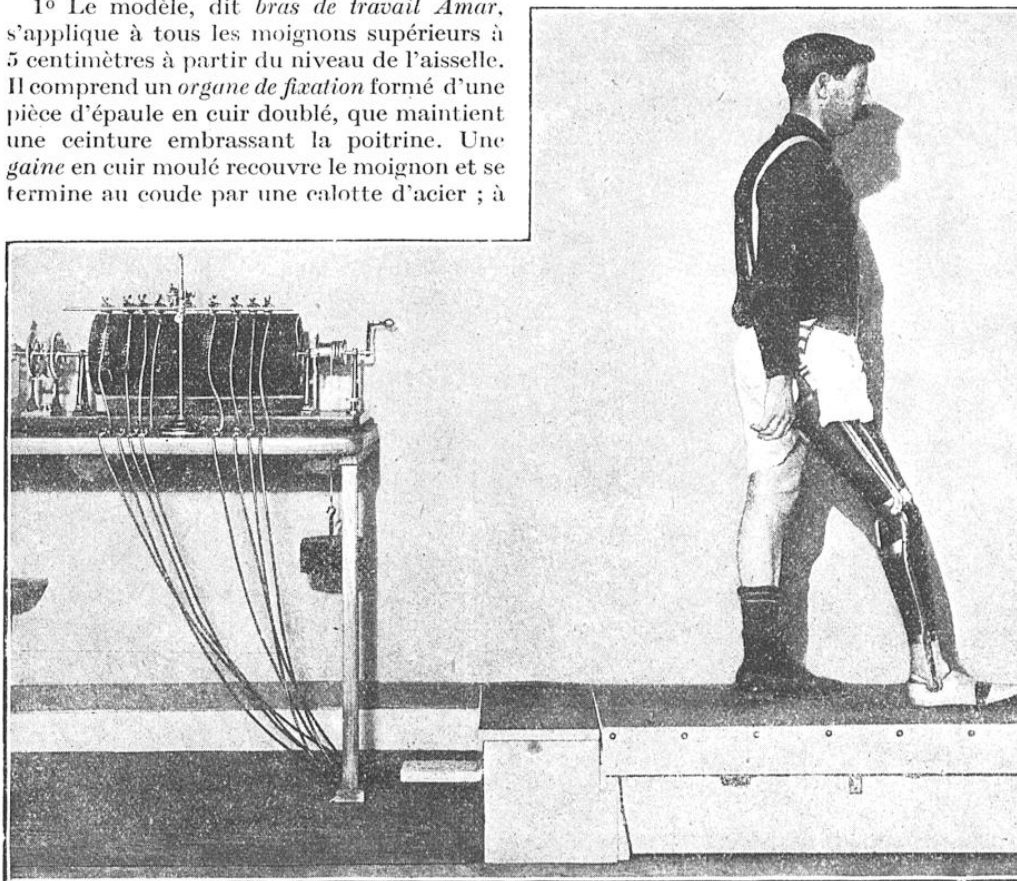
TROTTOIR DYNAMOGRAPHIQUE AMAR POUR L'EXPERTISE DES JAMBES ARTIFICIELLES
