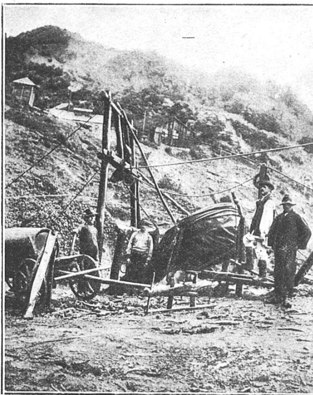
SOUFFLAGE D'UN PUIT ROUNAIN POUR PROVOQUER LA MONTÉE DU PÉTROLE
