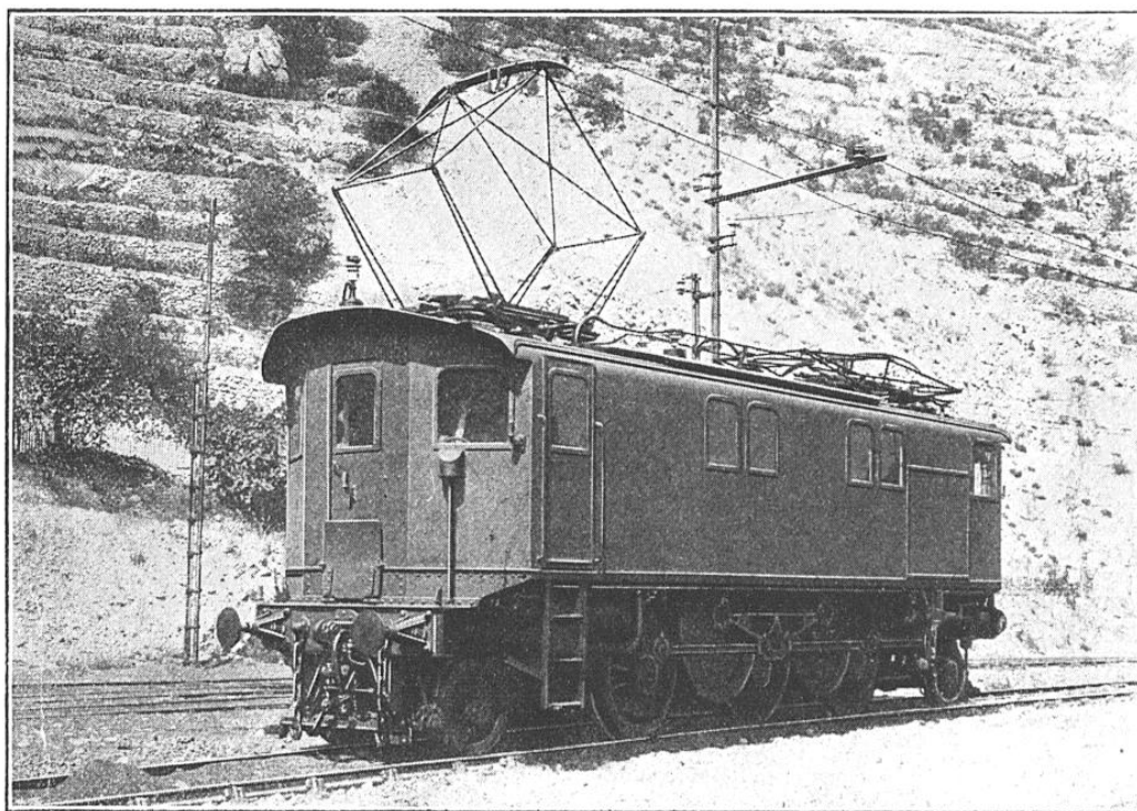
LOCOMOTIVE ÉLECTRIQUE DU SYSTÈME OERLIKON, DE LA LIGNE DE LÖTSCHBERG
