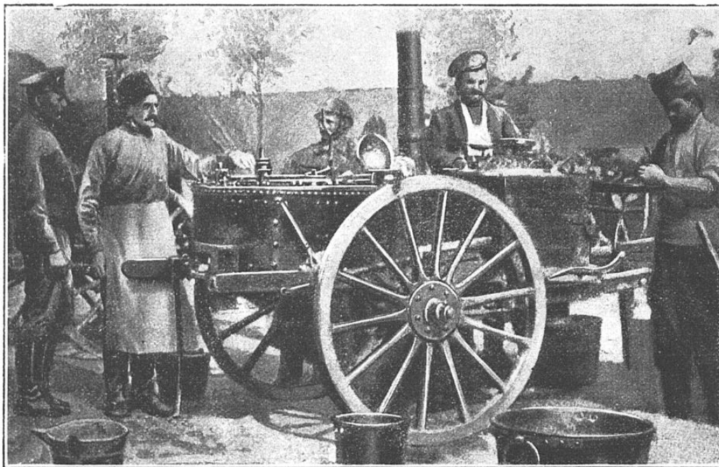
LE DERNIER TYPE DE CUISINE ROULANTE EN USAGE DANS L'ARMÉE RUSSE
