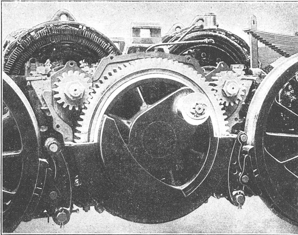
MOTEURS D'UNE LOCOMOTIVE AVEC PIGNONS ET ENGRENAGE ACTIONNANT UN FAUX ESSIEU
