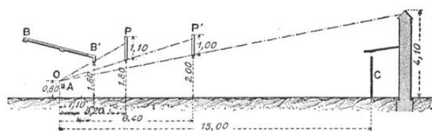
MODÈLE DE DISPOSITIF D'UN STAND DE TIR RÉDUIT ET ABRITÉ PAR UNE COUVERTURE BB'
