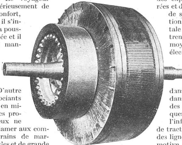
ROTOR D'UN MOTEUR DE 1250 CHEVAUX
