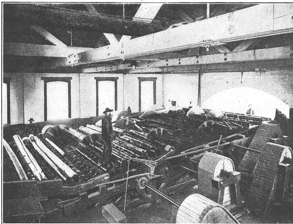
DÉBITAGE DES TRONCS EN BUCHES DANS UNE USINE CANADIENNE
