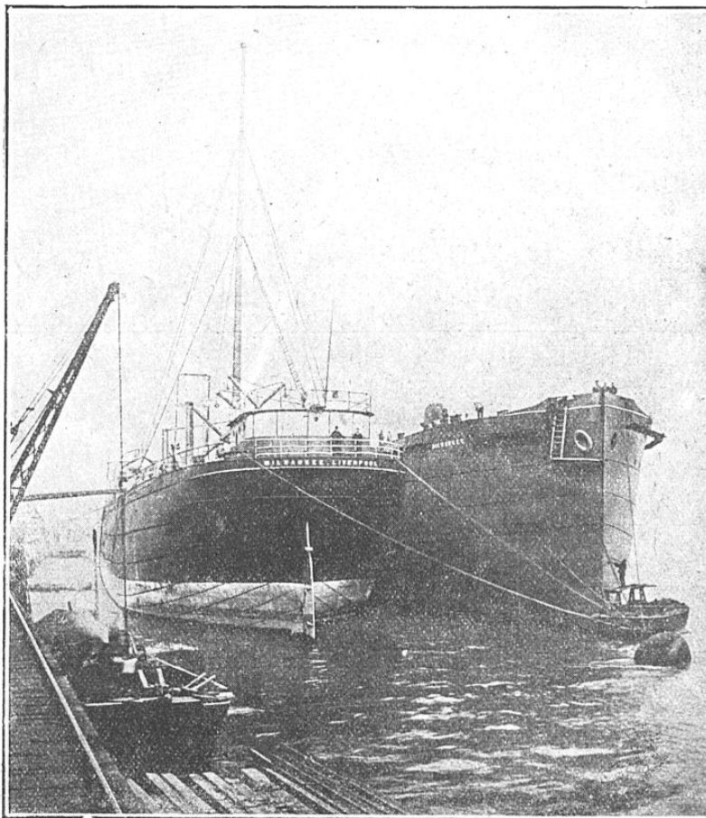
LES DEUX MOITIÉS DU « MILWAUKEE » RÉPARÉ AMARRÉES CÔTÉ À CÔTÉ
