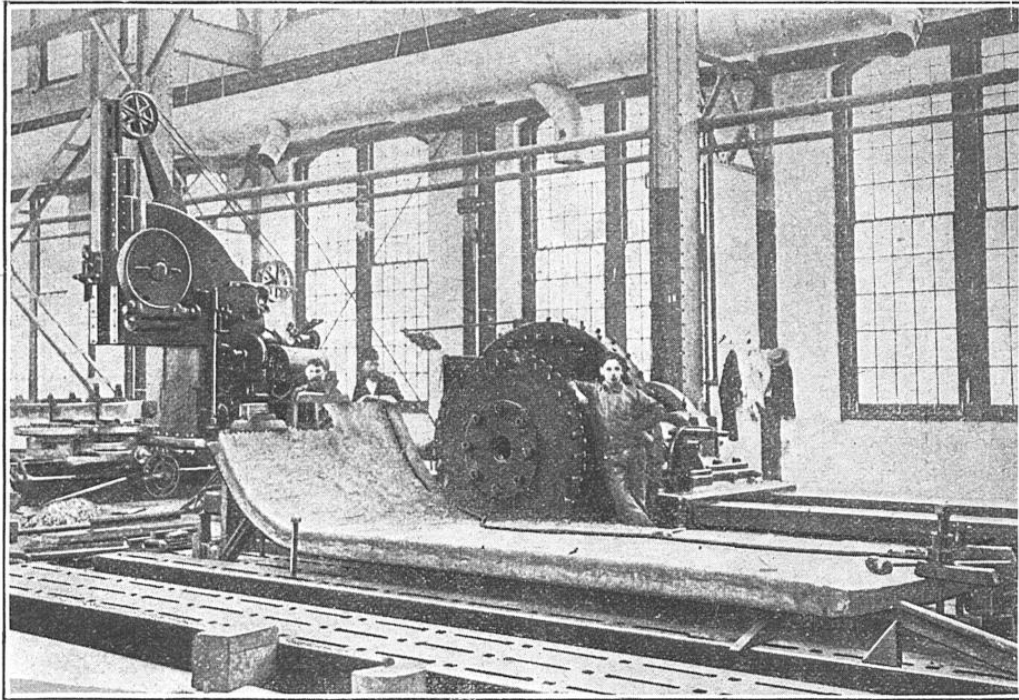
SCIE CIRCULAIRE SERVANT A TRAVAILLER LES PLAQUES DE BLINDAGE Cette photo représente le sciage d'un blindage de casemate ayant 180 millimètres d'épaisseur.
