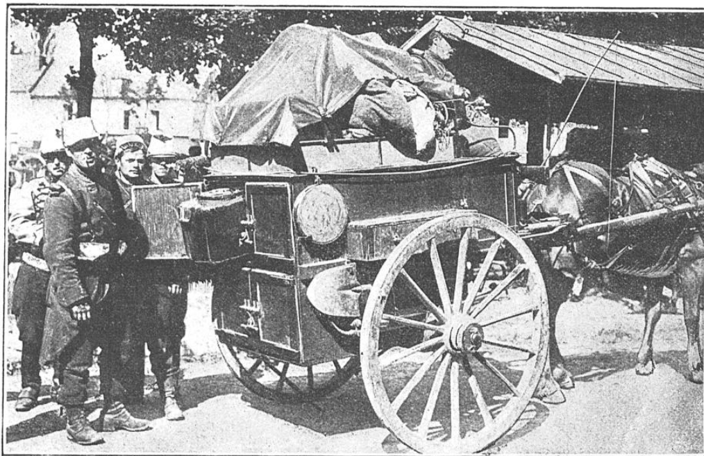
NOUVELLE CUISINE ROULANTE FRANÇAISE DU TYPE SANS FOYER
