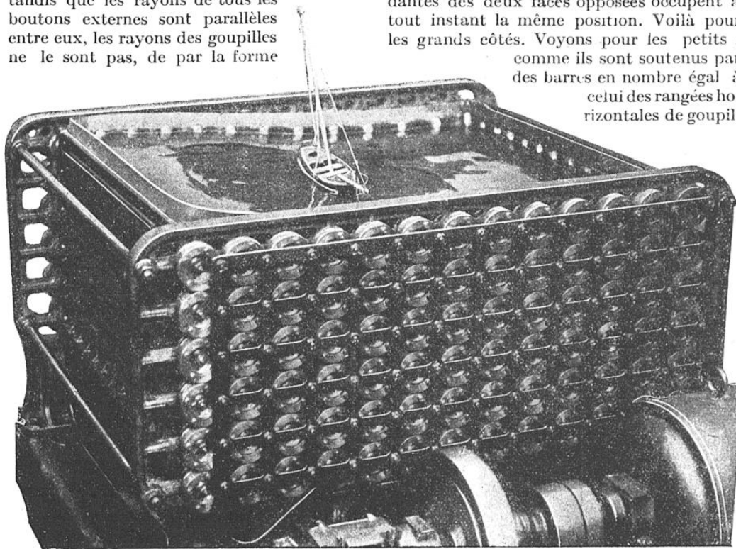
LE ROULIS SUR HOULE ARTIFICIELLE EXPÉRIMENTÉ AVEC UN PETIT MODÈLE DE NAVIRE
