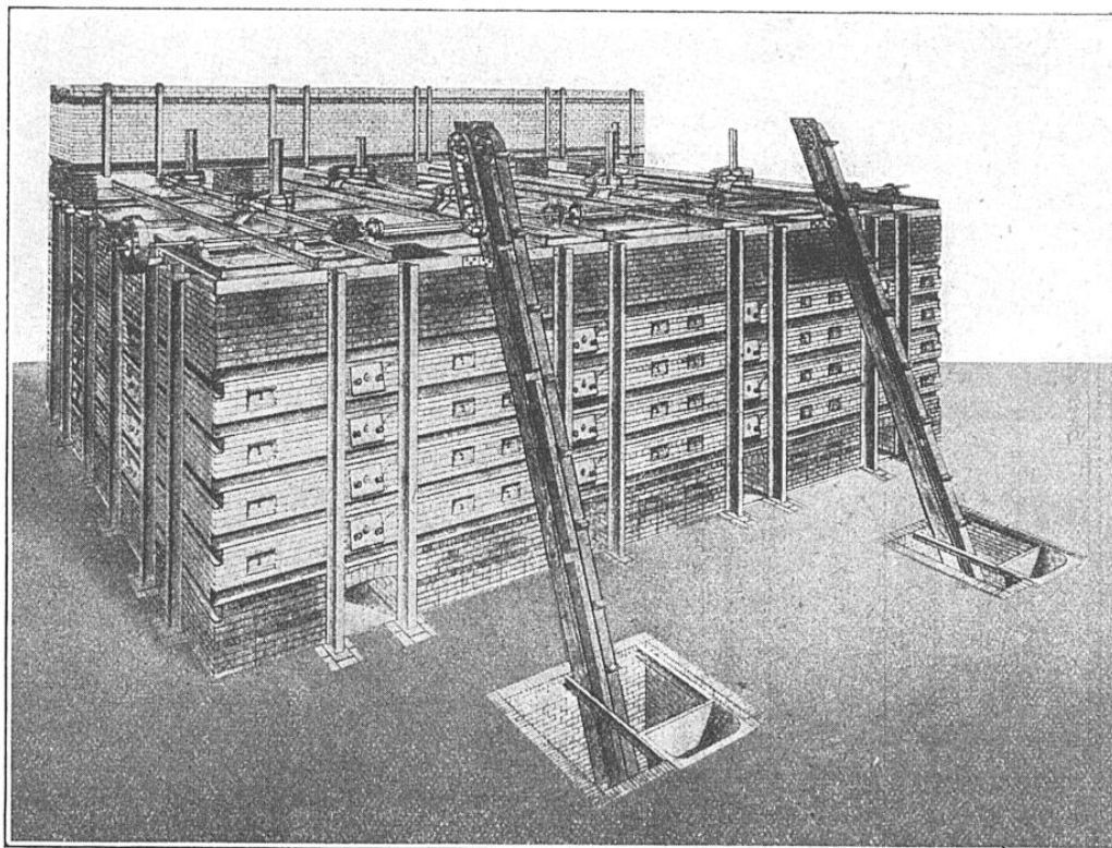
FOUR MALETRA POUR LA PRÉPARATION DE L'ACIDE SULFUREUX PAR LE GRILLAGE DES PYRITES
