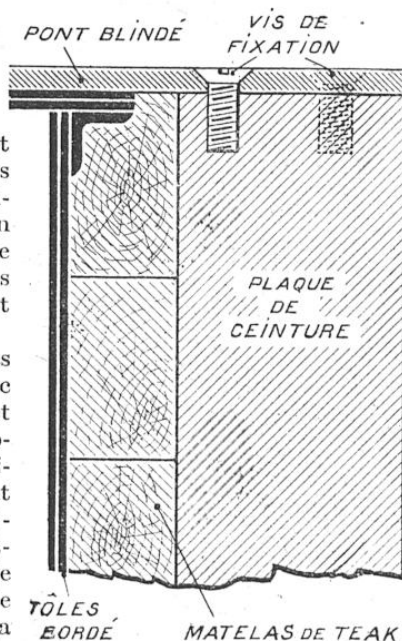
MODE DE FIXATION DÉFECTUEUX D'UN PONT BLINDÉ
