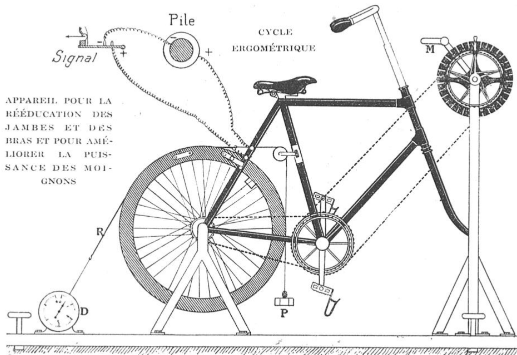
La roue arrière est un volant dans la gorge duquel frotte un ruban d'acier R. On règle la résistance ainsi offerte, et qui est indiquée par un dynamomètre D, en suspendant des poids appropriés au plateau P. La cadence des mouvements est donnée par un métronome sur lequel on règle le tic-tac du volant au passage de la fourche, tic-tac indiqué par un signal électrique. Le blessé, suivant le traitement prescrit, pédale ou tourne la manivelle M.
