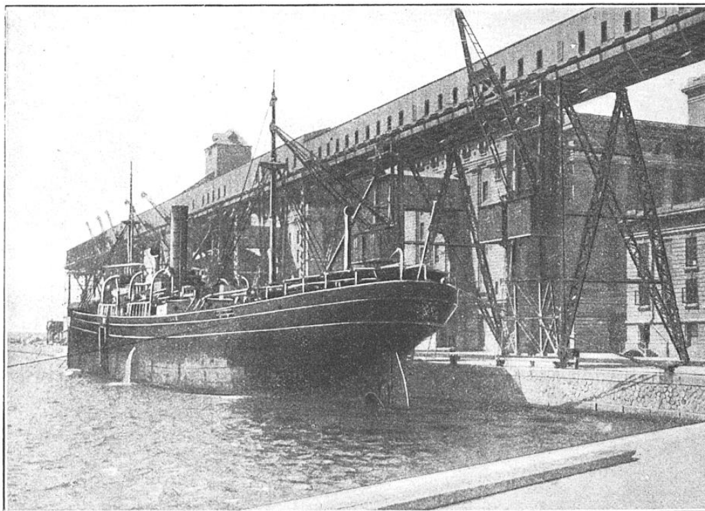
POSTE DE CHARGEMENT DES NAVIRES PÉTROLIERS, A CONSTANTZA
