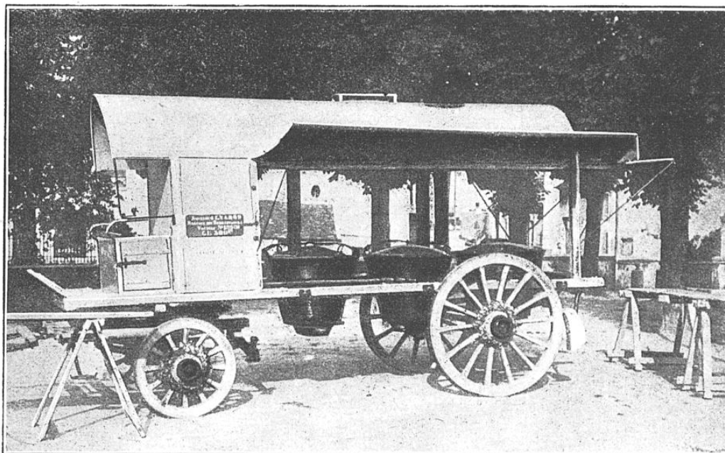
CUISINE A TROIS MARMITES DONT LE REMORQUAGE SE FAIT PAR AUTO
