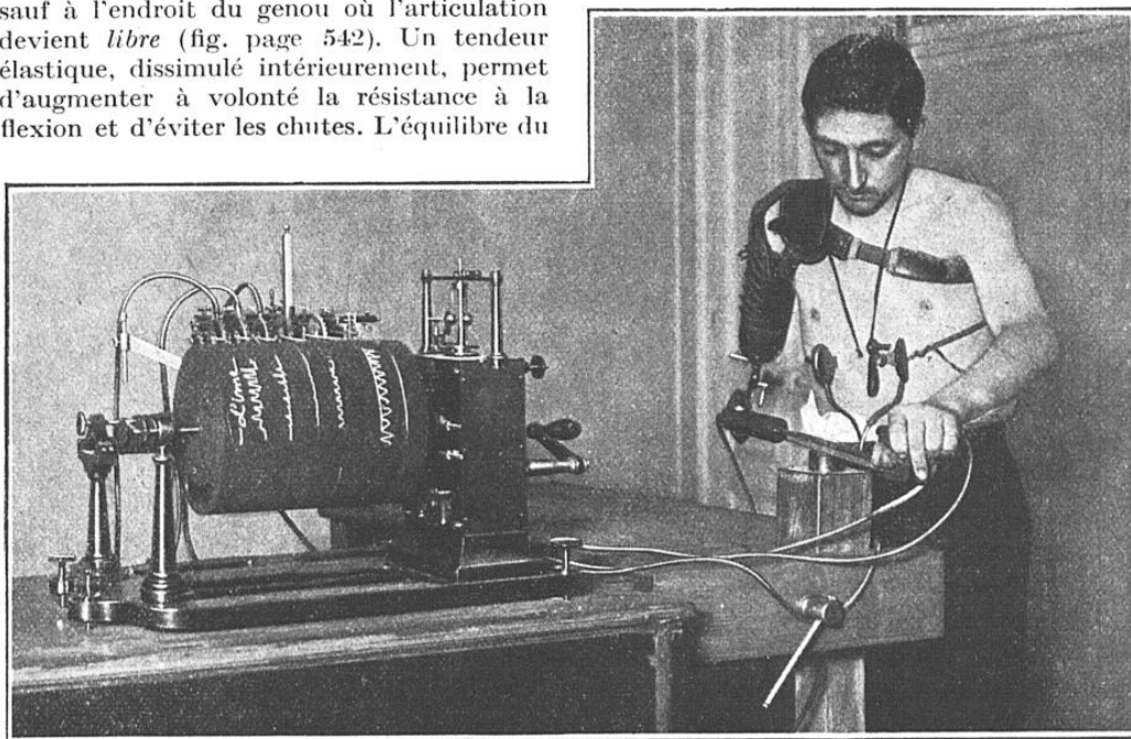
LA LIME DYNAMOMÉTRIQUE PERMET D'APPRÉCIER EN TOUTE SÛRETÉ LES QUALITÉS OU LES DÉFAUTS DU BRAS ARTIFICIEL DONT EST MUNI LE MUTILÉ ET LE DEGRÉ D'INCAPACITÉ DE TRAVAIL DE CE DERNIER
