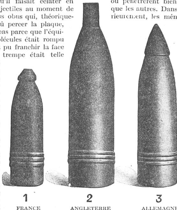
Trois types de projectiles à chapeau ou à coiffe dont le principe fut imaginé par l'amiral russe Makaroff.
