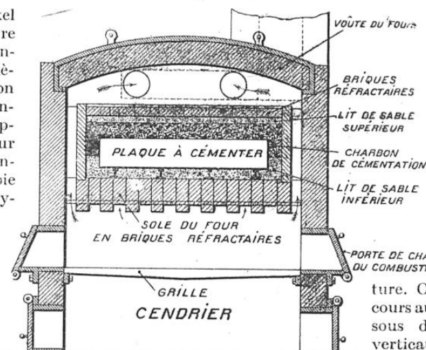
COUPE TRANSVERSALE D'UN FOUR A CÉMENTER
