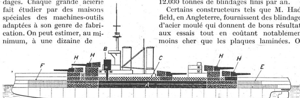
SCHEMA DU CUIRASSEMENT D'UN DREADNOUGHT ANGLAIS
