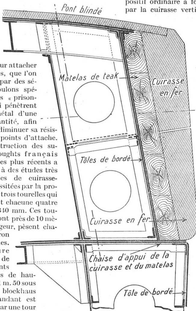
CUIRASSEMENT D'UN ANCIEN VAISSEAU
