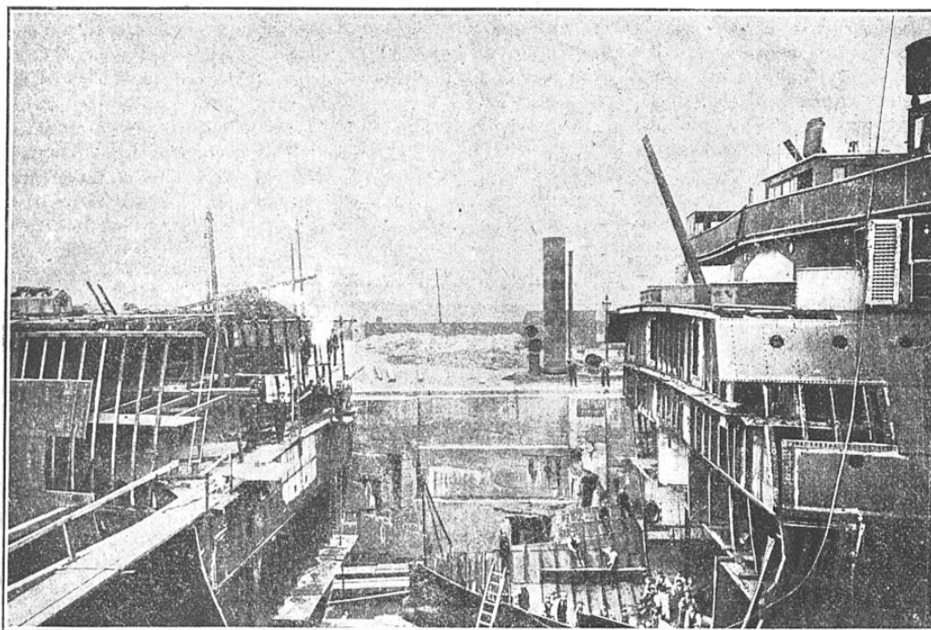
REMPLACEMENT DE L'AVANT DU BRISE-GLACES RUSSE « ERMAK »
