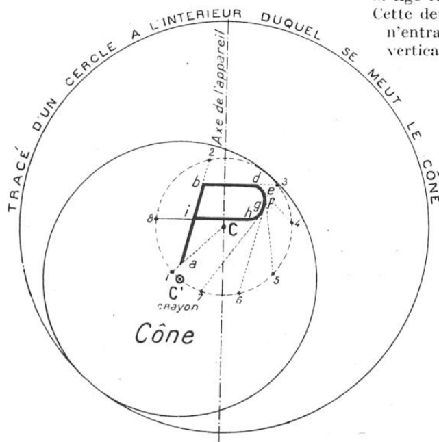
CROQUIS EXPLIQUANT LA MARCHE DU CRAYON
