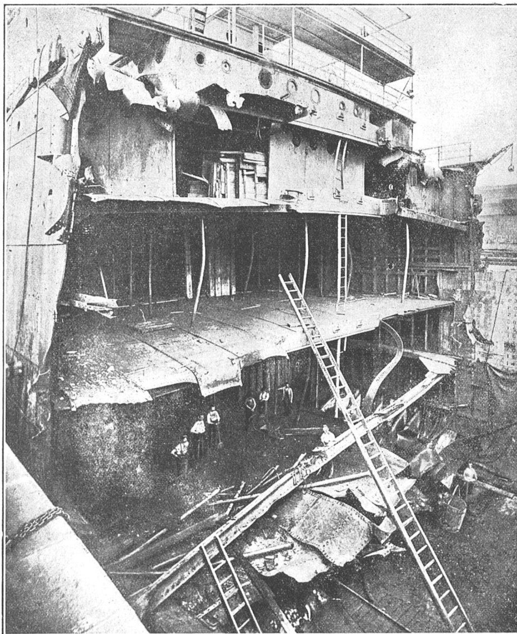
LE STEAMER « MILWAUKEE » DÉCOUPÉ À LA DYNAMITE APRÈS SON ÉCHOÛAGE
