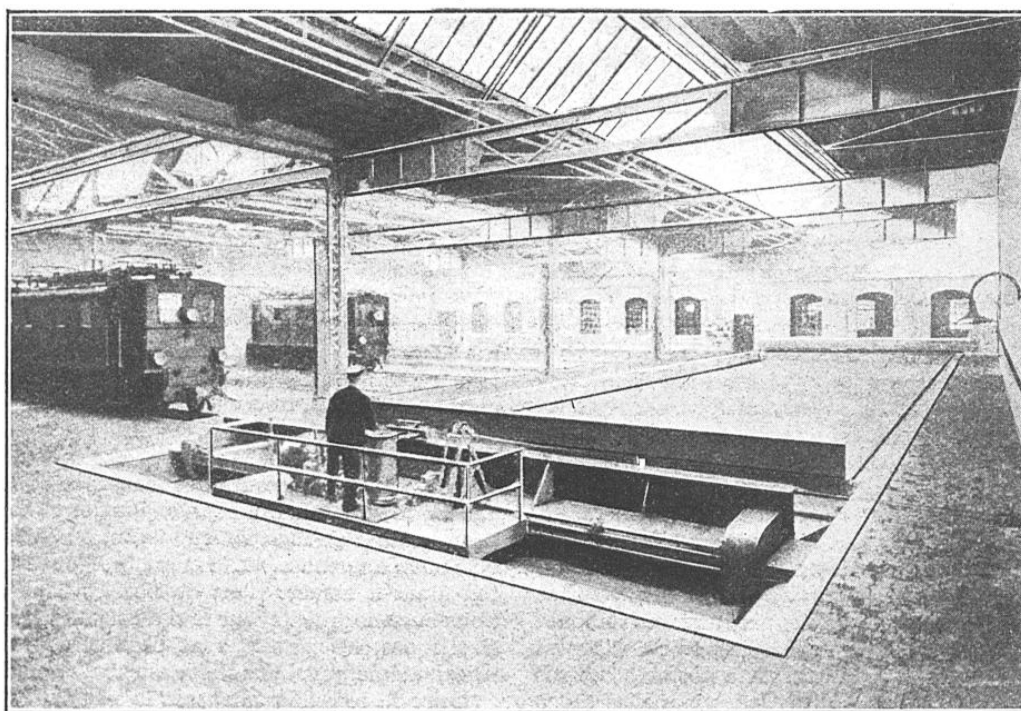
GRANDE REMISE, AVEC TRANSBORDEUR, POUR LOCOMOTIVES ÉLECTRIQUES.
