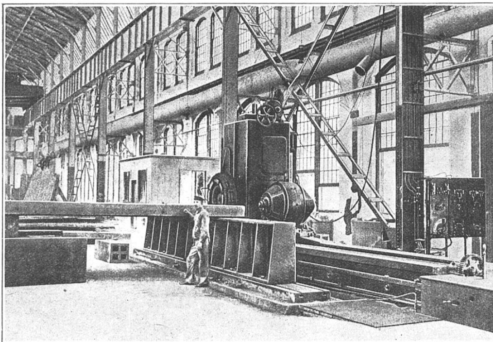
MACHINE A MEULER ACTIONNÉE PAR UNE COMMANDE ÉLECTRIQUE
