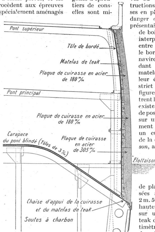
COUPE TRANSVERSALE D'UNE CUIRASSE D'ACIER
