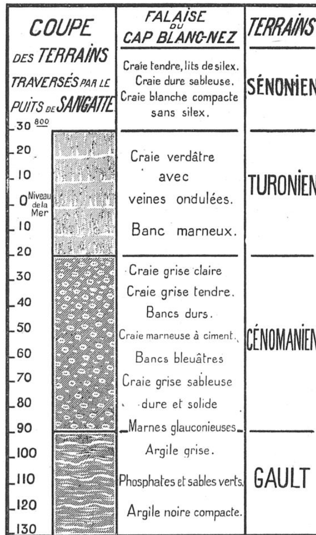
COUPE GÉOLOGIQUE A SANGATTE ET AU CAP BLANC-NEZ
