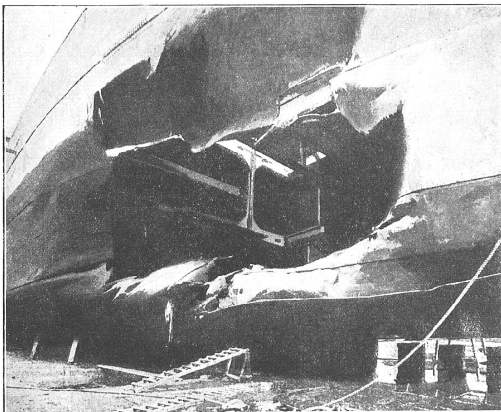
LE PÉTROLIER AMÉRICAIN « GULFLIGHT » MIS EN CALE SÈCHE À SOUTH SHIELDS, APRÈS SON TORPILLAGE, POUR ÊTRE RÉPARÉ
