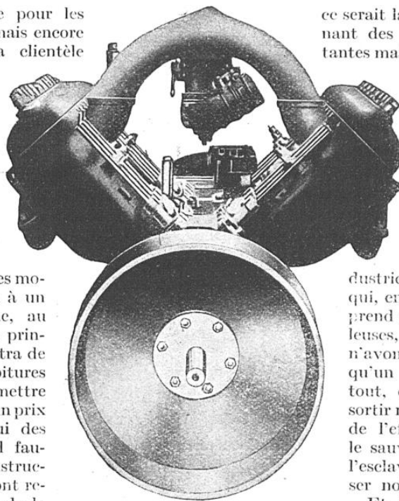
VUE ARRIÈRE D'UN MOTEUR EN V
