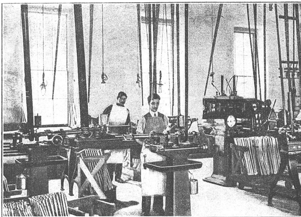
FILETAGE DE L'EXTRÉMITÉ D'UN CANON POUR LA FIXATION DU MAGASIN
