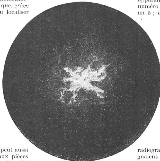
RÉVÉLATION DU MANQUE D'HOMOGENÉITÉ DANS UNE PLAQUE D'ACIER
