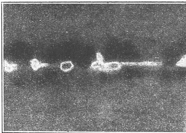
SOUDURE AUTOGENE DÉFECTUEUSE
