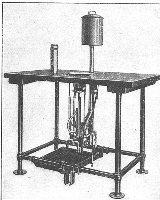
MACHINE A VERNIR INTÉRIEUREMENT LES PROJECTILES DE 75 A 150 MILLIMÈTRES
