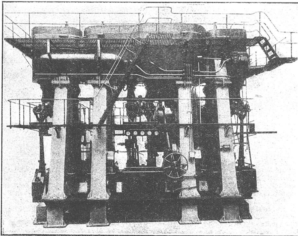
MACHINE MOTRICE A QUADRUPLE EXPANSION, POUR PAQUEBOT.
