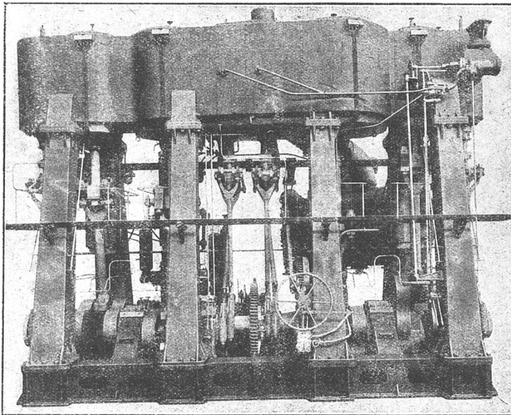
MOTEUR A QUADRUPLE EXPANSION, POUR CARGO-BOAT DE FORT TONNAGE
