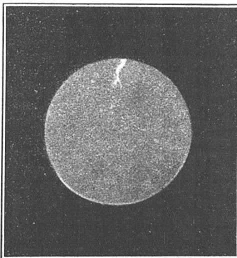
RADIOMÉTALLOGRAPHIE D'UNE RONDELLE DE CUIVRE ROUGE FISSURÉE
