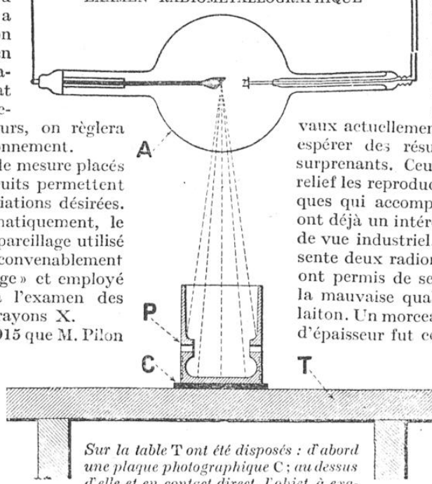
SCHEMA DE L'INSTALLATION GÉNÉRALE POUR UN EXAMEN RADIODÉTALLOGRAPHIQUE
