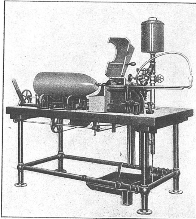
VERNISSAGE DE LA SURFACE EXTÉRIEURE D'UN OBUS
