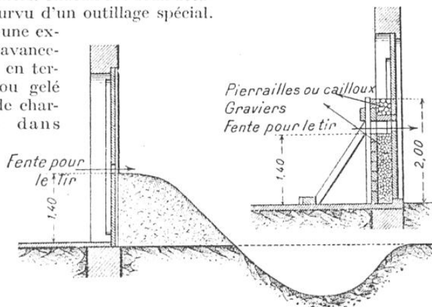
ORGANISATION DÉFENSIVE D'UNE PORTE, D'APRÈS LE MANUEL DES PIONNIERS ALLEMANDS ET AUTRICHIENS
