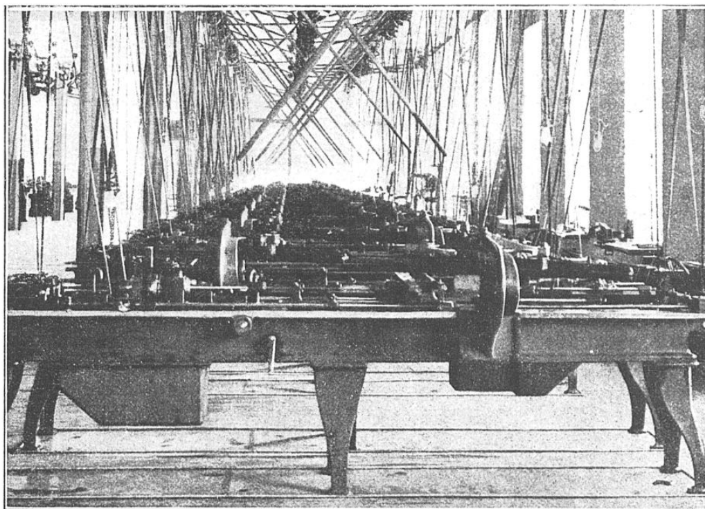
QUAND LES CANONS DE FUSILS ONT ÉTÉ FORÉS, CES MACHINES SERVENT À LES RAYER
