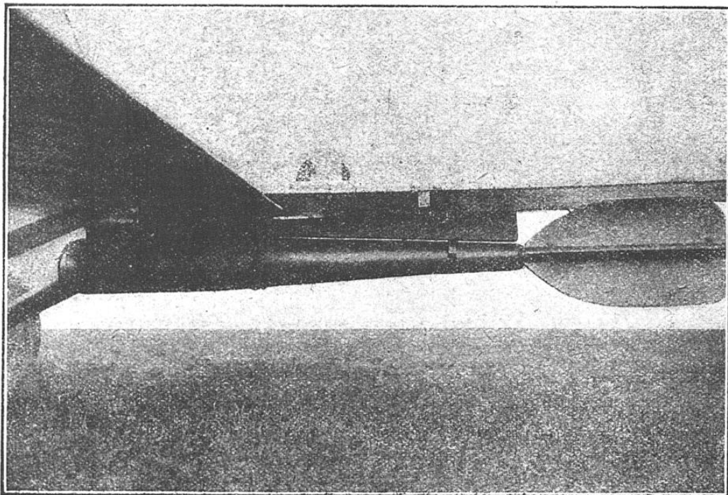
DÉTAIL DE LA FIXATION D'UNE AÉRO-TORPILLE SOUS UN AVION
