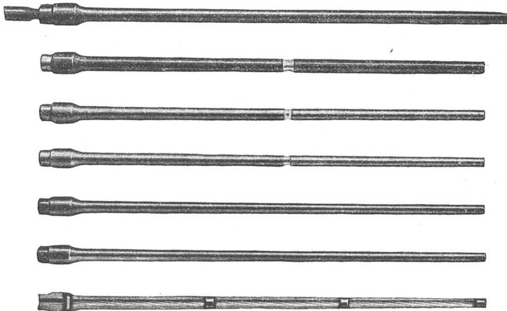
LES DIFFÉRENTS PHASES DE LA FABRICATION D'UN CANON DE FUSIL, PERMETTANT D'OBTENIR UN FORAGE ABSOLUMENT RÉGULIER
