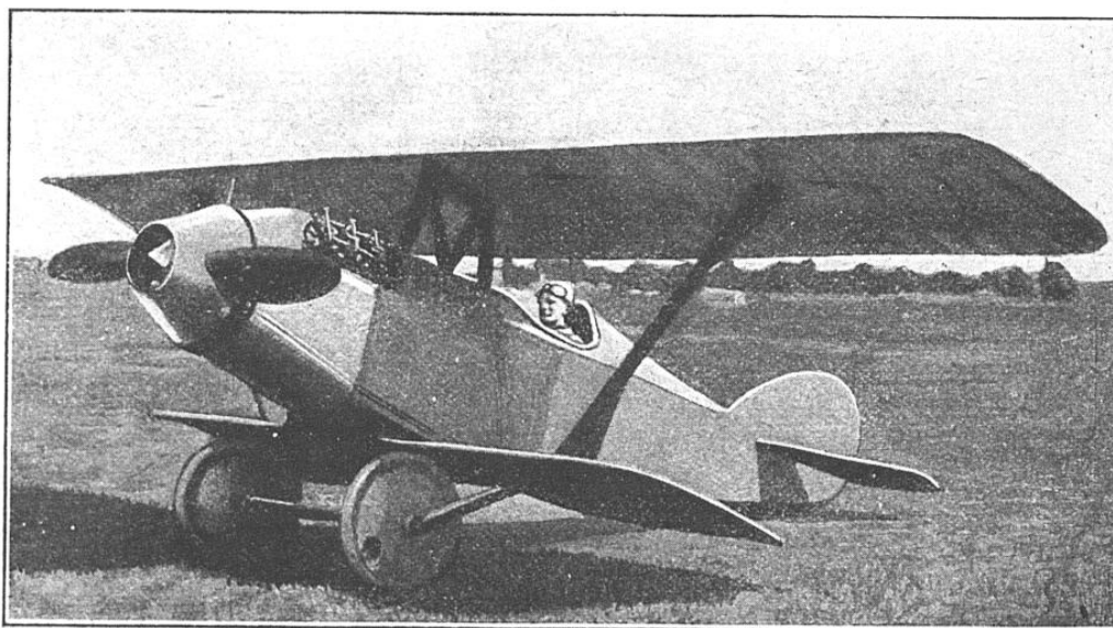
LES PLANS DU NOUVEL AÉROPLANE CURTISS NE SONT ENTRETOISÉS QUE PAR DEUX MONTANTS
