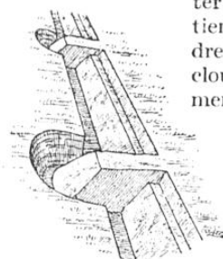
TRANCHÉE AVEC TRAVERSES POUR ÉVITER LES TIRS D'INFILADE
