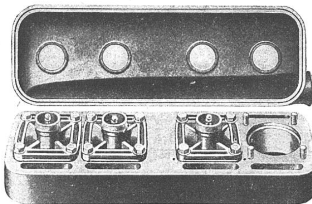
DANS CERTAINS MOTEURS AMÉRICAINS, LE HAUT DU CYLINDRE — LA CALOTTE — SE DÉMONTÉ POUR PERMETTRE L'ACCÈS AUX DIFFÉRENTES PARTIES DU MÉCANISME
