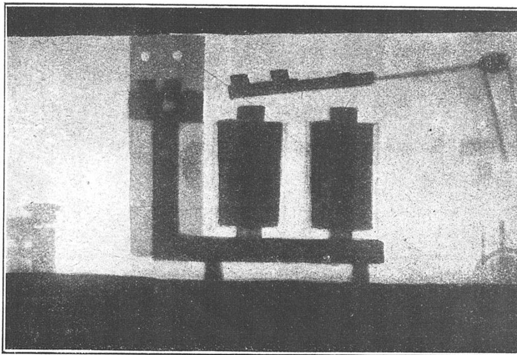
RELAÏ ÉLECTRIQUE RADIOGRAPHIÉ A TRAVERS 28 MILLIMÈTRES D'ACIER
