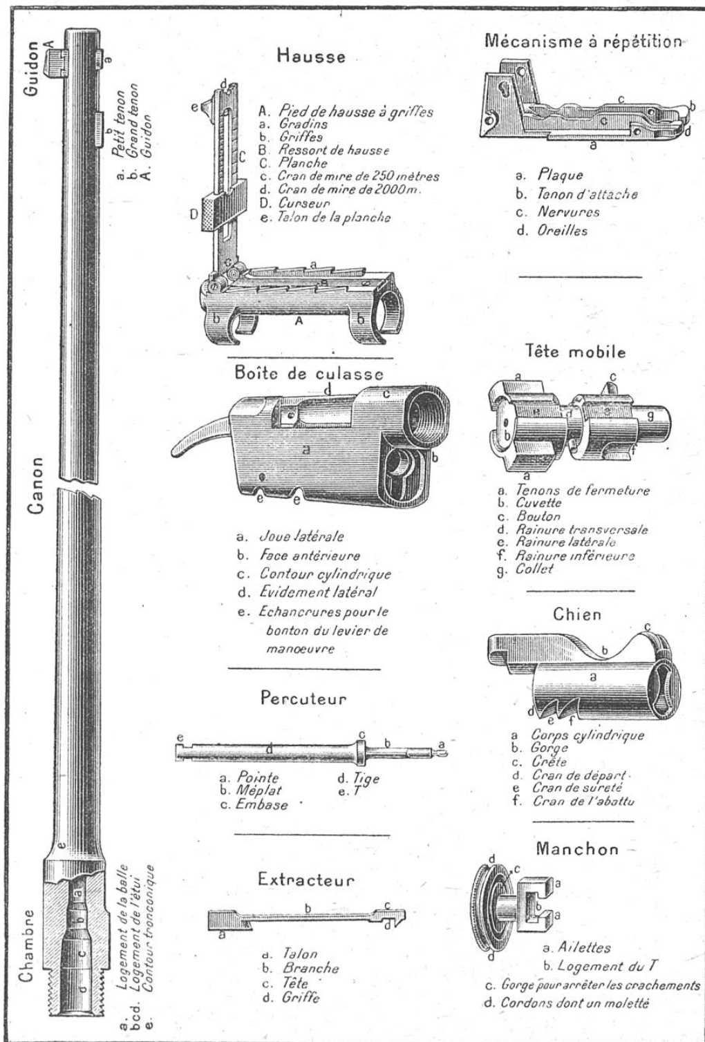
SÉRIE DE PIÈCES ENTRANT DANS LA CONSTRUCTION DU FUSIL LEBEL
