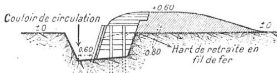
VUE LATÉRALE D'UNE TRAVERSE DE TRANCHÉE
