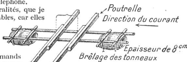
RADEAU DE TONNEAUX EMPLOYÉ COMME CORPS DE SUPPORT POUR LES PONTS DE FORTUNE
