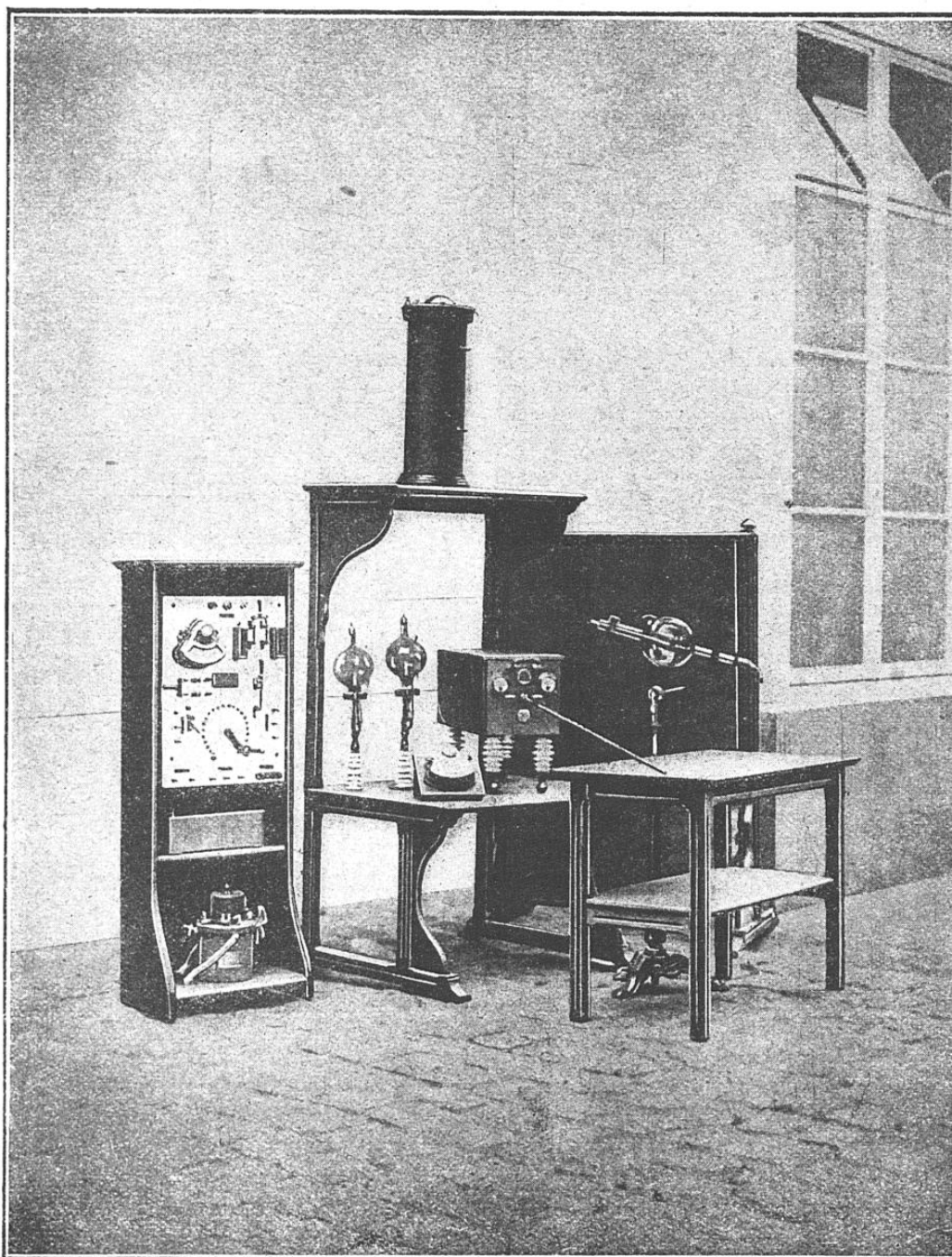
Au-dessus de la table, au premier plan : le tube « Coolidge » ; sur la tablette inférieure de la crédence : la boîte contenant la batterie d'accumulateurs, les appareils de mesure et de réglage et le milliampère-mètre ; sur la tablette supérieure : le transformateur. A gauche : le tableau de réglage et ses commandes. A droite : paravent de plomb destiné à protéger l'opérateur.
