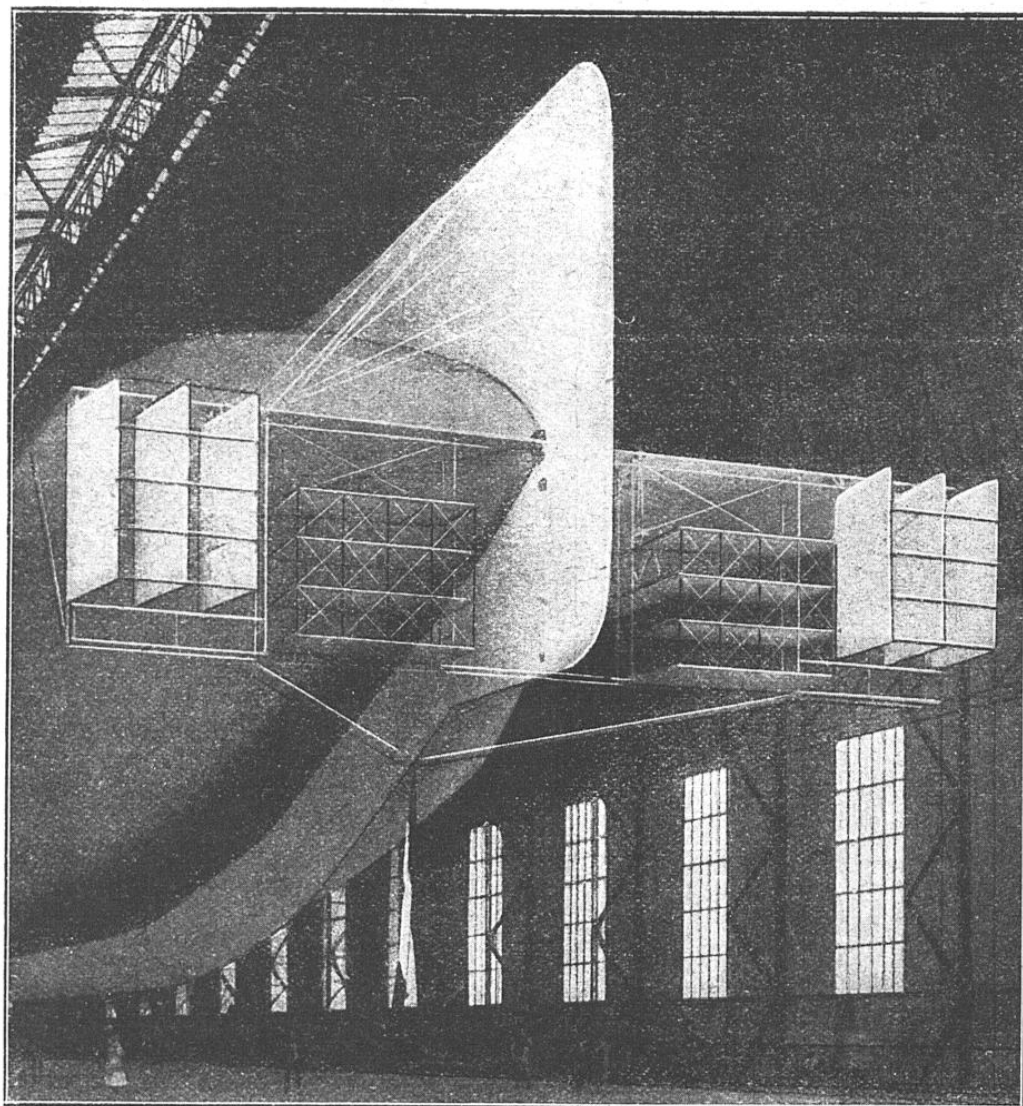
DISPOSITIF COMPLET DE L'EMPENNAGE D'UN ZEPPELIN DE GUERRE
