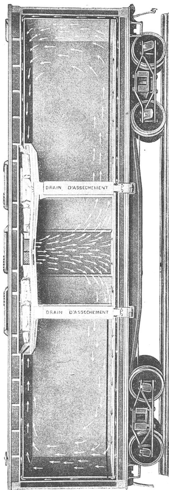
COUPE D'UN WAGON FRIGORIFIQUE AMÉRICAIN MONTRANT LA RÉPARTITION DU COURANT D'AIR A L'INTÉRIEUR DE LA CAISSE
