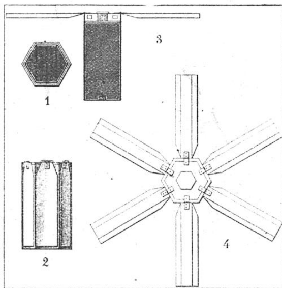
NOUVEAU MODÈLE D'« ÉTOILE » A PARACHUTE D'UN OBUS ÉCLAIRANT KRUPP
