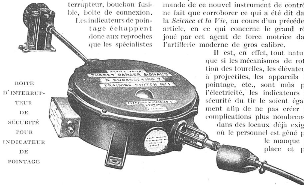
Le schéma inférieur de la page 63 représente le montage de cet appareil sous le pont d'un navire et dans sa véritable position, à l'inverse de celui-ci, qui a été retourné pour plus de clarté dans le dessin.
