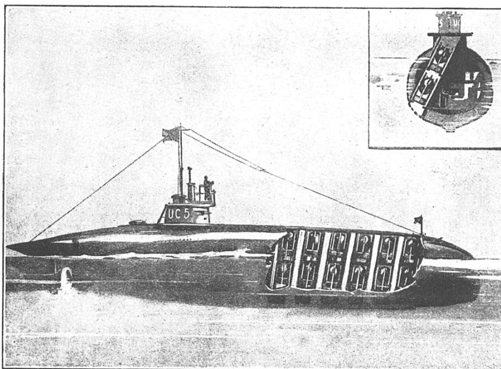
ILLUSTRATION DE LA MANIÈRE DONT LES SOUS-MARINS ENNEMIS PORTENT LEURS MINES
