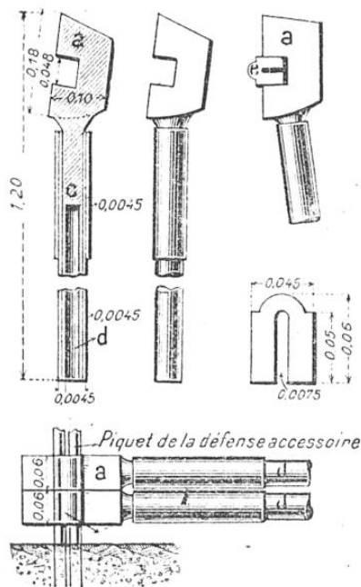
DOUBLE GRIFFE EN ACIER POUR ARRACHER LES PIQUETS MÉTALLIQUES DES RÉSEAUX DE FILS DE FER DE FORTERESSE
