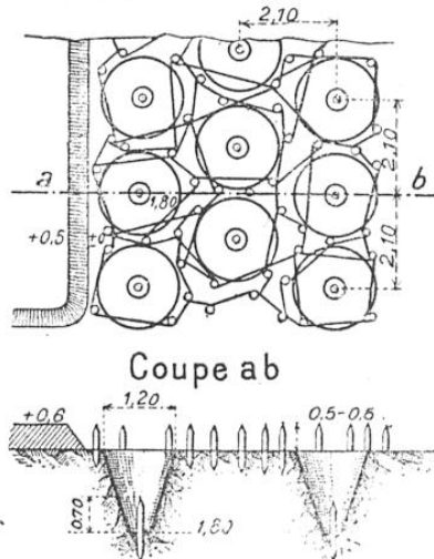
TROUS-DE-LOUP EN AVANT D'UN OUVRAGE DE CAMPAGNE
