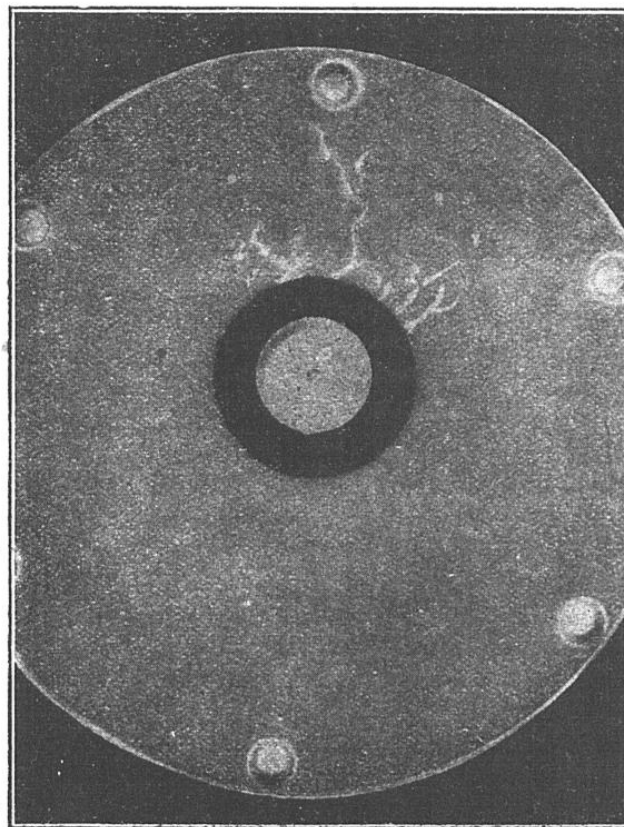
SOUFFLURES DANS UNE PIÈCE DE BRONZE USINÉE
