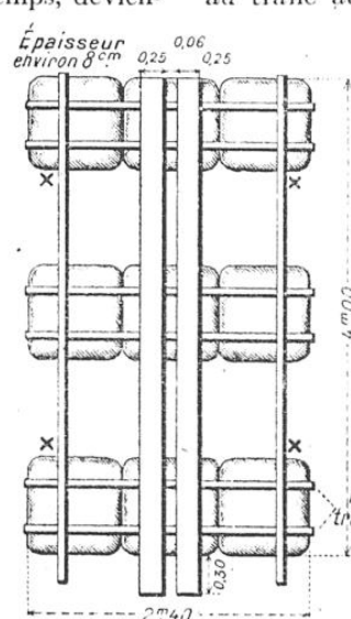
ÉLÉMENT DE PONT RAPIDE DE L'ARMÉE ALLEMANDE
