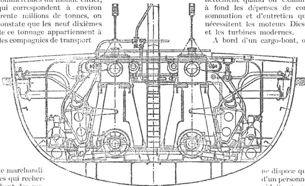
COUPE DE LA CHAMBRE DES MACHINES D'UN PAQUEBOT
