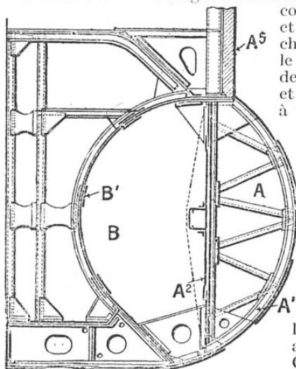
COUPE D'UN CAISSON PROTECTEUR, MONTRANT LA CHAMBRE AVANT ET LA CHAMBRE ARRIÈRE
