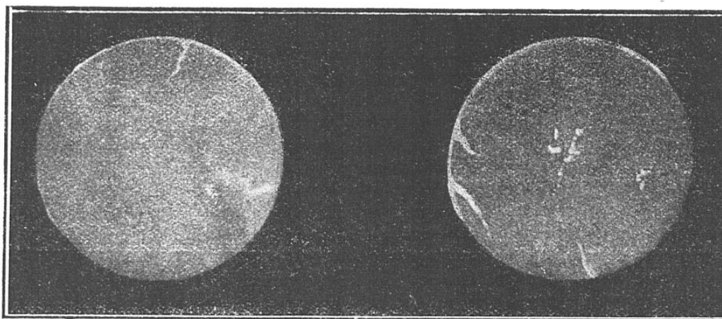
ÉPREUVES RADIOMÉTALLOGRAPHIQUES DE RONDELLES DE LAITON
