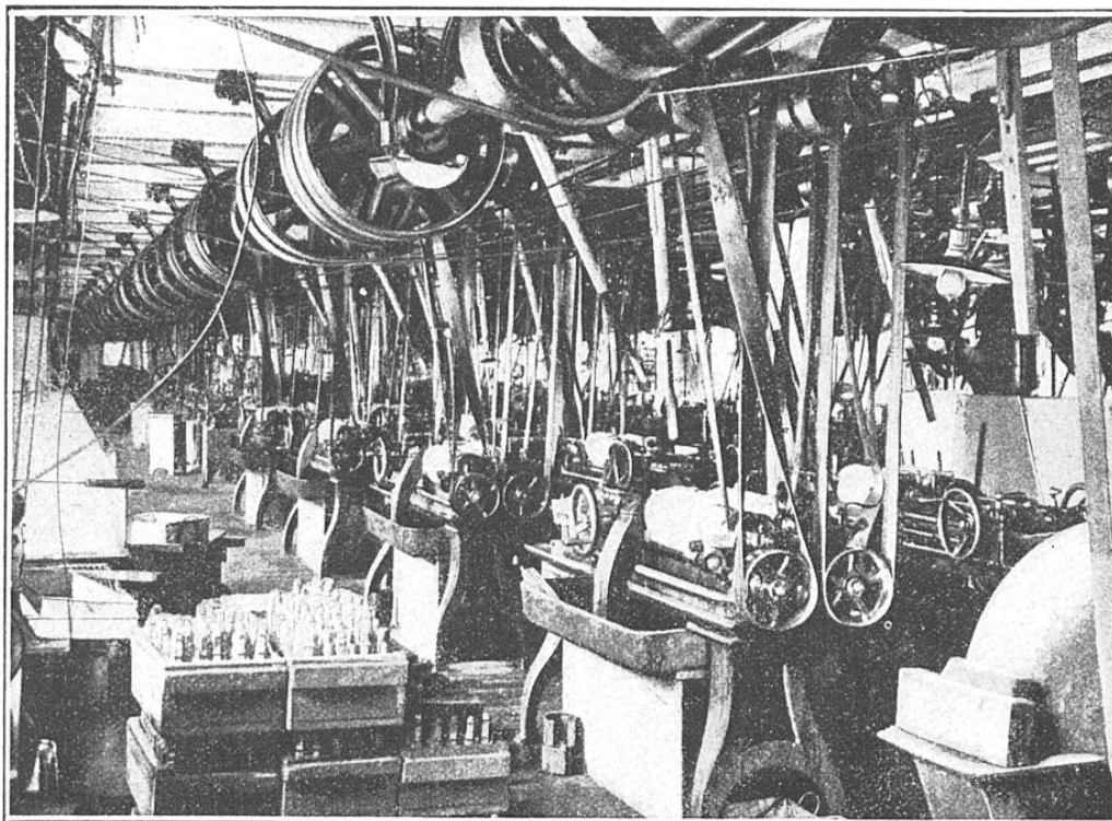
BATTERIE DE PERCEUSES POUR LE FORAGE MÉCANIQUE DES CANONS DE FUSILS
