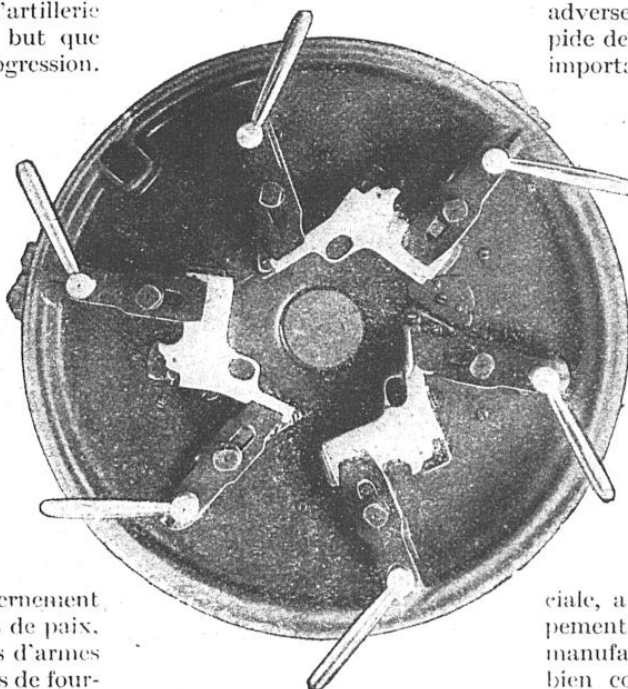
MANDRIN A SIX MACHOIRES POUR LE SERRAGE DES CANONS DE FU- SIL EN COURS DE FABRICATION
