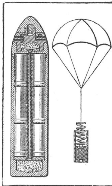
OBUS ÉCLAIRANT DU SYSTÈME ALLEMAND
