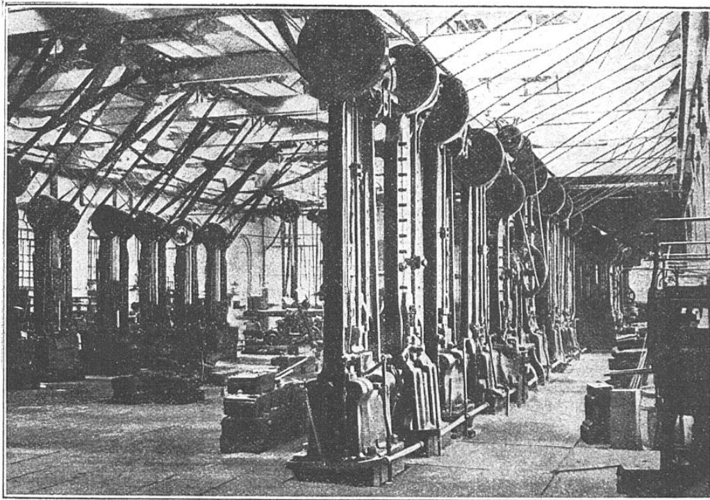
FORGE MUNIE DE MARTEAUX MÉCANIQUES DANS UNE MANUFACTURE D'ARMES
