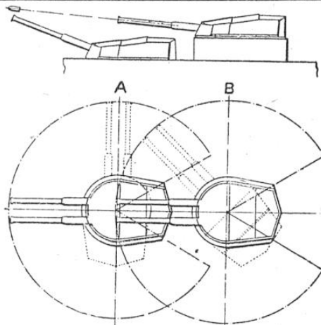
ANGLE DE TIR DE DEUX TOURELLES SUPERPOSÉES
