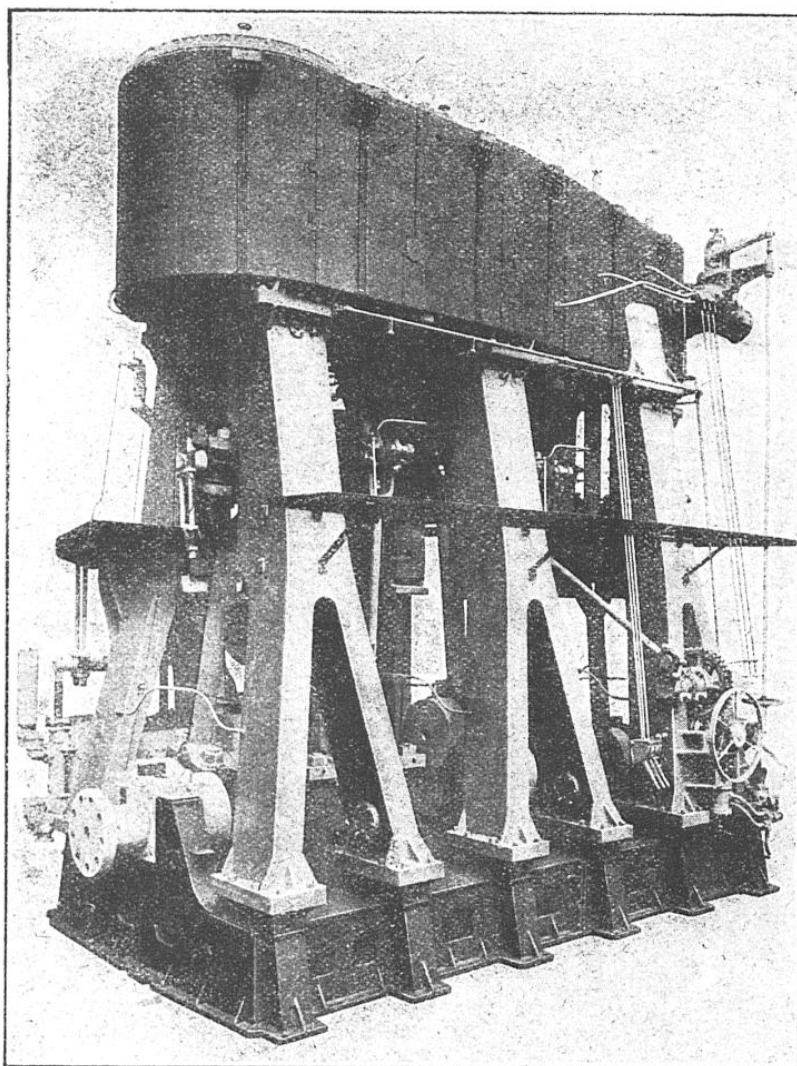
MOTEUR A TRIPLE EXPANSION, POUR VAPEUR CHARBONNIER
