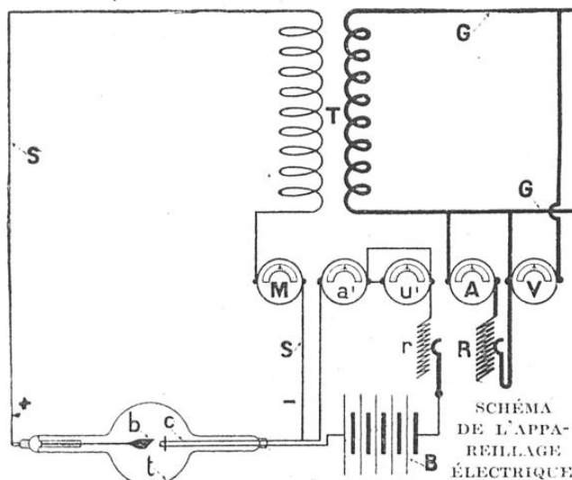
t, tube « Coolidge »; c, cathode; b, anticathode; T, transformateur du courant à haute tension; SS, connexions + et — du courant à haute tension; GG, connexions + et — du courant à basse tension alimentant le transformateur T; A, V, R, ampèremètre, voltmètre, rhéostat de réglage du courant à basse tension; M, milliampèremètre du courant à haute tension; a', u', r, ampèremètre, voltmètre et rhéostat de réglage du courant d'alimentation de la cathode; B, batterie d'accumulateurs fournissant le courant à la cathode.
