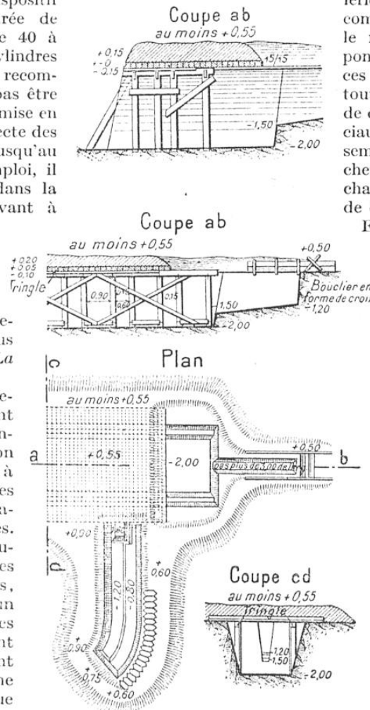
SAPE COUVERTE OU BLINDÉE DU TYPE DÉCRIT AU MANUEL DU PIONNIER ALLEMAND
