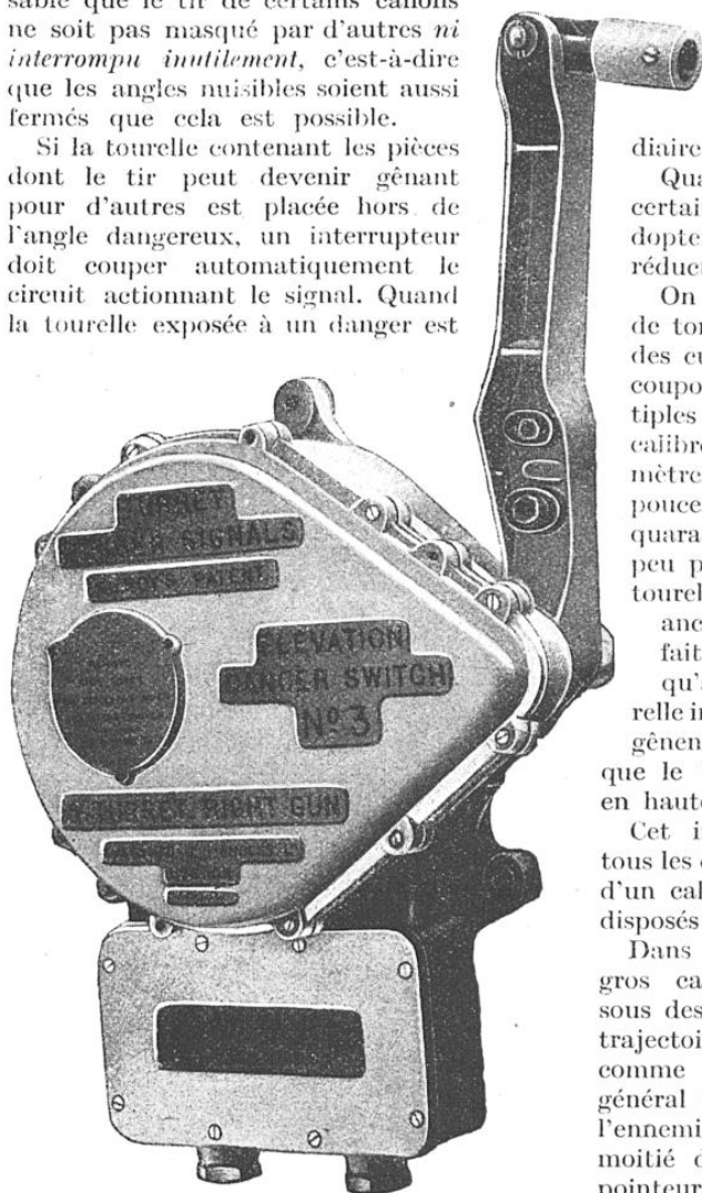
ANCIEN MODÈLE D'INTERRUPTEUR DE SÉCURITÉ
