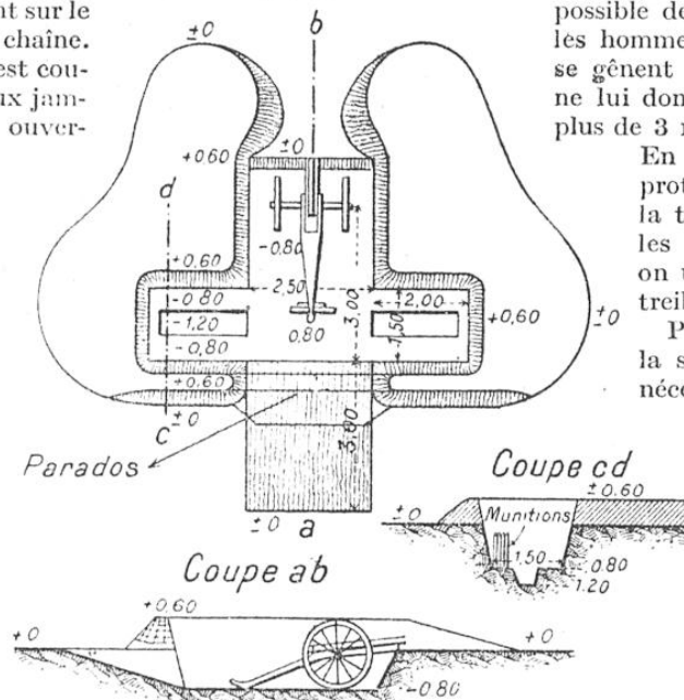
AUTRE DISPOSITIF DE COUVERT POUR PIÈCE D'ARTILLERIE
