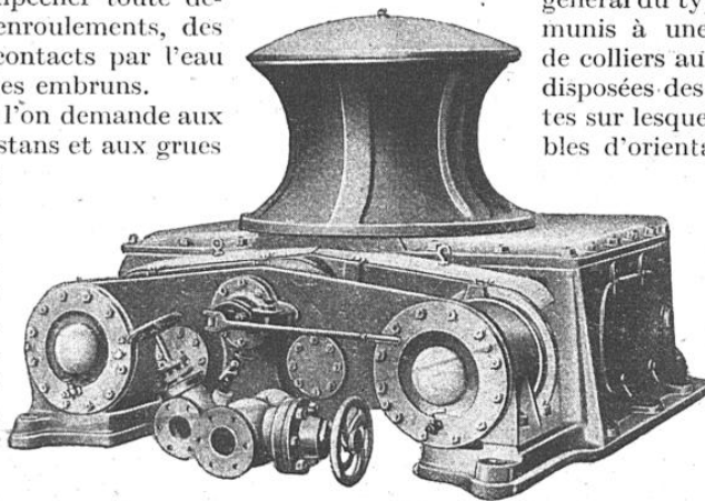
CABESTAN A VAPEUR MODÈLE RENFORCÉ
