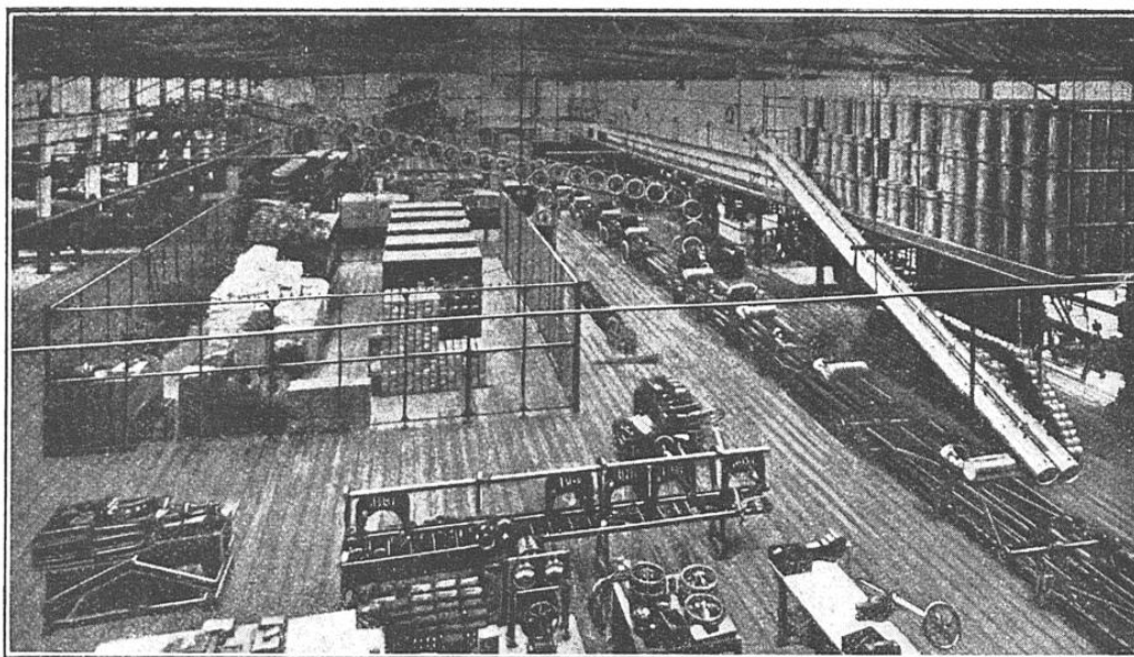
L'UN DES ATELIERS DE MONTAGE DANS UNE GRANDE FABRIQUE D'AUTOS DES ÉTATS-UNIS Toutes les pièces arrivent automatiquement au point où elles doivent être utilisées. On distingue notamment, au dernier plan de la photo, toute une théorie de roues qui viennent d'un autre atelier et se placent d'elles-mêmes aux côtés d'une file de châssis en montage, qu'on voit sur la droite.
