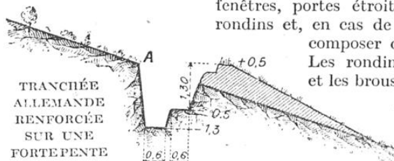
Quand la tranchée est construite sur une position dominante, on arrondit l'arête A afin de la rendre invisible.
