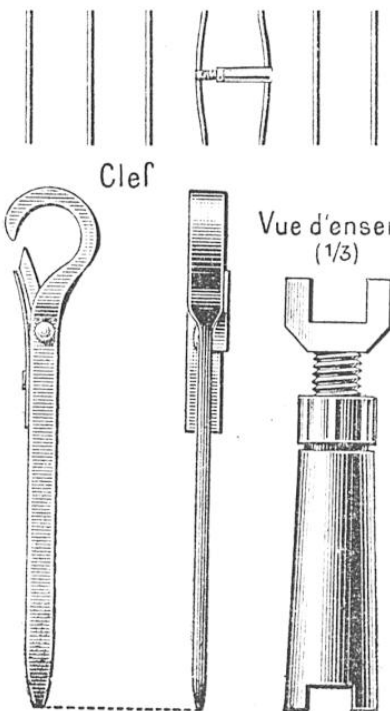
OUTIL SPÉCIAL DE PIONNIER DESTINÉ À ÉCARTER LES BARREAUX D'UNE GRILLE
