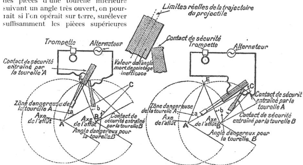
SCHEMA MONTRANT LE PRINCIPE DU FONCTIONNEMENT DES APPAREILS DE SÉCURITÉ DU SYSTÈME ANGLAIS KILROY
