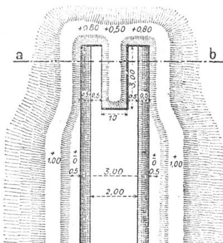
SAPE SIMPLE CONSTRUITE PAR LES PIONNIERS ALLEMANDS EN CAMPAGNE
