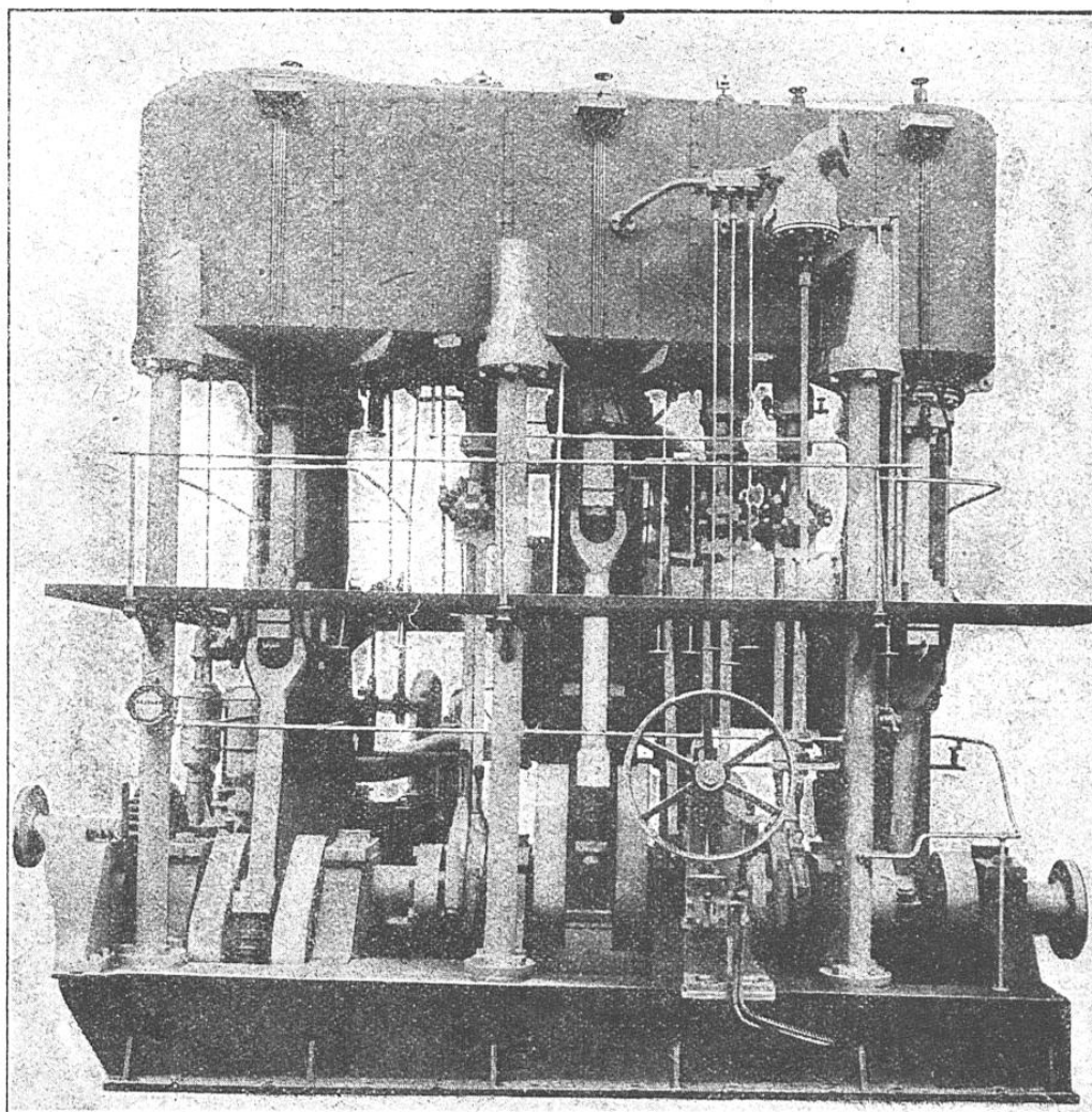
MACHINE A TRIPLE EXPANSION, POUR STEAMER A PASSAGERS
