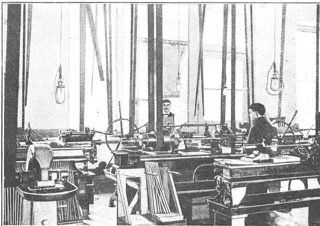
MACHINE A « CHAMBRER » LES CANONS DE FUSILS, DANS UNE FABRIQUE AMÉRICAINE
