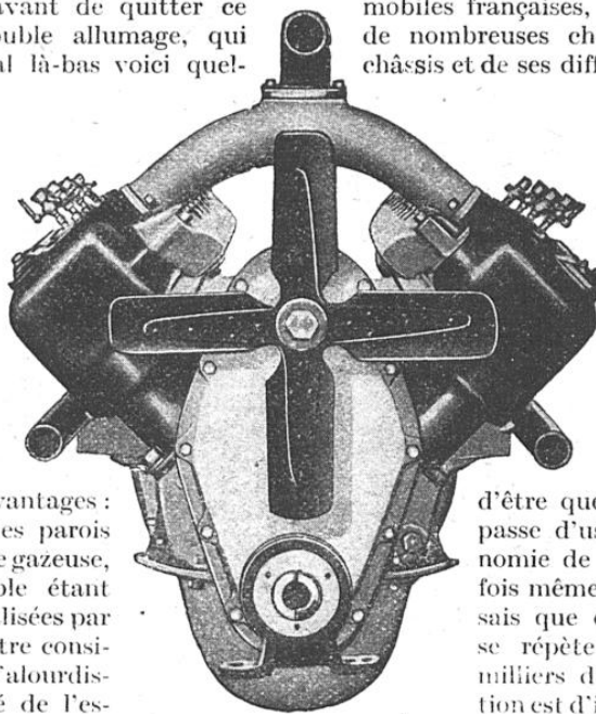
AVANT DU MOTEUR EN V
