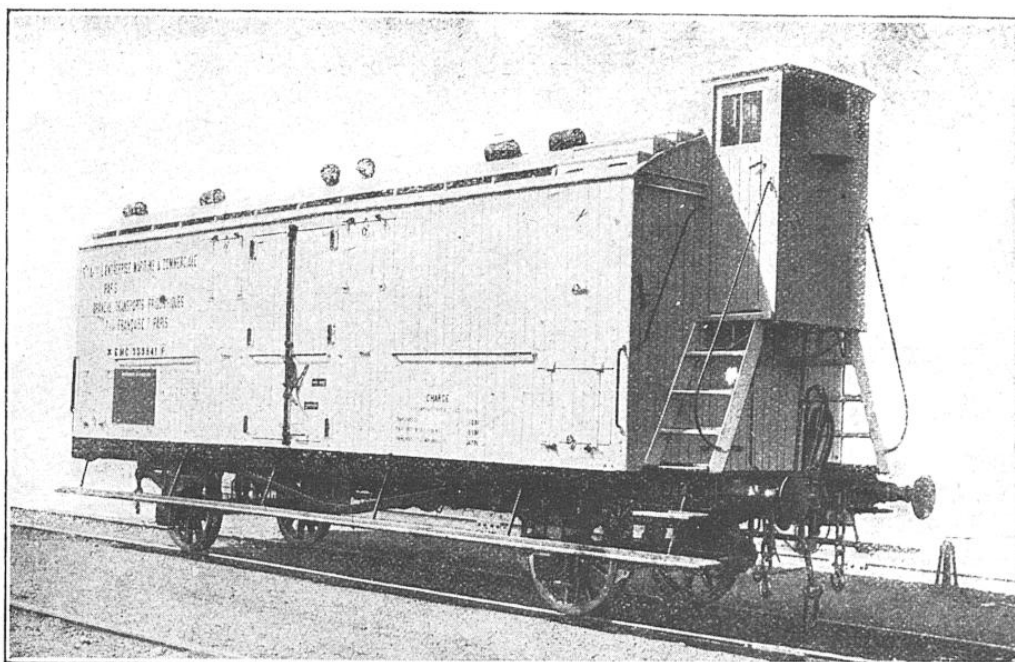
WAGON FRIGORIFIQUE FRANÇAIS AMÉNAGÉ POUR LE TRANSPORT DES VIANDES CONGELÉES ENTRE LES PORTS ET LES POINTS DE RAVITAILLEMENT DU FRONT
