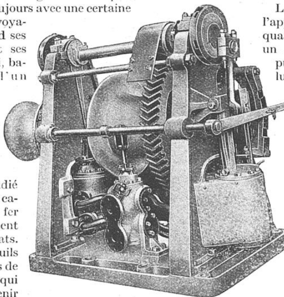
TREUIL MIXTE TYPE « VERTICAL »
