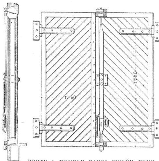
PORTE A DOUBLE PAROI ISOLÉE POUR LA FERMETURE D'UN FOURGON FRIGORIFIQUE
