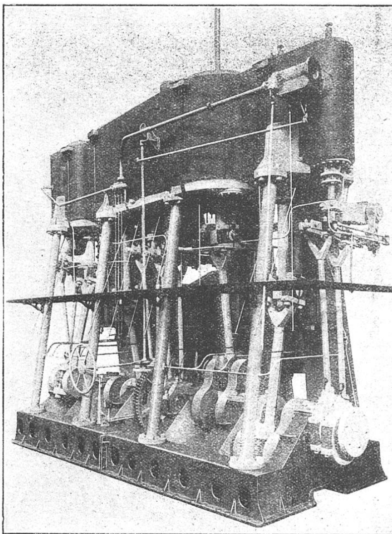
MACHINE LÉGÈRE A QUADRUPLE EXPANSION, POUR STEAMER.
