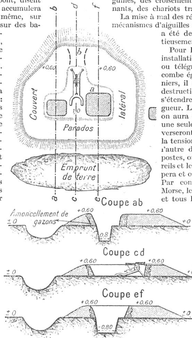
INSTALLATION D'UN COUVERT DE MITRAILLEUSE
