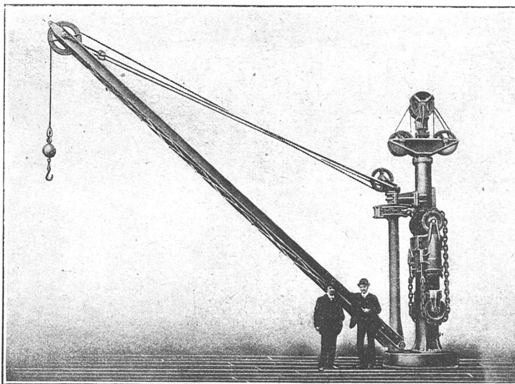
GRUE A COMMANDE HYDRAULIQUE POUR CARGO-BOAT
