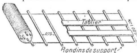
PLATE-FORME DÉROULABLE POUR LA TRAVERSÉE DES TERRAINS MARÉCAGEUX OU MOUS Ce chemin mobile est construit par la méthode dite du "tapis d'escalier", avec rondins de support et tablier en planches.
