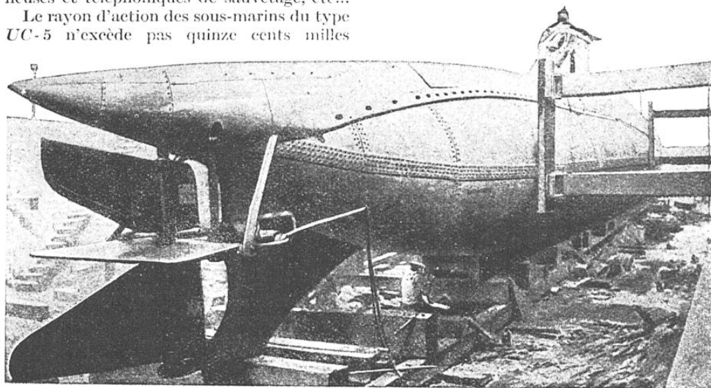
FORME ARRIÈRE, GOUVERNAIL DE DIRECTION ET GOUVERNAIL DE PLONGÉE (PLAN HORIZONTAL) DU SOUS-MARIN ALLEMAND « UC-5 »
