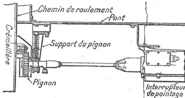
VUE EN ÉLÉVATION DU MONTAGE D'UN INTERRUPTEUR DE DANGER
