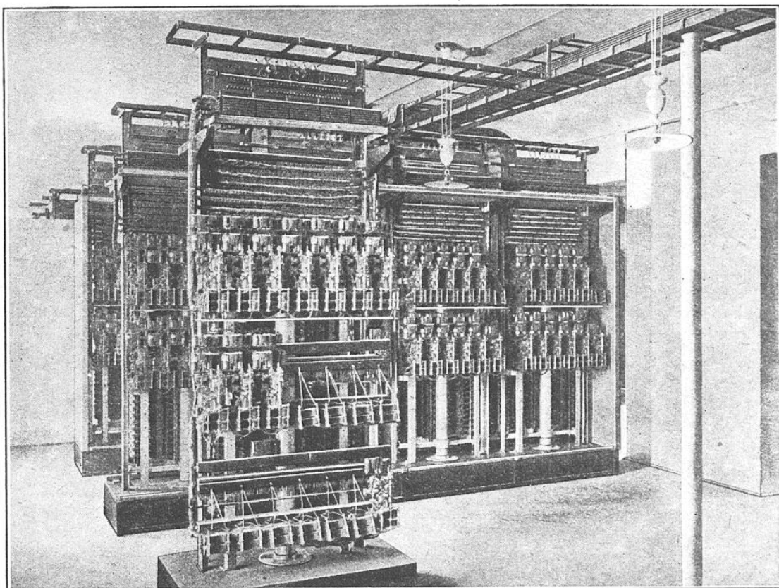
VUE D'ENSEMBLE DE CONNECTEURS ET DE CHEMINS DE CABLES AU CENTRAL DE NICE
