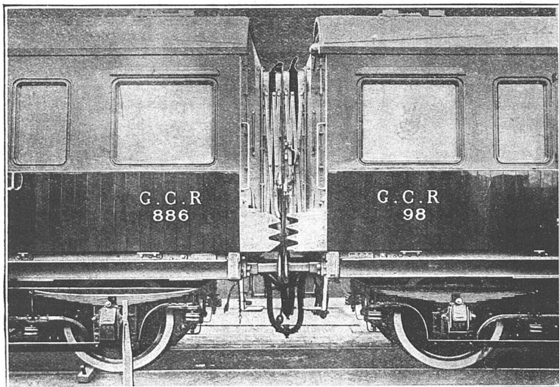
TAMPONS D'AMORTISSEURS DE DEUX VOITURES CONSÉCUTIVES D'UN TRAIN
