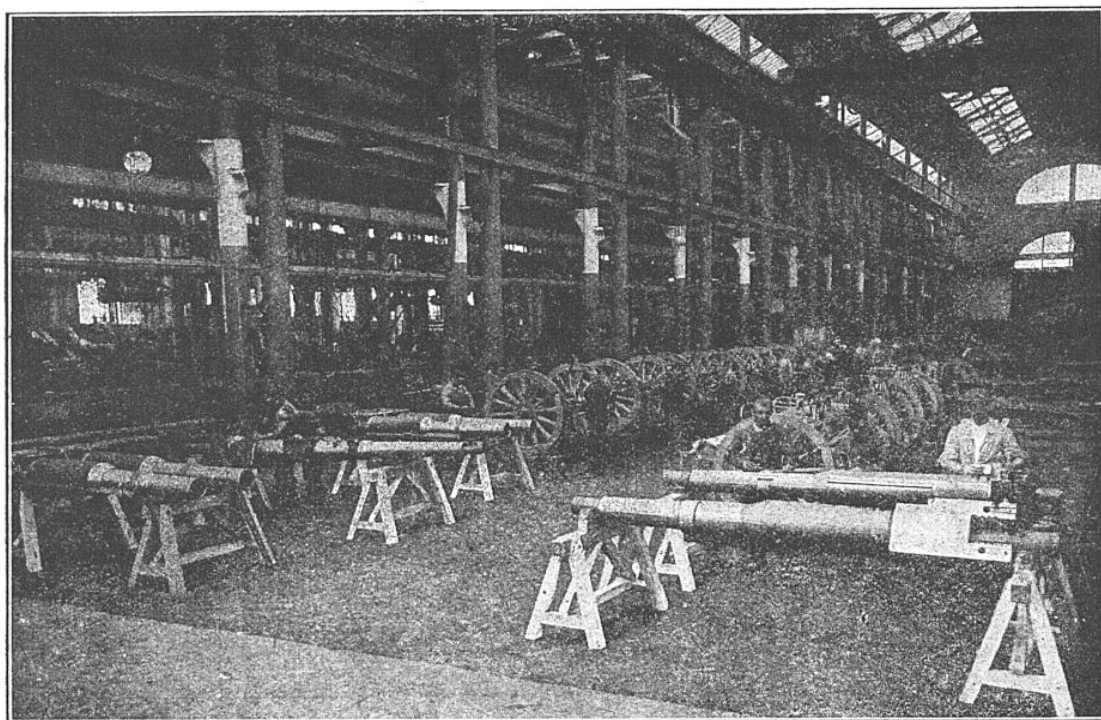
ATELIER DE MONTAGE DES AFFUTS ET DES CAISSONS POUR CANONS DE 155
