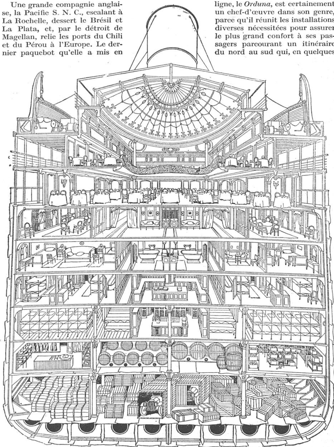
SECTION TRANSVERSALE DU « GIULIO CESARE », DE LA NAVIGAZIONE GENERALE ITALIANA Ce paquebot a les mêmes caractéristiques que le « Duilio » de la même compagnie.
