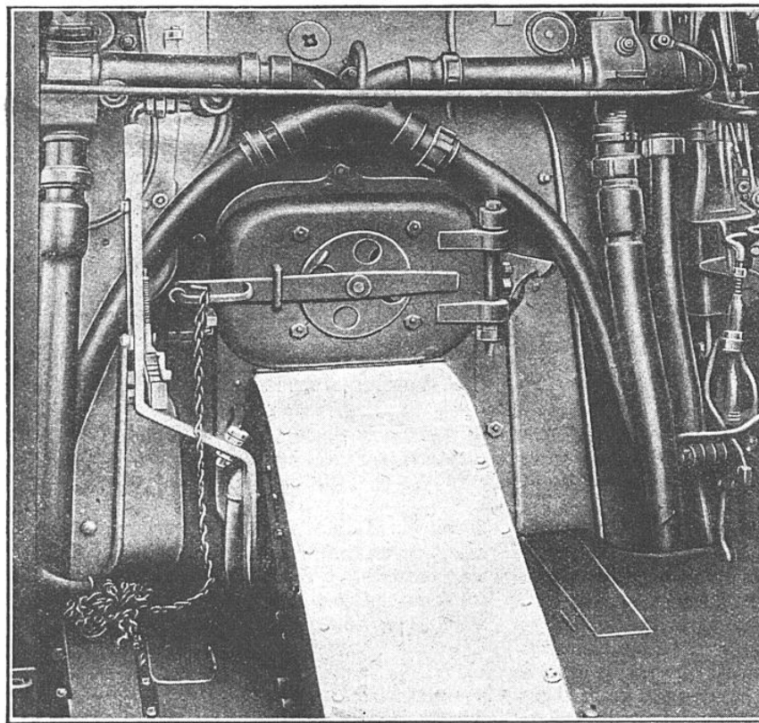
VUE GÉNÉRALE D'UN CHARGEUR AUTOMATIQUE SYSTÈME « GEE »
