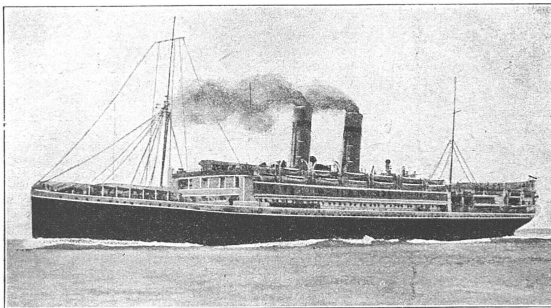
LE PAQUEBOT A DEUX HÉLICES « GELRIA », DU LLOYD ROYAL HOLLANDAIS Ce bâtiment est le similaire du « Tubantia », coulé par un sous-marin allemand. Il a été construit en 1913, à Glasgow, aux Chantiers navals Alex. Stephen et fils; il mesure 170 m. 64 de long et sa jauge brute est de 14.053 tonneaux.
