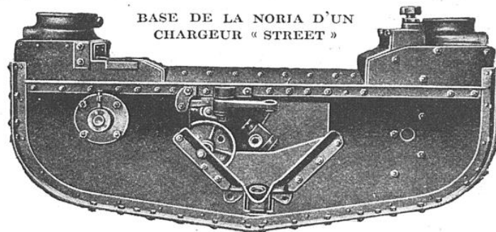
BASE DE LA NORIA D'UN CHARGEUR « STREET » Les godets se déplacent horizontalement dans cette enveloppe, qui comporte, à droite et à gauche, deux embases sur lesquelles sont montés les tuyaux du transporteur.
