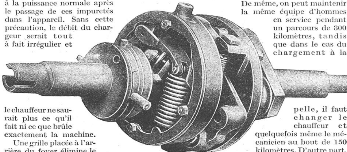
RÉGULATEUR DU MOTEUR A VAPEUR SERVANT A ASSURER LE DÉBIT DU COMBUSTIBLE (SYSTÈME "STREET")
