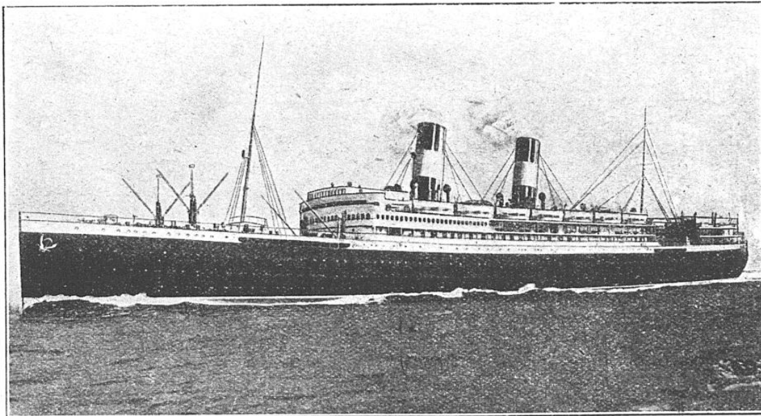
LE PAQUEBOT A QUATRE HÉLICES « DUILIO », DE LA NAVIGAZIONE GÉNÉRALE ITALIANA Construit en 1916 aux Chantiers G. Ansaldo et Co, à Sestri Ponente, ce superbe navire à 194 mètres de longueur; sa jauge brute est de 22.000 tonneaux.
