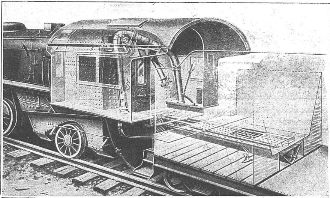
AGENCEMENT D'UN CHARGEUR DU SYSTÈME « STREET » SUR UNE LOCOMOTIVE
