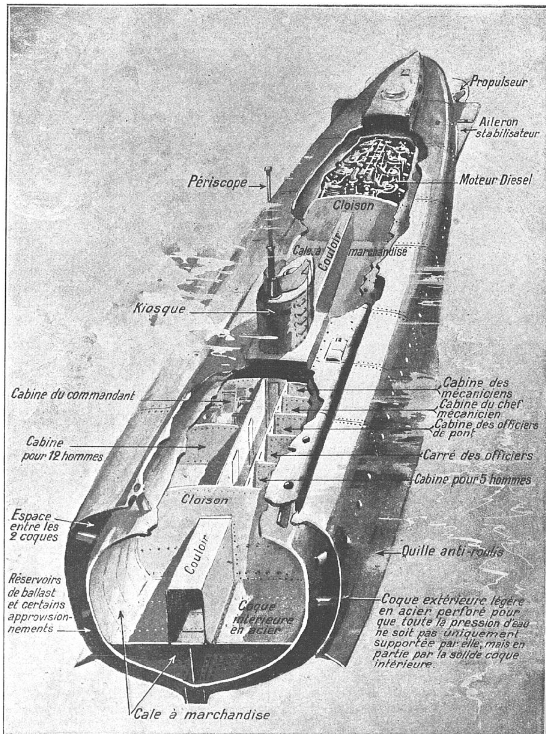
LE CARGO-BOAT SOUS-MARIN « DEUTSCHLAND », QUI TRAVERSA QUATRE FOIS L'ATLANTIQUE Ce dessin a été exécuté d'après des indications précises fournies par des Américains qui le visitèrent.
