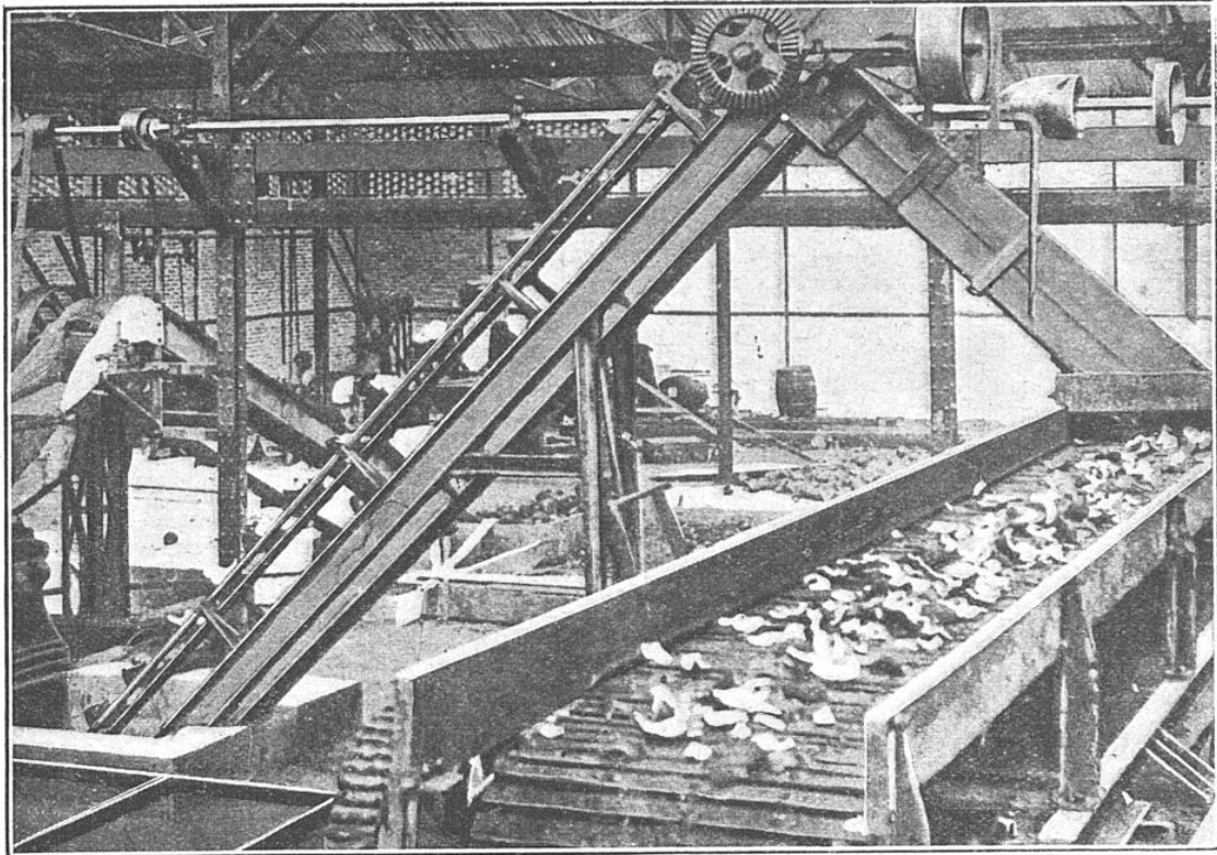
MACHINERIE INTÉRIEURE DE L'USINE REPRÉSENTÉE À LA PAGE PRÉCÉDENTE
