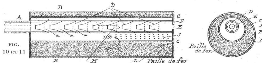
SILENCIEUX DE THURLER (COUPE LONGITUDINALE ET COUPE VERTICALE)
