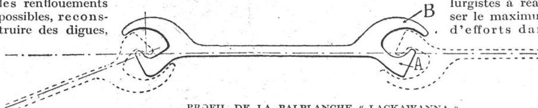
PROFIL DE LA PALPLANCHE « LACKAWANNA »
