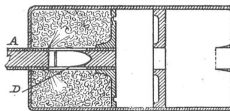
FIG. 7. — VARIANTE DE LA FIGURE PRÉCÉDENTE, AVEC DIVISION EN TROIS CHAMBRES
