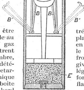
OBUS A GRIFFES
