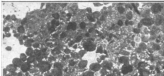
LE MINÉRAI DE FER OOLITHIQUE DE BRIEY, TAILLÉ EN LAME DE DEUX À TROIS CENTIÈMES DE MILLIMÈTRES D'ÉPAISSEUR. Cette lame a été photographiée avec un grossissement de huit diamètres. On y voit la forme des granules ferrugineux et même leur structure, qui est à la fois concentrique et rayonnée.
