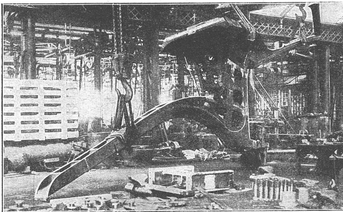
ETAMBOT POUR CUIRASSÉ, EN COURS DE FABRICATION
