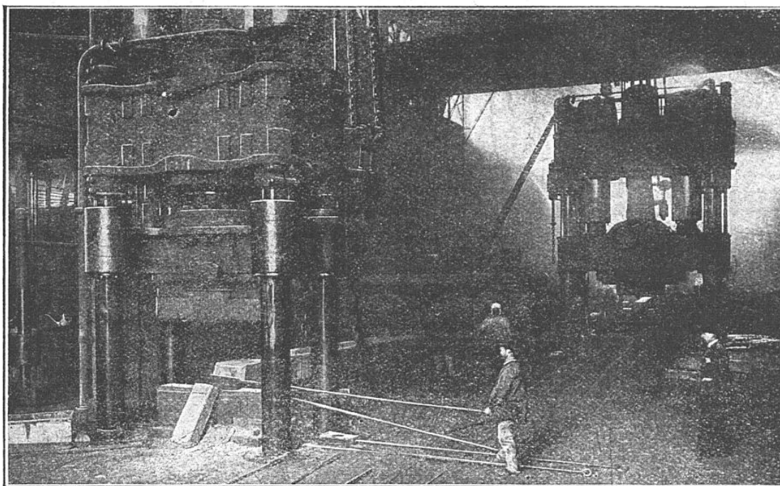
PRESSES A FORGER HYDRAULIQUES DE 1.500 ET 6.000 TONNES
