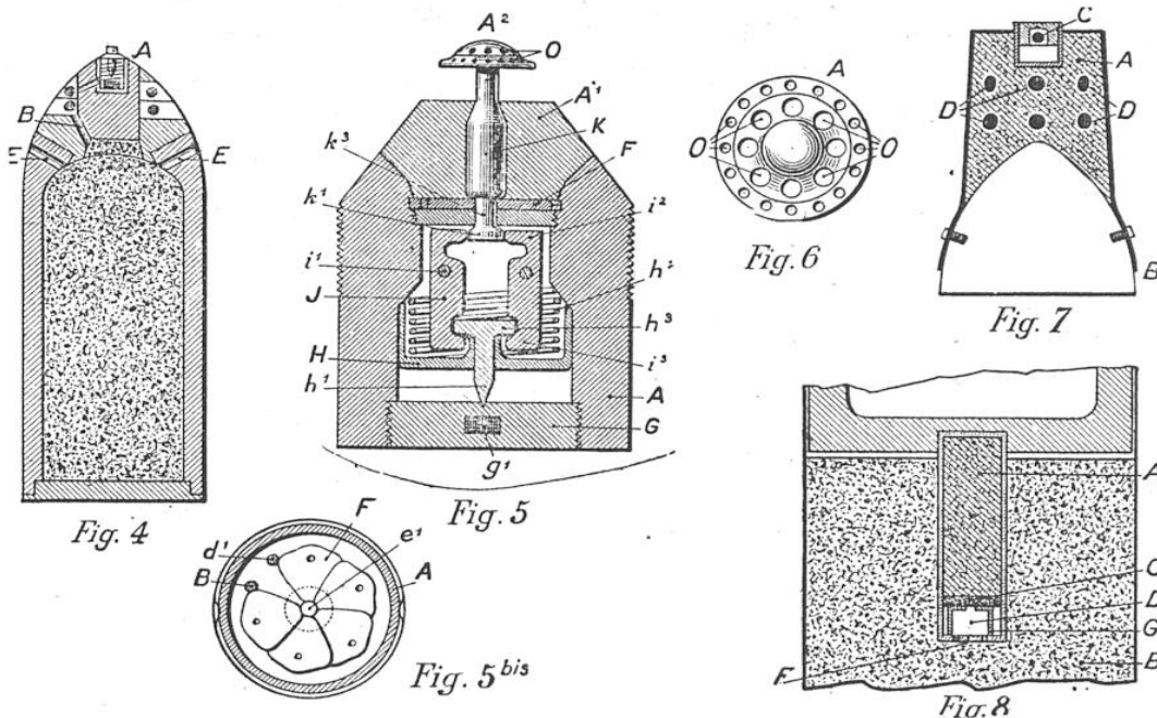
FIGURE 4. — OBUS A CHARGE INTÉRIEURE (COUPE VERTICALE) : A, fusée de tête allumant la composition par le conduit B ; EE, évents par lesquels sortent la fumée (indiquant très nettement la trajectoire pendant le jour) et le feu (pour la nuit et pour incendier).
