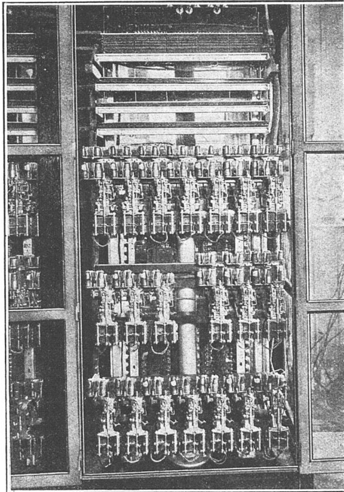
BÂTI UNITAIRE VU DU CÔTÉ DES CONNECTEURS (INSTALLATION PRIVÉE)
