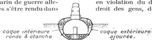
COUPE TRANSVERSALE DU SOUS-MARIN COMMERCIAL DE LA COMPAGNIE TRANSOCÉANIQUE ALLEMANDE AYANT SON SIÈGE A BRÊME
