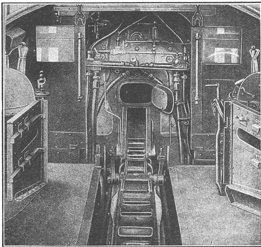
VUE DU TRANSPORTEUR D'UN CHARGEUR SYSTÈME « GEE »
