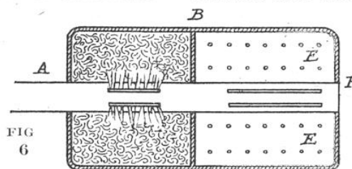
FIG. 6. — A, canon du fusil; B, corps du silencieux divisé en deux chambres par une cloison; E, petits trous dans la deuxième chambre, permettant aux gaz de se diffuser partiellement dans l'atmosphère.
