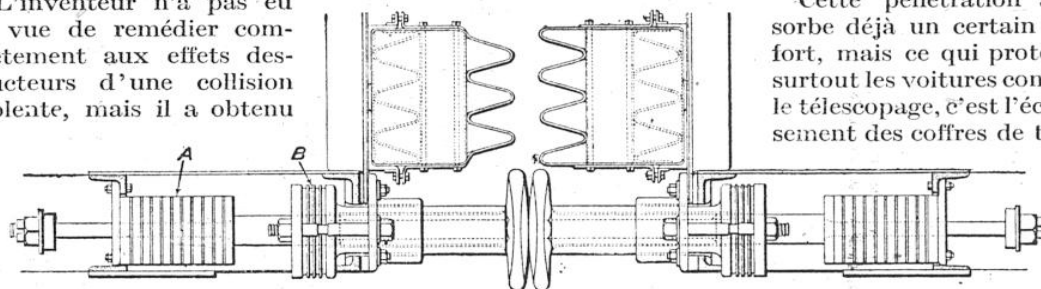
FIG. 3. — RESSORT DE TAMPON ORDINAIRE A ET RESSORT DE TAMPON A COURSE DE RÉSERVE B COMPRIMÉ A BLOC
