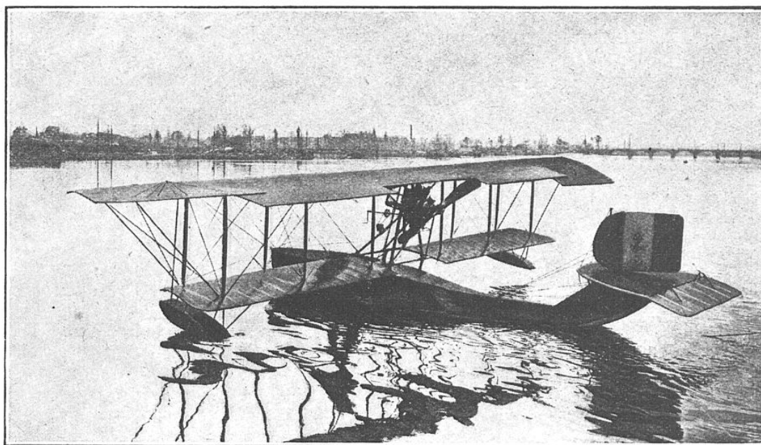
UN HYDRAVION A COQUE-FUSELAGE FLOTTANT AU REPOS, EN EAU CALME
