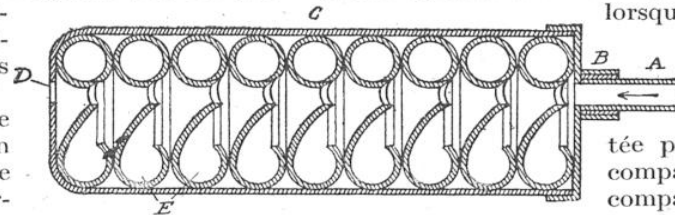
FIG. 5. — A, canon de l'arme; B, collier fixant l'appareil au bout du canon; C, corps du silencieux divisé en compartiments spiraliformes et conchoïdaux, en coupe transversale; D, orifice de sortie du projectile; E, chambres successives formées par les cloisons.
