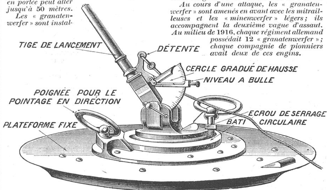
« GRANATENWERFER » CONSTRUIT PAR KRUPP AU DÉBUT DE L'ANNÉE 1915
