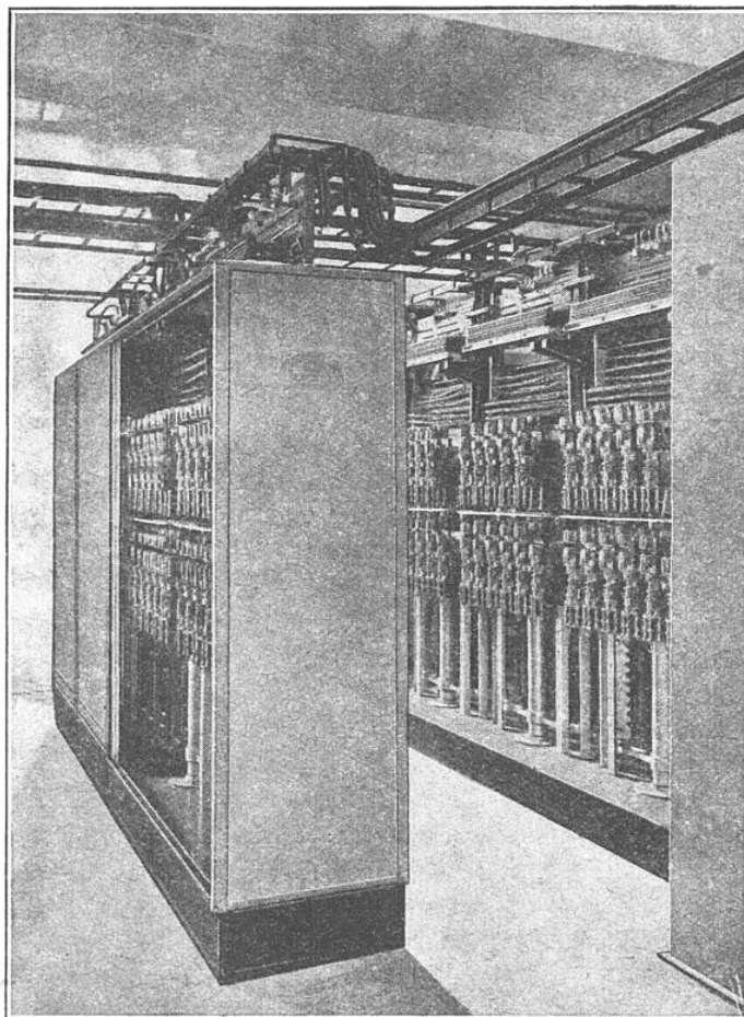
VUE D'ENSEMBLE DE DEUX GROUPES DE 400 LIGNES AU CENTRAL TÉLÉPHONIQUE DE NICE
