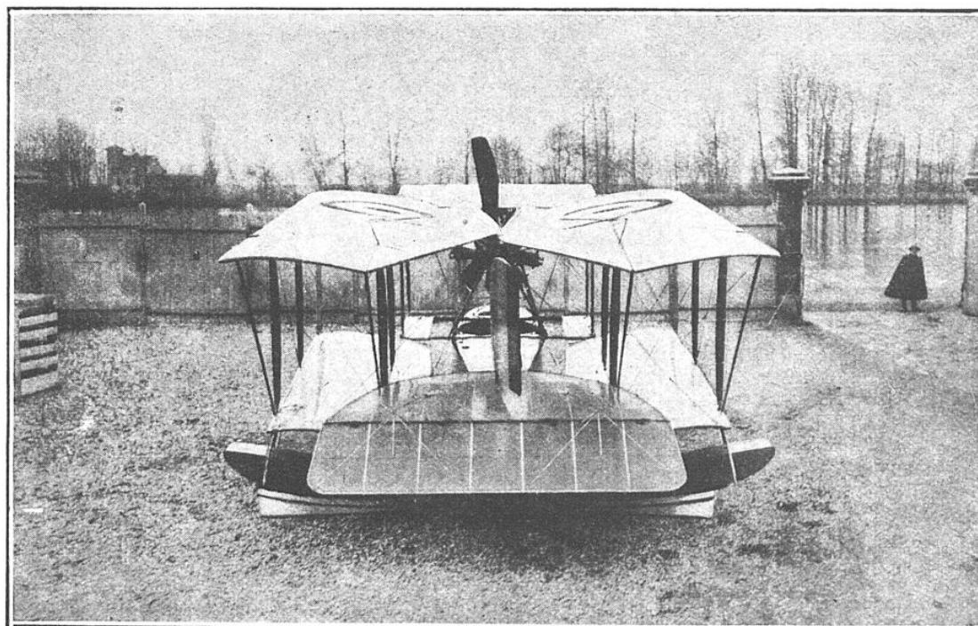
VUE ARRIÈRE D'UN APPAREIL A COQUE-FUSELAGE DONT LES AILES ONT ÉTÉ REPLIÉES
