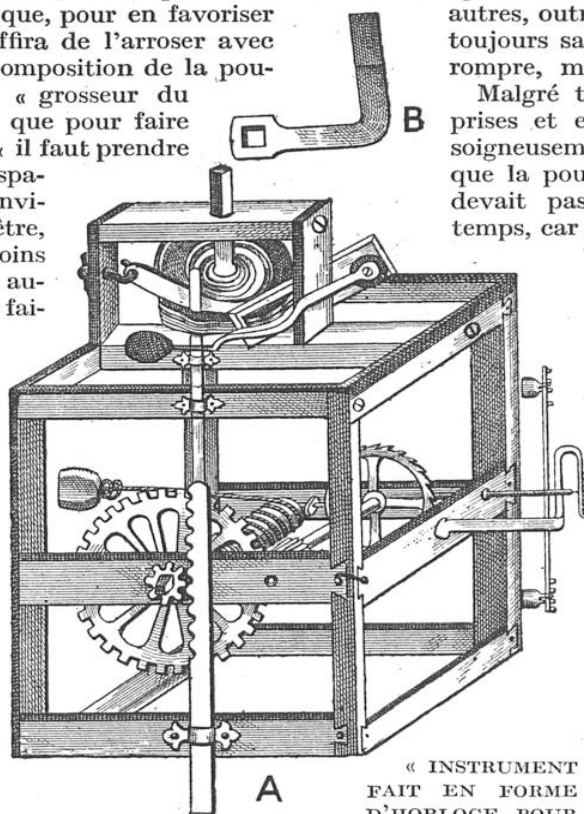
« INSTRUMENT FAIT EN FORME D'HORLOGE POUR DONNER LE FEU AUX BATEAUX SAUTANS » A, mouvement d'horlogerie ; B, manivelle-remontoir.
