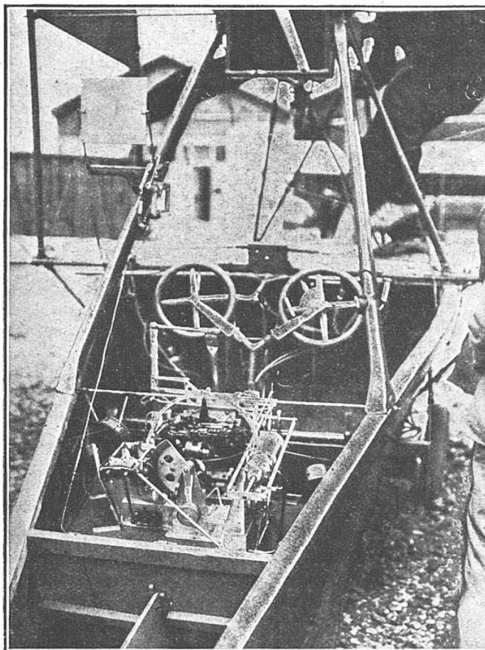
MONTAGE D'UN STABILISATEUR GYROSCOPIQUE SPERRY SUR UN « FLYING BOAT » CURTISS A DOUBLE COMMANDE
