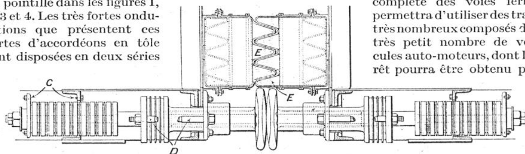
FIG. 4. — DISPOSITION DES ORGANES DE SÉCURITÉ DES WAGONS APRÈS UN CHOC VIOLENT Les bords de retenue C du ressort de tampon ordinaire et les bords de retenue D du ressort de tampon à course de réserve ont été brisés, et les amortisseurs E sont entrés en prise.
