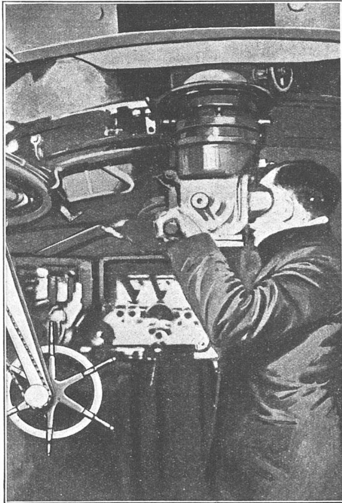
LA CHAMBRE DU PÉRISCOPE DU « DEUTSCHLAND »
