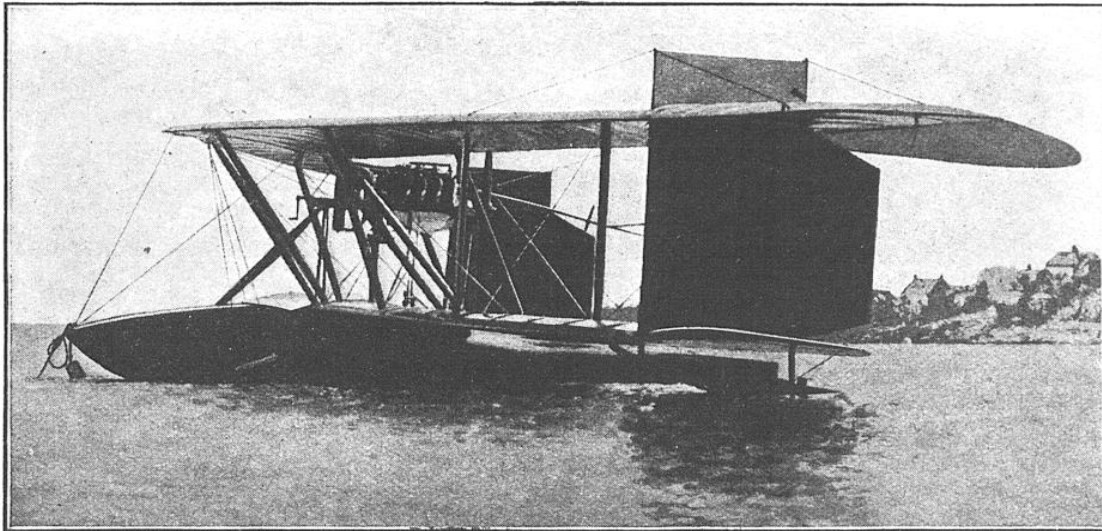
L'HYDRAVION AMÉRICAIN DU SYSTÈME BURGESS-DUNNE
