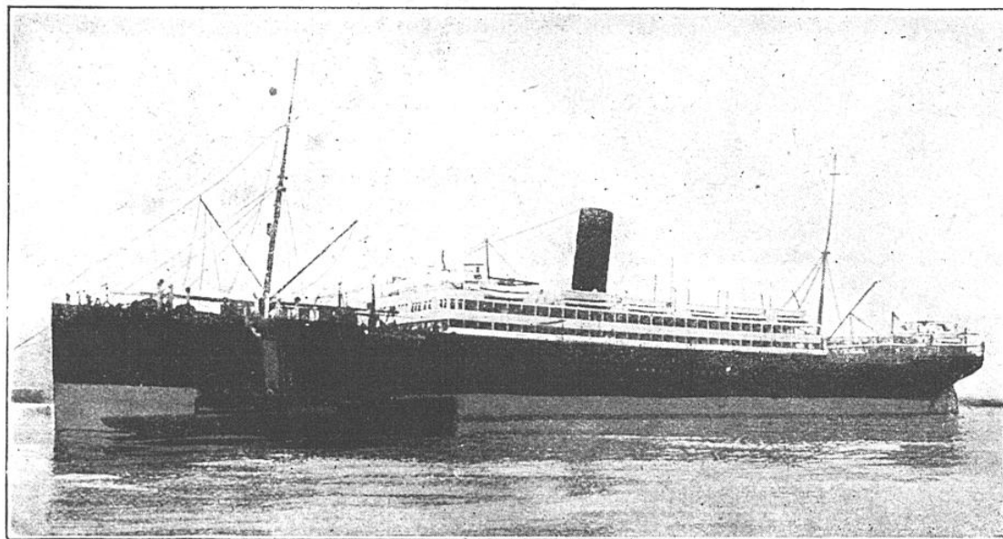
LE PAQUEBOT A TROIS HÉLICES «ORDUNA», DE LA PACIFIC STEAM NAVIGATION CO Construit en 1913, à Belfast, ce navire a 173 m. 50 de long et jauge 15,498 tonneaux.
