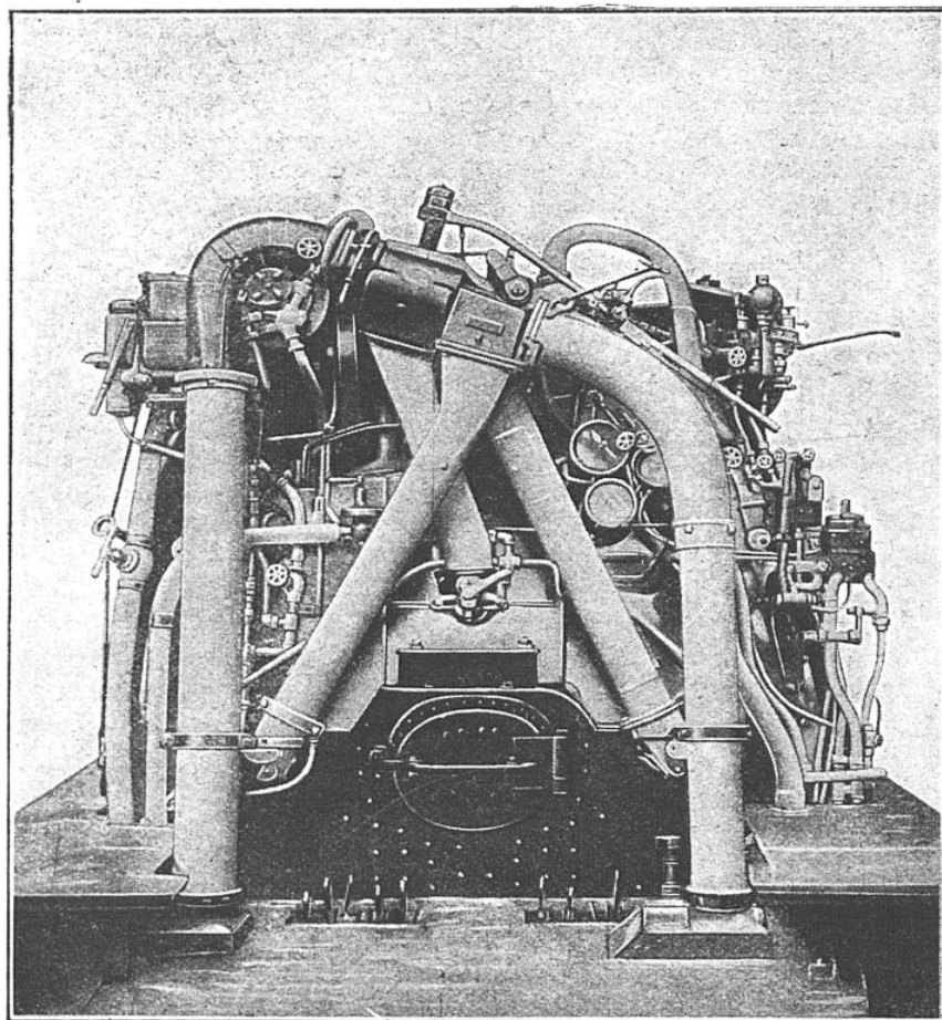
ARRIÈRE D'UNE CHAUDIÈRE DE LOCOMOTIVE MUNIE D'UN CHARGEUR
