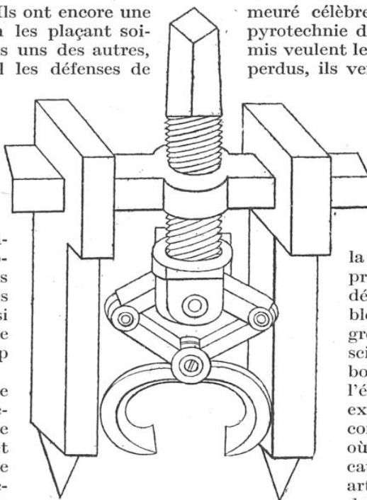
CURIEUSE TENAILLE MÉCANIQUE « Instrument fort gentil pour arracher palissades, barricades, verroulz et choses semblables, sans bruit et sans être découvert. »
