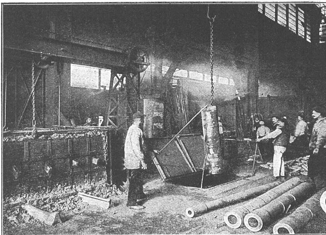
TRÈMPE D'UNE JAQUETTE POUR CANON DE 155 MILLIMÈTRES.
