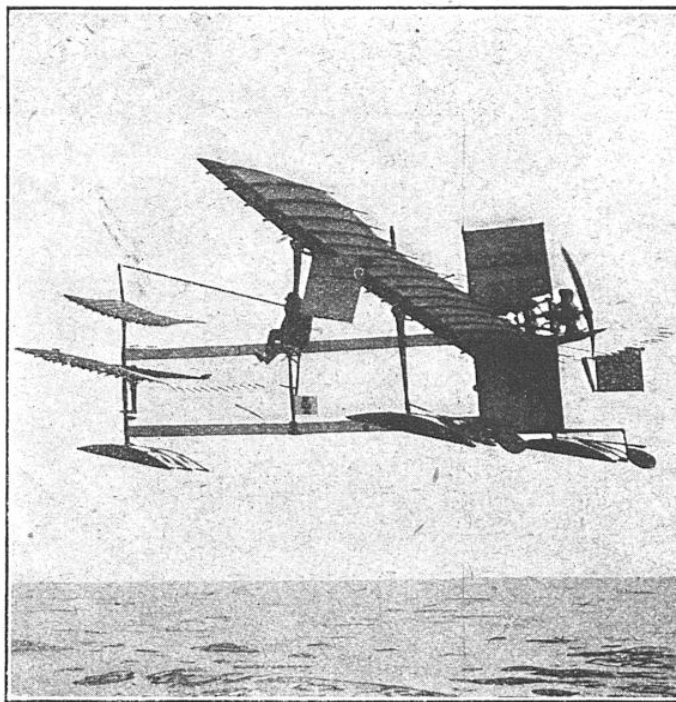
UN VOL DE L'HYDROAÉROPLANE FABRE
