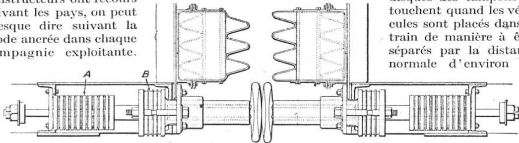
FIG. 2. — RESSORT DE TAMPON ORDINAIRE A COMPRIMÉ ET RESSORT DE TAMPON A COURSE DE RÉSERVE B
