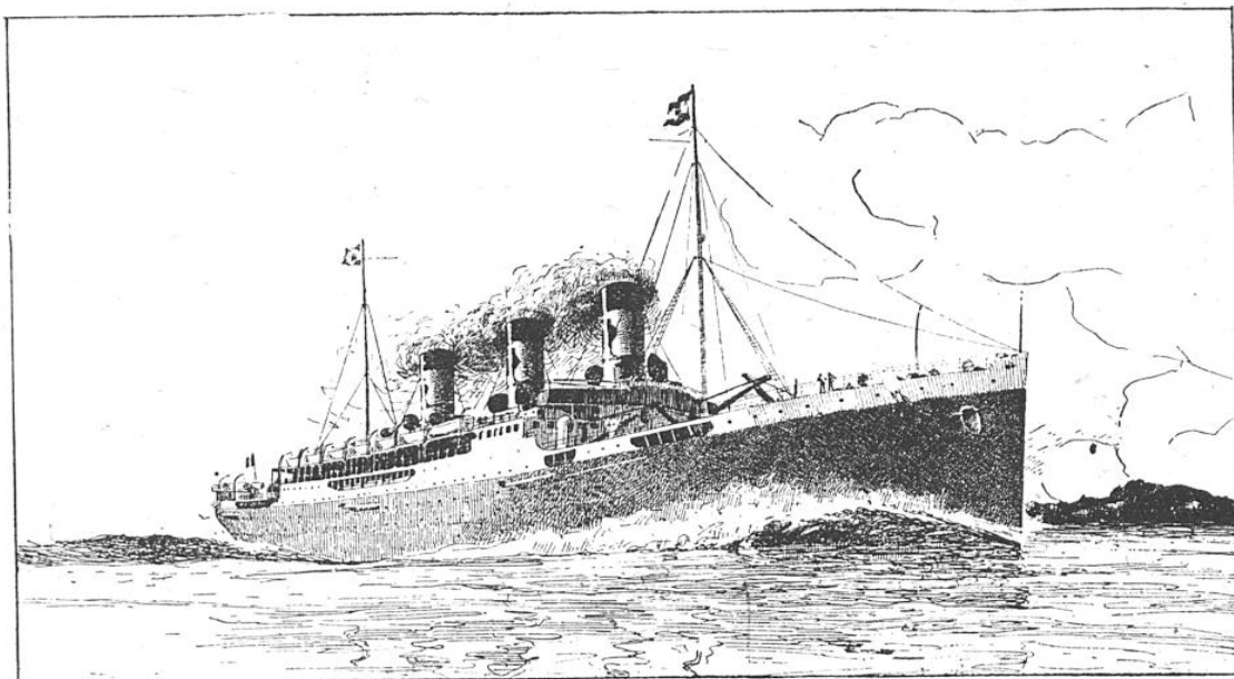
LE PAQUEBOT A QUATRE HÉLICES « LUTETIA », DE LA COMPAGNIE SUD-ATLANTIQUE Construit en 1913 aux Chantiers de l'Atlantique, à Saint-Nazaire, il est le similaire du « Gallia » (182 m. 73 de long, 14,581 tonneaux) coté par un sous-marin allemand.
