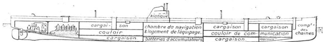
COUPE LONGITUDINALE (AU-DESSUS) ET VUE EN PLAN (AU-DESSOUS) DU « DEUTSCHLAND »
