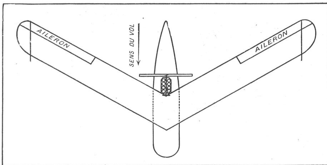
VUE SCHÉMATIQUE DE L'HYDROAÉROPLANE SANS QUEUE BURGESS-DUNNE
