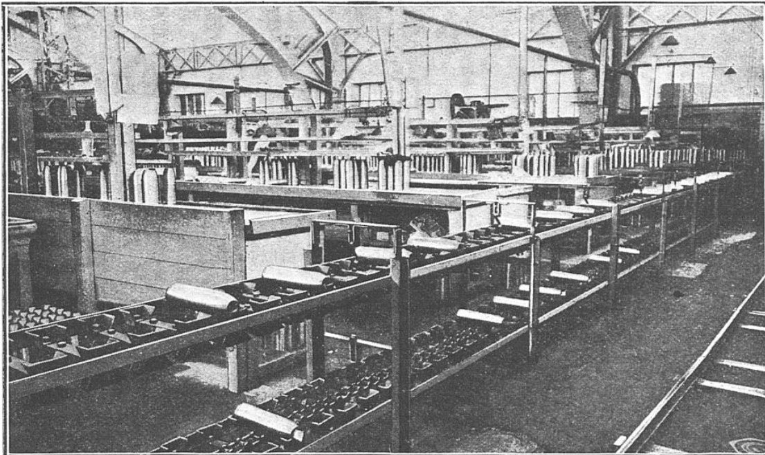
TRANSPORTEUR DE PROJECTILES DU TYPE A AUGETS TRANSVERSAUX.
