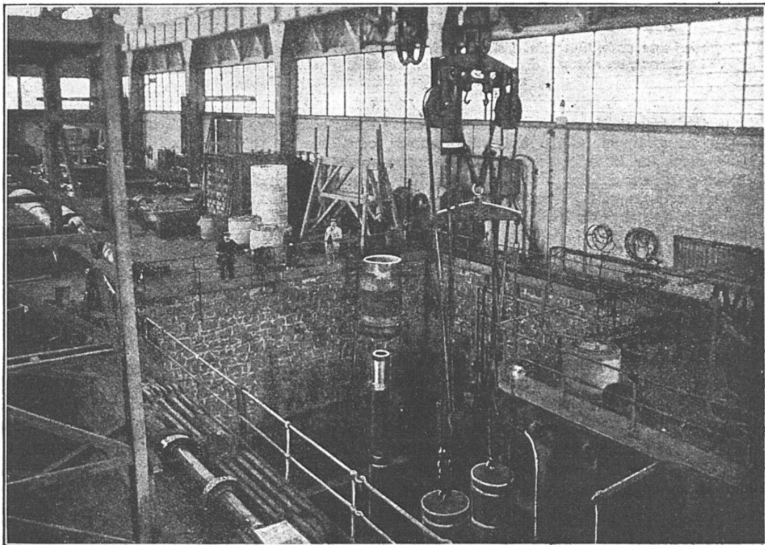
OPÉRATION DU FRETAGE D'UNE PIÈCE D'ARTILLERIE DE 340
