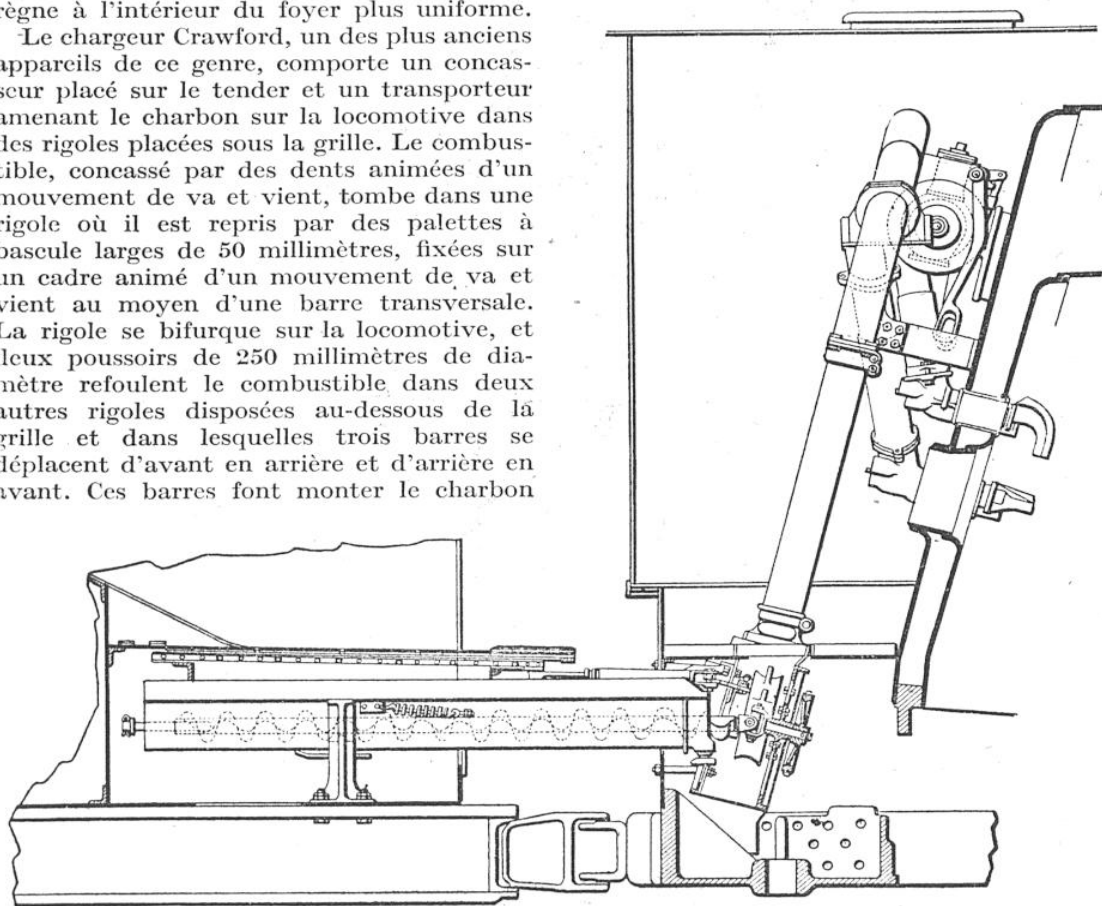
VUE LATÉRALE D'UN CHARGEUR AUTOMATIQUE DU SYSTÈME « STREET »
