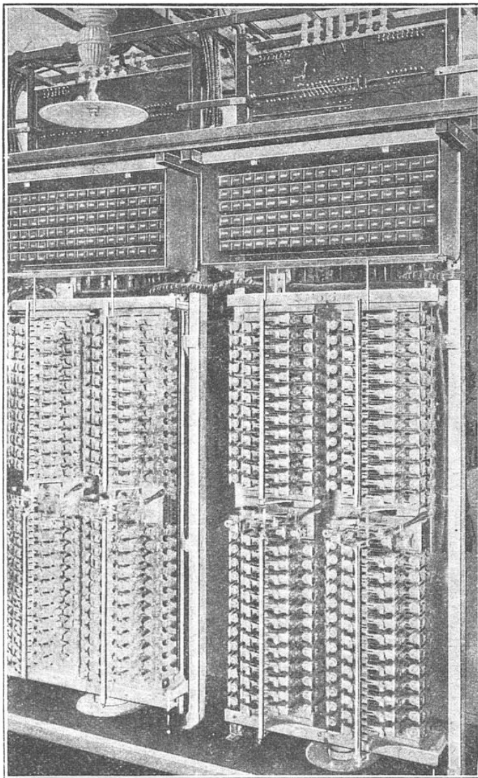
BATIS UNITAIRES DU COTÉ DES PLONGEURS ET COMMUTATEURS PRINCIPAUX (CENTRAL AUTOMATIQUE DE NICE)
