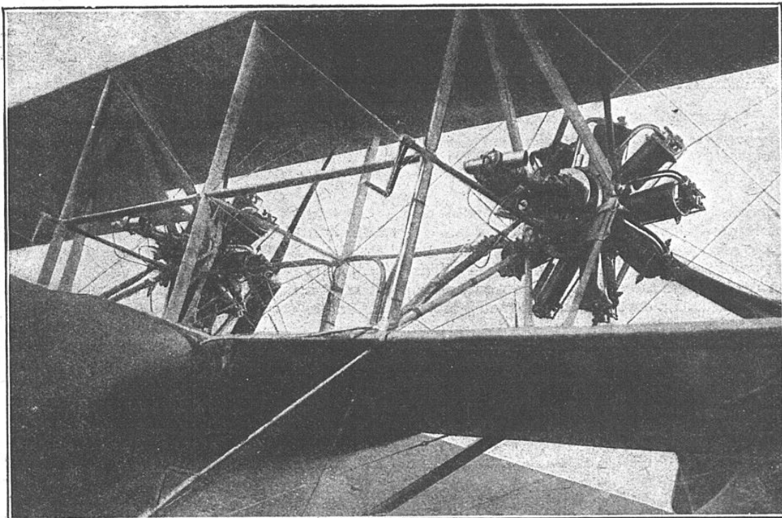
DISPOSITION DES DEUX MOTEURS ROTATIFS D'UN GRAND "BATEAU-VOLANT"
