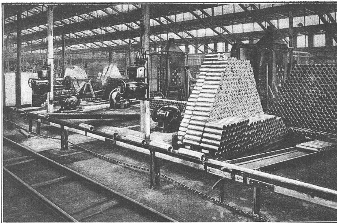
TRANSPORTEUR A CHAÎNE DESSERVANT UN ATELIER DE MUNITIONS
