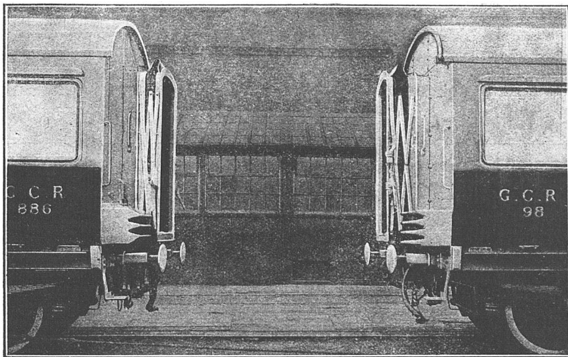
VUE LATÉRALE DES EXTRÉMITÉS DE DEUX VOITURES A INTERCOMMUNICATION
