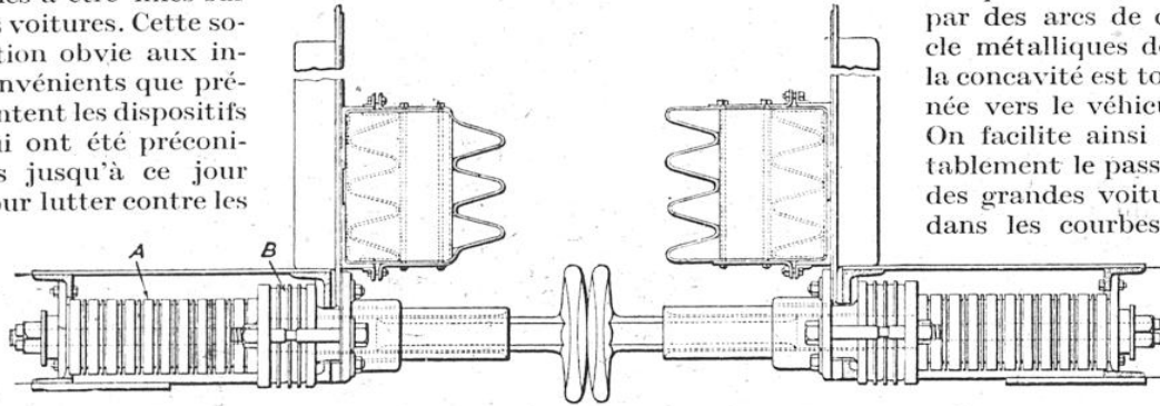
FIG. 1. — RESSORT DU TAMPON ORDINAIRE A ET RESSORT DU TAMPON A COURSE DE RÉSERVE B DANS LEUR POSITION NORMALE
