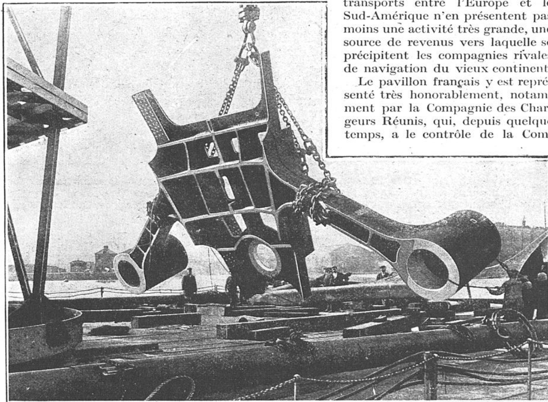
L'ÉTAMBOT DU « BRITANNIC » ET LES CHAISES DES ARBRES DES HÉLICES LATÉRALES On peut juger, d'après la grandeur des personnages qui sont sur les chantiers, des dimensions véritablement colossales de cette pièce métallique.
