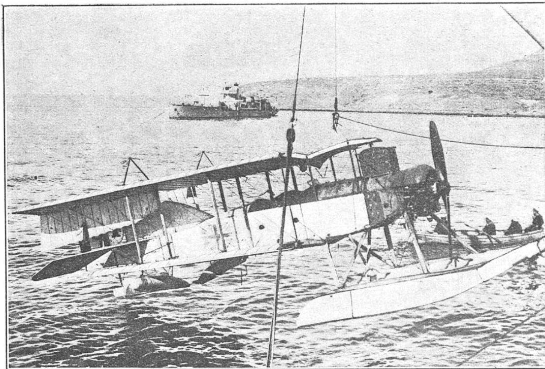
HISSAGE D'UN HYDRAVION ANGLAIS A BORD D'UN NAVIRE PORTE-AVIONS
