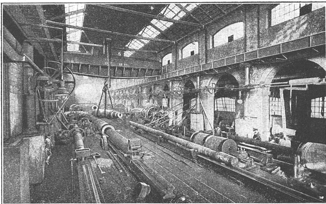
ATELIER DE FORAGE DES TUBES POUR CANONS DE TOUS CALIBRES
