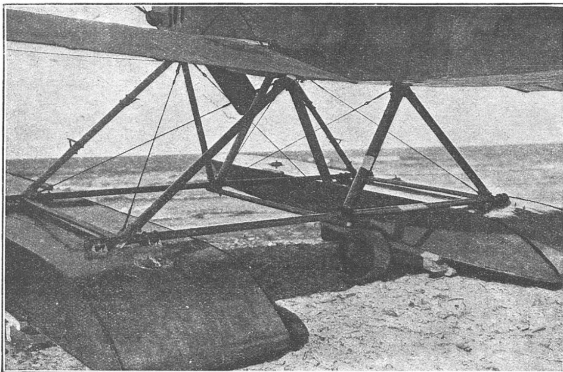
VUE DÉTAILLÉE DU SYSTÈME FLOTTEUR D'UN HYDROAÉROPLANE « ALBATROS »
