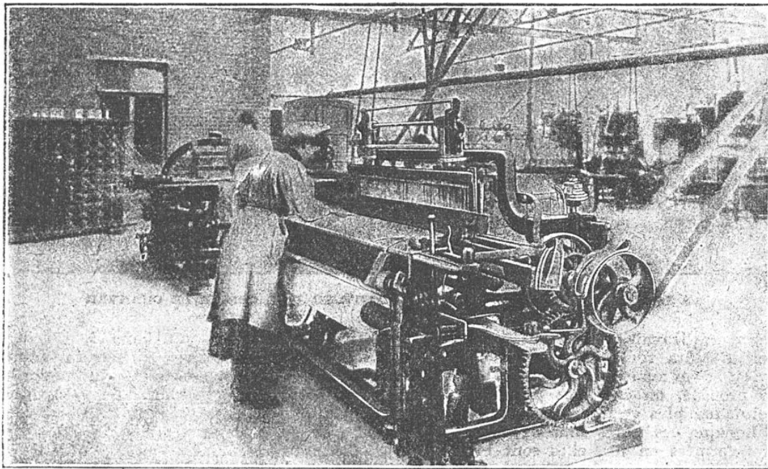
MÉTIER HORIZONTAL SERVANT A FABRIQUER DES TOILES D'AMIANTE
