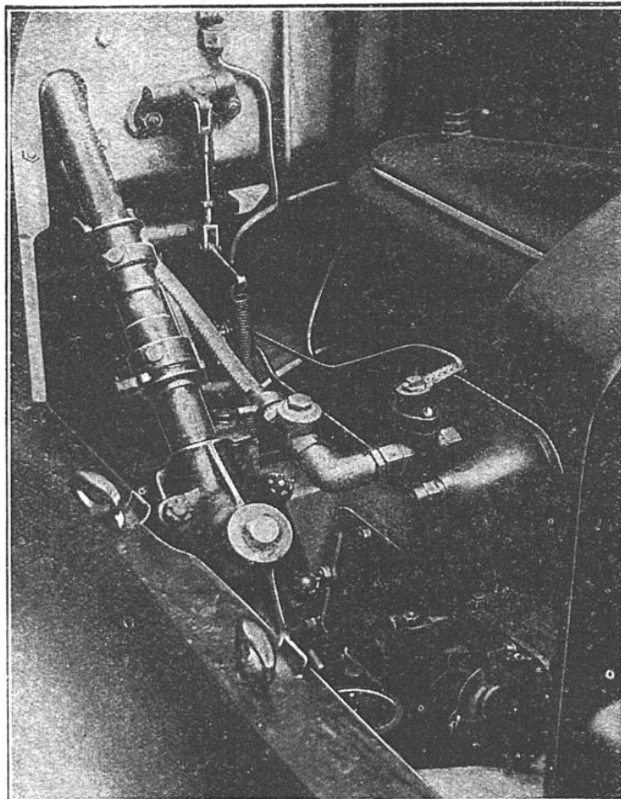
COMMENT LA CANALISATION DE GAZ ABOUTIT AU MOTEUR DE LA VOITURE LYON-SPENCER
