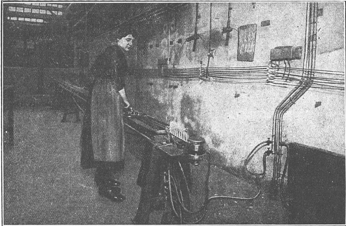
PREMIER ÉTIRAGE AU BANC DU FIL PROVENANT DU MARTELAGE
