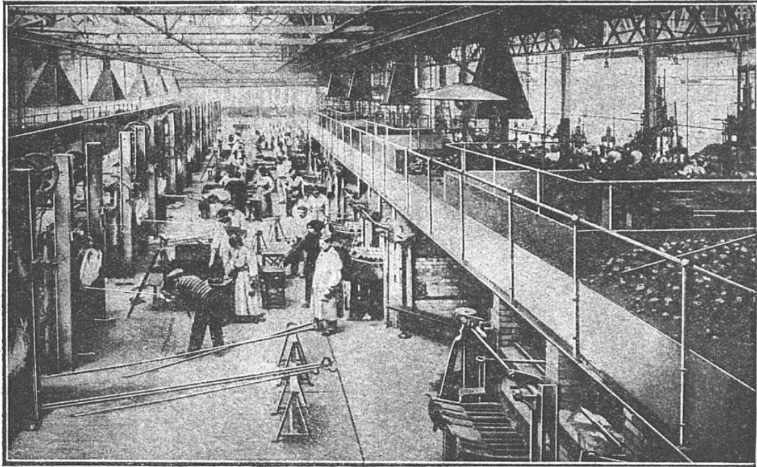
VUE GÉNÉRALE DU HALL DES FOURS SERVANT AUX TRAITEMENTS THERMIQUES
