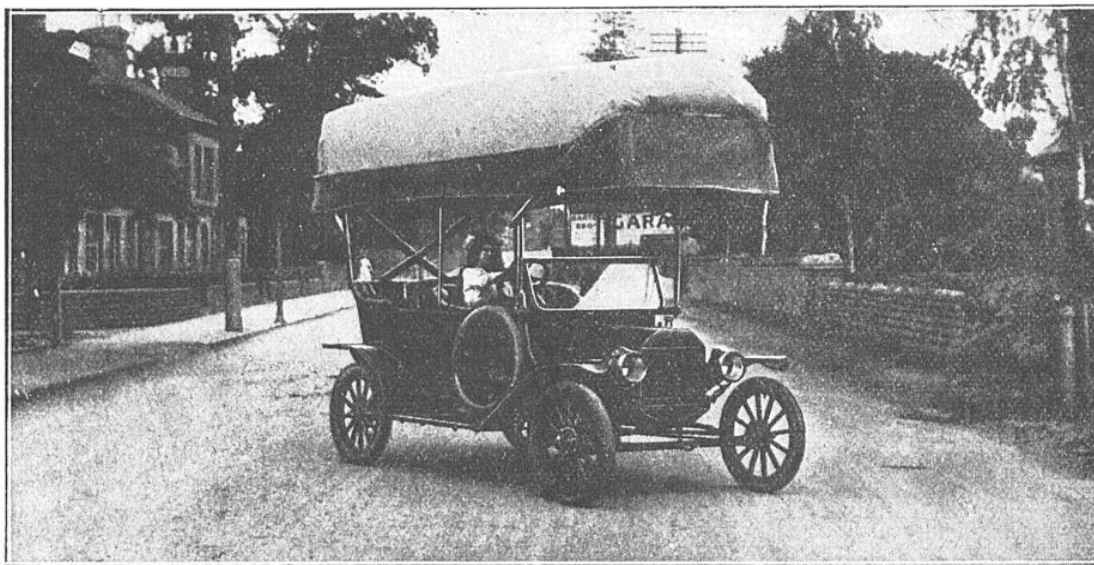
DISPOSITION D'UNE ENVELOPPE A GAZ SUR UNE VOITURETTE AUTOMOBILE
