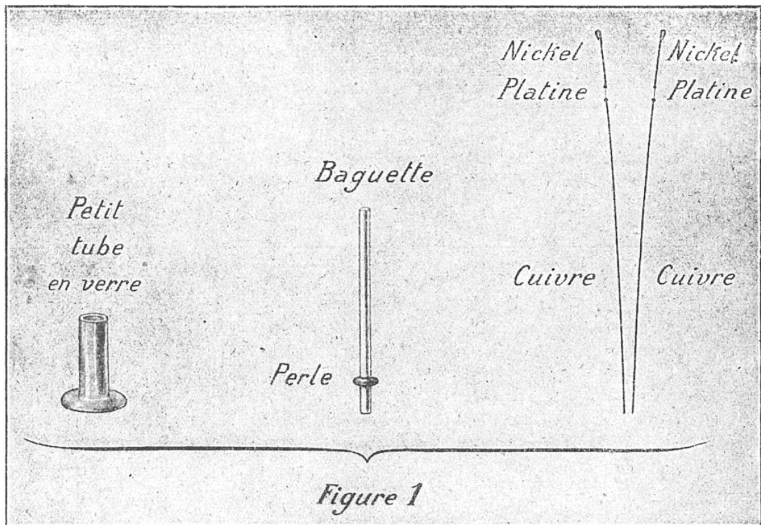
LES ÉLÉMENTS QUI ENTRENT DANS LA CONFECTION DU « PIED » D'UNE LAMPE « Z »
