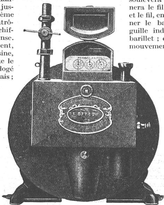
ASPECT EXTÉRIEUR D'UN COMPTEUR HYDRAULIQUE A GAZ ORDINAIRE
