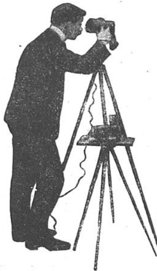
DÉTERMINATION DE LA TEMPÉRA- TURE DE CUISSON DANS UN FOUR CÉRAMIQUE AU MOYEN D'UN TÉLESCOPE PYROMÉTRIQUE, TYPE INDUSTRIEL
