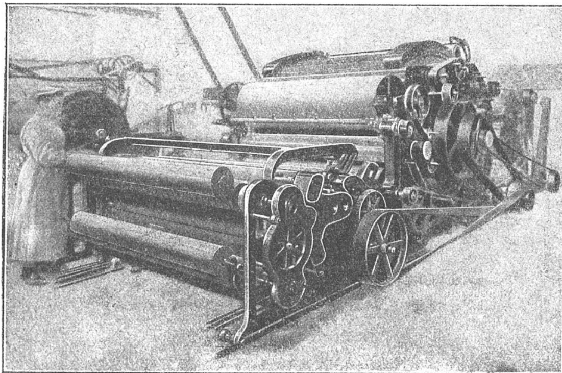
MACHINE CONSTRUITE SPÉCIALEMENT POUR CARDER LES FIBRES D'AMIANTE
