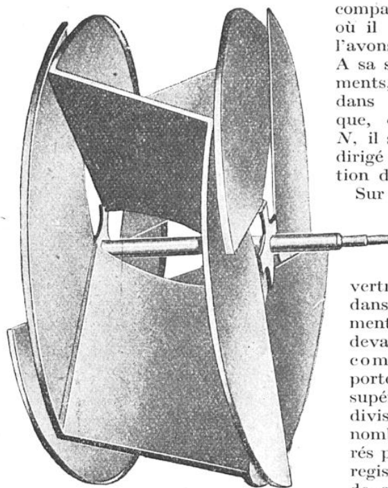
VOLANT MESUREUR D'UN COMPTEUR ORDINAIRE
