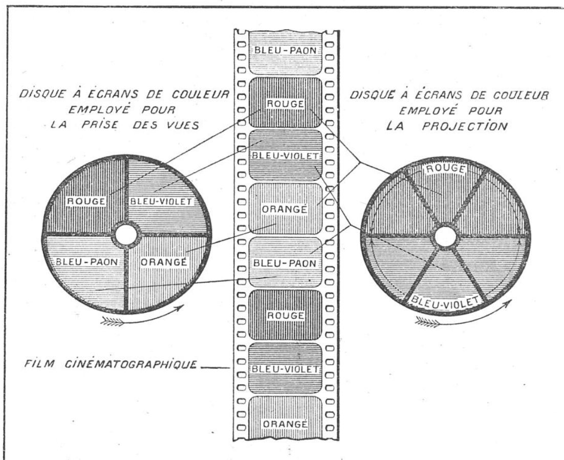
SCHÉMA MONTRANT LES RELATIONS EXISTANT ENTRE LES IMAGES DU FILM ET LES ÉCRANS DE COULEUR À TRAVERS LESQUELS ELLES SONT ENREGISTRÉES OU PROJETÉES
