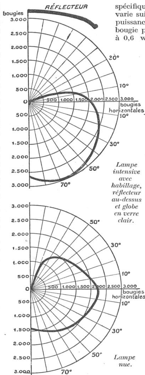
RÉPARTITION DE LA LUMIÈRE DANS LA LAMPE INTENSIVE « NITRA » DITE « DEMI-WATT », A ATMOSPHERE GAZEUSE, AVEC ET SANS RÉFLECTEUR
