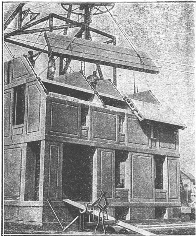
LA MISE EN PLACE DE LA TOITURE, EN LARGES PANNEAUX DE CIMENT ARMÉ
