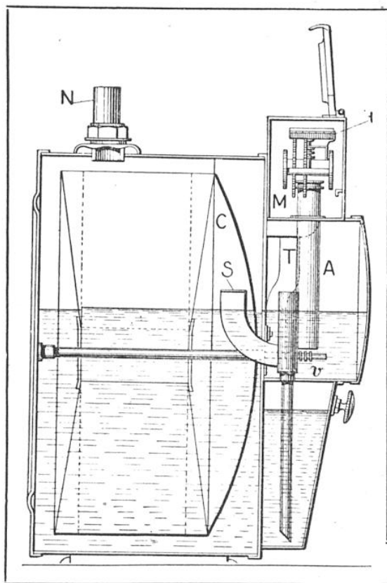
COUPE D'UN COMPTEUR ORDINAIRE
