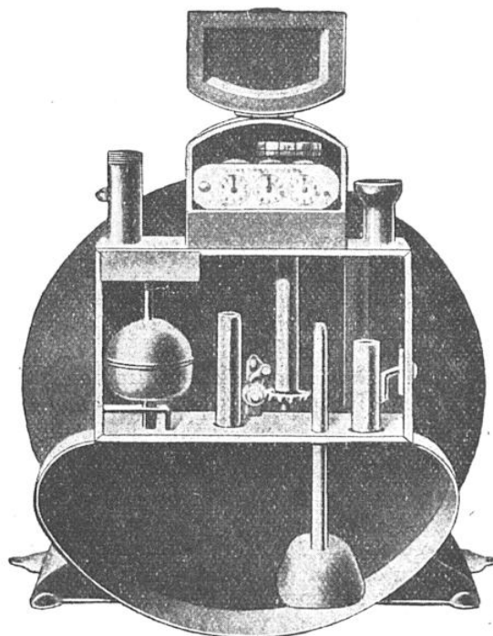
ASPECT INTÉRIEUR D'UN COMPTEUR ORDINAIRE MUNI DU COMPENSATEUR A INJECTEUR IMAGINÉ PAR M. DUPOY
