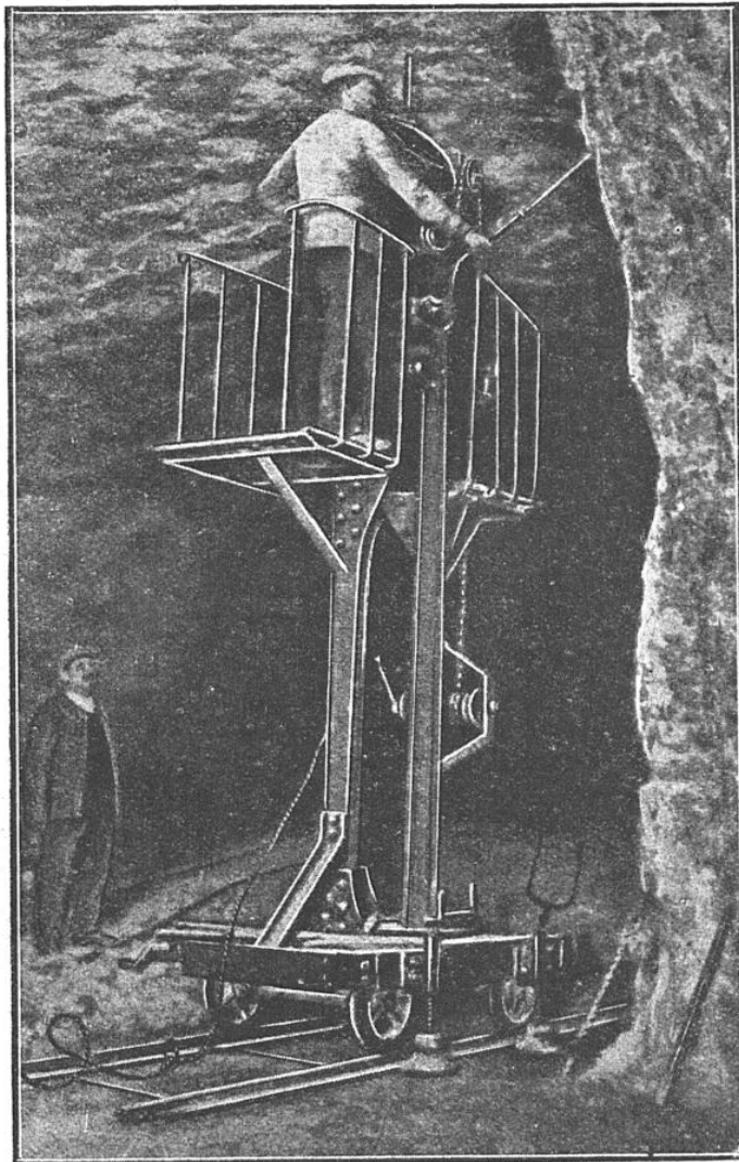
EXTRACTION DU SEL GEMME AU MOYEN D'UNE PERFORATRICE ÉLECTRIQUE
