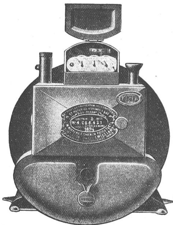
VUE DE FACE D'UN COMPTEUR ORDINAIRE TRANSFORMÉ EN COMPTEUR A MESURAGE EXACT AVEC COMPENSATEUR DE NIVEAU
