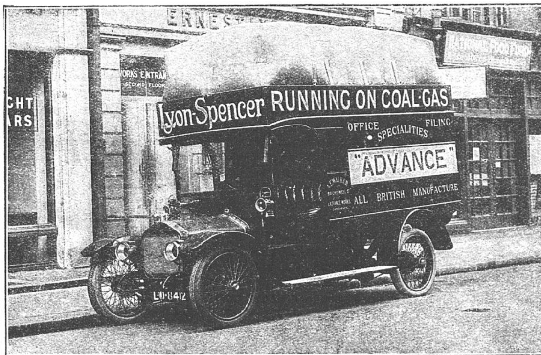
L'ENVELOPPE COMPLÈTEMENT GONFLÉE SUR UNE VOITURE DE LIVRAISON Le véhicule peut rouler facilement pendant 20 kilomètres sans avoir besoin d'être ravitaillé en gaz.
