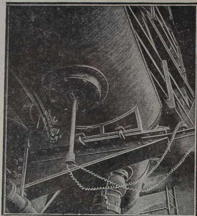
CONDUITE DE SOUFFLERIE D'UN HAUT FOURNEAU AVEC THERMO-ÉLÉMENT DANS SON TUBE PROTECTEUR
