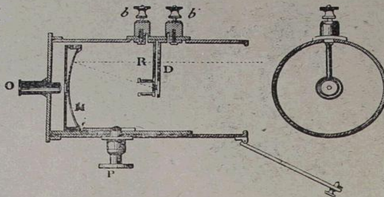
COUPE SCHÉMATIQUE D'UN PYROMÈTRE DU TYPE DIT INDUSTRIEL
