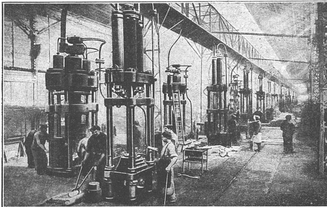
ATELIER D'EMBOUTISSAGE DES CORPS D'OBUS A LA PRESSE HYDRAULIQUE
