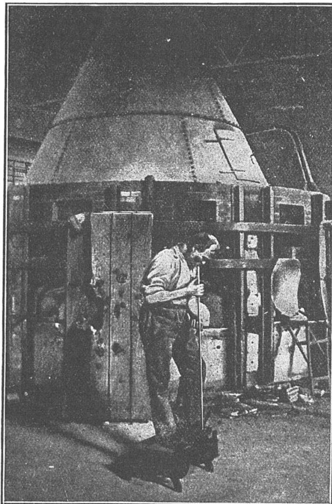
SOUFFLAGE D'UNE AMPOULE DE LAMPE « MÉTAL »
