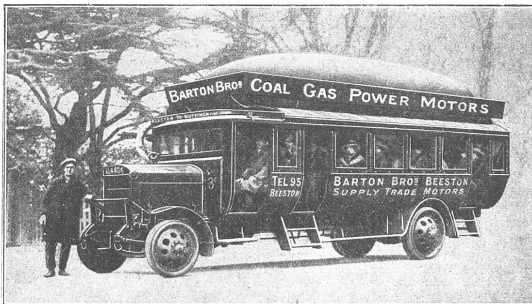
SUR CET AUTOBUS, LE GAZ A AVANTAGEUSEMENT REMPLACÉ L'ESSENCE
