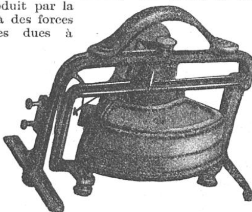
GALVANOMÈTRE SENSIBLE A SUSPENSION
