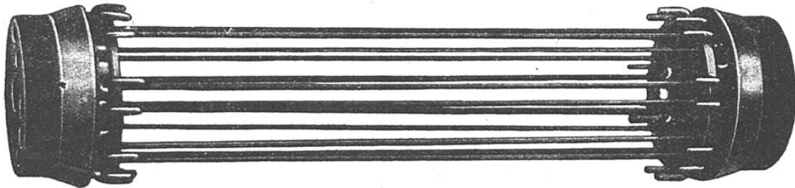
LES TRINGLES D'ACIER ASSURANT LA RÉSISTANCE AXIALE DU TUBE MURPHY
