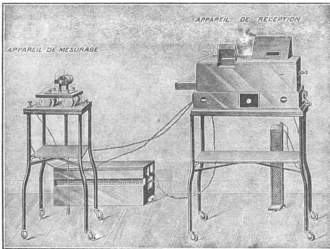
FIG. 4. — VUE D'ENSEMBLE DE L'ÉLECTROCARDIOGRAPHE A BOBINE
