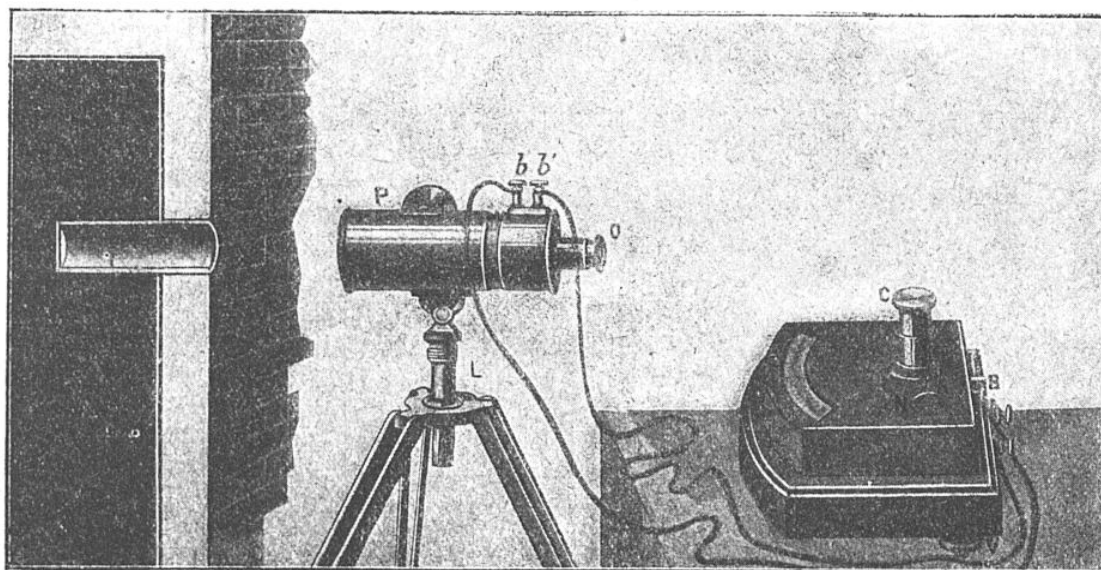
INSTALLATION D'UNE LUNETTE PYROMÉTRIQUE AVEC GALVANOMÈTRE
