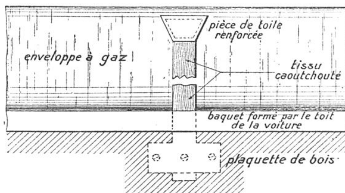
DISPOSITIF POUR ASSURER L'AFFAISSEMENT DE L'ENVE- LOPPE AU MOMENT DU DÉGONFLEMENT
