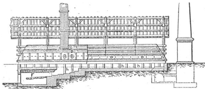
INSTALLATION D'UNE POÊLE SERVANT A CONCENTRER LES SOLUTIONS SALINES
