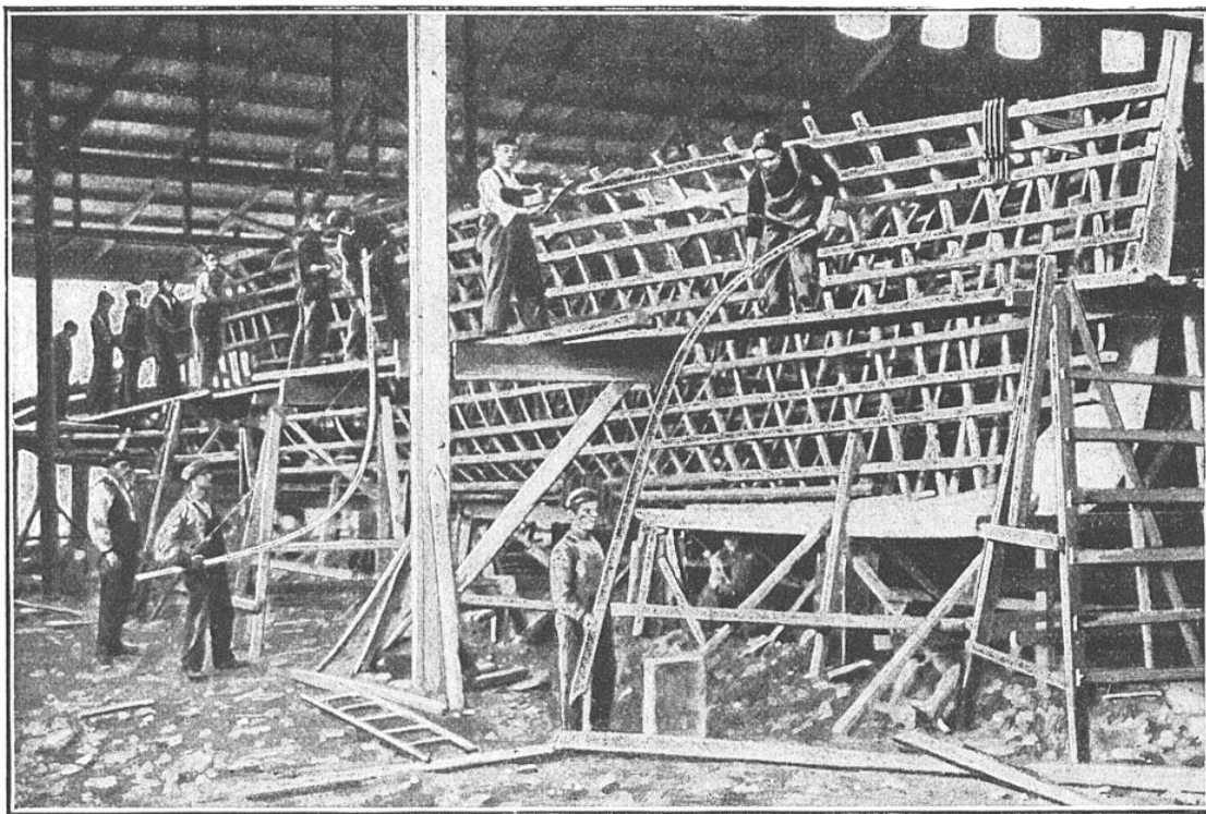
MONTAGE DE LA CARÈNE D'UN « CHASSEUR » DANS UN CHANTIER CANADIEN
