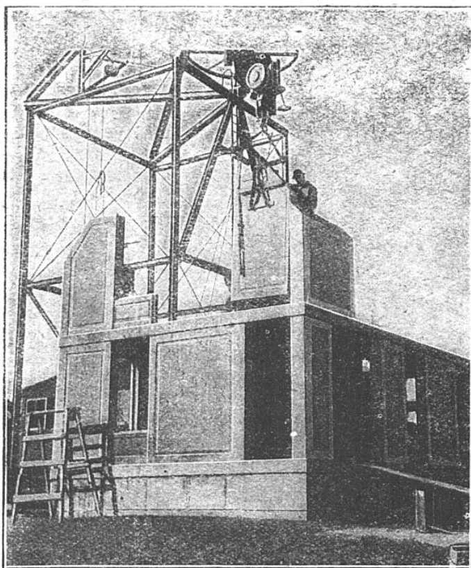
LE REZ-DE-CHAUSSÉE TERMINÉ, ON PROCÈDE AVEC DILIGENCE AU MONTAGE DU PREMIER ÉTAGE
