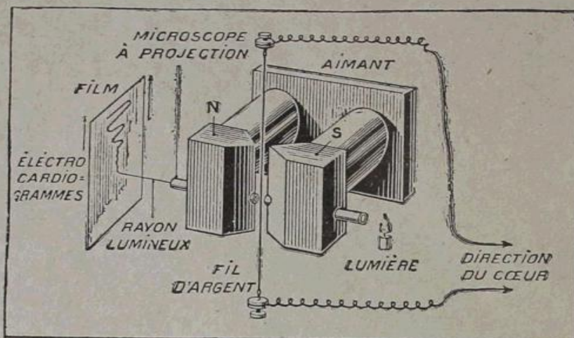
FIG. 2. — SCHÉMA DU GALVANOMÈTRE À CORDE DE EINTHOVEN ET SON UTILISATION POUR LA REPRODUCTION DES COURANTS DU CŒUR
