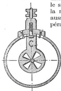
COUPE D'UNE LUNETTE PYROMÉTRIQUE INDUSTRIELLE CH. FÉRY
