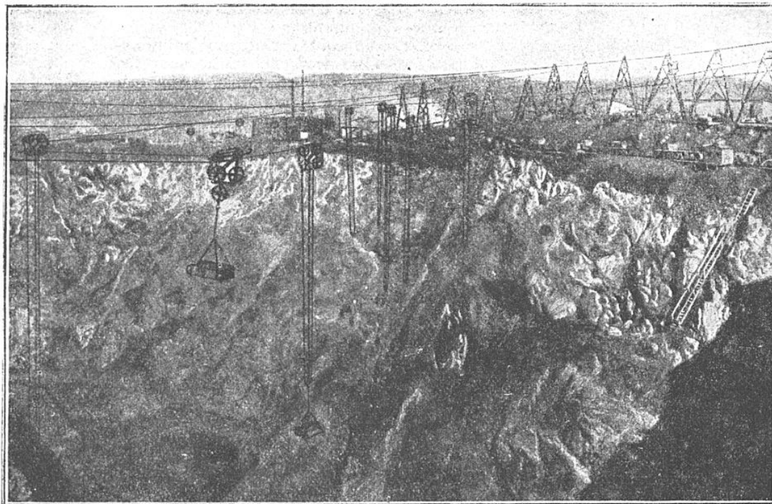
INSTALLATIONS MÉCANIQUES POUR L'EXPLOITATION D'UNE MINE D'AMIANTE
