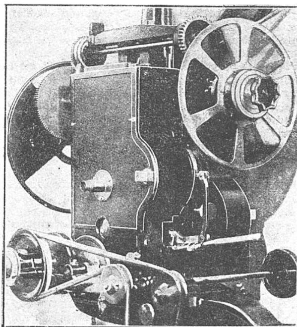
LE DISQUE A ÉCRANS COLORÉS MONTÉ SUR L'APPAREIL DE PROJECTION
