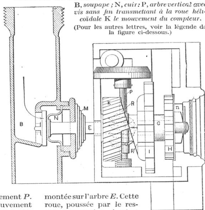
COUPE DE LA SOUPAPE DU « COMPTEUR A SOUS »
