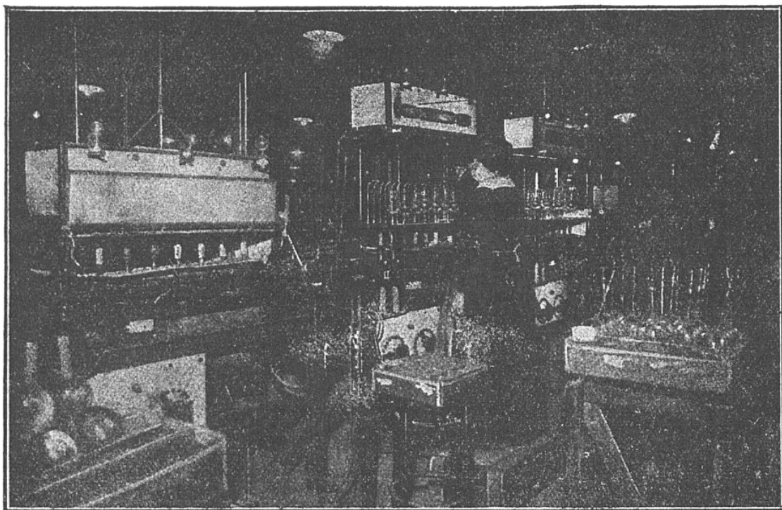
LAMPES MONTÉES PAR LEUR QUEUSOT SUR LE TUBE COLLECTEUR DE LA MACHINE A FAIRE LE VIDE, DANS DES FOURS AMOVIBLES EN TOLE
