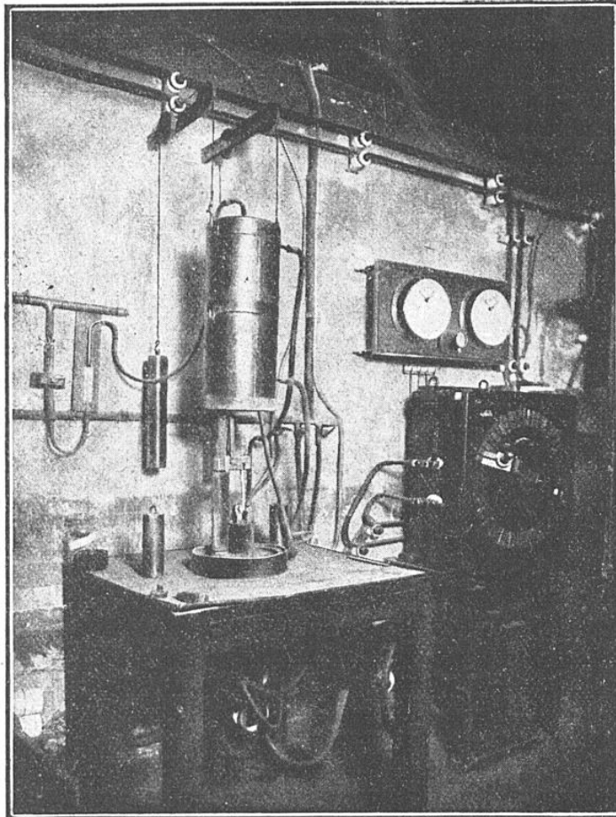
FOUR OUVERT, AVEC SES TUYAUX D'AMENÉE DU GAZ ET DE L'EAU, SES CABLES CONDUCTEURS DU COURANT ÉLECTRIQUE ET SES CONTREPOIDS
