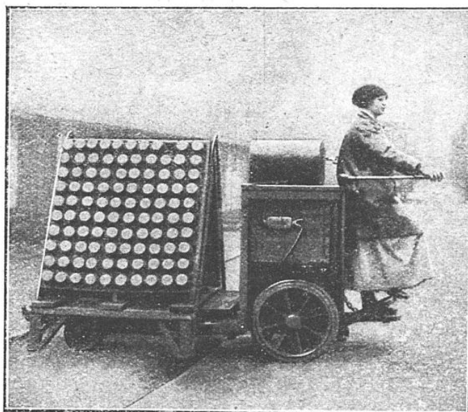
VUE LATÉRALE D'UN TRANSPORTEUR ÉLECTRIQUE
