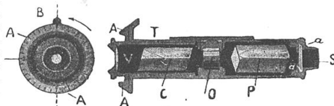
COUPE DU TUBE OPTIQUE D'UNE LUNETTE PYROMÉTRIQUE DE MM. MESURÉ ET NOUËL
