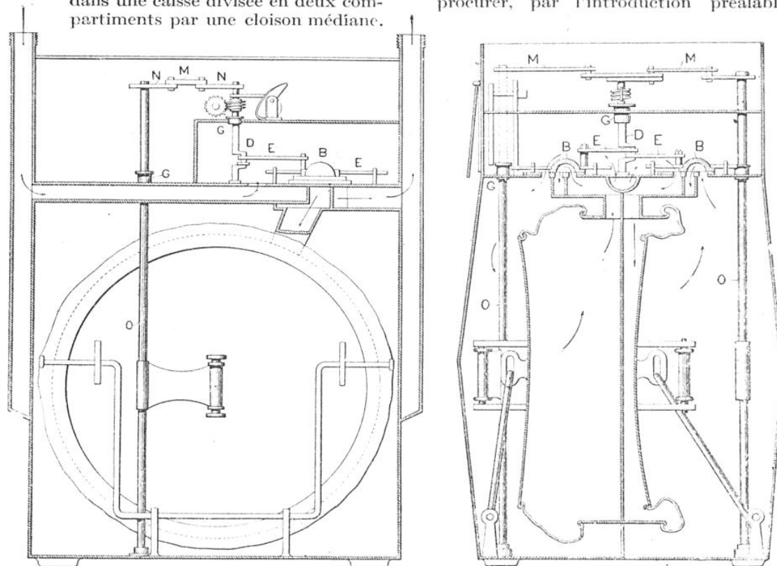
COUPES DU COMPTEUR SEC EMPLOYÉ DANS LES PAYS FROIDS
