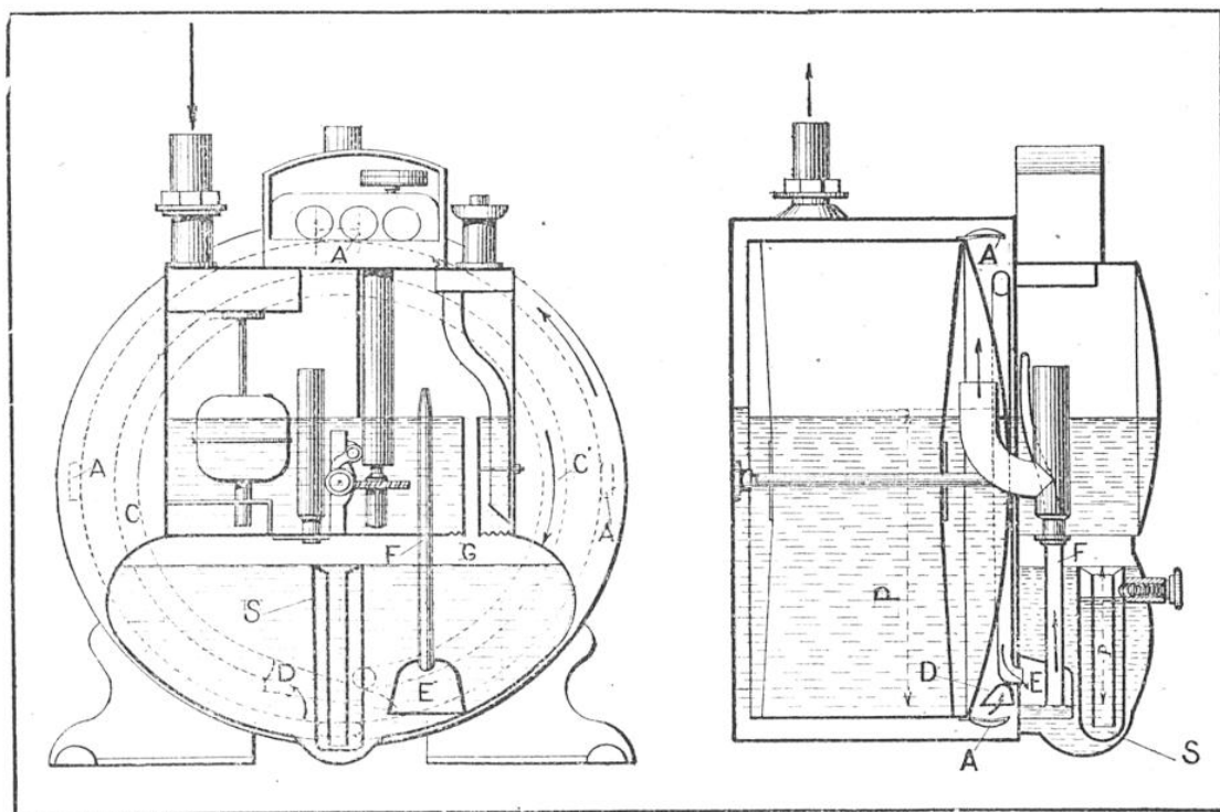
SCHEMA DU COMPENSATEUR DE NIVEAU A INJECTEUR, SYSTEME DUFOY
