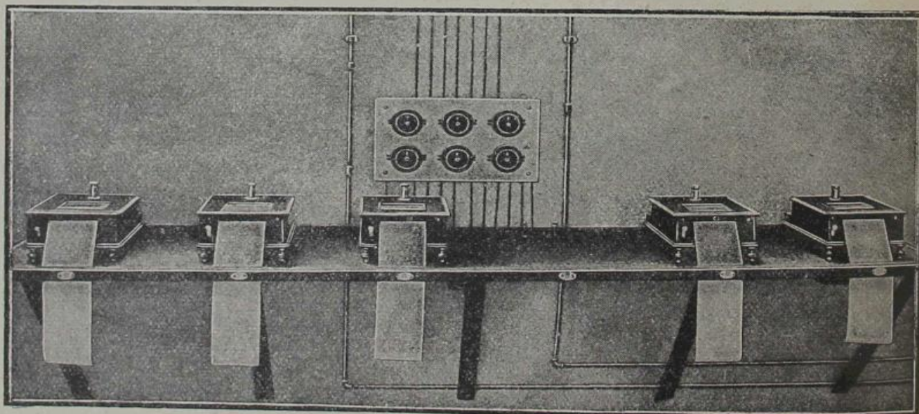
DISPOSITION DES APPAREILS ENREGISTREURS DES TEMPÉRATURES DE L'AIR CHAUD D'UNE BATTERIE DE CINQ HAUTS FOURNEAUX
