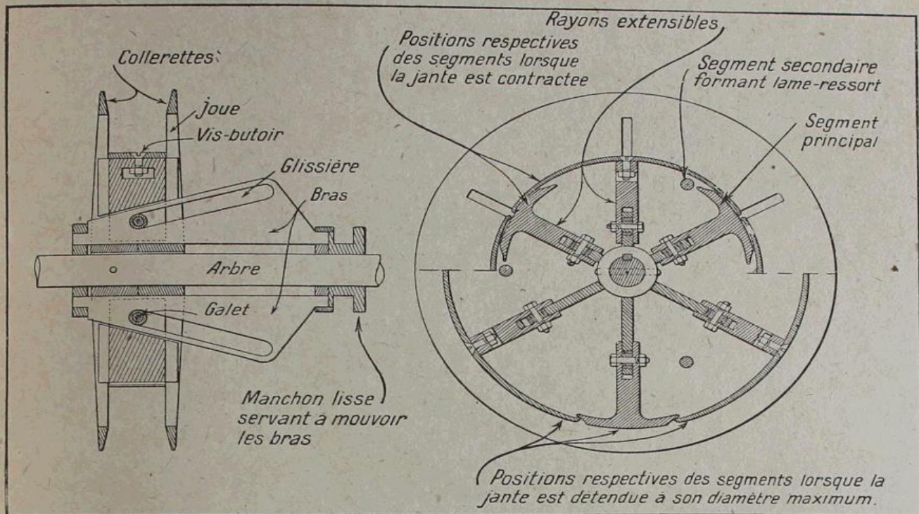
SCHÉMA MONTRANT LES DÉTAILS DE CONSTRUCTION DE LA POULIE EXTENSIBLE
