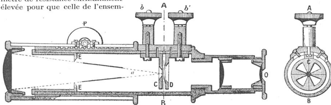
COUPE D'UNE LUNETTE PYROMÉTRIQUE AVEC OBJECTIF EN FLUORINE
