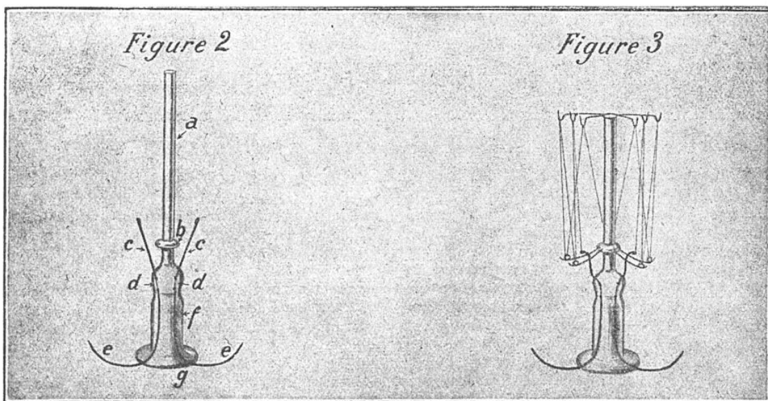
PIED TERMINÉ (FIG. 2) ET FILAMENT MONTÉ SUR SES SUPPORTS (FIG 3).
