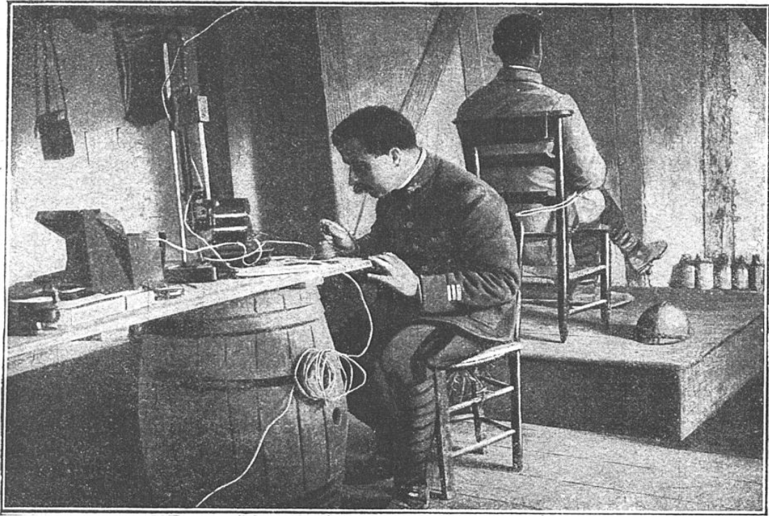
CHRONOSCOPE LAHY POUR LA MESURE DES TEMPS DE RÉACTION DES MITRAILLEURS Cette photo montre les positions respectives de l'opérateur et du sujet pendant les expériences.
