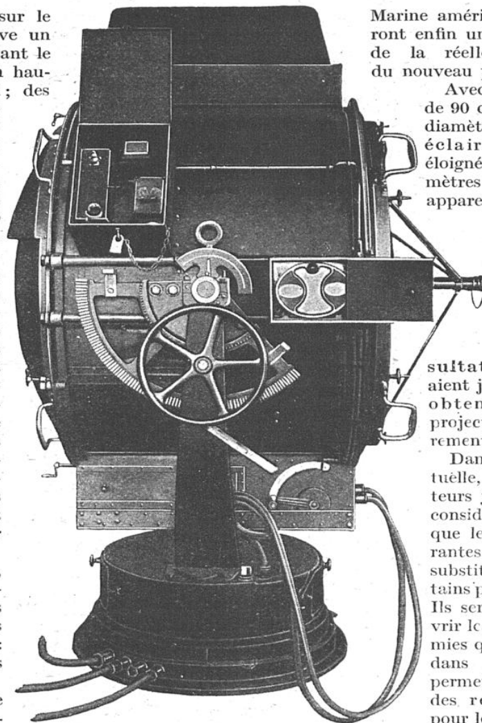
LE PROJECTEUR SPERRY DERNIER MODÈLE
