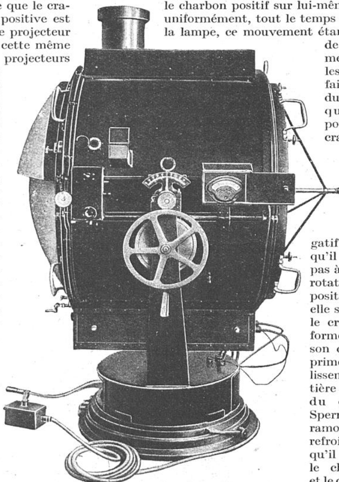
QUELQUES DÉTAILS EXTÉRIEURS DE LA CAGE DU PROJECTEUR SPERRY
