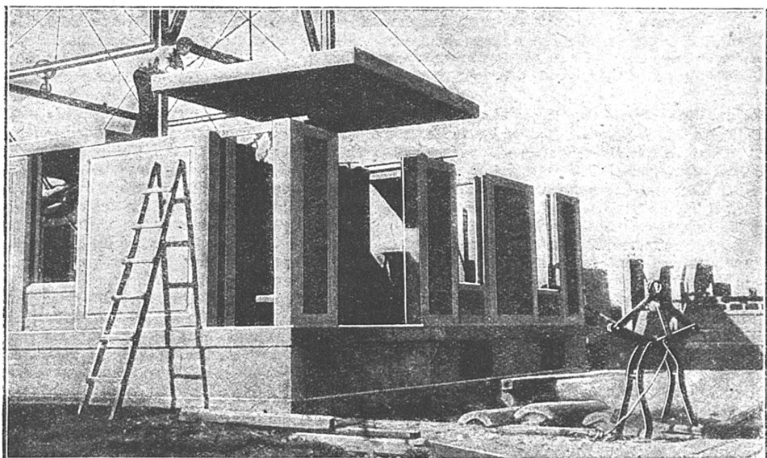
LA POSE DU PLANCHER EST AUSSI SIMPLE QUE LE MONTAGE DES MURAILLES Le plancher est également fait de larges panneaux de ciment que l'on dispose horizontalement.
