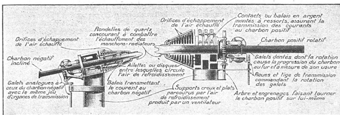
COUPE DES MANCHONS-RADIATEURS ENTOURANT LES ÉLECTRODES DANS UN PROJECTEUR SPERRY, AVEC LE DESSIN DES ORGANES DE TRANSMISSION ET DE TRANSPORT DU COURANT
