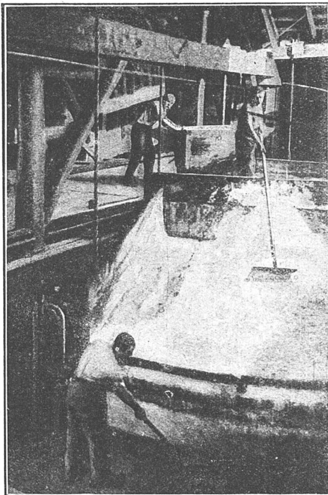
INTÉRIEUR D'UNE RAFFINERIE DE SEL
