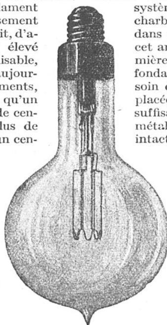
LAMPE « MÉTAL », DITE DEMI-WATT, A ATMOSPHÈRE GAZEUSE
