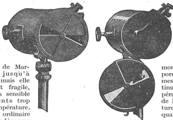
VUE EXTÉRIEURE D'UN TÉLESCOPE A DIAPHRAGME BASCULANT
