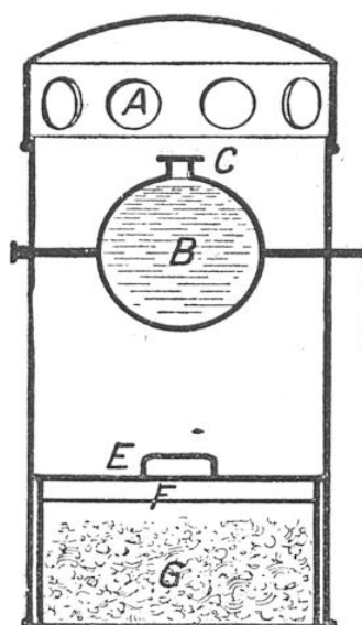
« NEBEL-TOPF » (Coupe verticale)
