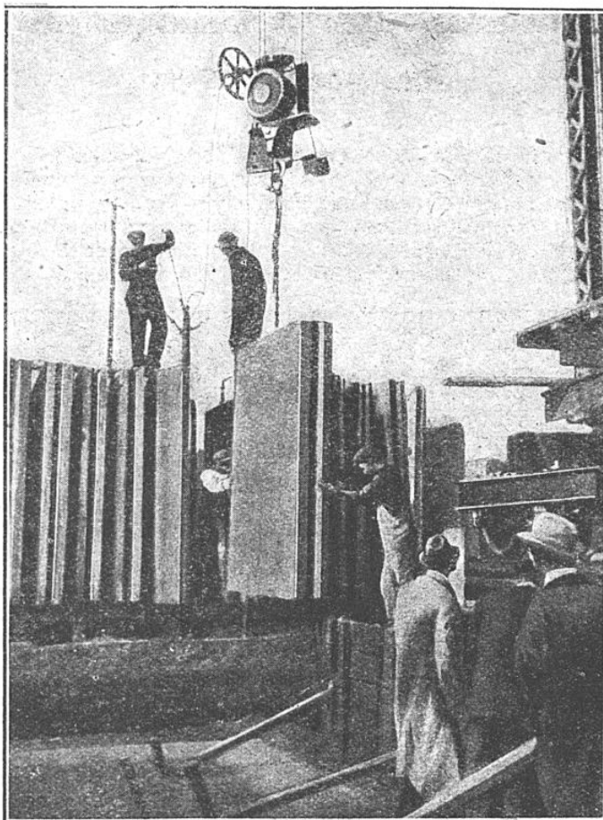
MISE EN STOCK DES PANNEAUX DE CIMENT
