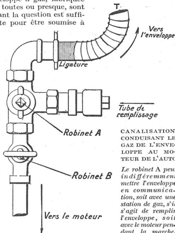
Dans ce dernier cas, on ouvre également le robinet B. Ce dispositif est généralement placé devant le conducteur, sur l'un des côtés du tablier de la voiture.
