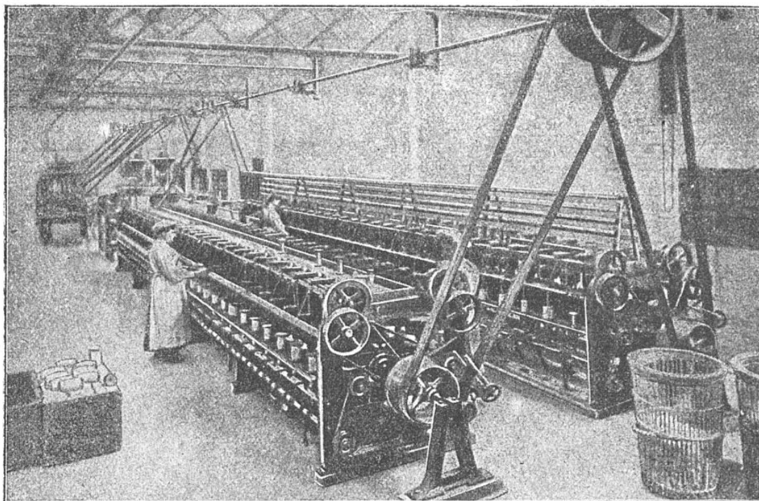
A L'AIDE DE CETTE MACHINE, L'AMIANTE SE FILE COMME LE CHANVRE
