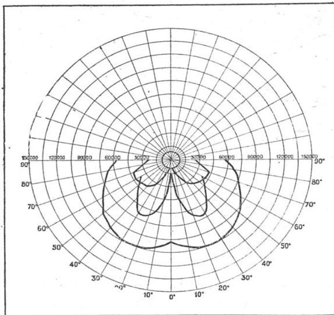
COMPARAISON DES COURBES D'INTENSITÉ LUMINEUSE DE DEUX PROJECTEURS ORDINAIRES ET D'UN PROJECTEUR SPERRY
