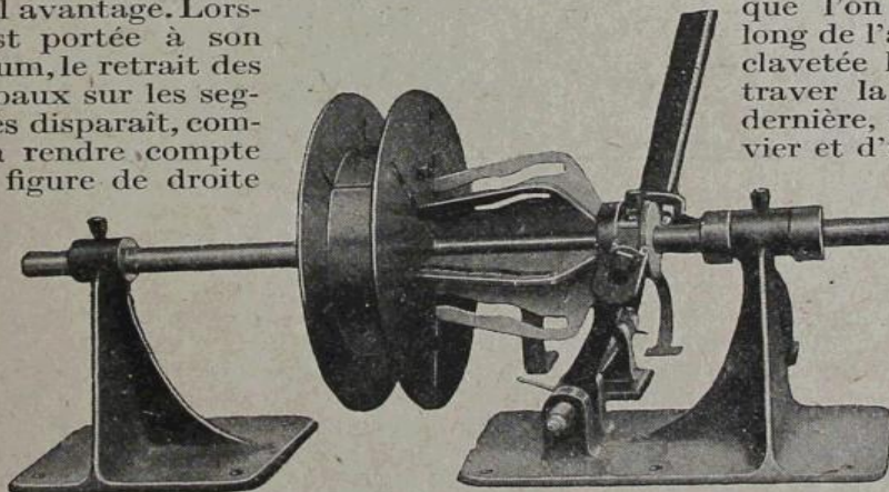
LA POULIE DUNBAR CONTRACTÉE A SON MINIMUM DE DIAMÈTRE
