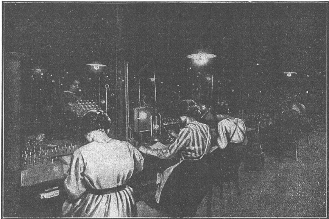
LE MONTAGE DU FILAMENT MÉTALLIQUE SUR LES SUPPORTS DU PIED
