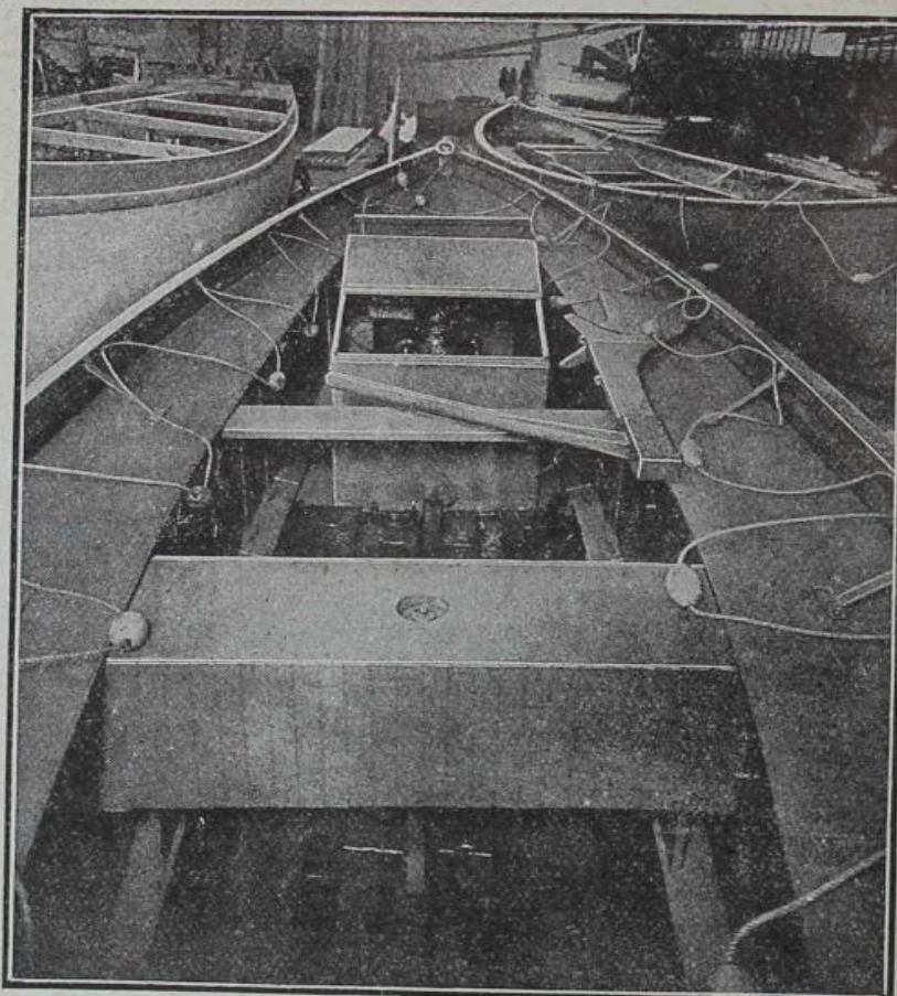
VUE INTÉRIEURE MONTRANT LES DISPOSITIFS DESTINÉS A ASSURER L'INSUBMERSIBILITÉ
