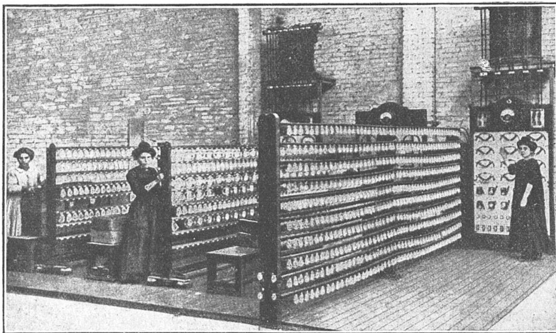
LES LAMPES A INCANDESCENCE DISPOSÉES SUR LES RAMPES D'ESSAI
