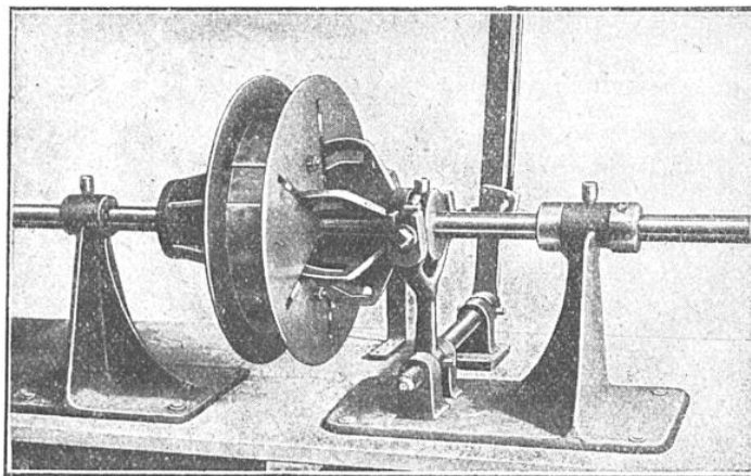
VUE DE LA POULIE EXTENSIBLE DE M. W.-B. DUNBAR
