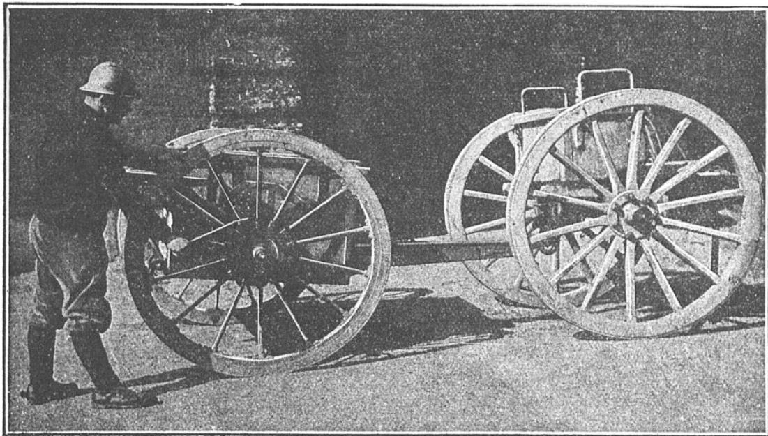
ADAPTATION D'UNE ROUE CONSTANCIA A UN CAISSON D'ARTILLERIE DE CAMPAGNE
