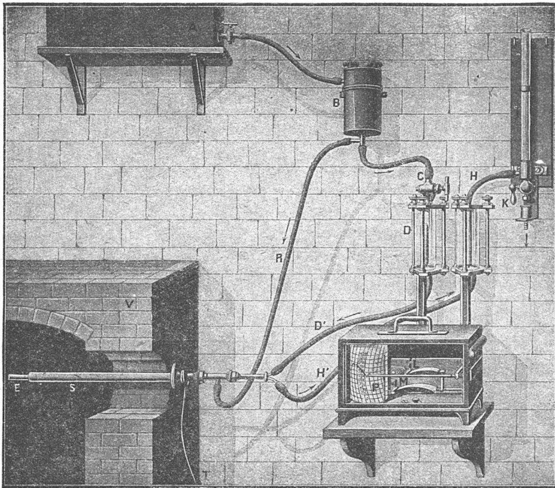
INSTALLATION D'UN PYROMÈTRE F. DE SAINTIGNON, A LA RAFFINERIE SAY
