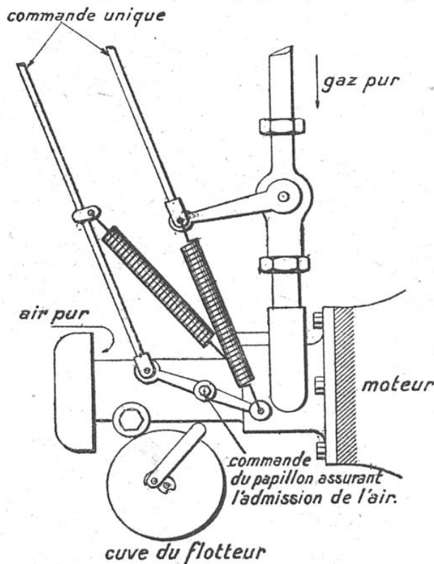
LA COMMANDE QUI ASSURE L'ARRIVÉE DU GAZ D'ÉCLAIRAGE AU CARBURATEUR
