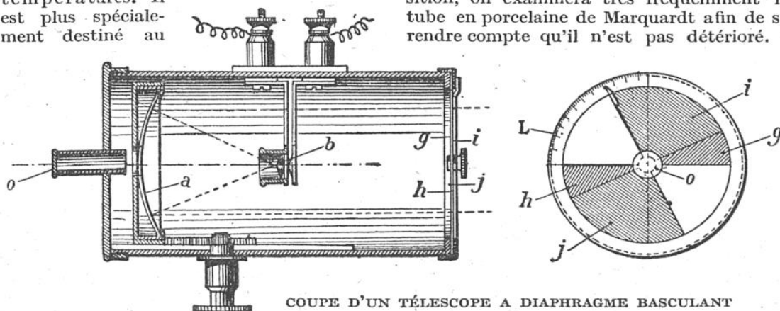
COUPE D'UN TÉLESCOPE A DIAPHRAGME BASCULANT
