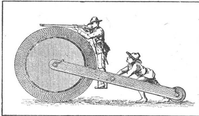
LE ROULEAU-BOUCLIER, ÉLÉVATION LATÉRALE
