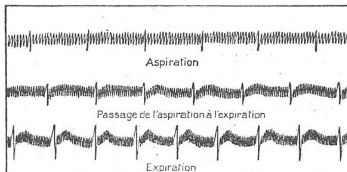
FIG. 9. — INFLUENCE DE LA RESPIRATION SUR L'ACTIVITÉ DU CŒUR, RÉVÉLÉE PAR L'ÉLECTROCARDIOGRAMME
