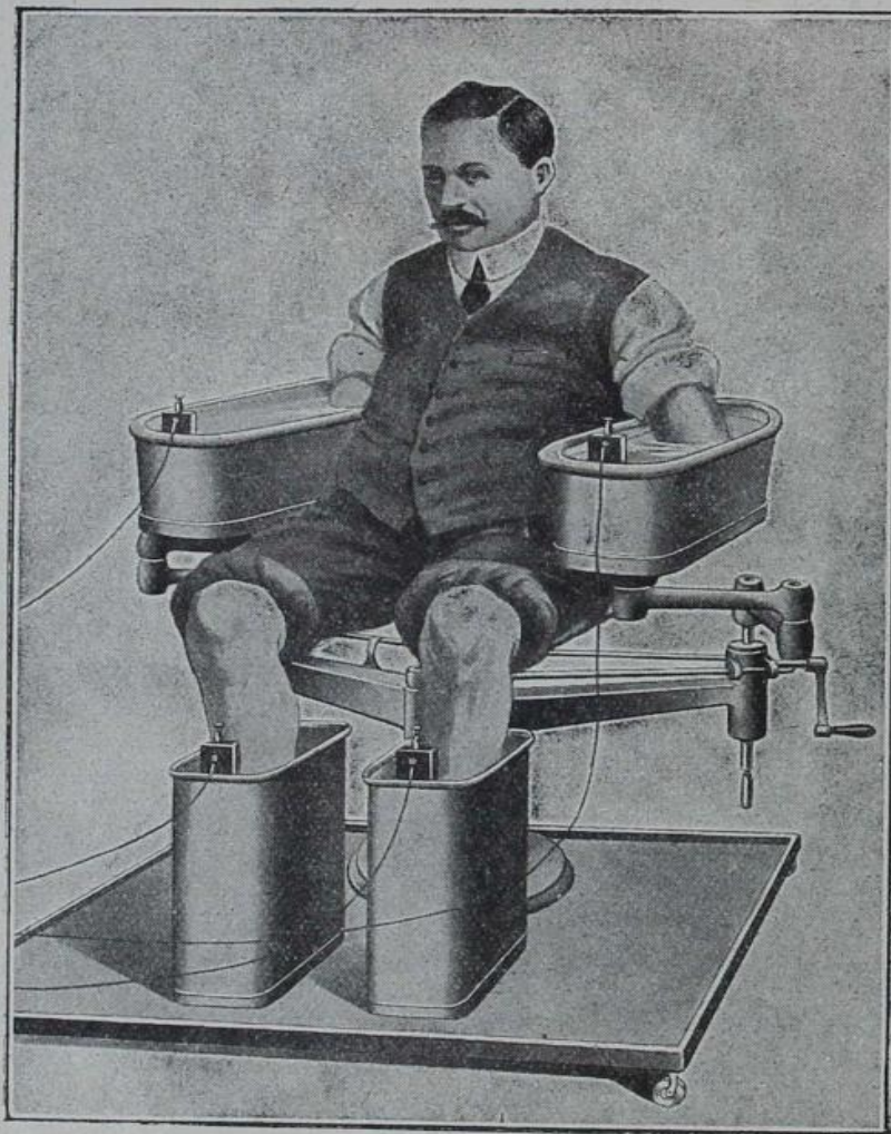
FIG. 6. — BAIN A QUATRE CELLULES AVEC L'AIDE DESQUELLES SE FAIT LA CONDUITE DES COURANTS DU CŒUR EN PASSANT PAR LES BRAS ET LES PIEDS
