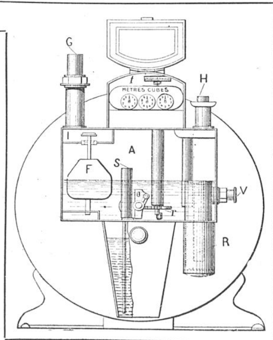
VUE DE FACE D'UN COMPTEUR ORDINAIRE
