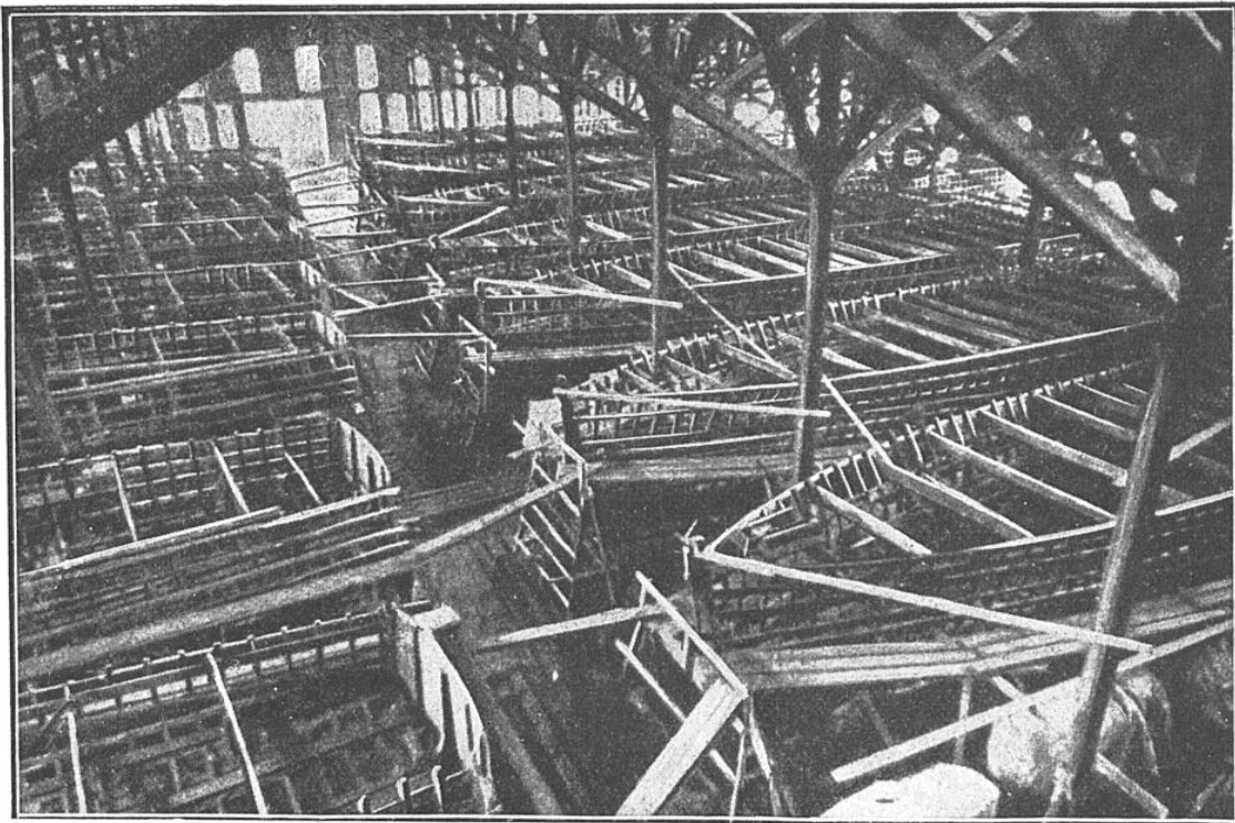
CINQUANTE NAVIRES SONT SIMULTANÉMENT CONSTRUITS SOUS CE HALL
