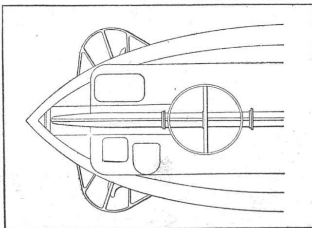
CRINOLINES DE PROTECTION DES HÉLICES
