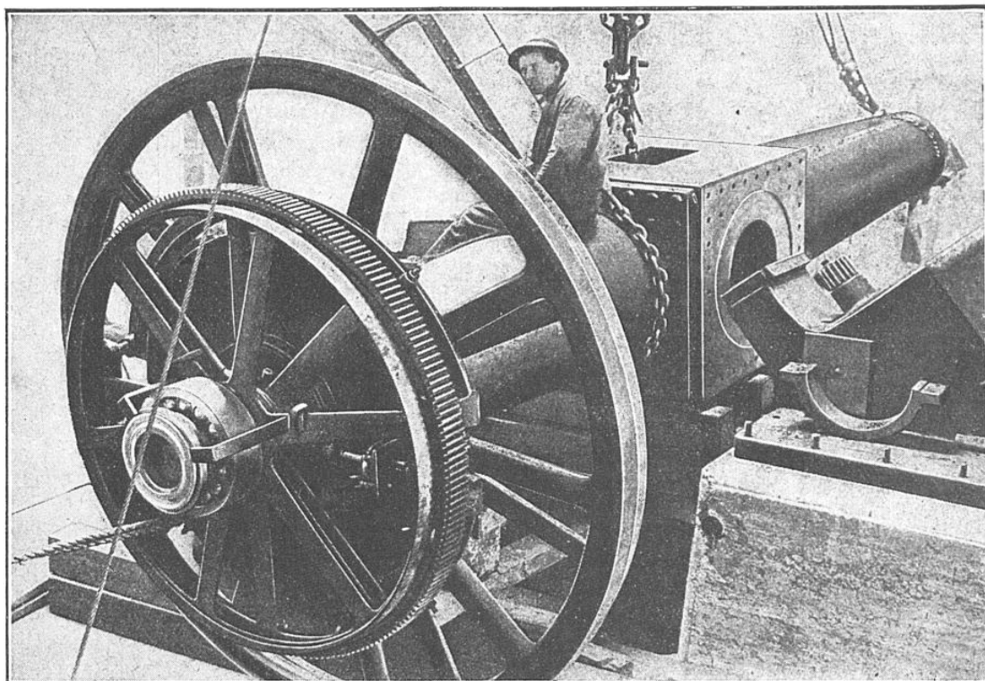
AXE DE DÉCLINAISON AVEC ENGRENAGE MOTEUR ET COUSSINET A BILLES
