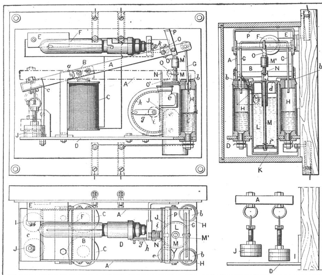
APPAREIL DE M. COURTOIS, MUNI D'UN FREIN A GLYCÉRINE (VUES DE FACE ET DE COTÉ, ET, AU-DESSOUS, COUPES PARTIELLES)
