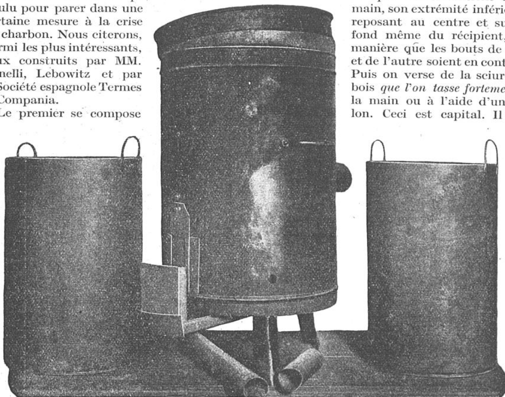
LE POÊLE A SCIURE DE BOIS, GRAND MODÈLE, SYSTÈME BENELLI
