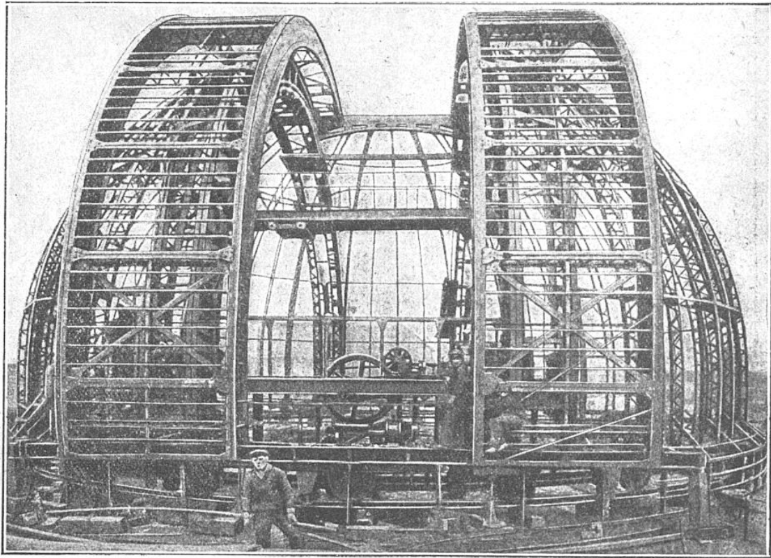
DOME MÉTALLIQUE DESTINÉ A ABRITER UN GRAND TÉLESCOPE
