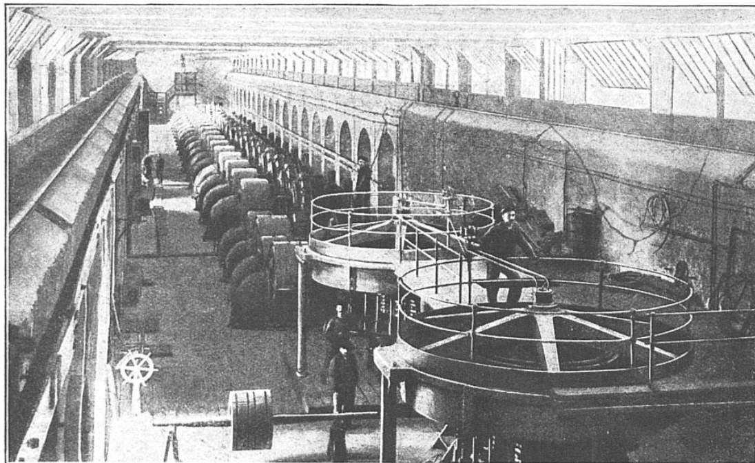
LA SALLE DES MACHINES DE L'USINE A ALUMINIUM DE LA PRAZ (SAVOIE)
