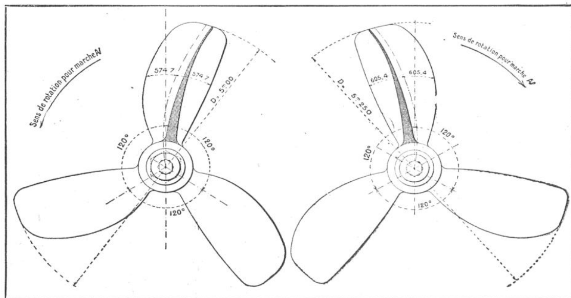
HÉLICES LATÉRALES A TROIS AILES DE L'ANCIEN CROISEUR CUIRASSÉ « LÉON-GAMBETTA »
