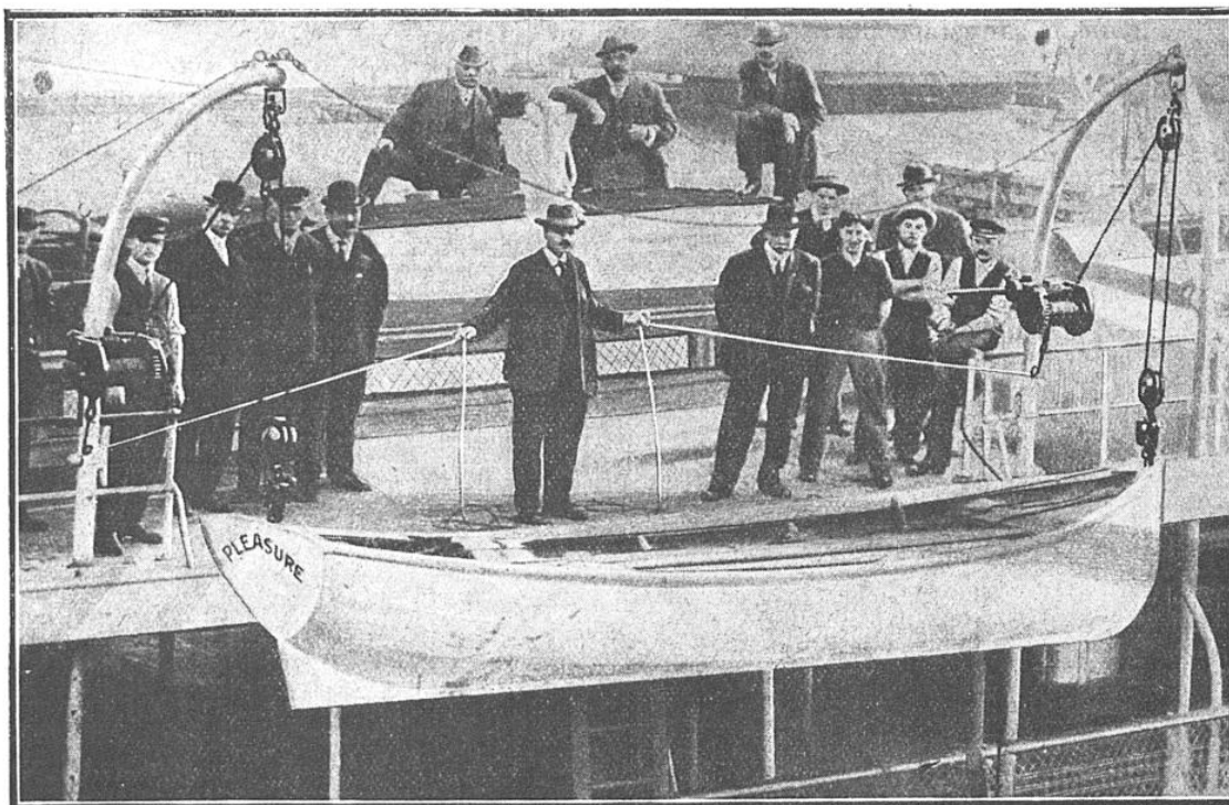
LA MANŒUVRE DE MISE À L'EAU D'UNE EMBARCATION DE SAUVÉTAGE
