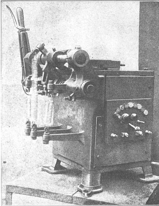
FIG. 5. — MACHINE A SOUDER ÉLECTRIQUEMENT LES ANNEAUX ET LES MAILLONS DES CHAINES
