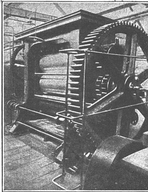
CALANDRE A TROIS CYLINDRES
