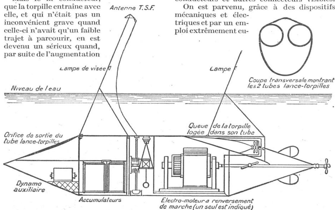
FIG. 1. — COUPE LONGITUDINALE DE L'AUTO-TORPILLEUR SOUS-MARIN
