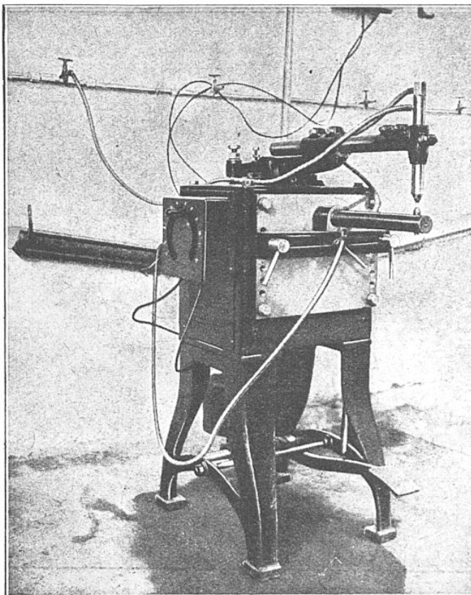
FIG. 7. — MACHINE CONSTRUITE POUR SOUDER ÉLECTRIQUEMENT PAR POINTS.
