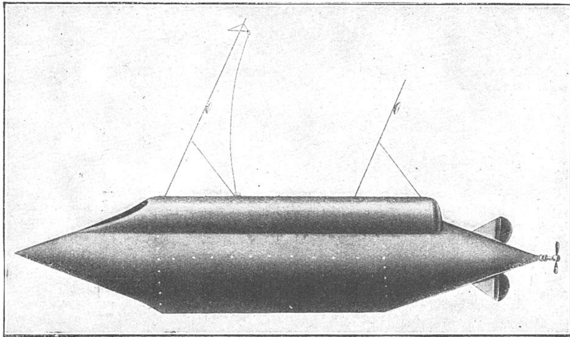
FIG. 3. — VUE GÉNÉRALE DE L'AUTO-PORTE-TORPILLES, AVEC SON ANTENNE Le renflement supérieur est l'un des tubes renfermant l'une des deux torpilles que porte l'engin.
