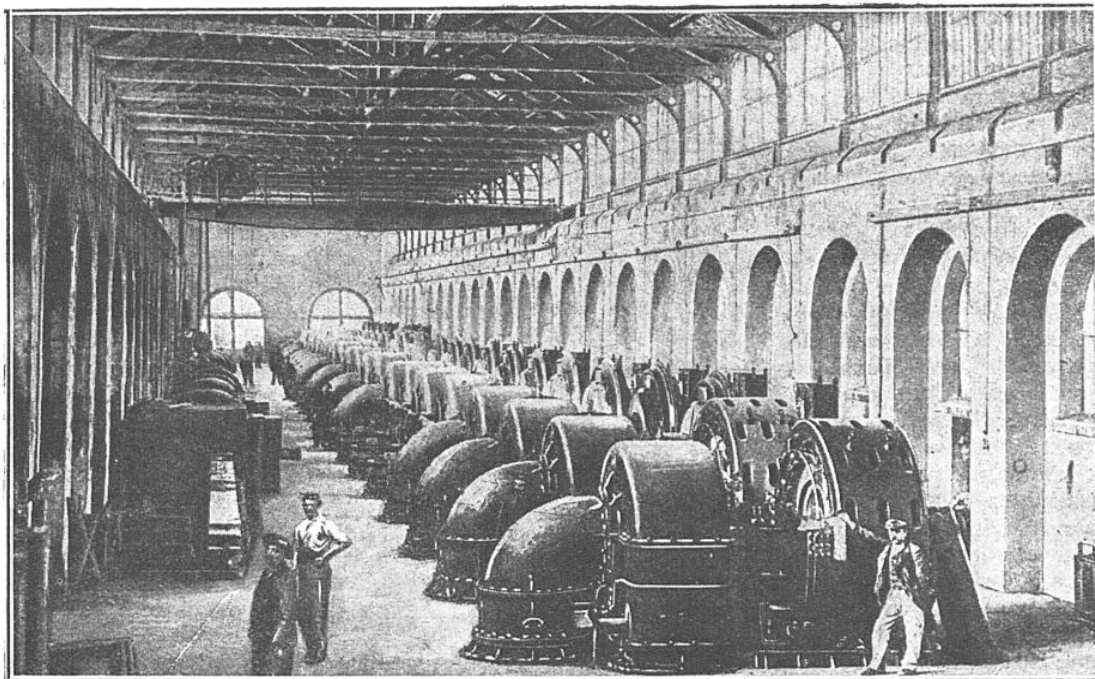
HALL DES TURBINES DE L'USINE A ALUMINIUM DE SAINT-MICHEL-DE-MAURIENNE
