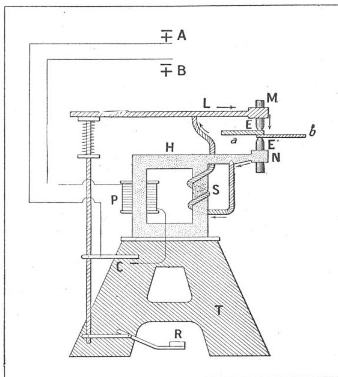
FIG. 3. — APPAREIL RÉALISANT LA SOUDURE ÉLECTRIQUE PAR COURT-CIRCUIT
