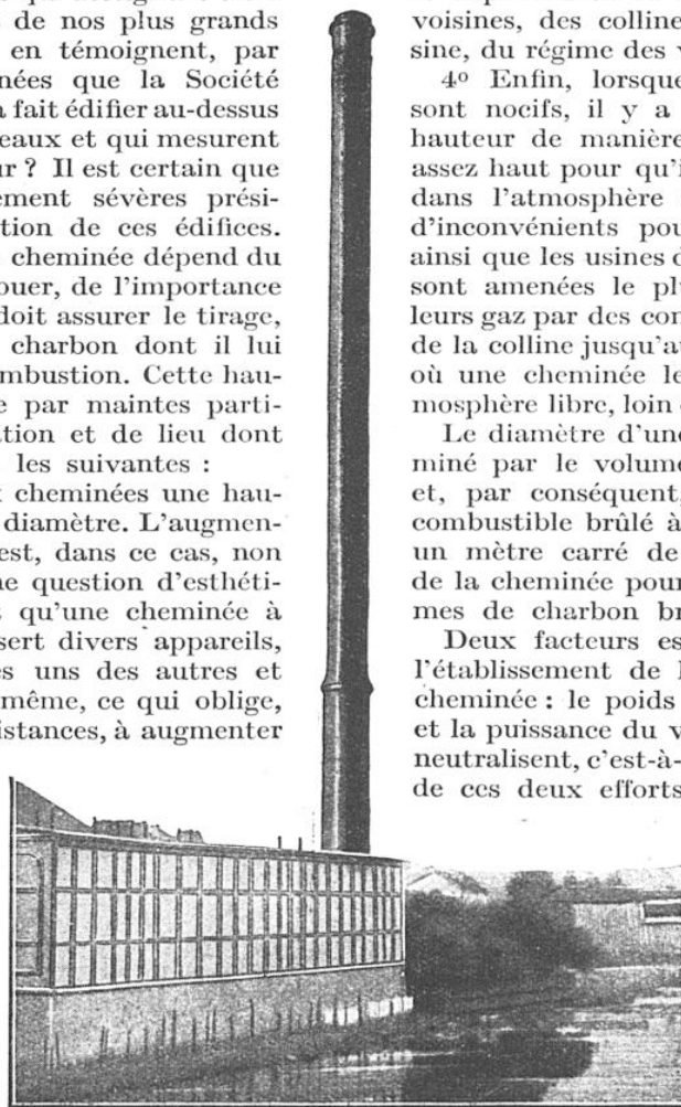
CHEMINÉE EN CIMENT ARMÉ, MONOLITHE
