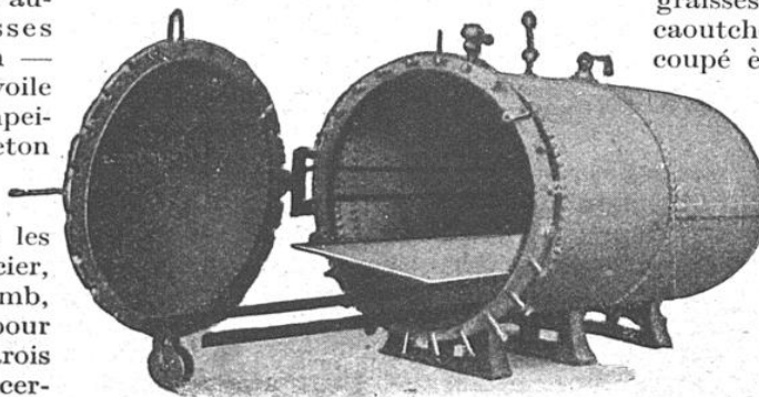
AUTOCLAVE HORIZONTAL EMPLOYÉ POUR LA VULCANISATION DU CAOUTCHOUC
