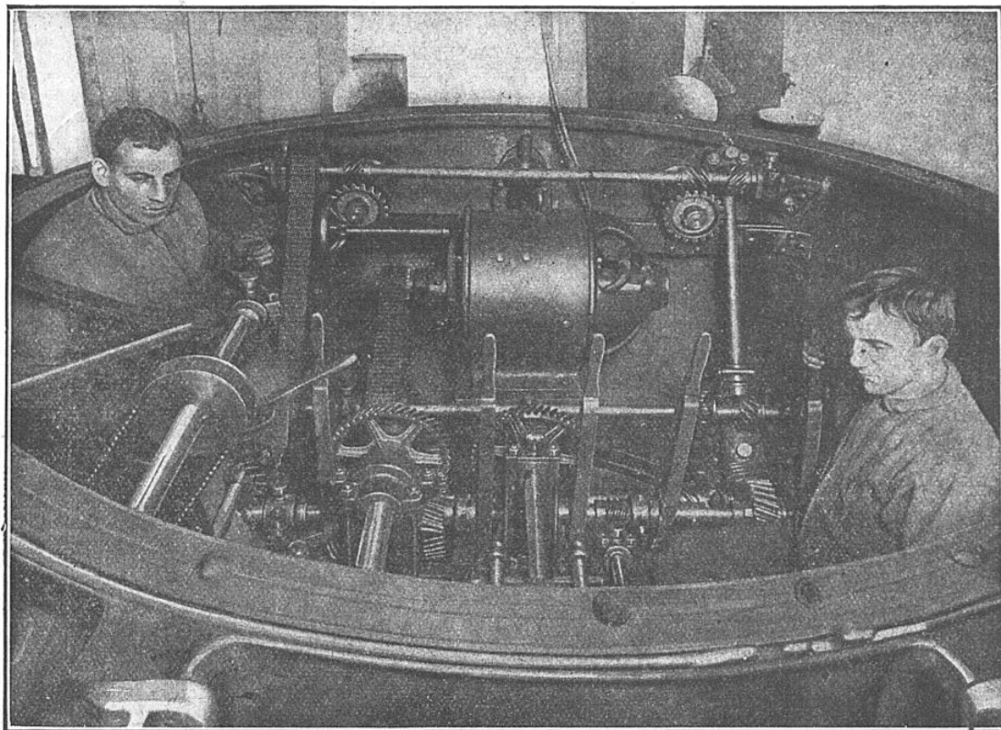
MACHINERIE INTÉRIEURE DU SOUS-MARIN DE RELEVAGE DE M. W. D. SISSON
