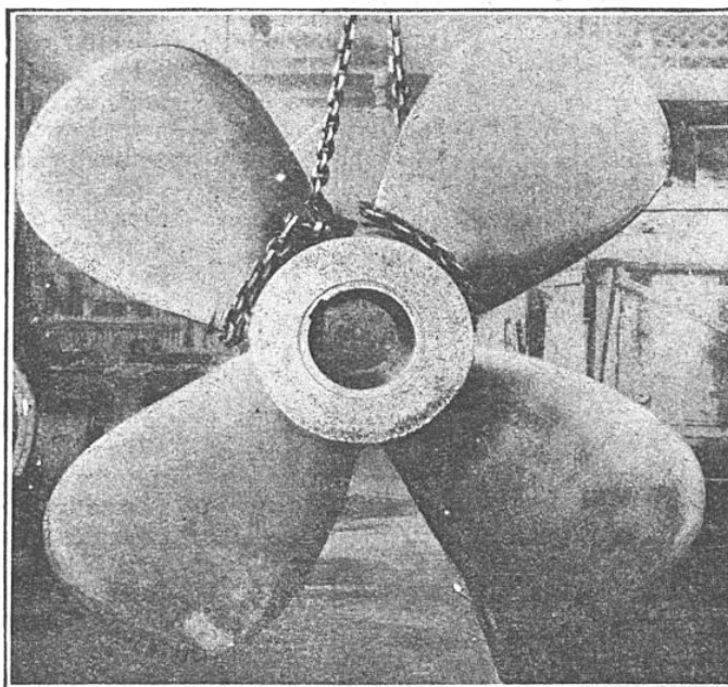
HÉLICE LATÉRALE A QUATRE AILES DE L'« OLYMPIC » Ce propulseur en bronze-manganèse, de 5 mètres de diamètre avec moyeu d'acier moulé, est actionné par une turbine Parsons tournant à 165 tours et qui développe une puissance de 16.000 HP.
