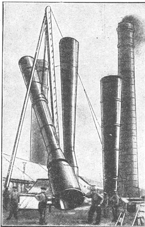
MONTAGE ET MISE EN PLACE D'UNE CHEMINÉE EN TÔLE
