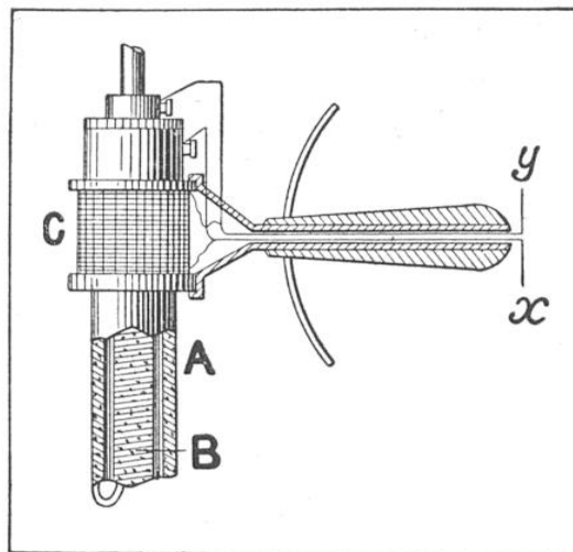
FIG. 18. — CHALUMEAU A ARC TOURNANT DE M. COFFIN
