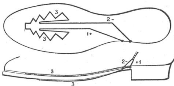
SEMELLE CHAUFFÉE A L'ÉLECTRICITÉ 1, fil positif; 2, fil négatif; 3, résistance.
