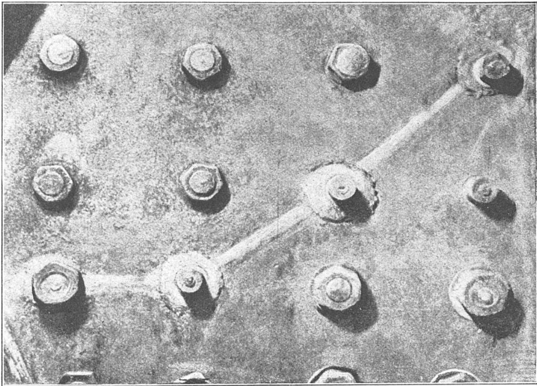
FIG. 9. — UNE RÉPARATION DE CHAUDIÈRE PAR LA SOUDURE ÉLECTRIQUE
