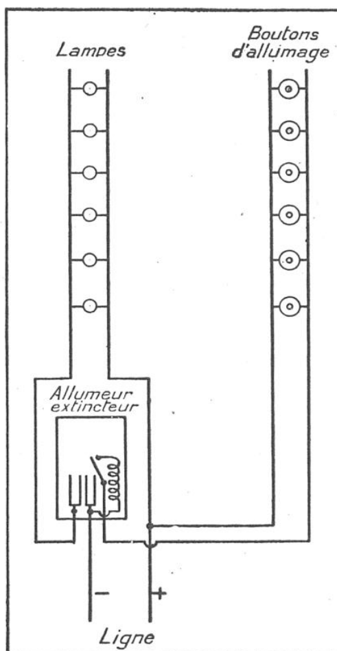
SCHÉMA DES CONNEXIONS DE LA MINUTERIE GRIVOLAS POUR LE VESTIBULE ET LES CINQ ÉTAGES D'UNE MAISON
