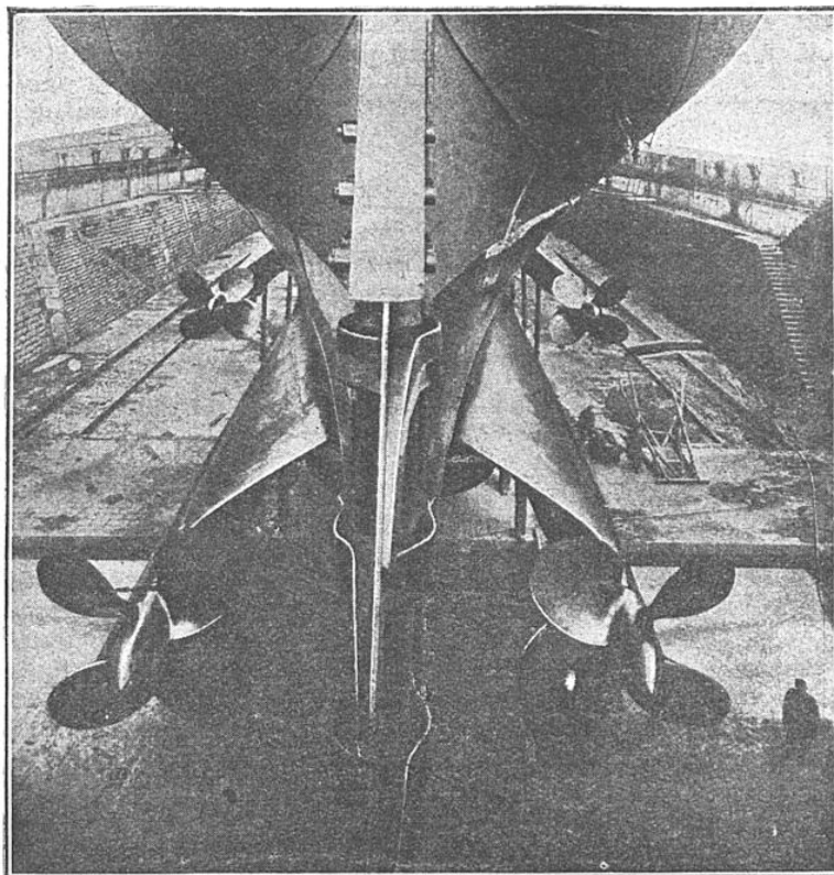
ÉTAMBOT DU PAQUEBOT A QUATRE HÉLICES « FRANCE »
