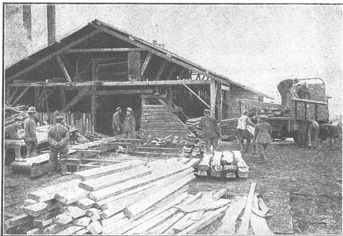
CAMION AUTOMOBILE CHARGEANT DES TRAVERSES A LA SCIERIE DU GUÉ-DES-GRUES Tous les jours plusieurs centaines de traverses sont mises par chaque scierie à la disposition du Service des chemins de fer militaires des fronts britannique et français.
