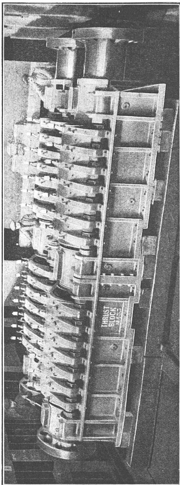
VUE GÉNÉRALE DU PALIER DE BUTÉE DU TRANSATLANTIQUE ANGLAIS « BRITANNIC » DE LA WHITE STAR LINE. Ces paliers sont destinés à absorber la poussée des propulseurs sur les lignes d'arbres centrales actionnées par des machines à vapeur verticales alternatives, à pistons, tandis que des turbines font tourner les hélices jumelles latérales.
