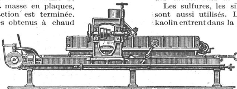
MACHINE A SCIER LES BLOCS RECTANGULAIRES DE CAOUTCHOUC
