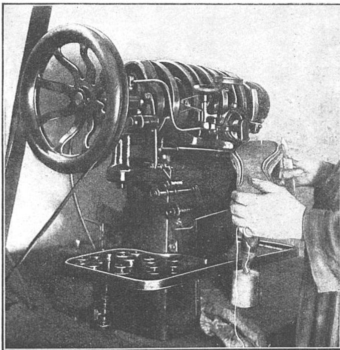
MACHINE SPÉCIALE POUR COUDRE LA SEMELLE
