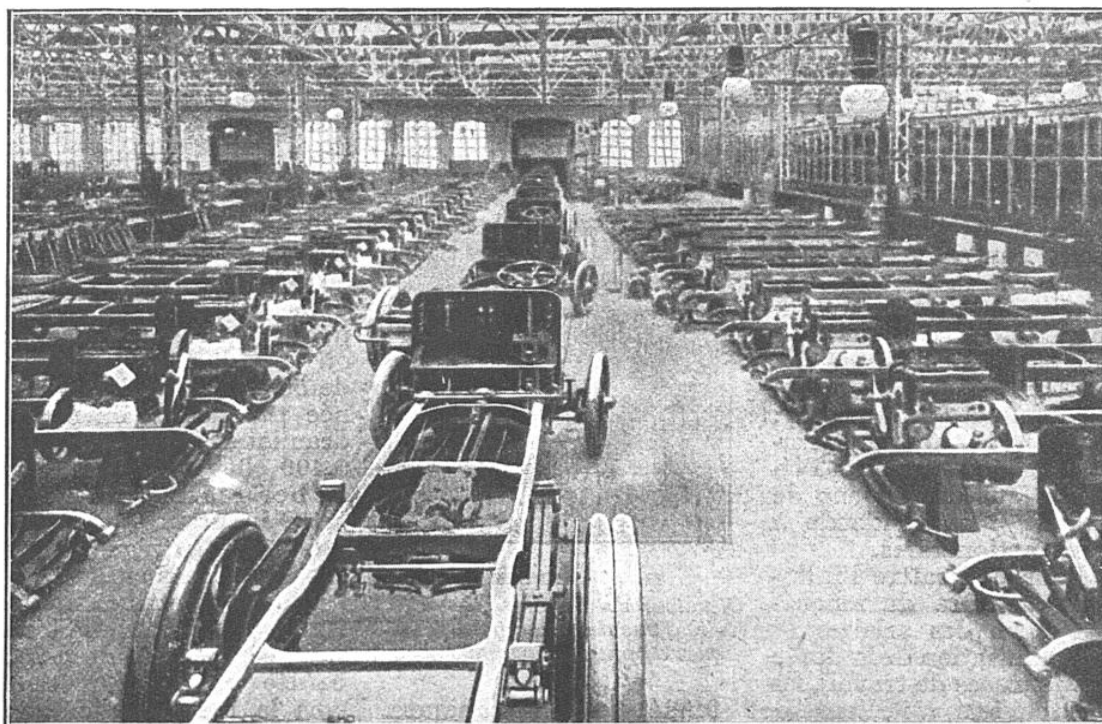
ATELIER DE MONTAGE DES CHASSIS DE CAMIONS AUTOMOBILES AUX USINES « F.I.A.T. »
