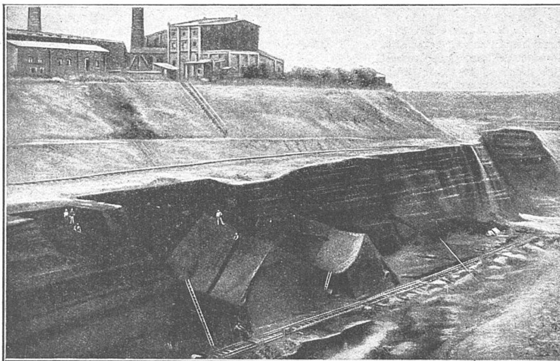
VUE DES TRAVAUX D'EXTRACTION D'UNE MINE DE LIGNITE SAXONNE
