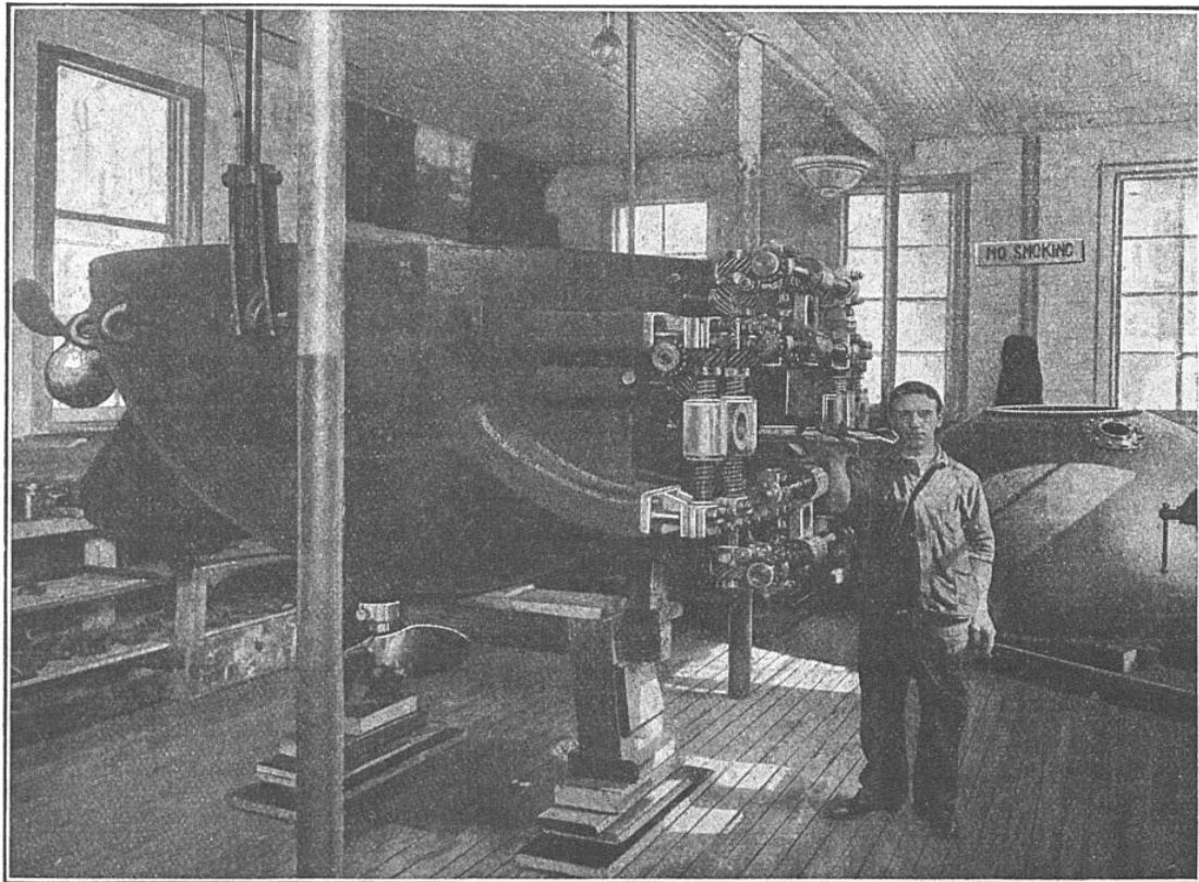
HÉMISPHERE INFÉRIEUR DU SOUS-MARIN POUR LE RELEVAGE DES NAVIRES
