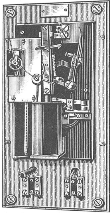
APPAREIL DE LA SOCIÉTÉ INDUSTRIELLE DES TÉLÉPHONES, A RÉGULATEUR ET A BOBINE
