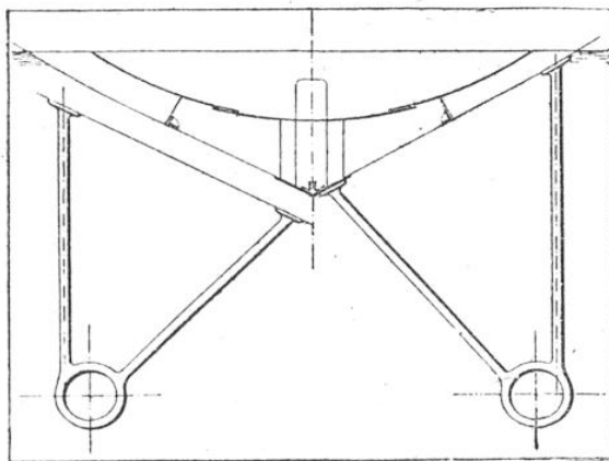
SUPPORTS DES DEUX ARBRES PORTE-HÉLICES DU CONTRE-TORPILLEUR « SABRE »
