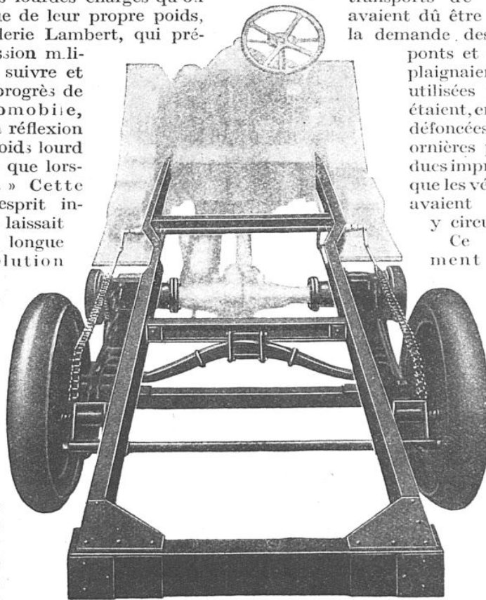
TRANSFORMATION DU CHASSIS AVEC COMMANDE PAR CHAINES DE GALLE
