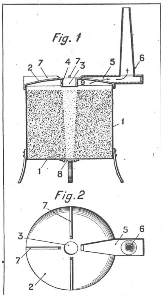
FOURNEAU A SCIURE (CUISINIÈRE) DE LA SOCIÉTÉ ESPAGNOLE « TERMES Y C ia »
