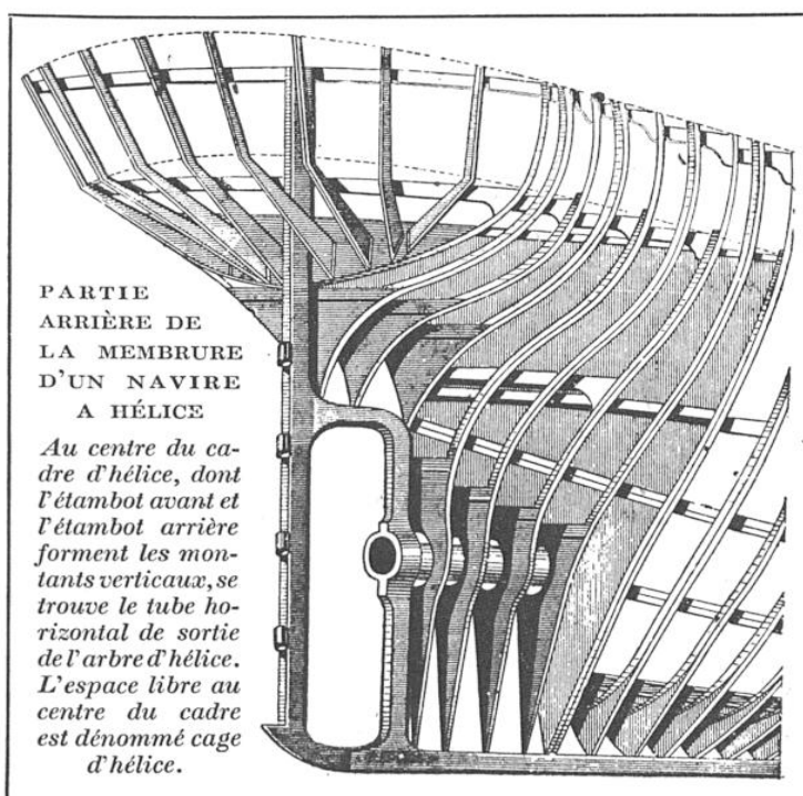
ARRIÈRE D'UN VAPEUR A HÉLICE CENTRALE
