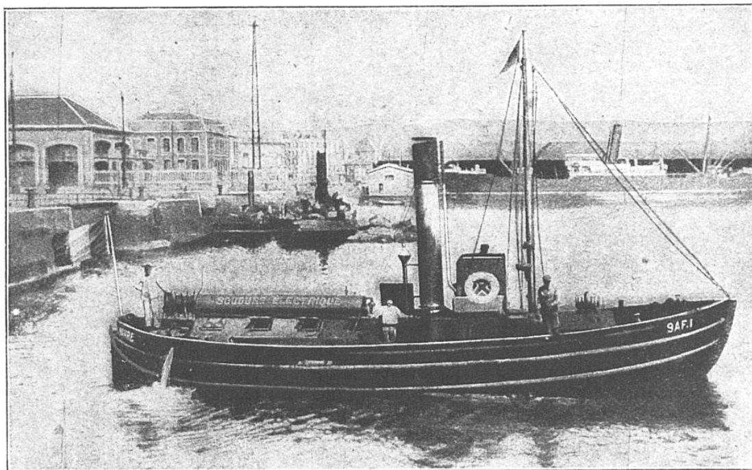
FIG. 16. — ATELIER FLOTTANT DE SOUDURE ÉLECTRIQUE POUR LES RÉPARATIONS À EFFECTUER AUX NAVIRES DANS LES PORTS DE MER
