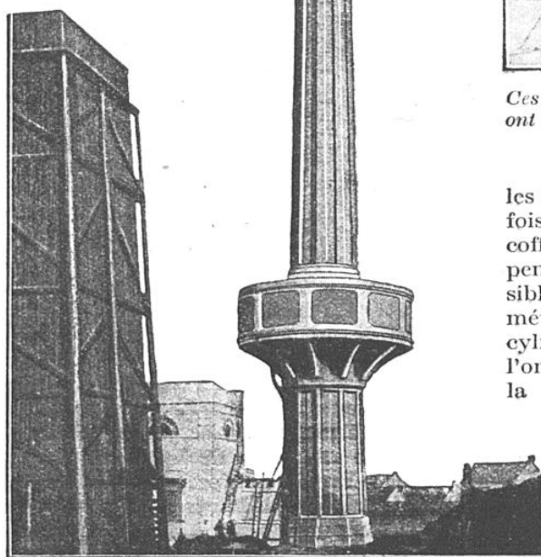
Les arêtes ou saillies qui se profilent sur toute la hauteur de cette cheminée, qui a 50 mètres d'élévation, sont formées par les crosses des claveaux.
