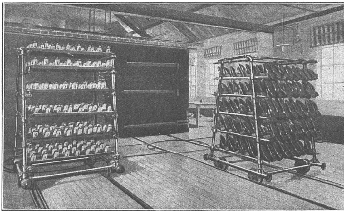
CHARIOTS EMPLOYÉS POUR LA VULCANISATION DES GALOCHES DE CAOUTCHOUC Les chariots-supports sont introduits avec leur chargement dans une étuve chauffée à la vapeur.
