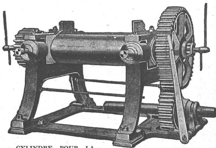
CYLINDRE POUR LA MASTICATION MÉCANIQUE DU CAOUTCHOUC BRUT
