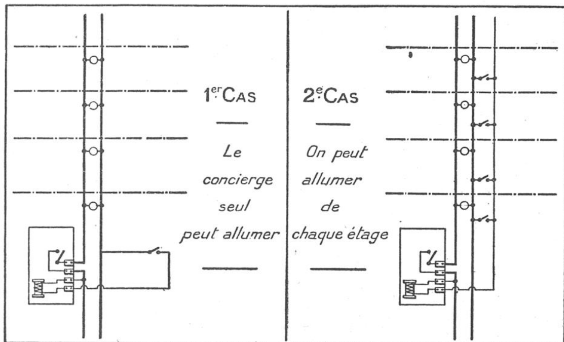
SCHEMAS DES CONNEXIONS, DANS DEUX CAS DÉTERMINÉS, DE L'APPAREIL CI-DESSUS
