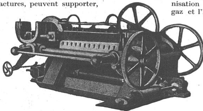
MACHINE AUTOMATIQUE A COUPER LES BLOCS ROUNDS DE CAOUTCHOUC
