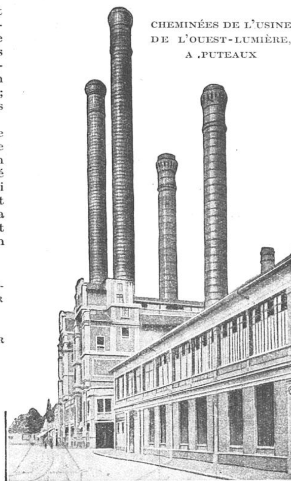
Ces cheminées mesurent 90 mètres de hauteur ; elles ont conservé la trace des manchons qui ont servi de coffrage pour disposer le ciment armé.
