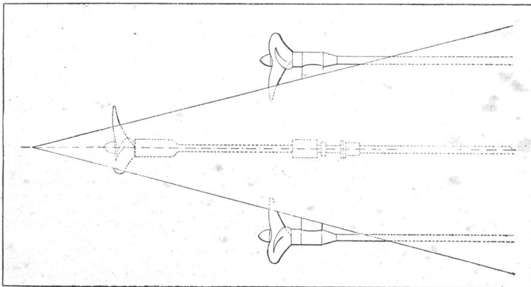
LES TROIS LIGNES D'ARBRES D'UN BATIMENT DE GUERRE A TROIS HÉLICES
