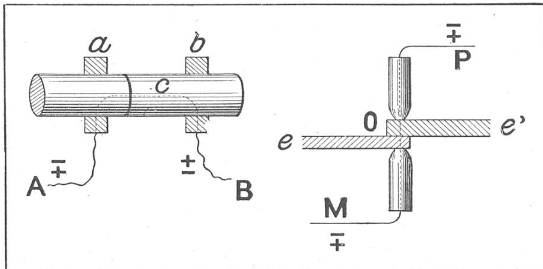
FIG. 1 ET 2. — LE PROCÉDÉ DE SOUDURE ÉLECTRIQUE PAR COURT-CIRCUIT
