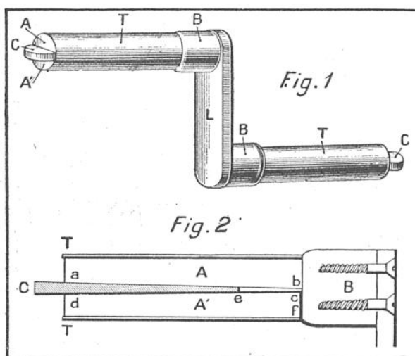
LE TOURNIQUET CHAUFFE-MAINS
