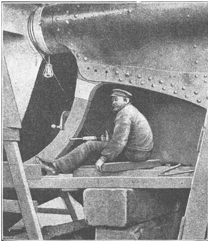
FIG. 11. — RÉPARATION À L'ARRIÈRE D'UN NAVIRE La légèreté du matériel utilisé pour la soudure électrique permet à l'ouvrier de s'engager dans les charpentes de soutien.
