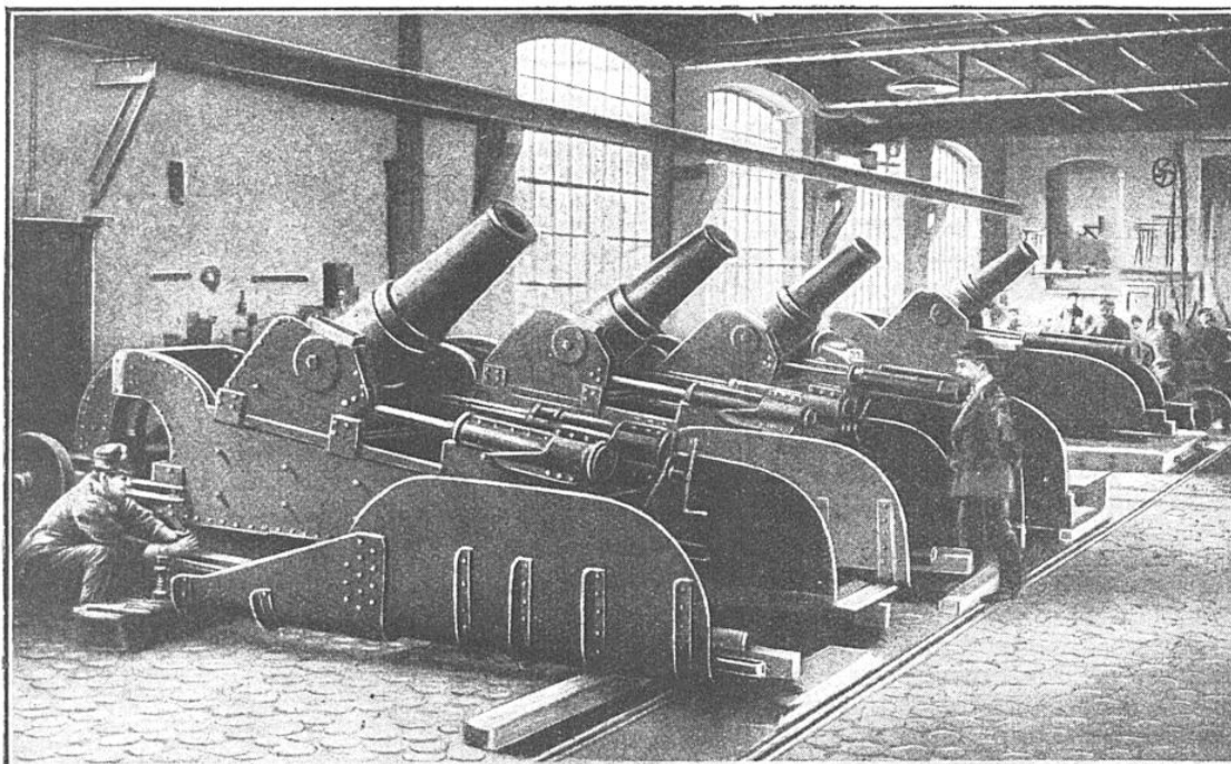
MONTAGE DES AFFUTS D'UNE BATTERIE DE MORTIERS ITALIENS DE 210 MILLIMÈTRES Ces pièces, d'un type tout à fait moderne, sont munies de tous les perfectionnements qui caractérisent aujourd'hui les canons et les obusiers : frein hydraulique, remise en batterie automatique, etc.
