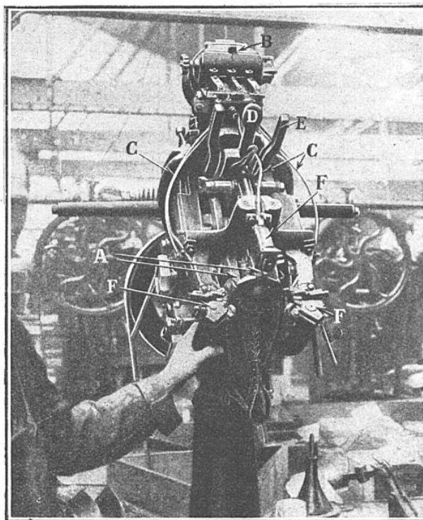
MACHINE A METTRE SUR FORME
