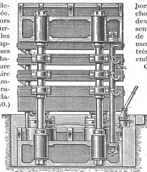
PRESSE HYDRAULIQUE A VULCANISER
