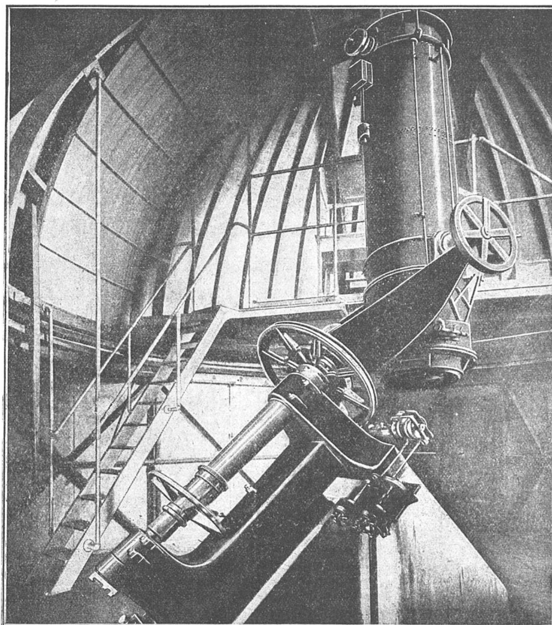
MONTAGE D'UN GRAND INSTRUMENT AVEC SUPPORT EN FORME DE FOURCHE
