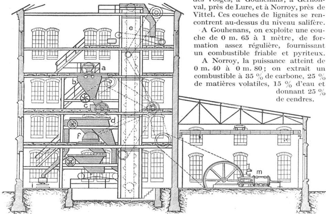
COUPE VERTICALE D'UN ATELIER DE MOUILLAGE DES LIGNITES
