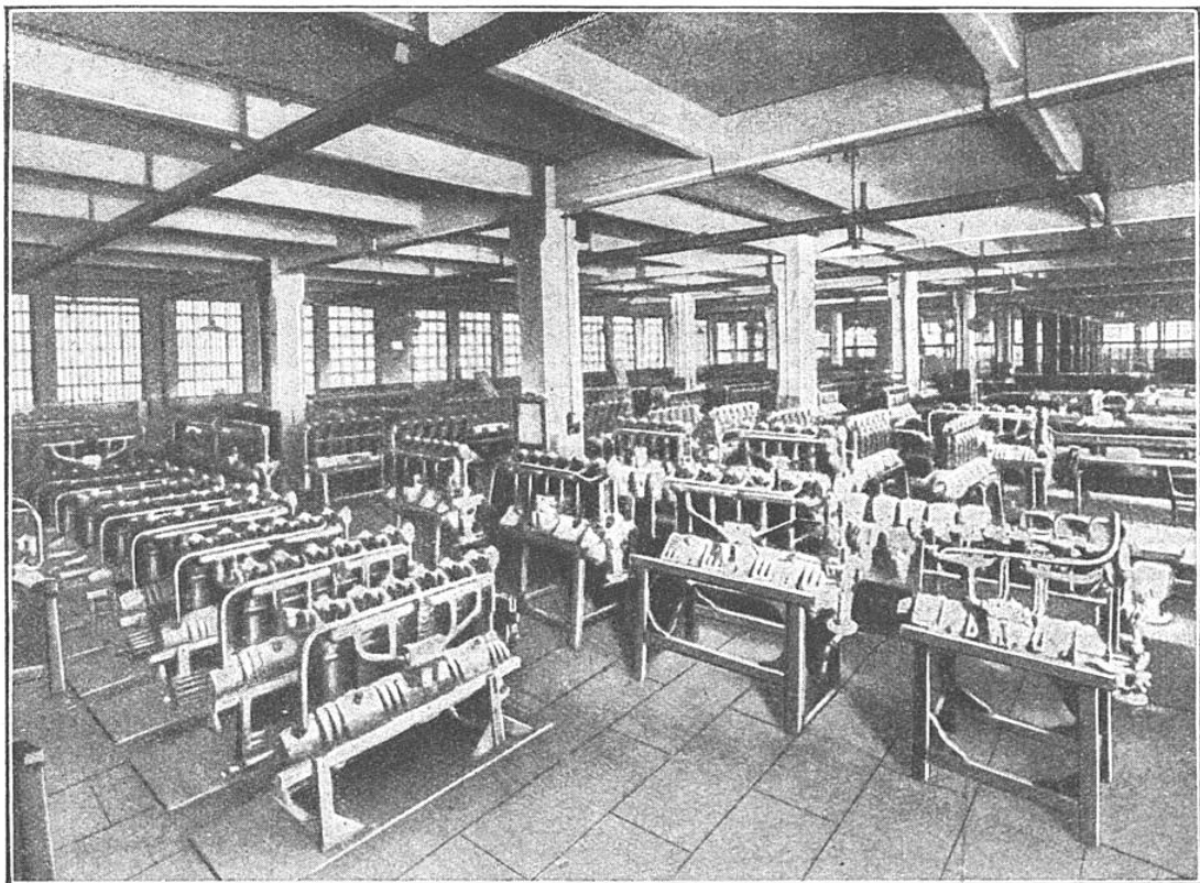
ATELIER DE REVISION DES MOTEURS D'AVIATION, AUX USINES « F. I. A. T. », A TURIN
