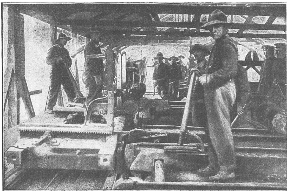
SCIE MONTÉE SUR BATI MOBILE SE DÉPLAÇANT PARALLÈLEMENT A L'ARBRE A ÉCORCER
