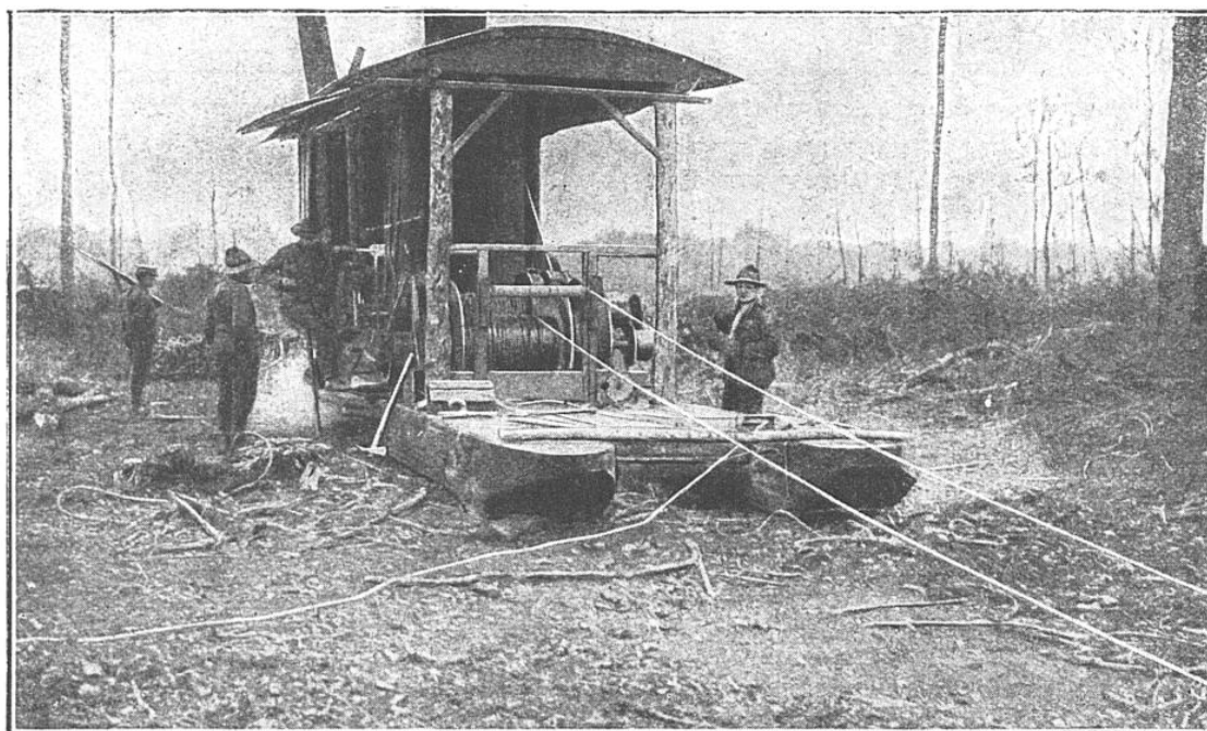
TREUIL A VAPEUR MONTÉ SUR SABOTS POUR LA MANUTENTION DES ARBRES ABATTUS
