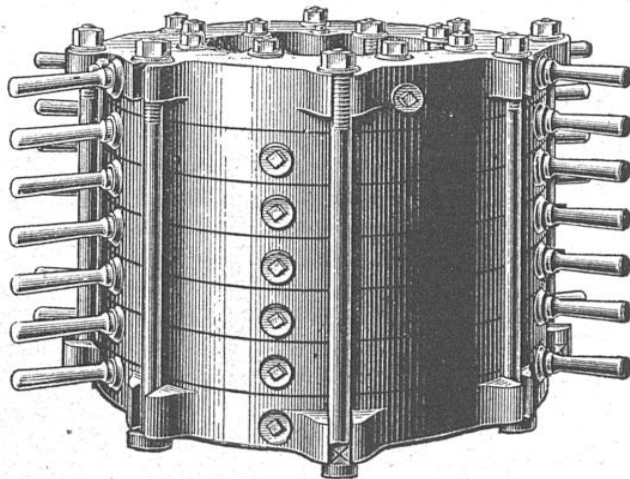
MACHINE A COQUILLE POUR PNEUMATIQUES
