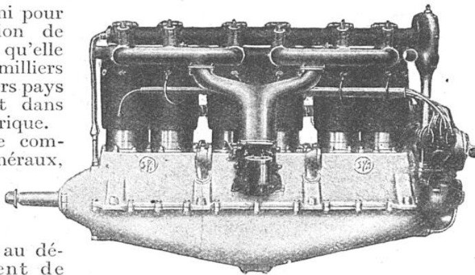
LE MOTEUR D'AVIATION ITALIEN « S. P. A. »
