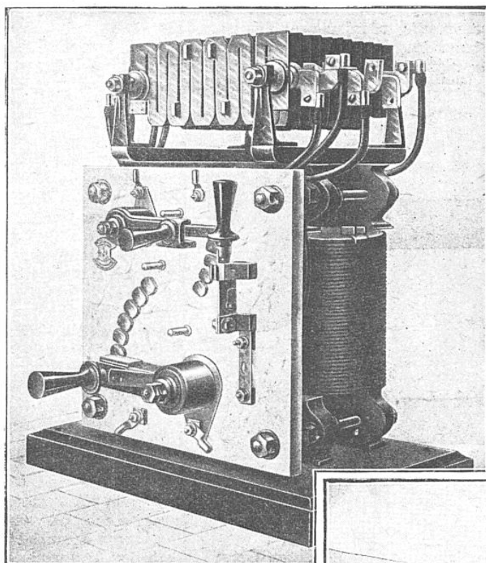
FIG. 13. — APPAREIL ÉCONOMISEUR DE COURANT CONSTRUIT PAR LA « CIE UNIVERSAL ÉLECTRIC »
