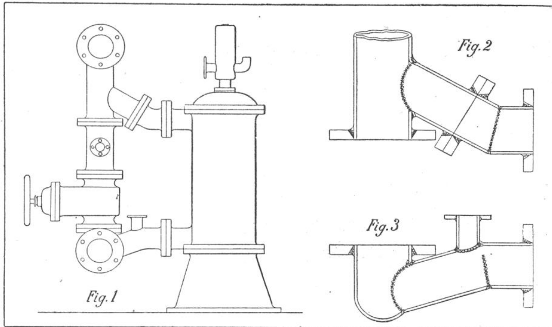
PLANCHE 12. — CONDUITES DÉTÉRIORÉES ET RÉPARÉES PAR LA SOUDURE ÉLECTRIQUE
