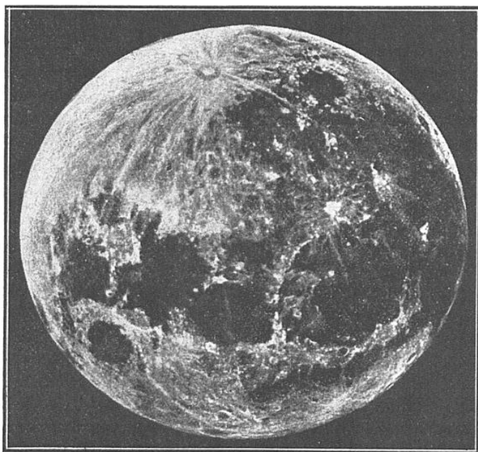
LA LUNE VUE DANS UN TÉLESCOPE A GRANDE OUVERTURE
