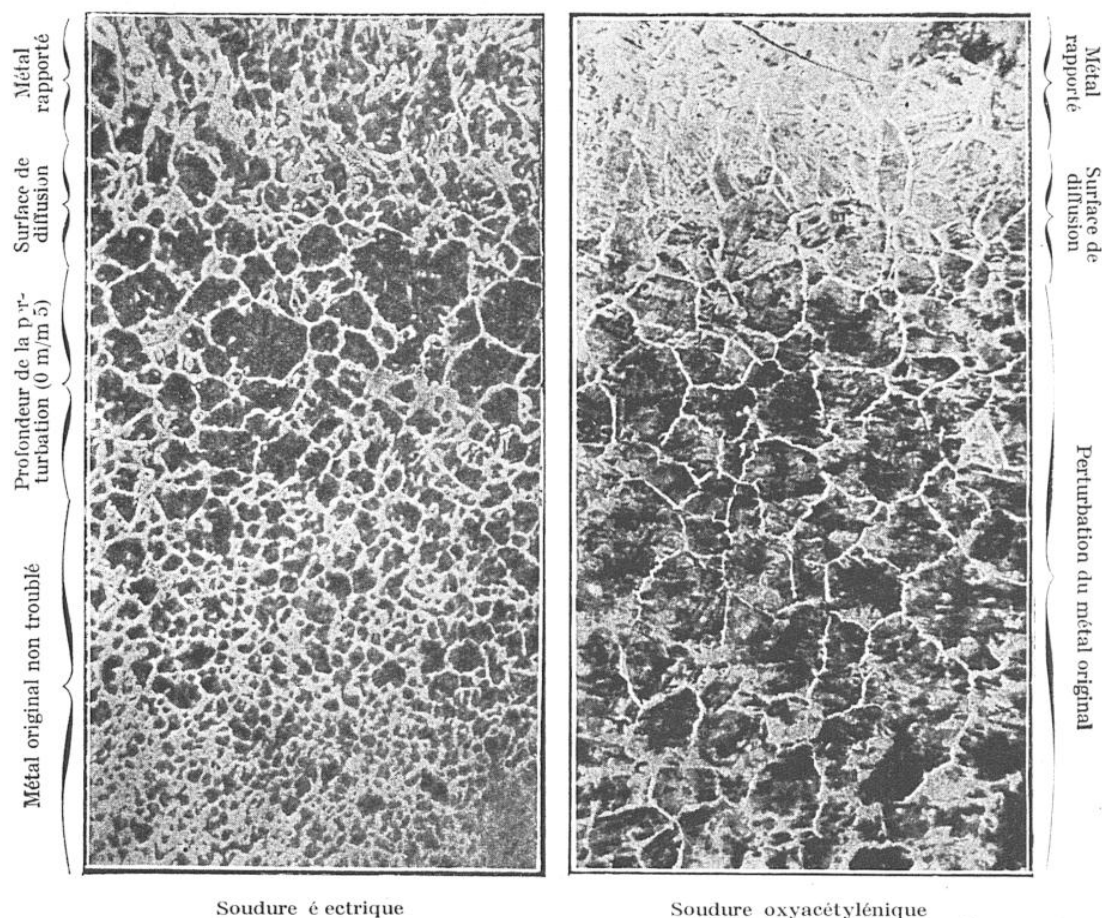
FIG. 19. — PHOTO-MICROGRAPHIES FAISANT RESSORTIR LA DIFFÉRENCE DES PERTURBATIONS INTRODUITES DANS LE MÉTAL PAR LES SOUDURES ÉLECTRIQUE ET OXYACÉTYLÉNIQUE. La profondeur de la perturbation, qui atteint seulement un demi-millimètre pour la soudure électrique, affecte toute l'épaisseur de la tôle pour la soudure oxyacétylénique. (Communiqué par le procédé Quasi-Arc).
