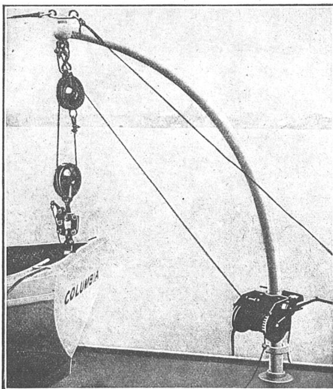
DÉTAIL DU TREUIL MONTÉ SUR CHAQUE BOSSOIR ET DU CROC D'EMBARCATION
