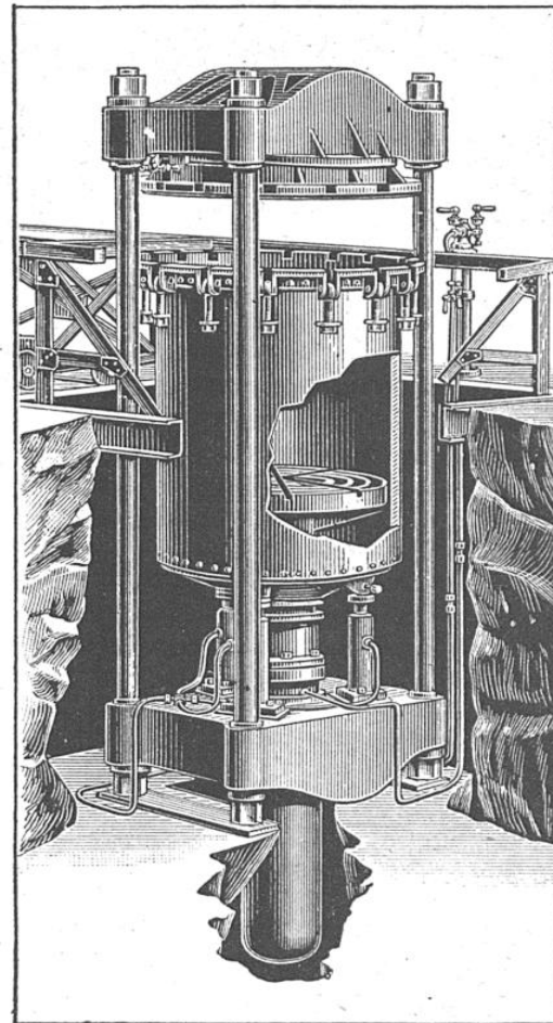
PRESSE HYDRAULIQUE AUTOCLAVE
