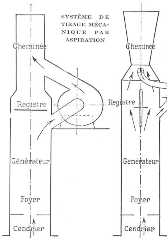
Le schéma de gauche montre un dispositif de tirage aspiré direct exigeant la fermeture du registre; celui de droite représente le tirage Prat, qui laisse le registre ouvert et permet d'utiliser le tirage naturel.
