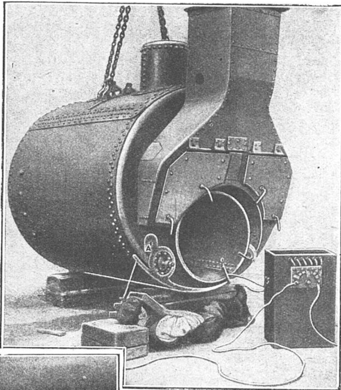
FIG. 11 BIS. — OUVRIER RÉPARANT ÉLECTRIQUEMENT UNE CHAUDIÈRE DE NAVIRE.
