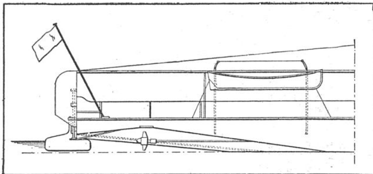
HÉLICE SOUS VOUTE D'UNE CANONNIÈRE FLUVIALE
