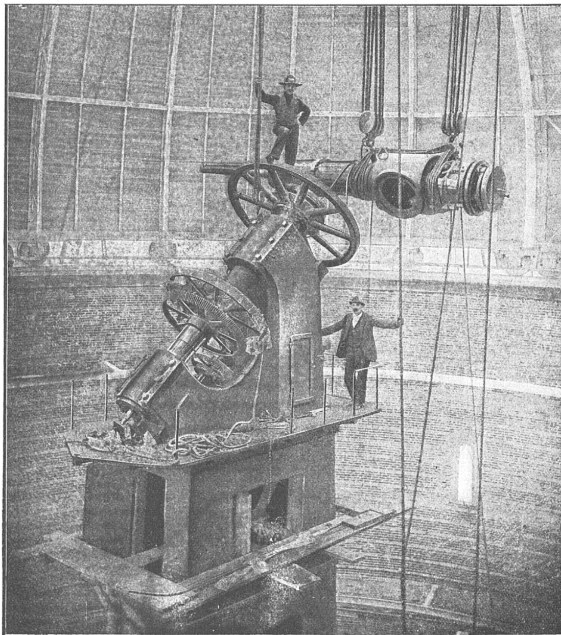
MONTAGE DE L'AXE POLAIRE ET DE L'AXE DE DÉCLINAISON D'UN TÉLESCOPE
