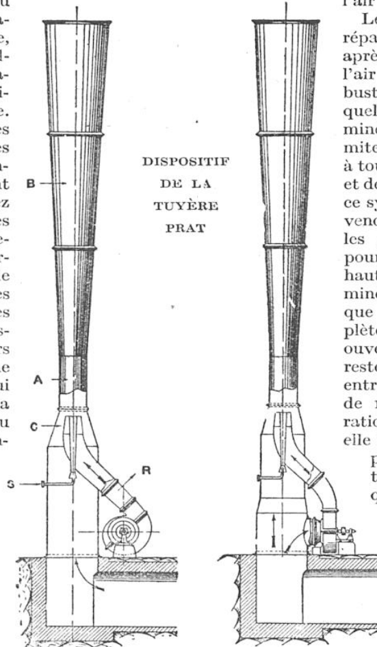
C, partie conique où convergent les gaz du foyer ; A, chambre de détente ; B, tube diffuseur ; R, souffleur ; S, éjecteur à vapeur. — Au gauche, le ventilateur envoie de l'air froid pris au dehors ; à droite, le ventilateur envoie des gaz chauds pris au foyer.
