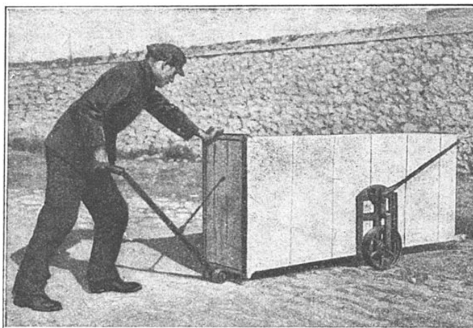
MANŒUVRE DE LA BROUETTE DE M. HARRASSOWITZ
