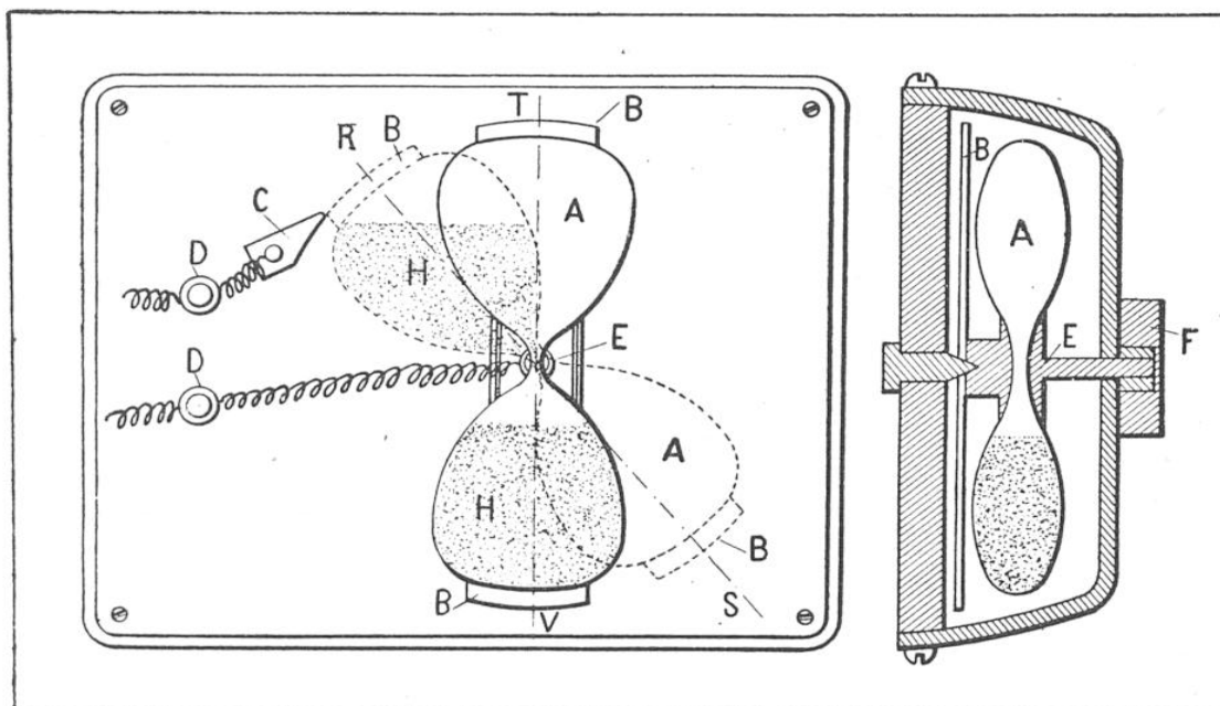
APPAREIL DE MM. FRIZI, CARDINETTI ET PAGANI (VUES DE FACE ET DE COTÉ)
