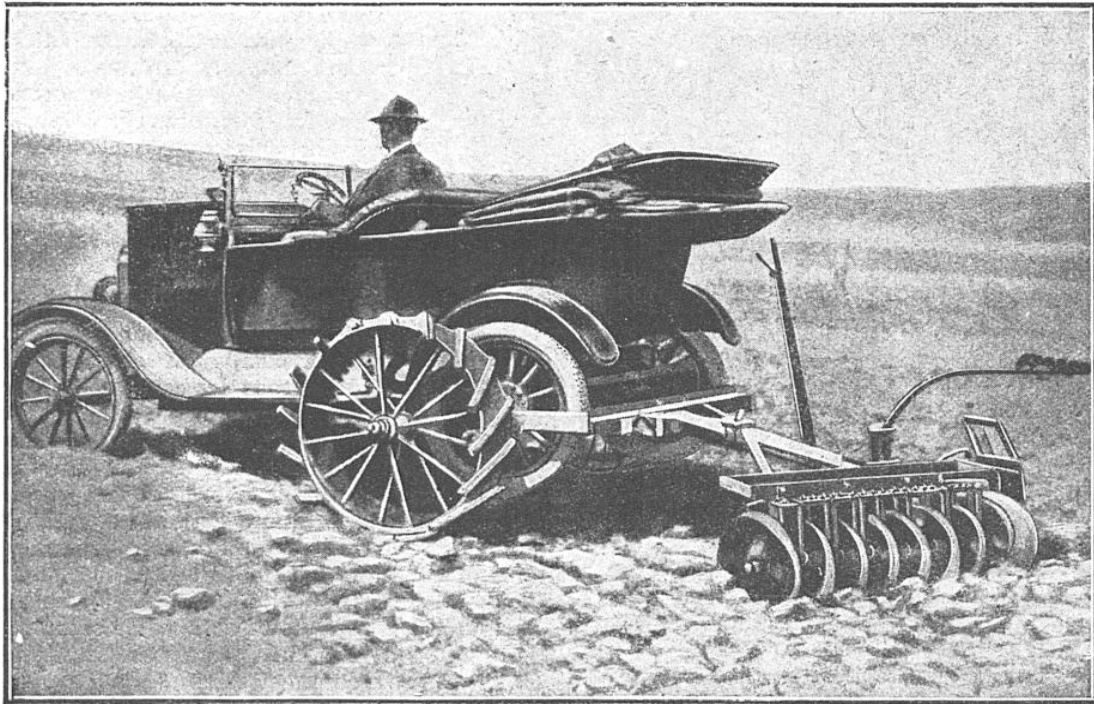
VOITURE LÉGÈRE TRANSFORMÉE POUR LES TRAVAUX AGRICOLES
