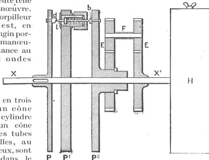
FIG. 2. — APPAREIL DE COMMANDE A DISTANCE PAR LES ONDES DE T. S. F.
