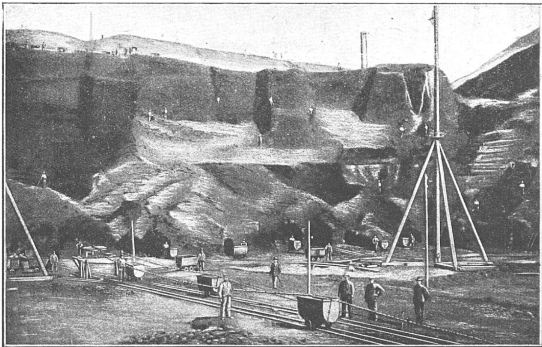
EXPLOITATION DE LIGNITE A CIEL OUVERT, EN ALLEMAGNE
