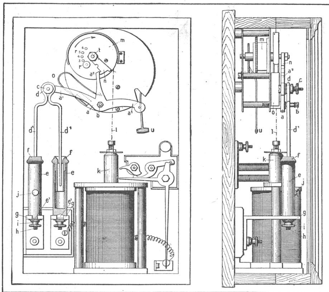
APPAREIL SALOMON A MOUVEMENT D'HORLOGERIE ET A BOBINE, REPRÉSENTÉ DE FACE, AVEC COUPE PARTIELLE, ET DE COTÉ
