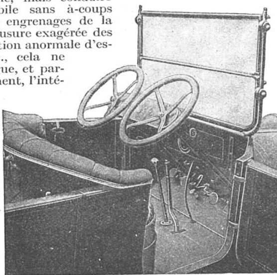
EN PLUS DES DEUX VOLANTS, TOUS LES ORGANES DE COMMANDE SONT DOUBLES
