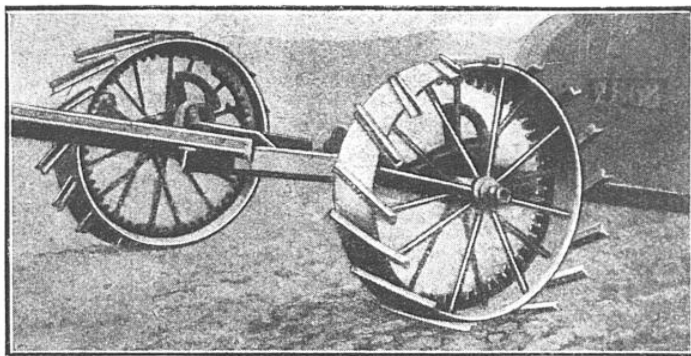
ARRIÈRE-TRAIN SE FIXANT À L'ARRIÈRE DU VÉHICULE Ce dispositif est celui adopté pour les travaux de l'agriculture. Les roues métalliques sont munies de cornières pour s'agripper dans les terres molles.
