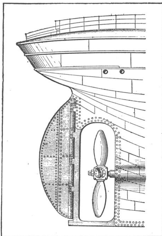
ARRIÈRE D'UN VAPEUR A HÉLICE CENTRALE
