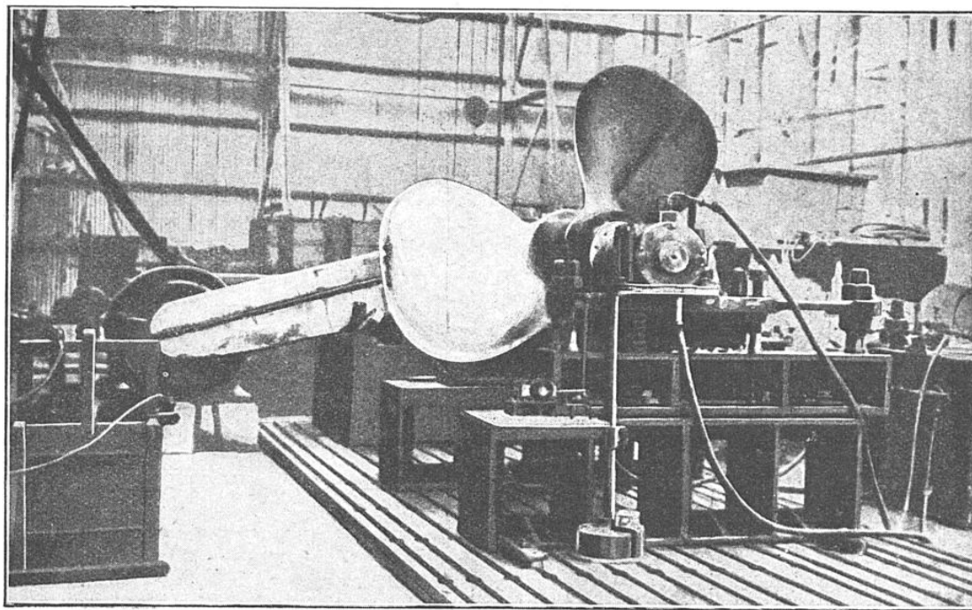
DISPOSITIF SERVANT A L'ÉQUILIBRAGE D'UNE HÉLICE A TROIS AILES
