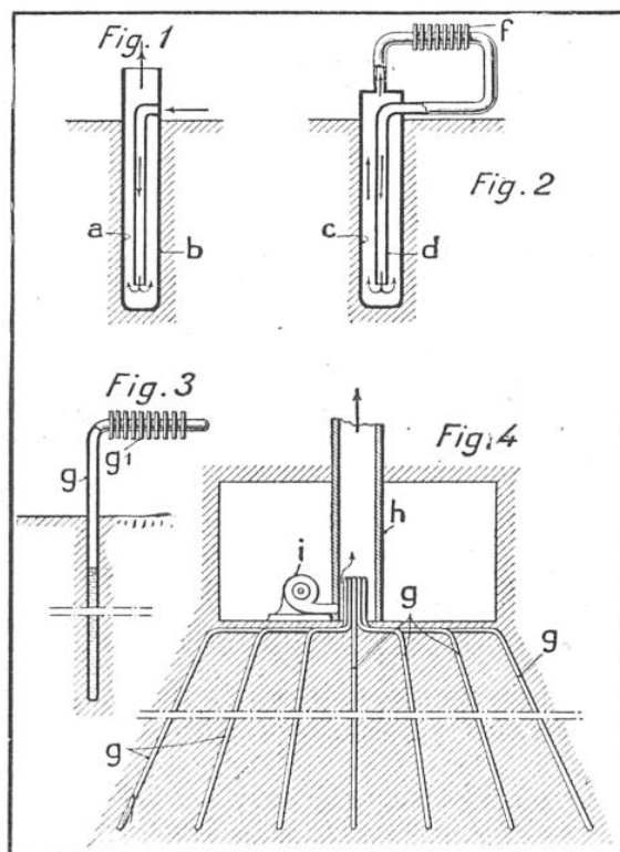
DISPOSITIFS POUR L'UTILISATION DE LA DIFFÉRENCE DE LA TEMPÉRATURE ENTRE LES COUCHES BASSES DU SOL ET L'ATMOSPHÈRE
