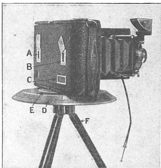
APPAREIL KODAK MODIFIÉ POUR LA PRISE DES VUES PANORAMIQUES
