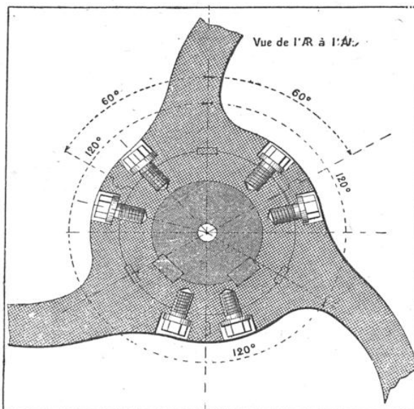
MODE DE FIXATION D'UNE HÉLICE A TROIS AILES SUR SON MOYEU
