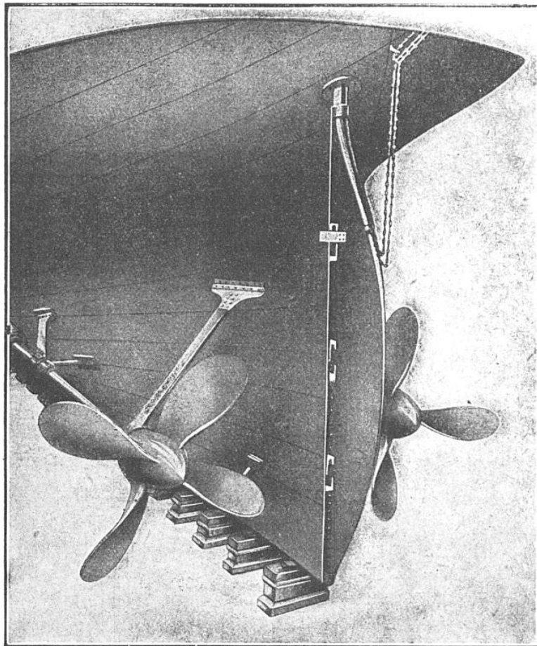
ARRIÈRE D'UN VAPEUR A HÉLICES JUMELLES
