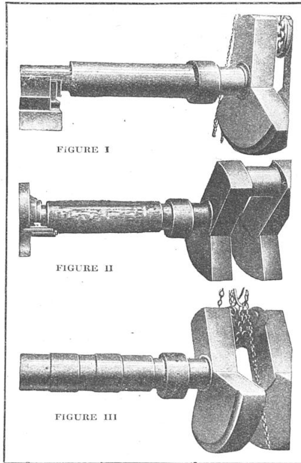
PL. 15. — UN BEAU TRAVAIL DE RENFORCEMENT DE PIÈCE RENDU POSSIBLE PAR LE PROCÉDÉ DE SOUDURE ÉLECTRIQUE PAR L'ARC
