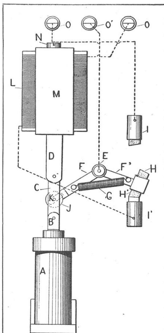
APPAREIL DE MINUTERIE D'ESCALIERS A FREIN A GLYCÉRINE IMAGINÉ PAR M. PRUDENCE
