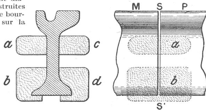
FIG. 6. — SOUDURE DES RAILS PAR COURT-CIRCUIT A gauche : coupe par le rail ; à droite : vue de face des deux extrémités des rails à souder M P suivant la ligne de jonction S S'. — a c et b d, pièces d'acier dont la fusion sert à assurer la soudure.
