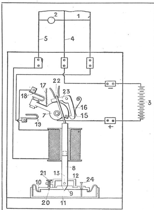
APPAREIL DE M. BENDIXEN, A FREIN A AIR
