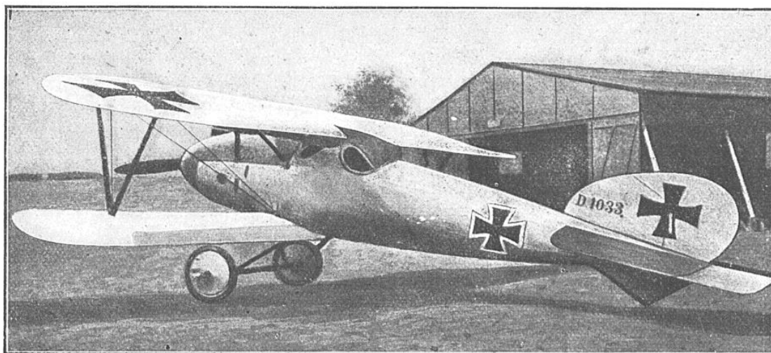
L'ALBATROS DE CHASSE D-III, TYPE 1917, COPIÉ SUR NOTRE NIEUPORT
