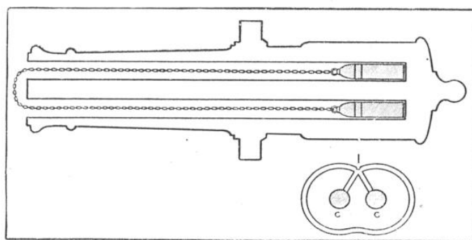
CANON A OBUS JUMELÉS DE M. BARON
