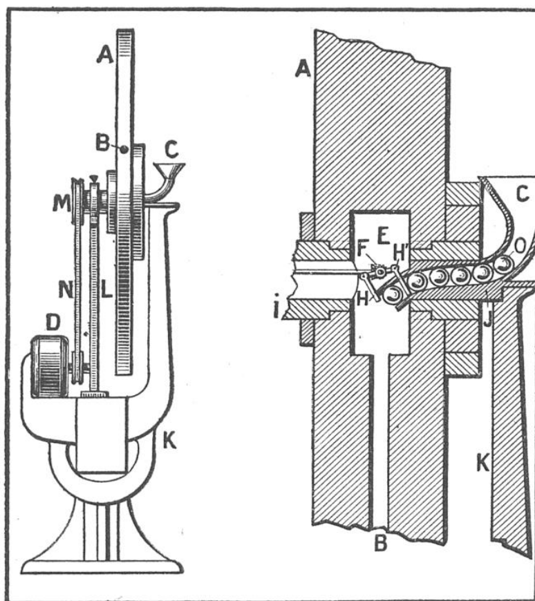
A GAUCHE : VUE EN ÉLEVATION DE COTÉ DU CANON CENTRIFUGE GOODWIN ; A DROITE : COUPE DE LA CHAMBRE D'ALIMENTATION EN PROJECTILES DU MÊME ENGIN
