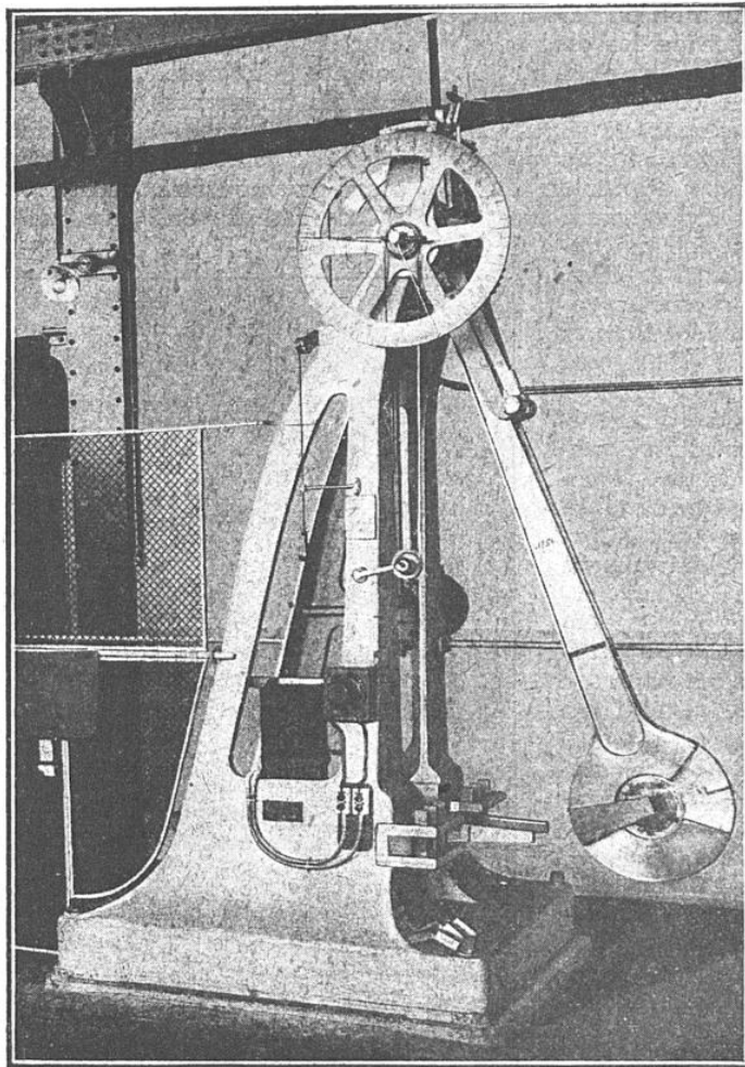
LE MOUTON-PENDULE DE CHARPY POUR MESURER LA FRAGILITÉ DU MÉTAL
