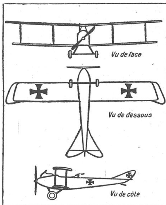
CARACTÉRISTIQUES DU RUMPLER C-III
