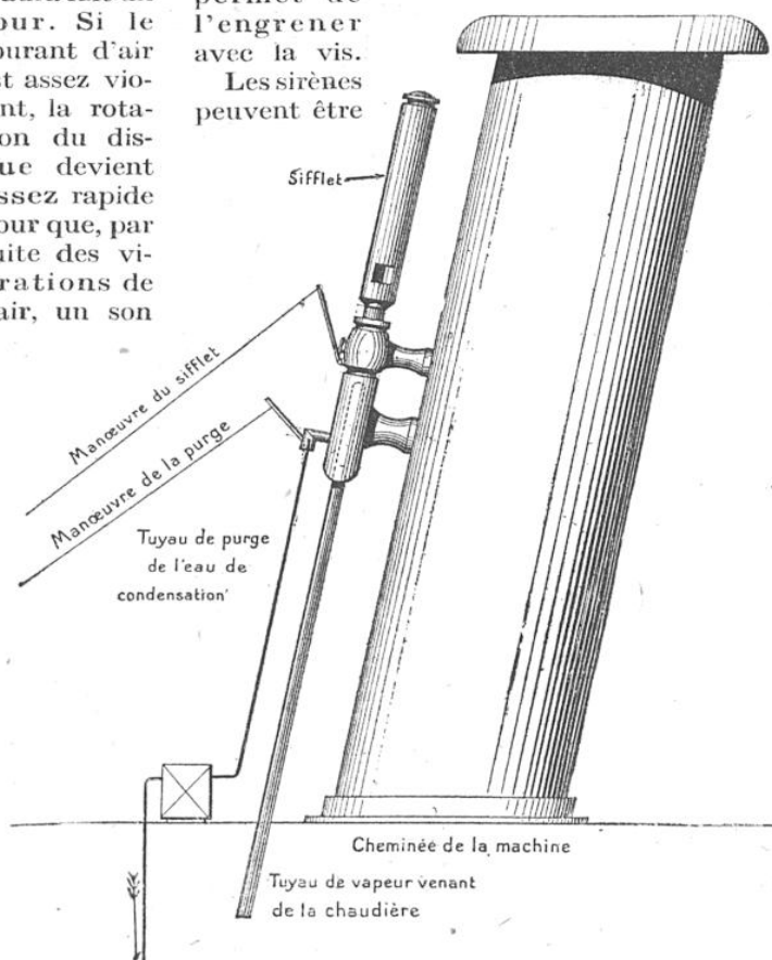
MONTAGE DU SIFFLET SUR LA CHEMINÉE D'UN NAVIRE La réception d'eau est placée sur le tuyau de purge, lequel descend à la soupape de la chaudière. (Dessin non à l'échelle.)
