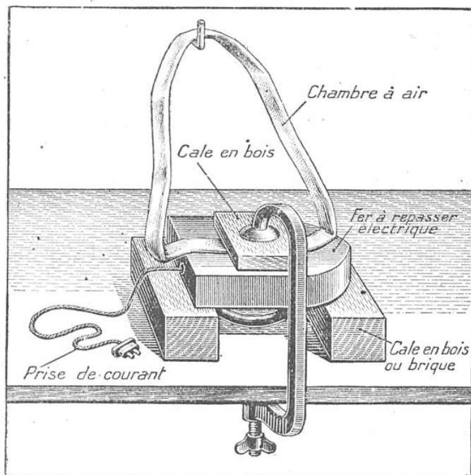
SERRÉE CONTRE LE FER ÉLECTRIQUE, LA PIÈCE EST VULCANISÉE SUR LA CHAMBRE À AIR EN CINQ MINUTES
