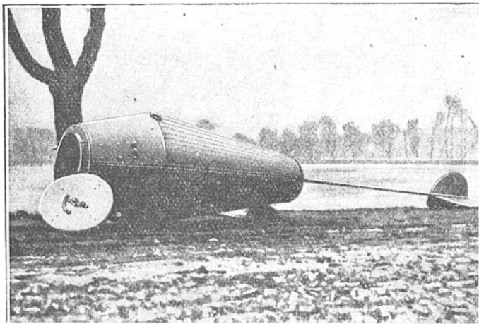
BOUÉE DE SAUVETAGE « TRITON », NON IMMERGÉE, AVEC SON COUVERCLE ENLEVÉ
