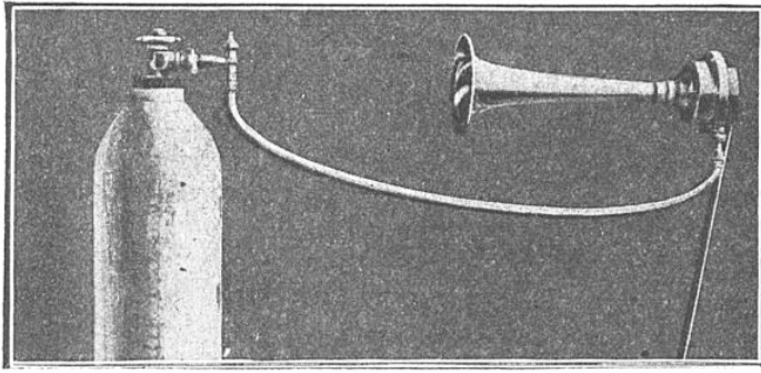
LE « TÉNOR » A SIMPLE PAVILLON, DE M. CHOLLET L'appareil est relié par un tube à un réservoir d'air comprimé.
