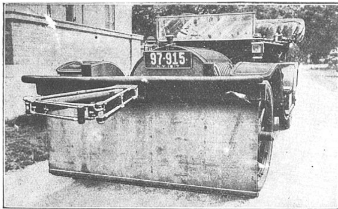
LES BRAS ARTICULÉS ET LE RIDEAU PROTECTEUR TELS QU'ILS APPARAISSENT QUAND LE CONDUCTEUR A DU AVOIR RECOURS A LEUR EMPLOI
