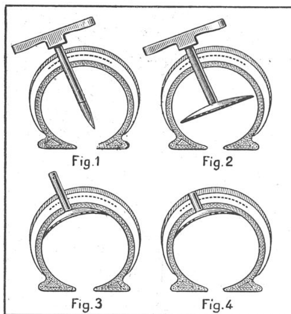
ÉTAPES DE LA RÉPARATION D'UNE DÉCHIRURE D'ENVELOPPE PAR UN PROCÉDÉ NOUVEAU
