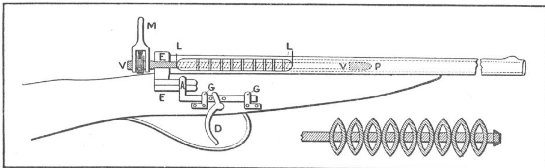
FUSIL A RESSORTS INVENTÉ EN 1871 PAR MM. CHAUVIN ET AUBIN
