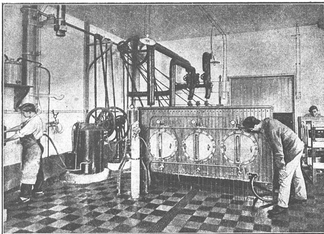
APPAREIL SPÉCIAL A DÉGLUTINER LA BIÈRE OU « CHILLING »
