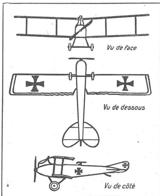
SCHÉMAS DE L'ALBATROS C-III
