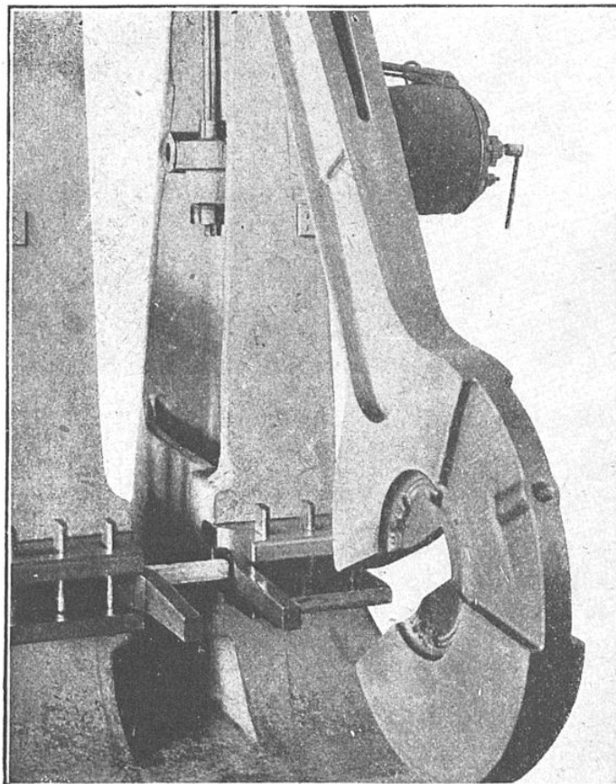
DÉTAIL DU BALANCIER-PENDULE ET DU COUTEAU DE L'APPAREIL CHARPY
