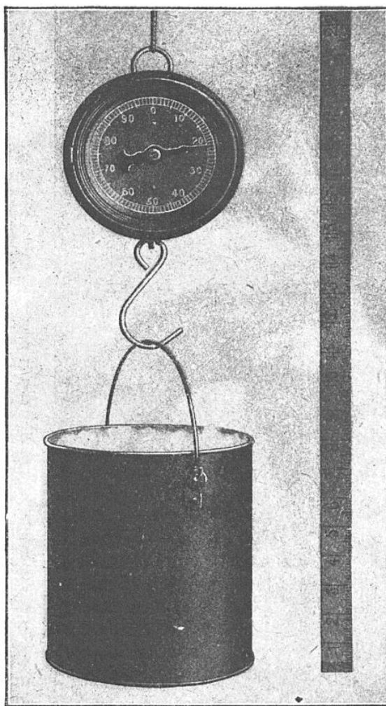
RÉCIPIENT COLLECTEUR DE NEIGE SUSPENDU A UNE BALANCE A RESSORT
