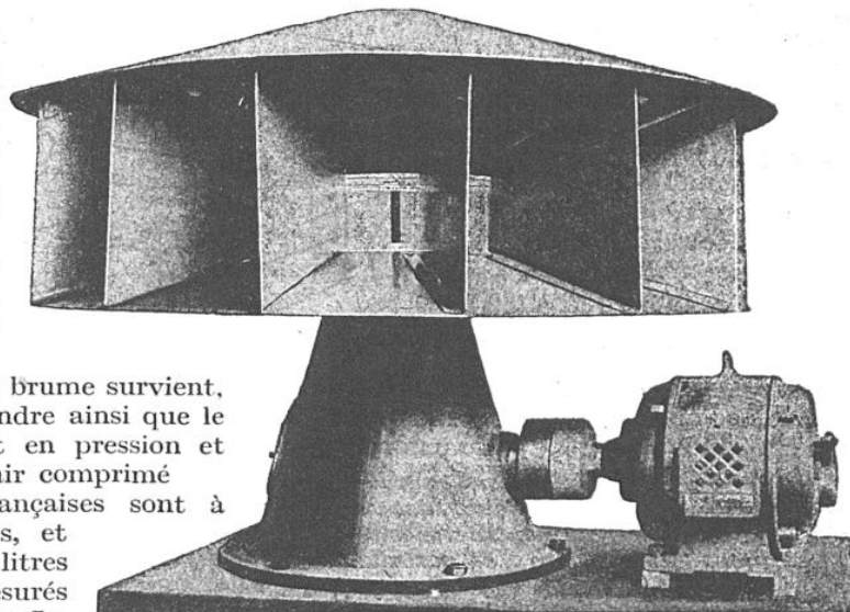
LA MÊME SIRÈNE AVEC AMPLIFICATEUR DE SON EN TOLE ET SURMONTÉE D'UN TOIT-ABRI CONIQUE
