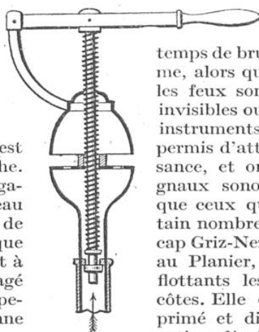
SIFFLET A MAIN DE MACHINE A VAPEUR OU DE LOCOMOTIVE
