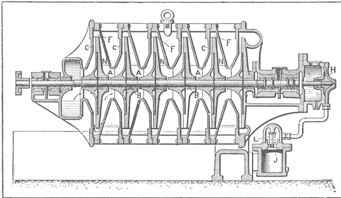
COUPE SCHÉMATIQUE LONGITUDINALE D'UN TURBO-COMPRESSEUR
