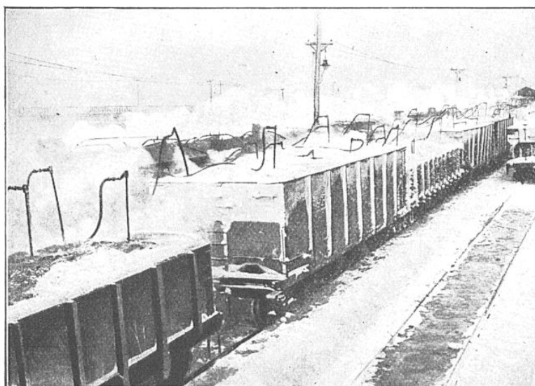
DES TUBES D'ACIER ENFONCÉS PROFONDÉMENT INJECTENT DE LA VAPEUR DANS LA MASSE DE CHARBON CONGELÉE
