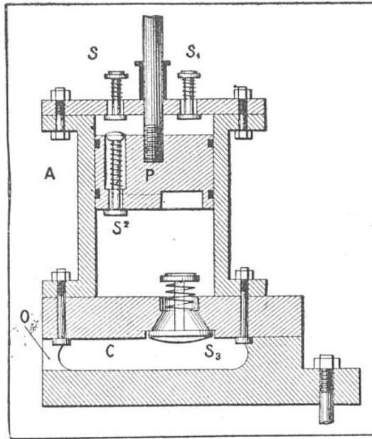
COMPRESSEUR A PISTON
