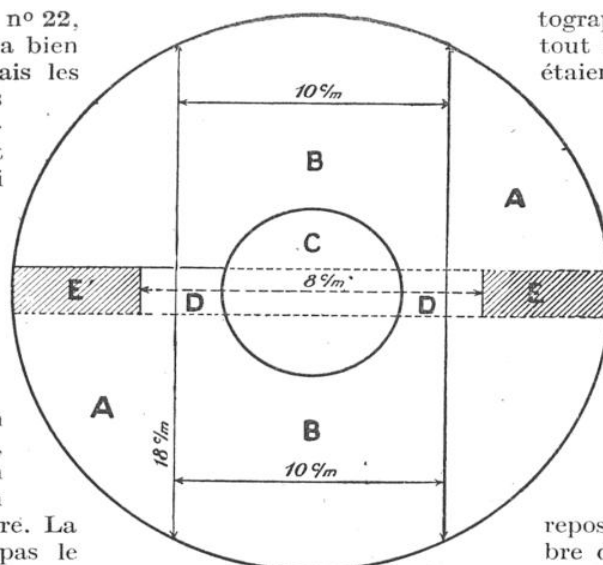
BOULE PORTE-DÉPÊCHES DE M. DELORT
