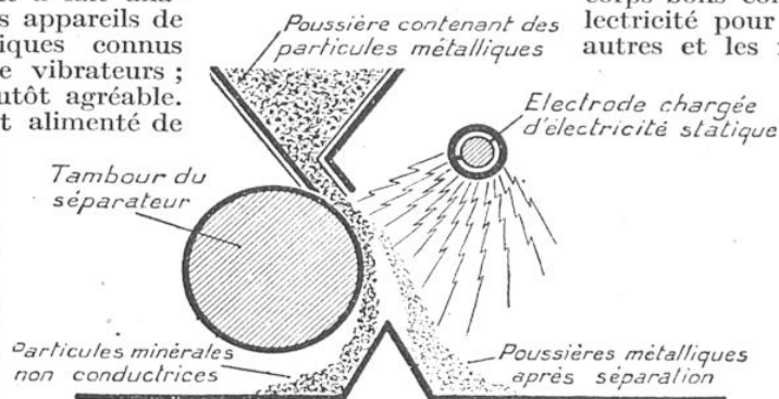
DISPOSITIF DU SÉPARATEUR ÉLECTROSTATIQUE
