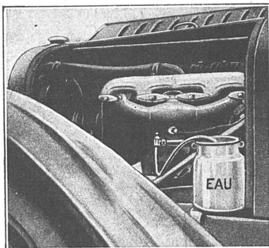
FIG. 3. — SI ON INJECTE DE L'EAU AU LIEU D'AIR, CETTE EAU SE TRANSFORME EN VAPEUR QUI AMOLLIT ET EXPULSE LE CARBONE DÉPOSÉ DANS LE MOTEUR
