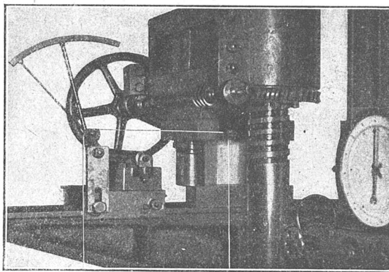
ESSAI DE COMPRESSION DU BOIS
