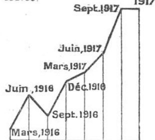
GRAPHIQUES INDICATIFS DES PERTES DE TONNAGE ALLIÉ ET DE SOUS-MARINS ALLEMANDS AU 31 DÉCEMBRE 1917.
