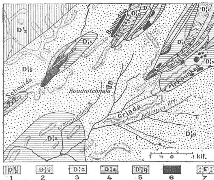
CARTE GÉOLOGIQUE DU MONT BOULANDIKHA, SUR L'IRKOUSKAN, ET DE LA CHAÎNE DU SCHOUIDA
