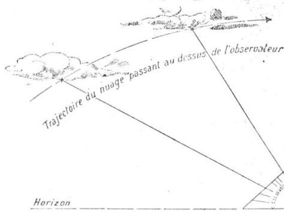
DÉTERMINATION DE LA TRAJECTOIRE D'UN NUAGE PASSANT AU-DESSUS DE L'OBSERVATEUR
