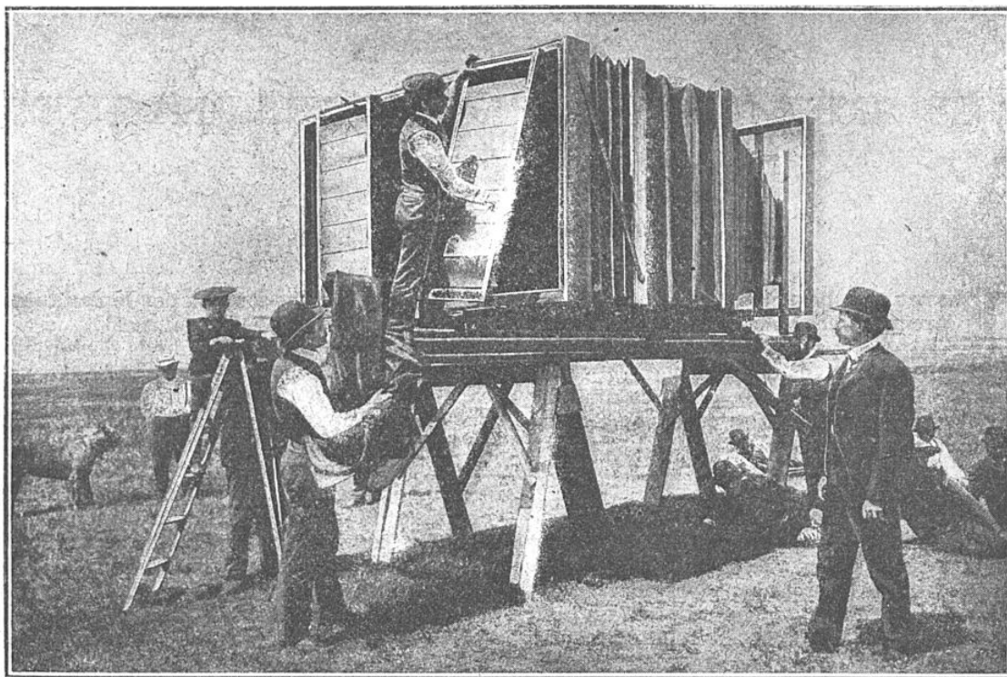
POSE DES CHASSIS EN BOIS DESTINÉS A ABRITER LA PLAQUE SENSIBLE
