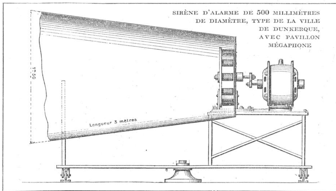
D'après le constructeur, cette sirène donne au son une portée de 7 à 8 kilomètres. Le montage sur un socle à pivot et sur un bâti muni de roulettes permet à l'appareil de faire un tour complet d'horizon.
