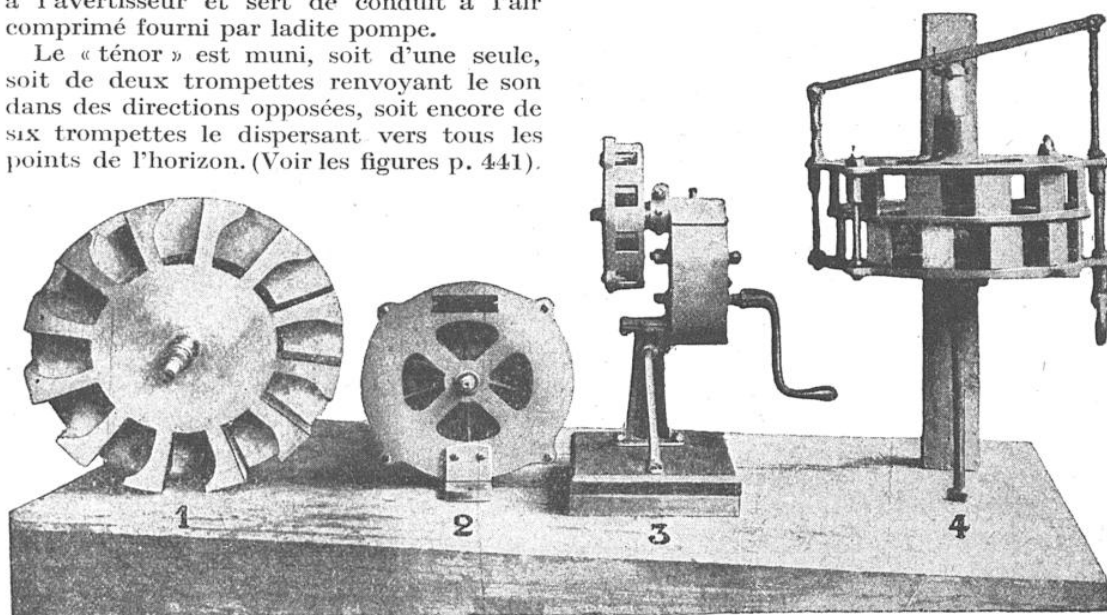
PIÈCES DÉTACHÉES ET MODÈLES DIVERS DE SIRÈNES DU SYSTÈME CHOLLET
