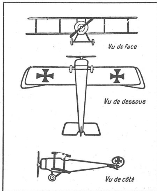
CARACTÉRISTIQUES DE L'AGO D-I
