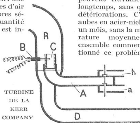
C, chambre de combustion, de petites dimensions; A, chambre; a et h, tubes d'arrivée de l'air et des vapeurs d'hydrocarbure; B, bougie d'allumage; D, arrivée de l'air comprimé (D et h aboutissent au même compresseur); R, chambre de refroidissement.
