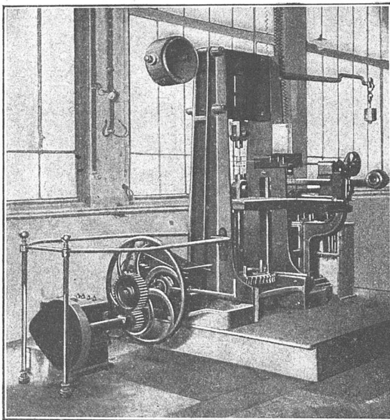
MACHINE TRAYVOU POUR DÉTERMINER LE DEGRÉ D'ÉLASTICITÉ ET D'ALLONGEMENT DES MÉTAUX
