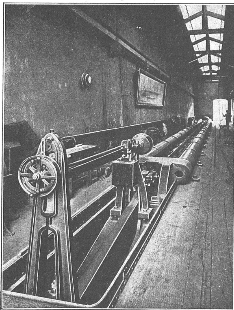
MACHINE A ESSAYER LES CHAINES PAR TRACTION DIRECTE
