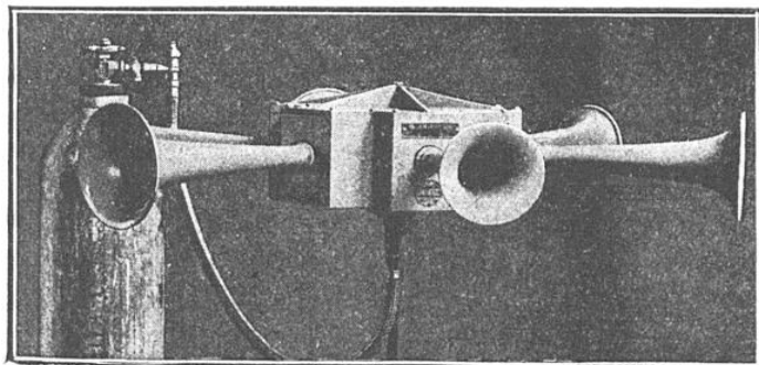
LE « TÉNOR » CHOLLET A SIX PAVILLONS Cet appareil multiple envoie des sons dans toutes les directions.
