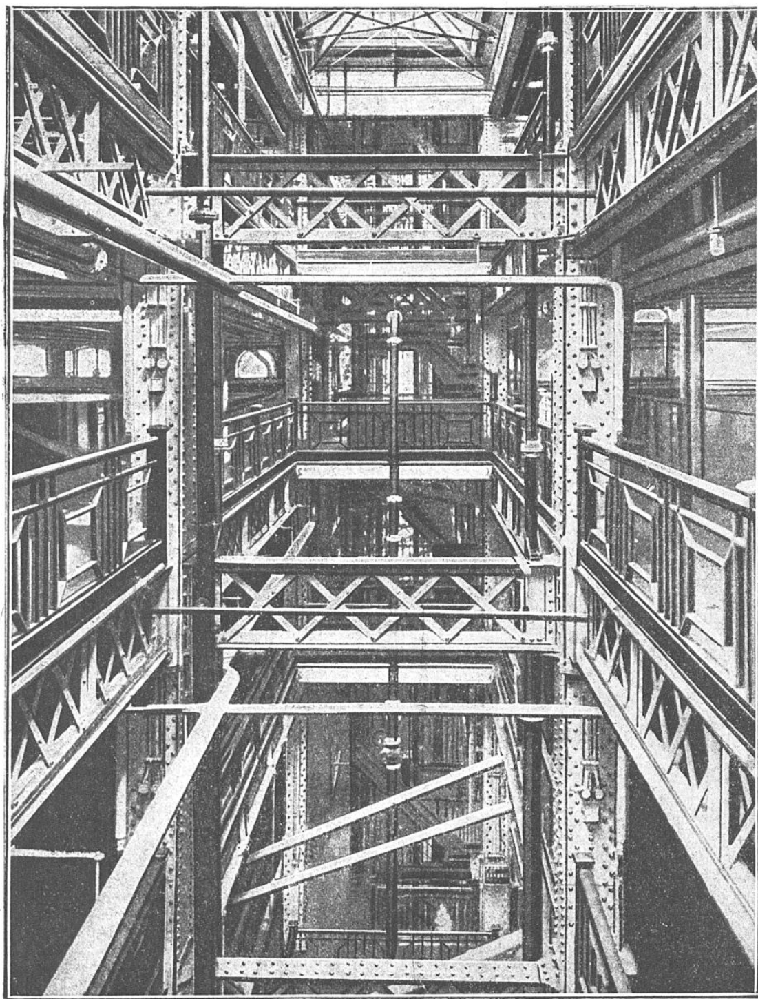
VUE PRISE A L'INTÉRIEUR DE LA BRASSERIE ARTHUR GUINNESS, A DUBLIN
