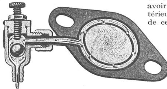
FIG. 2. — TOURBILLON INJECTÉ DANS LA TUBULURE D'ASPIRATION POUR RENDRE PLUS INTIME L'ASSOCIATION DES MOLÉCULES D'AIR ET D'ESSENCE
