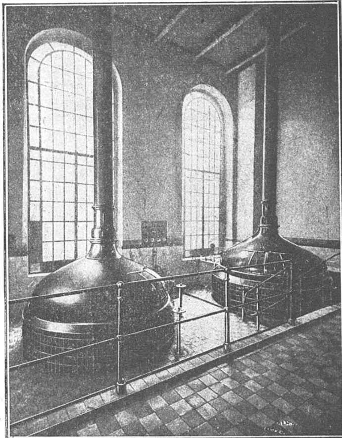
CHAUDIÈRES EN CUIVRE POUR CUIRE LE MOUT
