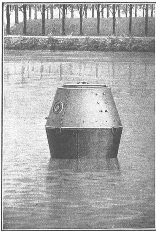
ESSAI DE FLOTTABILITÉ DE LA BOUÉE Chargée d'un poids de 225 kilos, représentant le poids de trois adultes, la bouée flotte dans d'excellentes conditions.
