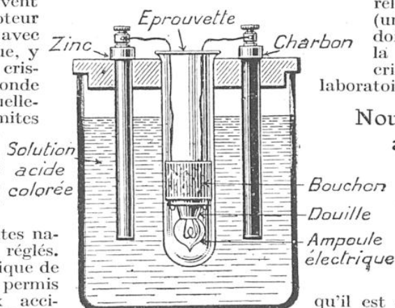
SCHÉMA INDICATIF DE LA CONSTRUCTION D'UNE PILE-LAMPE ÉLECTRIQUE
