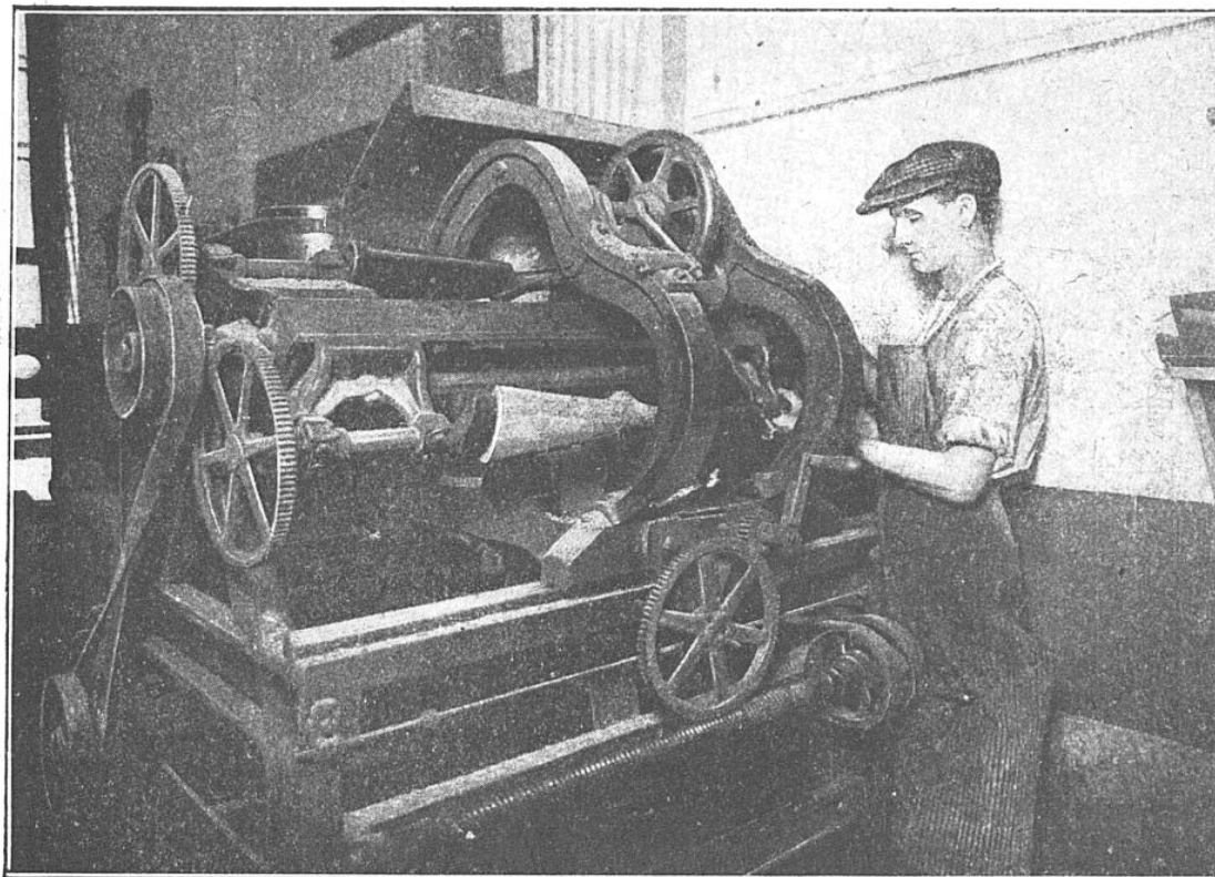
LES CROSSES SONT OBTENUES AU TOUR EN DE GRANDES QUANTITÉS
