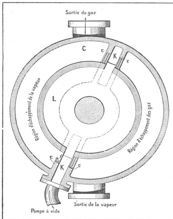
TURBINE SYSTÈME CHASSELOUP-LAUBAT c c, cloisons ménagées dans le canal annulaire C; L, cavité annulaire intérieure en communication constante avec les deux compartiments K.
