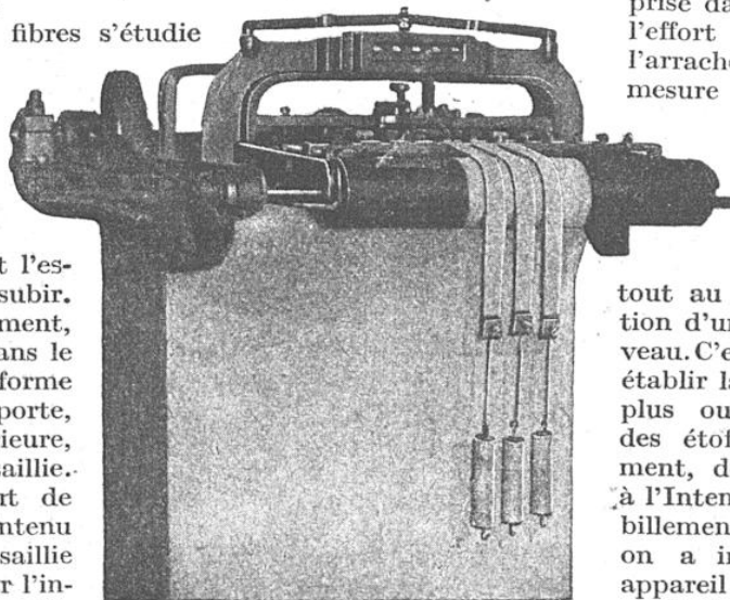
MACHINE A USER LES ÉTOFFES
