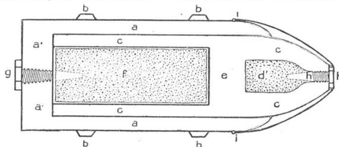
L'OBUS-CANON BAZIN DANS LA PREMIÈRE PARTIE DE SA TRAJECTOIRE
