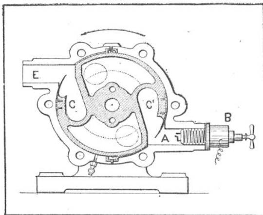
AUTRE MODÈLE DE TURBINE A RÉACTION
