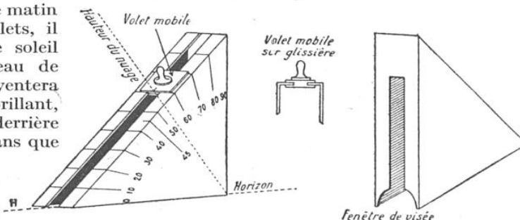
L'ÉQUERRE CÉLESTE, VUE AVANT ET VUE ARRIÈRE (On trouvera la description de ce petit instrument dans le texte.)
