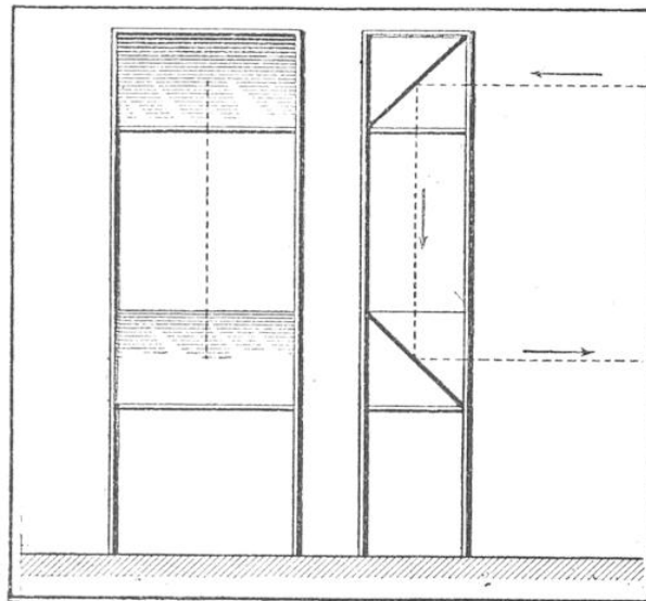
VUE DE FACE ET DE PROFIL DU PÉRISCOPE DE TRANCHÉES CONNU EN 1870
