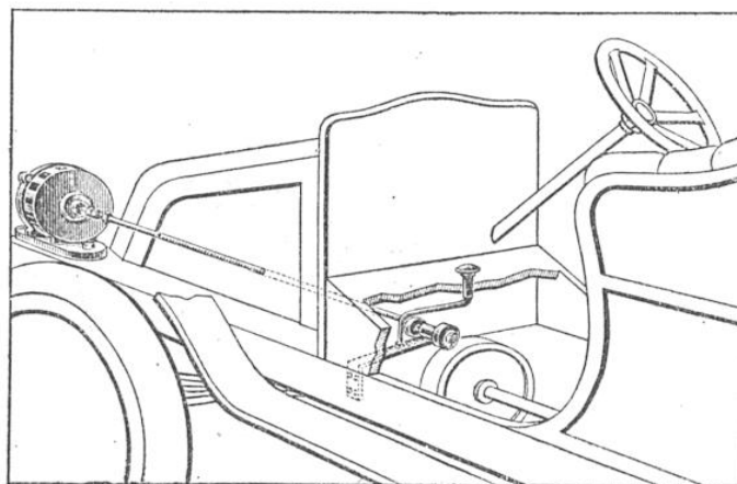
INSTALLATION D'UNE SIRÈNE SUR UNE AUTO DES SAPEURS-POMPIERS DE LA VILLE DE PARIS
