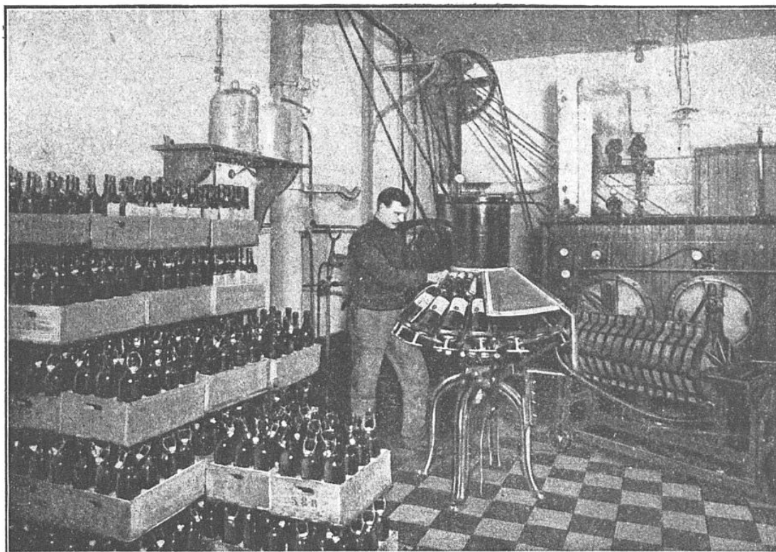
LE REMPLISSAGE AUTOMATIQUE DES CANETTES DE BIÈRE
