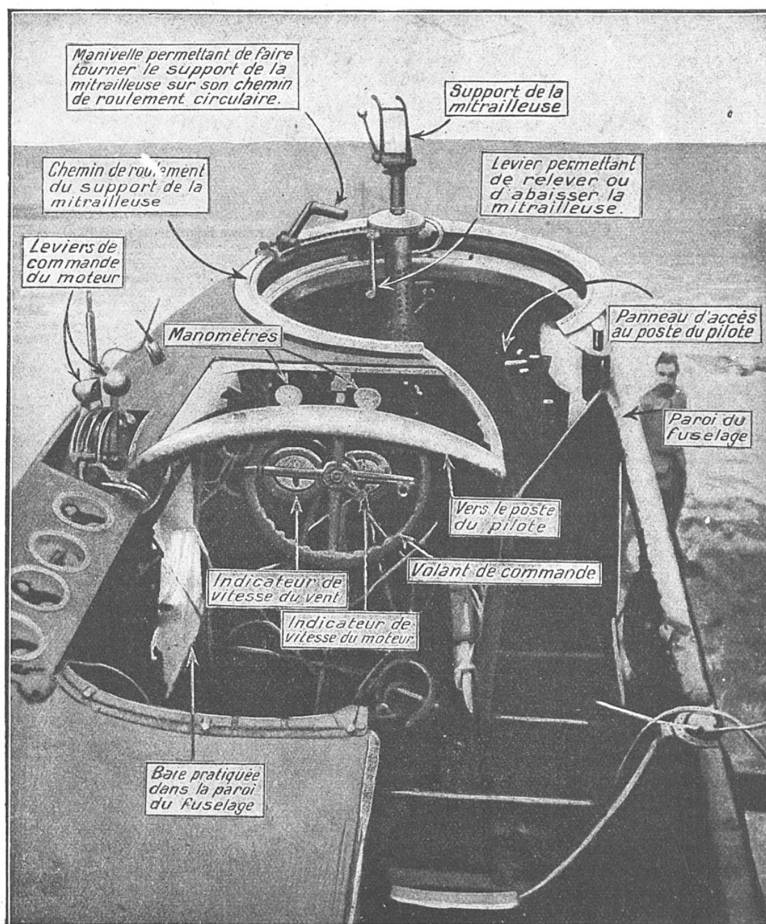
DISPOSITION DES APPAREILS ET DES ENGIN A L'AVANT DE LA CARLINGUE D'UN GOTHA
