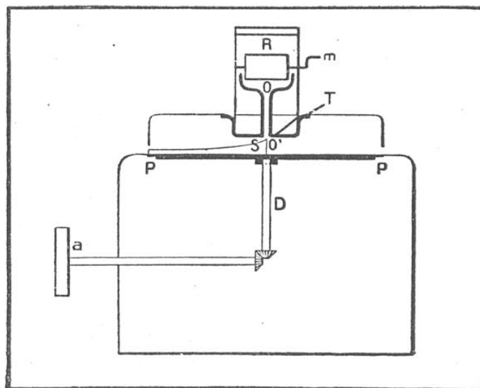
FIGURE SCHÉMATIQUE DE LA MITRAILLEUSE A FORCE CENTRIFUGE LANÇANT 400 BALLES A LA MINUTE
