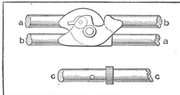
CHARNIÈRE DU CHEVAL DE FRISE MOBILE
