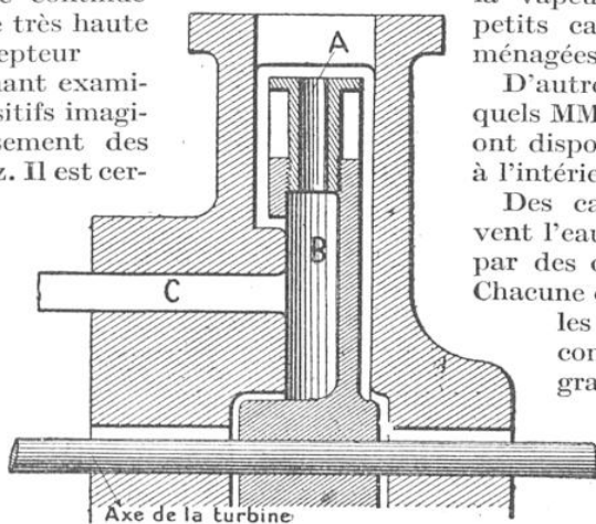
DISPOSITIF DE LA TURBINE FULLAGAR
