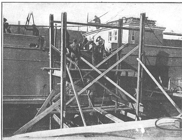
LES DEUX MOITIÉS DU BATEAU SONT RACCORDÉES PAR UNE CEINTURE EN TOLE D'ACIER BOULONNÉE
