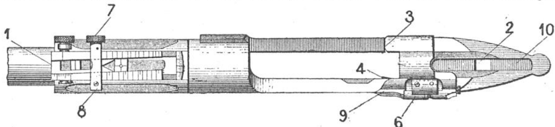
LA HAUSSE ET LA BOÎTE DE CULASSE DU SPRINGFIELD
