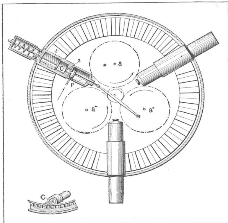
TURBINE A GAZ SYSTÈME FASBENDER
