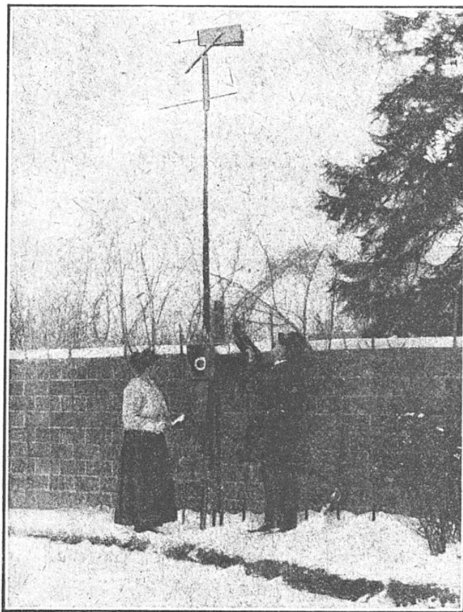
MODE D'OBSERVATION POUR LA PRÉVISION DU TEMPS
