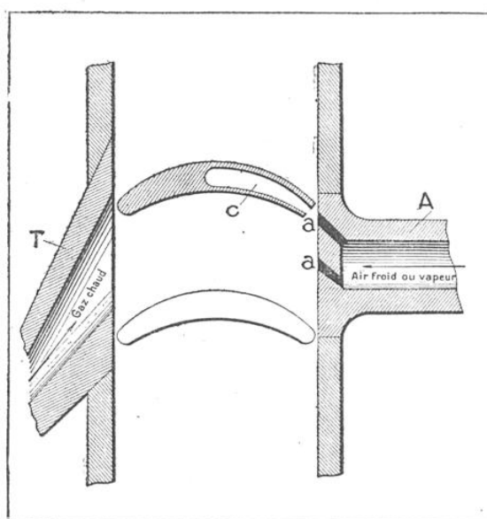
COUPE D'UNE AUBE A CIRCULATION D'EAU
