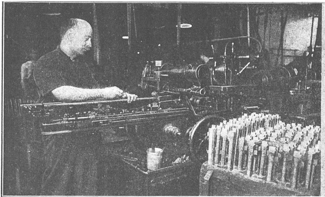
L'ALÉSAGE DU CANON D'UN FUSIL AMÉRICAIN SPRINGFIELD, MODÈLE 1914
