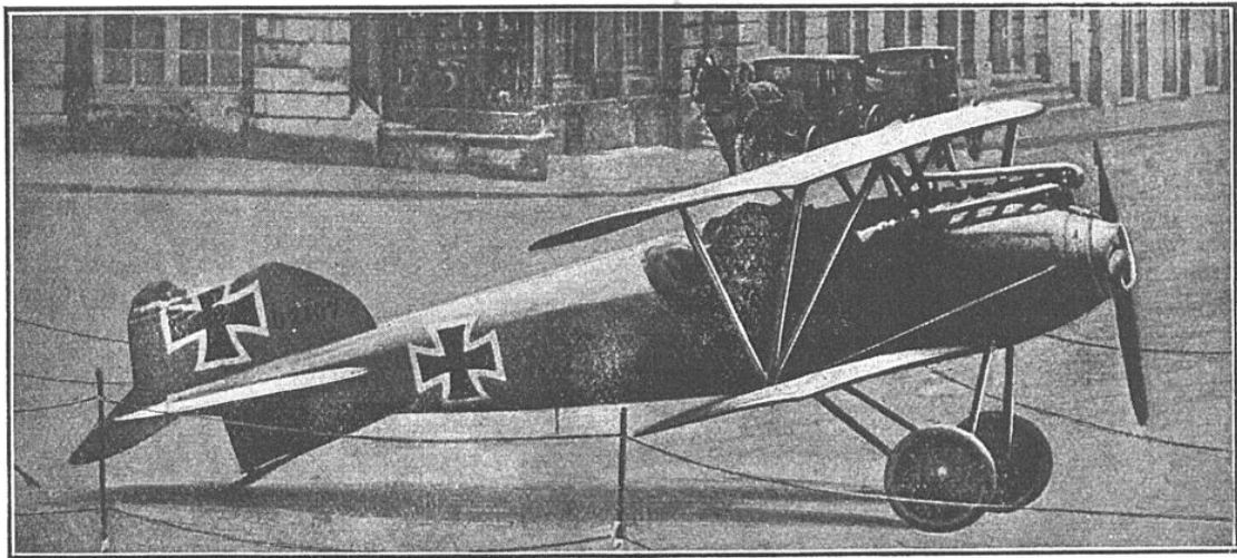
HALBERSTADT DE 160 CHEVAUX CAPTURÉ DANS LA RÉGION DE RAMBERVILLERS
