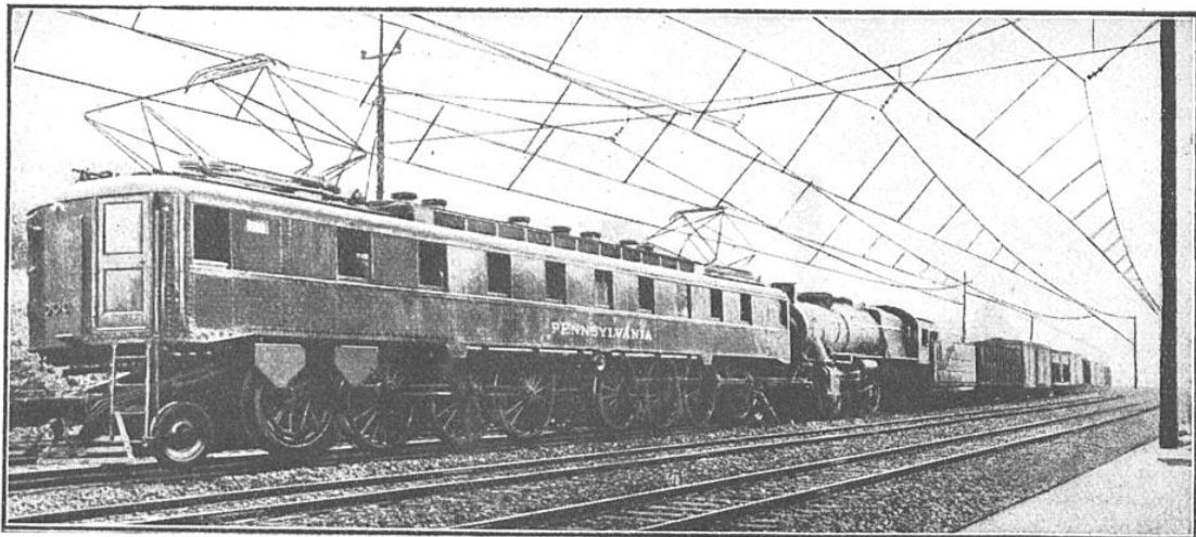
CETTE MACHINE GÉANTE PÈSE 240 TONNES ET MESURE 25 MÈTRES DE LONG Elle a été étudiée et construite aux Etats-Unis pour remorquer les trains de marchandises lourdement chargés dans des régions particulièrement accidentées.
