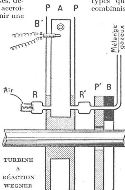
TURBINE A RÉACTION WEGNER A, tube cylindrique (ces tubes sont au nombre de quatre) ; PP, plateaux circulaires ; RR', réservoirs dont l'un, R, destiné à l'admission de l'air, est muni d'un clapet (R' est prolongé par un tube s'engageant dans le plateau P' tournant avec l'ensemble) ; B, pièce fixe formant distributeur ; B', bougies d'allumage.
