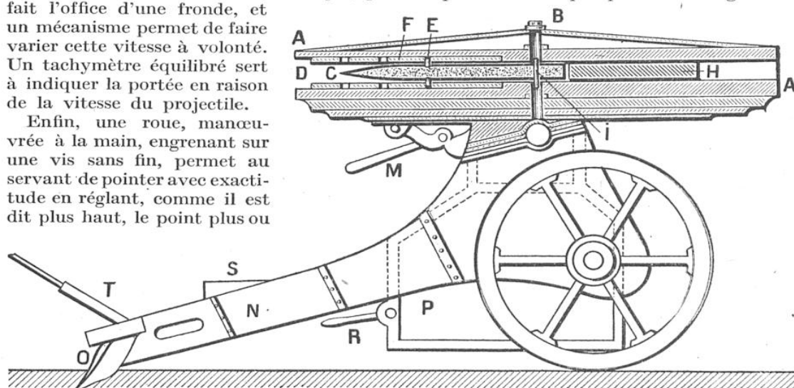
CANON CENTRIFUGE SYSTÈME BEZOBRAZOFF (ÉLÉVATION ET COUPE PARTIELLE)
