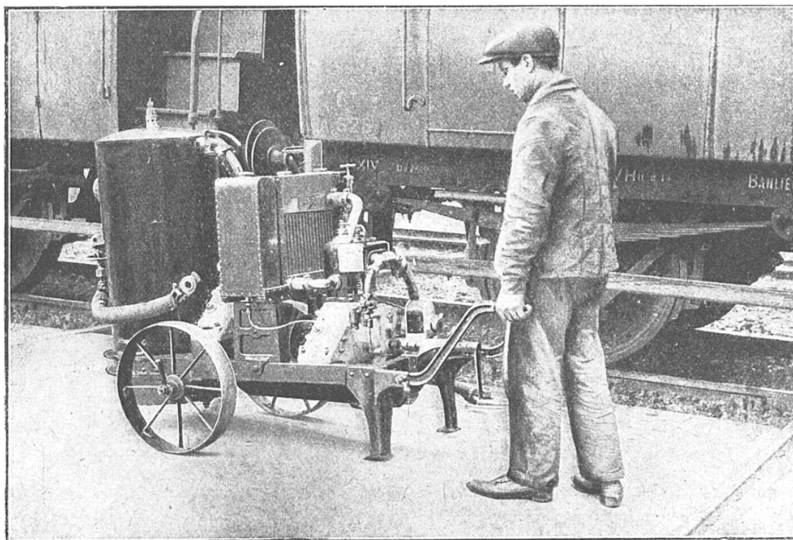
LE GROUPE COMPRESSEUR CAMPAGNE SE TRANSPORTE SUR UNE BROUETTE
