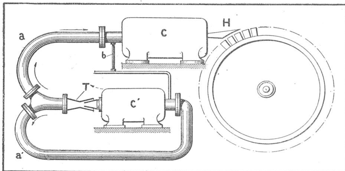
FIGURE SCHÉMATIQUE D'UN COMPRESSEUR A TROMPE
