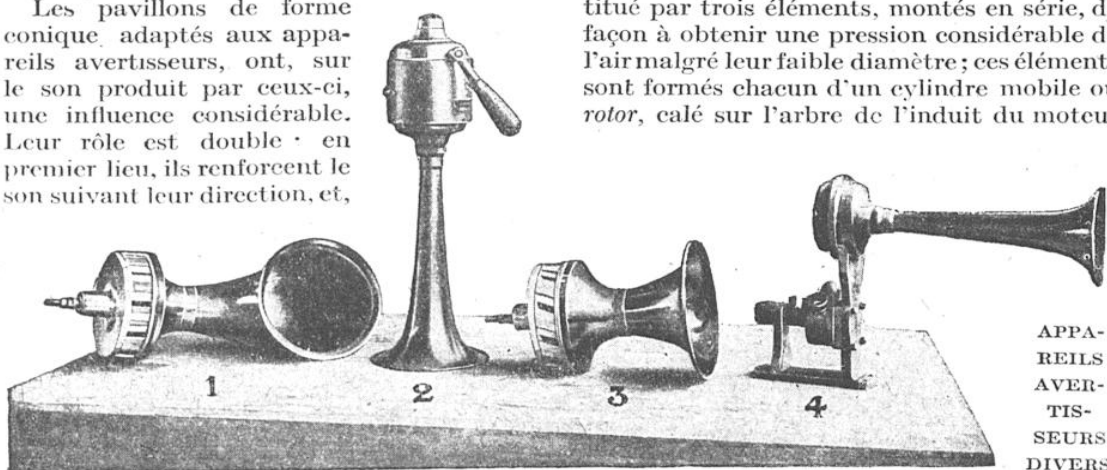
1, sirène à conque pour canot automobile; 2, « ténor » à levier pour camion militaire; 3, sirène à double pavillon renvoyant tout le son vers l'avant; 4, « ténor » monté sur pompe à air.
