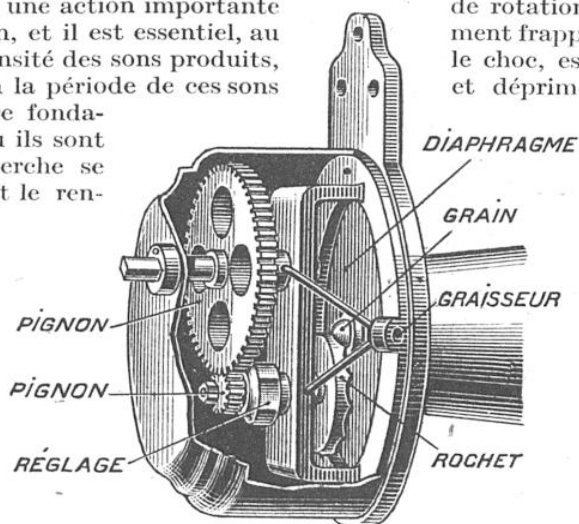
MÉCANISME PRODUCTEUR DU SON DU « KRACFORT » DESPONTS
