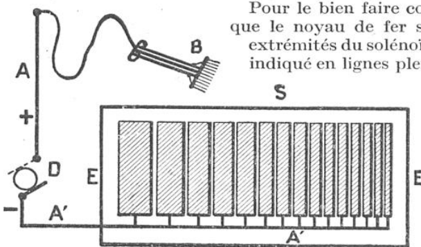
FIGURE SCHÉMATIQUE POUR LA DÉMONSTRATION DU FONCTIONNEMENT DU COMMUTATEUR D'UN CANON ÉLECTRO-MAGNÉTIQUE « WOLTERECK »
