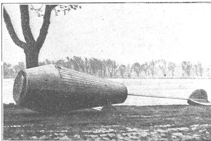
BOUÉE TOUTE MONTÉE ET MUNIE, DANS SON AXE, DE SA QUEUE STABILISATRICE
