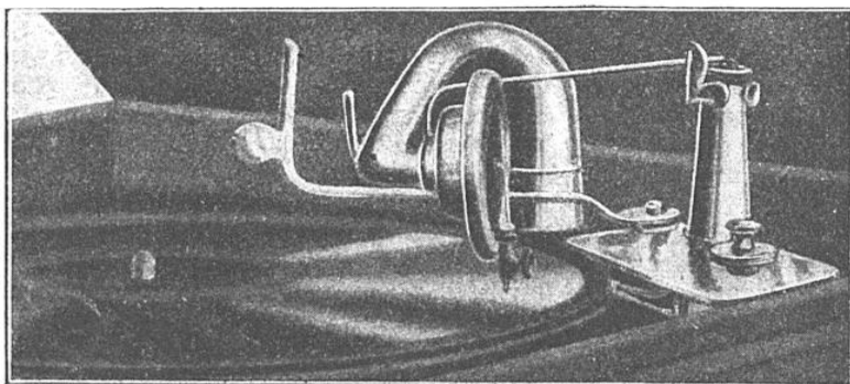
DISPOSITIF REPLAÇANT AUTOMATIQUEMENT L'AIGUILLE OU LE SAPHIR DU DIAPHRAGME DES PHONOGRAPHES
