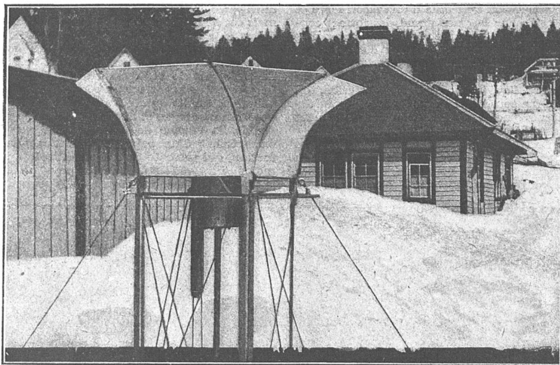
« NEIGÉOMÈTRE » DU PROFESSEUR MARVIN, INSTALLÉ A BLUE CANYON (CALIFORNIE)
