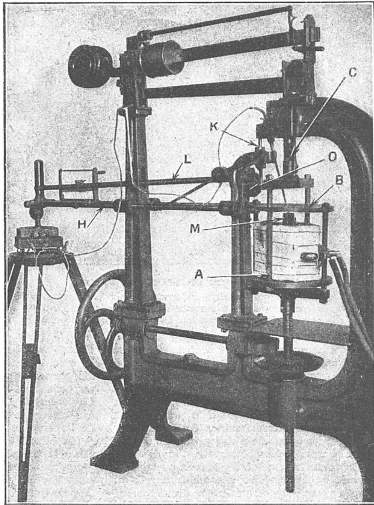
APPAREIL D'ÉCRASEMENT A HAUTE TEMPÉRATURE
