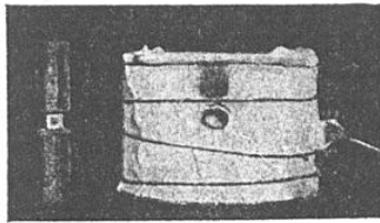
FOUR A FLAMME SPIRALÉE A gauche, on voit, entre deux mandrins, l'éprouvette à écraser.
