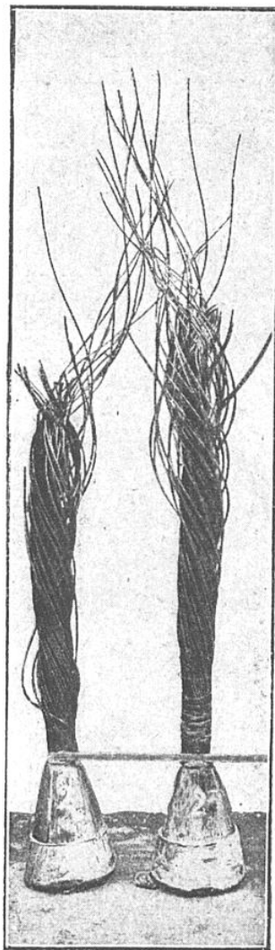
CABLES MÉTALLIQUES ROMPUS
