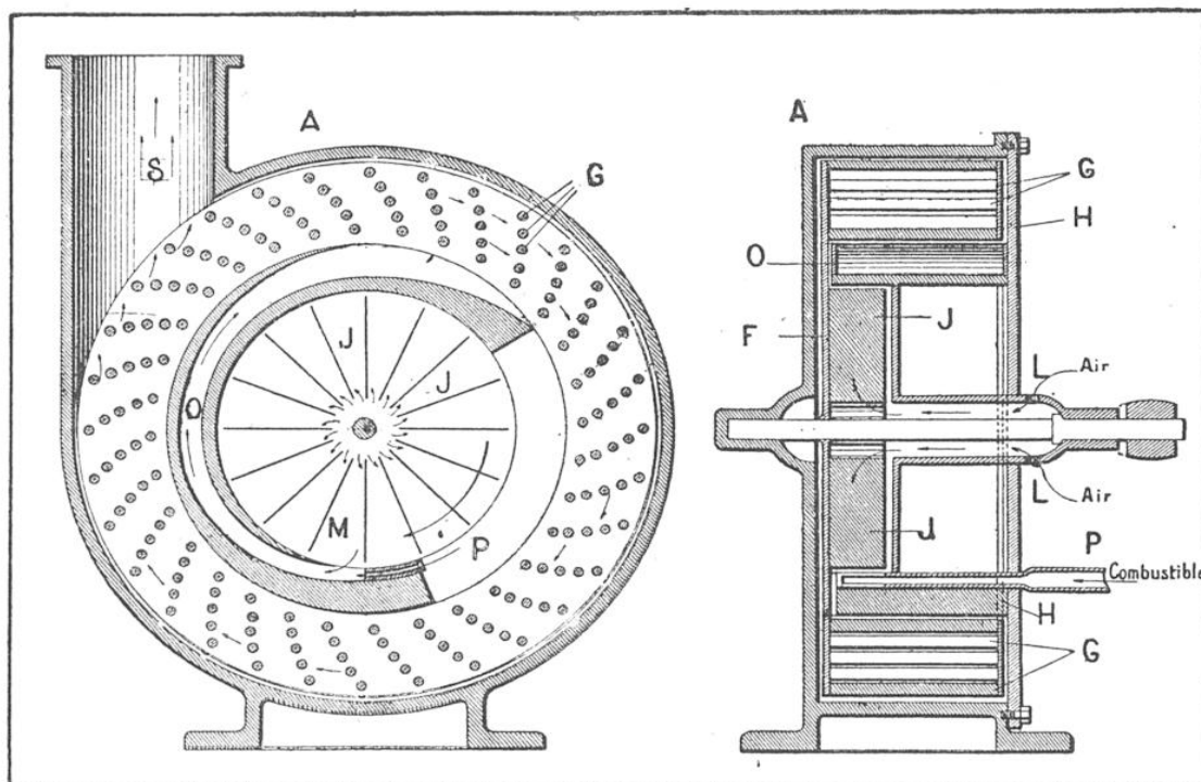
AUTRE MODÈLE DE TURBINE A GAZ DU SYSTÈME KARAVODINE
