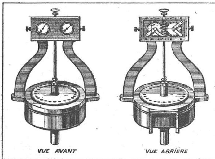
SIRÈNE CAGNIARD-LATOUR, AVEC SES DEUX CADRANS COMPTEURS DE TOURS
