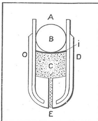
TORPILLE AÉRIENNE (1871)
