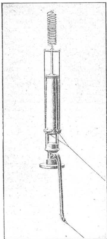
LE NOUVEAU SIFFLET A MODULATIONS SYSTÈME MAUGARS-BÉRANGÉ
