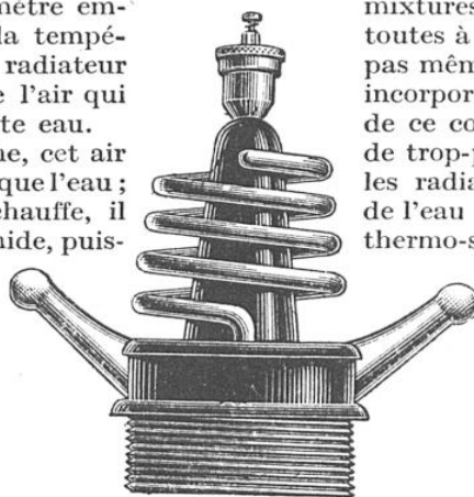
CET APPAREIL CONDENSE DANS LE RADIATEUR LA VAPEUR D'EAU ET, ÉVENTUELLEMENT, D'ALCOOL
