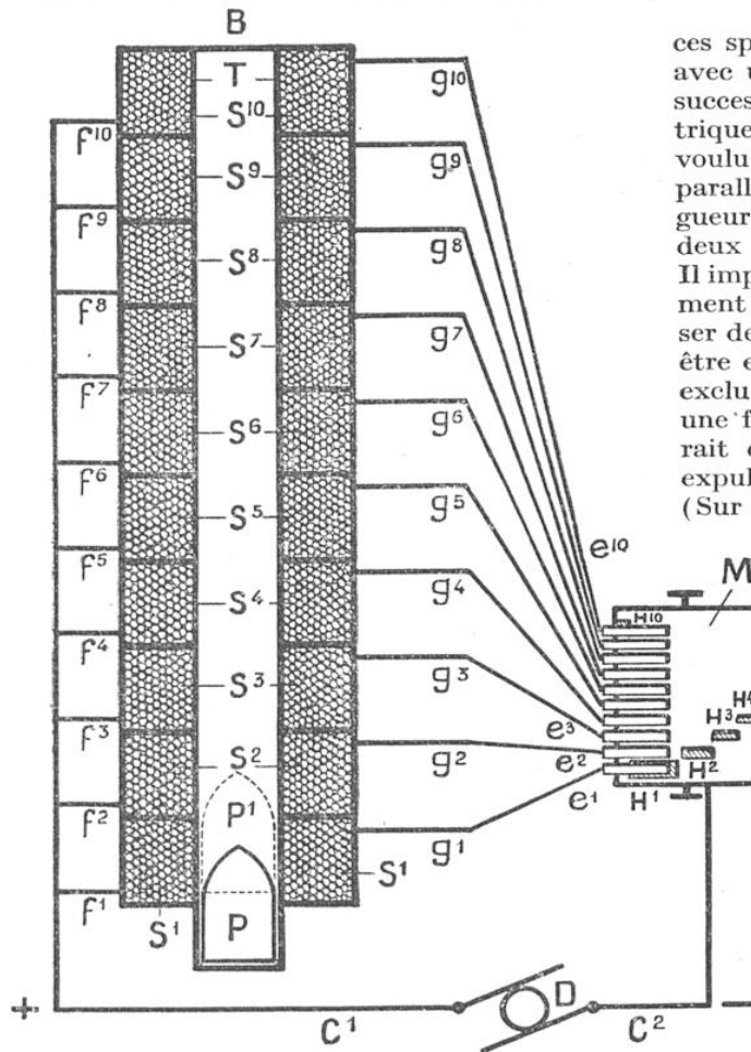
SCHEMA DU CANON ÉLECTRO-MAGNÉTIQUE DE M. WOLTERECK ET DE SON COMMUTATEUR
