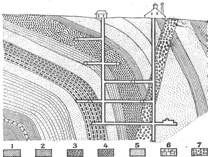
COUPE DU GISEMENT DE MERCURE DÉCOUVERT AU LIEU DIT SOPHIA, DANS LE BASSIN HOUILLER DU DONETZ
