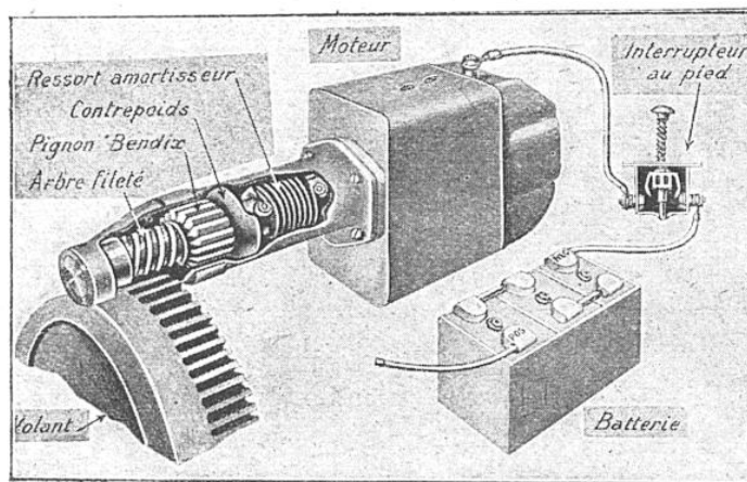
FIGURE MONTRANT LE FONCTIONNEMENT DU DÉMARREUR ÉLECTRIQUE GRADA
