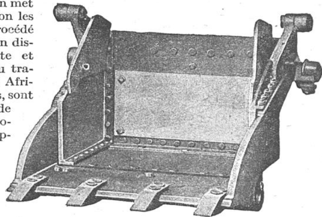
VUE DE FACE DE LA PELLE D'UNE MACHINE A DÉROCHER MODÈLE N° 4
