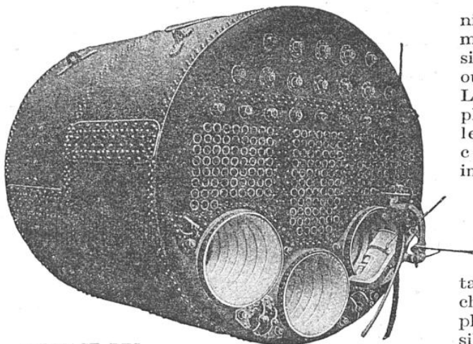
RIVETAGE DES CADRES DU FOYER D'UNE CHAUDIÈRE MARINE
