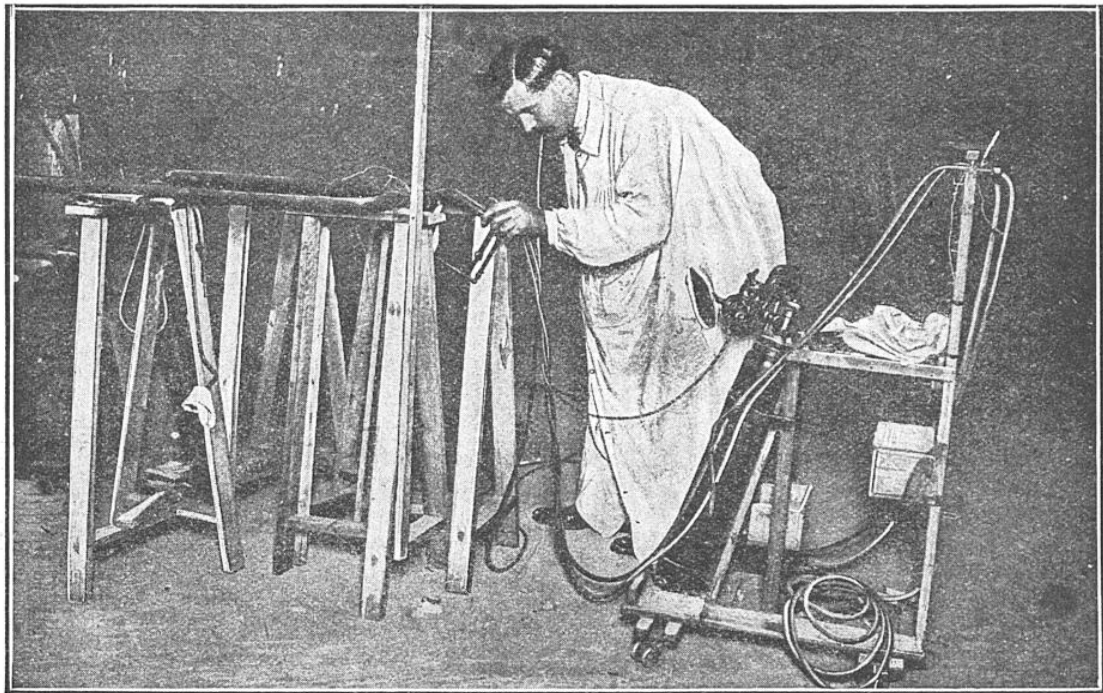
CONTOURNAGE, AU MOYEN DU CHALUMEAU, DES TUBES-PUBLICITÉ AU NÉON
