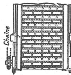
PORION EXTRÊME, VUE EN PLAN, DU TRANSPORTEUR A TABLIER MÉTALLIQUE
