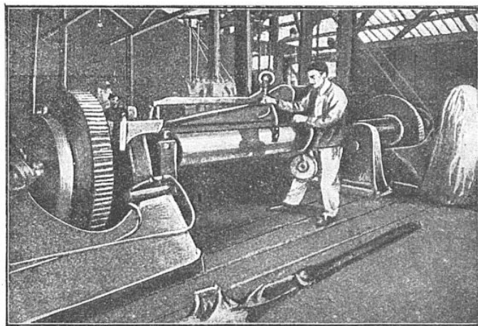
DÉROULEUSE DÉBITANT EN FEUILLES EXTRA-MINCES UN TRONC D'OKOUMÉ
