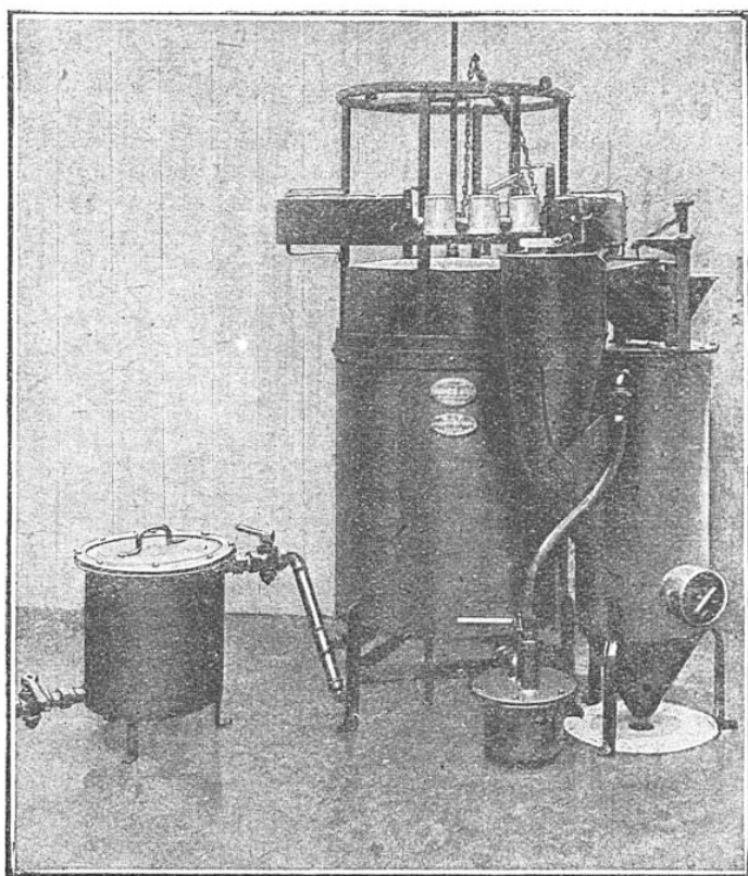
APPAREIL SYSTÈME JAVAL, COMPLET Cet appareil à acétylène comporte un générateur à chute automatique de carbure dans l'eau et un épurateur.
