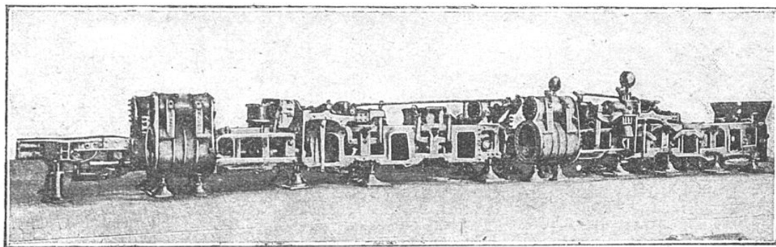
CYLINDRES AVANT ET MILIEU MONTÉS SUR LEUR LONGERONS RESPECTIFS
