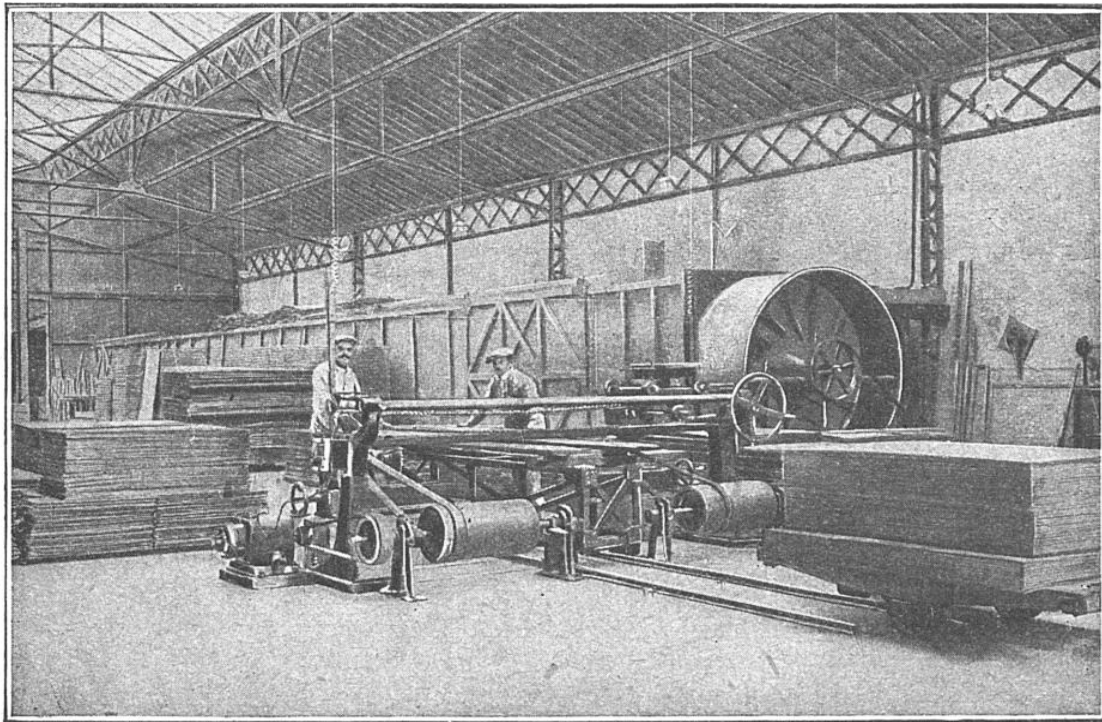
SCIE SERVANT A DÉLIGNER LES PLATEAUX, EN PLEIN FONCTIONNEMENT
