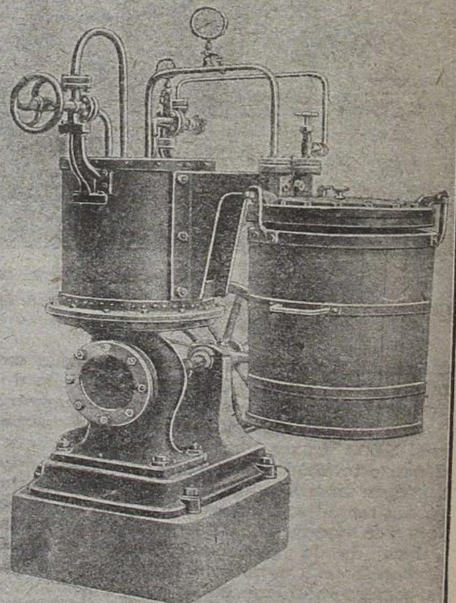
APPAREIL DOUANE A CARTOUCHE INSTANTANÉE POUR LA FABRICATION DE LA GLACE 1, la machine en marche ; 2 et 3, avant et pendant le démoulage ; 4, le même appareil plus grand.
