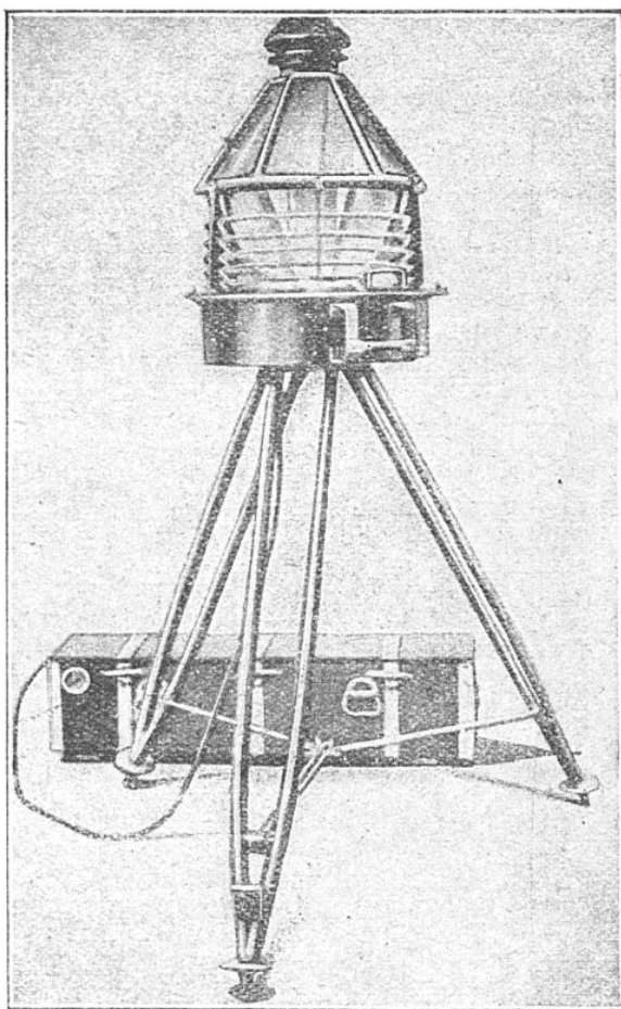
PHARE A ACÉTYLÈNE DISSOUS
