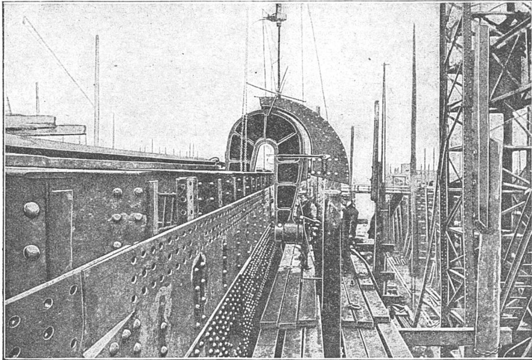
ÉQUIPE D'OUVRIERS POSANT DES RIVETS SUR LA CARÈNE D'UN PAQUEBOT
