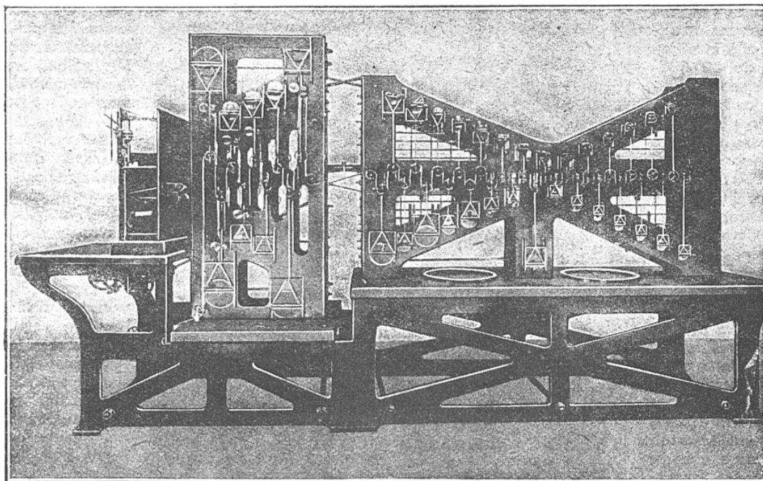
MACHINE A PRÉDIRE LES MARÉES, DU SERVICE HYDROGRAPHIQUE AMÉRICAIN
