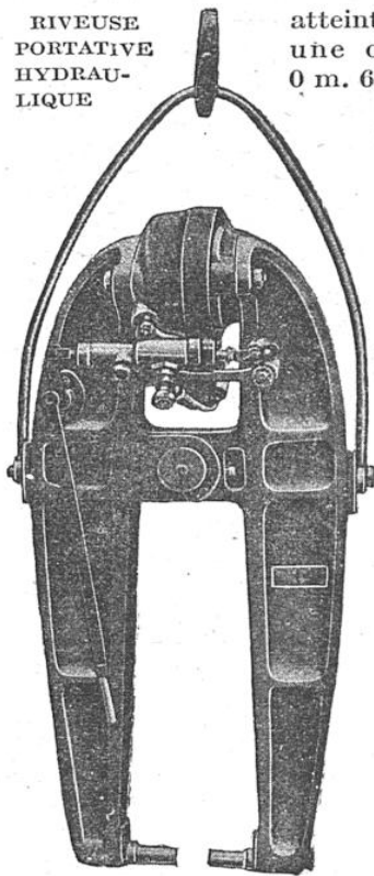
Cette machine, système Felding, est simplement suspendue au crochet d'une grue.
