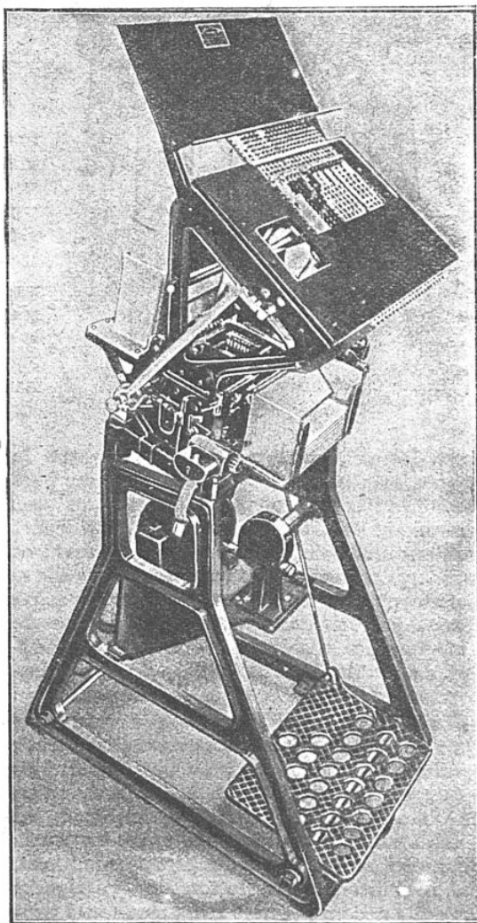
FIG. 10. — MACHINE A PERFORER LES CARTES
