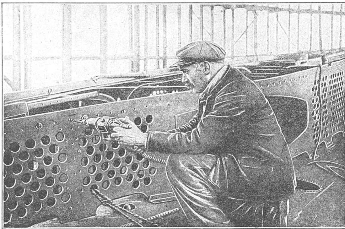
PERÇAGE DE TROUS DE RIVETS AU MOYEN D'UN FORET A AIR COMPRIMÉ
