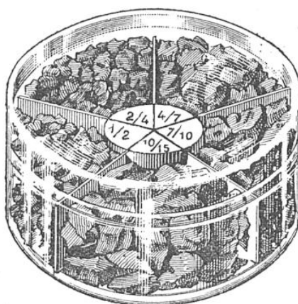
CARBURE DE CALCIUM GRANULÉ DE DIFFÉRENTES GROSSEURS
