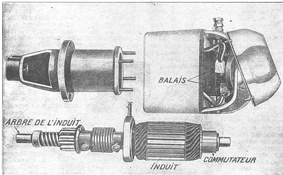
VUE D'UN DÉMARREUR ÉLECTRIQUE, TYPE GRADA, DÉMONTÉ EN TROIS PARTIES
