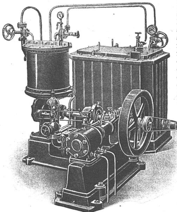
GROUPE FRIGORIGÈNE SYSTÈME DOUANE
