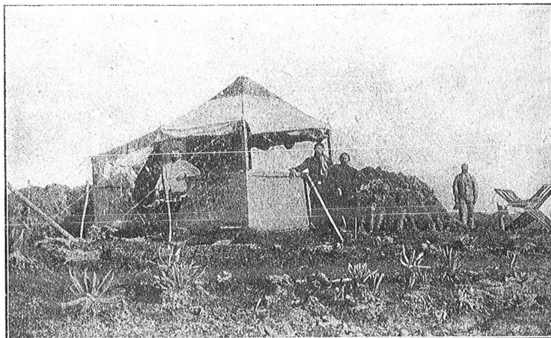
BARAQUE GÉODÉSIQUE ÉDIFIÉE POUR LES OBSERVATIONS A TULCAN (ÉQUATEUR) Elle abritait contre les intempéries le pilier d'observation et le cercle azimuthal pour la mesure des angles.
