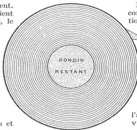
DÉBIT D'UN TRONC D'ARBRE PAR DÉROULAGE
