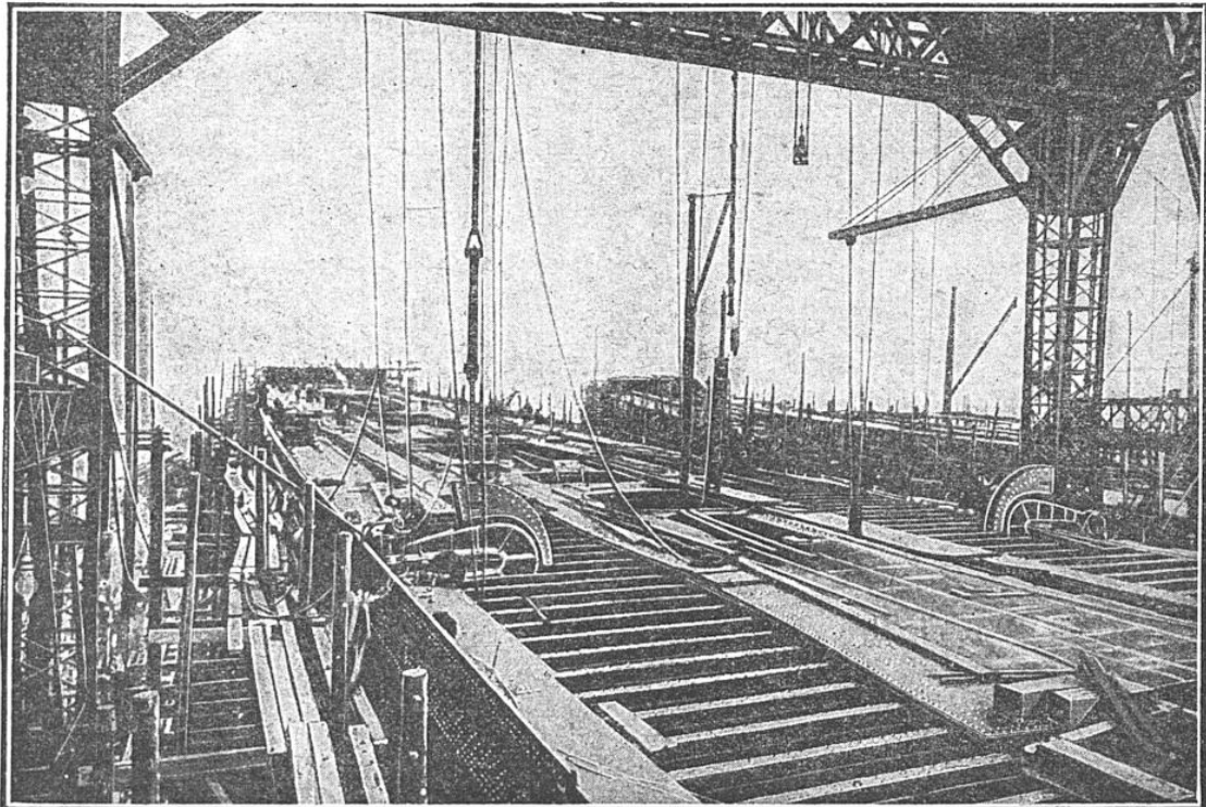
EMPLOI DES RIVEUSES A ACTION DIRECTE SUR UN PONT DE NAVIRE
