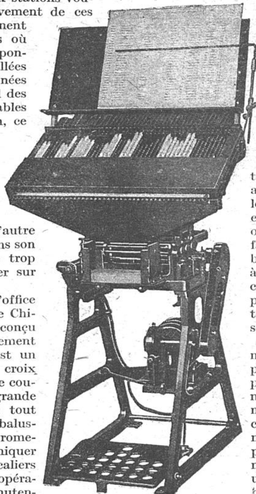
FIG. 13. — AUTRE SYSTÈME DE MACHINE A PERFORER
