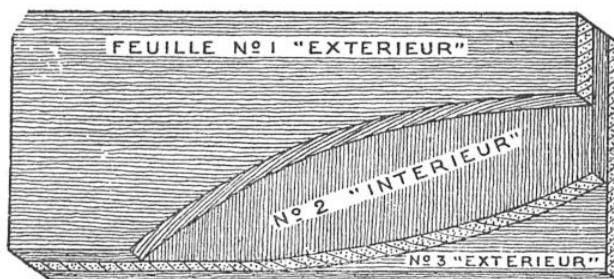
PANNEAU CONTRE-PLAQUÉ EN « TROIS PLIS »
