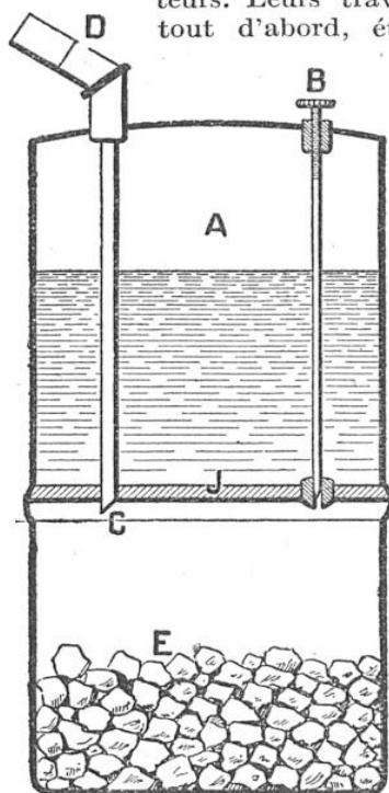
COUPE SCHÉMATIQUE D'UNE LAMPE DE MINE
