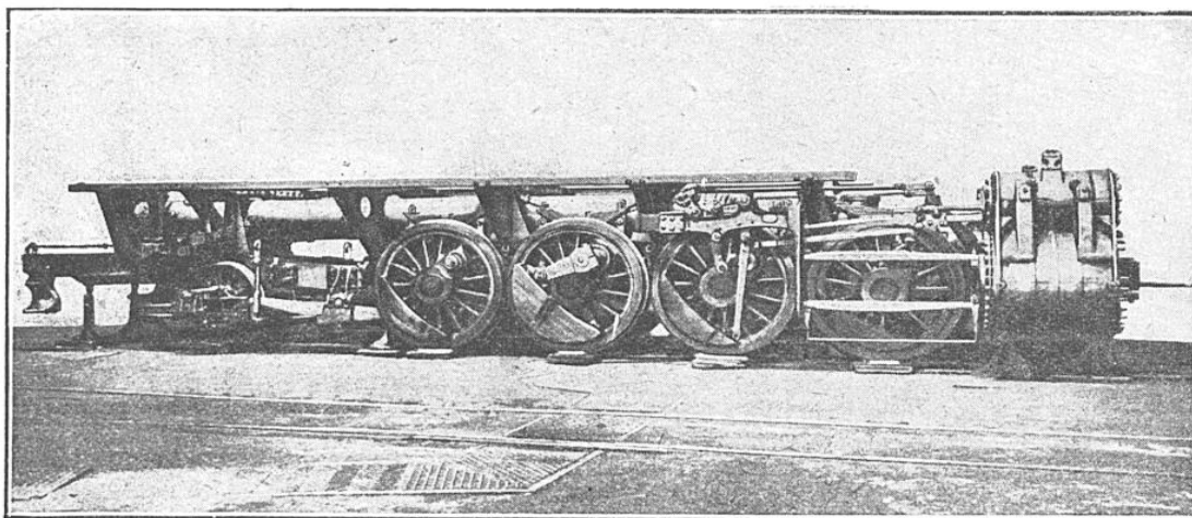
VUE DU GROUPE DE HUIT ROUES MOTRICES PLACÉES SOUS LE TENDER
