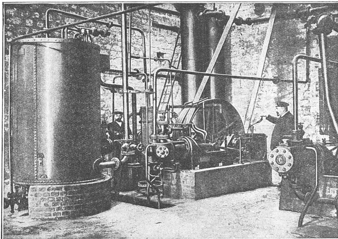
MACHINE DE COMPRESSION (A DROITE) ET GAZOMÈTRE (A GAUCHE)
