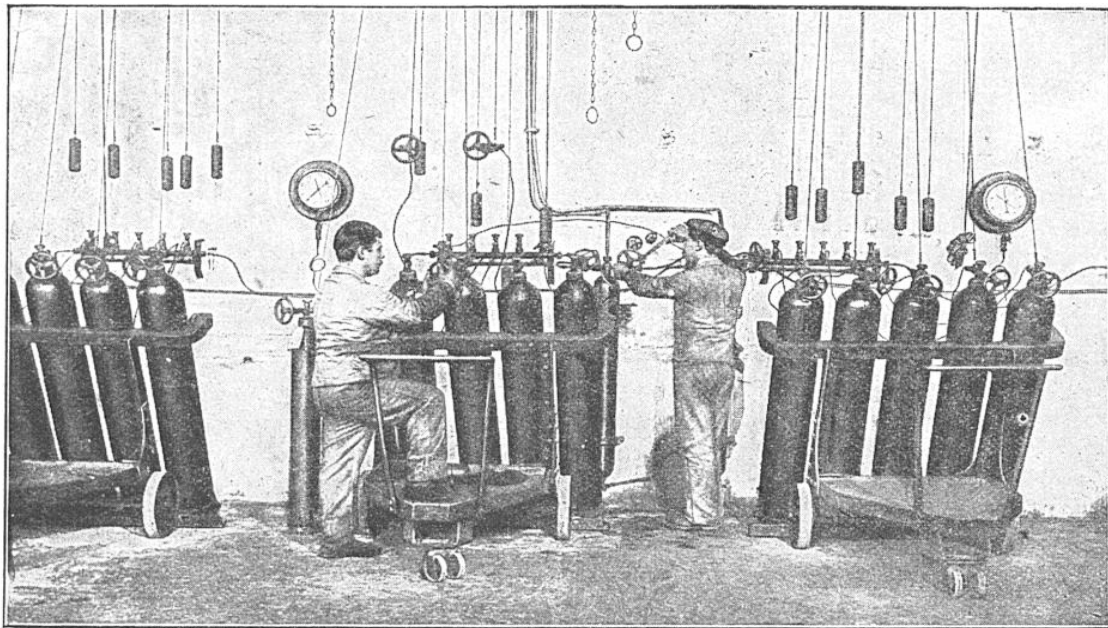
REMPLISSAGE DES CYLINDRES DE GAZ LIQUÉFIÉS (ACIDE CARBONIQUE ET AUTRES) Chaque poste permet de remplir en même temps cinq cylindres au moyen de tubes de petit diamètre.
