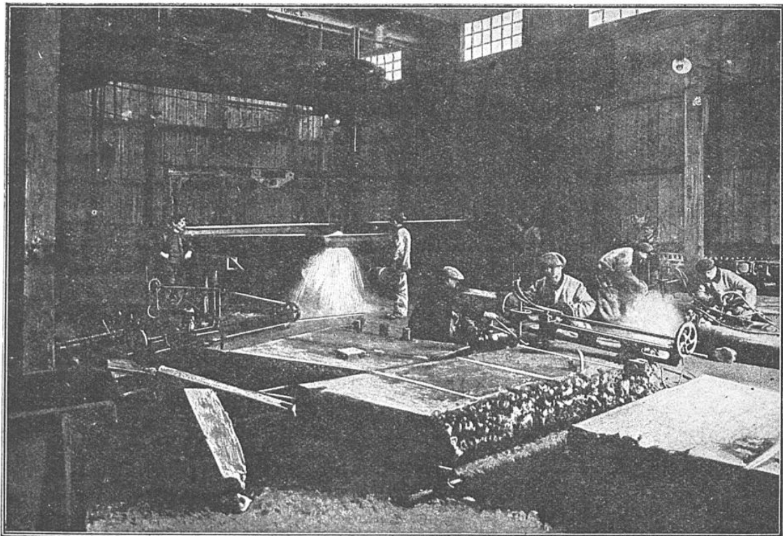
DÉCOUPAGE D'UNE PLAQUE DE BLINDAGE AU CHALUMEAU OXYACÉTYLÉNIQUE Cette opération, qui exigeait autrefois l'emploi de formidables machines-outils, se fait ainsi simplement.
