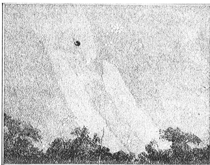
FIG. 8. — CE DESSIN PERMET DE JUGER DE L'INCOMPARABLE ÉCLAT DE L'ÉTOILE DU 8 JUIN
