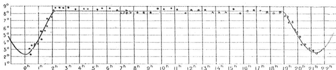
FIG. 3. — COURBE REPRÉSENTANT LA VARIATION D'ÉCLAT D'UNE ÉTOILE DU TYPE D'ALGOL.
