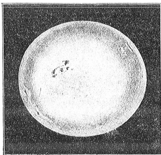
FIG. 2. — LE SOLEIL AVEC SES TACHES, VU DANS UNE LUNETTE ASTRONOMIQUE
