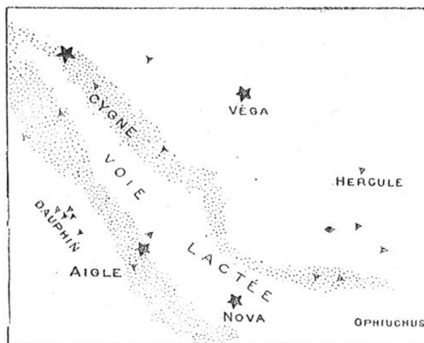
FIG. 7. — POSITION DE L'ÉTOILE NOUVELLE (« NOVA ») DANS LE CIEL
