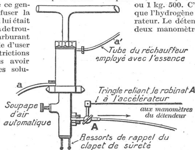
SCHÉMA DU MONTAGE DU CARBURATEUR CAUET Un carburateur spécial remplace le carburateur ordinaire. Il est disposé en dessous du réchauffeur, qui n'est pas utilisé, n'étant point nécessaire.
