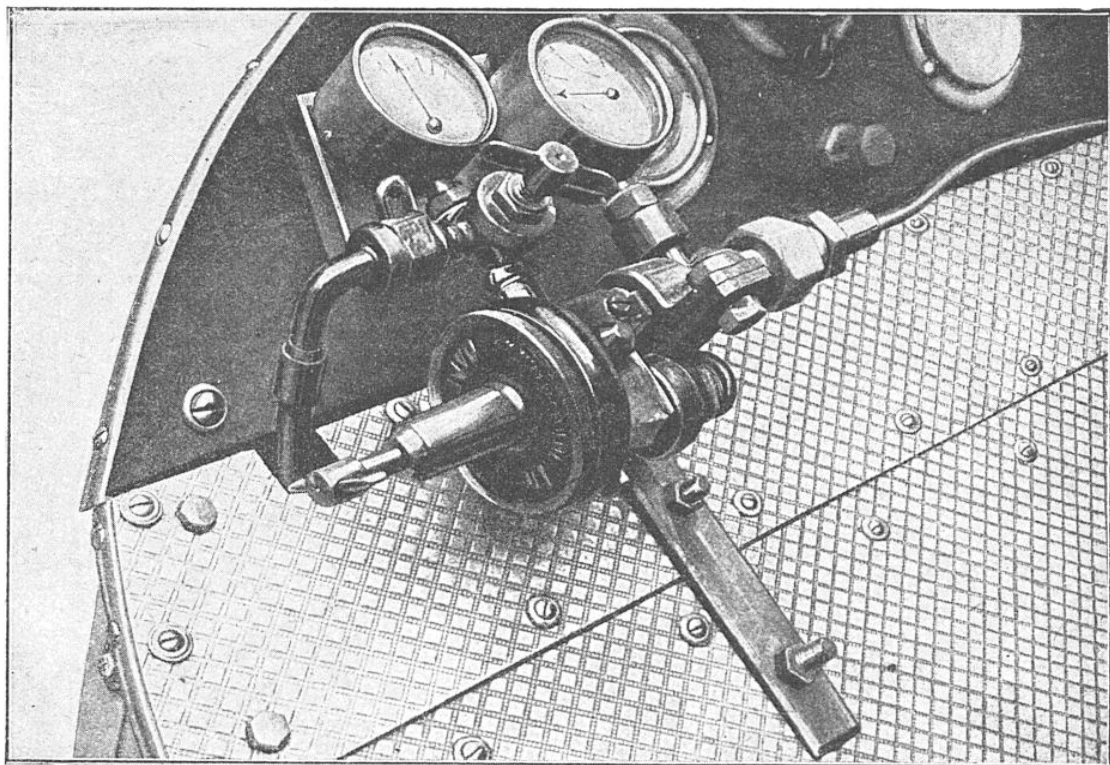
LE DÉTENDEUR EST FIXÉ SUR LA VOITURE, A PORTÉE DU CONDUCTEUR
