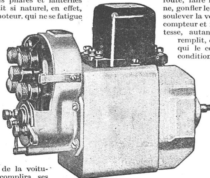
DYNAMO ALLUMEUSE ET GÉNÉRATRICE
