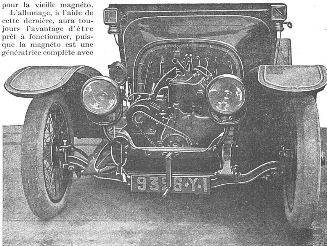
DÉMARREUR INSTALLÉ SUR UNE VOITURE D'UN ANCIEN MODÈLE
