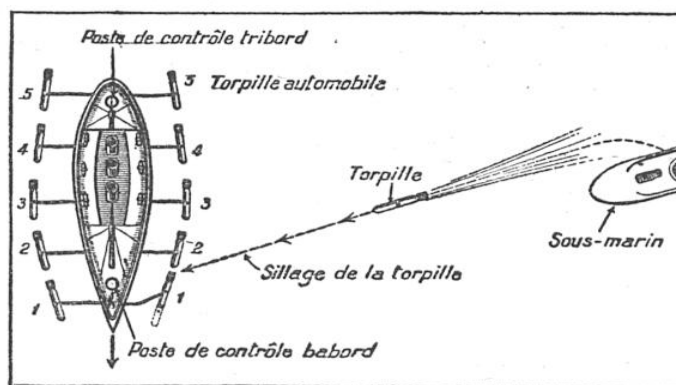
NAVIRE DE 180 MÈTRES DE LONGUEUR ENTOURÉ DE DIX TORPILLES AUTOMOBILES PROTÉCTRICES
