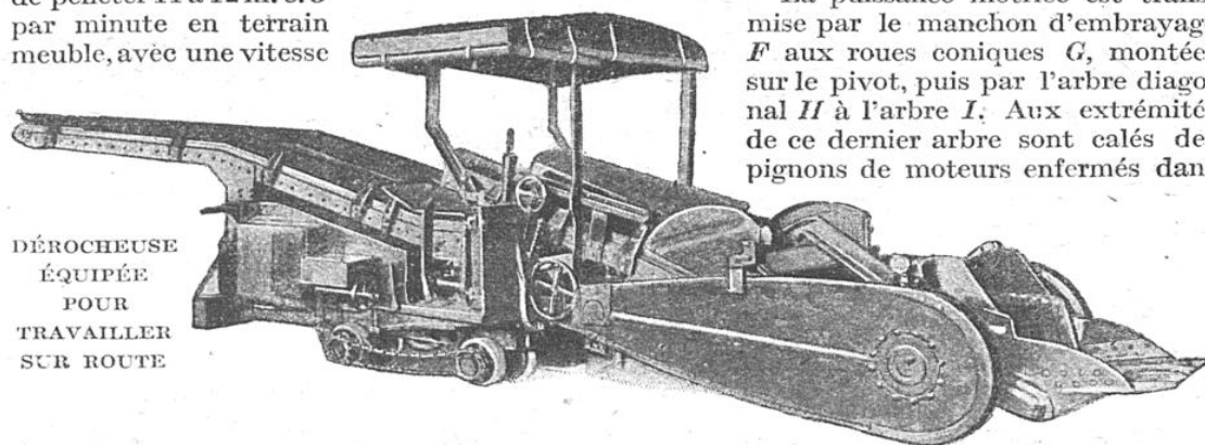
Ce modèle est muni d'un abri servant à protéger le conducteur. Avec un seul homme et une dépense de 22 kilowatts-heures par tonne manutentionnée, on obtient un rendement de 200 à 400 tonnes par poste. C'est le travail ordinaire de 15 à 20 ouvriers vigoureux dans les mines de la vieille Europe.
