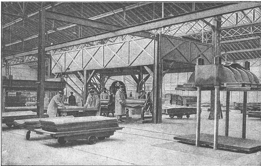
VUE GÉNÉRALE DE L'ATELIER OU S'EFFECTUE L'ENCOLLAGE DES PANNEAUX Au second plan, on voit les cylindres des machines servant à l'encollage.
