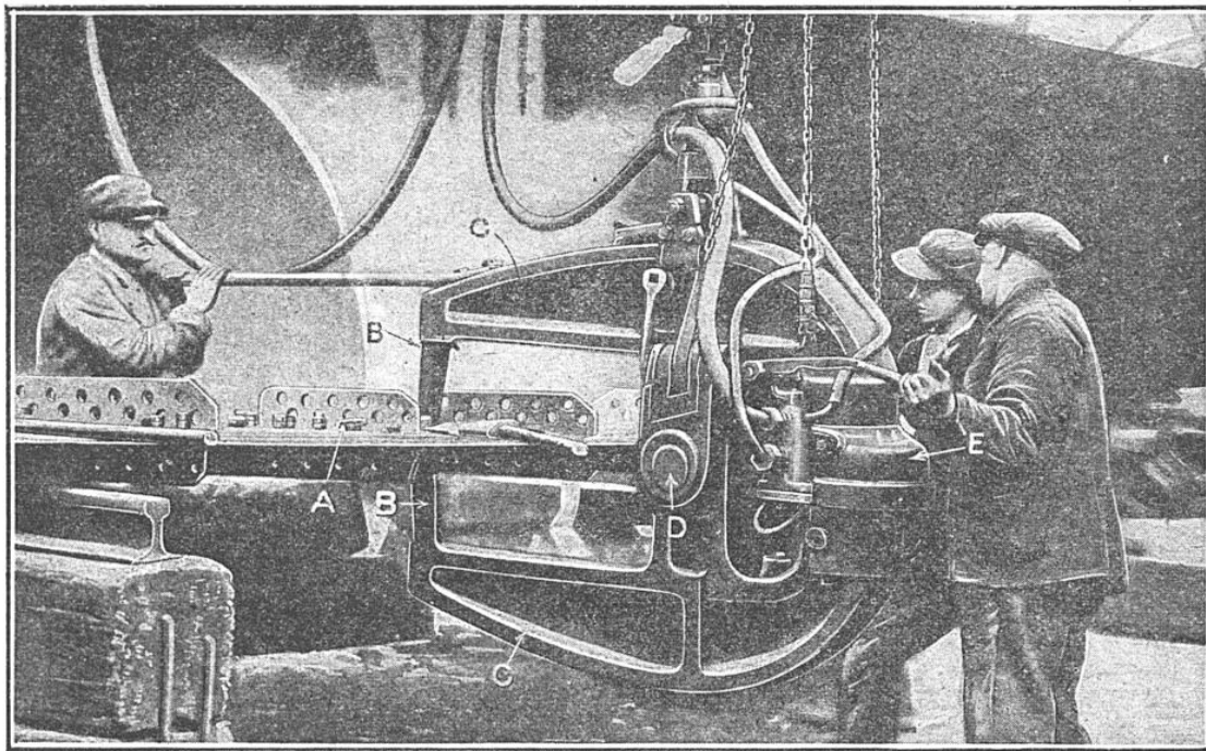
OUVRIERS ANGLAIS POSANT DES RIVETS AVEC UNE MACHINE HYDRAULIQUE
