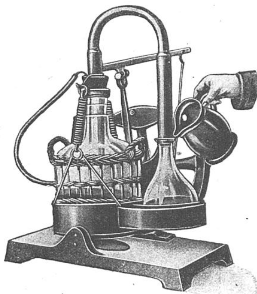
APPAREIL DOUANE « LE POLAIRE » A ÉVAPORATION DE L'EAU DANS LE VIDE
