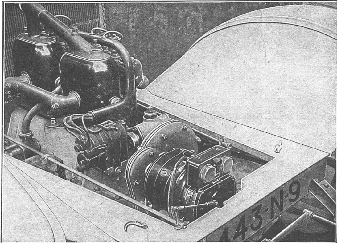
DYNAMO GÉNÉRATRICE ET MOTRICE PLACÉE EN AVANT DU MOTEUR
