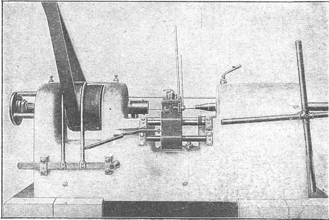
TOUR DESTINÉ A L'USINAGE DES OBUS DE PETIT CALIBRE
