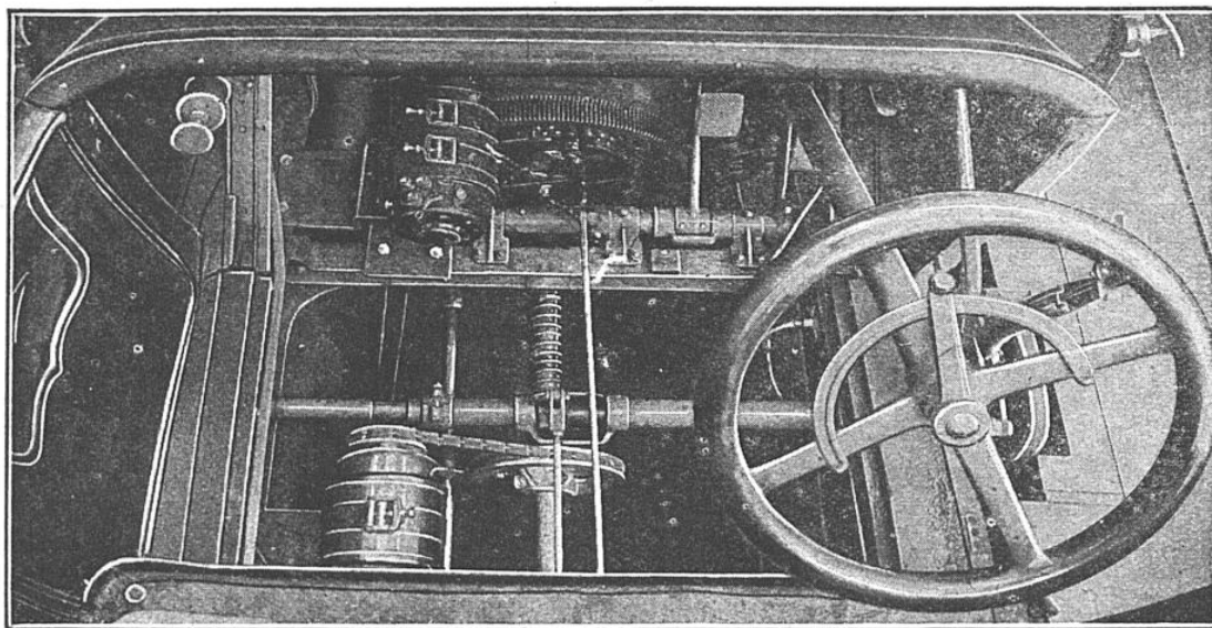
LE DÉMARREUR ÉLECTRIQUE ACTIONNE DIRECTEMENT LE VOLANT
