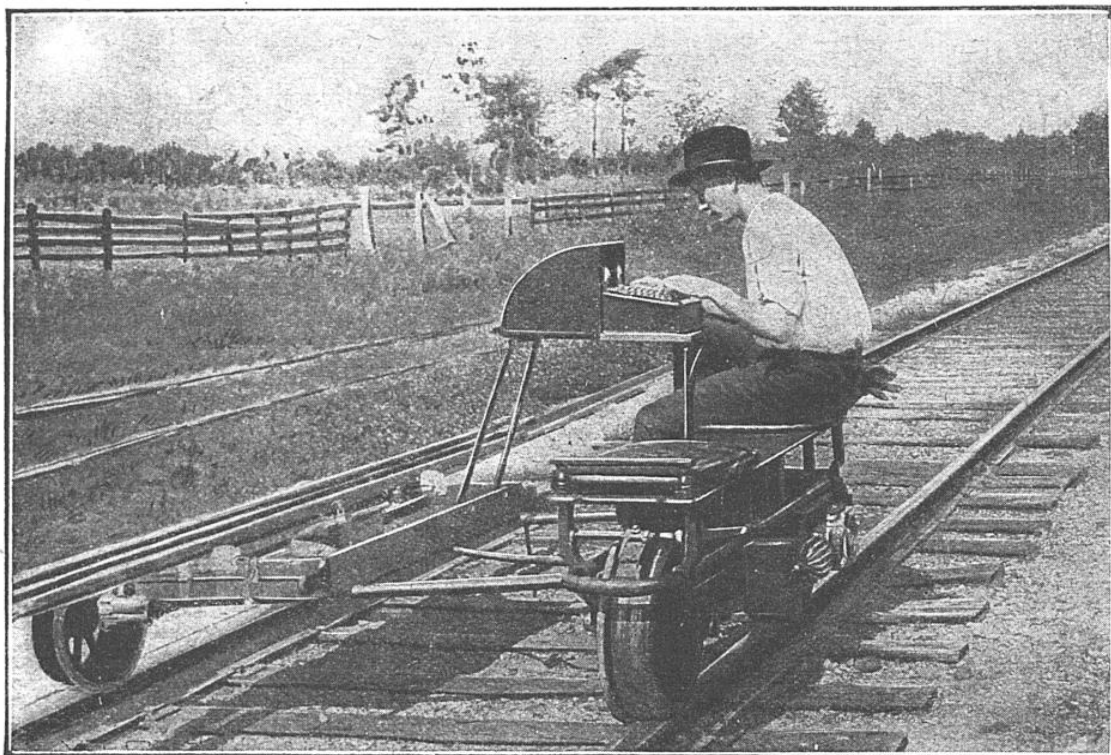
MONTÉ SUR SON CHARIOT, L'AIDE ENREGISTRE LES CHIFFRES DES VISÉES
