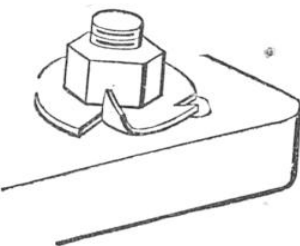
LES TROIS SYSTÈMES POUR IMMOBILISER UN ÉCROU
