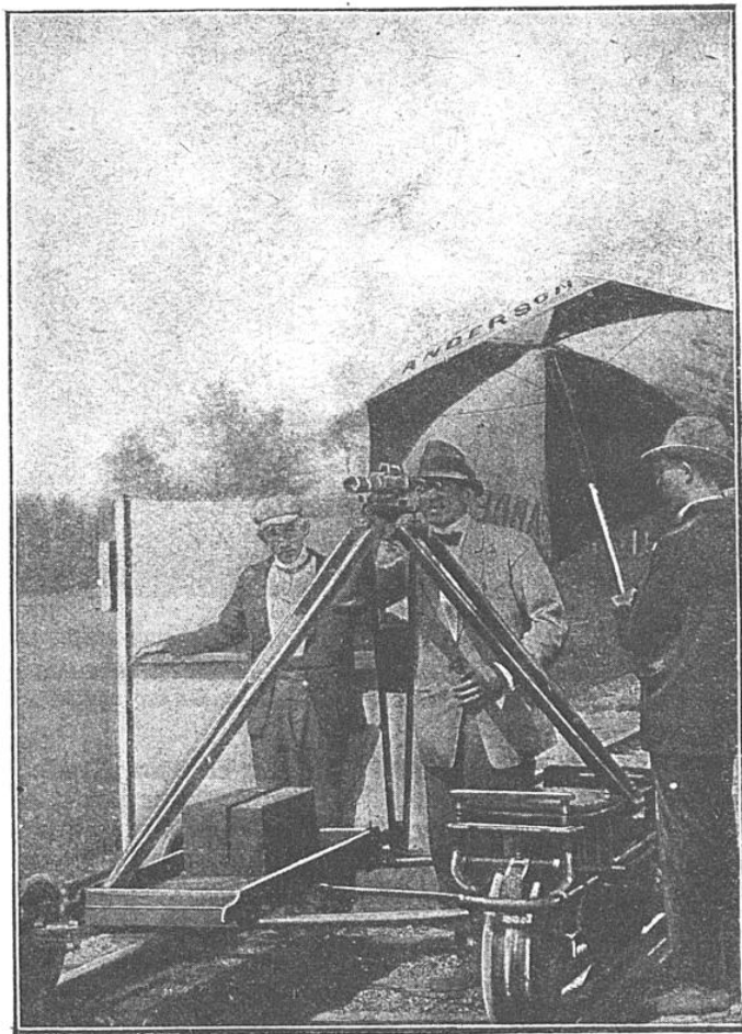
UNE VISÉE AVEC LA LUNETTE D'ALIGNEMENT
