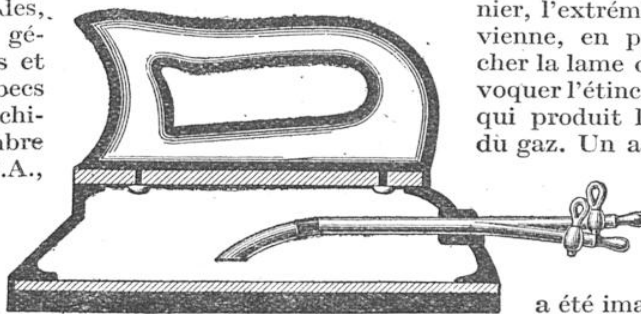
FER A REPASSER CHAUFFÉ INTÉRIEUREMENT PAR L'ACÉTYLÈNE
