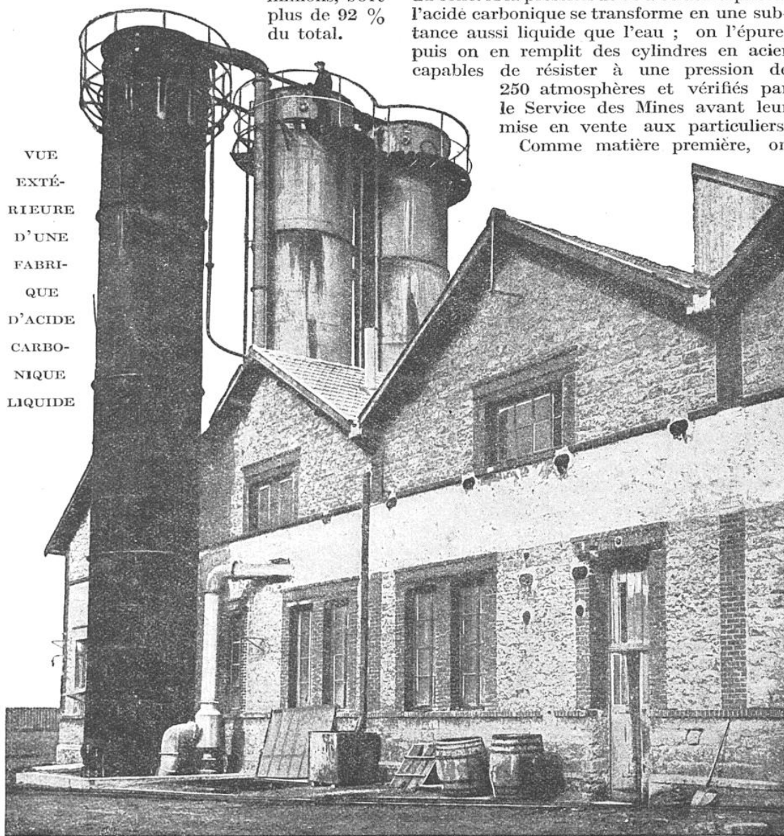
L'acide carbonique, l'oxygène et l'azote provenant de la combustion du coke s'introduisent successivement, par des canalisations spéciales, dans trois colonnes cylindriques, d'une hauteur approximative de 25 mètres, dans lesquelles ces gaz circulent de bas en haut.
