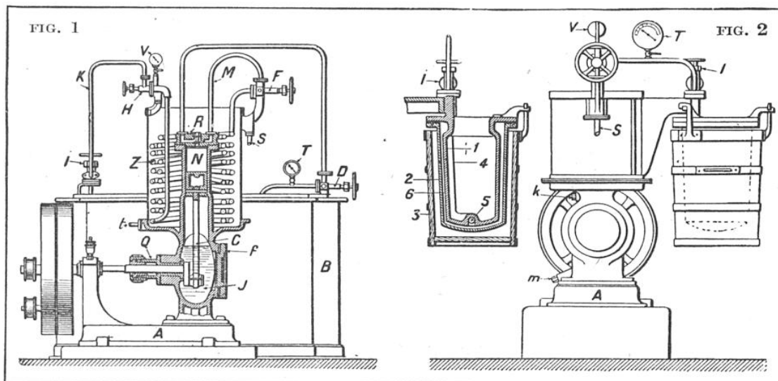
APPAREILS A GLACE SYSTEME DOUANE, FONCTIONNANT AU CHLORURE DE METHYLE
