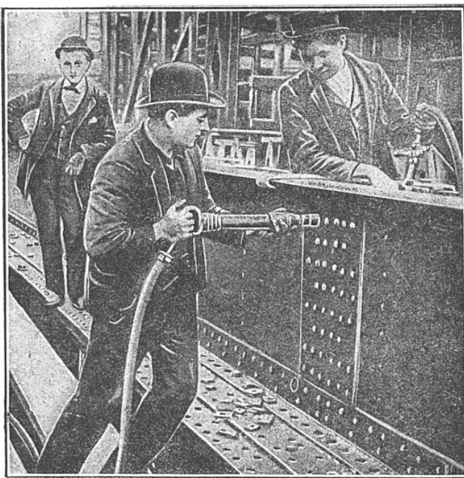
POSE DE RIVETS AU MOYEN D'UN MARTEAU PNEUMATIQUE
