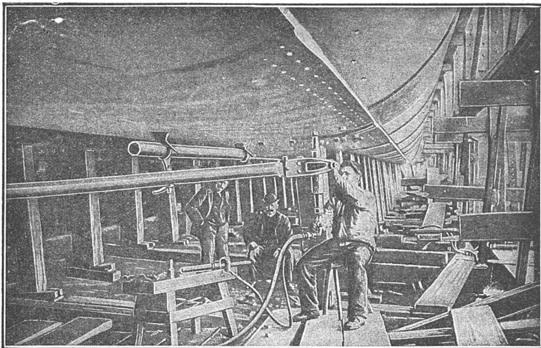
RIVETAGE DES TÔLES DU FOND D'UNE COQUE DE NAVIRE
