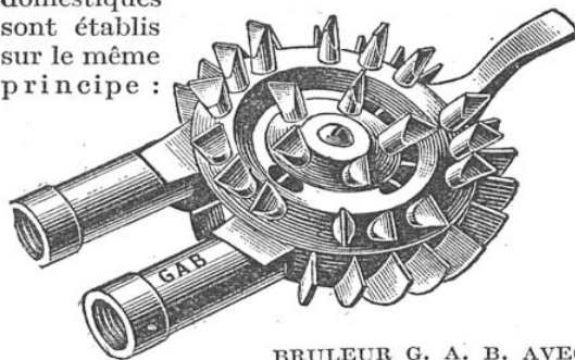
BRULEUR G. A. B. AVEC AILETTES POUR REFROIDIR LA MASSE
