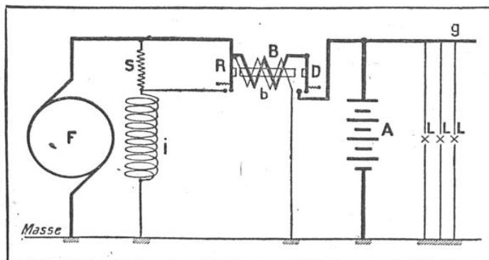
SCHEMA DES CONNEXIONS DE LA DYNAMO S. E. V A, accumulateurs; B, bobine gros fil; b, bobine fil fin; F, dynamo; I, inducteur; S, résistance; R, régulateur; D, disjoncteur; g, ligne; L, lampes. — Ce montage est à un seul fil avec retour par la masse.
