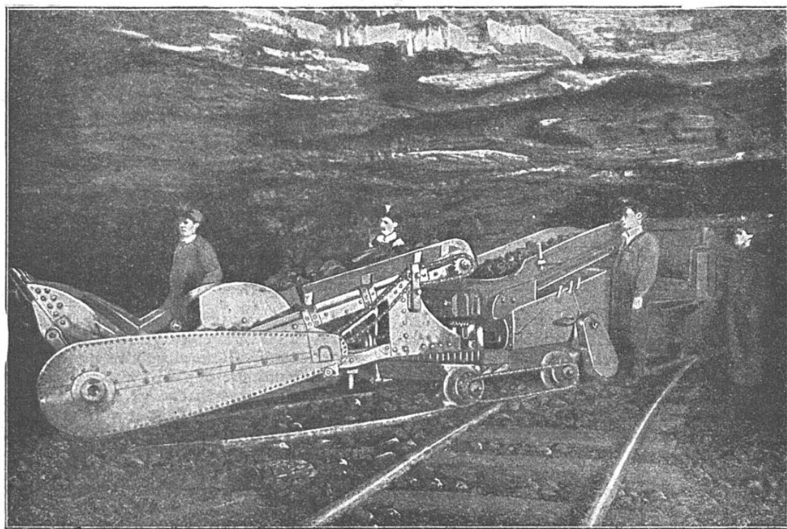
LA DÉROCHEUSE MYERS-WHALEY EN SERVICE DANS UNE MINE DE HOUILLE
