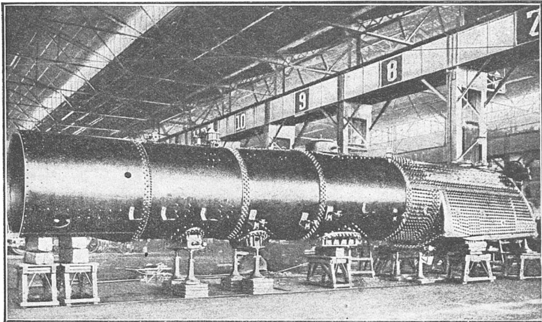
CHAUDIÈRE ET FOYER D'UNE LOCOMOTIVE A 24 ROUES MOTRICES
