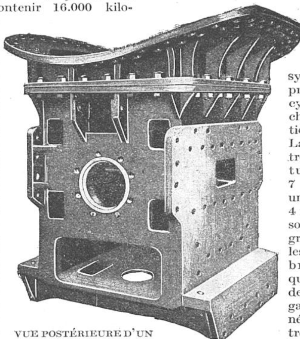
VUE POSTÉRIEURE D'UN SUPPORT DE CYLINDRE A HAUTE PRESSION
