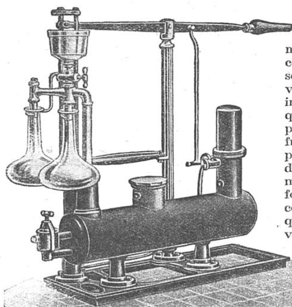
CONGÉLATEUR SYSTÈME CARRÉ A ÉVAPORATION D'EAU DANS LE VIDE, MODÈLE SIMPLE A DEUX CARAFES, FONCTIONNANT A LA MAIN
