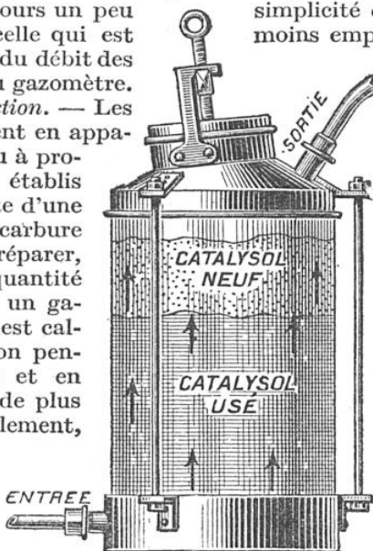
UN ÉPURATEUR ÉCONOMIQUE
