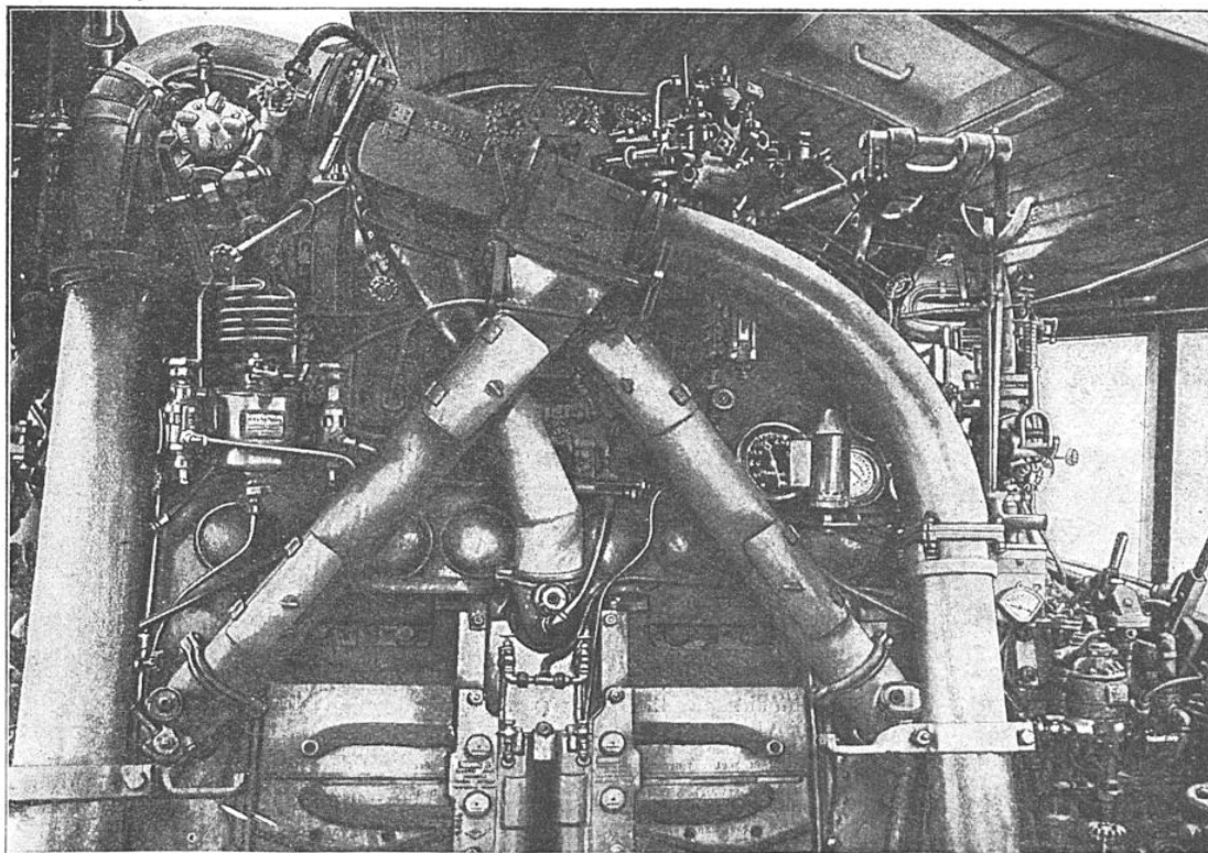
LA PARTIE POSTÉRIEURE DE LA LOCOMOTIVE, SURMONTÉE DE SON ABRI
