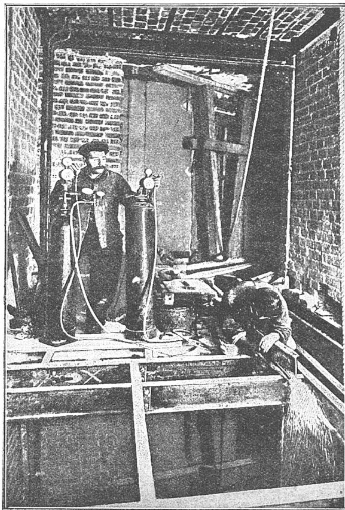
DÉCOUPAGE DES POUTRES DE FER A L'AIDE DU CHALUMEAU OXYDRIQUE
