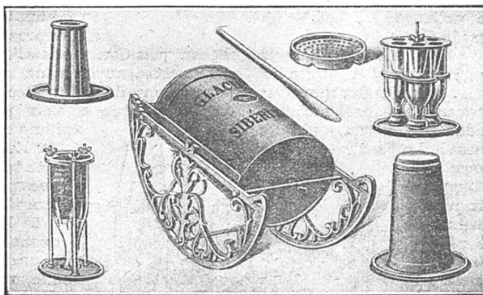
GLACIÈRE DE MÉNAGE DITE « SIBÉRIENNE » A MÉLANGE RÉFRIGÉRANT, MONTÉE SUR SUPPORT A BASCULE
