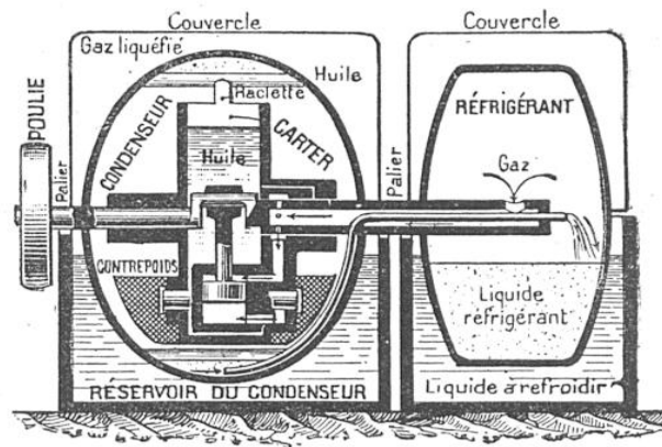
COUPE SCHÉMATIQUE DU « FRIGORIGÈNE » MONTRANT SON FONCTIONNEMENT INTÉRIEUR (Voir la figure de la page précédente.)
