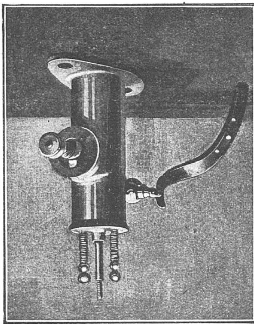
LE CARBURATEUR CAUET
