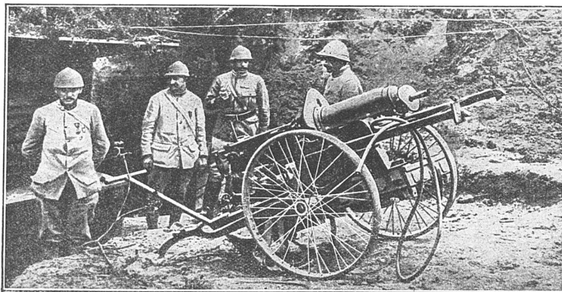
MITRAILLEUSE LOURDE MONTÉE SUR UN AFFUT SPÉCIAL A ROUES
