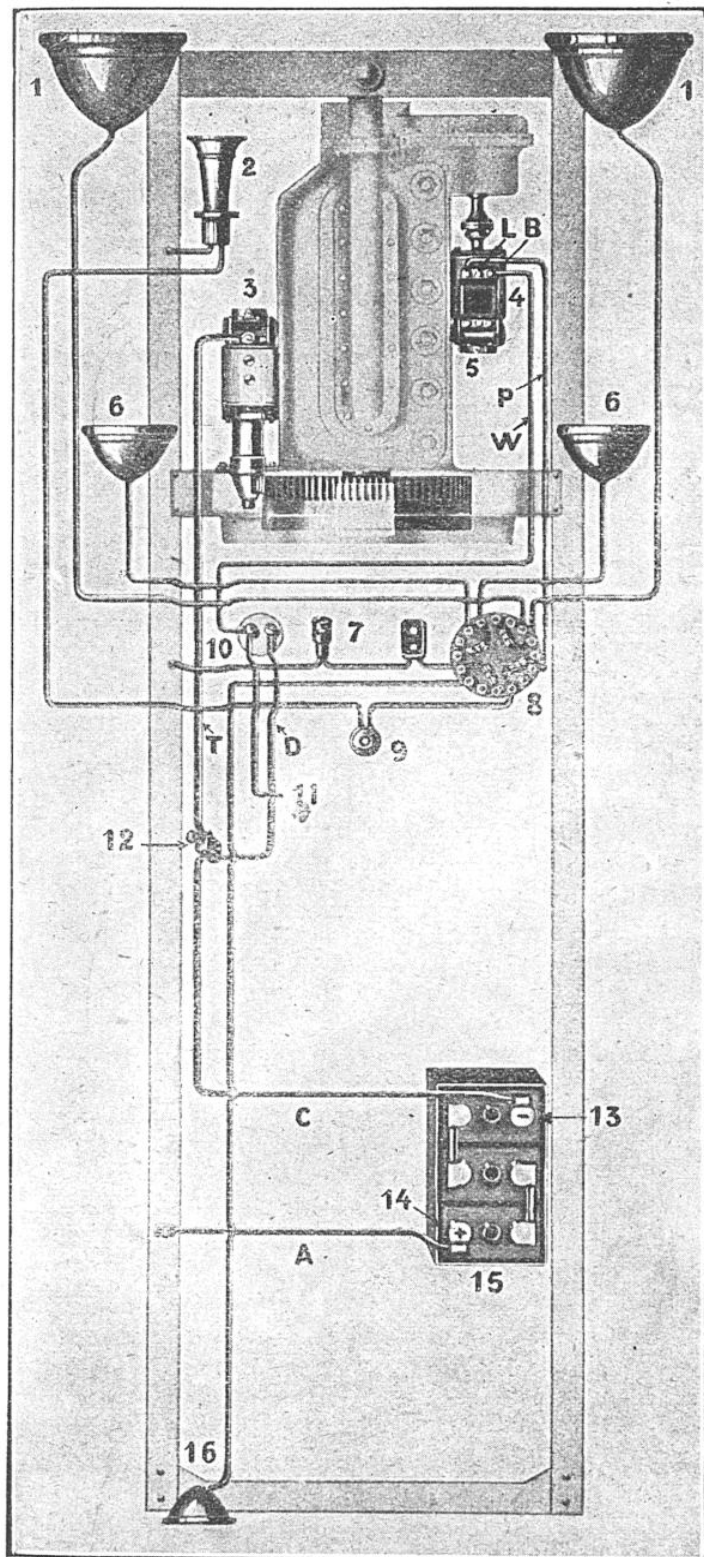
SCHÉMA MONTRANT LE DISPOSITIF D'UN APPAREILLAGE ÉLECTRIQUE SUR UNE VOITURE AUTOMOBILE
