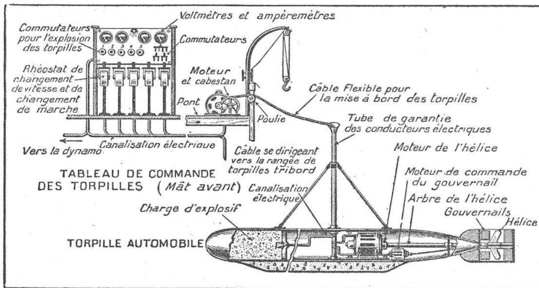
TORPILLE A PROPULSION ET A DIRECTION AUTOMOBILES SPÉCIALEMENT AMÉNAGÉE
