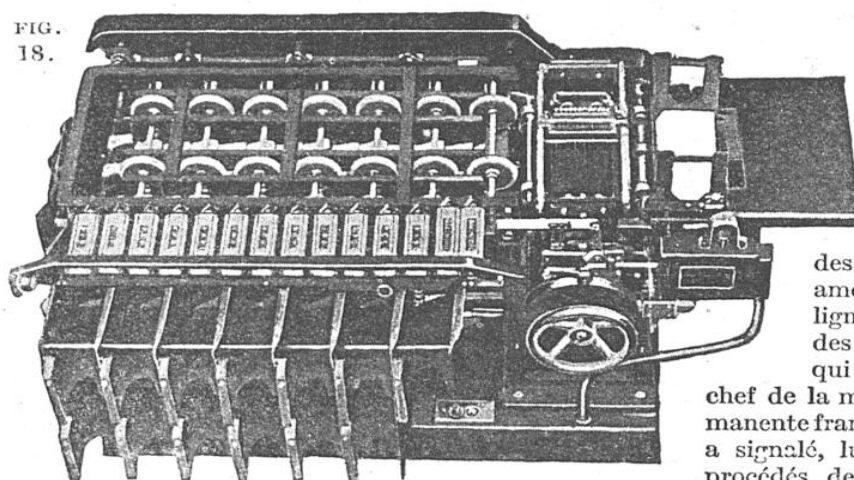
LA MACHINE A CLASSER POWERS, POURVUE D'UN COMPTEUR QUI ADDITIONNE ENSUITE LES SOMMES INSCRITES SUR LES CARTONS PERFORÉS
