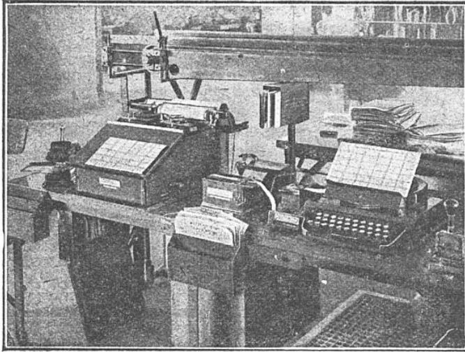
LES NOUVEAUX APPAREILS TÉLÉGRAPHIQUES ; A DROITE, LE TRANSMETTEUR ; A GAUCHE, LE RÉCEPTEUR
