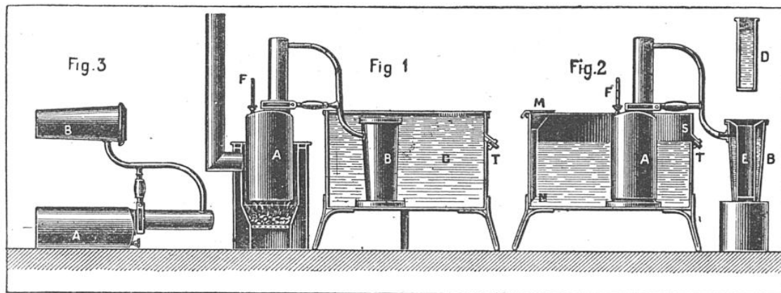
MACHINE PERFECTIONNÉE CARRÉ, A ABSORPTION, POUR LA CONGÉLATION DES LIQUIDES
