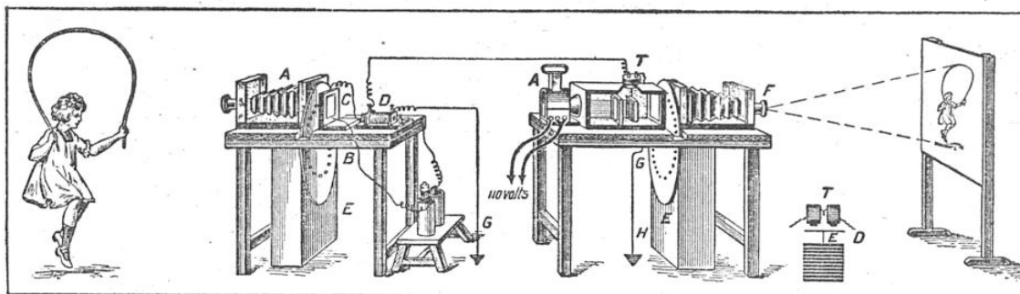
FIG. 2. — TÉLÉPHOTE FRANÇAIS SYSTÈME DUSSAUD, CONSTRUIT EN 1898
