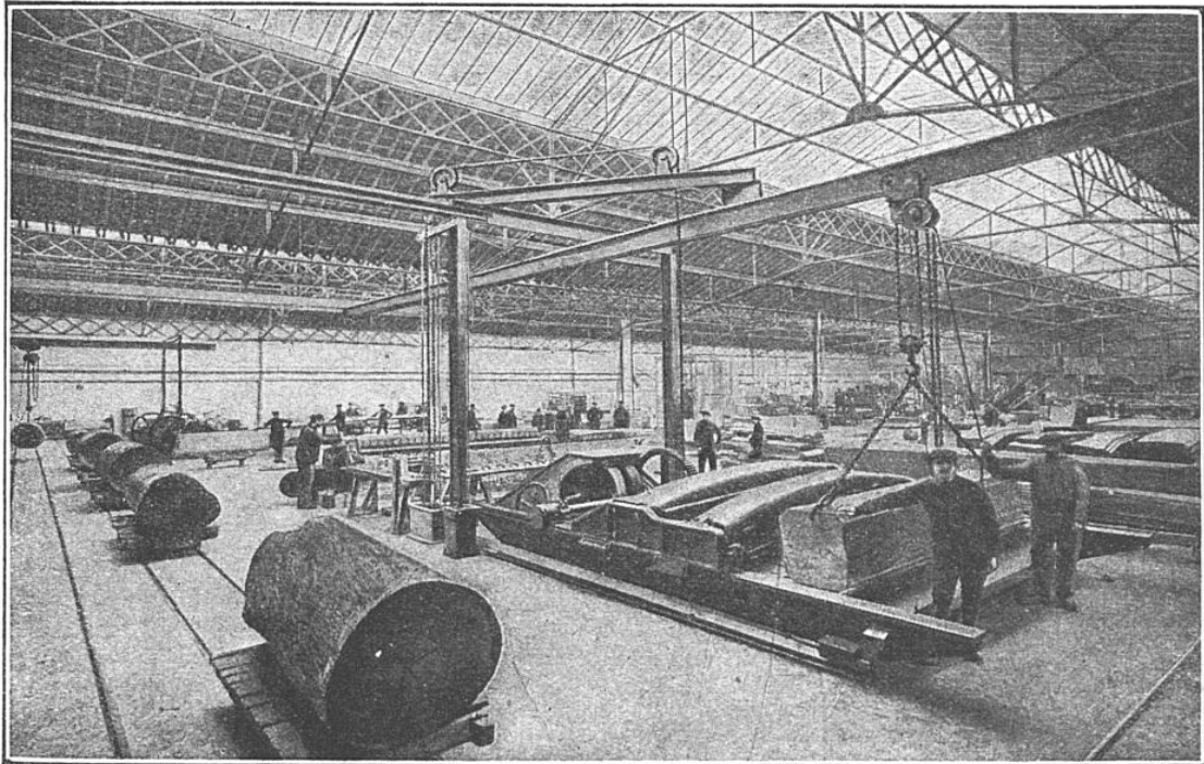
ATELIER DE DÉROULAGE, DE TRANCHAGE ET DE FABRICATION DES PANNEAUX
