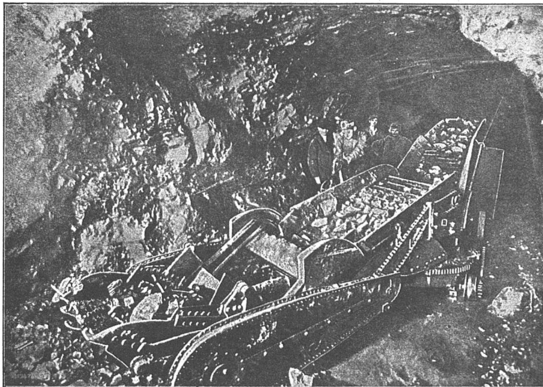
DÉROCHEUSE EN ACTION SUR LES CHANTIERS D'UN AQUEDUC SOUTERRAIN
