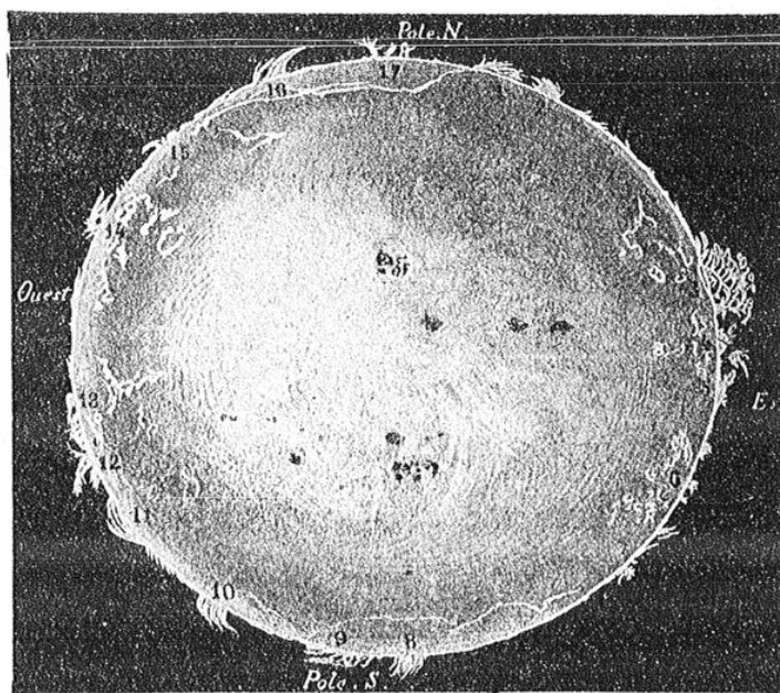
FIG. 6. — LE SOLEIL AVEC SES PROTUBÉRANCES Ces protubérances sont figurées sur ce dessin telles que le spectroscope permet de les voir.
