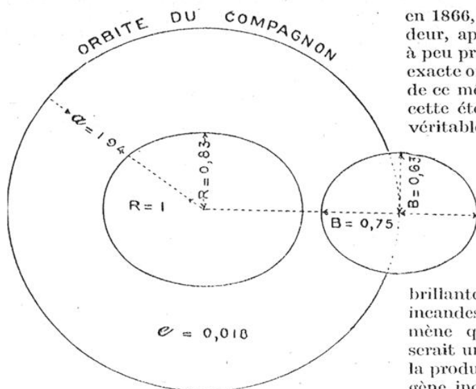
FIG. 5. — EXPLICATION DES VARIATIONS D'ÉCLAT DE B LYRE
