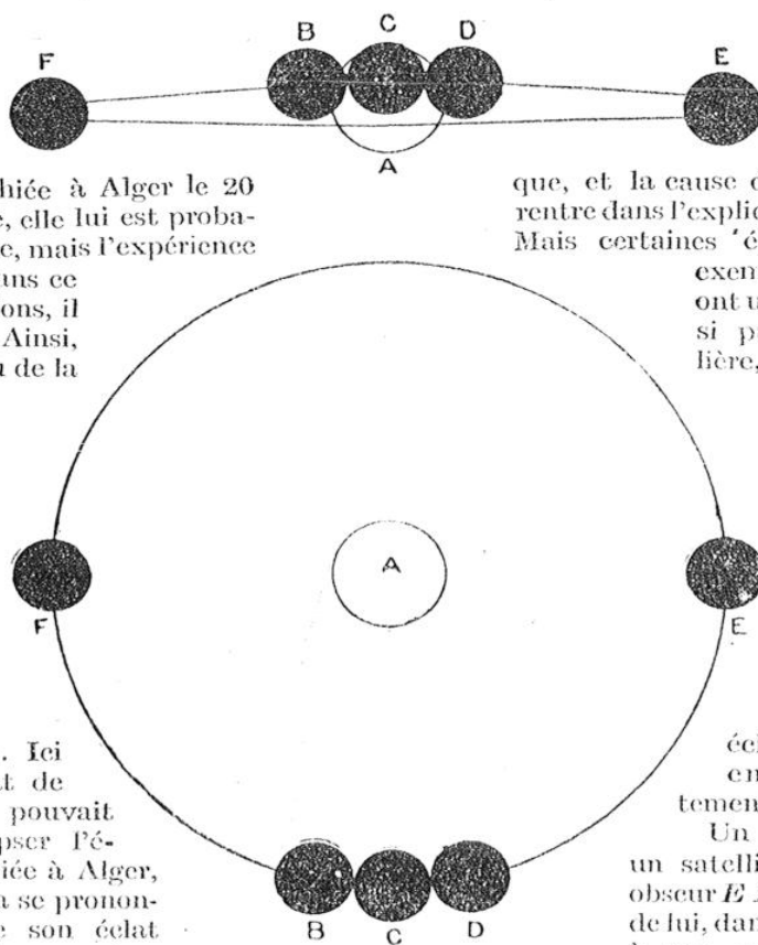
FIG. 4. — EXPLICATION DE LA VARIABILITÉ DE L'ALGOL.
