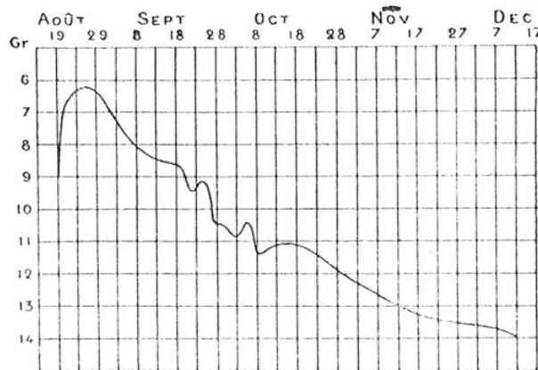
FIG. 1. — COURBE FIGURANT LA VARIATION D'ÉCLAT DE L'ÉTOILE NOUVELLE D'ANDROMÈDE
