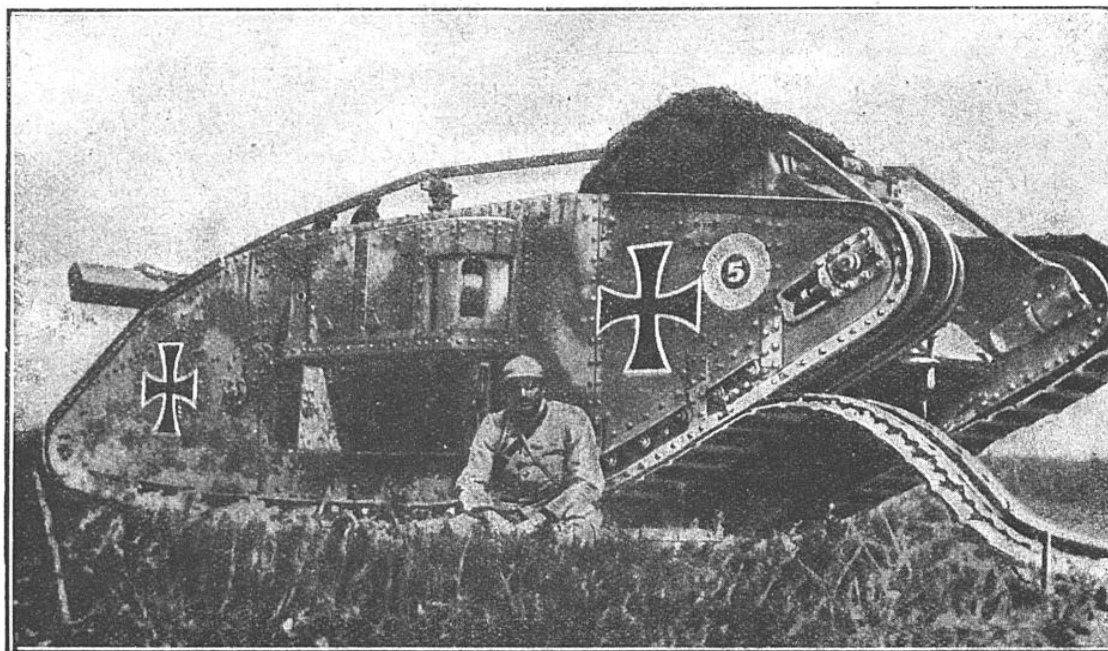
VUE LATÉRALE DU TANK ANGLAIS PRÉCÉDENT, TOMBÉ AU POUVOIR DE L'ENNEMI Pour affirmer leur prise de possession, les Allemands avaient peint des « croix de fer » sur les faces latérales de l'engin de guerre britannique repris par nos troupes.
