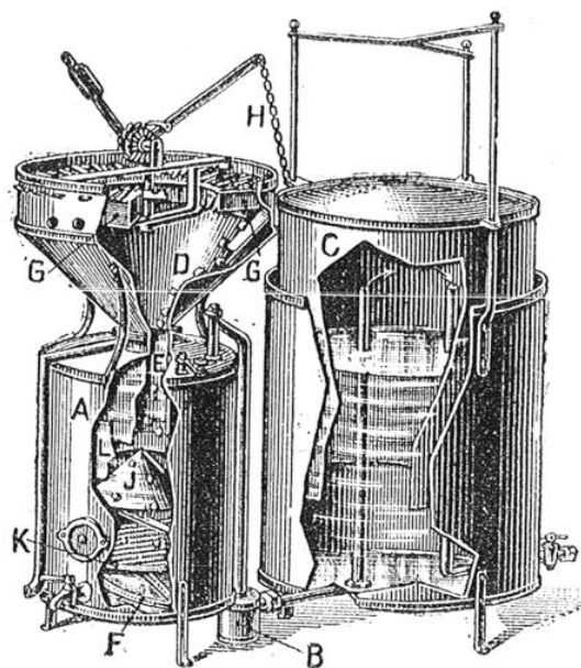
APPAREIL AUTOMATIQUE A CHUTE DE CARBURE DANS L'EAU
