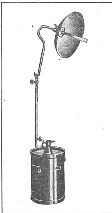
APPAREIL PORTATIF A RÉFLECTEUR POUR L'ÉCLAIRAGE DES CHANTIERS SITUÉS EN PLEIN AIR
