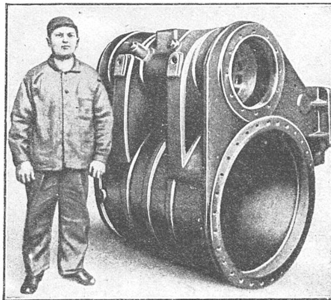
UN DES SIX CYLINDRES DE LA LOCOMOTIVE
