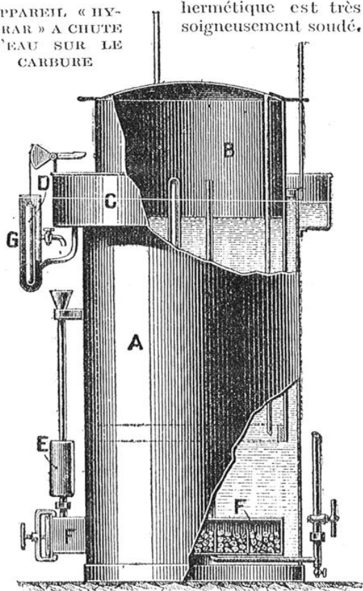
A, cuve du gazomètre mobile; B, gazomètre; C, réservoir d'eau de décomposition; D et G, dispositifs d'écoulement d'eau; E, boîte hydraulique; FF, générateurs.
