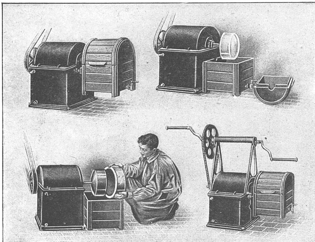
FABRICATION IMMÉDIATE D'UNE PETITE QUANTITÉ DE GLACE AVEC LE « FRIGORIGÈNE »
