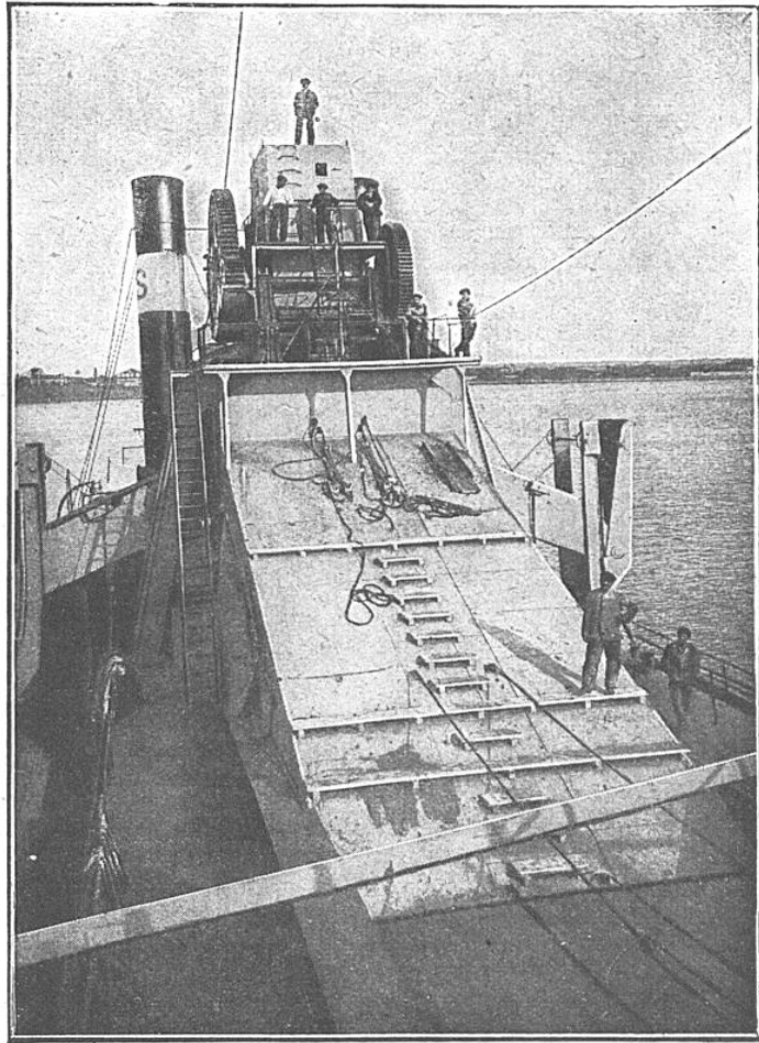
SUPERSTRUCTURE DE « LA PUISSANTE »
