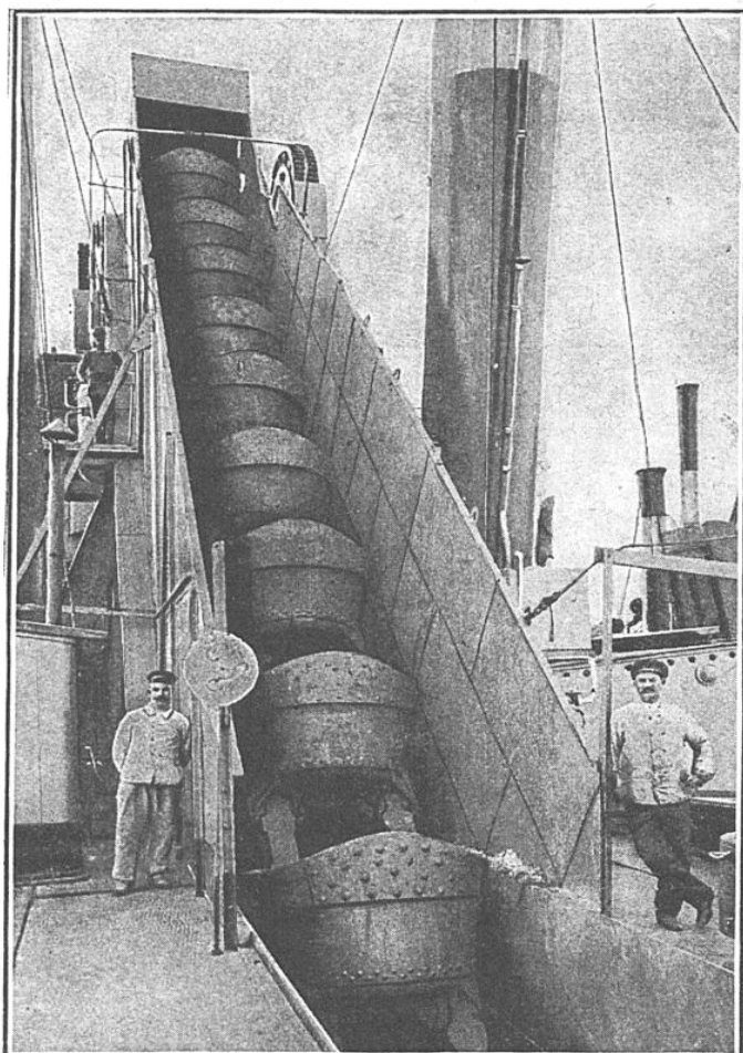
GODETS DE LA DRAGUE « LA PUISSANTE »
