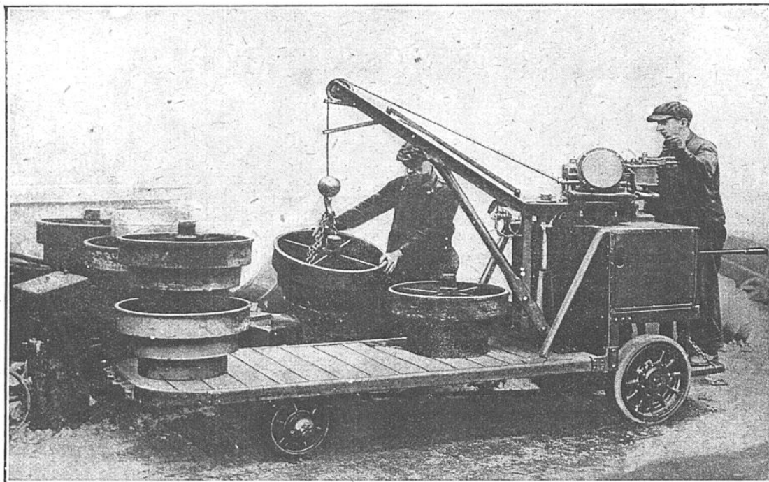
PIÈCES DE FONDERIE DÉCHARGÉES A L'AIDE DE LA GRUE DU CAR ÉLECTRIQUE Avec cet engin, deux hommes peuvent manutentionner quotidiennement, sans grands efforts et sans aucune fatigue, des milliers de kilogrammes d'objets divers.
