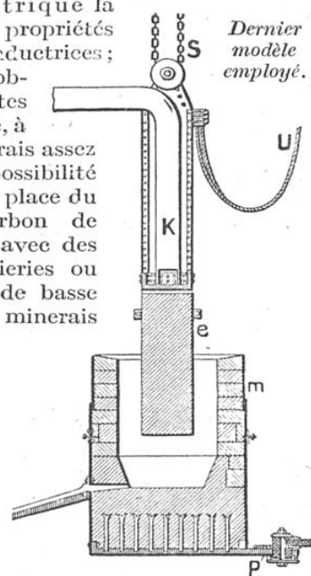
FOUR ÉLECTRIQUE DE SAULT-SAINTE-MARIE
