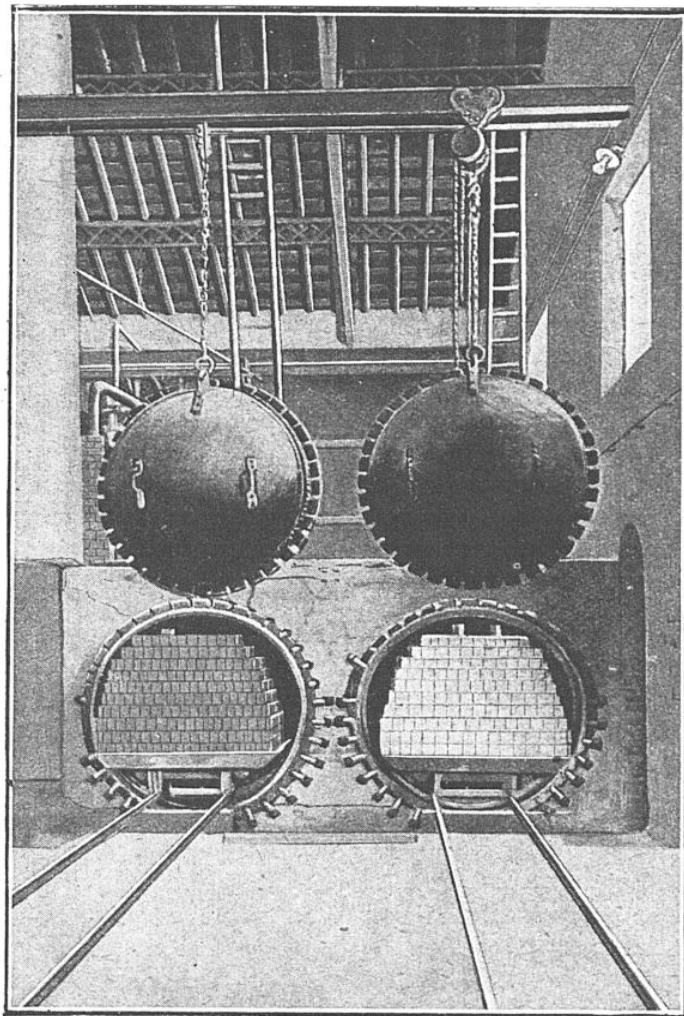
AUTOCLAVE DE DURCISSEMENT, VU DE FACE
