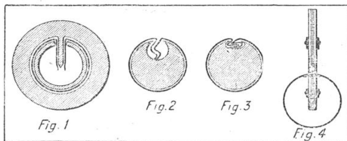
FIG. 16. — LES DIFFÉRENTES PHASES DE LA FABRICATION DES TUBES À CIGARETTES SANS COLLE, PAR AGRAFAGE ET SERTISSAGE
