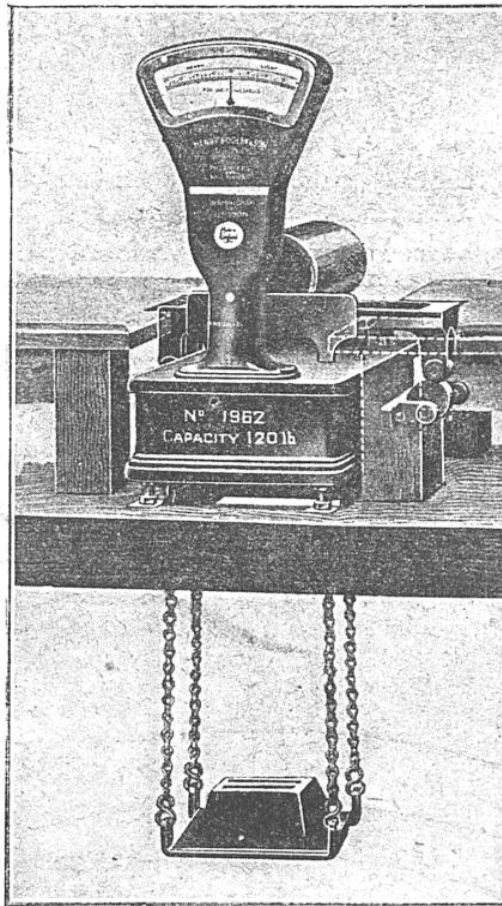
BALANCE AUTOMATIQUE SYSTÈME POOLEY POUR PROJECTILES DE MOYENS CALIBRES
