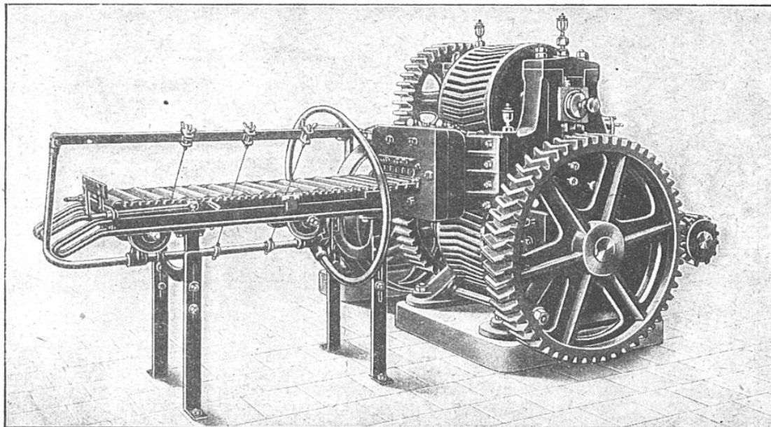
UNE MACHINE A BRIQUES A CYLINDRES PROPULSEURS
