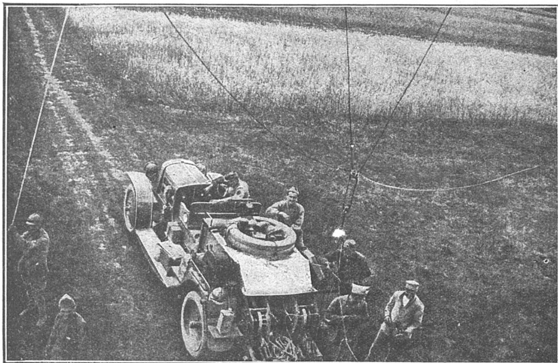
LE CAMION-TREUIL SACCONNEY VU DE LA NACELLE DU BALLON
