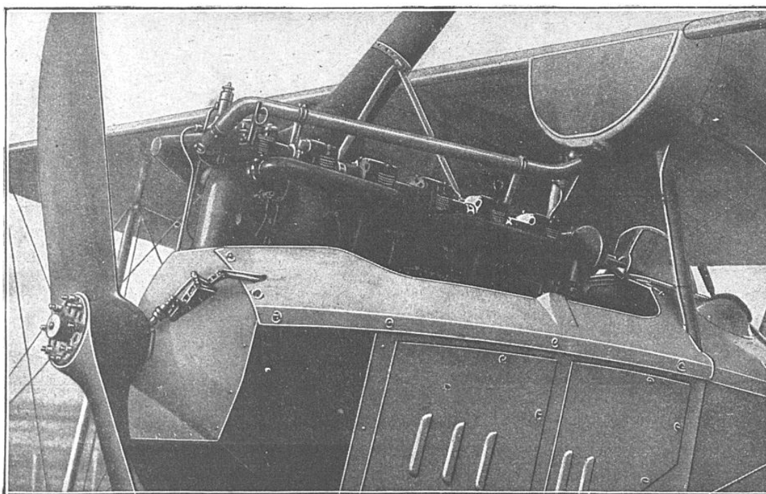
DISPOSITION D'UN MOTEUR MERCEDES SUR UN AVION BIPLACE ALLEMAND
