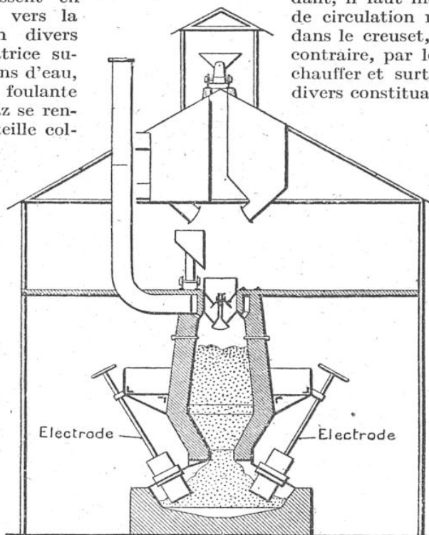
ENSEMBLE SCHÉMATIQUE DU HAUT FOURNEAU ÉLECTRIQUE FONCTIONNANT À HÉROULT (CANADA)
