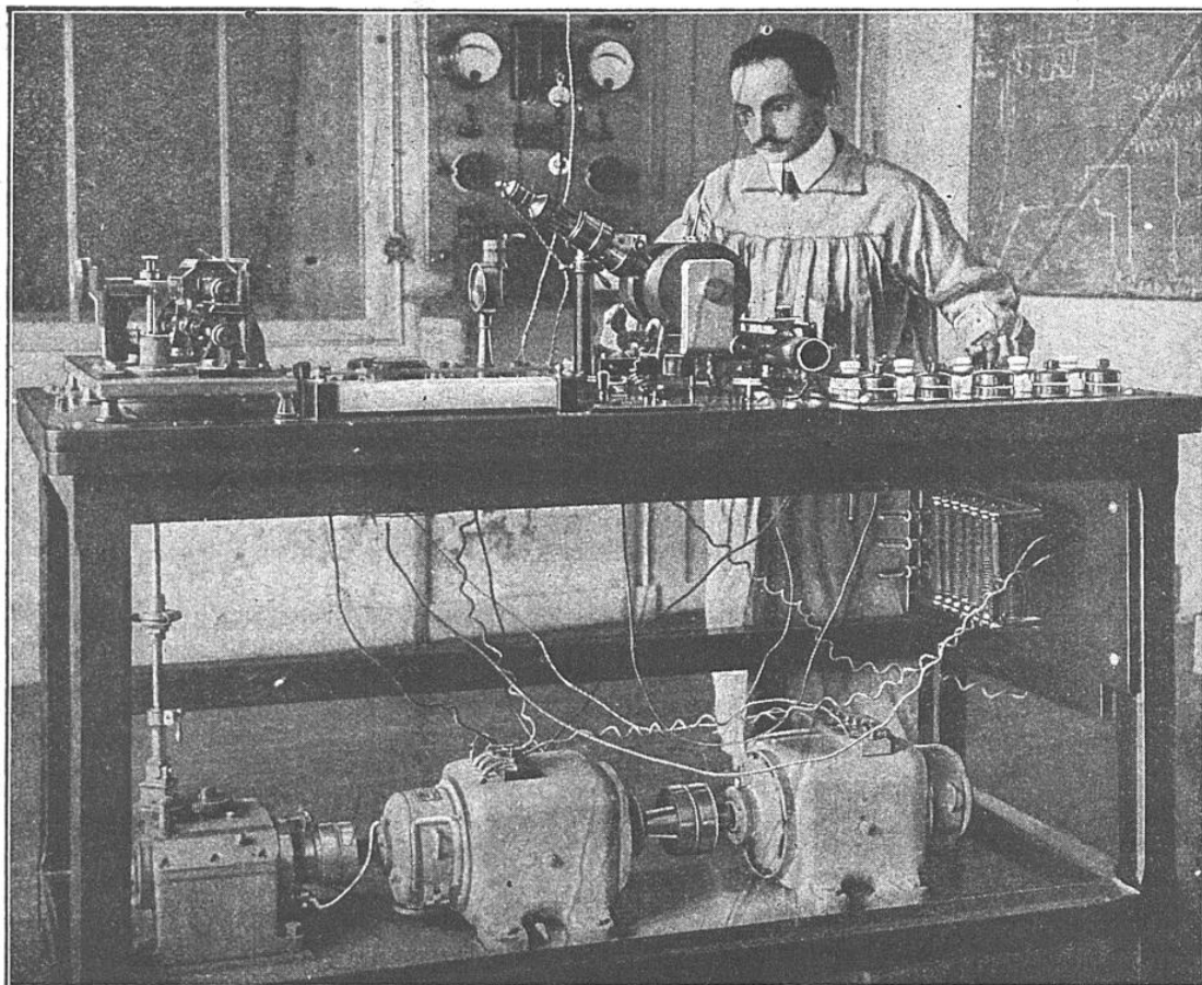
FIG. 11. — STATION RÉCEPTRICE DU TÉLÉPHOTOGRAPHE BELIN
