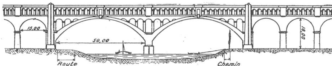
PORTION CENTRALE DU PONT-CANAL QUI TRAVERSA LA VALLÉE DE L'OISE ENTRE MÉRY ET VALMONDOIS
