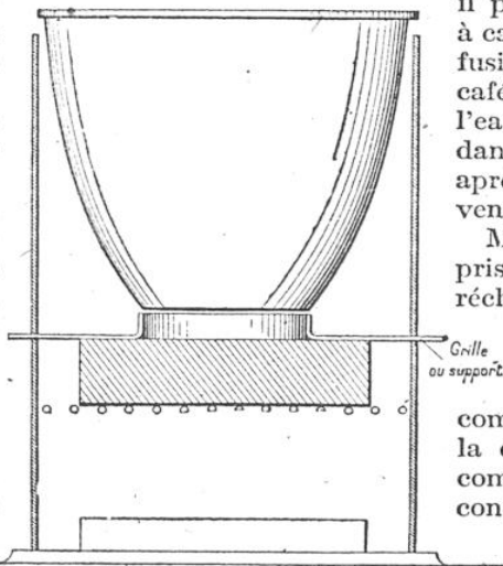
FIG. 9. — RÉCHAUD DE M. ESNAL
