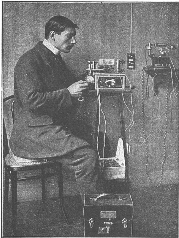
FIG. 13. — REPORTER DE JOURNAL ILLUSTRÉ « TÉLÉPHONANT » UNE PHOTOGRAPHIE DANS UNE CABINE PUBLIQUE À L'AIDE DE L'APPAREIL PORTATIF BELIN
