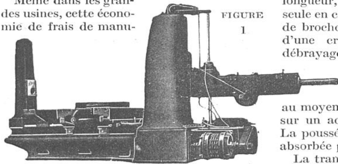
LA MACHINE ÉQUIPÉE POUR ÊTRE UTILISÉE COMME FRAISEUSE
