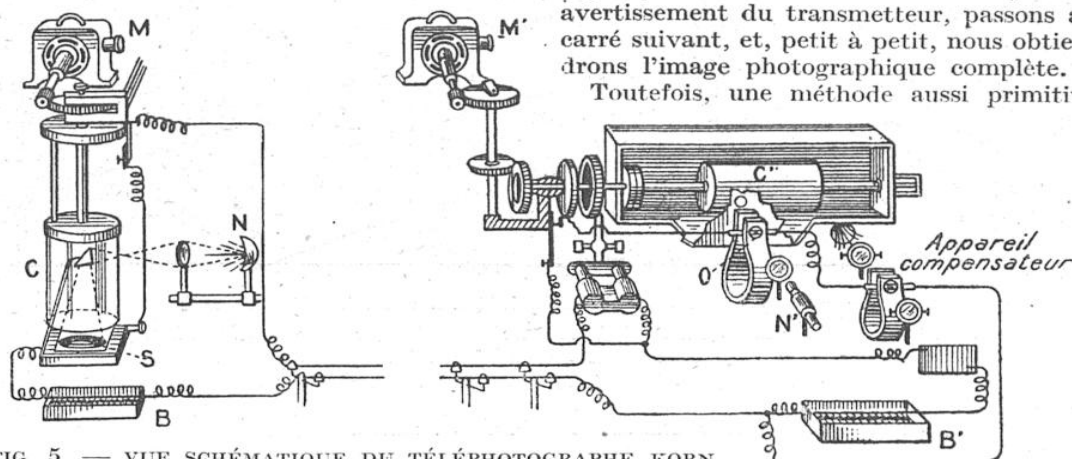
FIG. 5. — VUE SCHÉMATIQUE DU TÉLÉPHOTOGRAPHE KORN
