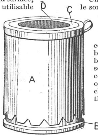
FIG. 8. — RÉCHAUD DE M. CHEVALLIER-APPERT A, cheminée-cylindre dite de Berthelot; B, lampe en godet contenant le liquide combustible ou l'alcool solidifié; C, couvercle avec un tamis D au milieu pour supporter les petits objets à chauffer.
