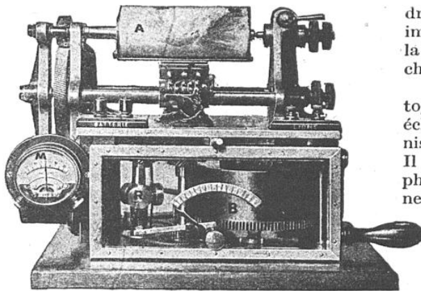
FIG. 12. — PHOTOTÉLÉGRAPHE PORTATIF BELIN
