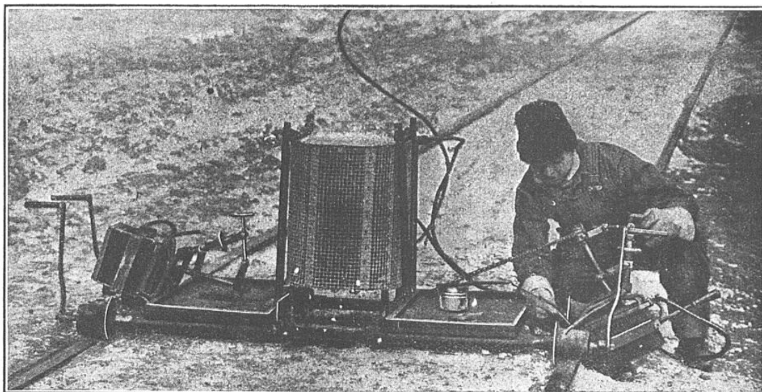
ICI, L'APPAREIL DE SOUDAGE EST MONTÉ SUR UN CHARIOT ROULANT SUR LES RAILS
