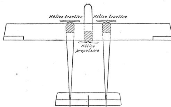
MULTI-MOTEUR A DEUX HÉLICES TRACTIVES ET UNE HÉLICE PROPULSIVE (CAPRONI)
