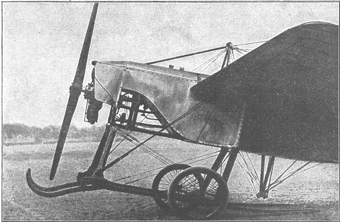
MOTEUR ROTATIF GNOME MONTÉ EN PORTE-A-FAUX SUR UN MONOPLAN DU TYPE BRISTOL (PHOTOGRAPHIE PRISE EN 1914, QUELQUES SEMAINES AVANT LA GUERRE)
