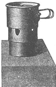
FIG. 3. — RÉCHAUD A CHEMINÉE-SUPPORT POUR BRULER L'ALCOOL SOLIDIFIÉ
