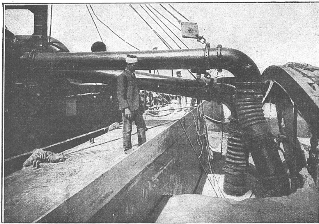
DISPOSITION DES TUYAUX D'UN BATEAU ASPIRATEUR
