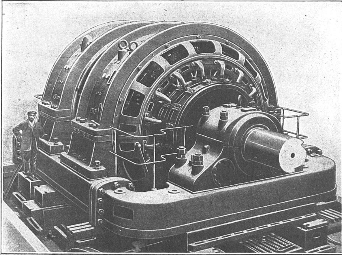
GROUPES DE DYNAMOS MOTRICES POUR LAMINOIR FONCTIONNANT A L'ÉLECTRICITÉ
