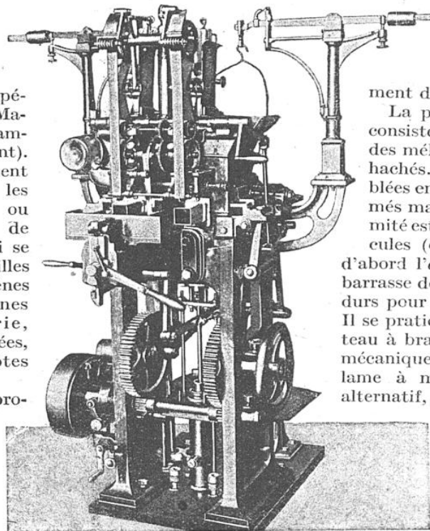
FIG. 12. — MACHINE A EMPAQUETER AUTOMATIQUEMENT LE TABAC
