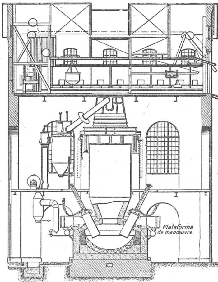
COUPE VERTICALE ET TRANSVERSALE DU HAUT FOURNEAU ÉLECTRIQUE DE TROLLHATTAN
