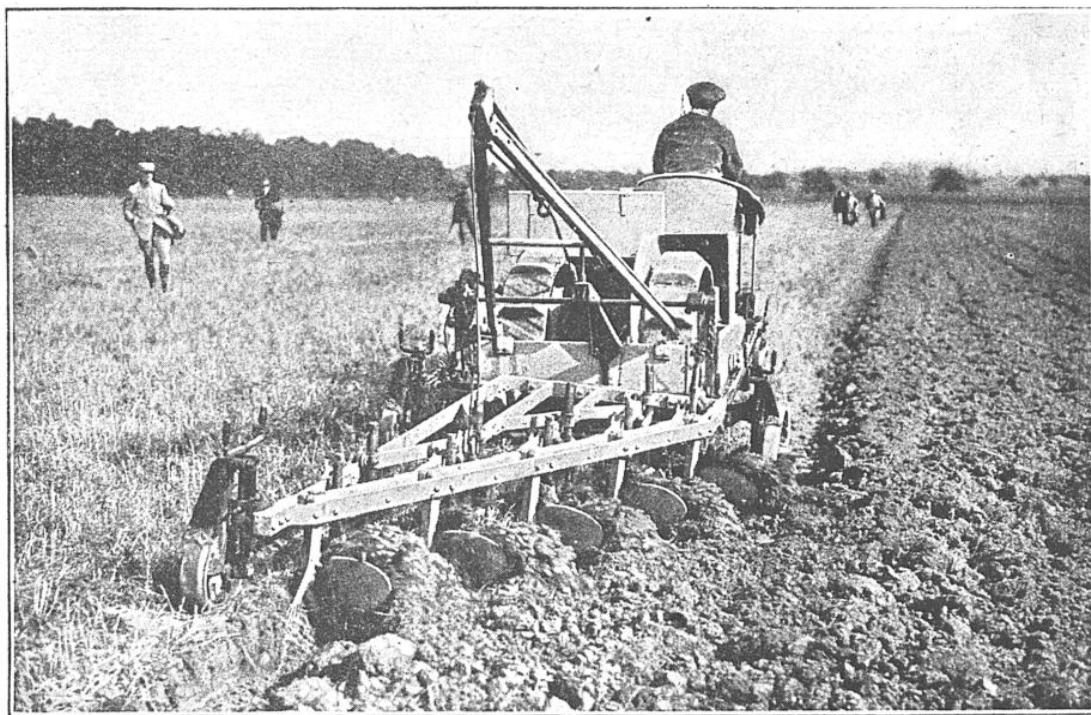
VUE ARRIÈRE D'UNE CHARRUE TOURAND-LATIL A CINQ SOCS
