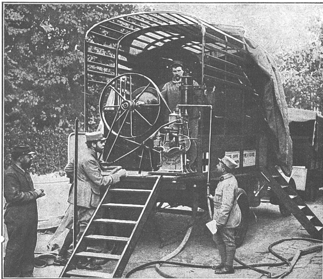
CAMION AUTOMOBILE AMÉNAGÉ POUR LA PRODUCTION DE LA GLACE ALIMENTAIRE A PROXIMITÉ DES ANCIENS HOPITAUX ET AMBULANCES DU FRONT
