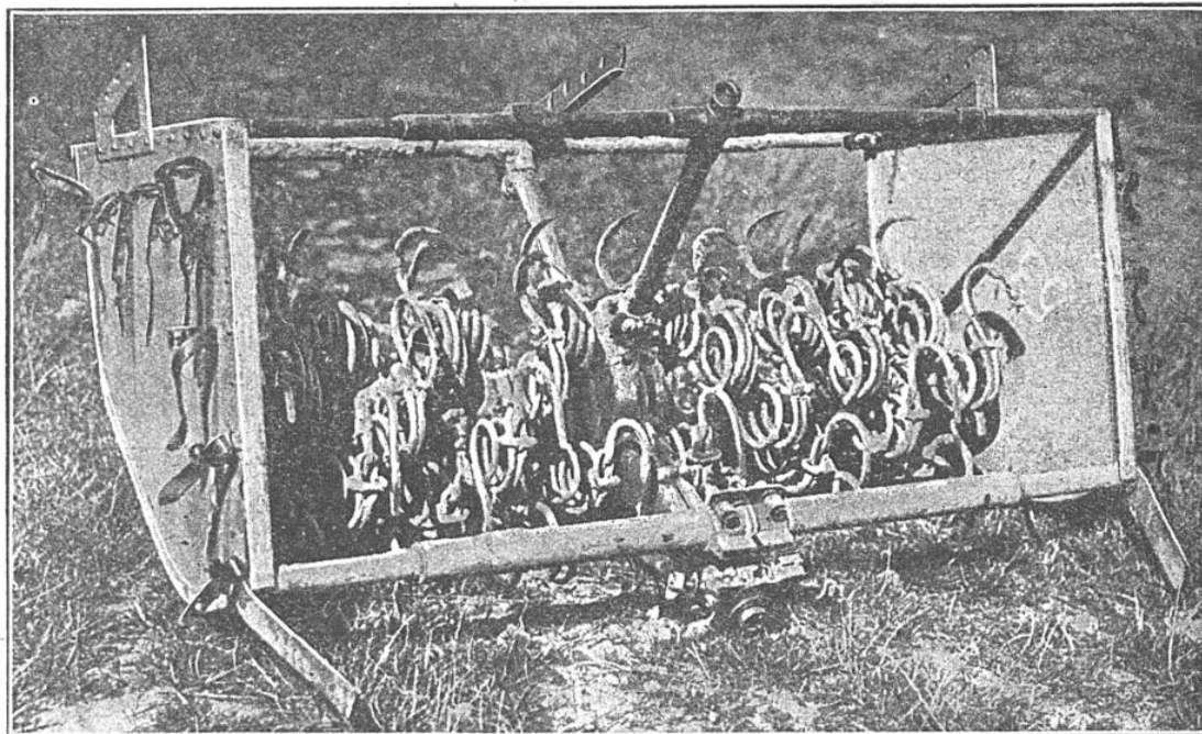
DÉTAIL DE LA FRAISE DU MOTOCULTEUR
