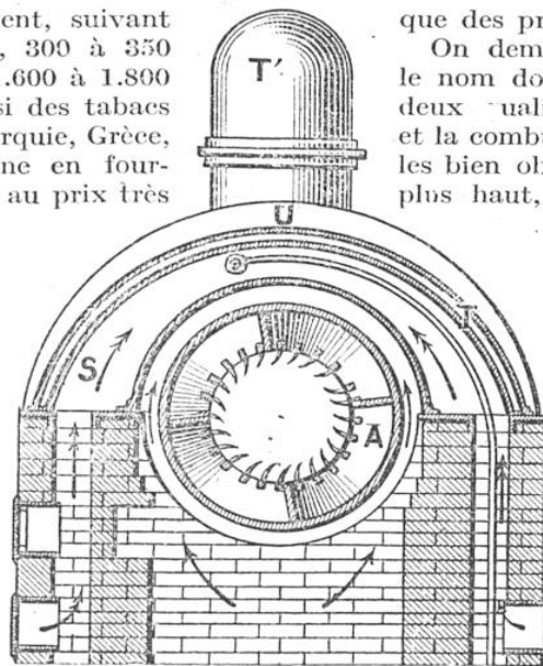
FIG. 11. — COUPE DU FOUR ROLLAND A, cylindre rotatif montrant les dents des lames radiales. (Voir la figure précédente pour l'explication des autres lettres.)
