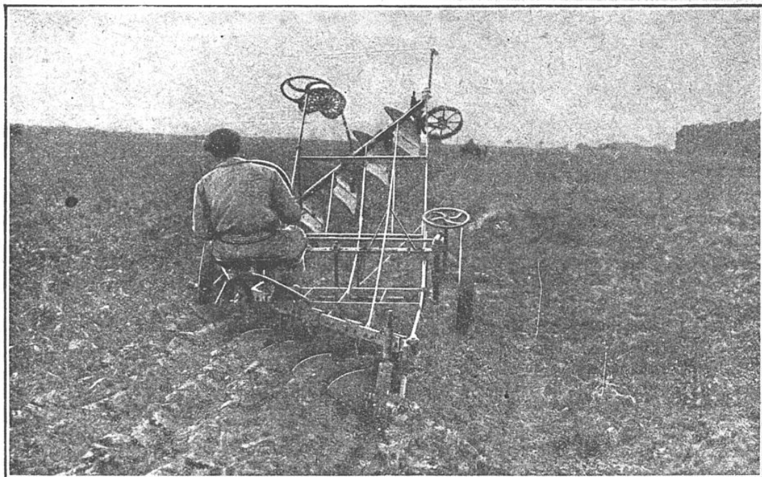
VUE D'UNE CHARRUE-BALANCE HALÉE PAR UN TRACTEUR-TREUIL
