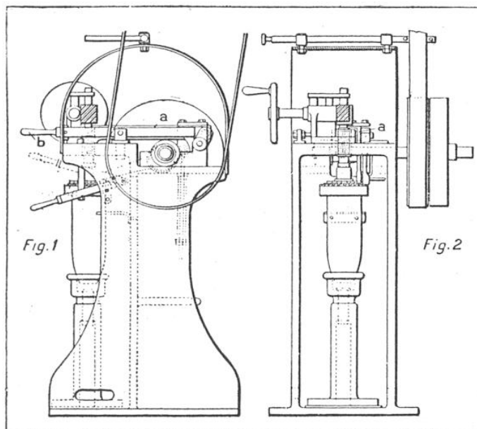
MACHINE MC LAREN POUR LE MARQUAGE DES PROJECTILES D'ARTILLERIE, VUE EN ÉLEVATION DE FACE (FIG. 1) ET EN ÉLEVATION DE CÔTÉ (FIG. 2)
