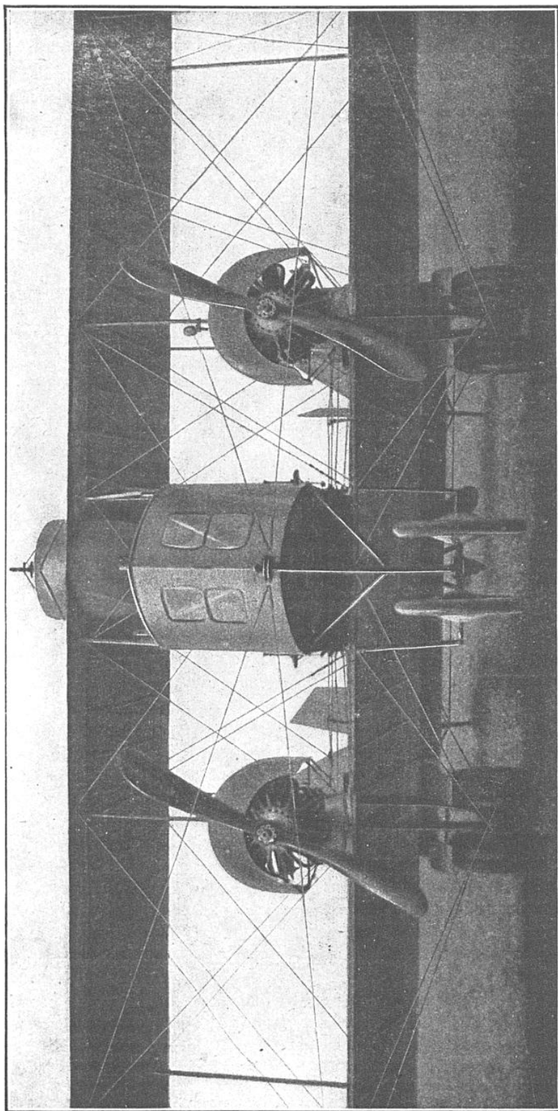
BIPLAN TRI-MOTEUR, VU DE FACE, DE L'INGÉNIEUR ITALIEN CAPRONI, DÉVELOPPANT 450 CHEVAUX (VOIR A LA PAGE HORS TEXTE 32 LES DÉTAILS DE L'UN DES MOTEURS DE CE PUISSANT APPAREIL DE BOMBARDEMENT)
