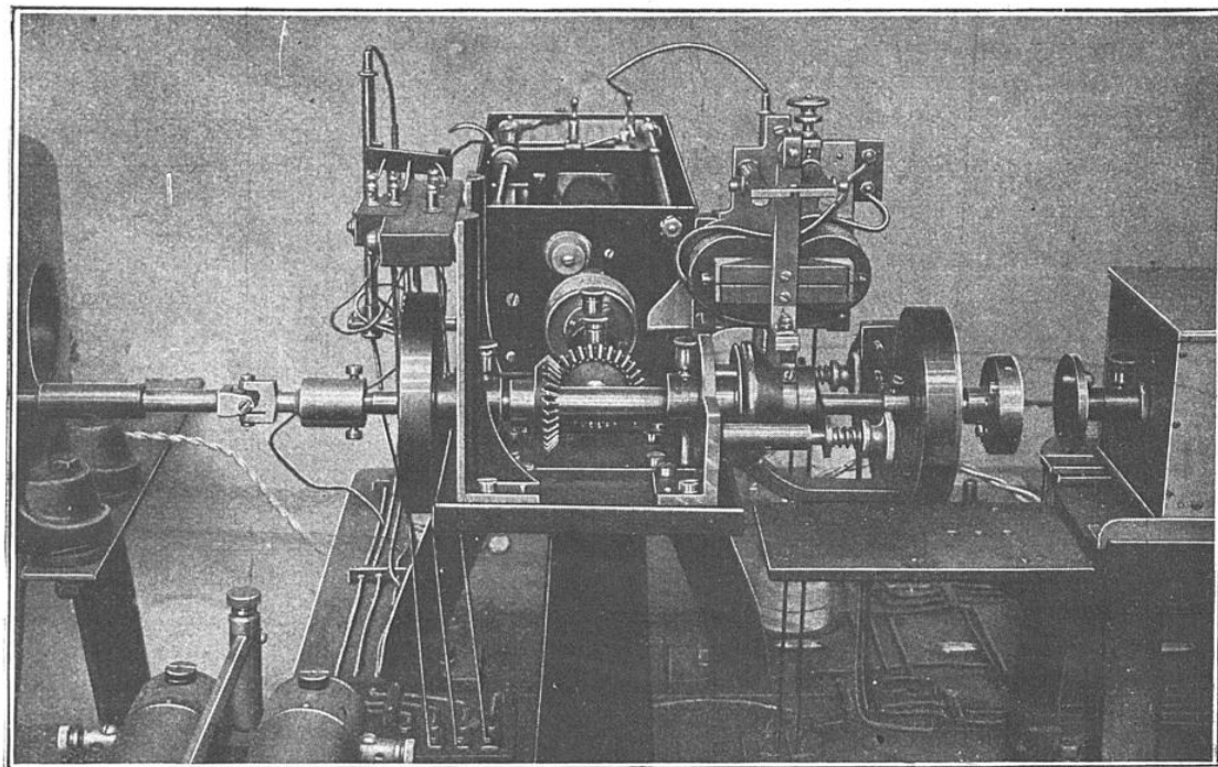
FIG. 6. — ORGANES DE SYNCHRONISATION DE L'APPAREIL KORN
