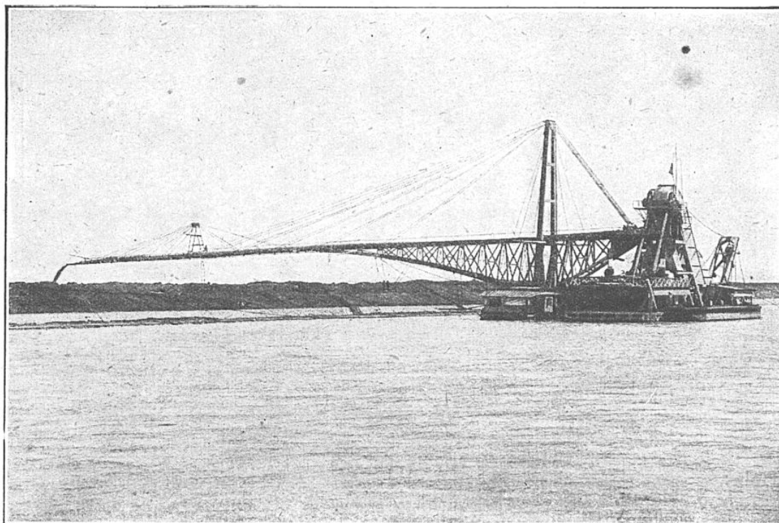
DRAGUE A DÉVERSOIR POSSÉDANT DES GODETS DE 500 LITRES ENVIRON
