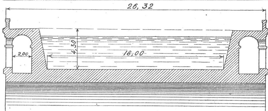
COUPE TRANSVERSALE DU GRAND PONT-CANAL DE LA VALLÉE DE L'OISE
