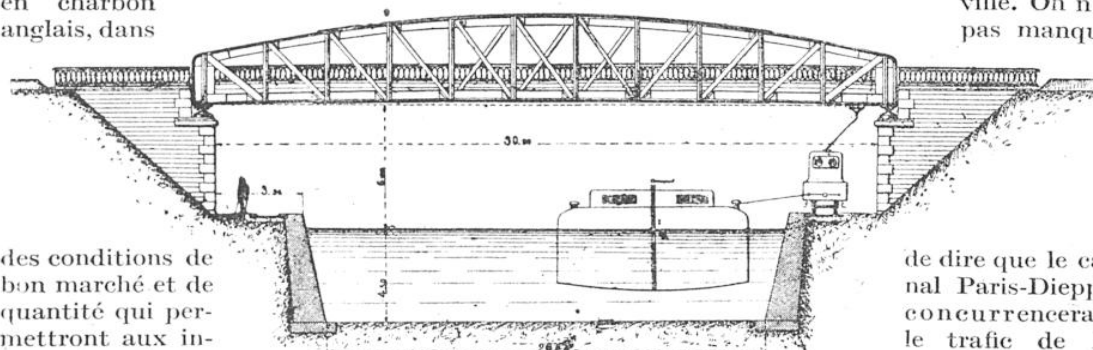
TYPE DE PONT-ROUTE MÉTALLIQUE DE 30 MÈTRES D'OUVERTURE
