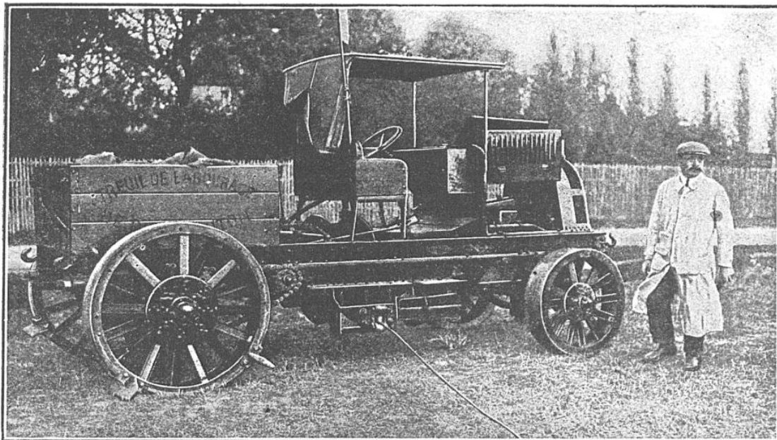
VUE LATÉRALE D'UN TREUIL A ESSENCE POUR LE LABOURAGE PAR CÂBLE
