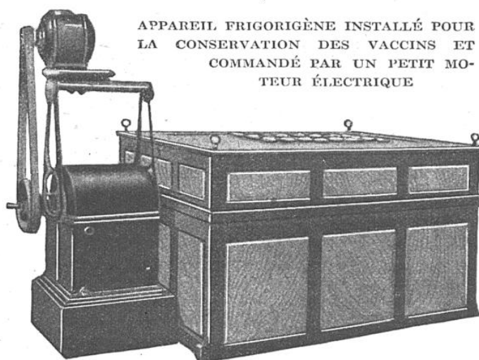
La caisse frigorifique renfermant les vaccins est maintenue par un thermostat extrêmement précis à la température de -15 à -18 degrés au-dessous de zéro.
