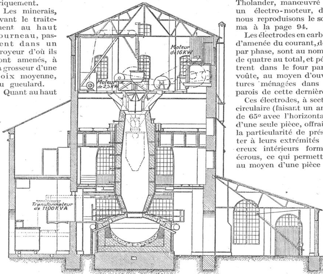
COUPE VERTICALE DU HAUT FOURNEAU ÉLECTRIQUE DE TROLLHATTAN
