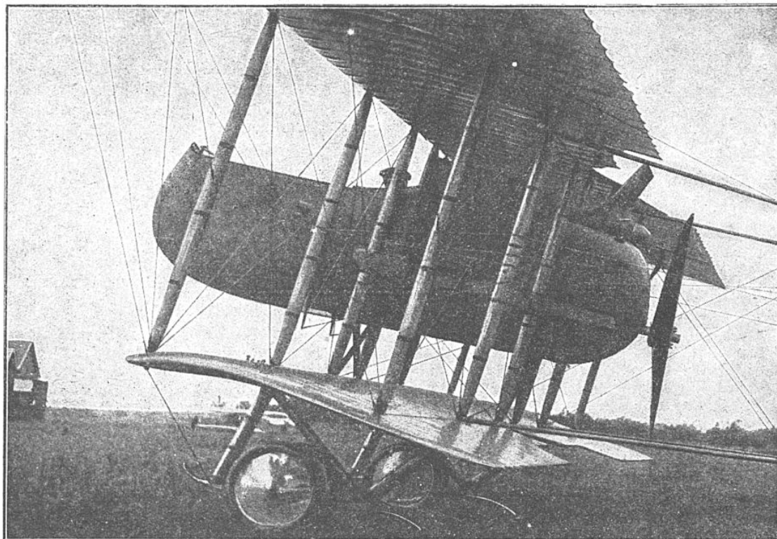
L'INSTALLATION DU GROUPE MOTO-PROPULSEUR SUR UN BIPLAN FARMAN
