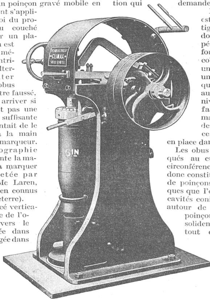
VUE GÉNÉRALE DE L'APPAREIL DE MM. J. ET M. MC LAREN POUR LE MARQUAGE DES OBUS DE MOYEN CALIBRE
