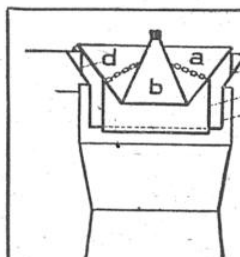
FERMETURE (SYSTÈME THOLLANDER) DU GUEULARD DU HAUT FOURNEAU ÉLECTRIQUE DE TROLLHATTAN
