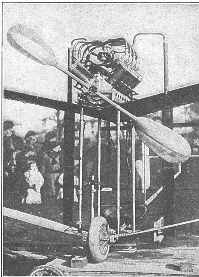
MOTEUR ET HÉLICE SUR L'UN DES PREMIERS AVIONS
