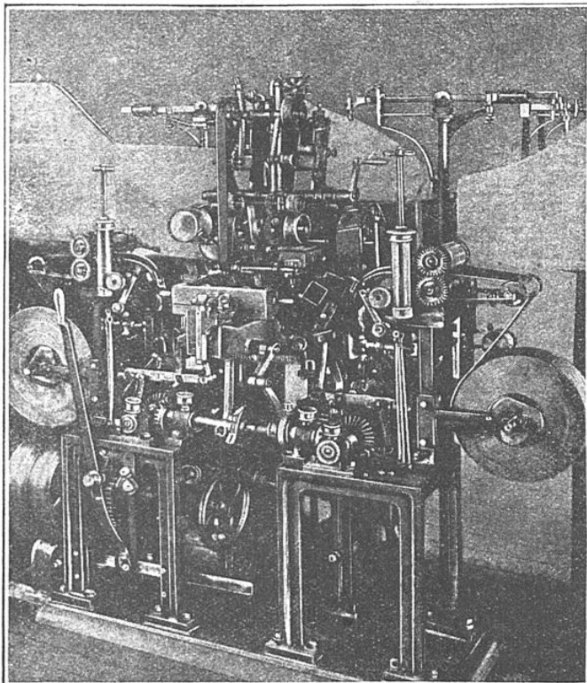
FIG. 13. — MÊME MACHINE QUE LA PRÉCÉDENTE (FIG. 12), MAIS À LAQUELLE ON A ADJOINT LES ORGANES COMPLÉMENTAIRES POUR FABRIQUER AUTOMATIQUEMENT LES SACS DESTINÉS À FORMER LES PAQUETS DE TABAC
