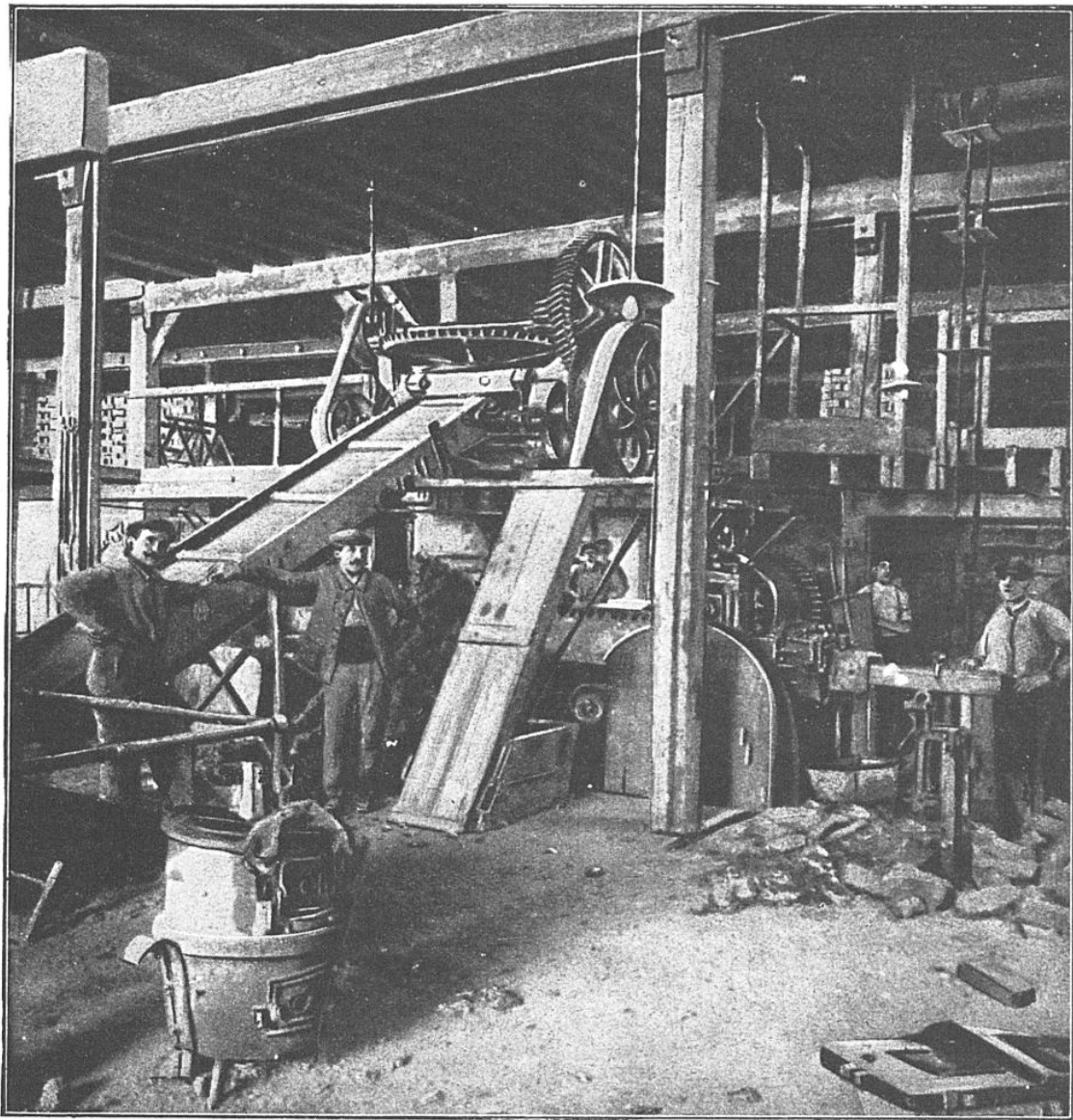
LES INSTALLATIONS DU REZ-DE-CHAUSSÉE D'UNE BRIQUETERIE
