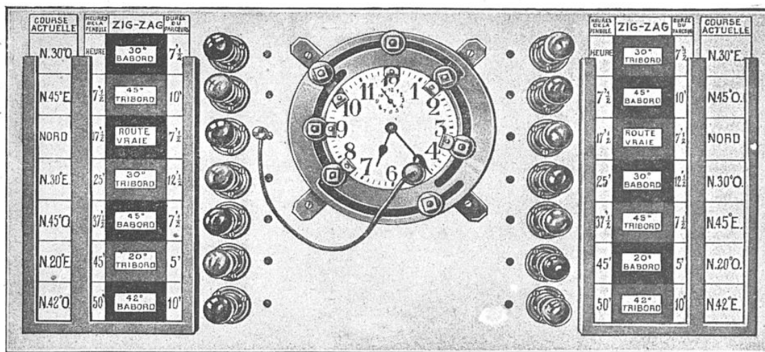
L'APPAREIL SPÉCIAL UTILISÉ POUR LA NAVIGATION EN ZIGZAG
