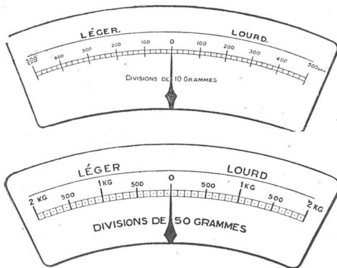
CADRANS GRADUÉS DES BASCULES POOLEY
