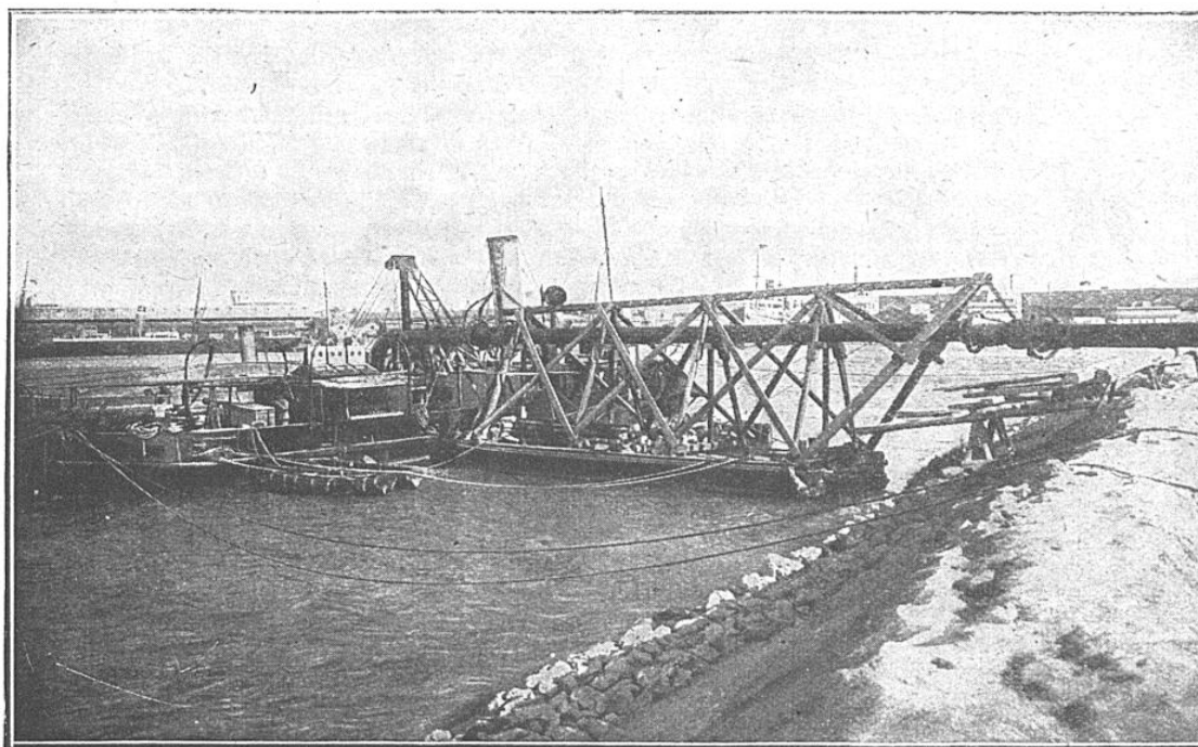
AGENCEMENT DE LA TUYAUTERIE AÉRIENNE D'UNE DRAGUE EXCAVATRICE
