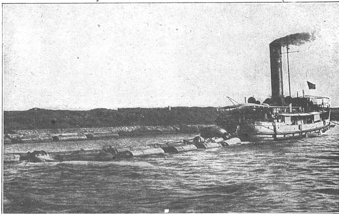
DRAGUE MARINE REMORQUANT SES CONDUITES FLOTTANTES
