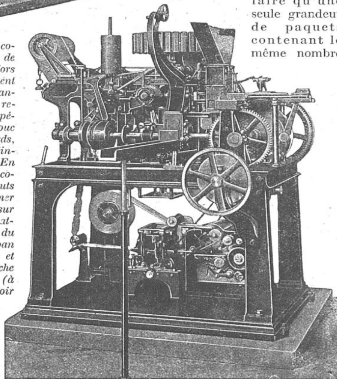
FIG. 20. — MACHINE BOULET, ÉGALEMENT DESTINÉE A METTRE LES CIGARETTES EN PAQUETS
