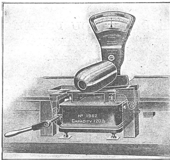
BASCULE AUTOMATIQUE A OBUS, AVEC MANIVELLE SERVANT A PROVOQUER LE DÉCLENCHEMENT DE L'APPAREIL
