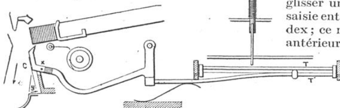
MÉCANISME REPRÉSENTÉ PAR LA FIGURE PRÉCÉDENTE, VU DE PROFIL.
