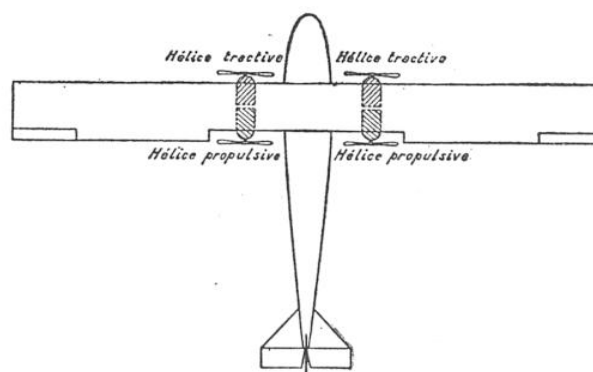
MULTI-MOTEUR A DEUX HÉLICES TRACTIVES ET DEUX HÉLICES PROPULSIVES (LIZENZ ZEPPELIN)
