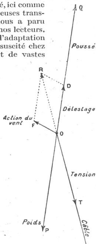
FORCES MISES EN JEU DANS L'ÉQUILIBRE D'UN BALLON CAPTIF (Voir dans le texte l'explication de la figure.)
