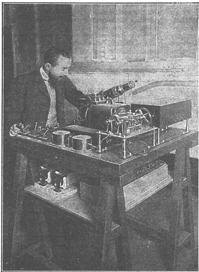
FIG. 8. — PREMIER PHOTOTÉLÉGRAPHE BELIN
