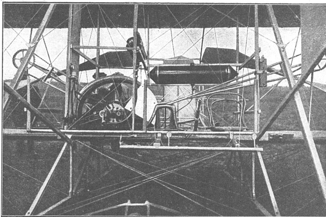
ESSAI D'UN MOTEUR ROTATIF SUR UN AVION WRIGHT (TYPE ANCIEN)
