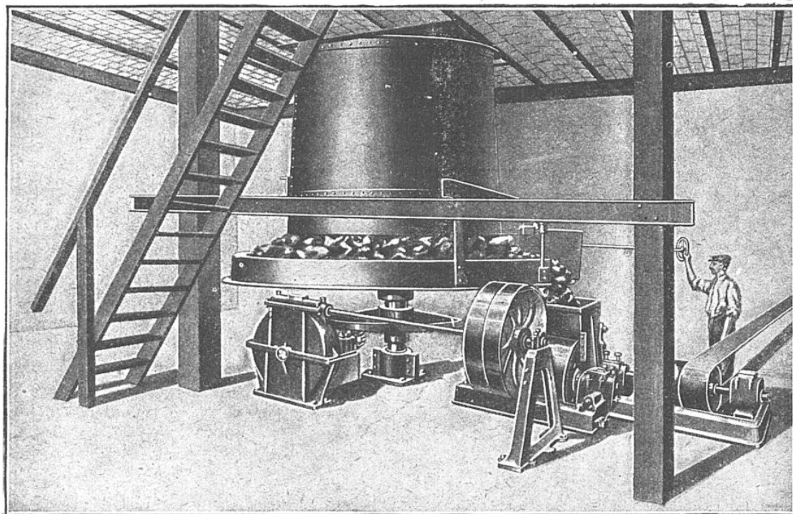
ASPECT GÉNÉRAL DE LA TRÉMIE MÉLANGEUSE-DISTRIBUTRICE
