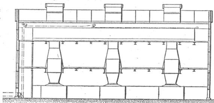
COUPE VERTICALE MONTRANT LA DISPOSITION DES TROIS HAUTS FOURNEAUX ÉLECTRIQUES INSTALLÉS À TINFOS (NORVÈGE)
