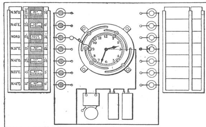
SCHEMA DES TRAJETS DES CONDUCTEURS ÉLECTRIQUES DE L'APPAREIL ZIGZAG
