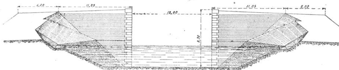
COUPE EN AVANT D'UNE ÉCLUSE, D'APRÈS LE PROJET DÉFINITIF
