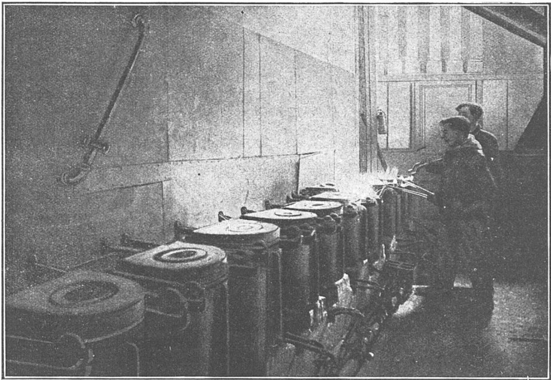
BATTERIE DE FOURS A GAZ SERVANT A OBTENIR LA TEMPÉRATURE DE 1.100 DEGRÉS NÉCESSAIRE A LA FUSION DE L'ALLIAGE DE FER ET DE CÉRIUM
