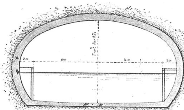
PROFIL EN TRAVERS DU TUNNEL POUR LE PASSAGE SOUTERRAIN DU CANAL A FORGES-LES-EAUX
