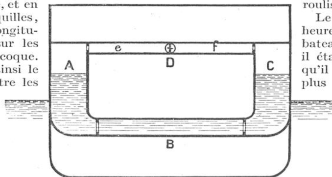
COUPE DU STABILISATEUR A CAISSES D'EAU
