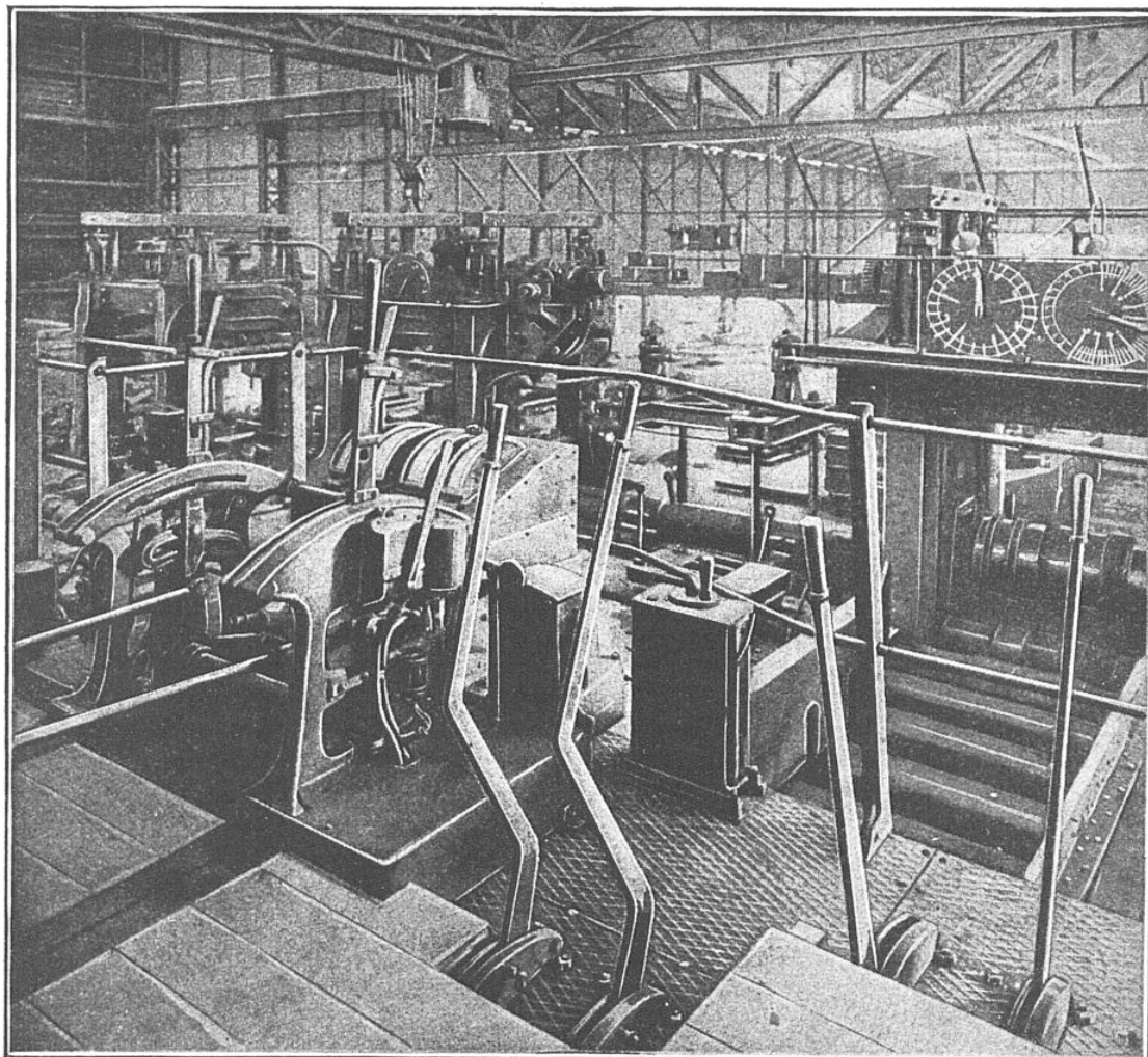
PLATE-FORME DU CHEF LAMINEUR DANS UN LAMINOIR A COMMANDE ÉLECTRIQUE
