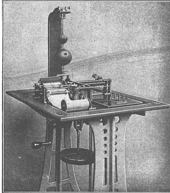
FIG. 3. — TÉLÉGRAPHE AUTOGRAPHIQUE INVENTÉ PAR L'EMPLOYÉ DES P. T. T. MEYER
