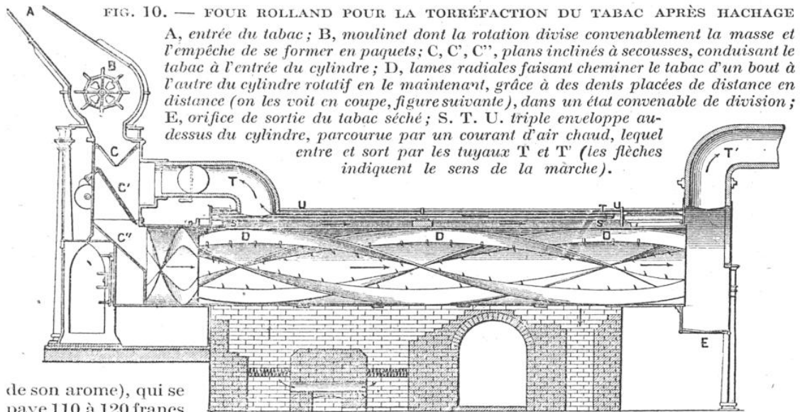
FIG. 10. — FOUR ROLLAND POUR LA TORRÉFACTION DU TABAC APRÈS HACHAGE
