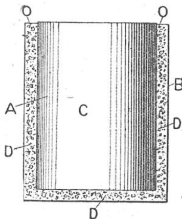
FIG. 1. — BOÎTE DE CONSERVE QUI SE CHAUFFE AUTOMATI- QUEMENT AVEC UN PEU D'EAU FROIDE
