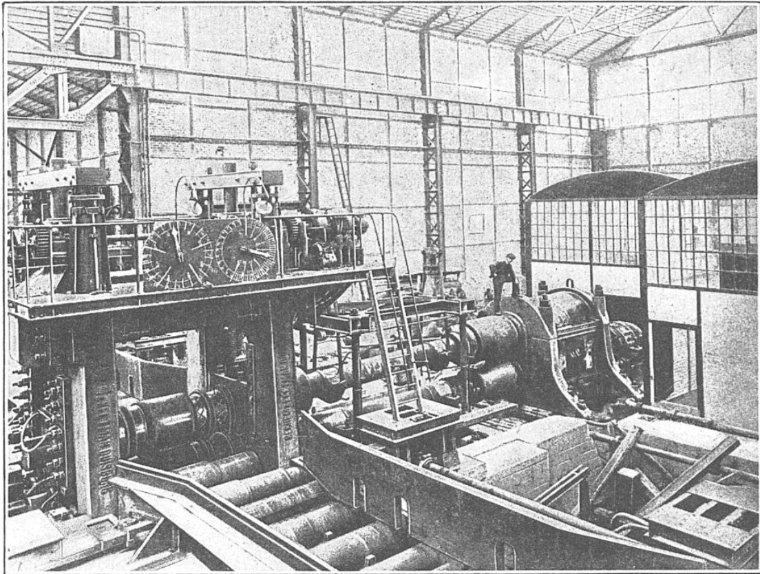
LAMINOIR ÉLECTRIQUE SYSTÈME SIEMENS DES ACIÉRIES DE SKINNINGROVE
