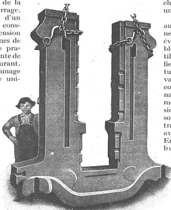
FLASQUE DE LAMINOIR EN ACIER MOULÉ, PESANT 5.500 KILOGRAMMES
