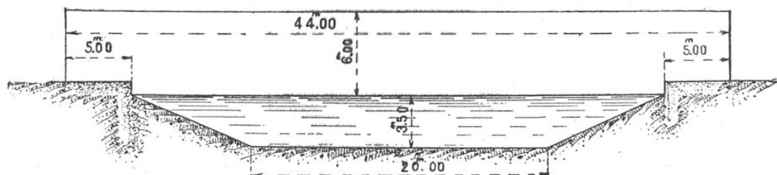
OUVERTURE DES PONTS MÉTALLIQUES JETÉS SUR LE CANAL (ÉTUDES PRÉLIMINAIRES)
