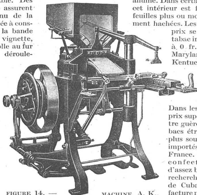
FIGURE 14. — MACHINE A. K., DE M. BELOT, POUR LA FABRICATION DES « POUPÉES » DE CIGARES
