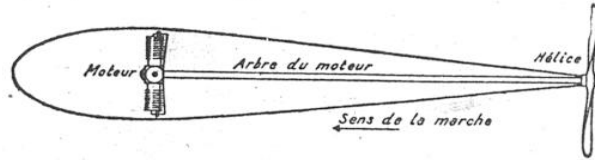
COUPE SCHÉMATIQUE DE LA TORPILLE PAULHAN-TATIN
