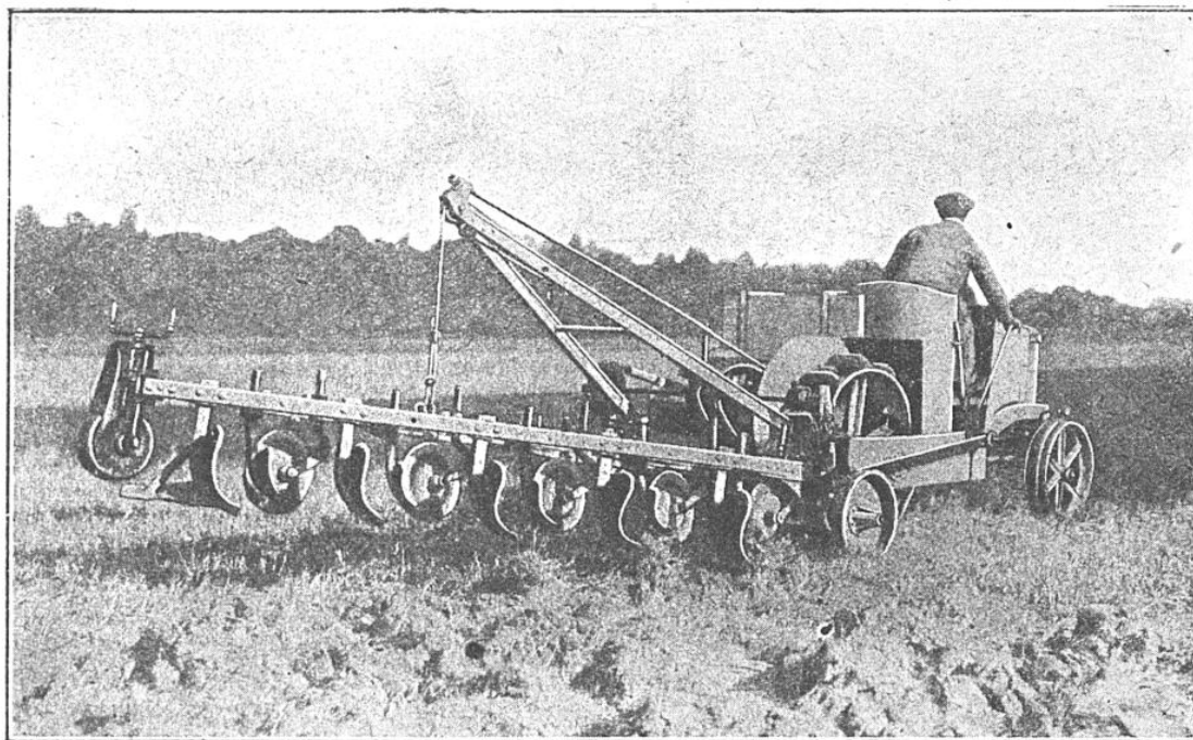
LE SYSTÈME DE RELEVAGE DE LA CHARRUE AUTOMOBILE TOURAND-LATIL
