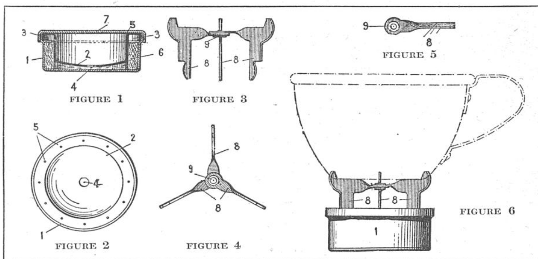
PLANCHE 2. — RÉCHAUD DE POCHÉ POUR SOLDATS EN CAMPAGNE OU EN MANŒUVRES
