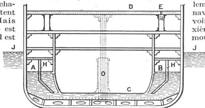
COUPE D'UN NAVIRE MUNI DE STABILISATEURS A CAISSES D'EAU AU-DESSOUS DE LA FLOTTAISON
