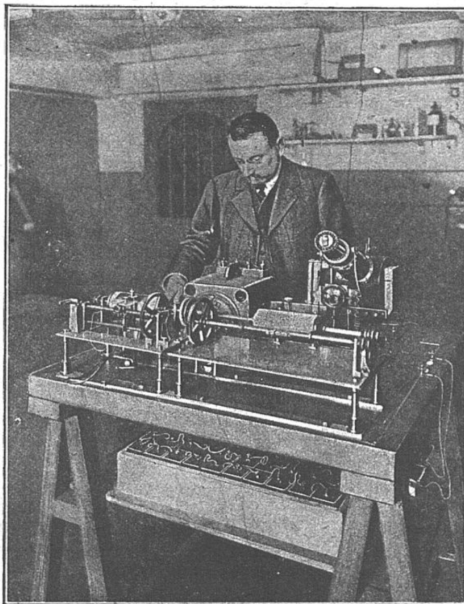
FIG. 10. — APPAREIL PHOTOTÉLÉGRAPHIQUE SYSTÈME BELIN (1907), VU DE FACE
