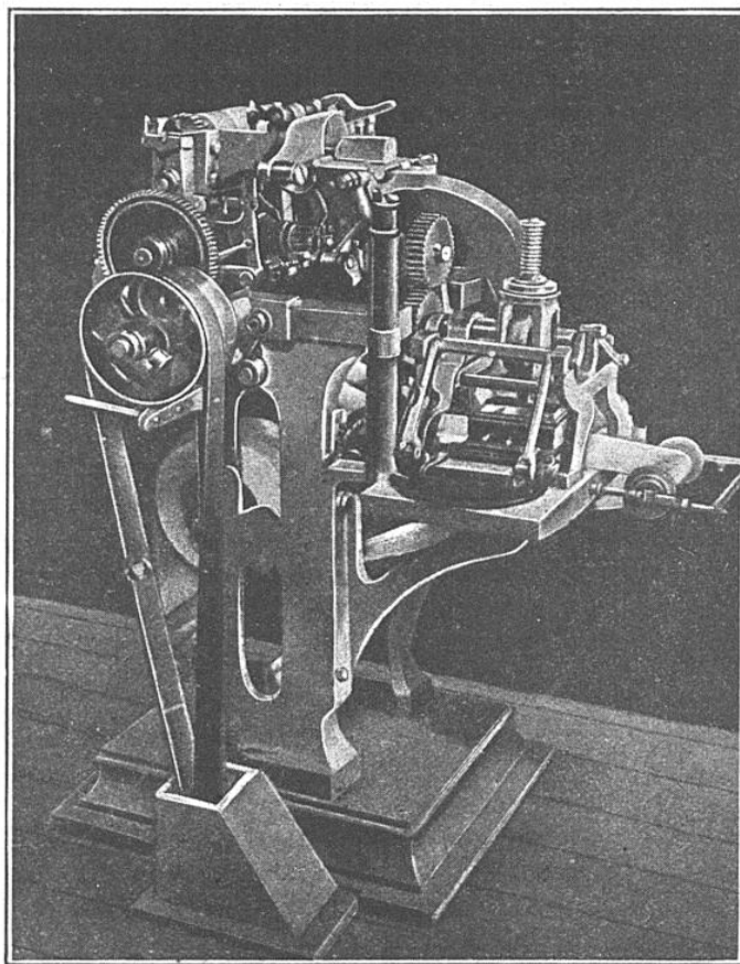
FIG. 18. — MACHINE SPÉCIALE A FABRIQUER LES CIGARETTES EN PAQUETS DITS « BONDONS »
