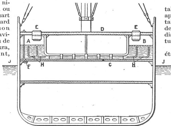
COUPE D'UN NAVIRE MUNI DE STABILISATEURS A CAISSES D'EAU AU-DESSUS DE LA FLOTTAISON
