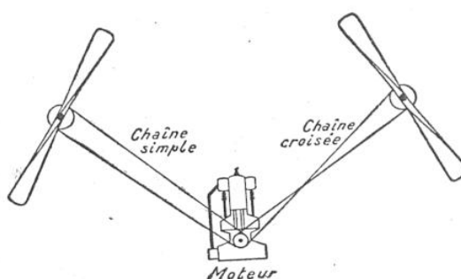
LA TRANSMISSION A DEUX CHAINES ADOPTEE PAR LES FRÈRES WRIGHT
