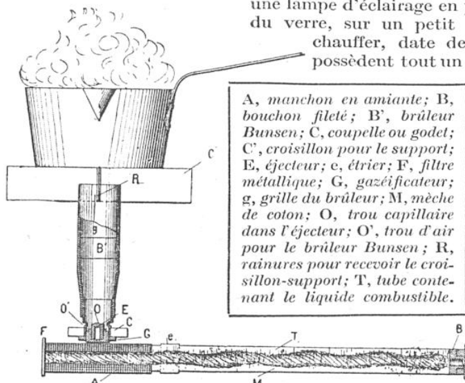
FIG. 13. — COUPE DU RÉCHAUD PORTATIF LANDI
