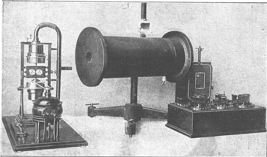
VUE GÉNÉRALE DU THERMOMÈTRE WATSON ET BOOTH ET DE SES DIVERS ACCESSOIRES
