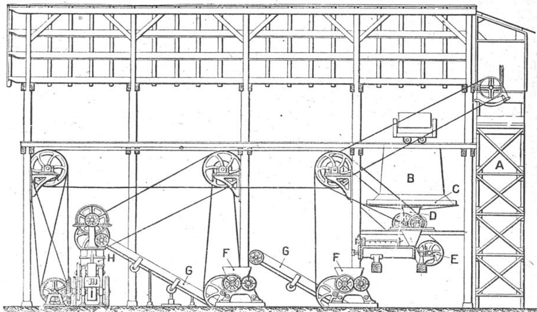
ENSEMBLE D'UNE INSTALLATION DE BRIQUETERIE MODERNE
