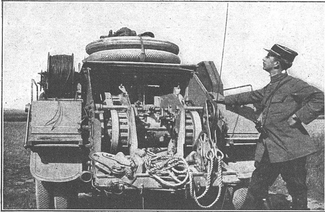
TREUIL DE MANŒUVRE DU LIEUTENANT-COLONEL SACONNEY, VU DE L'ARRIÈRE
