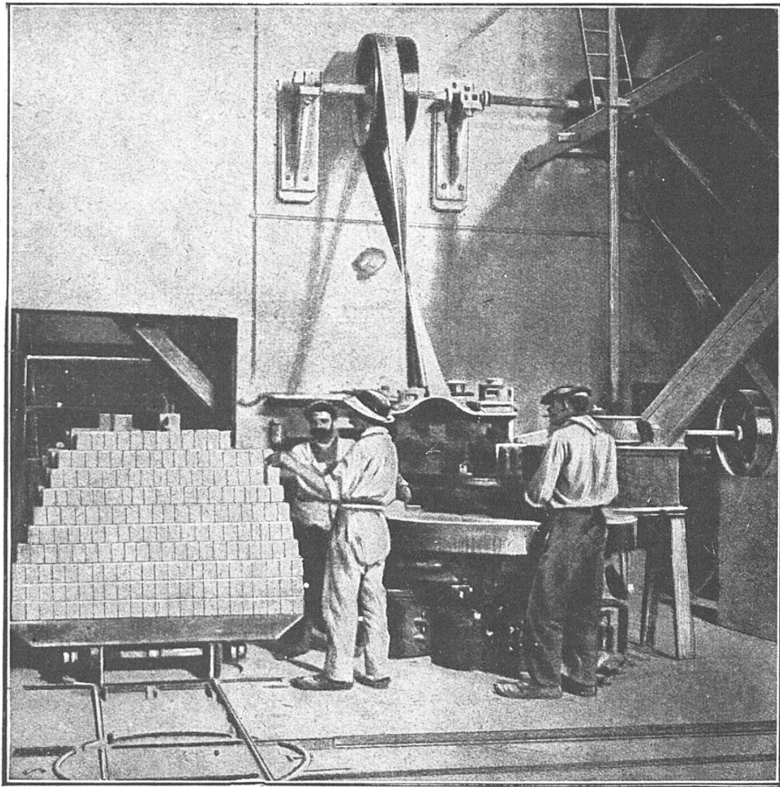
LA FABRICATION DES BRIQUES SPÉCIALES SILICO-CALCAIRES
