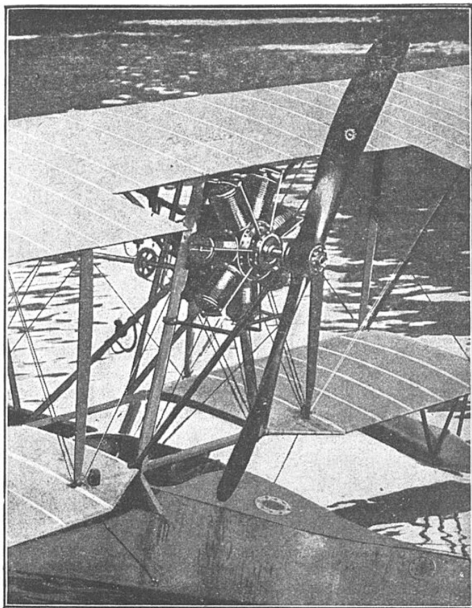
LE GROUPE PROPULSEUR D'UN HYDRAVION
