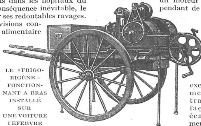
Ce type spécial produit cinq kilogrammes de glace à l'heure. Un autre modèle, installé de la même façon, fonctionne au moyen d'un moteur à essence.
