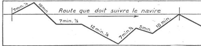
DIAGRAMME ÉTABLI PAR LES CAPITAINES DE NAVIRES QUI UTILISENT L'APPAREIL ZIGZAG
