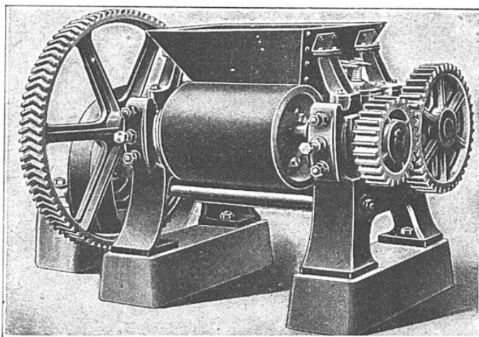
UNE PAIRE DE CYLINDRES BROYEURS
