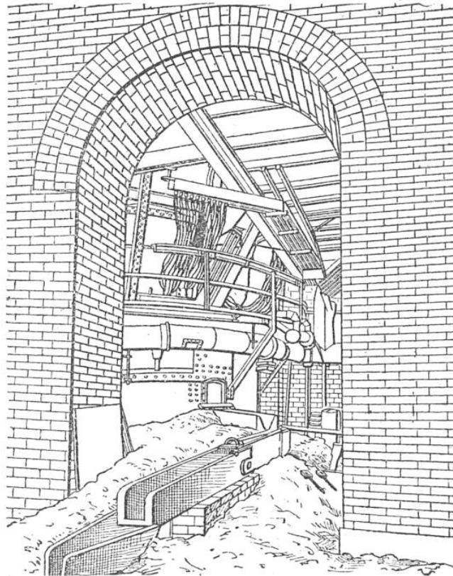
VUE ANTÉRIEURE D'UN HAUT FOURNEAU ÉLECTRIQUE INSTALLÉ A TROLLHATTAN (SUÈDE)
