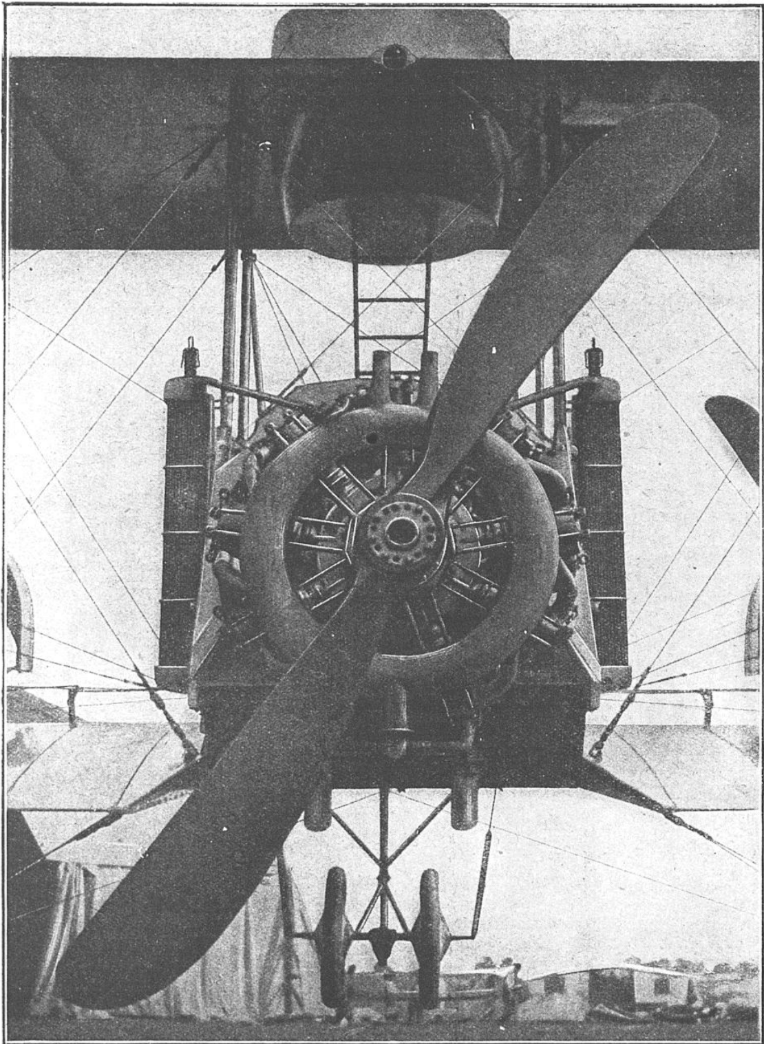
GROUPE MOTO-PROPULSEUR ARRIÈRE SUR UN BIPLAN ITALIEN CAPRONI.
