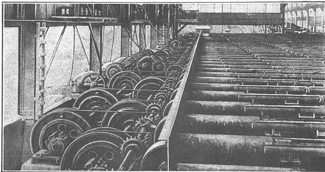
HALL DE LAMINAGE ÉLECTRIQUE DANS UNE ACIÉRIE AMÉRICAINE
