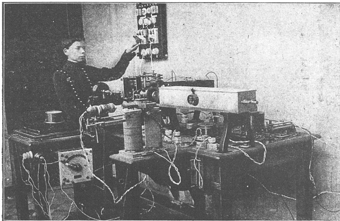
FIG. 7. — POSTE TÉLÉPHOTOGRAPHIQUE INSTALLÉ DANS UN JOURNAL PARISIEN
