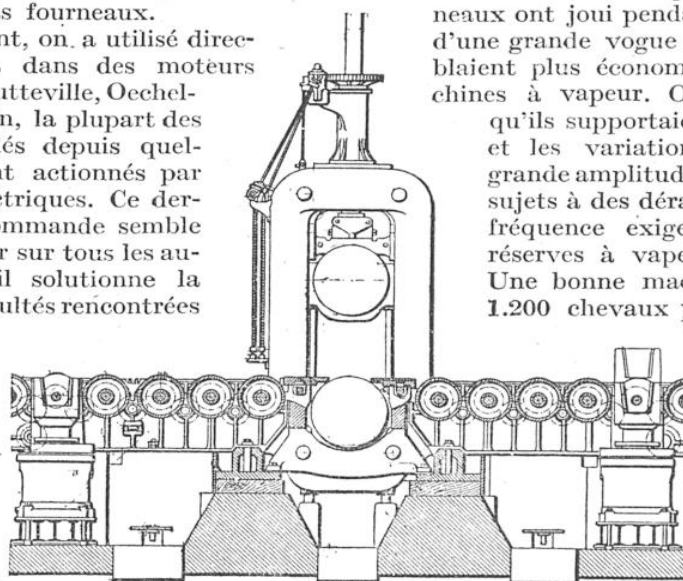
VUE LATÉRALE SCHÉMATIQUE D'UN LAMINOIR A COMMANDE ÉLECTRIQUE
