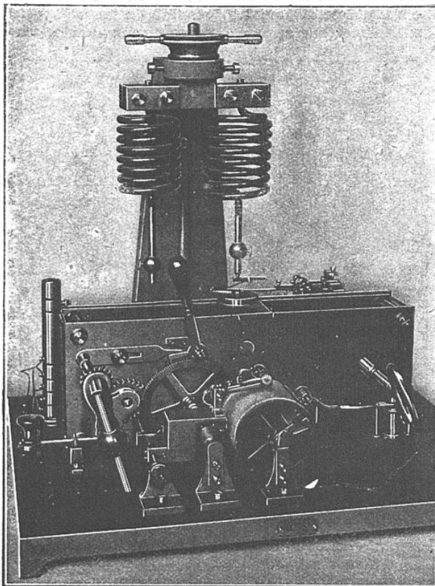
FIG. 4. — APPAREIL DE D'ARINCOURT (1872)
