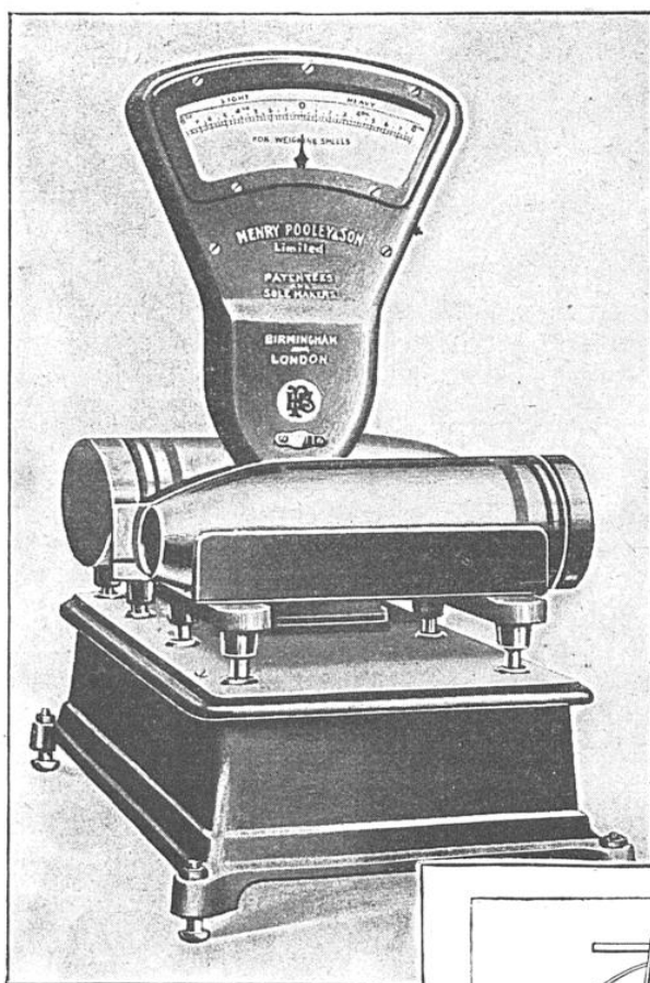
BALANCE GENRE ROBERVAL POUR LE CONTROLE DES OBUS DE 75 A 120 MILLIMÈTRES
