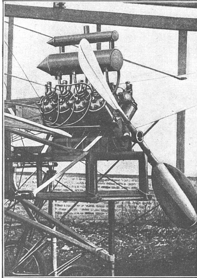
LE MOTEUR D'UN AVION EN 1908
