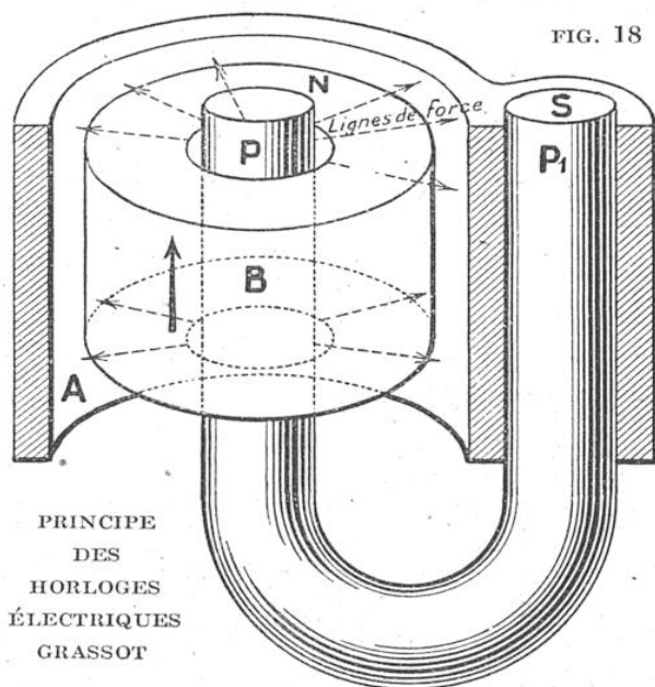
PRINCIPE DES HORLOGES ÉLECTRIQUES GRASSOT P P 1 , aimant permanent ; A, anneau métallique entourant l'aimant permanent et la bobine B. — Sous l'action des courants transmis par l'horloge distributrice, la bobine se déplace dans le sens de la flèche (verticale sur notre dessin). Ces déplacements sont utilisés pour actionner le mécanisme récepteur.
