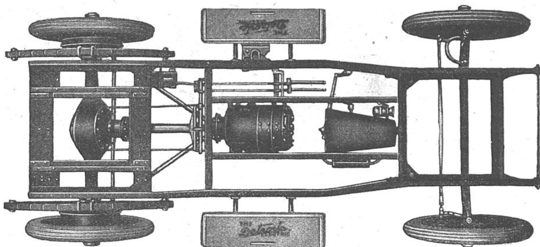
CHASSIS, COMBINEUR ET MOTEUR D'UNE AUTO ÉLECTRIQUE
