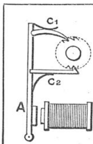
FIG. 24. — LE ROCHET EST ACTIONNÉ ALTERNATIVEMENT ET TOUJOURS DANS LE MÊME SENS PAR LES CLIQUETS C 1 ET C 2 SOUS L'ACTION DES MOUVEMENTS DU BARREAU AIMANTÉ A
