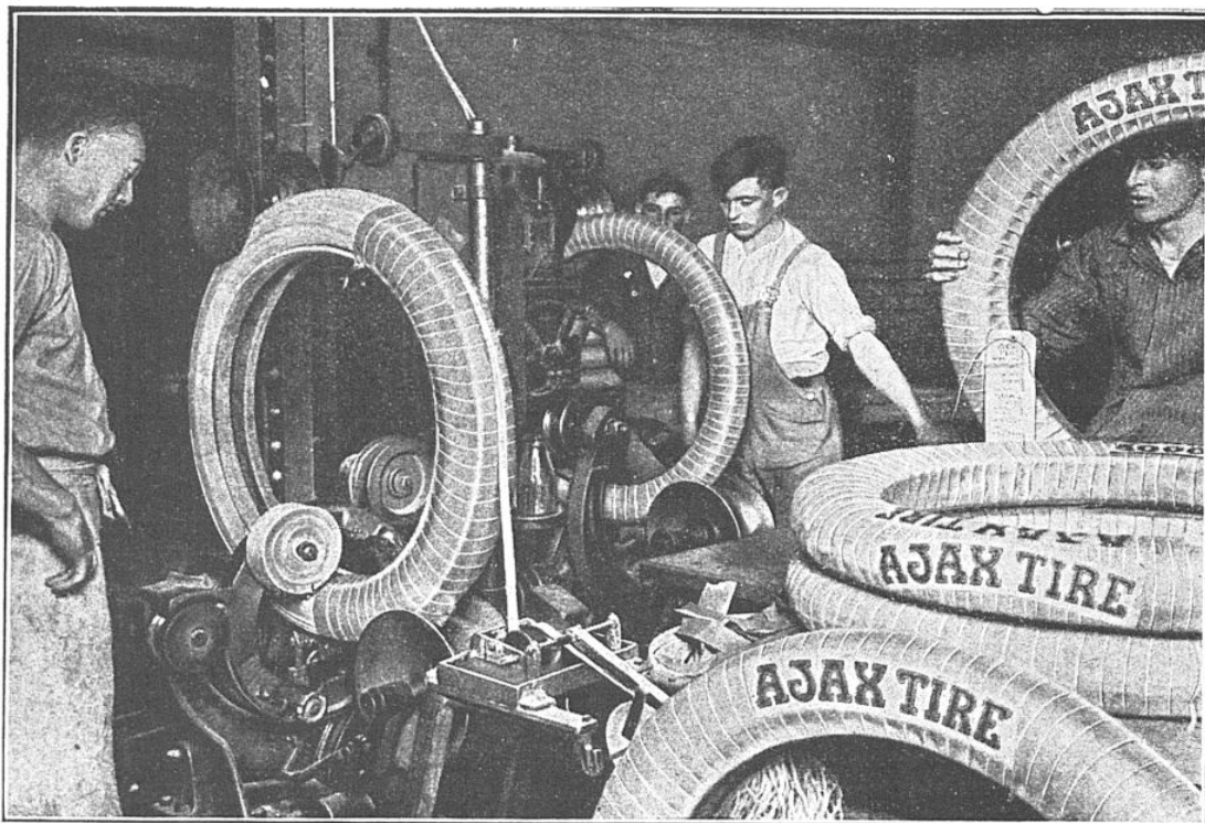
AVEC CETTE MACHINE, RELATIVEMENT SIMPLE, UNE MINUTE SUFFIT POUR ENVELOPPER COMPLÈTEMENT DE PAPIER UN PNEUMATIQUE D'AUTOMOBILE
