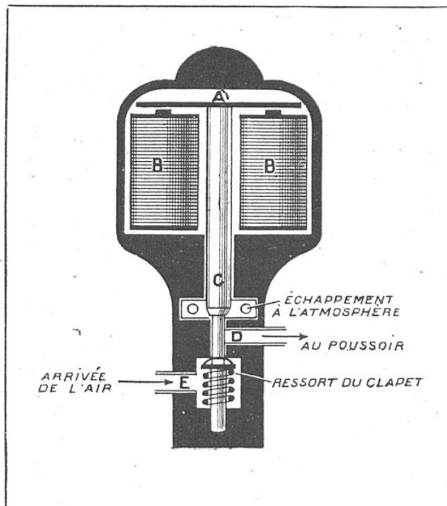
SCHÉMA DE LA VALVE ÉLECTRO-PNEUMATIQUE
