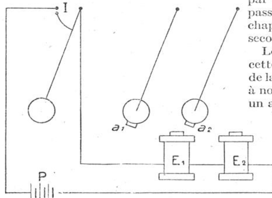
FIG. 7. — PRINCIPE DES HORLOGES SYNCHRONISÉES
