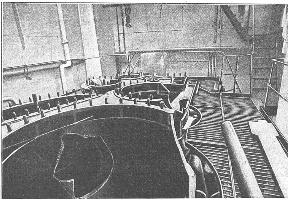
DÉCHIRURE VOLONTAIRE FAITE AU CYLINDRE A BASSE PRESSION DE L'« ALFENAS »
