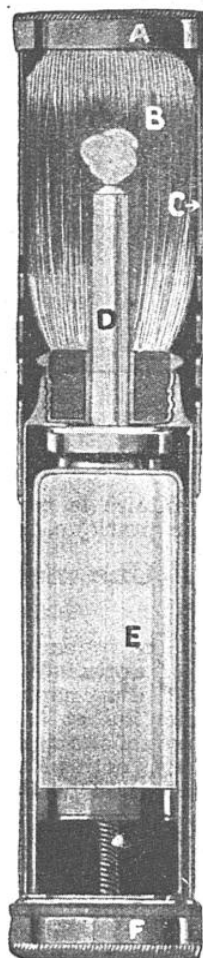
A, couvercle ; B, blaireau ; C, étui télescopique ajouré ; D, tube de caoutchouc amenant la crème de savon E dans le blaireau lorsque le bouton F est tourné.
