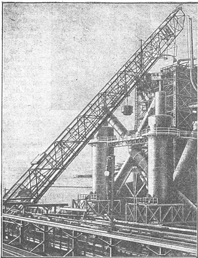
VUE PARTIELLE DES HAUTS FOURNEAUX LORRAINS D'AUMETZ-LA-PAIX, A KNUTANGE
