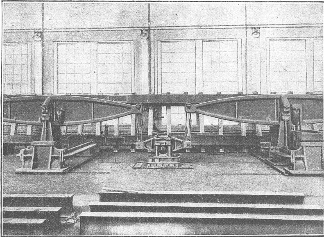
AGENCEMENT DES COUTEAUX ET DES LEVIERS DE LA BASCULE GÉANTE
