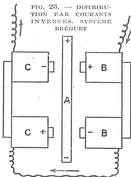
A , barreau aimanté; B , C , électro-aimants polarisés. Sous l'action des courants inversés, le barreau aimanté est porté alternativement vers la droite et vers la gauche. Ces mouvements sont utilisés pour actionner le rochet. (Voir la figure suivante.)
