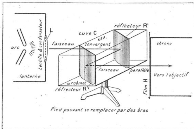
VUE PERSPECTIVE DE LA CUVE EN CRISTAL OU EN VERRE RENFERMANT LES RÉFLECTEURS
