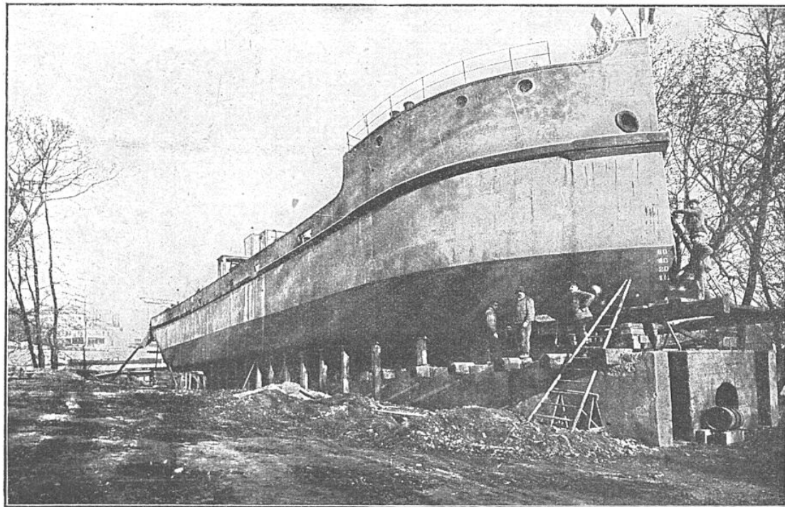
LE CARGO-BOAT EN CIMENT ARMÉ EST PRÊT A ÊTRE LANCÉ
