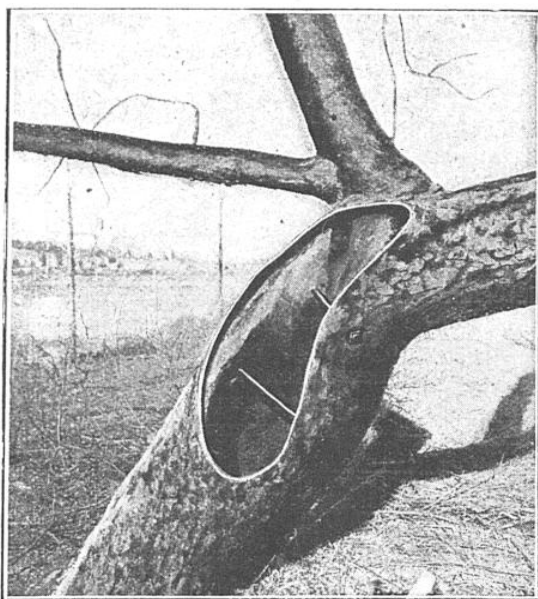
FIG. 2 — LES DEUX LÈVRES DE LA PLAIE SONT MAINTENUES SOLIDEMENT PAR DES LONGS TIRE-FONDS DE FER
