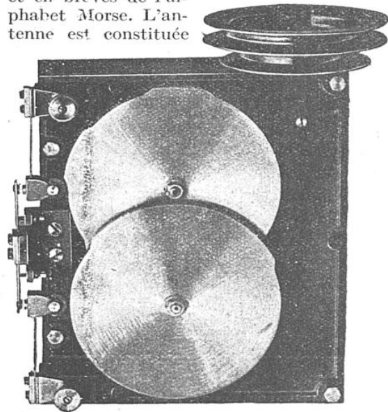
FIG. 5. — ÉMETTEUR AUTOMATIQUE BLONDEL
