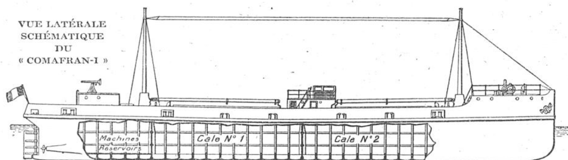
Ce dessin montre la structure générale du navire et le quadrillage formé par les membrures et les serres. Cinq cloisons étanches divisent la coque en six compartiments. Le déplacement total du navire est de 964 tonnes, son port en lourd est de 550 tonnes et sa cargaison en charbon de 500 tonnes, soit 250 par cal.
