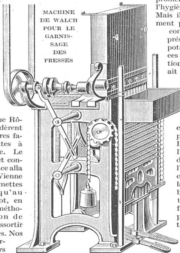
La presse est placée verticalement devant la machine, suspendue à deux chaînes de Galle, à contrepoids. Une pédale, qui actionne aussi les autres organes, la fait descendre d'un cran à chaque mouvement, afin que la règle supérieure (c'est-à-dire la dernière mise en place) soit toujours à un niveau qui lui permette de recevoir les tiges qui lui sont envoyées.
