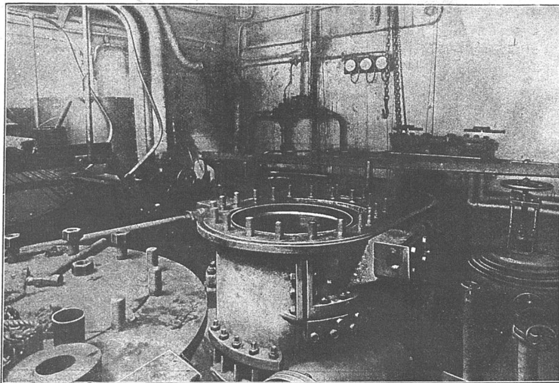
ASPECT D'UN RÉPARATION DE CYLINDRE SUR L'« ARACAJU », EX-« PERSIA »
