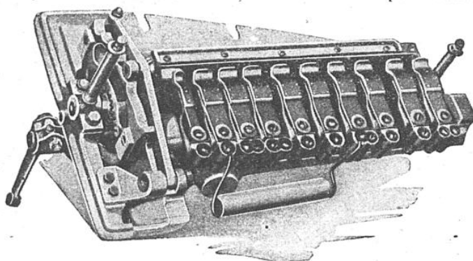
La voiture électrique ne comportant pas de changement de vitesse, c'est par l'intermédiaire de cet organe que l'on règle le régime du moteur et, par conséquent, l'allure de l'automobile. Le combineur joue, en somme, le rôle d'un rhéostat.
