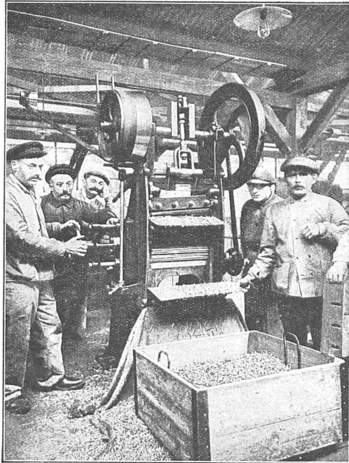
VUE AVANT DE LA MACHINE SEVÈNE ET CAHEN
