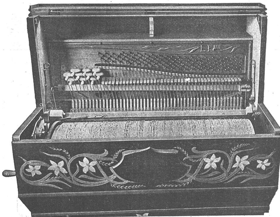
INTÉRIEUR D'UN PIANO MÉCANIQUE A CYLINDRE
