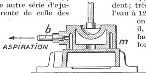
COUPE TRANSVERSALE DU PATIN SYSTÈME MANIGUET ET DU RAIL ASSUJÉTI DANS SA TRAVERSE
