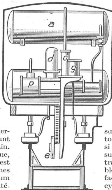
VUE EN COUPE TRANS- VERSALE DE LA MA- CHINE PRÉCÉDENTE
