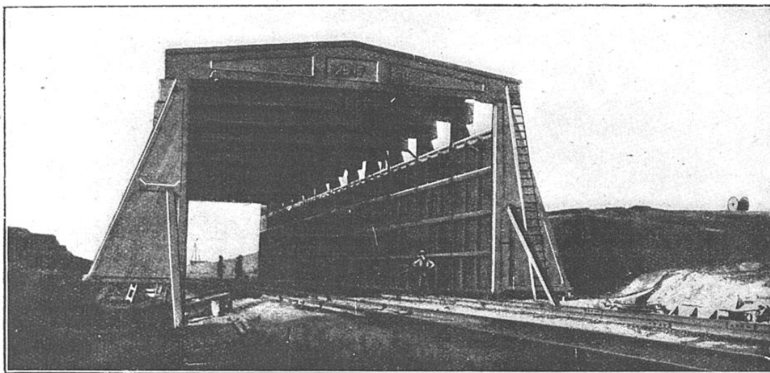
TUNNEL PARA-NEIGE EN CIMENT ARMÉ EN COURS DE CONSTRUCTION
