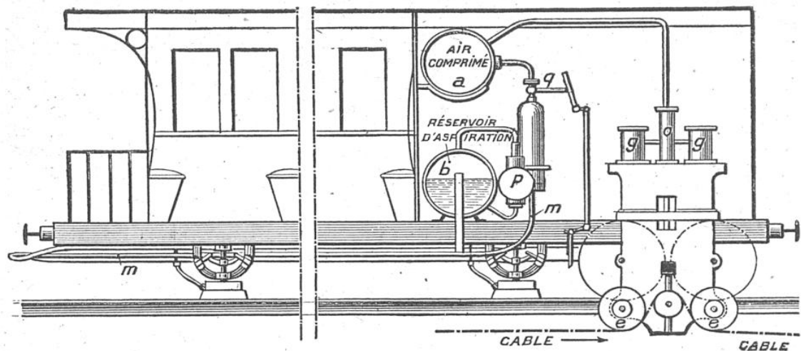
CHEMIN DE FER GLISSANT A PATINS ET A TRACTION FUNICULAIRE, SYSTÈME MANIGUET (COUPE LONGITUDINALE MONTRANT LES DIVERS MÉCANISMES)
