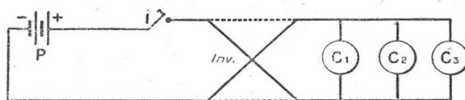
FIG. 22. — PRINCIPE DE DISTRIBUTION ÉLECTRIQUE DE L'HEURE PAR COURANTS INVERSES
