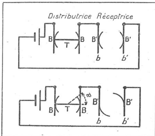
FIG. 35. — SCHÉMAS EXPLIQUANT LE FONCTIONNEMENT DU SYSTÈME O'KEENAN T, tambour; B B', balais du distributeur; b b', balais du récepteur.
