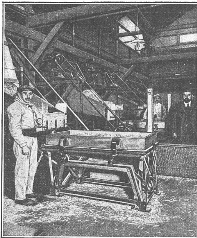
PUIS LES TIGES TOMBENT SUR DES TABLES A SECOUSSES POURVUES DE GRILLAGES A MAILLES RECTANGULAIRES
