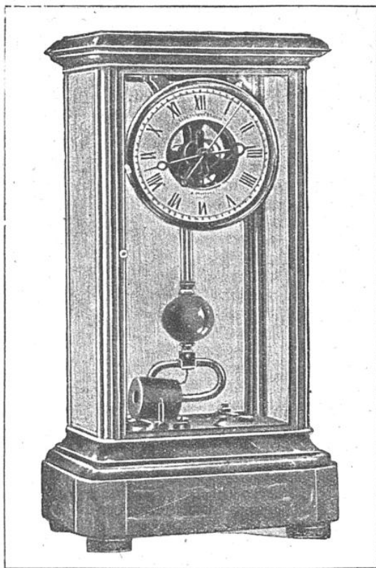
FIG. 8. — RÉGULATEUR ÉLECTRIQUE SYSTÈME BRILLIÉ
