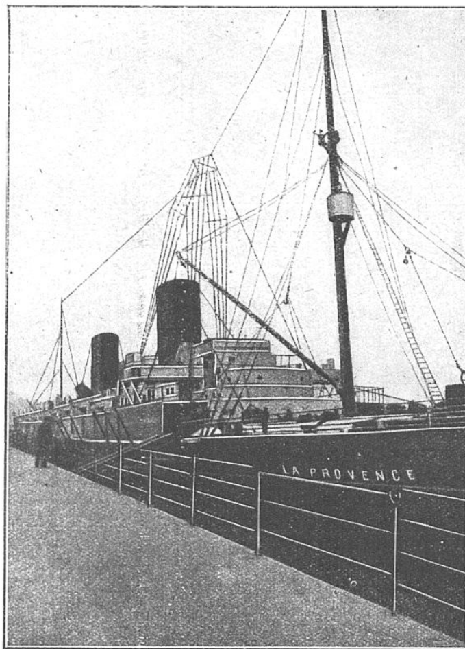
FIG. 9. — INSTALLATION DES ANTENNES SUR LE PAQUEBOT « LA PROVENCE »
