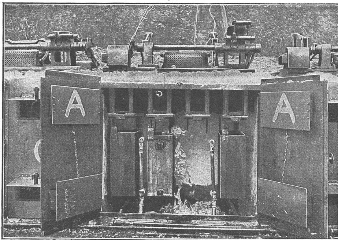
UNE DES CELLULES D'INTERRUPTION ÉQUIPÉE POUR L'EXPÉRIENCE
