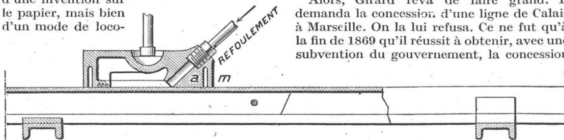
PATIN SYSTÈME MANIGUET A REFOULEMENT ET ASPIRATION
