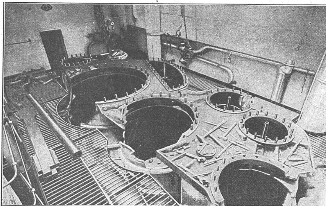
VUE DES CYLINDRES DU STEAMER « ALFENAS », PRÉCÉDEMMENT « SAN-NICOLAS »
