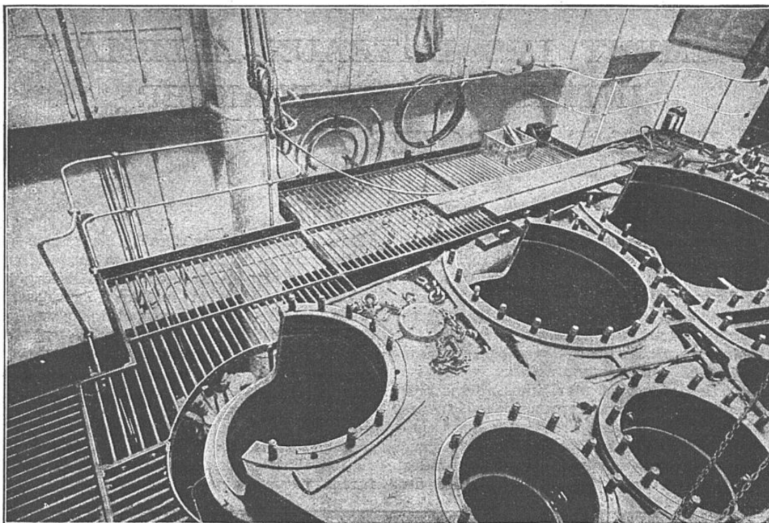
VUE DES CYLINDRES INTERMÉDIAIRES DU VAPEUR « BAEPENDY », EX-« TIJUCA »
