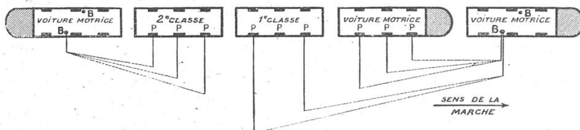
COMPOSITION D'UN TRAIN DE LA LIGNE N° 1 (PORTE-MAILLOT-VINCENNES)
