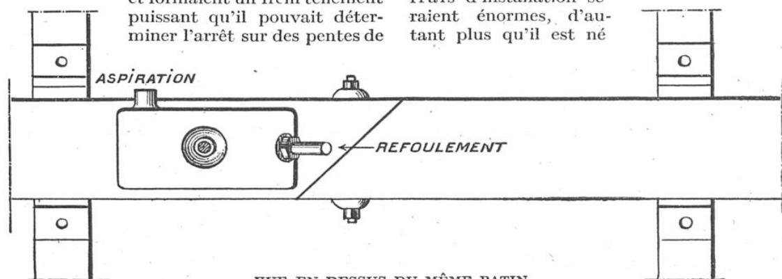
VUE EN DESSUS DU MÊME PATIN, MONTRANT, EN OUTRE, LA JONCTION EN BISEAU DE DEUX RAILS ABOUTÉS ET LES TRAVERSES
