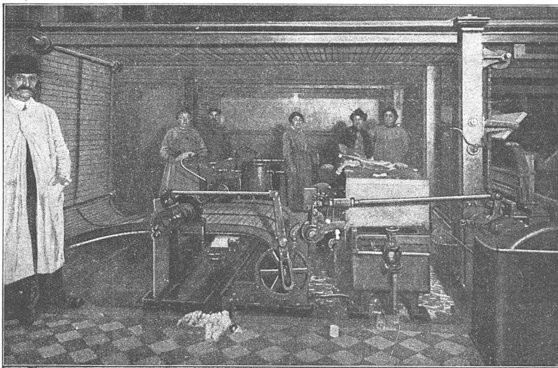
L'OPÉRATION DU « CHIMICAGE » PAR LA MACHINE SEVÈNE ET CAHEN
