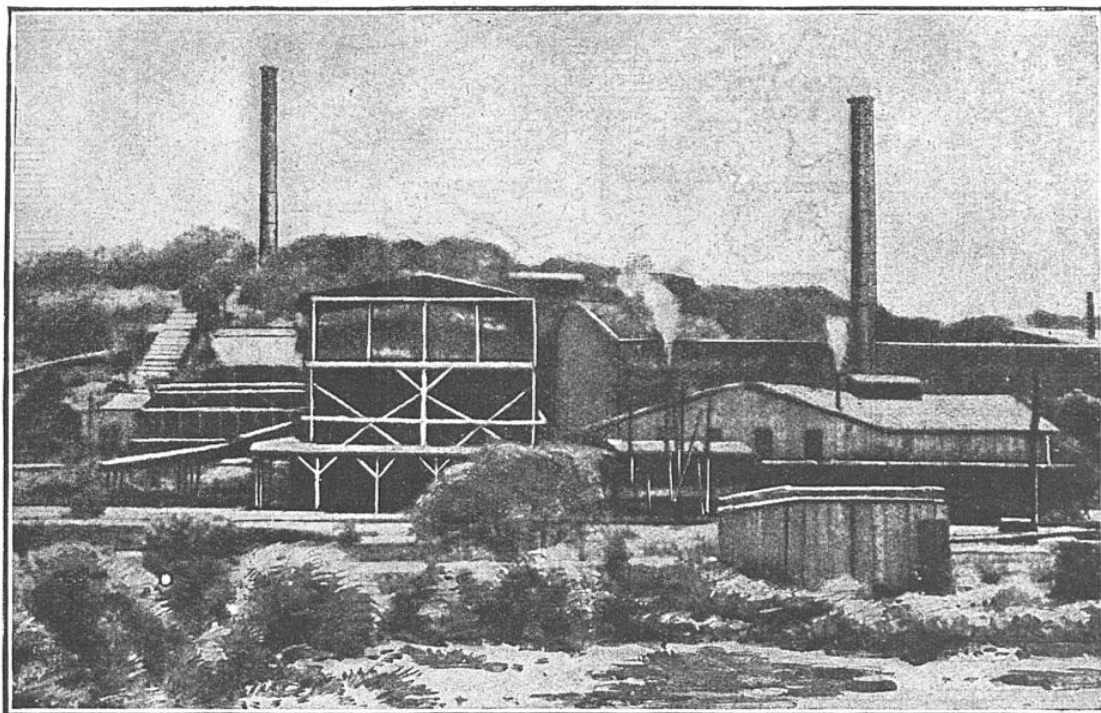
USINE CONSTRUITE PAR LES ALLEMANDS A TSOUMEB (SUD-OUEST AFRICAINE)
