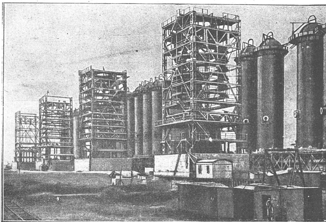
BATTERIE DE HAUTS FOURNEAUX MODERNES A HAGONDANGE (USINES THYSSEN)
