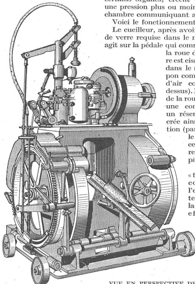
VUE EN PERSPECTIVE DE LA MACHINE WILZIN MUNIE D'UN DISPOSITIF DE COMPRESSION INITIALE DE LA PARAISON
