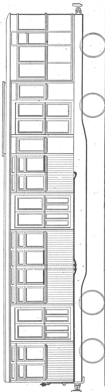
LA CANALISATION QUI ALIMENTE LES POUSSOIRS NE S'ÉTEND PAS SUR TOUTE LA LONGUEUR DE CETTE VOITURE. Toutes les portes de cette motrice peuvent être fermées automatiquement par l'intermédiaire de la valve électro-pneumatique qui se trouve à l'extrémité postérieure de la voiture. Un seul poussoir par porte est suffisant pour faire jouer simultanément les deux panneaux, puisque ceux-ci sont conjugués.
