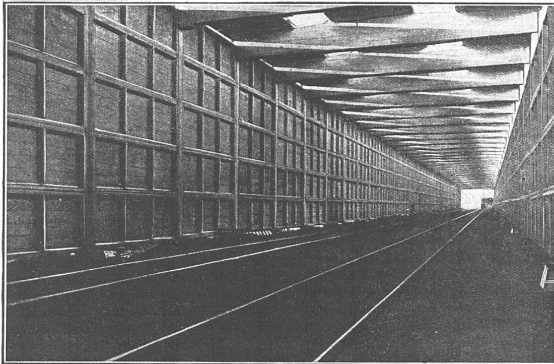
VUE INTÉRIEURE D'UN TUNNEL PARANEIGE EN CIMENT ARMÉ
