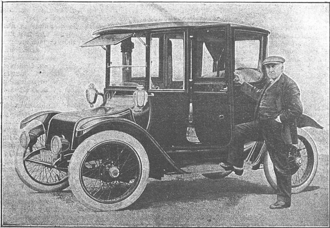
LA VOITURE ÉLECTRIQUE DE L'ILLUSTRE INVENTEUR AMÉRICAIN THOMAS EDISON Cette voiture, construite dans les ateliers de l'Anderson Electric Car Company, à Detroit, a un rayon d'action de 95 à 130 kilomètres. Sa vitesse est de 35 kilomètres à l'heure, ce qui est suffisant pour son usage spécial ; son poids total est, en ordre de marche, de 1.700 kilogrammes.
