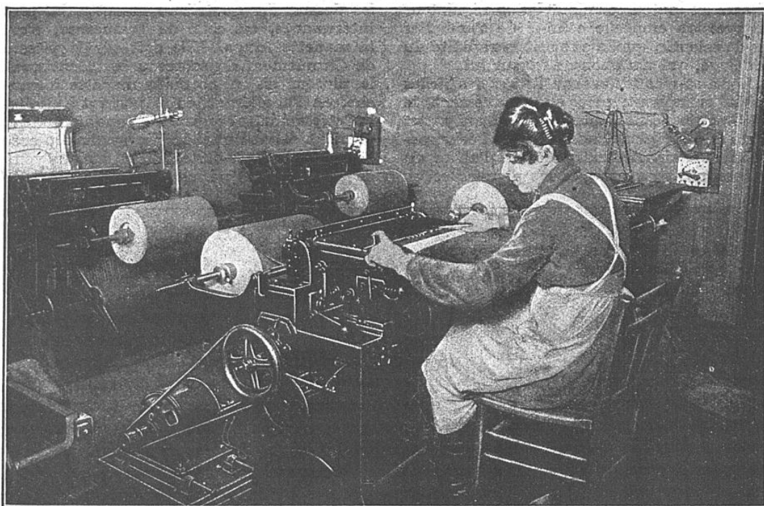
MACHINE SPÉCIALE SERVANT A LA PERFORATION DU CARTON MUSICAL
