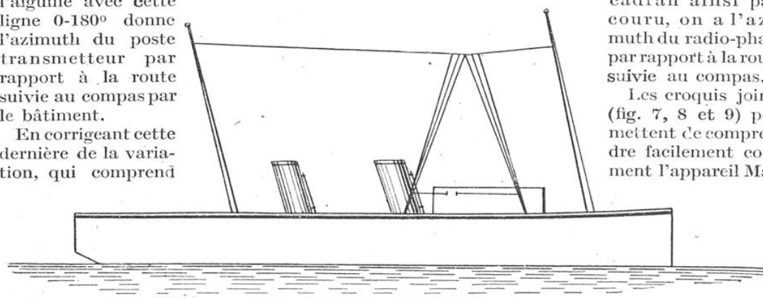
FIG. 8. — FIXATION DES ANTENNES DANS LA MATURE D'UN NAVIRE
