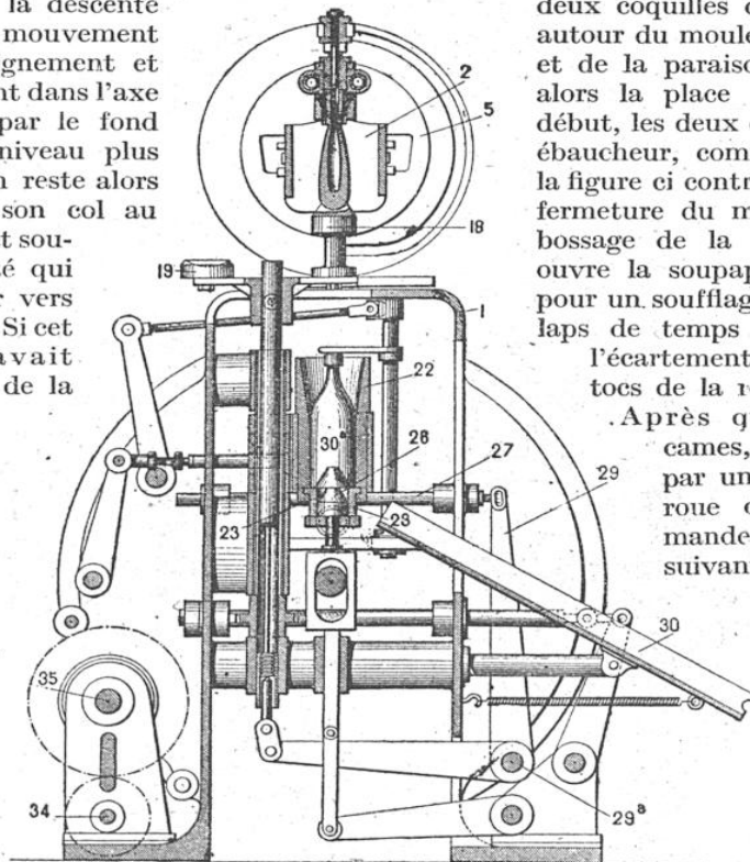
COUPE, APRÈS RENVERSEMENT, DU MOULE ÉBAUCHEUR, OU DE PARAISSON. LE GOULOT DE LA BOUTEILLE EST ALORS TOURNÉ VERS LE HAUT
