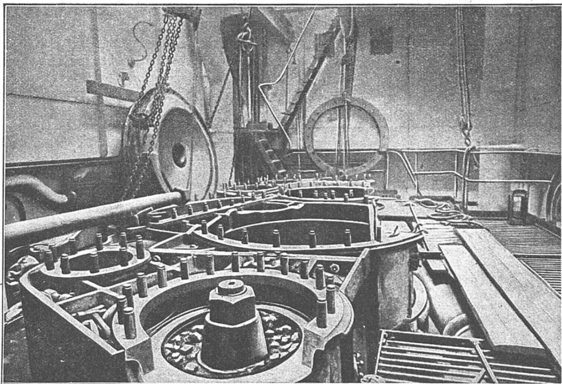
CYLINDRES DÉTÉRIORÉS DU VAPEUR « BEAPENDY », EX-« TIJUCA »
