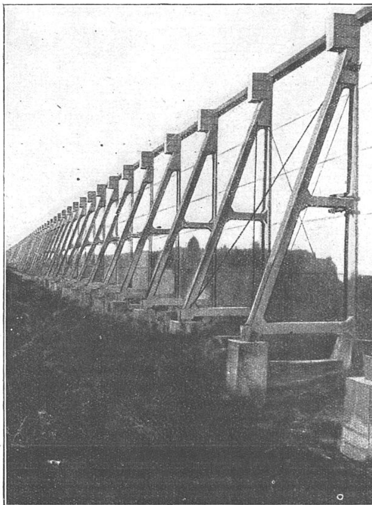
VUE LATÉRALE EXTÉRIEURE D'UN PARANEIGE DE L'UNION PACIFIC RAILROAD (ÉTATS-UNIS)
