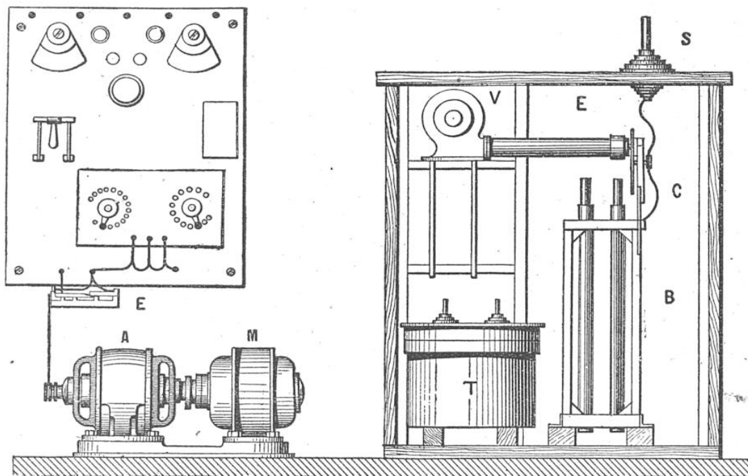
FIG. 3. — DISPOSITIFS DU RADIO-PHARE SYSTÈME BÉTHENOD
