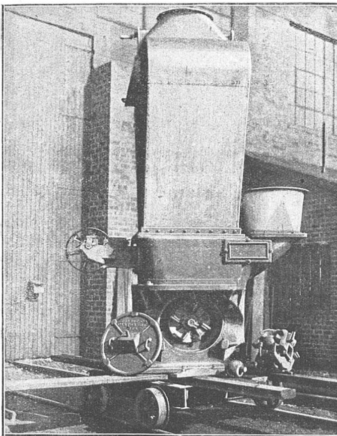
VUE INTÉRIEURE D'UN BROYEUR A GALETS
