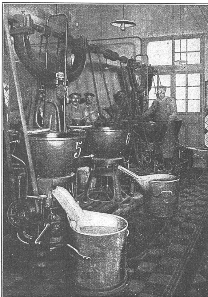
GROUPES DE MALAXEURS DE LA PÂTE AU SESQUISULFURE DE PHOSPHORE ET CHLORATE DE POTASSE
