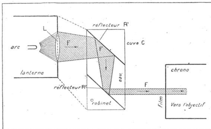
LE DISPOSITIF DE RÉFRIGÉRATION DE LA LUMIÈRE CONDENSÉE VU EN DESSUS
