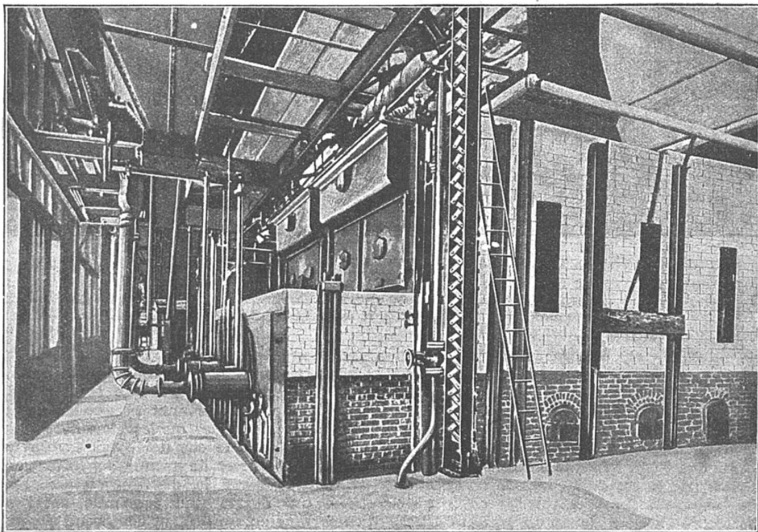
BATTERIE DE CHAUDIÈRES TUBULAIRES CHAUFFÉES A LA HOUILLE PULVÉRISÉE
