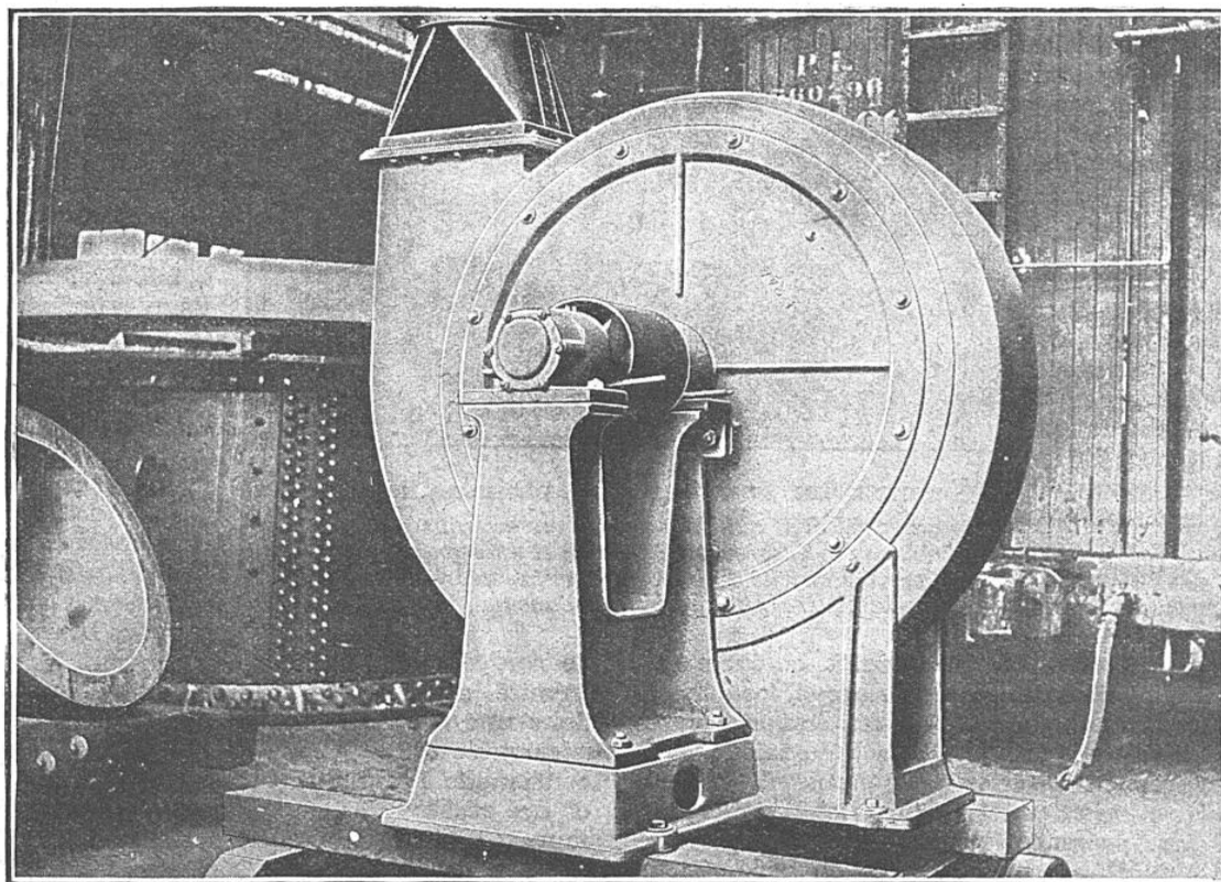
VENTILATEUR POUR LE FORÇAGE DE L'AIR DANS LES CONDUITES PNEUMATIQUES
