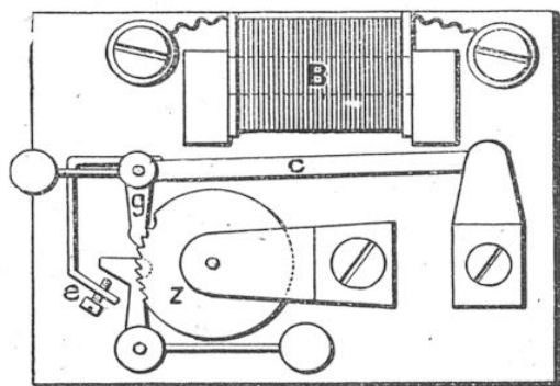
B, électro-aimant; C, armature; Z, rochet; c, vis de butée empêchant le rochet de tourner sous l'action du cliquet qui lui fait face. — Quand l'armature retombe, le cliquet supérieur g fait tourner le rochet d'une dent.
