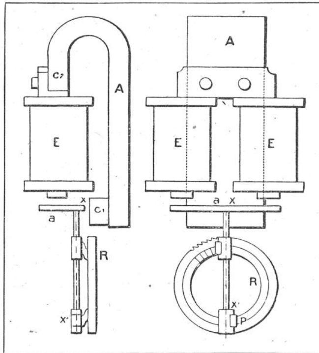
FIGURE 23. — RÉCEPTEUR HIPPI (PROFIL ET FACE) A, aimant permanent, a, armature aimantée; E, électro-aimant polarisé par l'aimant A; x, x' , axe de l'armature a; c_2 , pôle aimantant le noyau de l'électro; c_1 , pôle aimantant l'armature r, r' , rochets actionnant la roue dentée latéralement R pour lui imprimer un mouvement de rotation.
