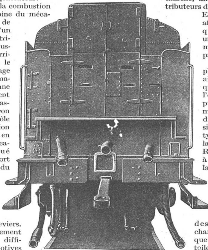
VUE ANTÉRIEURE D'UN TENDER MONTRANT LA TUYAUTERIE FLEXIBLE POUR L'ARRIVÉE DU COMBUSTIBLE EN POUDRE A LA MACHINE
