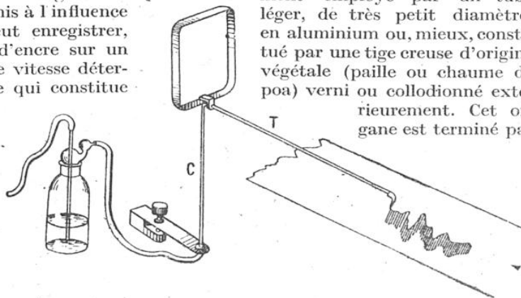
INSCRIPTION DES OSCILLATIONS D'UN CADRE GALVANIQUE
