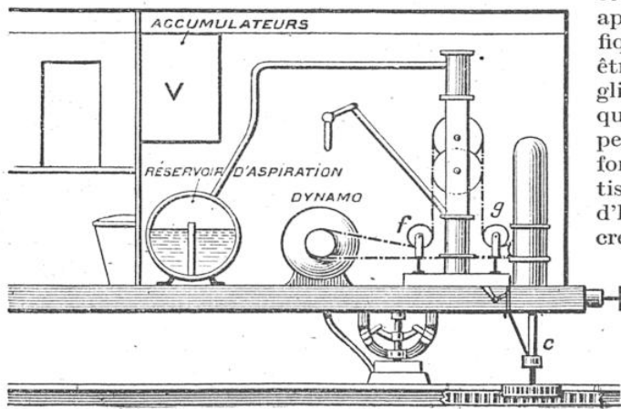
CHEMIN DE FER GLISSANT A TRACTION ÉLECTRIQUE ET A CRÉMAILLÈRE (COUPE LONGITUDINALE)
