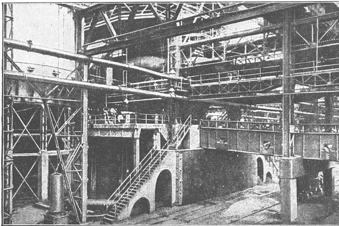
PLATE-FORME DE COULÉE DES HAUTS FOURNEAUX D'HAGONDANGE
