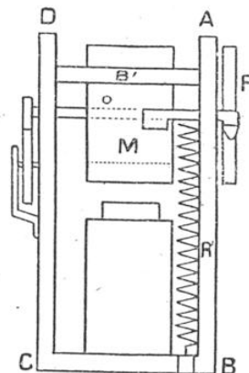
A B C D, châssis en fer magnétique; M, armature de l'électro-aimant; R, rochet calé sur l'axe de l'armature; R', ressort de rappel de l'armature.
