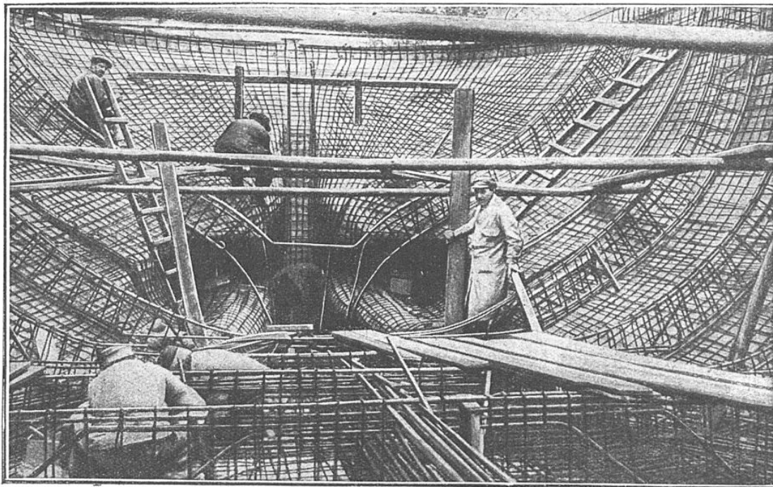
FERRAILLAGE DE LA COQUE D'UN CARGO-BOAT EN CIMENT ARMÉ
