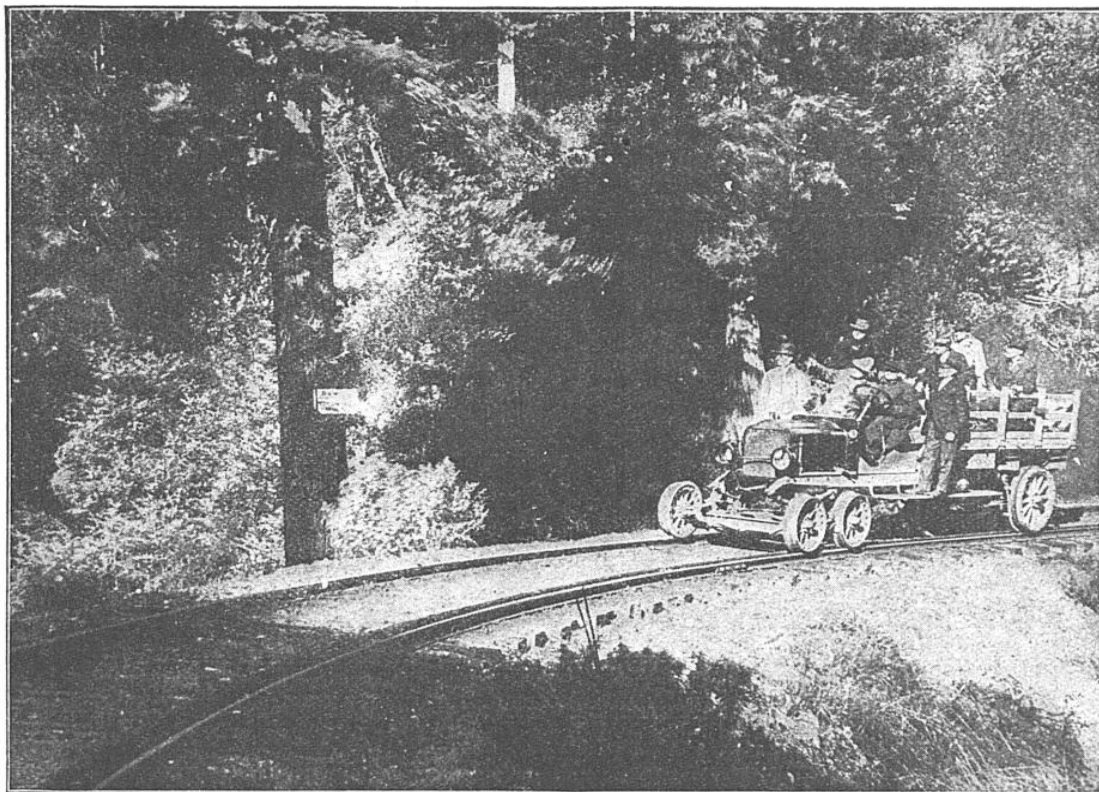
LE CAMION AUTOMOBILE SUR RAILS DU MONT TALMAPAIS (CALIFORNIE)
