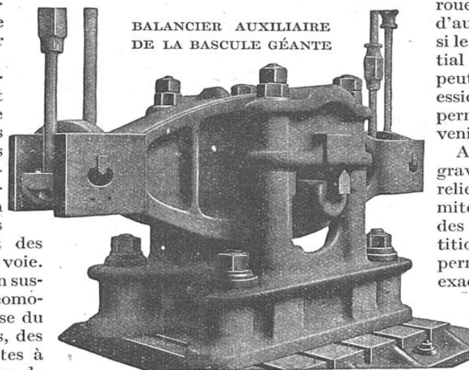
Comme le montre cette photographie, le couteau a son tranchant orienté vers le haut, à l'inverse de celui des grands balanciers principaux, dont les couteaux ont leurs arêtes dirigées vers le bas.
