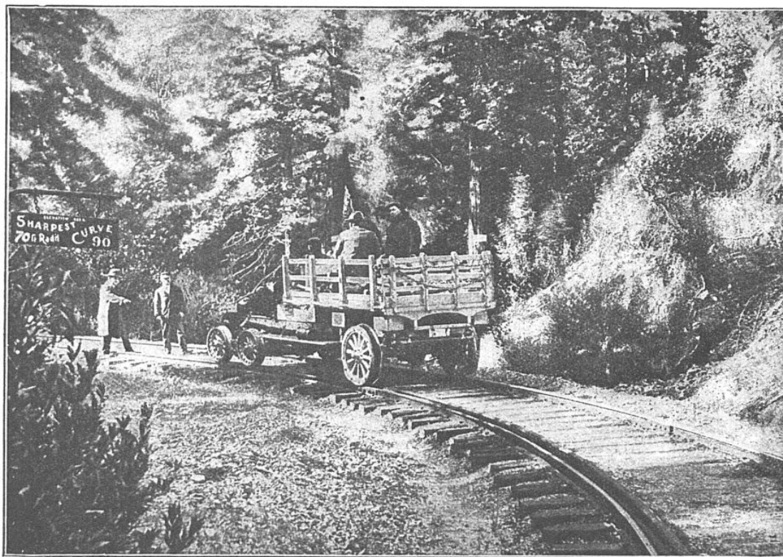
UN TOURNANT A 90°, DE 23 MÈTRES DE RAYON, SUR UNE RAMPE A 7 0/0
