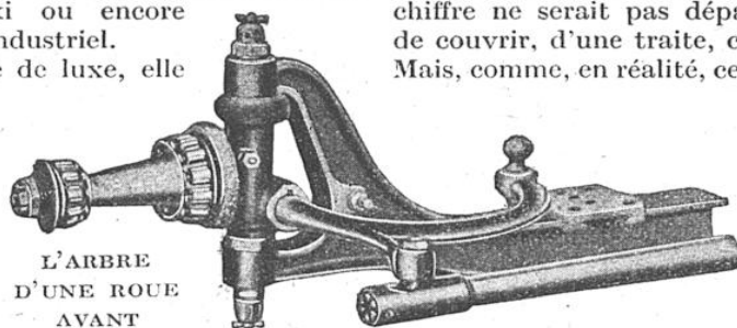
La direction d'une voiture électrique est commandée par un dispositif analogue à celui des automobiles à essence.
