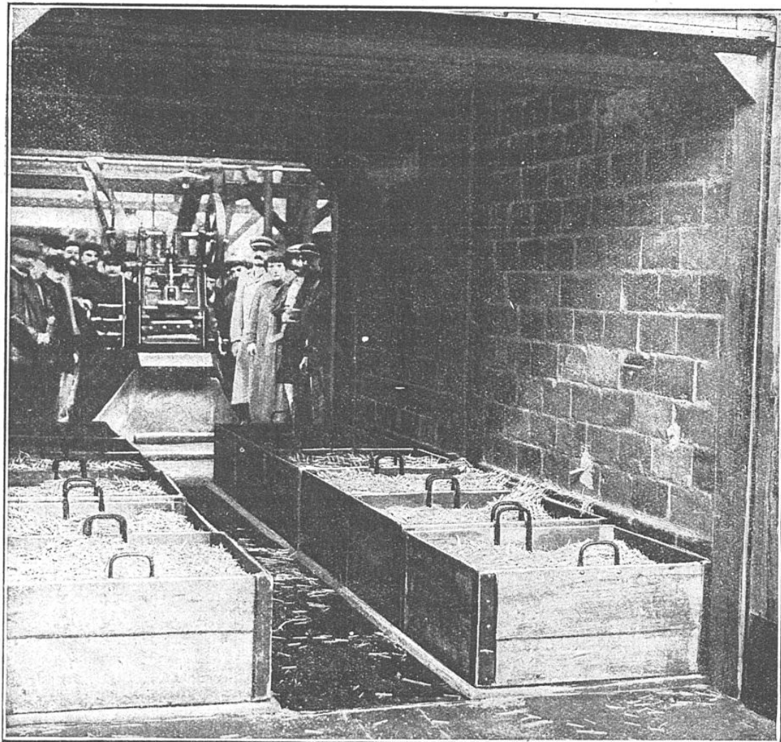
LES TIGES SONT DESSÉCHÉES PENDANT UNE HEURE DANS DES SÉCHOIRS A VAPEUR
