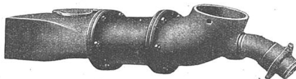
MÉLANGEUR D'AIR ET DE POUDRE DE CHARBON PULVÉRISÉ POUR LOCOMOTIVE
