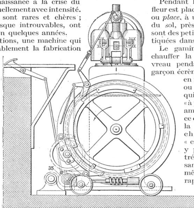
LA MACHINE WILZIN EN ÉLÉVATION LATÉRALE
