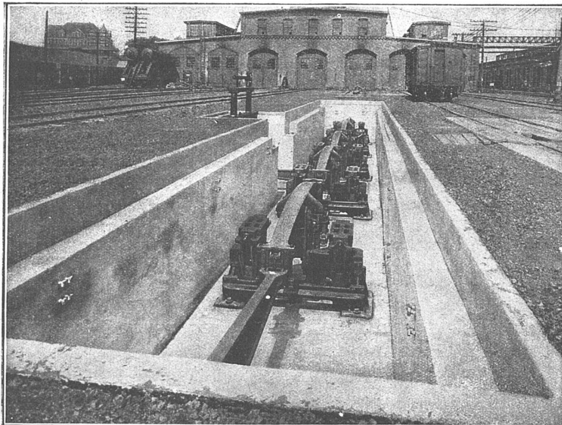
LA FOSSE EN CIMENT QUI ABRITE LE MÉCANISME DE LA BASCULE
