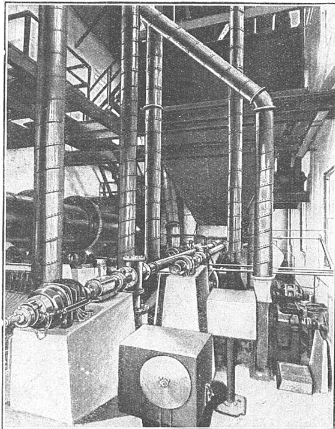
ATELIER DE PULVÉRISATION POUR COMBUSTIBLES
