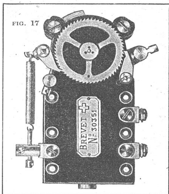
VUE GÉNÉRALE DE LA RÉCEPTRICE DU SYSTÈME DAVID PERRET
