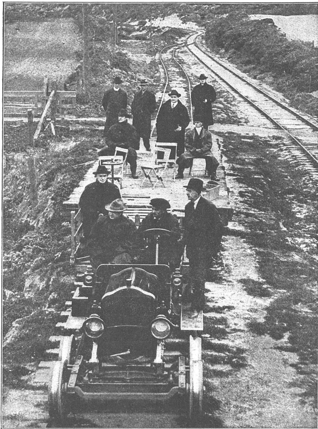
CAMION AUTOMOBILE MUNI DE ROUES SPÉCIALES CIRCULANT SUR UNE VOIE FERRÉE On voit ici le véhicule, actionné par un moteur à essence, remorquant un truck aménagé en plate-forme roulante. Le premier véhicule pèse deux tonnes seulement et le second plus de neuf.
