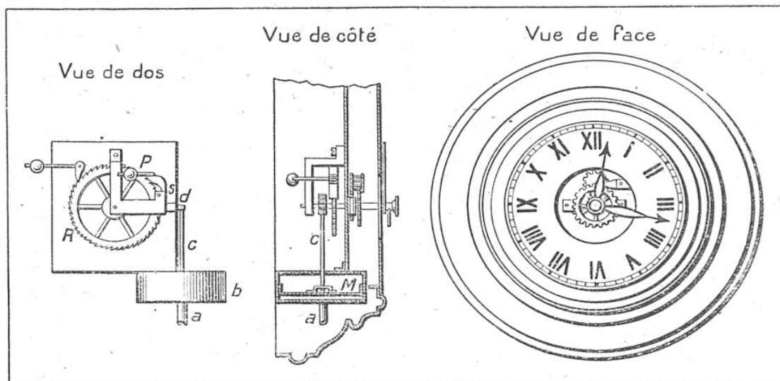
FIGURES 4, 5 ET 6. — MÉCANISME INTÉRIEUR D'UNE HORLOGE RÉCEPTRICE
