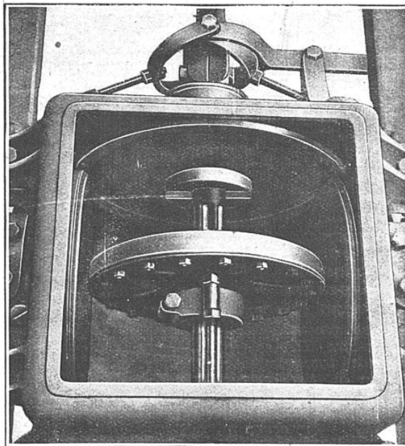
LA TRANSMISSION PAR PLATEAUX MONTÉE SUR UN CHASSIS D'AUTOMOBILE
