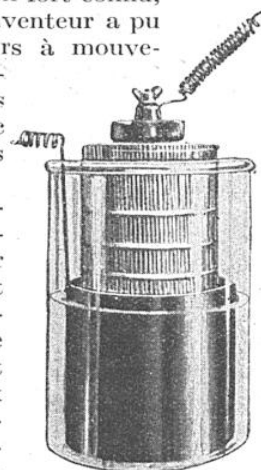
FIG. 36. — PILE WARNON DE 120 A.H. CONVENANT POUR L'HORLOGERIE ÉLECTRIQUE
