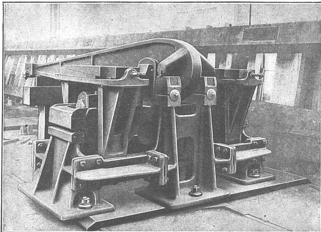
VUE D'UN LEVIER ISOLÉ D'UNE BASCULE A LOCOMOTIVES
