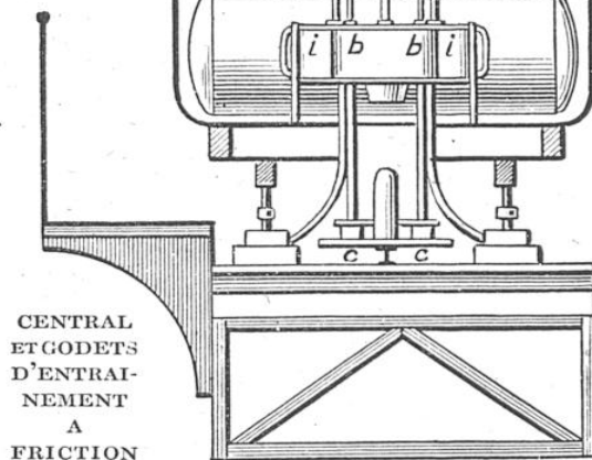
MACHINE DU CHEMIN DE FER GLISSANT A TRACTION ÉLEC- TRIQUE PAR RAIL
