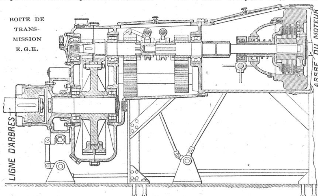
Cet organe mécanique est intercalé entre le moteur et la ligne d'arbres sur laquelle est fixée l'hélice. Elle contient l'embrayage, le renversement de marche, et le démultiplicateur qui réduit à 200 tours la vitesse de rotation de l'hélice, permettant ainsi l'emploi d'un moteur à essence tournant à 1.200 tours.
