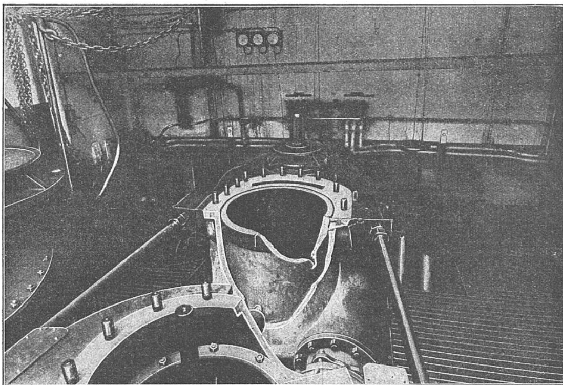
BOÎTE À TIROIR CYLINDRIQUE BRISÉE SUR LE VAPEUR « ARACAJU », EX-« PERSIA »
