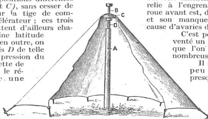
TENTE MUNIE DE SON SYSTÈME TENDEUR
