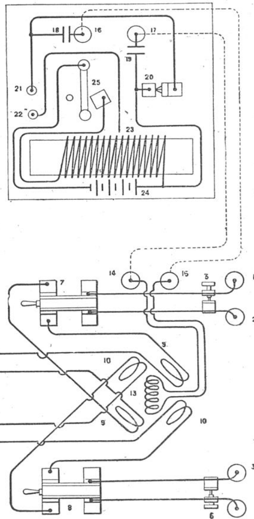
FIG. 10. — DISPOSITIONS INTÉRIEURES ET CONNEXIONS PAR FILS ISOLÉS DE L'APPAREIL RÉCEPTEUR MARCONI-BELLINI-TOSI
