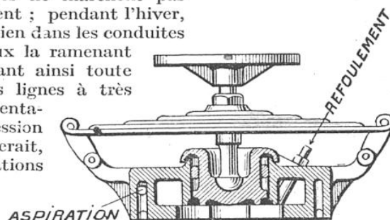
AUTRE MODE D'ATTACHE DE LA CAISSE DE LA VOITURE AU PATIN
