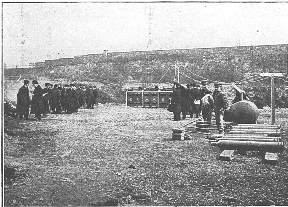
VUE D'ENSEMBLE D'UNE INSTALLATION EXPÉRIMENTALE POUR L'EXTINCTION DES FEUX D'HUILE PAR LE PROCÉDÉ R. FRÈRE
