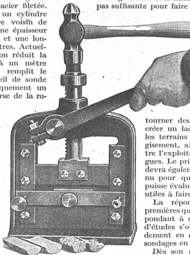
CISAILLE SERVANT A SECTIONNER LES FRAGMENTS DE « CAROTTES »
