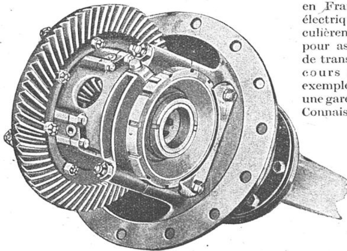
VUE D'UNE PARTIE DU MÉCANISME DU DIFFÉRENTIEL.
