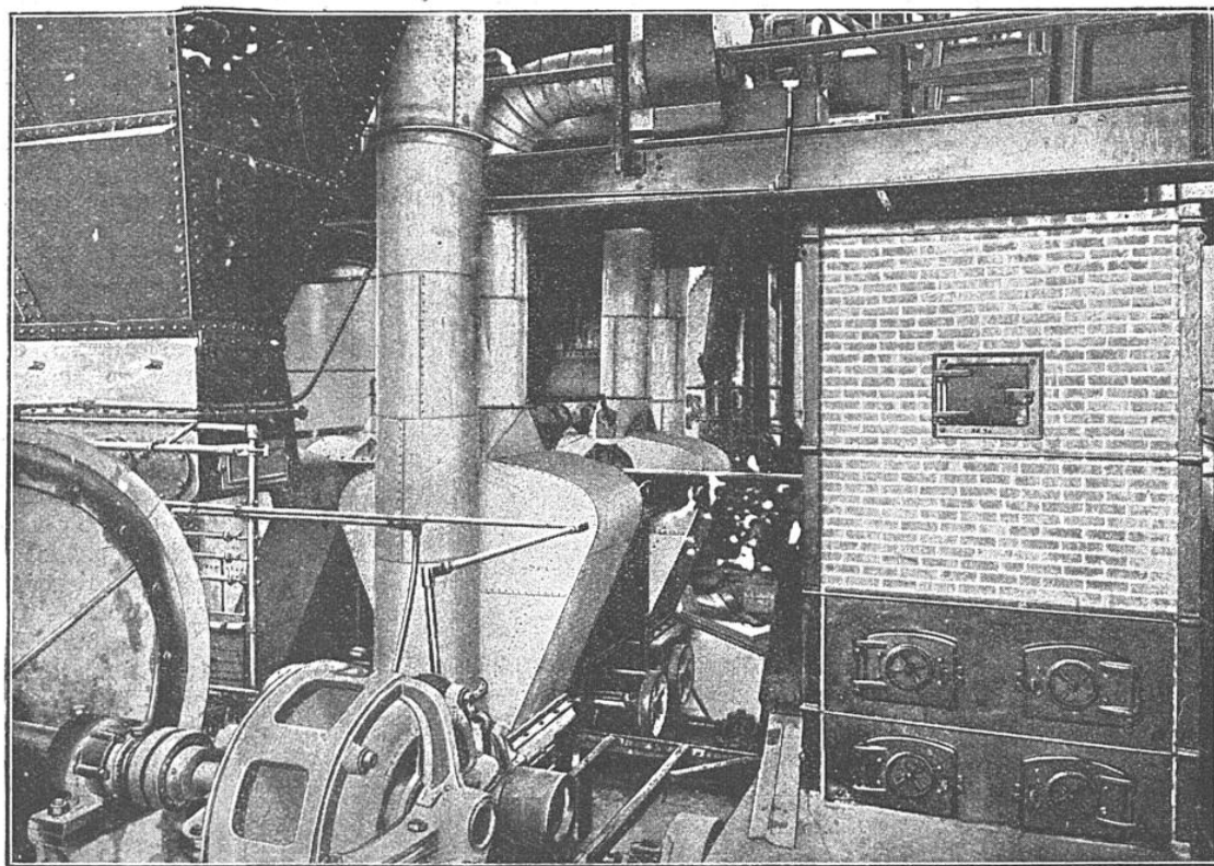
VUE PRISE DANS L'ATELIER DE BROYAGE DE CHARBONS DES ACIÉRIES ARMSTRONG WHITWORTH, A MONTRÉAL (CANADA)
