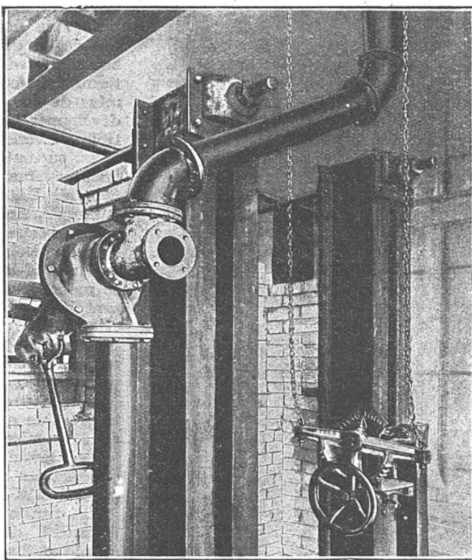
BRÛLEUR POUR L'EMPLOI DE CHARBON PULVÉRISÉ DANS UN FOUR SIDÉRURGIQUE
