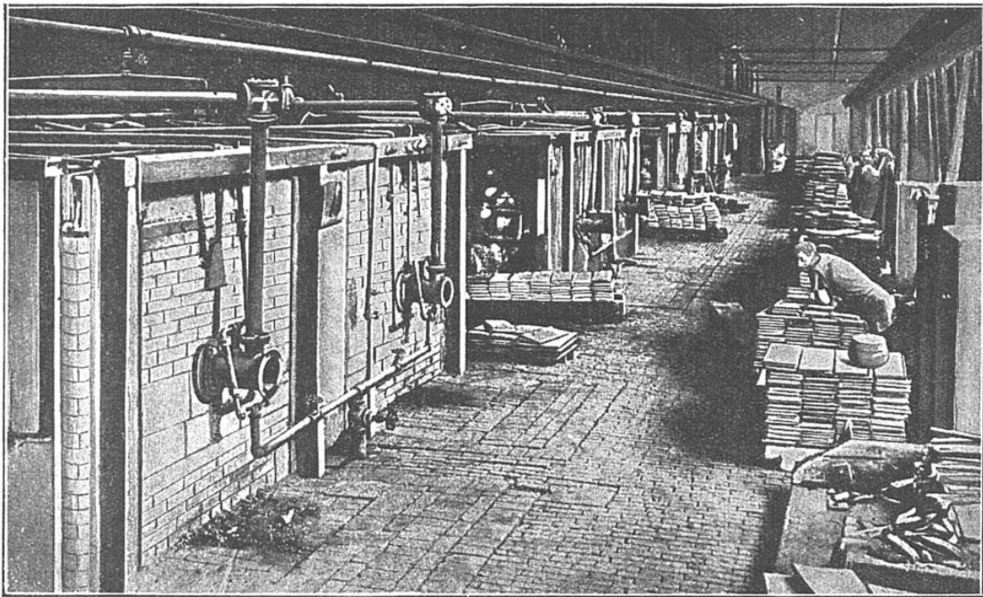
FOURS CHAUFFÉS AU CHARBON PULVÉRISÉ DANS UNE FABRIQUE DE FER-BLANC
