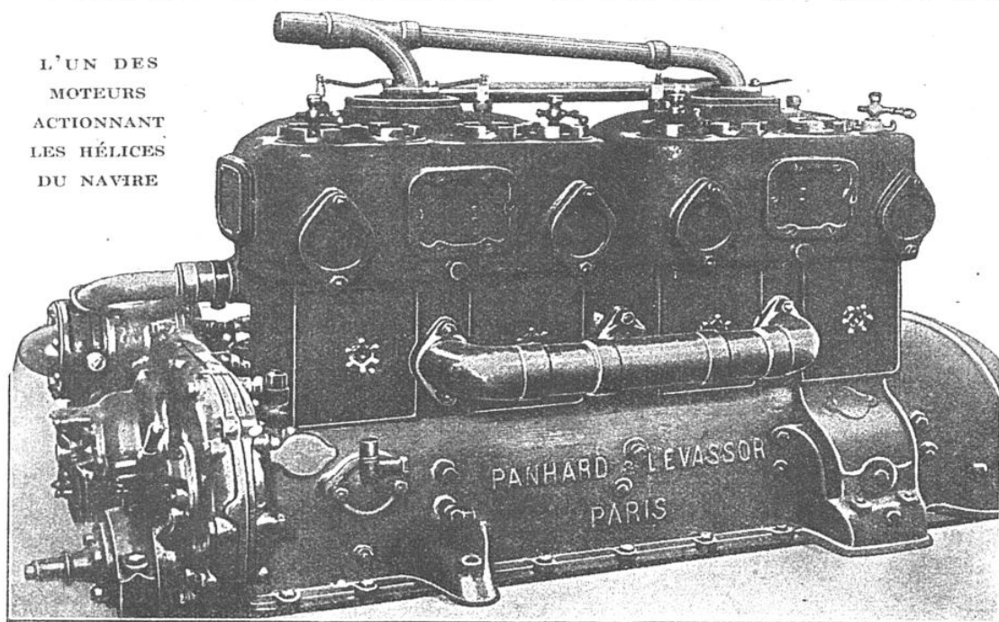
Le bateau est muni de deux moteurs semblables du type automobile à essence. Chaque moteur développe une puissance de 120 HP à 1.200 tours. Il est muni d'un régulateur qui l'empêche de dépasser ce régime.
