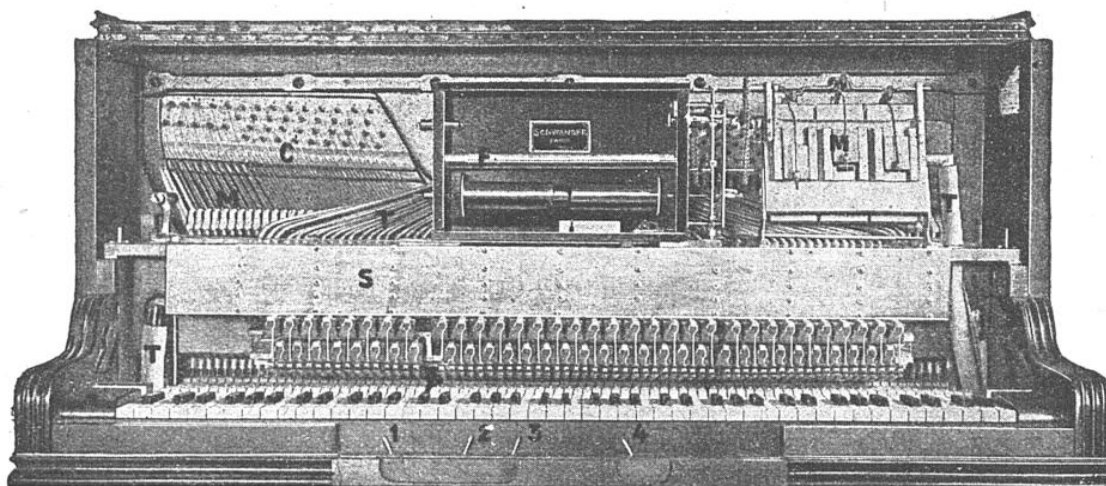
PARTIE SUPÉRIEURE D'UN PIANO AUTOMATIQUE DU SYSTÈME COURANT
