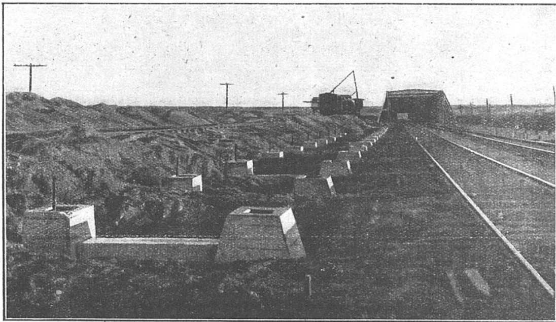
INFRASTRUCTURE D'UN ABRI CONTRE LES NEIGES, AUX ÉTATS-UNIS
