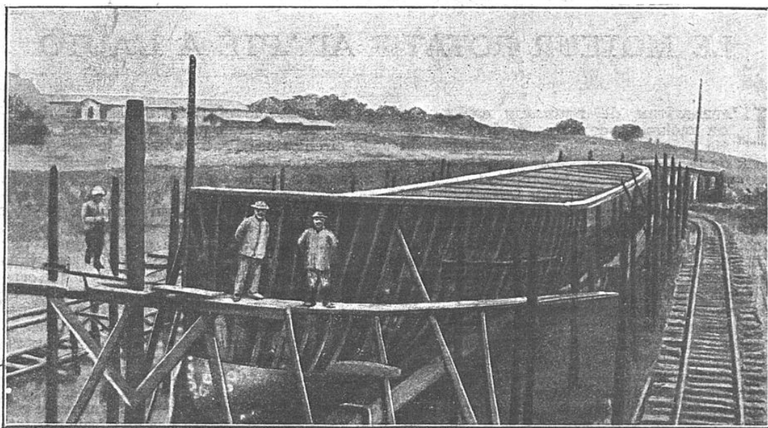
UN CHANTIER DE CONSTRUCTIONS NAVALES A KIGOMA, SUR LE LAC TANGANYIKA
