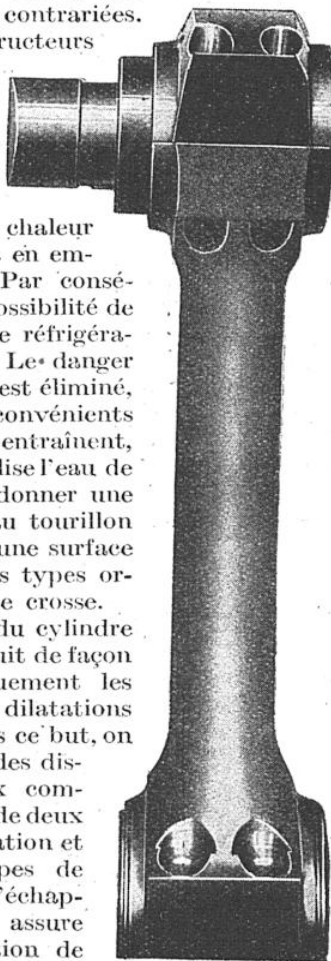
BIELLE D'UN MOTEUR DIESEL DE 1.500 CHEVAUX 4 temps, 8 cylindres.
