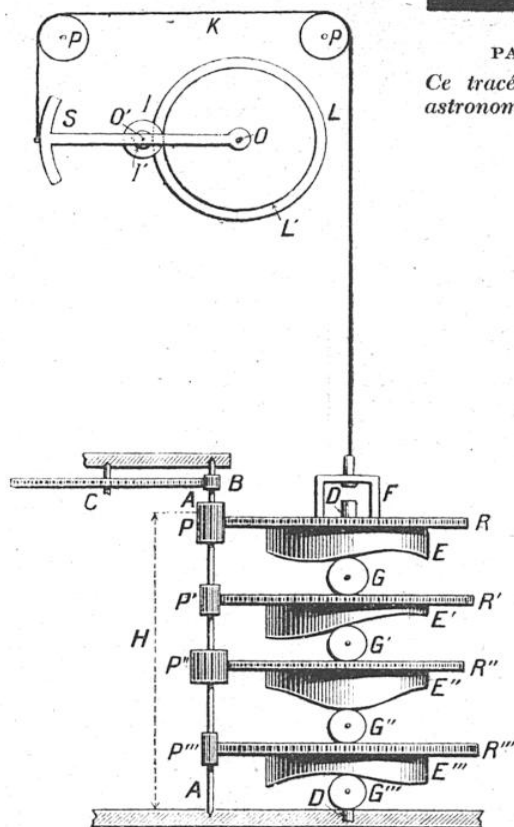
SCHEMA DU MÉCANISME INTÉGRATEUR INVENTÉ PAR SCHWILGUÉ POUR LA CORRECTION DES MOUVEMENTS DU SOLEIL ET DE LA LUNE
