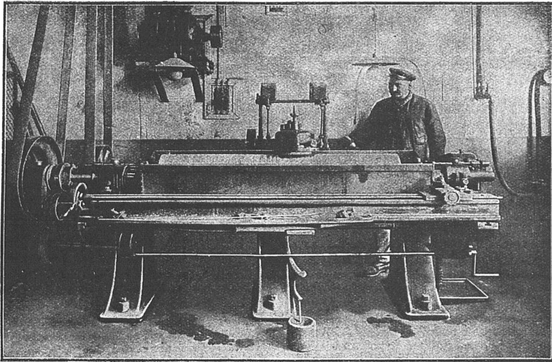
TOUR A RECTIFIER ET A POLIR LES CYLINDRES DE ROTOGRAVURE
