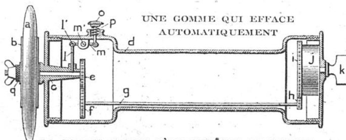
LA GOMME REÇOIT D'UN RESSORT UN MOUVEMENT DE ROTATION EXTRÊMEMENT RAPIDE
