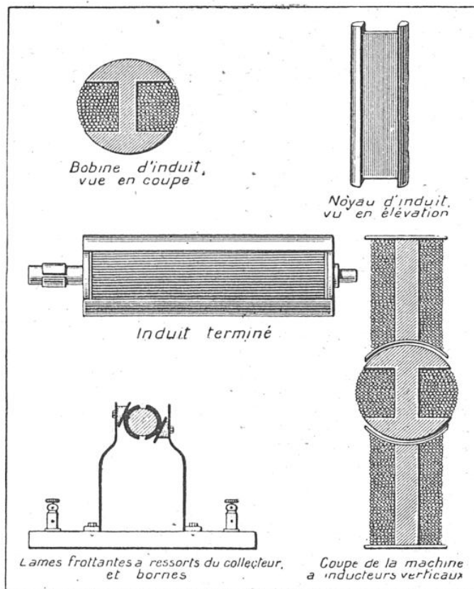
PETITE DYNAMO, GENRE SIEMENS POU- VANT ÊTRE CONSTRUITE PAR UN AMATEUR Planche montrant les différentes pièces de la machine avant leur montage.
