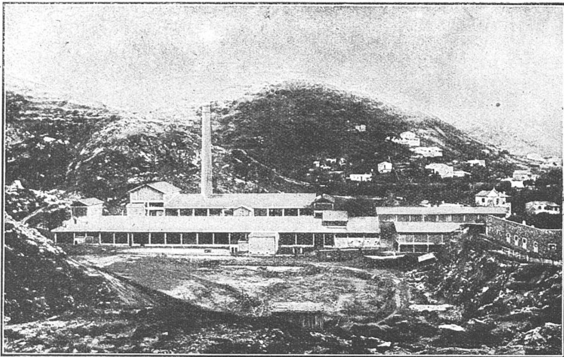
USINE A CIMENT ARTIFICIEL A FOURS ROTATIFS. AVEC EXPLOITATION EN CARRIÈRE Les frais de transport et de manutention de la matière première sont ainsi réduits au minimum.
