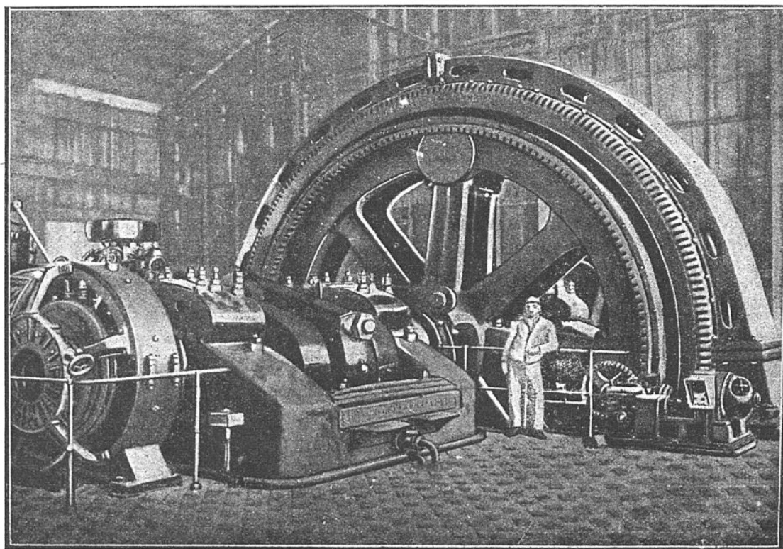
GÉNÉRATEUR ÉLECTRIQUE A COURANTS TRIPHASÉS DE 4.300 KILOWATTS, 3.500 VOLTS, 50 PÉRIODES, TOURNANT A RAISON DE 94 TÔURS PAR MINUTE
