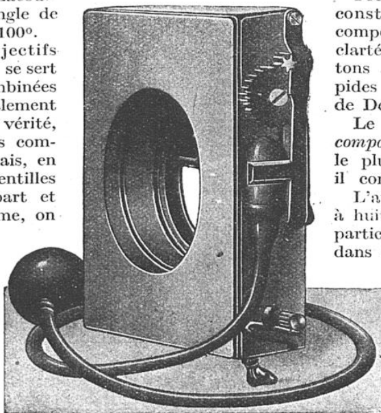
OBTURATEUR A RIDEAU TH. PICKARD
