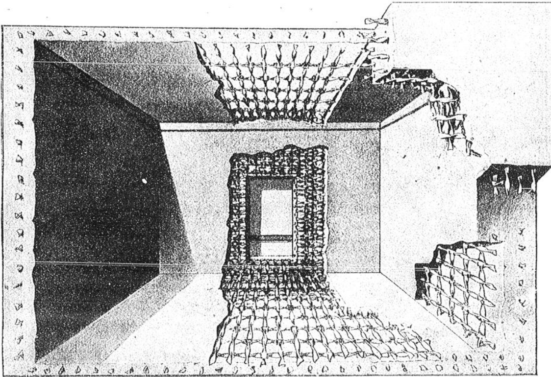
DESSIN MONTRANT LA CONSTRUCTION DE L'ENVELOPPE D'UNE CHAMBRE-FORTE
