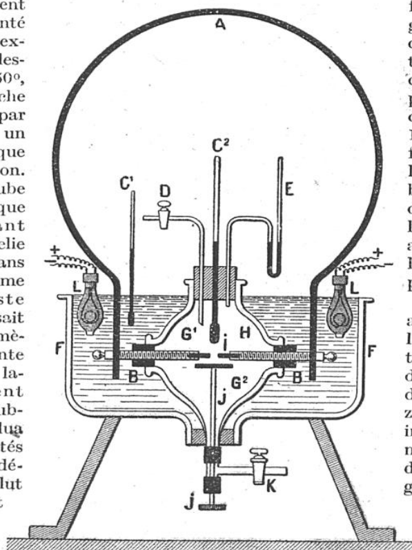
FIG. 2. — SCHÉMA DU RÉSONATEUR-INFLAMMATEUR A, cercle métallique; B B, tubulures latérales; C 1 C 2 , thermomètres; D, robinet de l'aspirateur; E, manomètre; F, cloche à douille; G 1 H G 2 , ballon en verre; I, électrode; J J, tige du plateau supportant les matières inflammables; K, robinet du tube abducteur; L L, lampes électriques servant au chauffage du bain d'huile de vaseline.
