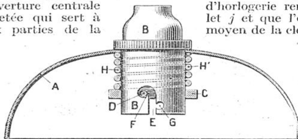
Le réflecteur A est assujéti à la douille B au moyen d'une bague C possédant deux tenons D qui, pénétrant par l'échancrure E de la douille, se logent dans les évidements F. Les évidements G sont utilisés pour fixer la lampe. Un ressort H assure la tenue de la bague C.
