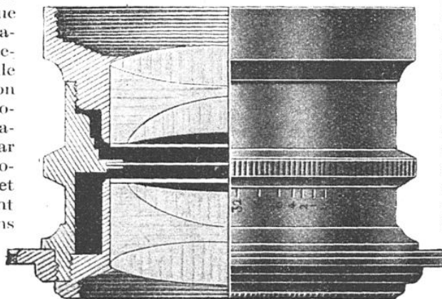
DEMI-COUPPE D'UN APLANASTIGMAT HERMAGIS
