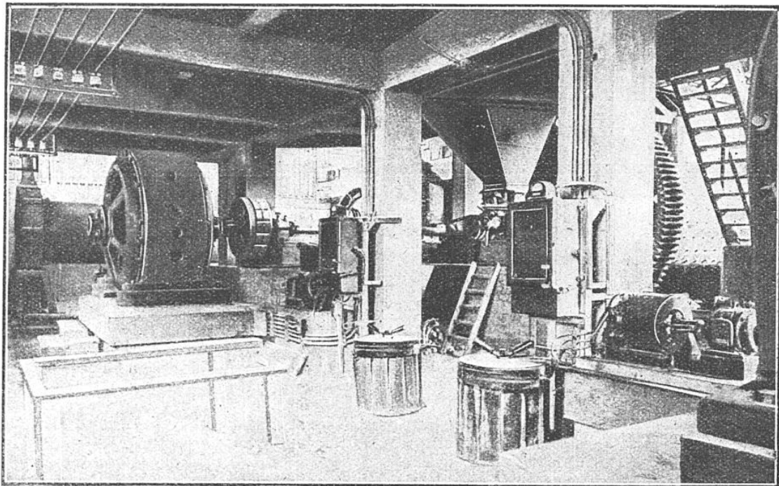
LES BROYEURS DE CET ATELIER SONT ACTIONNÉS ÉLECTRIQUEMENT
