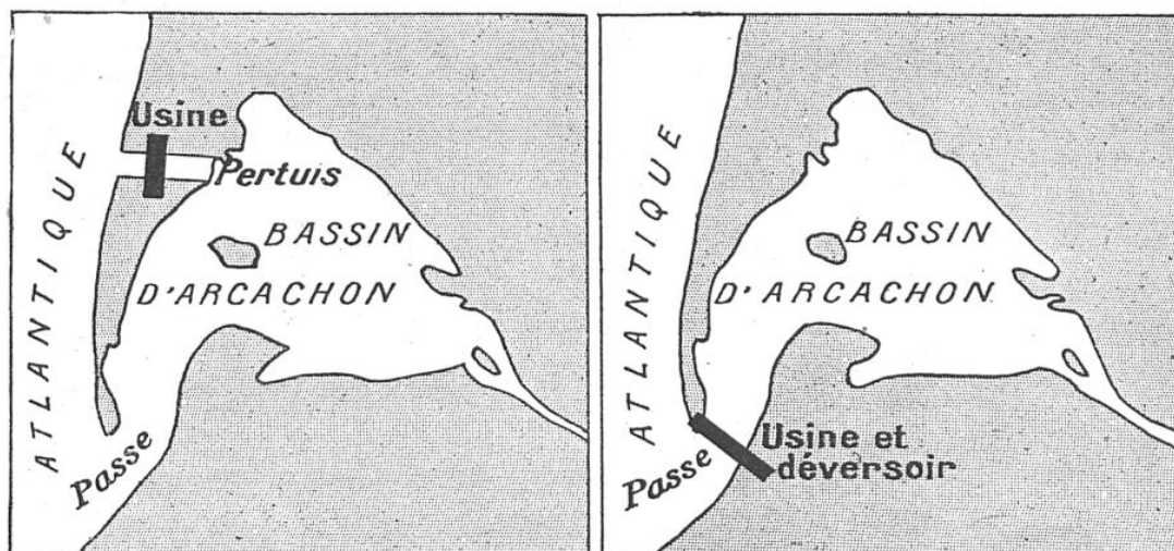
FIG. 7 ET 8. — PROJETS POUR L'AMÉNAGEMENT DU BASSIN D'ARCACHON
