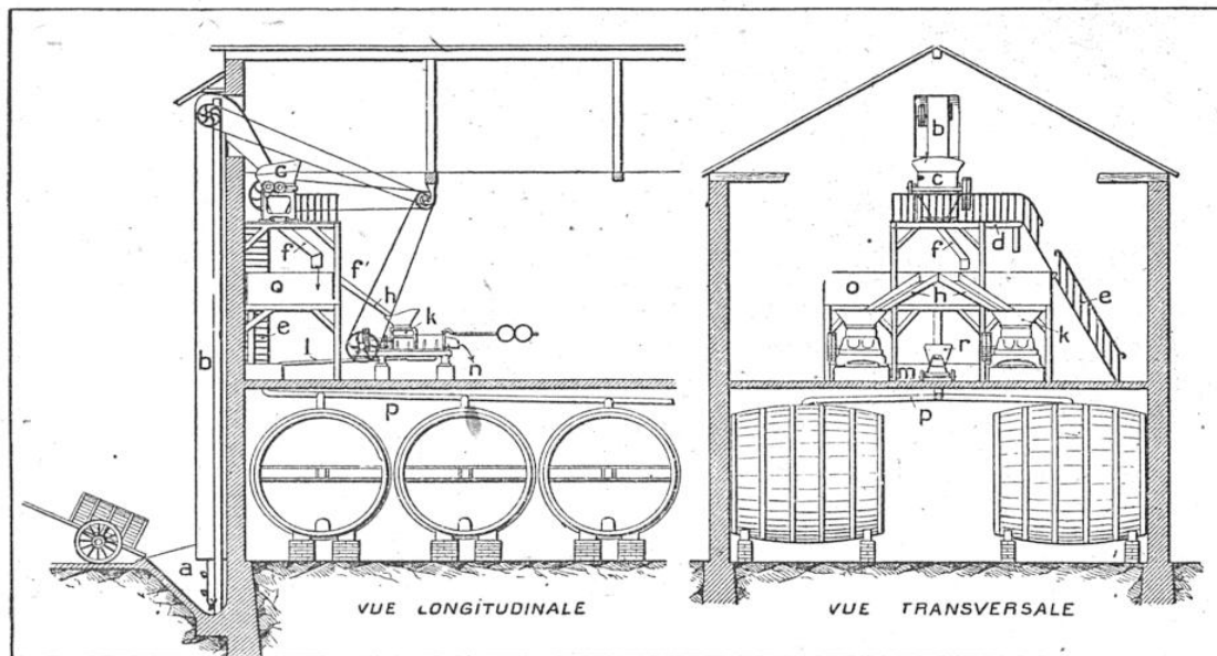
SCHEMA DE L'INSTALLATION D'UN CELLIER A PRESSEUR CONTINU
