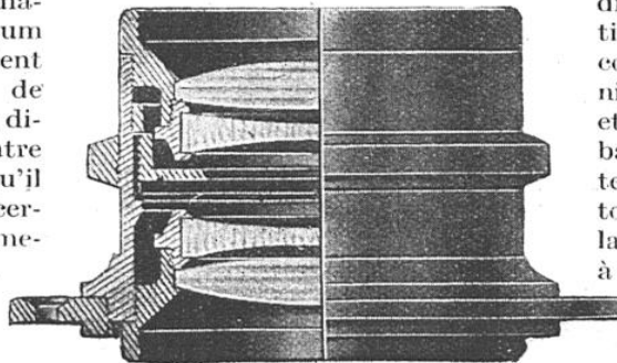
OBJECTIF DOUBLE ANASTIGMAT (F : 6.8)
