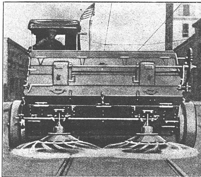
DEUX COURONNES ROTATIVES PERMETTENT À CETTE BALAYEUSE DE RÉPANDRE DU SABLE SUR LA CHAUSSEE
