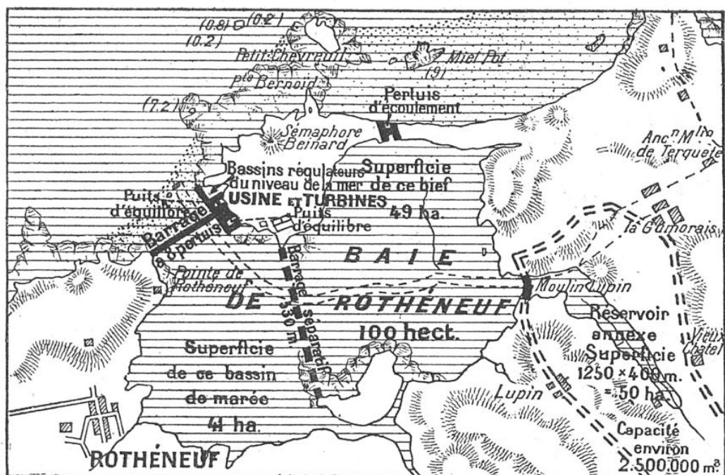
FIG. 11. — PROJET D'AMÉNAGEMENT DE LA BAIE DE ROTHÉNEUF (ILLE-ET-VILAINE) Il s'agirait d'établir un bassin de marée unique au moyen d'un barrage au travers du goulet d'entrée. On pourrait obtenir ainsi une puissance moyenne de 16.000 chevaux.
