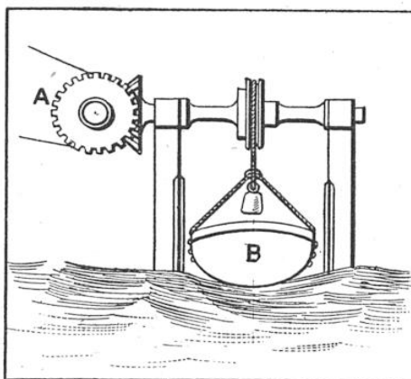
FIG. 2. — AUTRE DISPOSITIF CONSTITUANT UN MARÉMOTEUR
