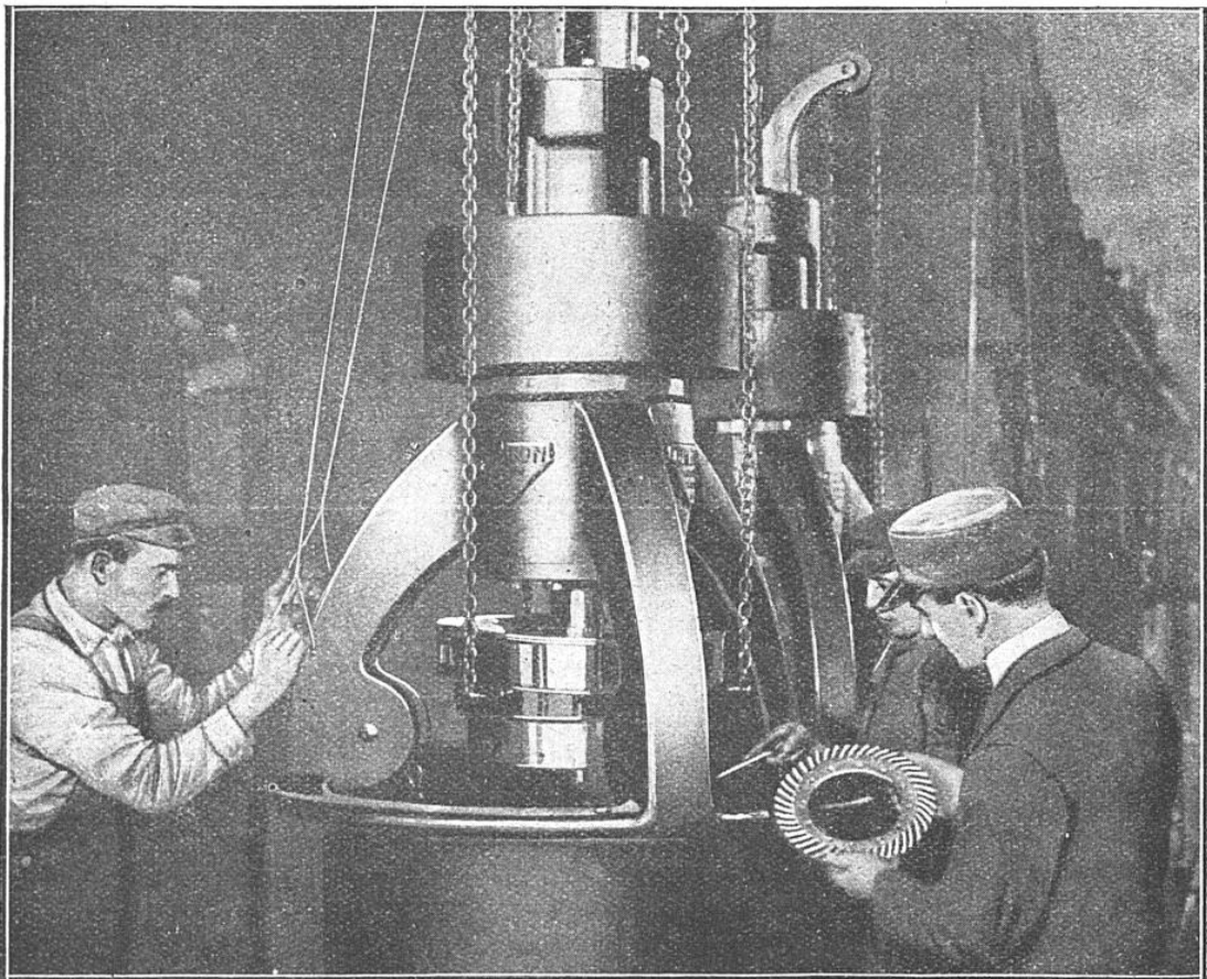
PRESSE EMPLOYÉE POUR EMPÊCHER LES ENGRENAGES DE SE DÉFORMER APRÈS TREMPÉ Pour empêcher les engrenages de se déformer en se contractant, quand on les refroidit brusquement dans un bain d'huile après les avoir portés au rouge, on a coutume maintenant, dans certains établissements métallurgiques, de les introduire dans des presses qui les maintiennent solidement durant l'opération de la trempé.
