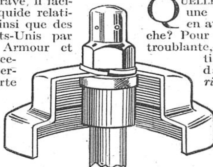
SOUPAPE AUTOMATIQUE POUR BOUCHON DE RÉSERVOIR D'ESSENCE
