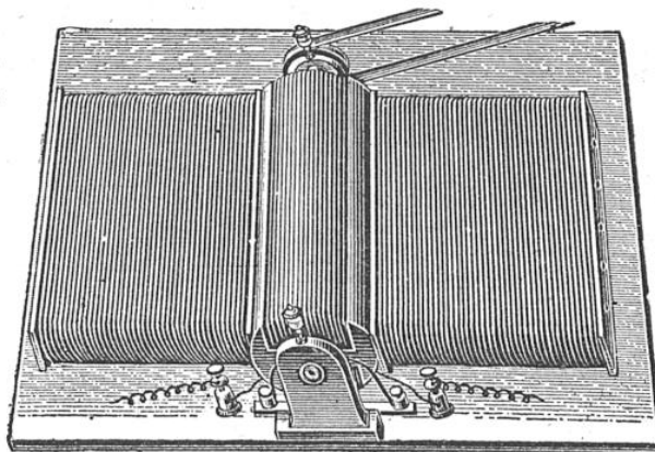
VUE PERSPECTIVE DE LA MACHINE À INDUC- TEURS HORIZONTAUX TERMINÉE
