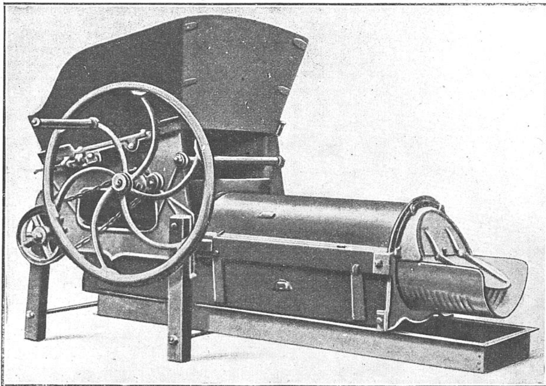
FOULOIR-ÉGOUTTOIR A VITESSES DIFFÉRENTIELLES, SYSTÈME MARMONNIER
