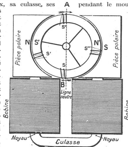
SCHEMA DE LA MACHINE GRAMME
