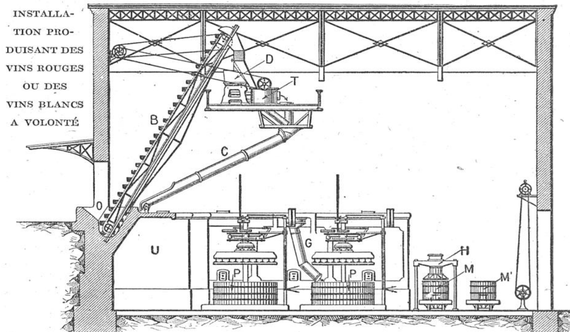
O, Fosse en ciment recevant la vendange amenée par les charrettes ; B, élévateur ; D, fouloir-égouttoir pour les vins blancs ; T, turbine pour les vins rouges ; C, coulote tournante allant aux cuves de fermentation U ou à la coulote G qui dessert les pressoirs P ; H et M, presses hydrauliques à maies roulantes M' pour assécher à fond les marcs.
