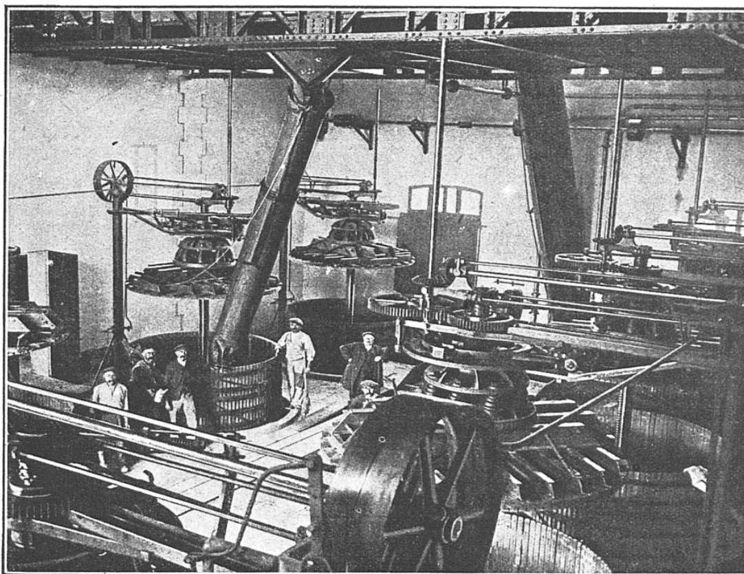
INSTALLATION MÉCANIQUE D'UN CELLIER DANS LE DÉPARTEMENT DE L'HÉRAULT
