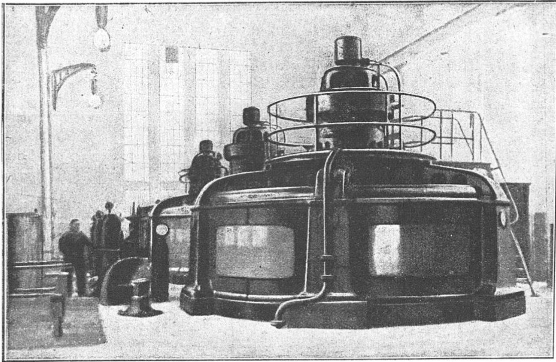
PHOTOGRAPHIE D'UN GROUPE DE TROIS ALTERNATEURS TRIPHASÉS A AXE VERTICAL
