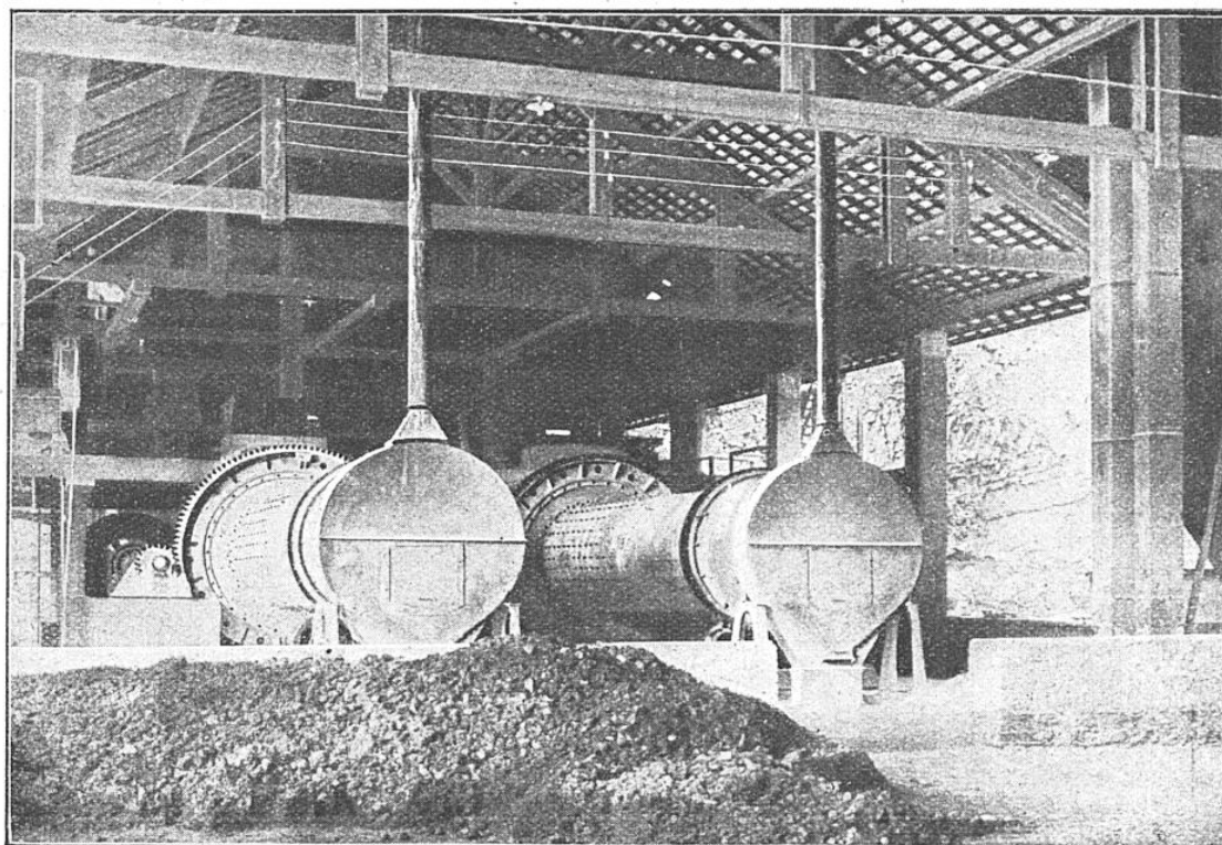
ATELIER DE BROYAGE DES MATIÈRES PREMIÈRES AVANT CUISSON
