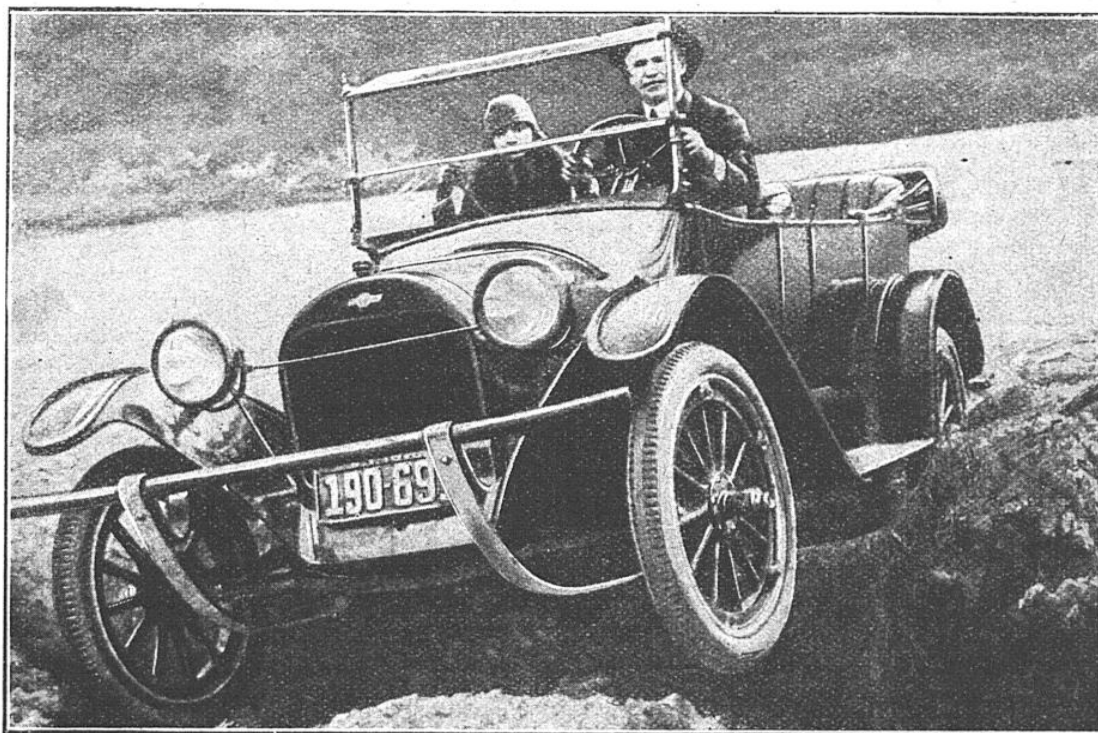
MUNIE DE DEUX PATINS LATÉRAUX, CETTE AUTOMOBILE SE RIT DES FOSSÉS ET FONDRIÈRES
