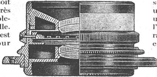
OBJECTIF GRAND ANGLE
