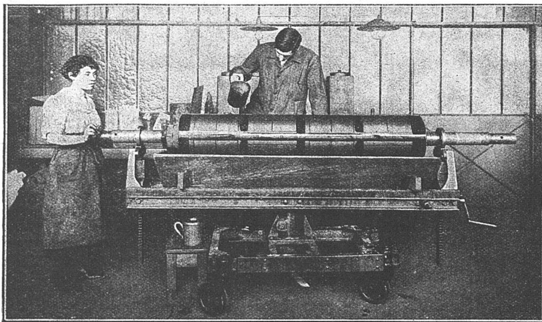
LA MORSURE AU PERCHLORURE DE FER DES CYLINDRES DE ROTOGRAVURE
