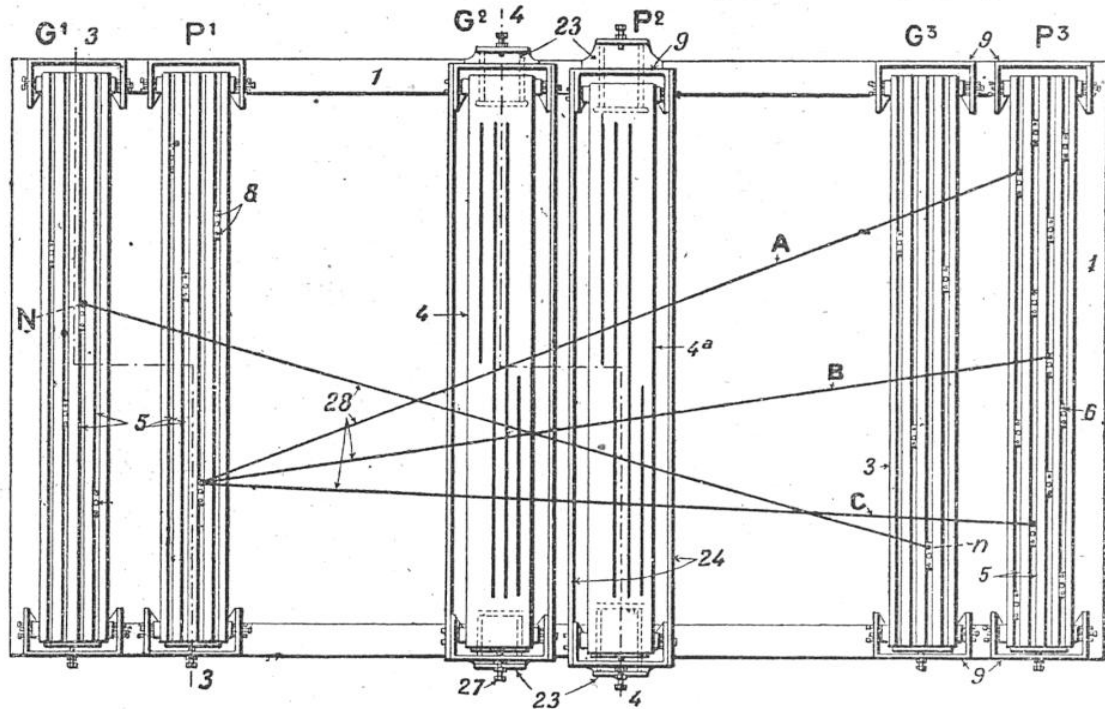
SCHEMA DE LA REGLE A CALCUL DE M. HENRY OLLER POUR L'OBTENTION RAPIDE DES CHIFFRES DE RÉPARTITION DES GAINS DU PARI MUTUEL
