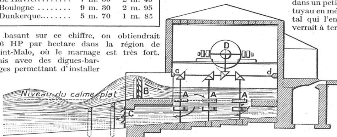
FIG. 3. — PROJET MAUREL POUR UTILISER LA FORCE VIVE DES VAGUES
