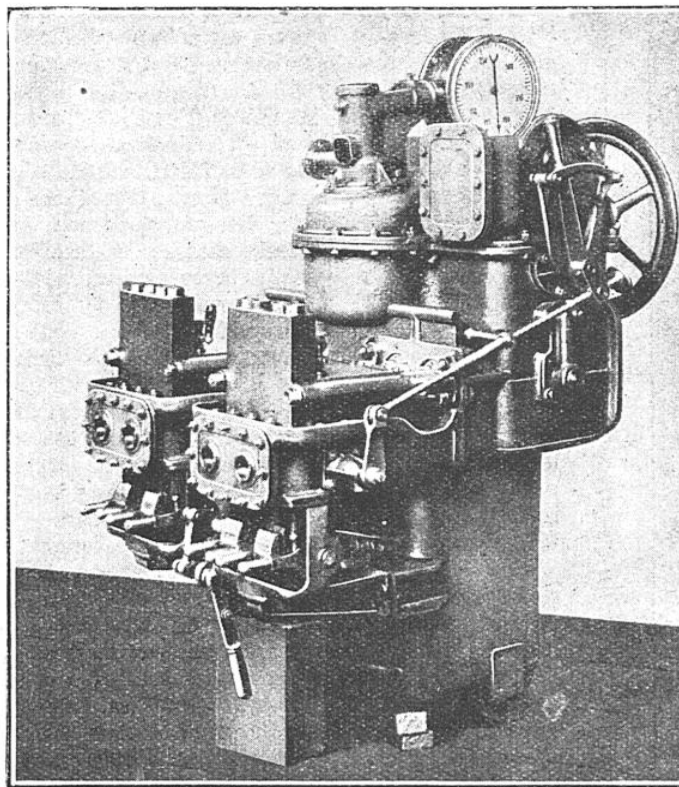
POMPE A COMBUSTIBLE D'UN MOTEUR DIESEL
