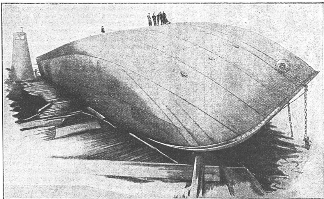
LA MOITIÉ AVANT DU « CHARLES-E. VAN HISE » FLOTTANT SUR LE FLANC, A PORT-COLBORNE (LAC ÉRIÉ) OU ELLE DEMEURA EN HIVERNAGE JUSQU'À LA REPRISE DE LA NAVIGATION
