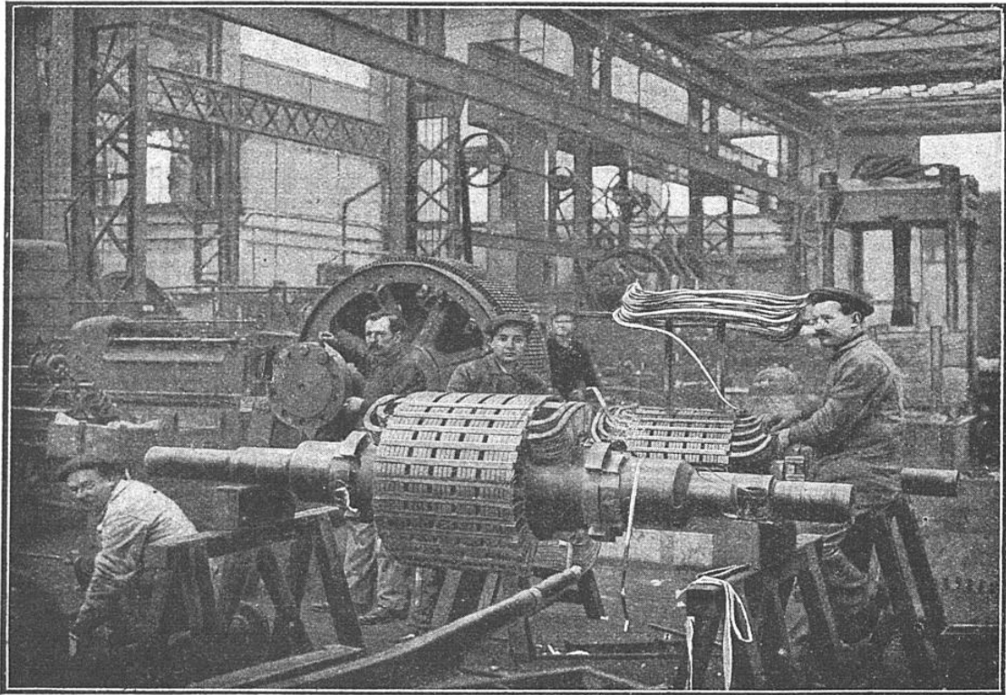
OUVRIERS PROCÉDANT AU BOBINAGE A LA MAIN D'UN ROTOR D'ALTERNATEUR
