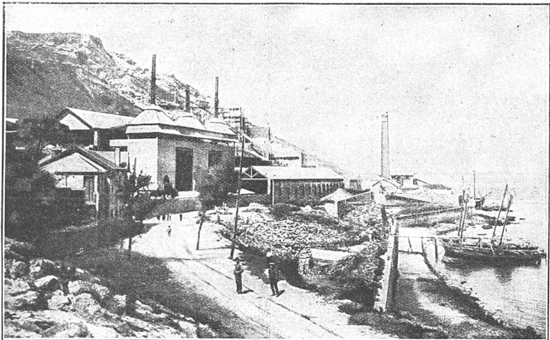
LA FABRICATION DU CIMENT ARTIFICIEL PAR VOIE SÈCHE AU BORD DE LA MER Cette installation moderne et très pratique, établie par une maison française, existe au Portugal.
