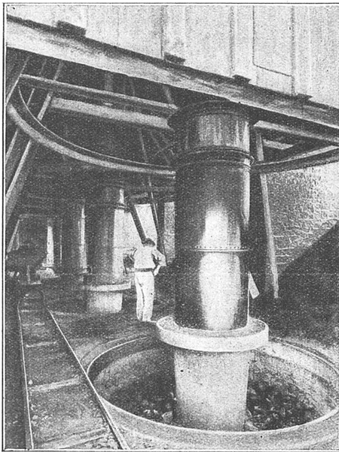
USINE A CEMENTS NATURELS DE VOREPPE (ISÈRE) Vue de la plate-forme de chargement des fours fixes verticaux. Une voie de service permet d'amener dans des wagonnets les combustibles et les calcaires dont la cuisson fournit le ciment.
