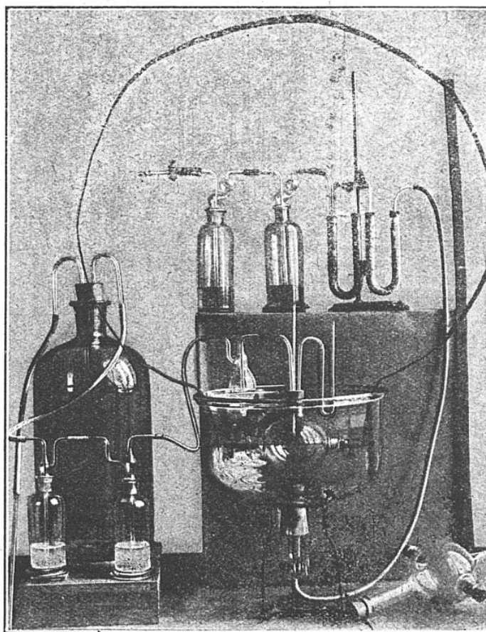
FIG. 1. — RÉSONATEUR-INFLAMMATEUR AVEC SES DISPOSITIFS D'ÉPURATION
