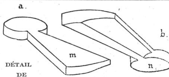
L'ESCALIER A VIS OU EN LIMAÇON
