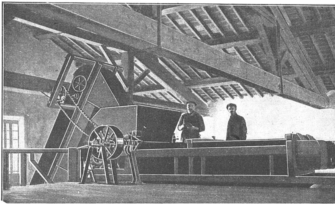
INSTALLATION COMPLÈTE D'UN FOULOIR-ÉGOUTTOIR AVEC ÉLÉVATEUR DE VENDANGE
