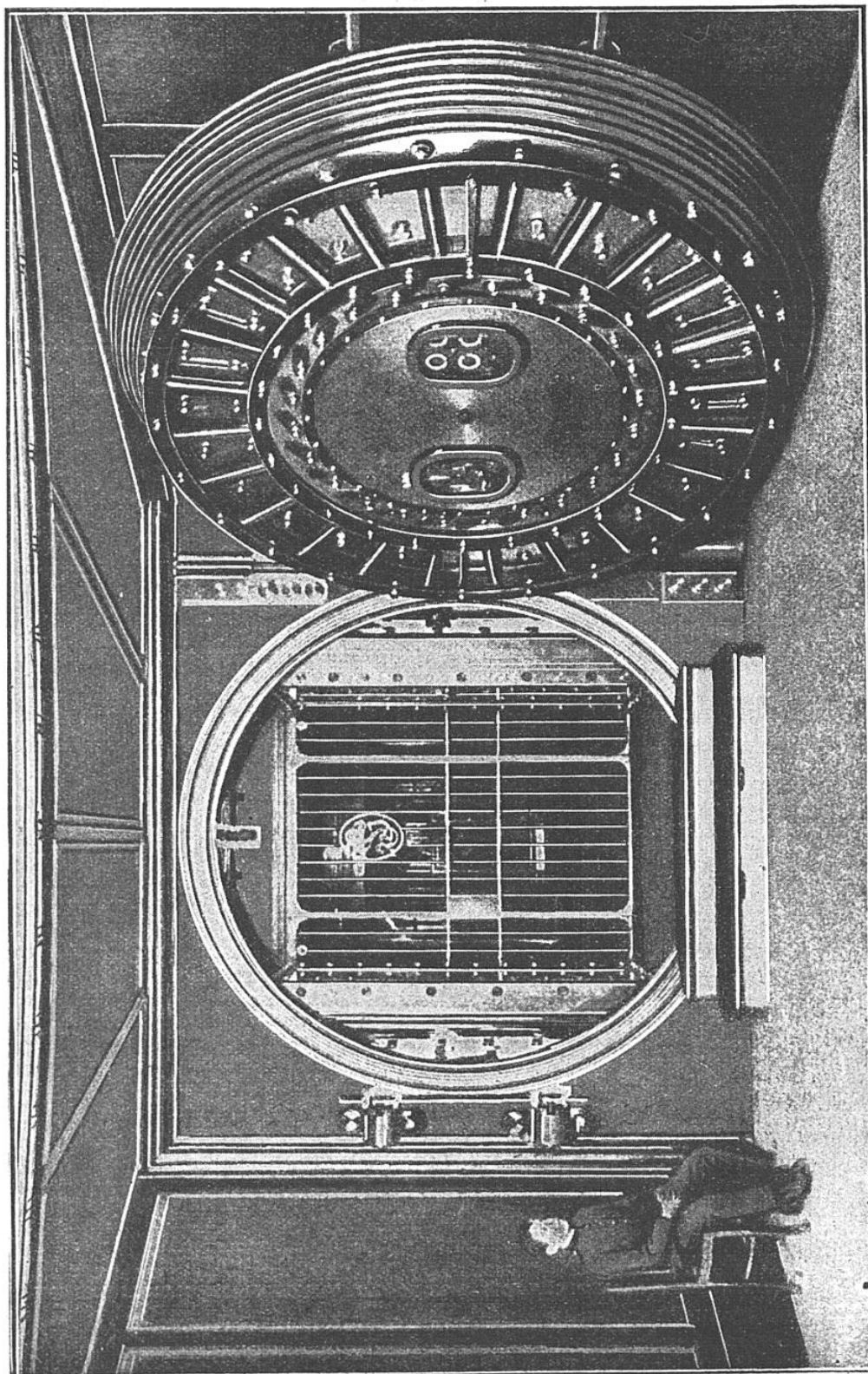
UNE FORMIDABLE ENTRÉE DE « CHAMBRE-FORTE » DANS UN GRAND ÉTABLISSEMENT FINANCIER PARISIEN. Cette construction circulaire mesure environ 2 m. 80 de diamètre. Fortement cuirassée et blindée, armée de substances réfractaires, elle se ferme à l'aide de vingt-quatre pénes rayonnantes commandées par un volant central. La porte obture un tambour fermé lui-même à l'intérieur par une grille pesant vingt tonnes.
