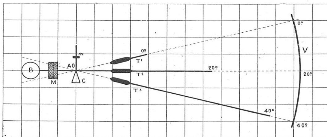
SCHÉMA MONTRANT LE FONCTIONNEMENT DU THERMOMÈTRE POUR AVEUGLES
