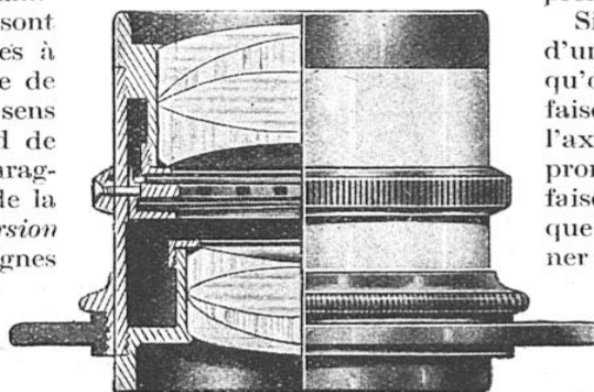
OBJECTIF DOUBLE DIT « DOUBLÉT »
