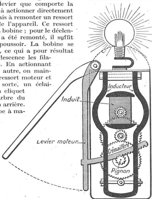
COUPE D'UNE LAMPE ANGLAISE A MAGNÉTO
