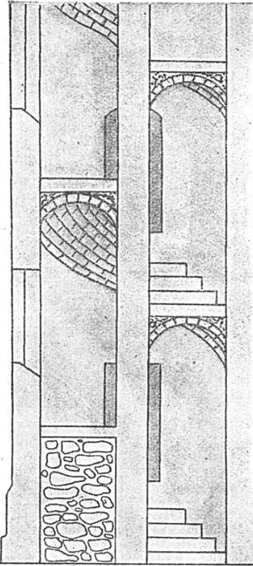
COUPE D'UN ESCALIER A VIS AVEC VOUTE RAMPANTE
