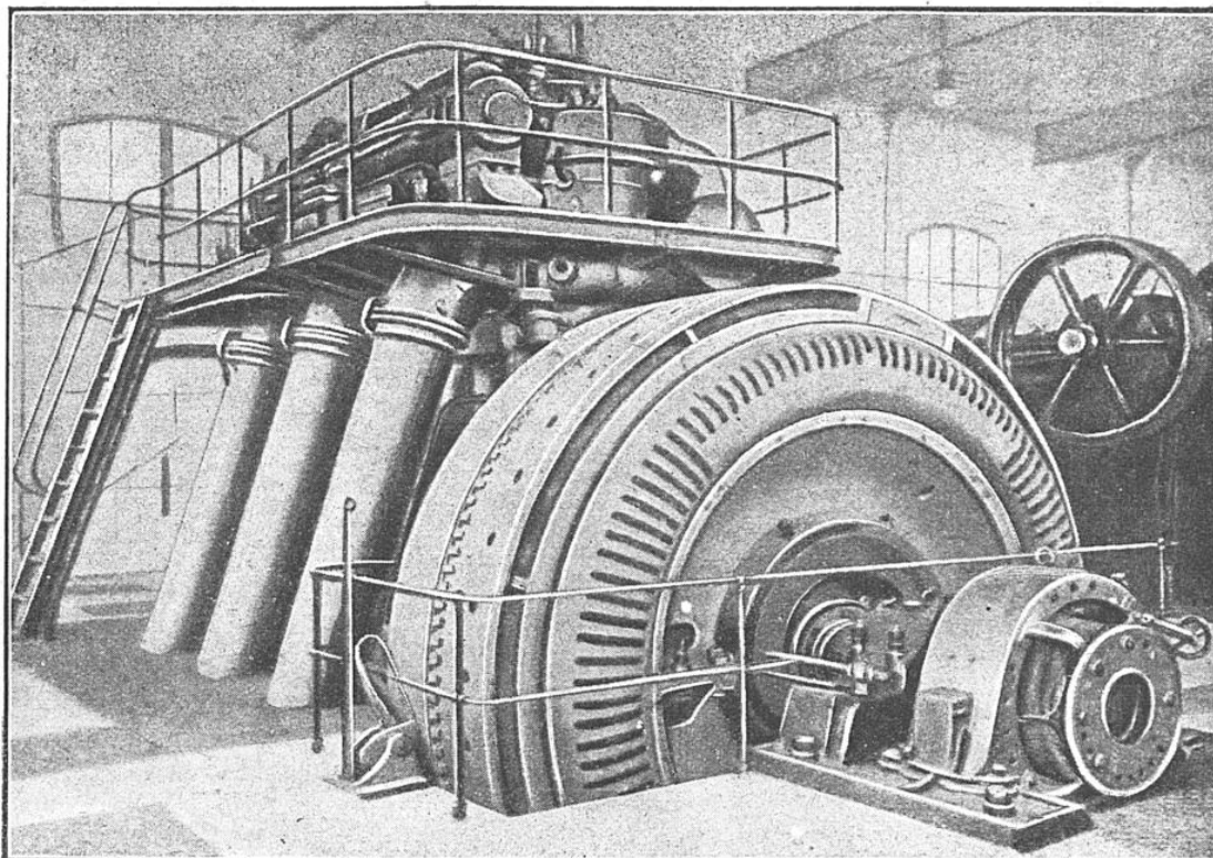
ALTERNATEUR TRIPHASÉ DE 630 KILOWATTS, 5.000 VOLTS, 50 PÉRIODES, 250 TOURS PAR MINUTE, ACCOUPÉ DIRECTEMENT A UN MOTEUR DIESEL
