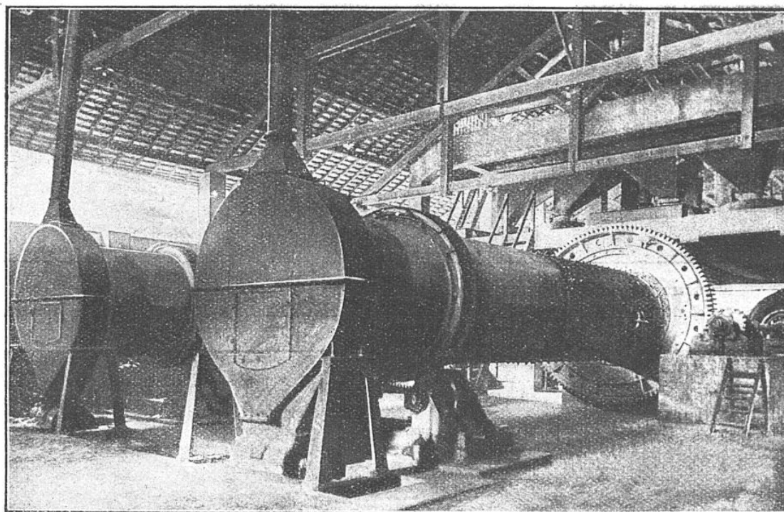
BROYEURS COMPOUND POUR LE BROYAGE DES CLINKERS
