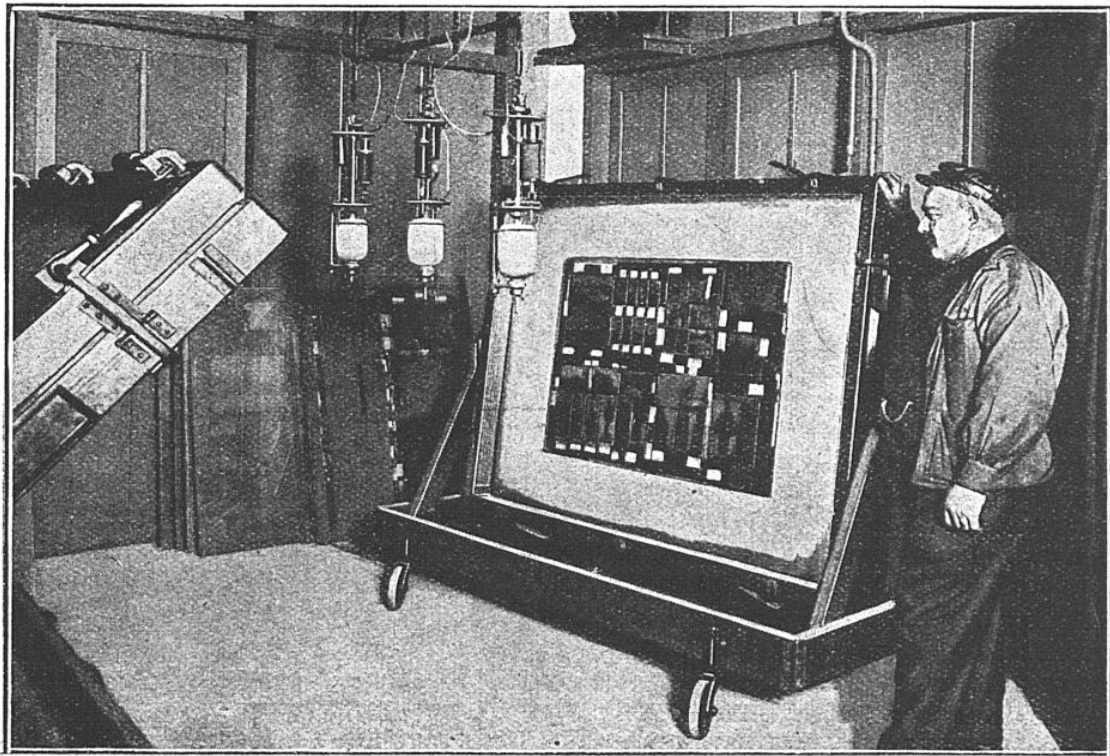
LE TIRAGE DES ÉPREUVES SUR PAPIER AU CHARBON
