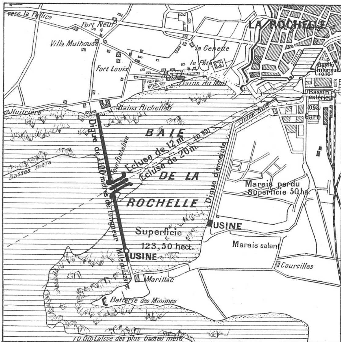
FIG. 9. — PROJET DES TRAVAUX A EXÉCUTER POUR LE CAPTAGE DE LA PUISSANCE DES MARÉES DANS LA BAIE DE LA ROCHELLE ET AU MARAIS-PERDU
