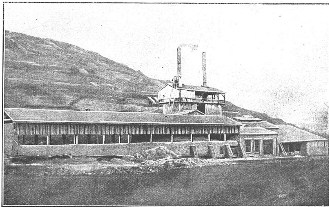
USINE FRANÇAISE POUR LA FABRICATION DES CEMENTS NATURELS
