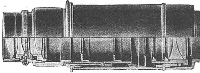
VUE EN DEMI-COUPÉ D'UN TÉLÉ-OBJECTIF
