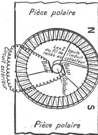
SCHÉMA DE LA MACHINE GRAMME MONTRANT L'ENROULEMENT DU FIL SUR LE NOYAU D'INDUIT EN FORME DE COURONNE
