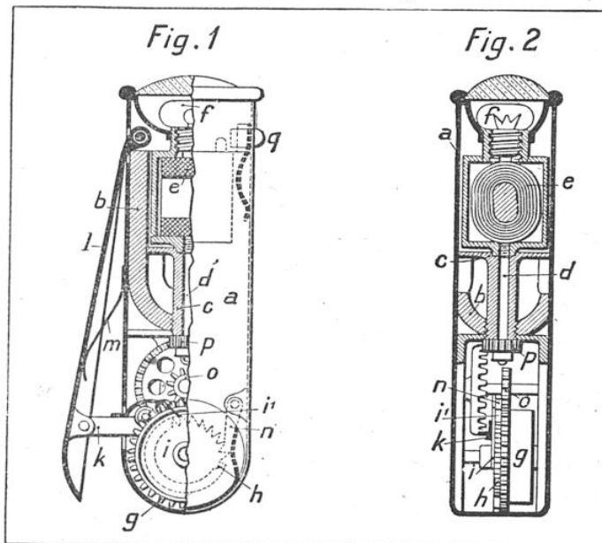
LA LAMPE A MAGNÉTO D'INVENTION SUISSE
