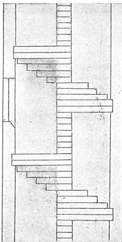
ESCALIER A VIS AVEC NOYAU ET MARCHE D'UNE SEULE PIÈCE
