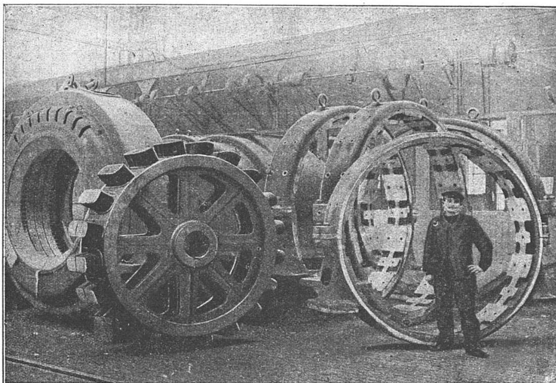
GROUPE DE CARCASSES MÉTALLIQUES DE DYNAMOS ET D'ALTERNATEURS
