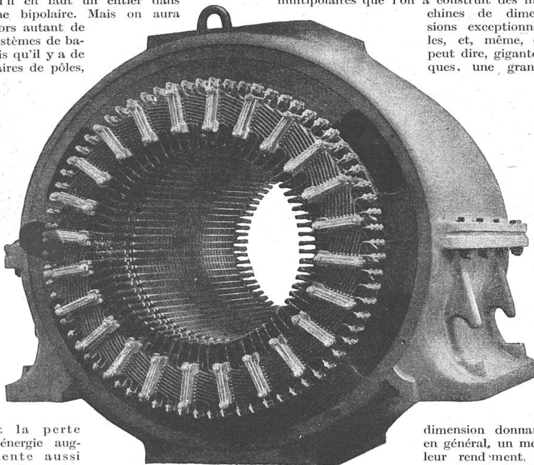
STATOR (PARTIE FIXE) D'UN ALTERNATEUR DE 5.000 KILOWATTS, 1.500 TOURS PAR MINUTE
