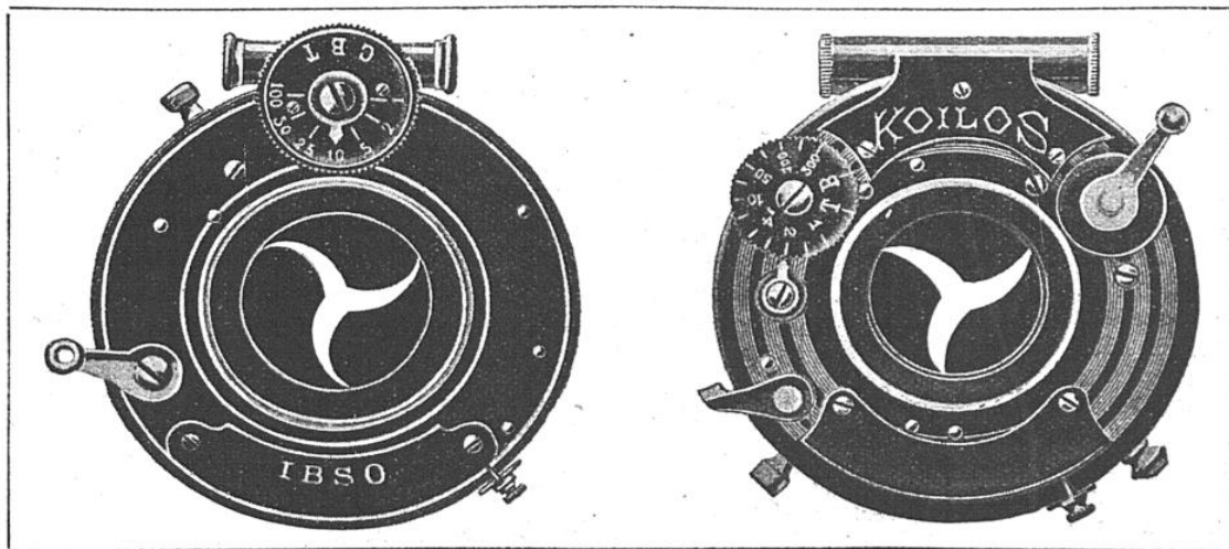
DEUX MODÈLES D'OBTURATEURS CENTRAUX A SECTEURS. A TROIS LAMES
