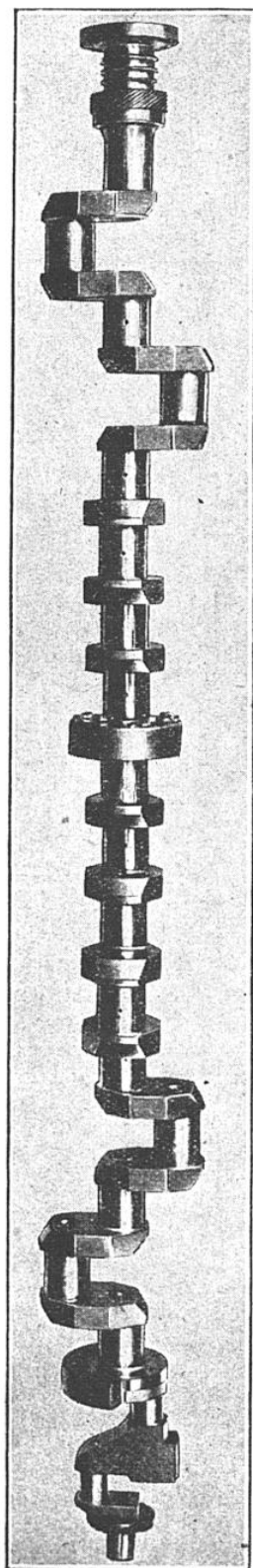
ARBRE PRINCIPAL (8 M. 75 DE LONG) D'UN MOTEUR DIESEL DE SUBMERSIBLE A HUIT CYLINDRES, A QUATRE TEMPS
