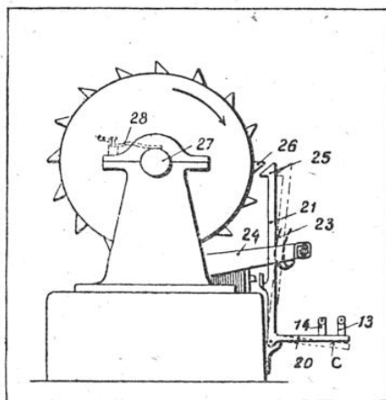
VUE DÉTAILLÉE D'UNE POSITION DE LA FIGURE 2 DE LA PLANCHE DE LA PAGE PRÉCÉDENTE
