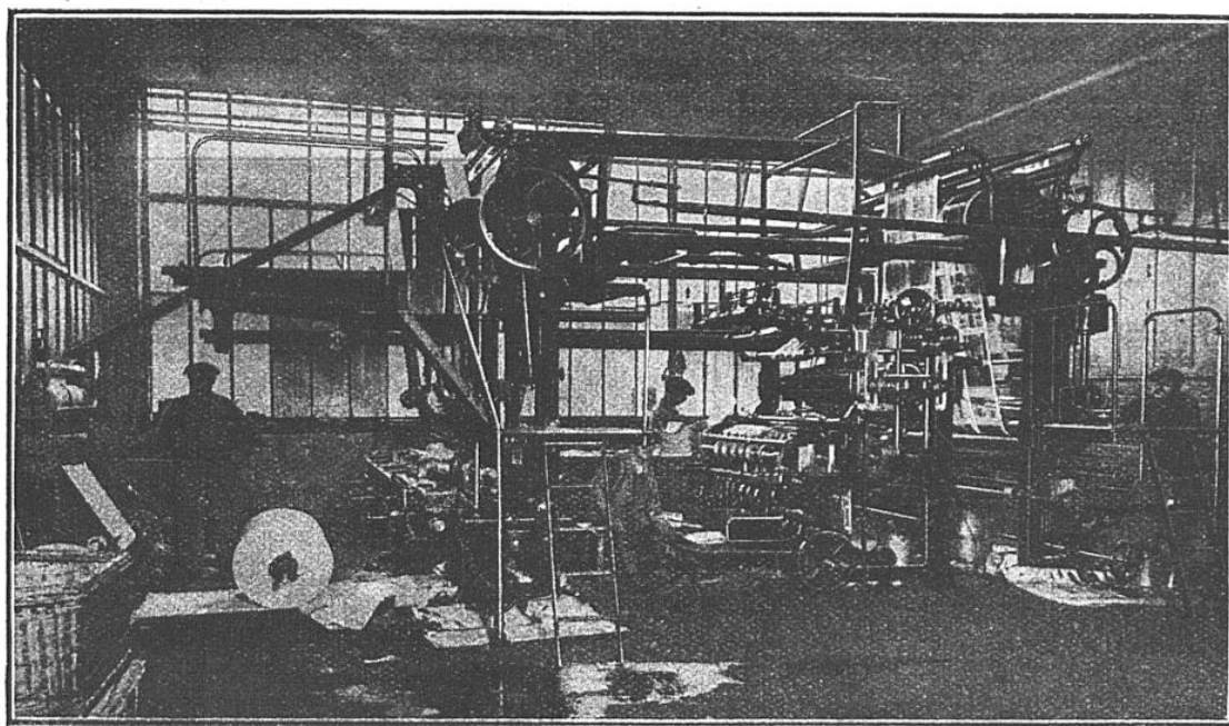
VUE GÉNÉRALE D'UNE PRESSE DE ROTOGRAVURE (IMPRIMERIE DU « MIROIR »)
