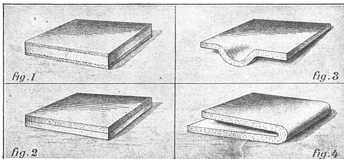
BLINDAGES EMPLOYÉS DANS LA CONSTRUCTION DES COFFRES-FORTS
