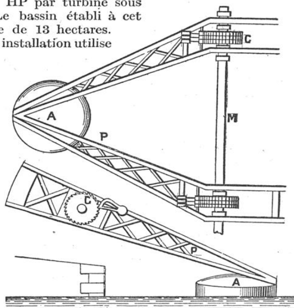
FIG. 1. — MARÉMOTEUR SYSTÈME FUSENOT (Vues en plan et en élévation.)
