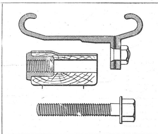
LA JANTE RÉUNIE PAR SES ÉPAULEMENTS
