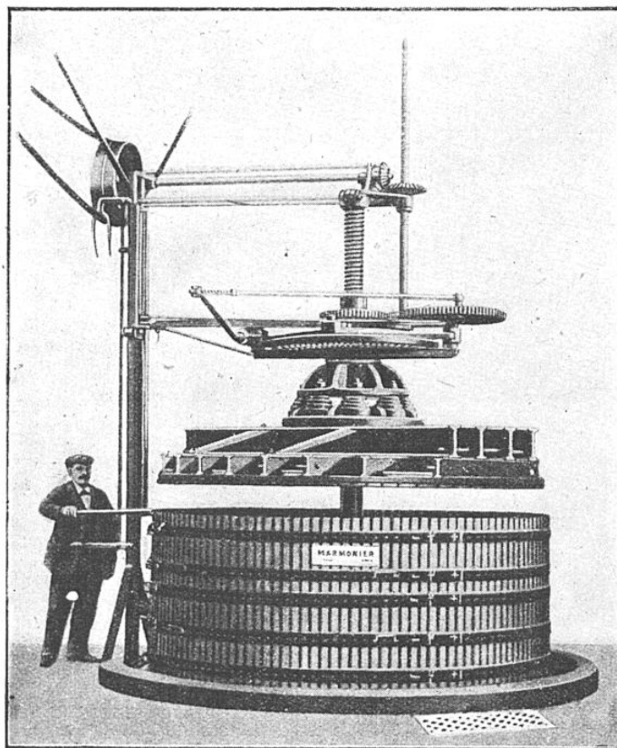
UN GRAND PRESOIR AVEC AUTO-DÉCLAT
