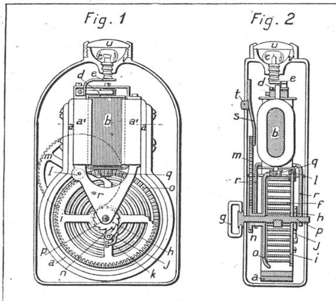
LAMPE A MAGNÉTO FRANÇAISE, A RESSORT D'HORLOGERIE
