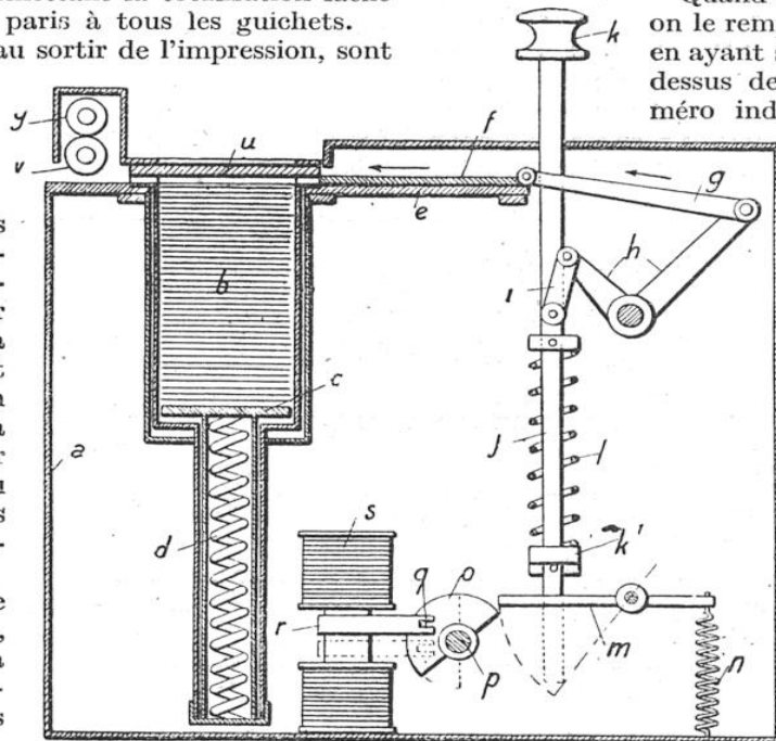
DISTRIBUTEUR-TOTALISATEUR DE M. SEIDLINGER
