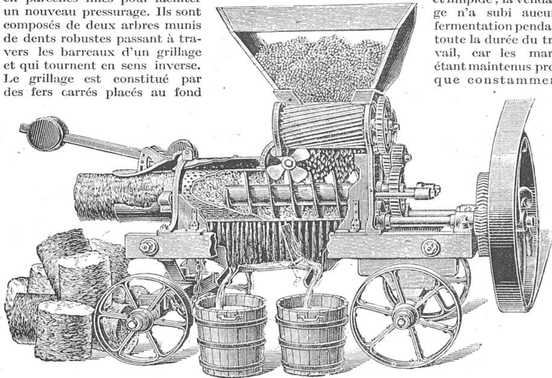
DISPOSITIF INTÉRIEUR D'UN PRESSEUR CONTINU, SYSTÈME MABILLE
