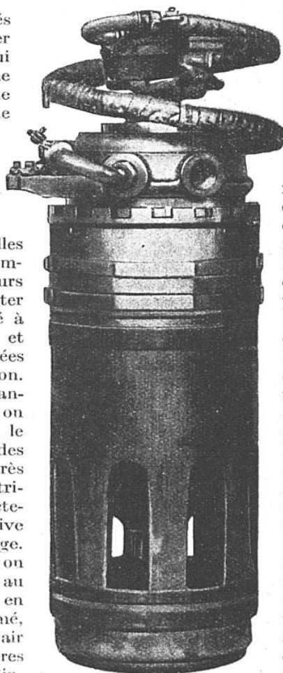
SOUPAPE DE DÉCHARGE DES CYLINDRES D'UN MOTEUR DIESEL-TOSI
