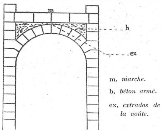
DÉTAIL DE LA VOUTE RAMPANTE
