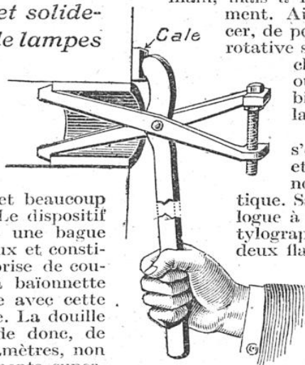
UN OUTIL QUI PERMET D'ARRACHER D'UNE PIÈCE UNE AUTRE PIÈCE ENTRÉE A FOND
