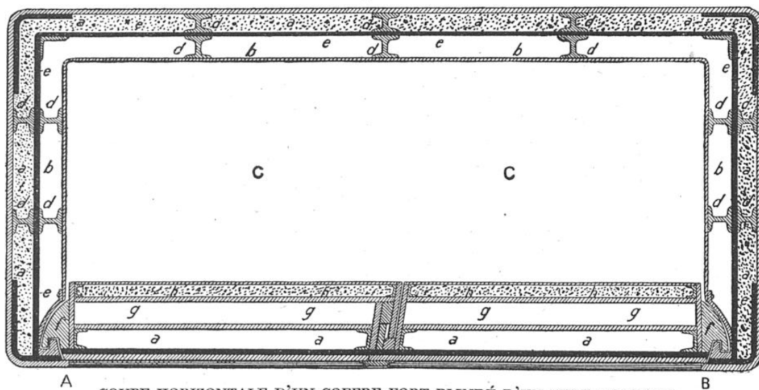
COUPE HORIZONTALE D'UN COFFRE-FORT BLINDÉ D'UN TYPE MODERNE
