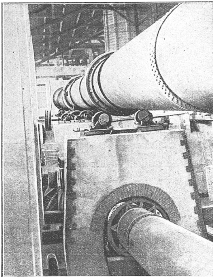
FOUR ROTATIF ET REFROIDISSEUR EMPLOYÉS* A ALGER
