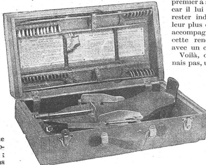
CETTE BOITE RENFERME L'APPAREIL A MESURER LA POINTURE DES BRODEQUINS MILITAIRES ET SON ASSORTIMENT DE LAMES VÉRIFICATRICES
