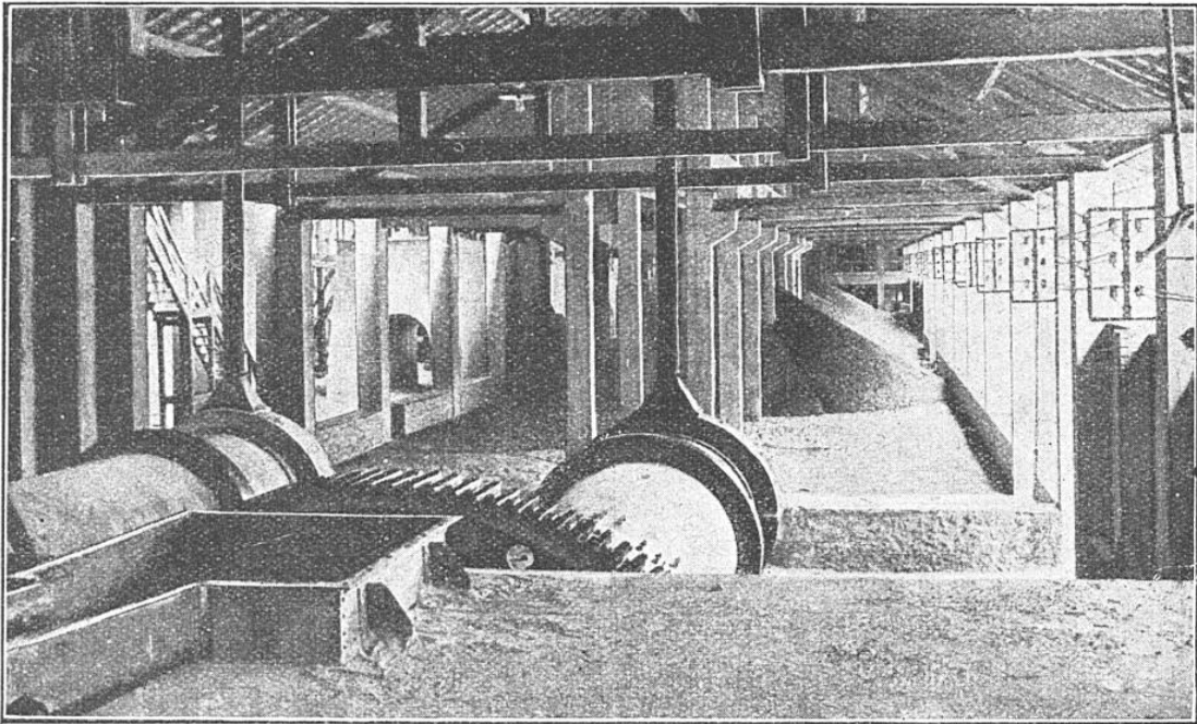
ATELIER DE BROYAGE DES MATIÈRES PREMIÈRES DANS UNE USINE A CIMENT
