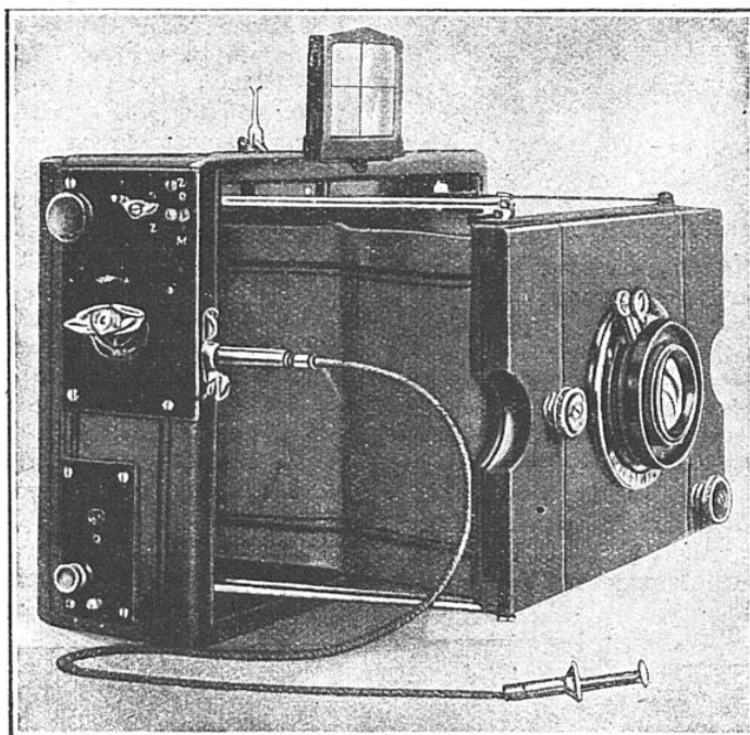
CHAMBRE PORTATIVE AVEC OBTURATEUR DE PLAQUE
