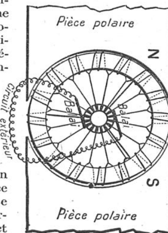
SCHÉMA DE LA MACHINE GRAMME, AVEC UN COLLECTEUR COMPOSÉ DE SEGMENTS ISOLÉS LES UNS DES AUTRES
