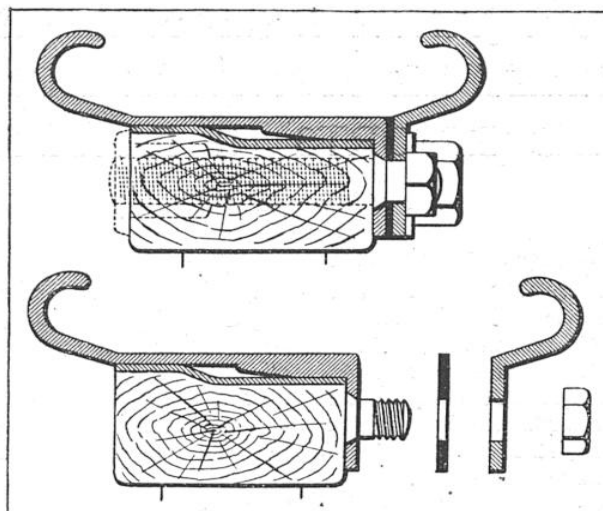
JANTE DIVISIBLE ET DÉTACHABLE
