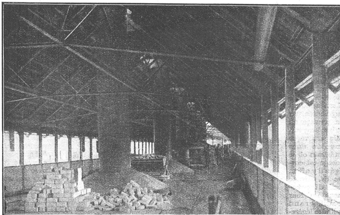
FOURS CANDLOT PERPIGNANI POUR LA FABRICATION DES CEMENTS NATURELS
