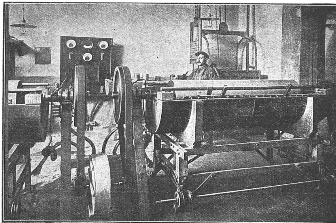
L'OPÉRATION DU CUIVRAGE DES CYLINDRES DE ROTOGRAVURE
