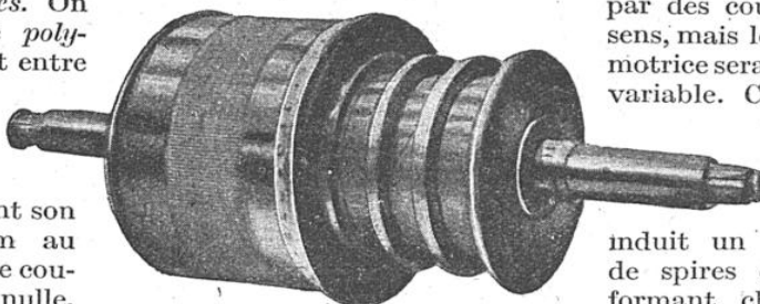
ROTOR (OU INDUIT) D'UN GÉNÉRATEUR A COURANT CONTINU DE 2.000 KILOWATTS ET 1.000 TOURS PAR MINUTE
