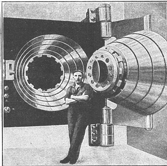
TROU D'HOMME DANS UNE CHAMBRE-FORTE
