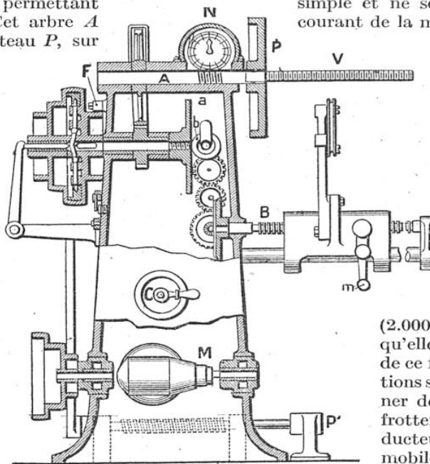
MACHINE A BOBINER-LES NOYAUX D'ELECTROS
