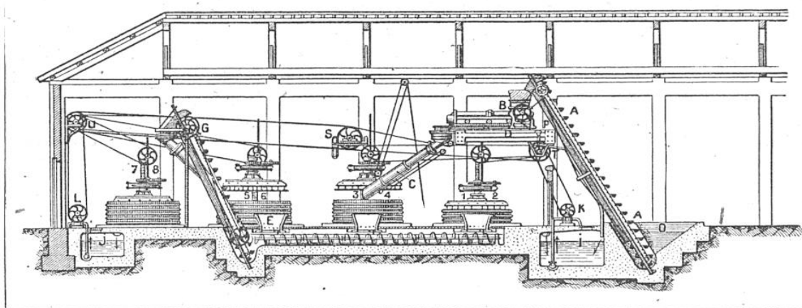
INSTALLATION MÉCANIQUE VINAIRE POUR LA FABRICATION DU VIN BLANC
