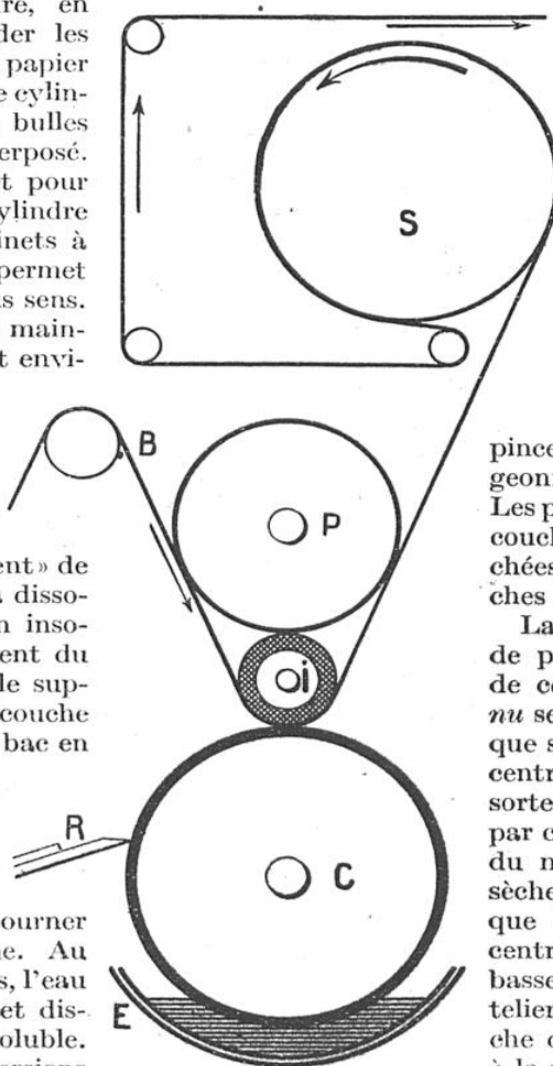
IMPRESSION DE L'HÉLIO GRAVURE ROTATIVE
