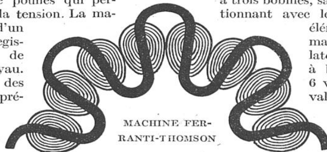
Ruban de cuivre formant l'armature de l'induit et passant devant les électro-inducteurs.
