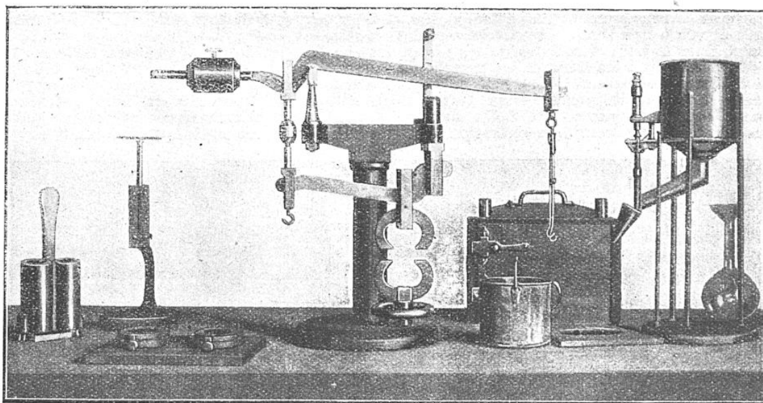
APPAREILS SERVANT A L'ESSAI PHYSIQUE DES CEMENTS AVANT L'EMPLOI
