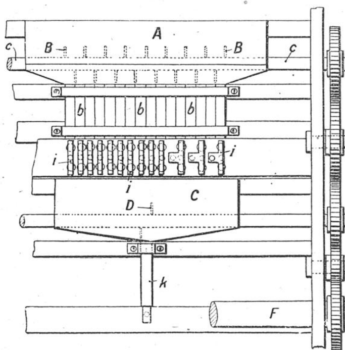
VUE DE COTÉ DE L'APPAREIL TUQUET MONTRANT LES CONNEXIONS ENTRE LES DIVERS ORGANES ET PIÈCES A, premier réservoir à billes. (Les autres lettres, comme dans les figures de la page 153).
