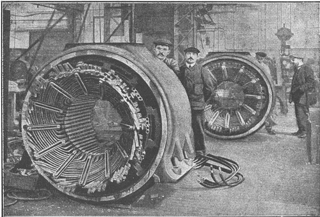
VUE PRISE DANS UN ATELIER DE BOBINAGE DE STATORS OU PARTIES FIXES D'ALTERNATEURS
