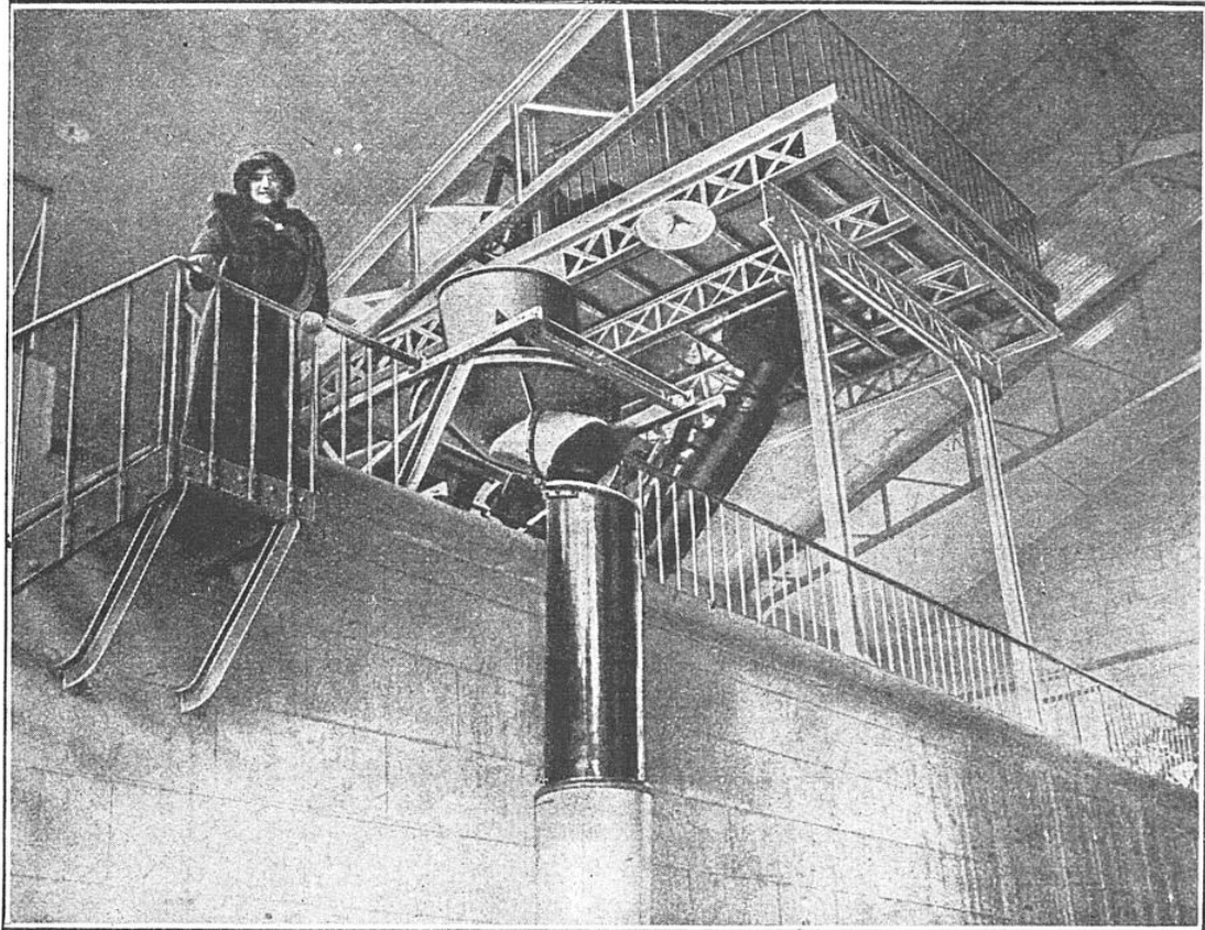
PLANCHER D'UN FOULOIR-ÉGOUTTOIR ET SON ÉLÉVATEUR
