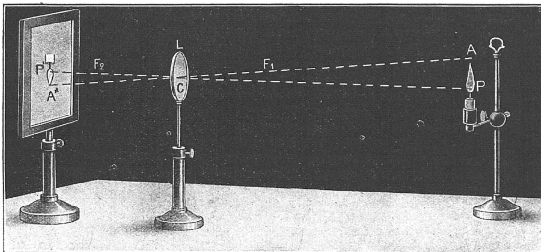
IMAGE SUR UN ÉCRAN D'UN OBJET LUMINEUX PLACÉ DEVANT UNE LENTILLE SIMPLE.
