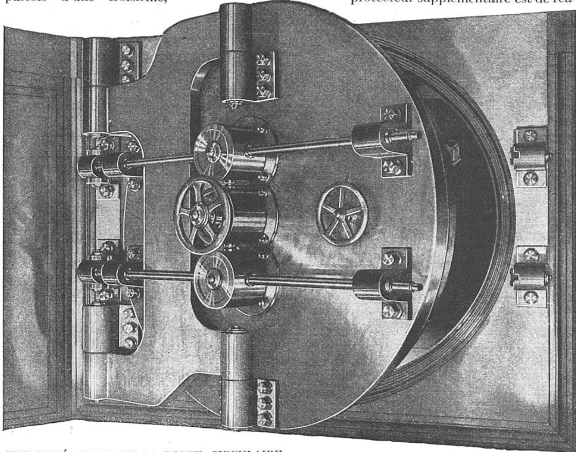
VUE EXTÉRIEURE DE LA PORTE CIRCULAIRE FERMANT LES CAVEAUX BLINDÉS DE CERTAINS GRANDS ÉTABLISSEMENTS FINANCIERS Les pènes du pourtour et les deux barres transversales de sécurité sont actionnés par des volants.
