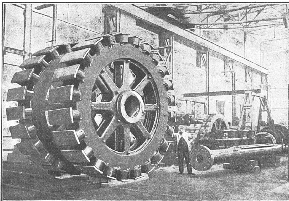
ROUE POLAIRE D'UN GÉNÉRATEUR DOUBLE AVANT L'OPÉRATION DU BOBINAGE
