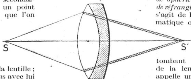
CORRECTION DE L'ABERRATION CHROMATIQUE
