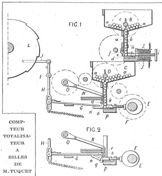
Fig. 1 : vue en élévation et en coupe ; fig. 2 : vue de détail de l'organe inférieur après son fonctionnement. — a, billes ; B, moulins ; b, couloirs verticaux ; c, arbre des moulins ; d, cavité ; e, paroi mobile fermant la cavité à gauche et pivotant autour d'un axe ; f, h, piston à ressort ; i, armature d'un électro ; j, bobines ; C, réservoir ; D, moulin du réservoir C ; k, couloir vertical ; o, cavité ; n, plaque mobile pivotant sur l'axe q, fermant la cavité à gauche ; p, piston à ressort fermant la cavité à droite ; E, excentrique sur l'arbre F ; G, tige qui est relevée quand la plaque n pivote sur son axe ; H, grande branche d'un levier pivotant sur l'axe I ; J, bielle ; L, rochet commandant la roue des dizaines du compteur.
