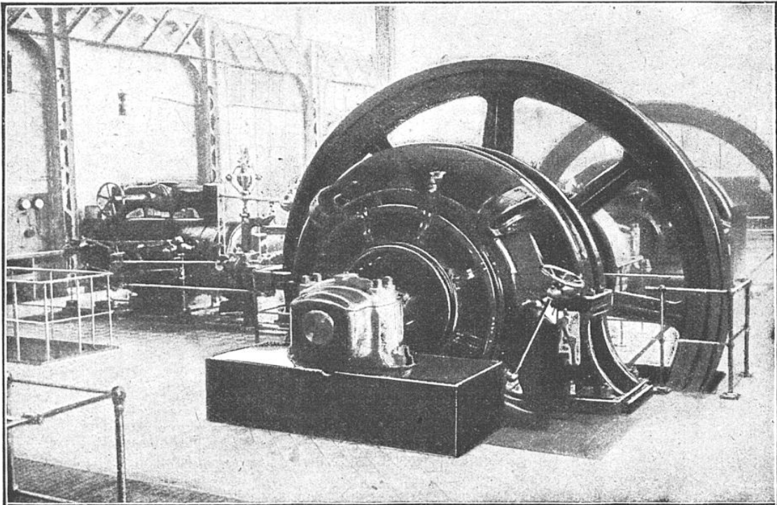
VUE D'UNE DYNAMO MULTIPOLAIRE ACCOUPÉE A UNE MACHINE A VAPEUR
