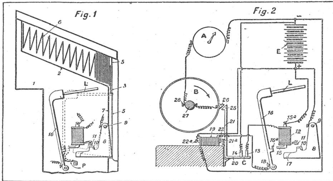
VUES SCHÉMATIQUES DU TOTALISATEUR DE M. KIPARSKI
