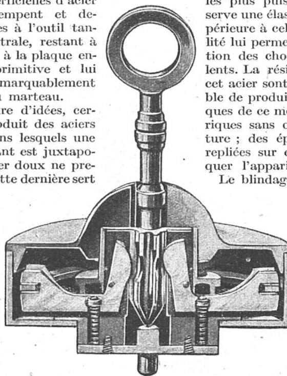
VUE EN COUPE D'UNE SERRURE DE COFFRE-FORT
