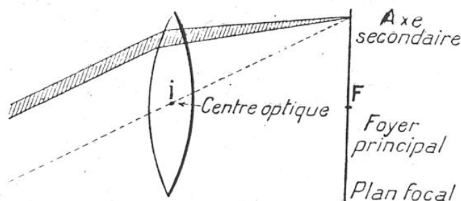
PROPRIÉTÉS OPTIQUES D'UNE LENTILLE CONVERGENTE Tous les rayons lumineux traversant une lentille convergente sont déviés, sauf ceux qui passent par un point i dénommé centre optique . Ces derniers rayons sont dits « axes secondaires » par opposition à l'axe principal i F .
