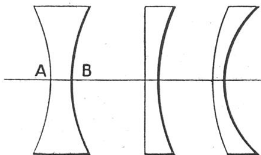
LES TROIS GENRES DE LENTILLES CONCAVES OU A BORDS ÉPAIS
