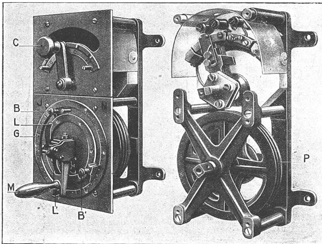
UN MANIPULATEUR A CADRAN
