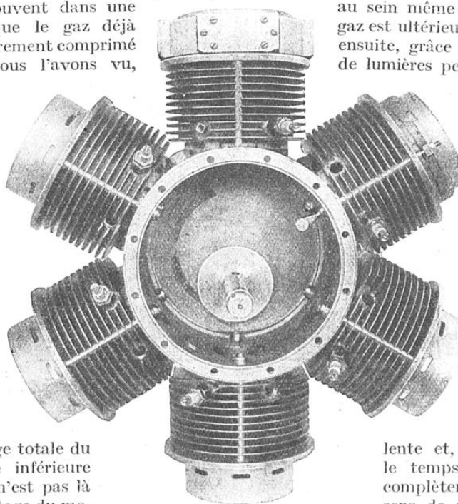
VUE DU CARTER ÉTANCHE (BOÎTE DE MANIVELLE) DANS LEQUEL SONT REFŒULÉS ET LÉGÈREMENT COMPRIMÉS LES GAZ FRAIS AVANT LEUR ADMISSION DANS LES CYLINDRES
