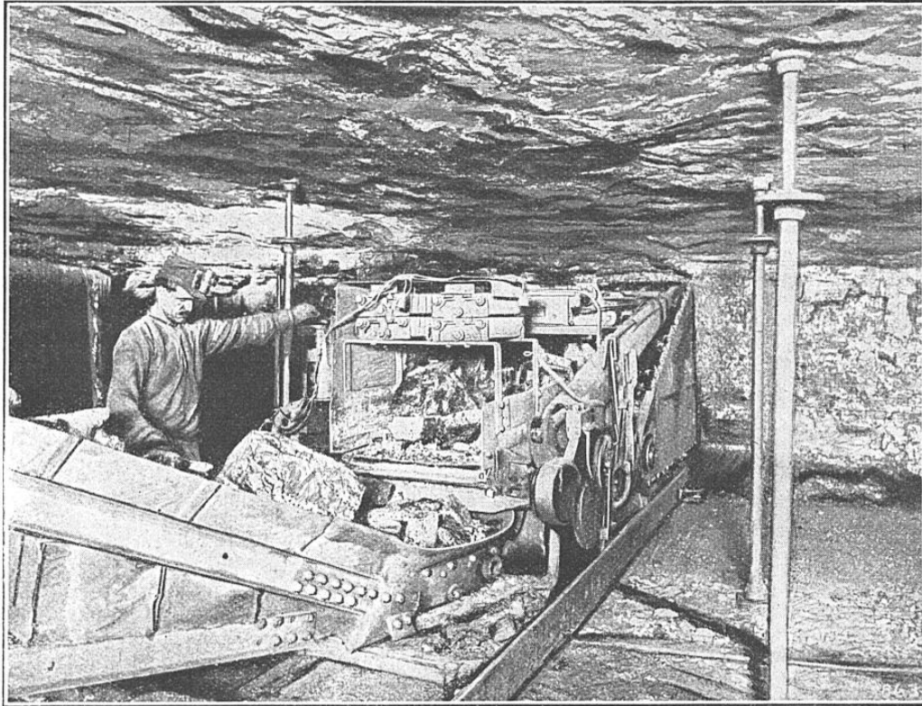
MACHINE A ABATTRE LE CHARBON EN ACTIVITÉ SUR UN FRONT DE TAILLE
