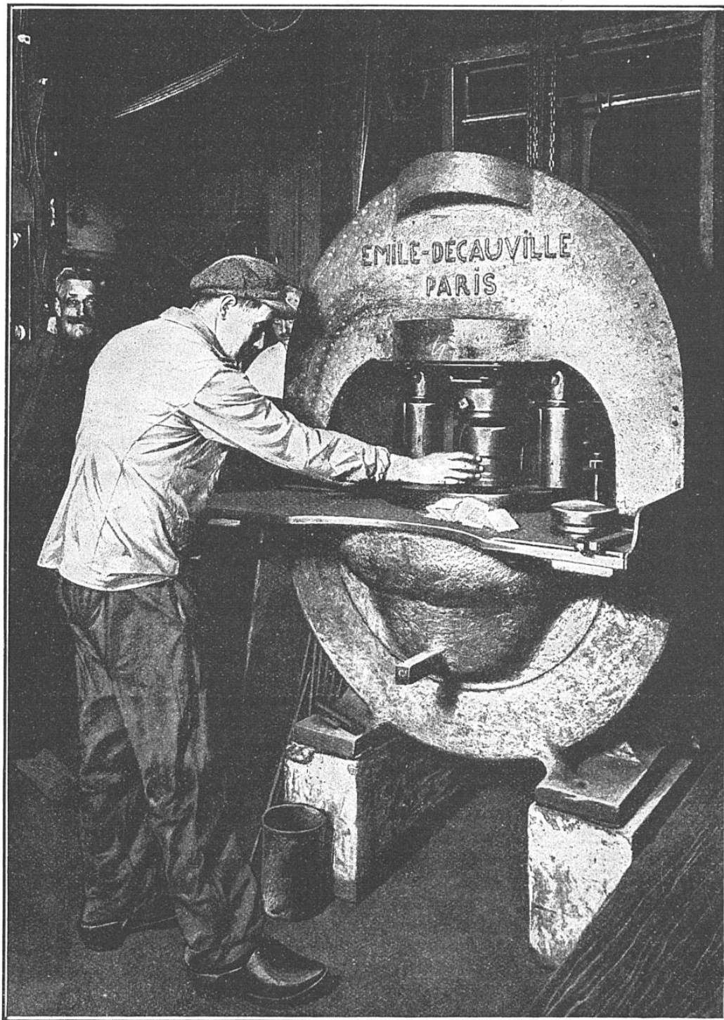
MANŒUVRE DE LA PRESSE DE MILLE TONNES POUR LA COMPRESSION DES « FLANS »
