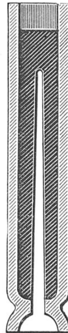
LA POUDRE FUSANTE EST INTRODUITE MÉCANIQUEMENT DANS LES « JETS » OU FUSÉES FIXES
