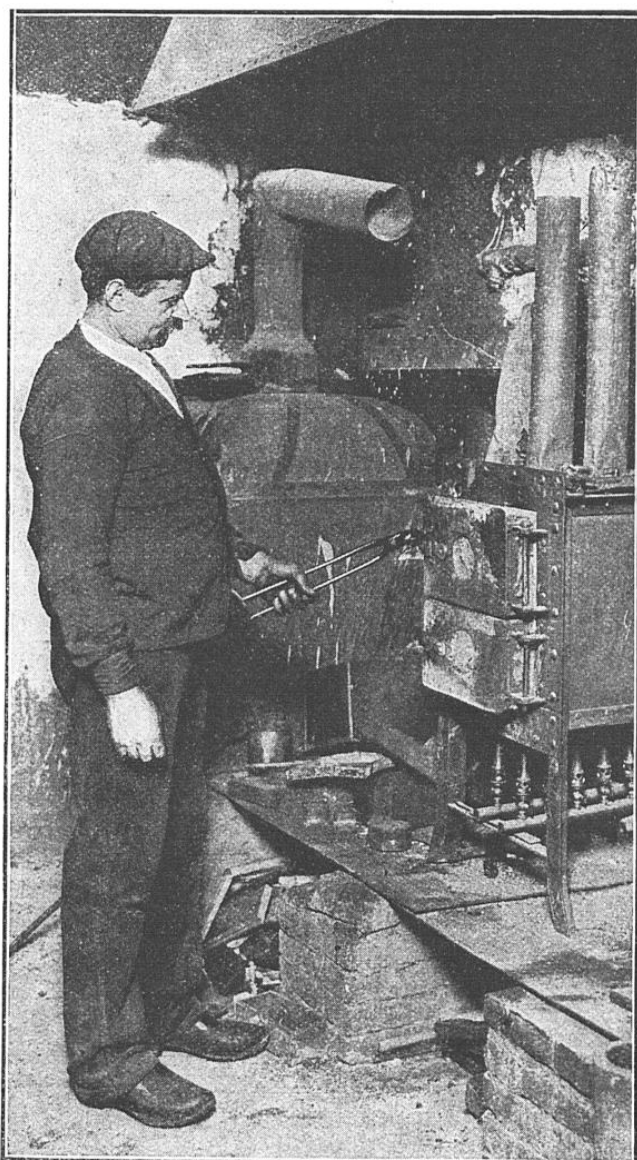
FOUR SPÉCIAL POUR LE CHAUFFAGE, A L'ABRI DE L'AIR, DES POINÇONS ET MATRICES DEVANT SUBIR LA TREMPÉ ET LA RECUISSE
