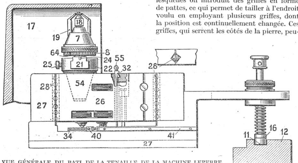
VUE GÉNÉRALE DU BÂTI DE LA TENAILLE DE LA MACHINE LEPERRE
