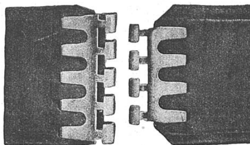
LES PARTIES MÂLE ET FEMELLE DE L'AGRAFE
