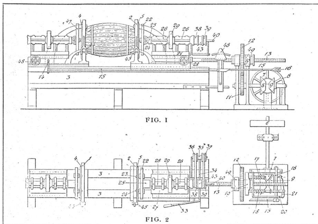
PLANCHE 12. — DÉTAILS DE LA MACHINE A CHAN- FREINER, A JABLER, A DOLER, DE MM. RITCHIE ET LINDSAY
