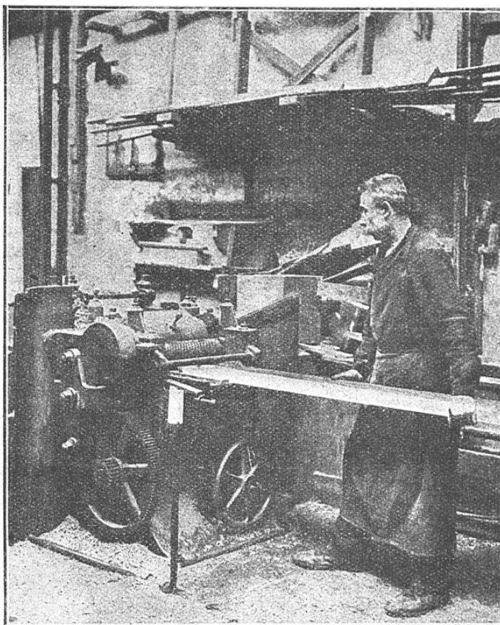
FIG. 8. — RABOTAGE DES DEUX FACES DES DOUVES
