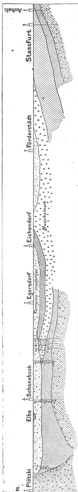
COUPE GÉNÉRALE, ENTRE PLÖTZKI ET ANHALT, DE L'IMPORTANT BASSIN SALIFÈRE PRUSSIEN DE STASSFURT
