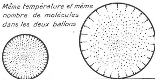
EXPLICATION DE LA PRESSION DES GAZ
