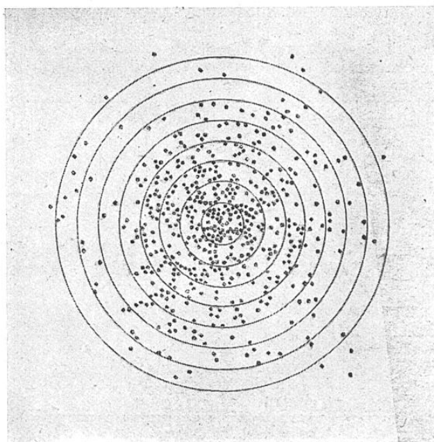
UNE IMAGE EN PLAN DU MOUVEMENT BROWNIEN
