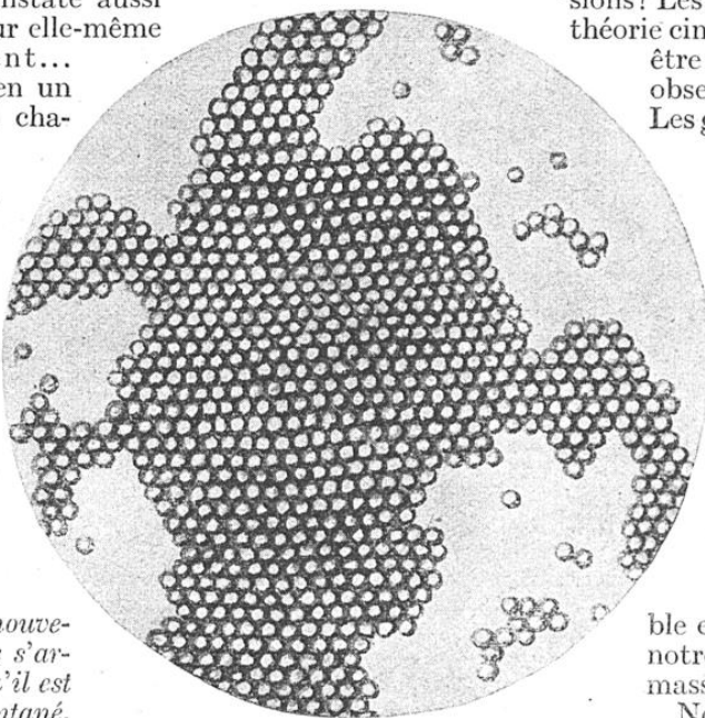
SPHÉRULES D'UNE ÉMULSION, TRIÉES PAR CENTRIFUGATION POUR LE CALCUL DU NOMBRE ET DE LA MASSE DES MOLECULES CONTENUES DANS LA MOLECULE-GRAMME DU CORPS ÉTUDIÉ
