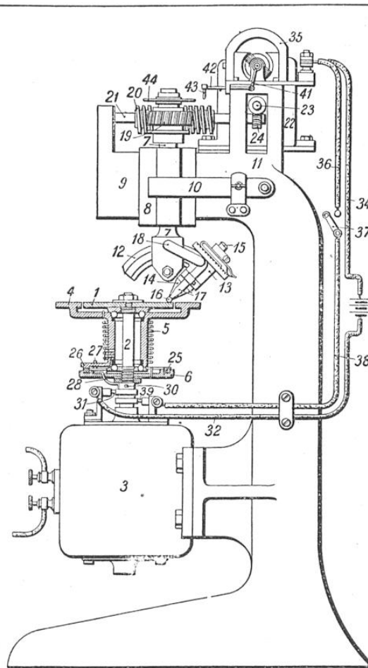
ÉLEVATION LATÉRALE ET COUPE PARTIELLE D'UN APPAREIL SERVANT A LA DÉTERMINATION DES FACES DE CLIVAGE DU DIAMANT (STERN COLEMAN C o )
