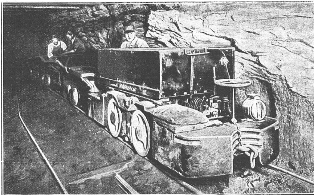
LOCOMOTIVE ÉLECTRIQUE A ACCUMULATEURS POUR GALERIES DE MINE
