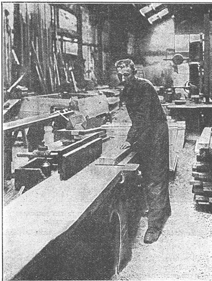
FIG. 4. — DÉGAUCHISSEUSE, POUR DÉGAUCHIR OU DRESSER LES SURFACES DES MERRAINS ET FAIRE MÉCANIQUEMENT LES JOINTS DES DOUVES ET DES FONDS
