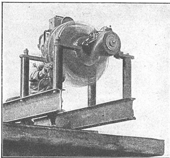
LA NETTETÉ DE CET INSTANTANÉ PROUVE QUE LE MOTEUR EST COMPLÈTEMENT EXEMPT DE VIBRATIONS PENDANT LA MARCHÉ
