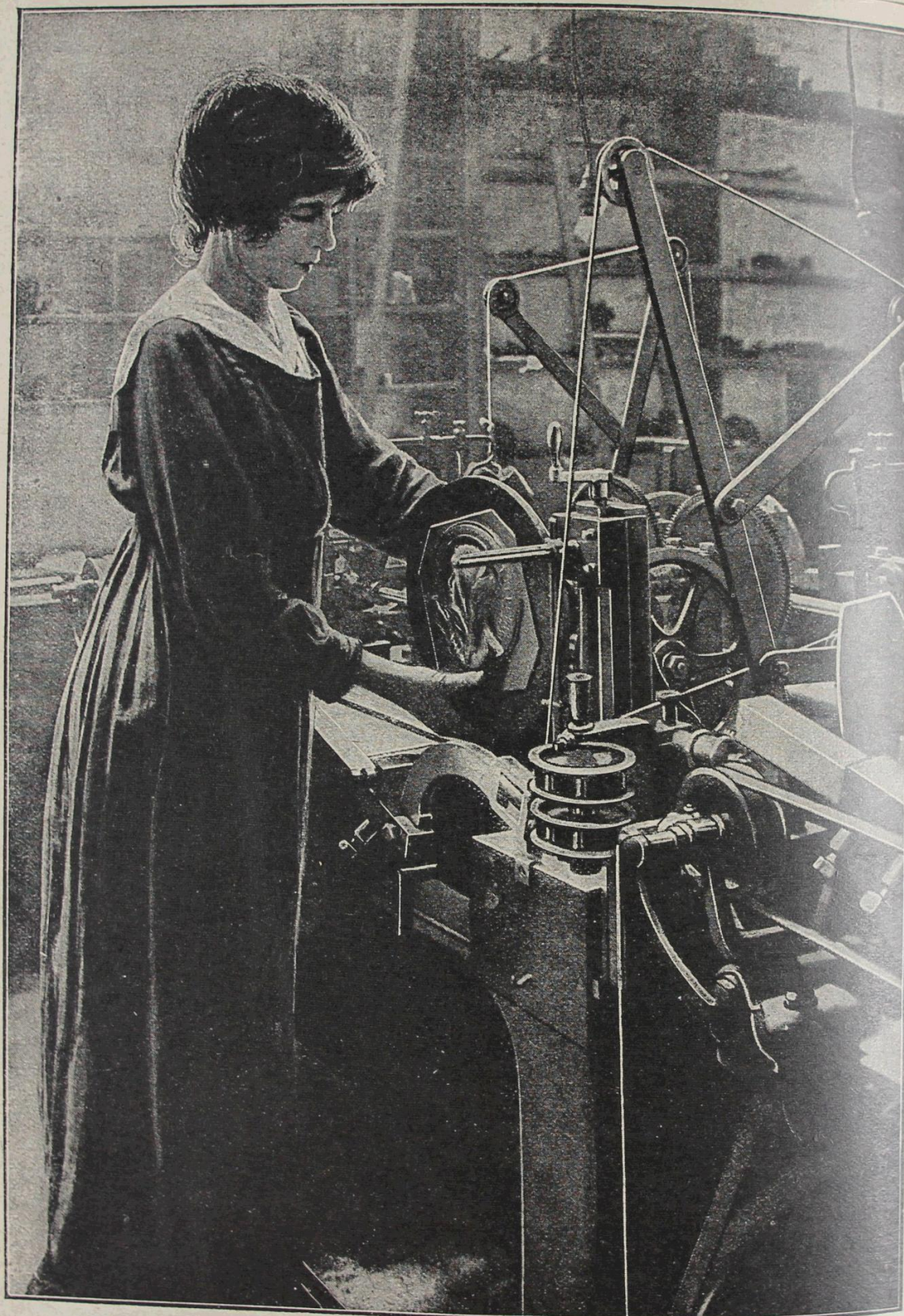
TYPE DE MACHINE A RÉDUIRE DES ATELIERS LUCIEN JANVIER ET C ie Le modèle, en fonte dure ou un galvano nickelé, provenant d'un moulage ou d'une empreinte du sujet en cire ou en terre glaise fait par l'artiste en médailles, est collé par l'ouvrière, au moyen d'un mastic spécial, sur le plateau porte-modèle que l'on voit au centre de la photographie.
