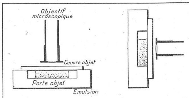
MESURES DE LA RARÉFACTION DES GRAINS
