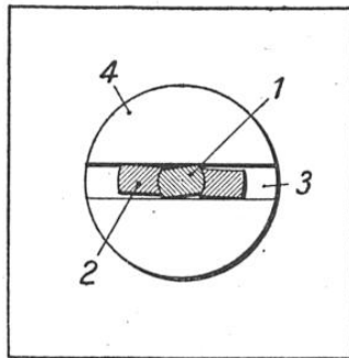
FIG. 2. — LE BISEAU MOBILE ET LE BISEAU FIXE SONT CONTRARIÉS DANS LA FENTE
