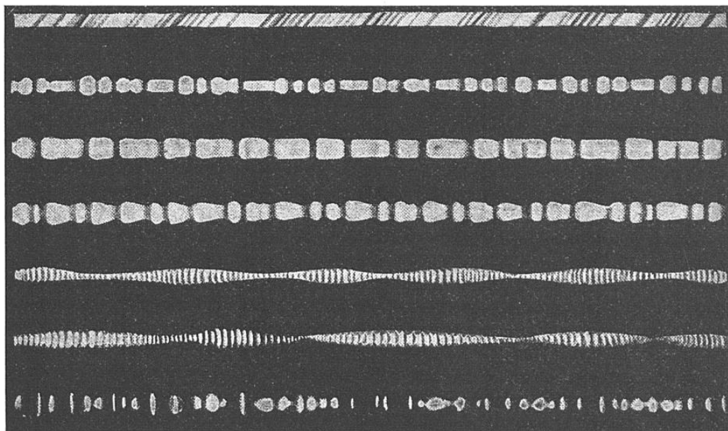
VUE, SOUS UN FORT GROSSISSEMENT, DE L'INSCRIPTION DANS LA CIRE DES VIBRATIONS SONORES
