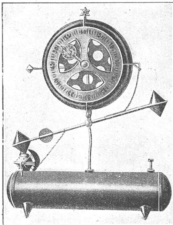
FIG. 8. — HORLOGE THERMIQUE DE M. CORNU Cette horloge utilise pour son fonctionnement la flamme d'une lampe à alcool qui produit, en l'échauffant, des basculements successifs d'un « bouillant de Franklin ».
