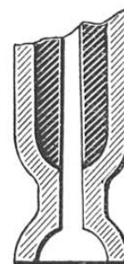
L'ÉTRANGLEMENT DES FUSÉES PAR OU PASSE LA MÈCHE QUI SERVIT À EN- FLAMMER CES ARTIFICES
