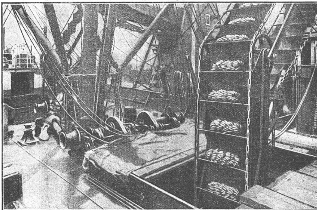
DÉCHARGEMENT A GALVESTON (ÉTATS-UNIS) D'UN VAPEUR CHARGÉ DE BANANES A l'arrivée du navire à quai, on installe, pour le déchargement de ce fruit délicat, un convoyeur mû par l'électricité et dans les poches duquel on place un à un les régimes.
