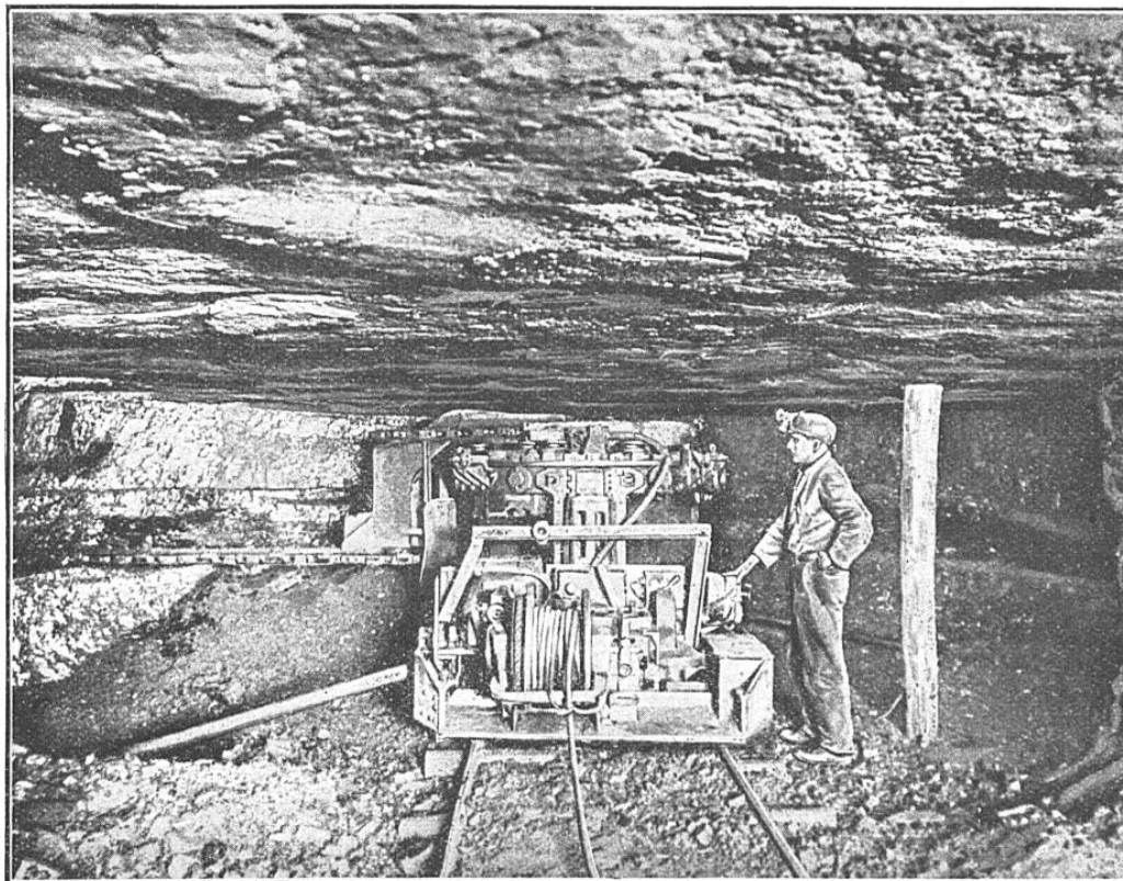
HAVEUSE ÉLECTRIQUE AMÉRICAINE REMPLAÇANT L'ABATAGE À LA MAIN
