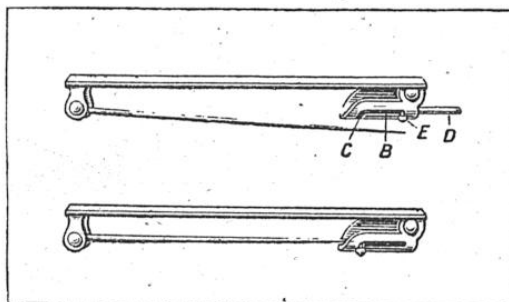
LA POINTE DE CETTE ÉPINGLE EST VERROUILLÉE, APRÈS FERMETURE, PAR UN COULISSEAU CREUX QUE L'ON RABAT SUR ELLE
