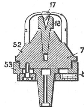
COUPE D'UN DOP DE LA MACHINE À TAILLER AUTOMATIQUE DE M. E. LEPPERRE
