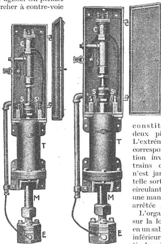
SABOT DE CONTACT SYSTÈME JULIAN BEGGS MONTÉ SUR LA LOCOMOTIVE
