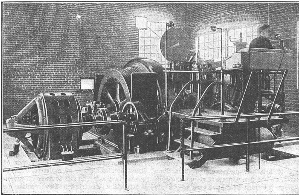
PETITE MACHINE D'EXTRACTION ÉLECTRIQUE POUR Puits INCLINÉ
