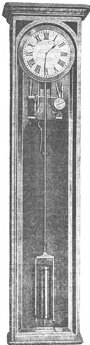
FIG. 30. — LE RÉGULATEUR CAMPICHE (VUE GÉNÉRALE)
