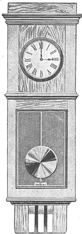
FIG. 17. — REMONTOIR-DISTRIBUTEUR PERRET
