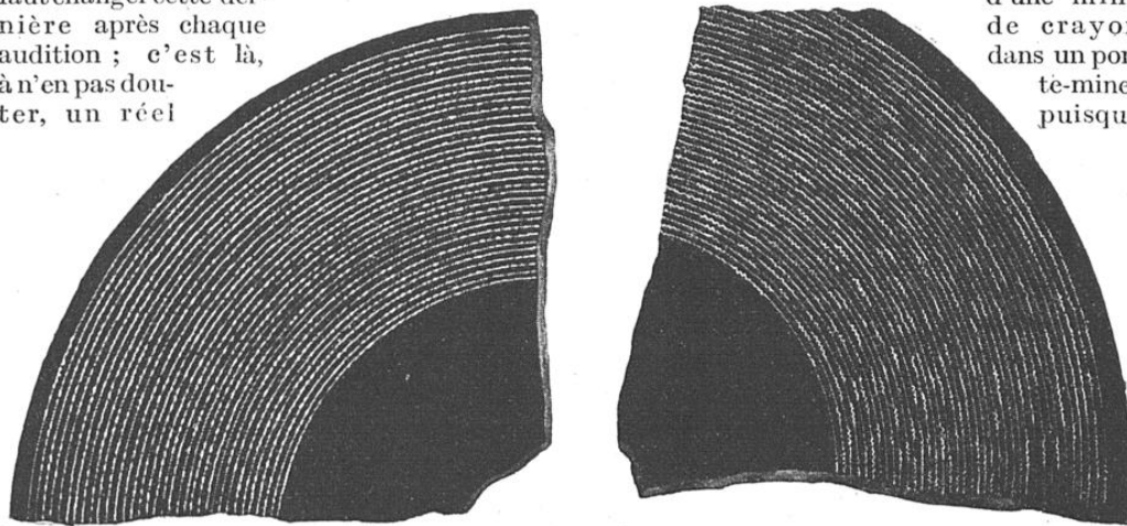
L'AIGUILLE, COMME LE SAPHIR, INTERPRÈTE LES VIBRATIONS DE FAIBLE AMPLITUDE L'aiguille d'acier attaque la cire superficiellement et latéralement (disque de droite) tandis que le saphir la travaille en profondeur à la façon d'un burin (disque de gauche).
