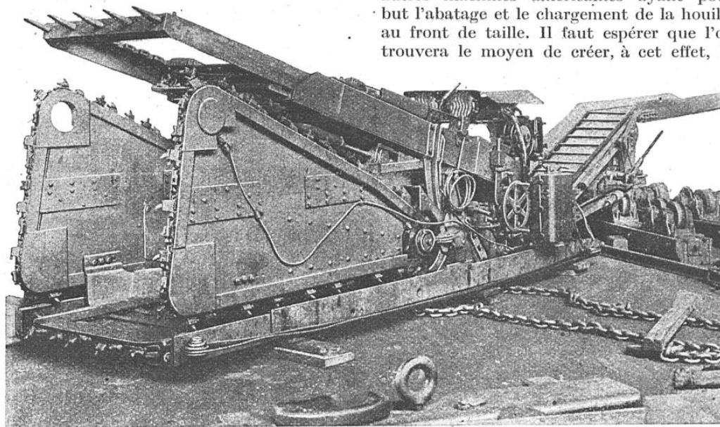
MACHINE SERVANT A L'ABATAGE ET A LA MISE SUR WAGON DE LA HOUILLE
