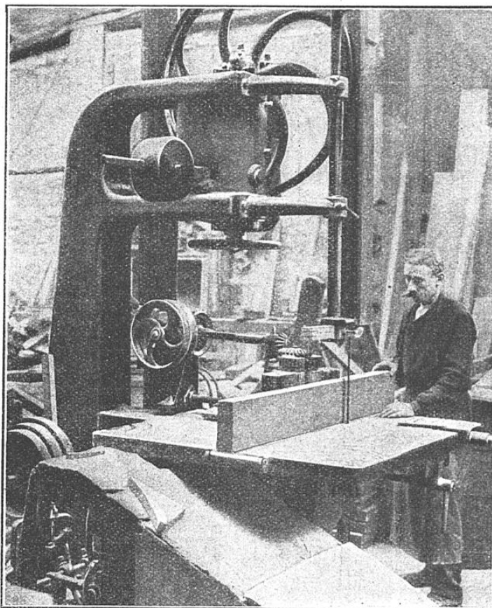
FIG. 6. — SCIE À RUBAN PLUS SPÉCIALEMENT EMPLOYÉE POUR LE DÉDOUBLEMENT DES MERRAINS
