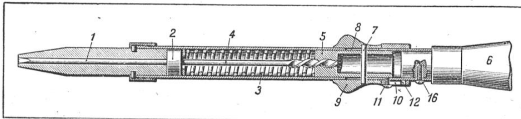
FIG. 3. — C'EST A LA FAÇON DONT L'EXTRÉMITÉ DE LA TIGE CENTRALE 1 S'ORIENTE DANS LA FENTE DE LA VIS, QUE L'OUTIL DOIT DE POUVOIR SAISIR ET MAINTENIR CETTE DERNIÈRE
