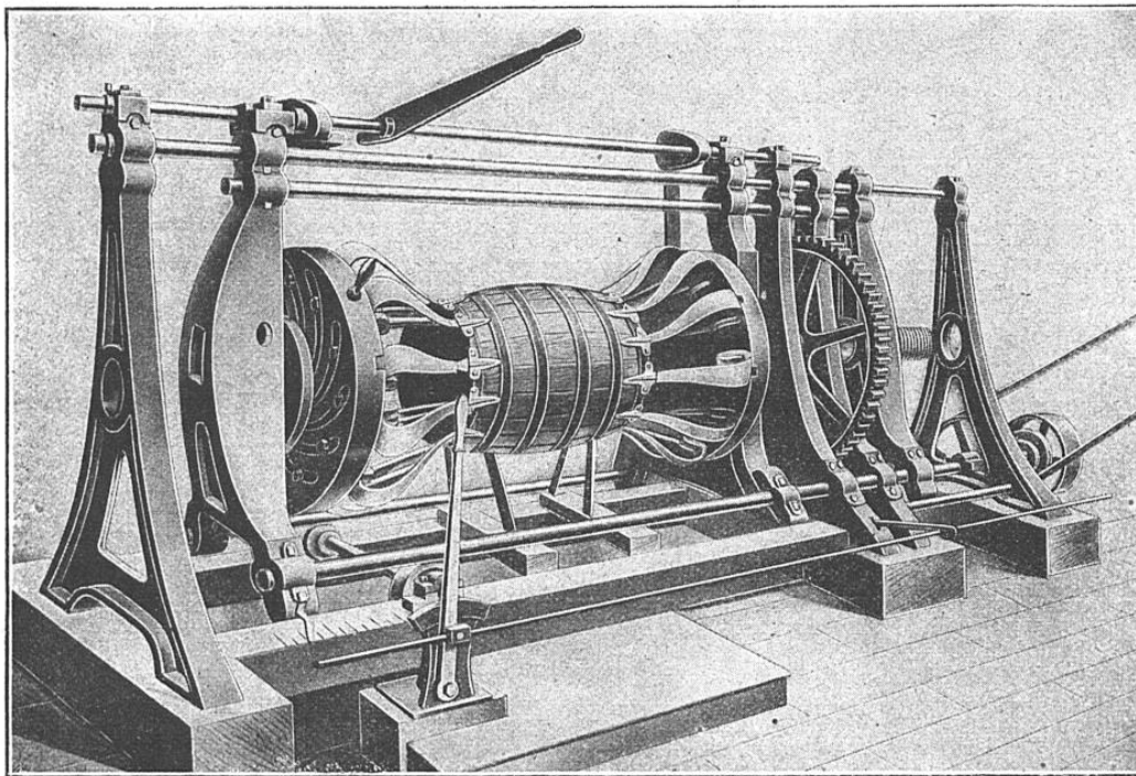
FIG. 13. — MACHINE AMÉRICAINE POUR LE CÉRCLAGE DES TONNEAUX
