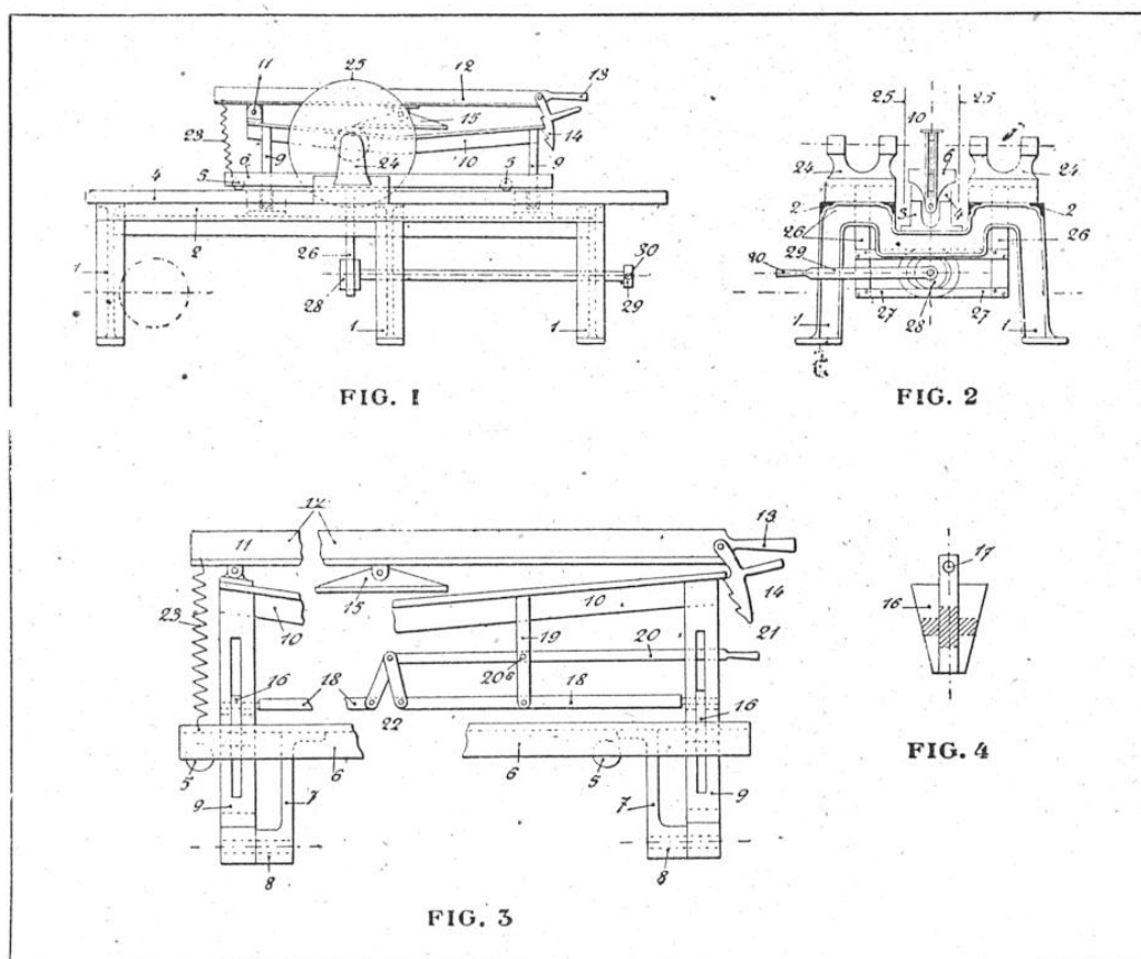
PLANCHE 11. — SCHÉMAS DE LA MACHINE A TAILLER LES DOUVES LACAZE
