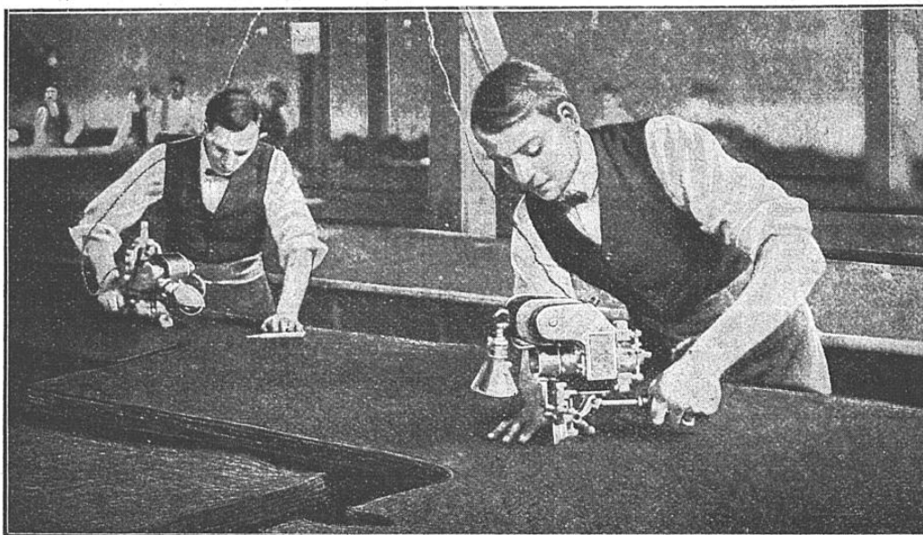
LES SCIES SONT MANIÉES COMME DE SIMPLES FERS A REPASSER ; ELLES SUIVENT LES TRACÉS LES PLUS COMPLIQUÉS ET COUPENT JUSQU'A 10 CENTIMÈTRES D'ÉPAISSEUR DE TISSU
