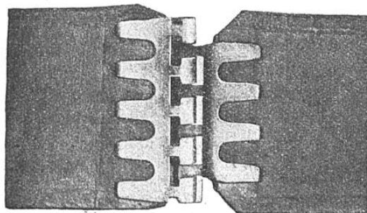
LES DEUX BOUTS DE LA COURROIE AGRAFÉS
