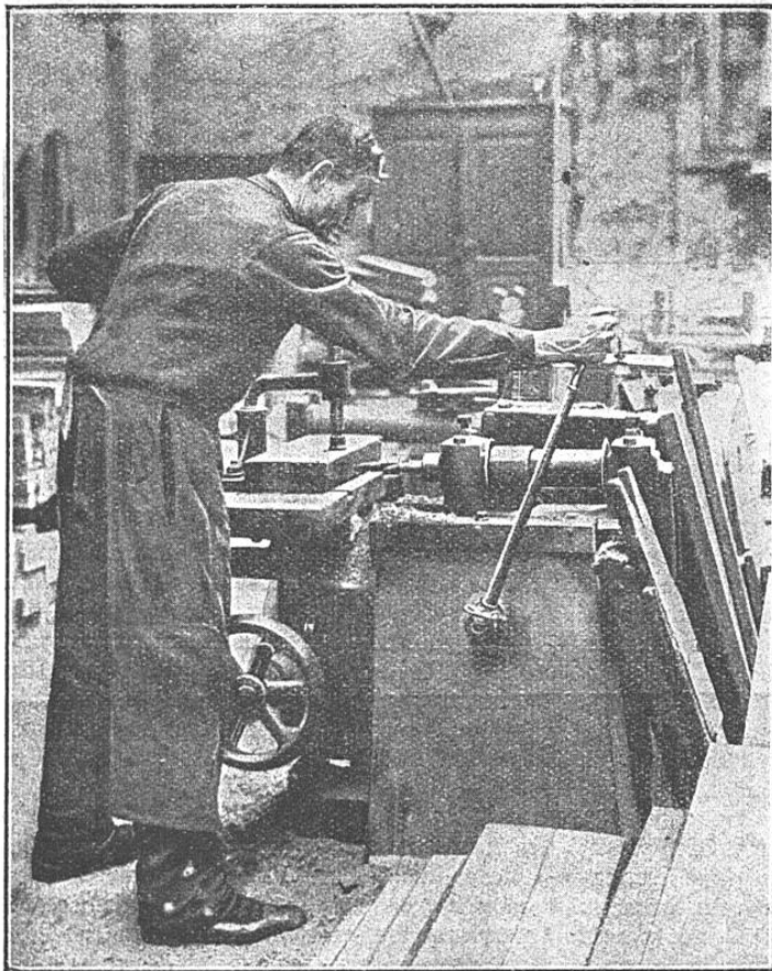
FIG. 7. — MACHINE POUR LE PERÇAGE DES FONDS
